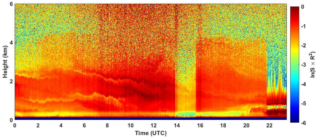
2024-09-08 RCS quick look CHM15k - ILVA LIDAR1 DIREZIONE
