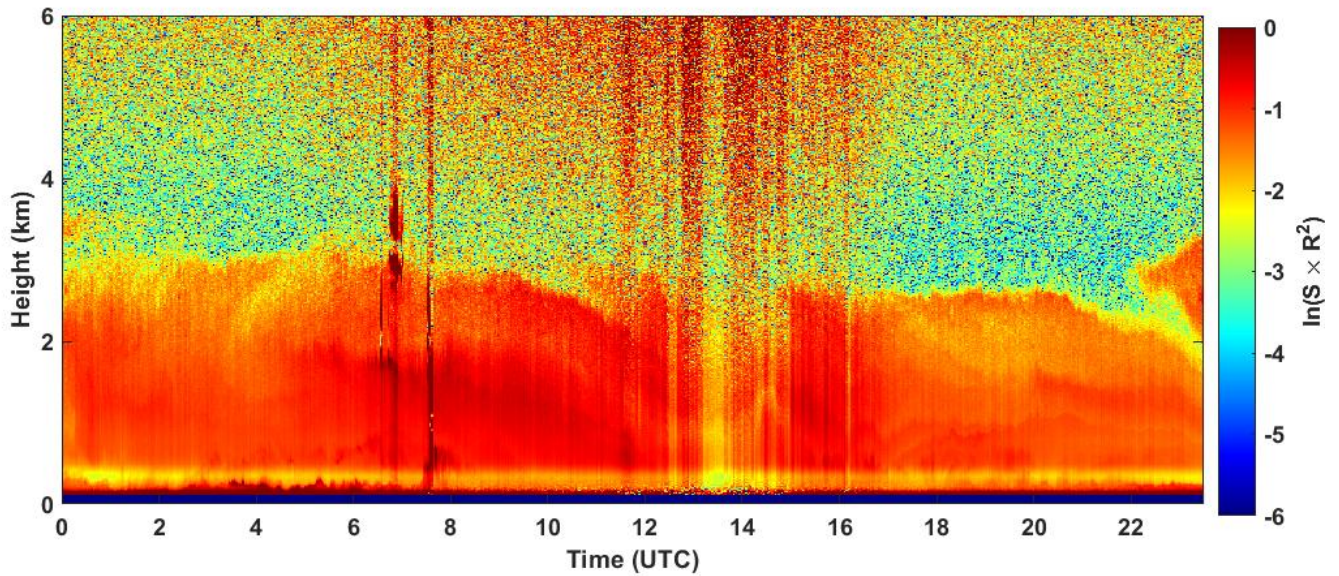
2024-09-06 RCS quick look CHM15k - ILVA LIDAR1 DIREZIONE
