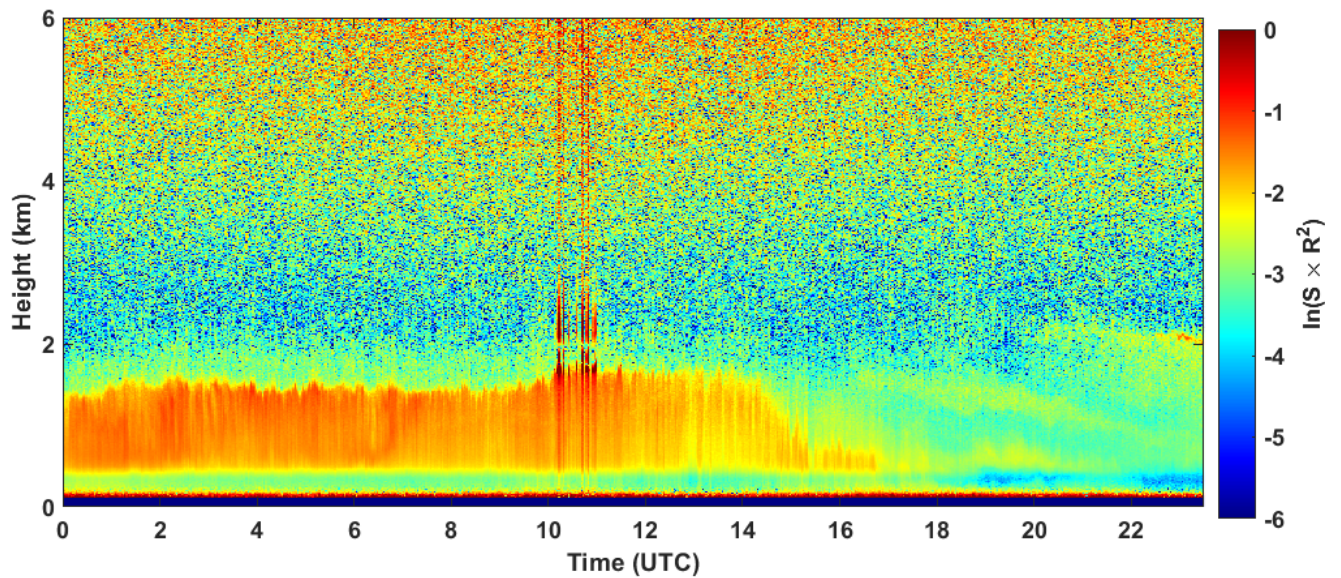
2024-09-30 RCS quick look CHM15k - ILVA LIDAR1 DIREZIONE
