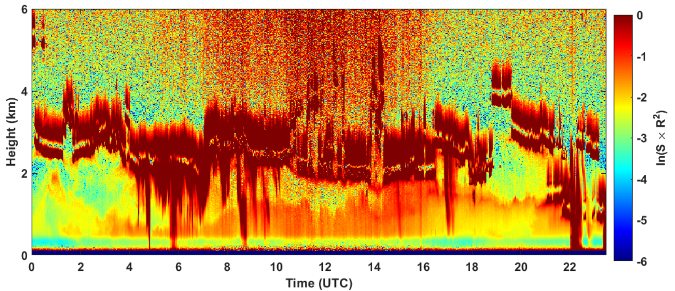
2024-09-16 RCS quick look CHM15k - ILVA LIDAR1 DIREZIONE
