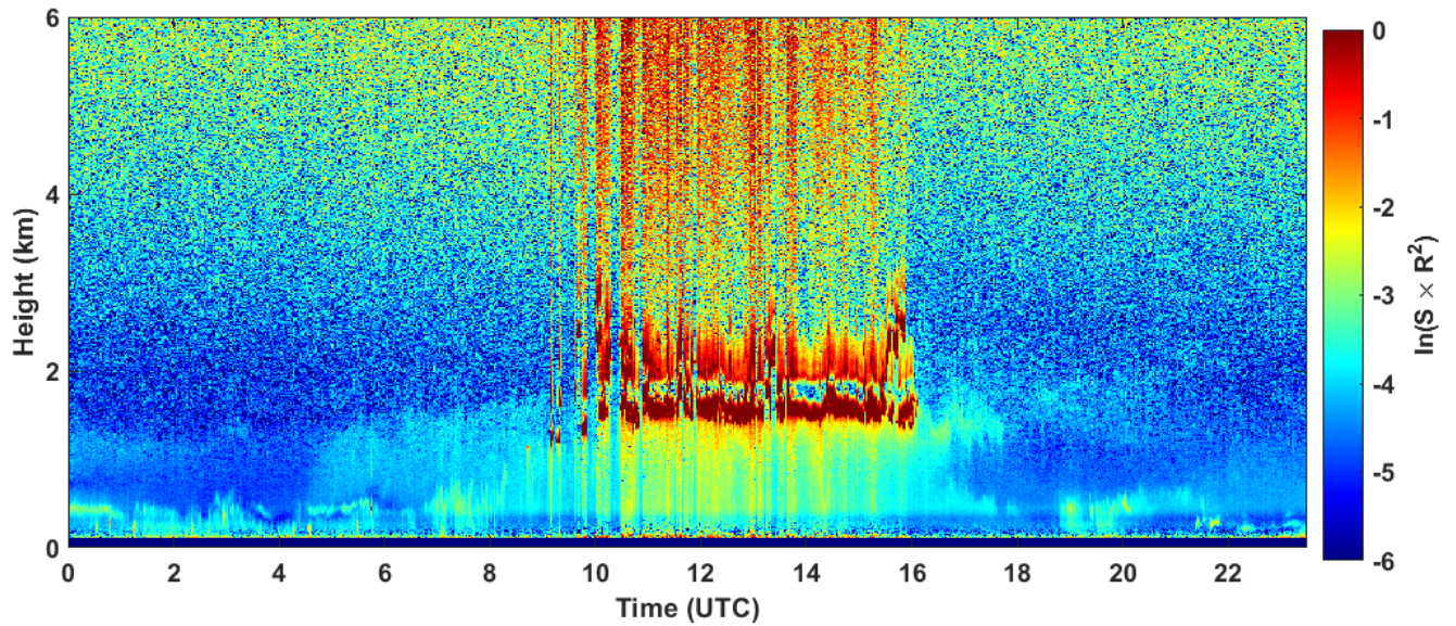
2024-09-22 RCS quick look CHM15k - ILVA LIDAR2 PARCHI
