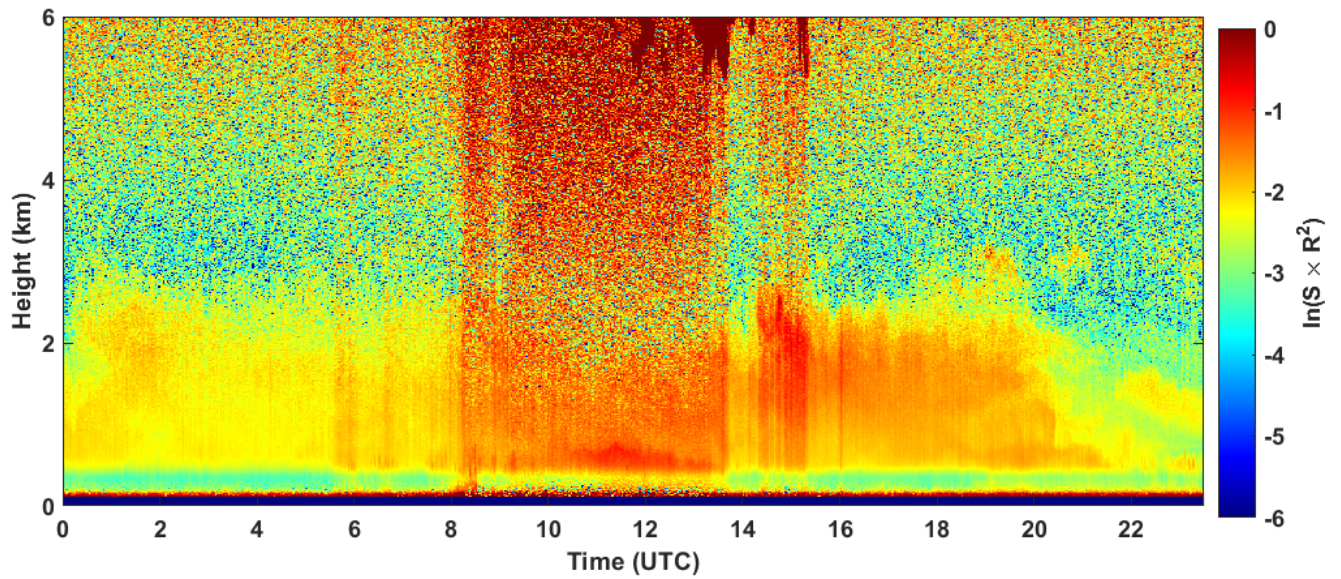
2024-09-26 RCS quick look CHM15k - ILVA LIDAR1 DIREZIONE
