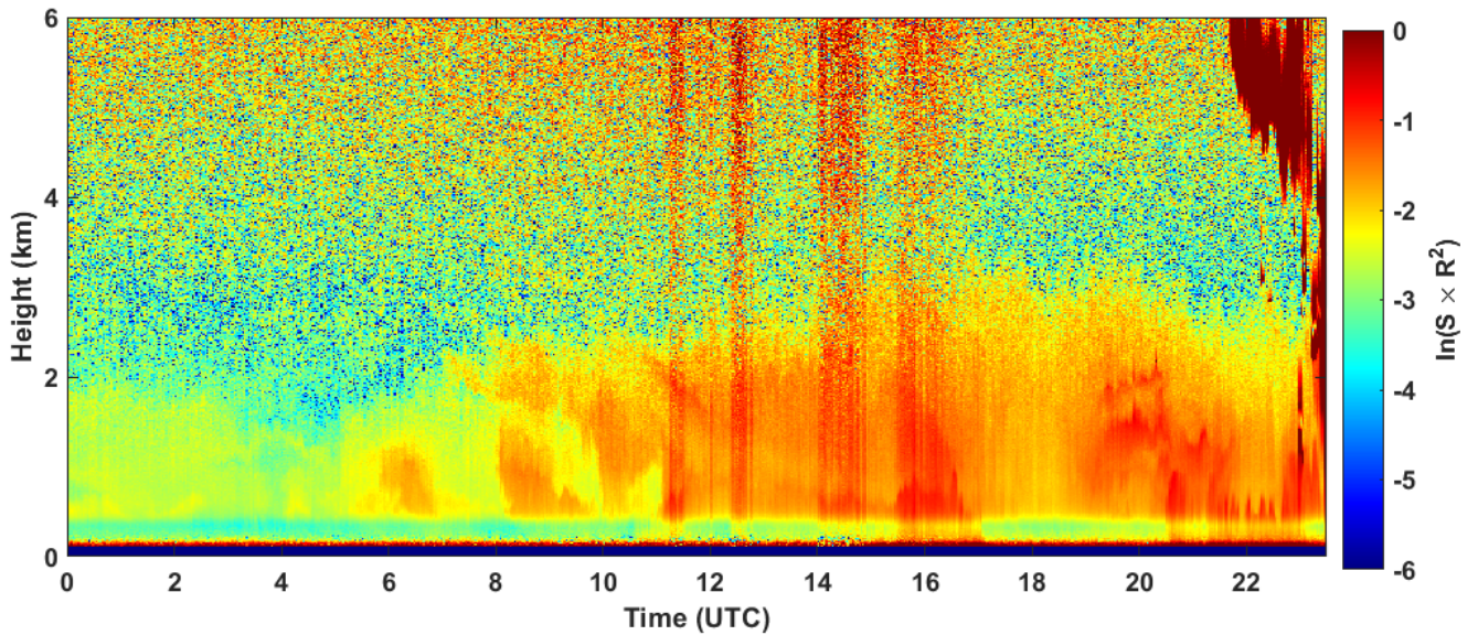
2024-09-12 RCS quick look CHM15k - ILVA LIDAR1 DIREZIONE
