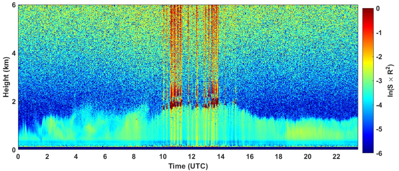
2024-09-30 RCS quick look CHM15k - ILVA LIDAR2 PARCHI
