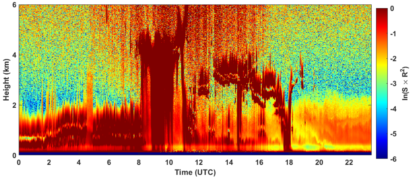
2024-09-10 RCS quick look CHM15k - ILVA LIDAR1 DIREZIONE
