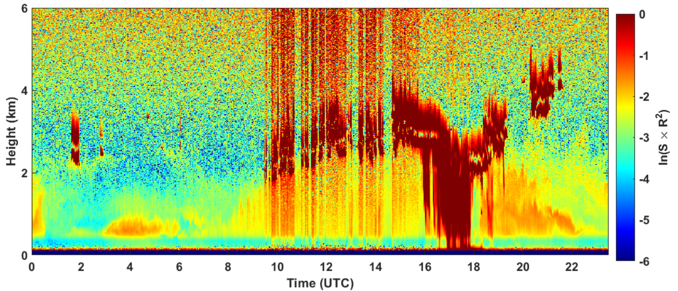
2024-09-14 RCS quick look CHM15k - ILVA LIDAR1 DIREZIONE
