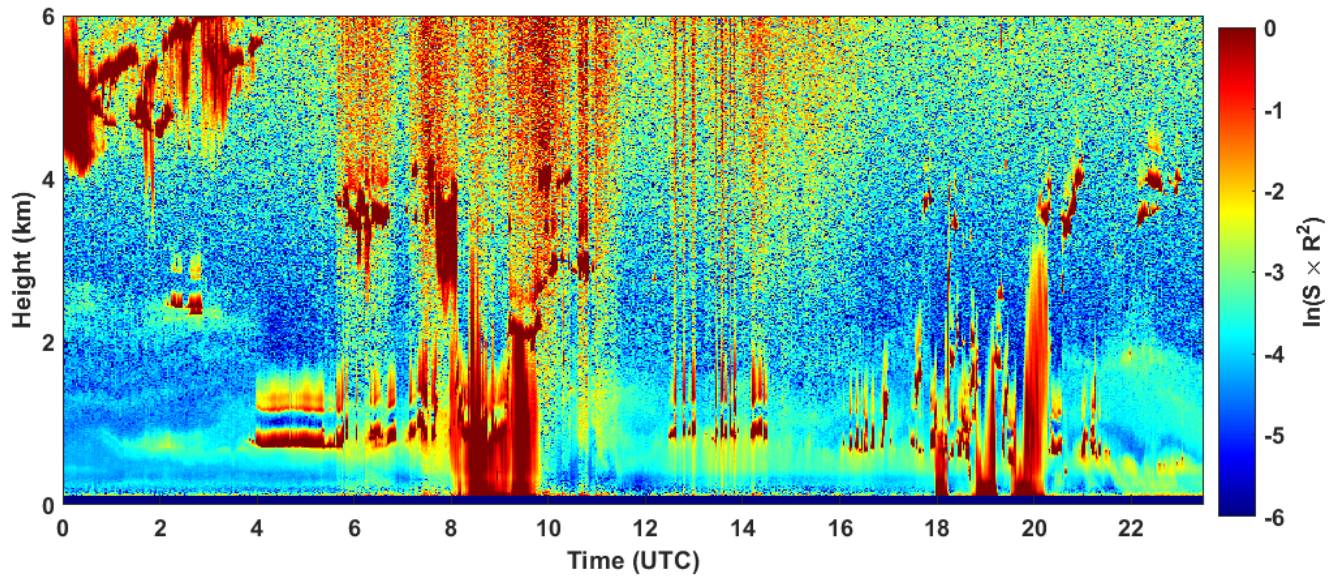
2024-09-24 RCS quick look CHM15k - ILVA LIDAR2 PARCHI
