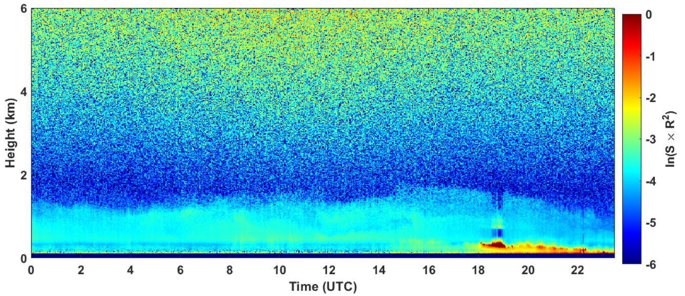
2024-09-28 RCS quick look CHM15k - ILVA LIDAR2 PARCHI
