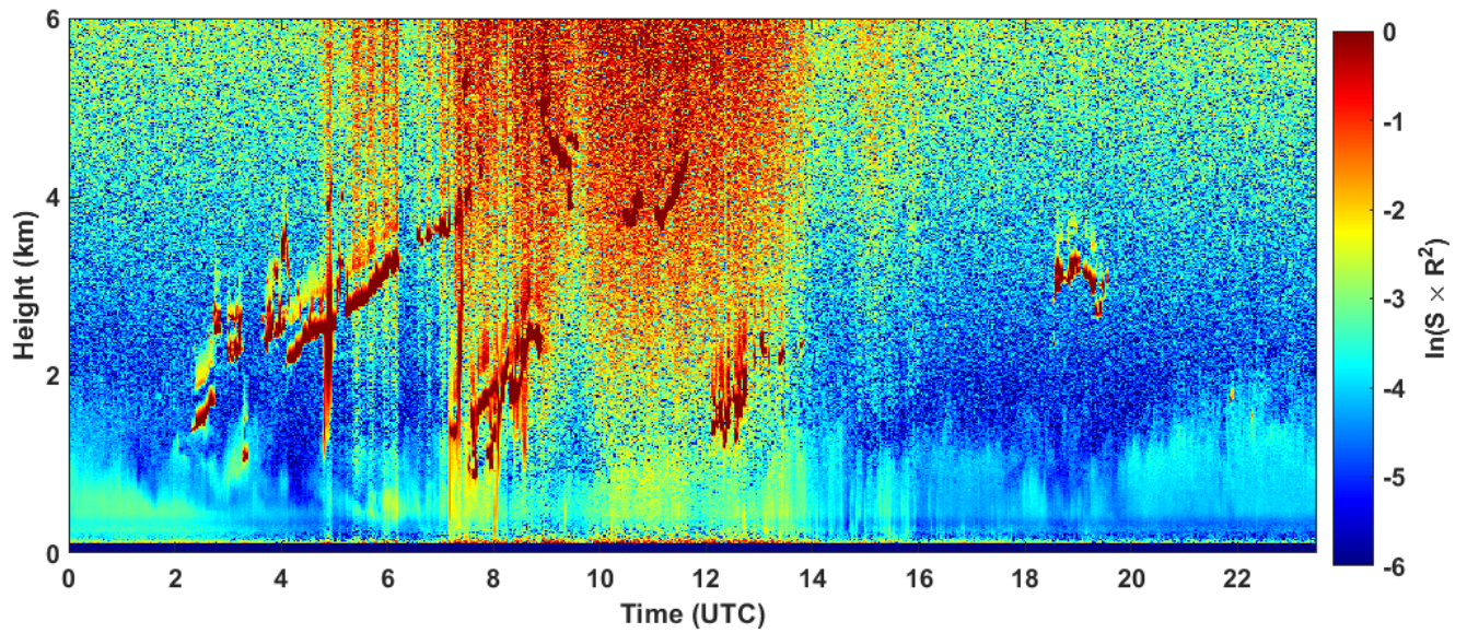
2024-09-10 RCS quick look CHM15k - ILVA LIDAR2 PARCHI
