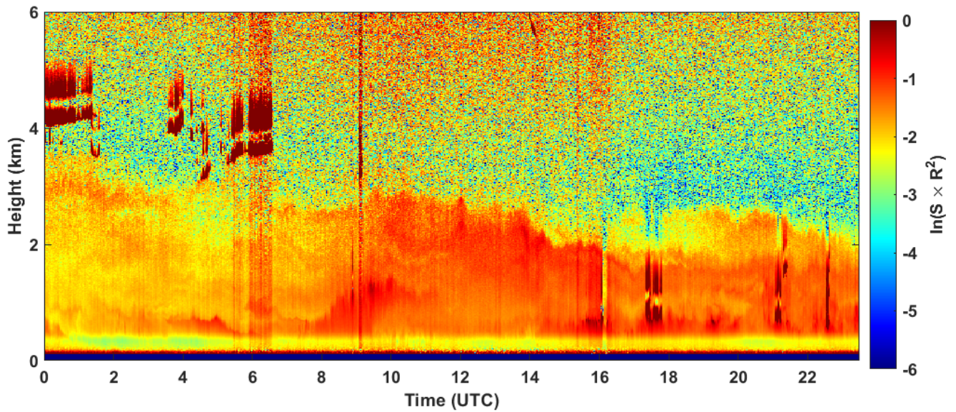
2024-09-04 RCS quick look CHM15k - ILVA LIDAR1 DIREZIONE
