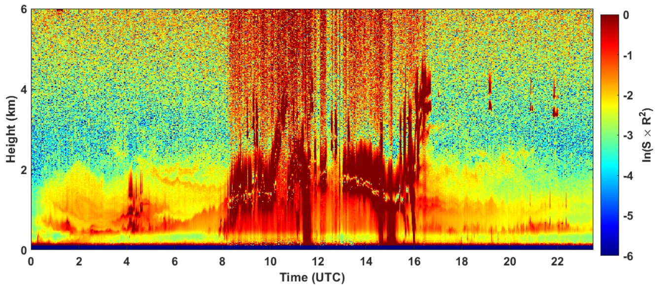
2024-09-20 RCS quick look CHM15k - ILVA LIDAR1 DIREZIONE
