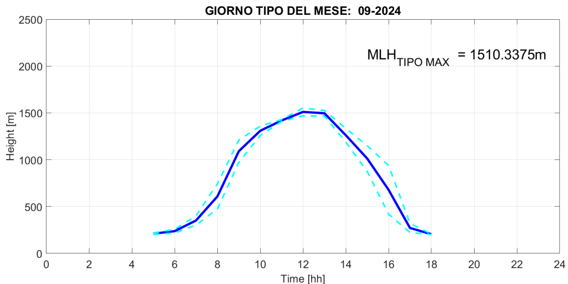
Fig. 2: Giorno tipo del parametro Mixing Layer Height nel mese di SETTEMBRE 2024, rappresentato mediante media oraria (linea blu continua) e deviazione standard (linee celesti tratteggiate).
