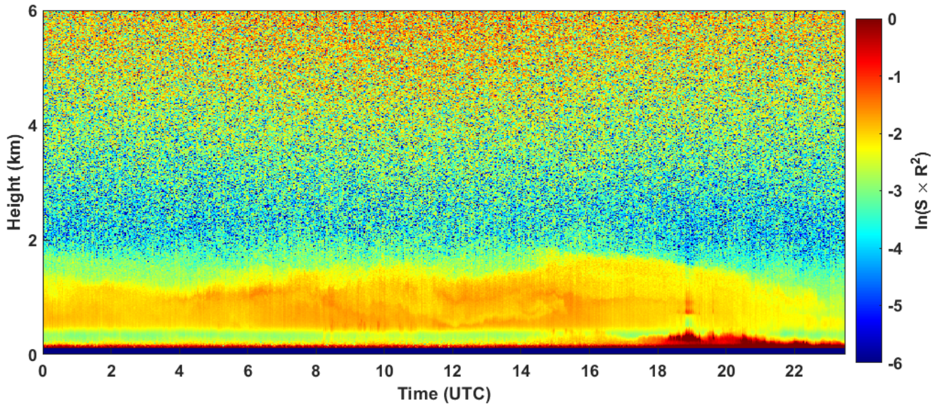
2024-09-28 RCS quick look CHM15k - ILVA LIDAR1 DIREZIONE
