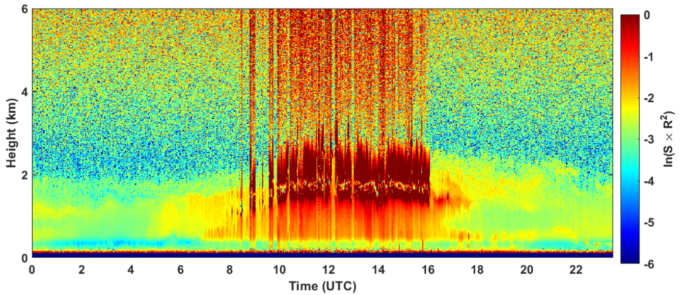
2024-09-22 RCS quick look CHM15k - ILVA LIDAR1 DIREZIONE
