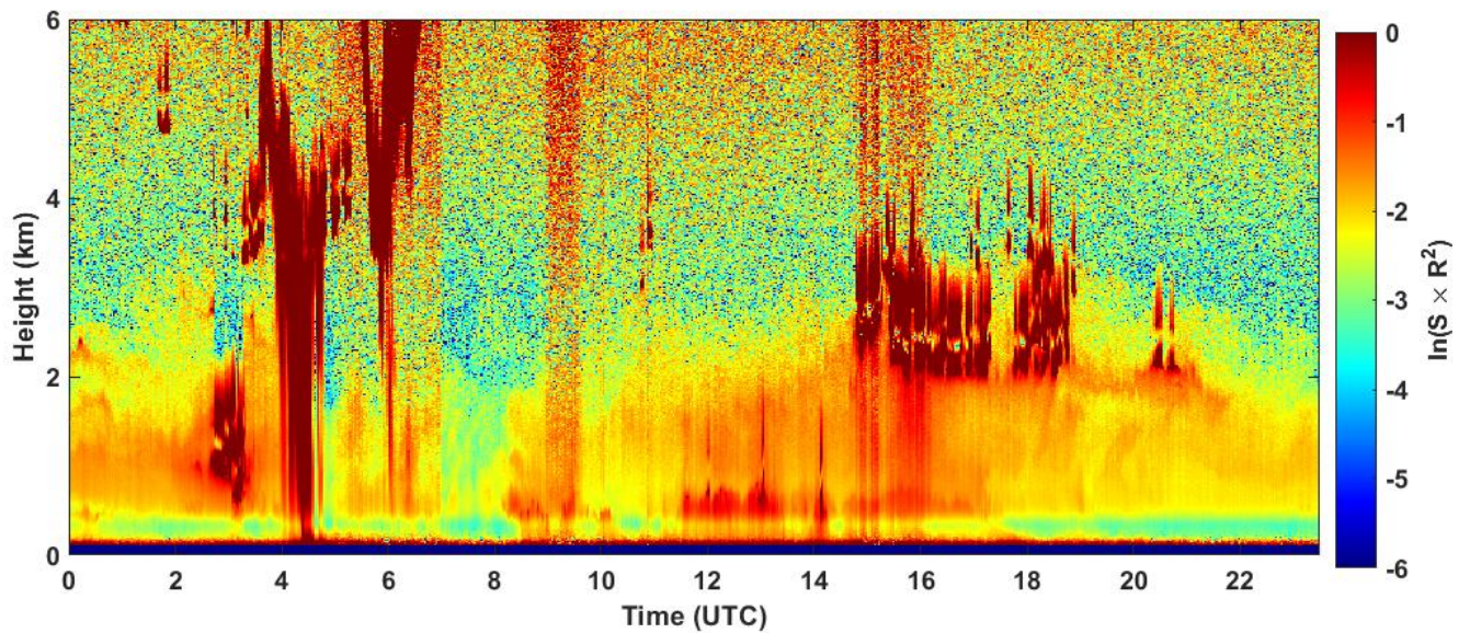
2024-09-24 RCS quick look CHM15k - ILVA LIDAR1 DIREZIONE
