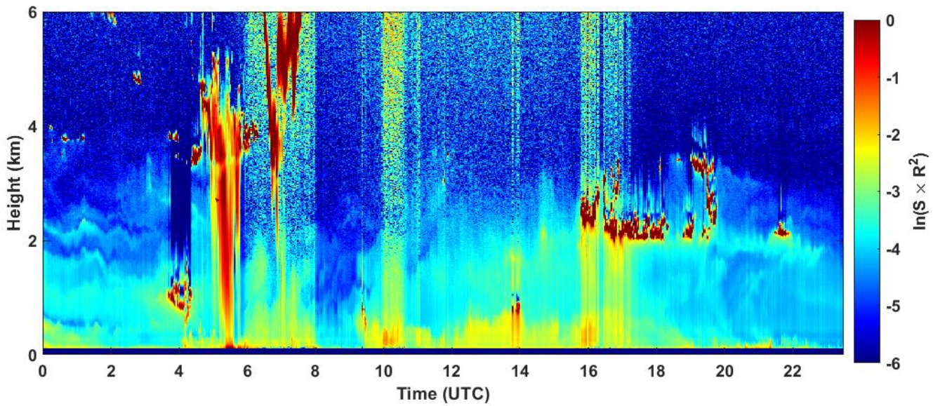
2024-09-24 RCS quick look CHM15k - ILVA LIDAR3 AGGLOMERATO
