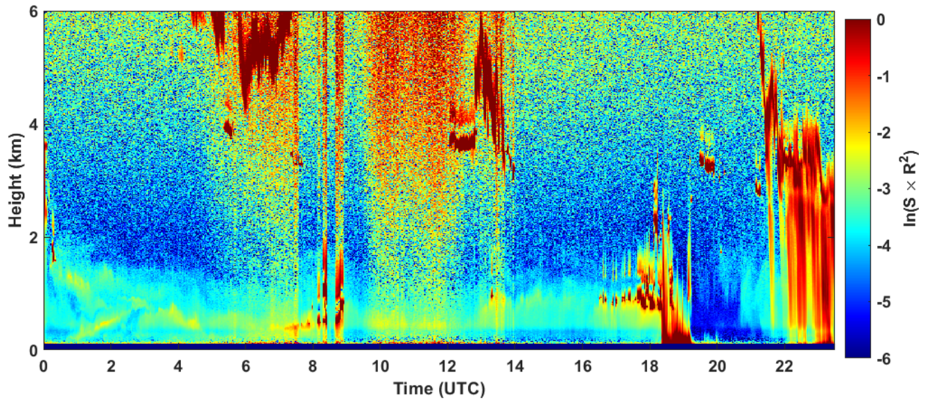
2024-09-20 RCS quick look CHM15k - ILVA LIDAR2 PARCHI
