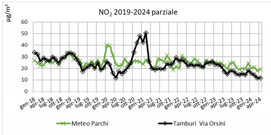
Figura 45 - Livelli medi mensili di concentrazione di NO 2 2019 ÷ 2024 (aprile) in µg/m 3
