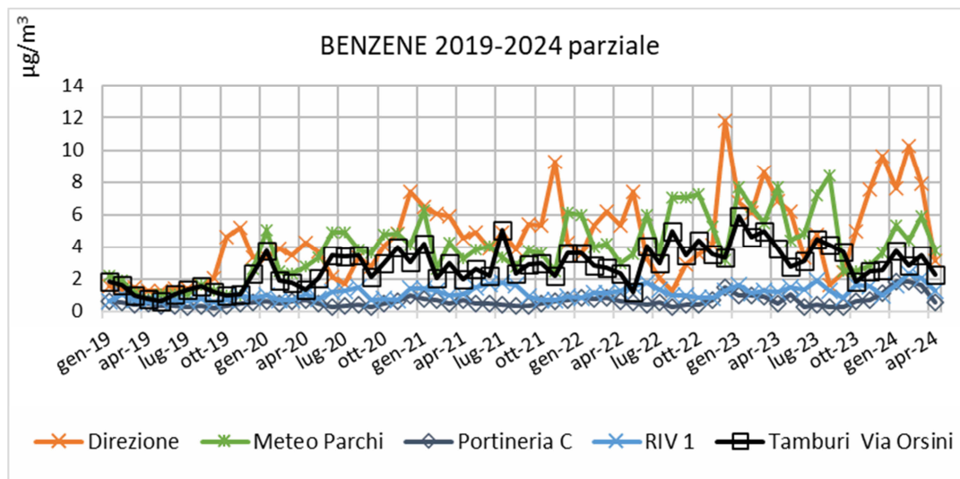
Figura 29 - Livelli medi mensili di concentrazione di Benzene 2019÷ aprile 2024 in µg/m 3 (Rete AdI senza Cokeria)
