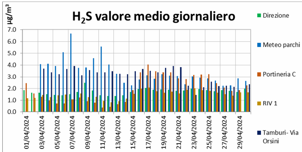
Figura 4 - Livelli medi giornalieri di concentrazione di H 2 S in µg/m 3 aprile 2024 (Rete AdI senza Cokeria)
