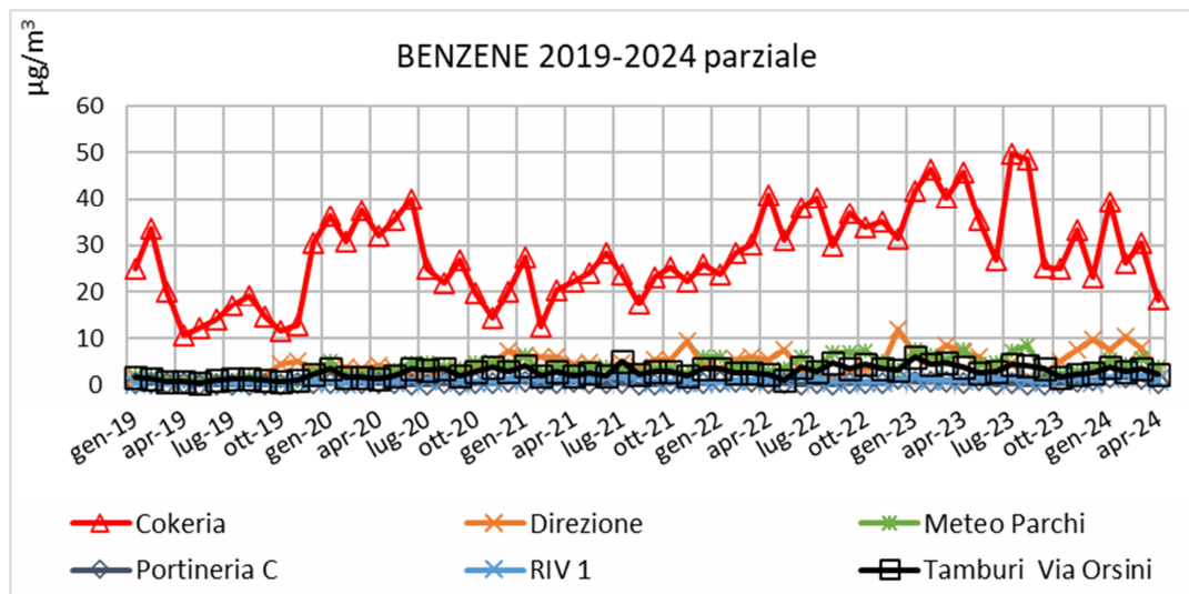
Figura 28 - Livelli medi mensili di concentrazione di Benzene 2019÷ aprile 2024 in µg/m 3 (Rete AdI con Cokeria)
