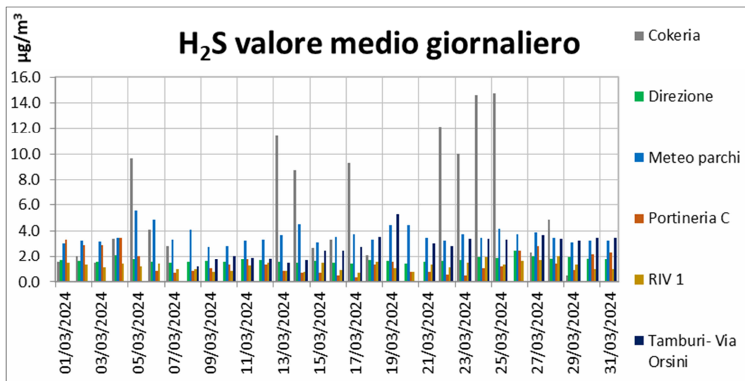
Figura 5 - Valori medi giornalieri H 2 S in µg/m 3 - marzo 2024 (Rete AdI con Cokeria)
