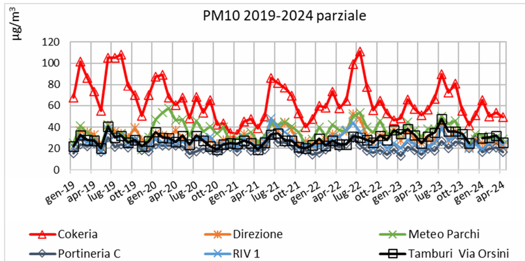
Figura 13 - Livelli medi mensili di concentrazione di PM10 2019÷ aprile 2024 in µg/m 3 (Rete AdI con Cokeria)
