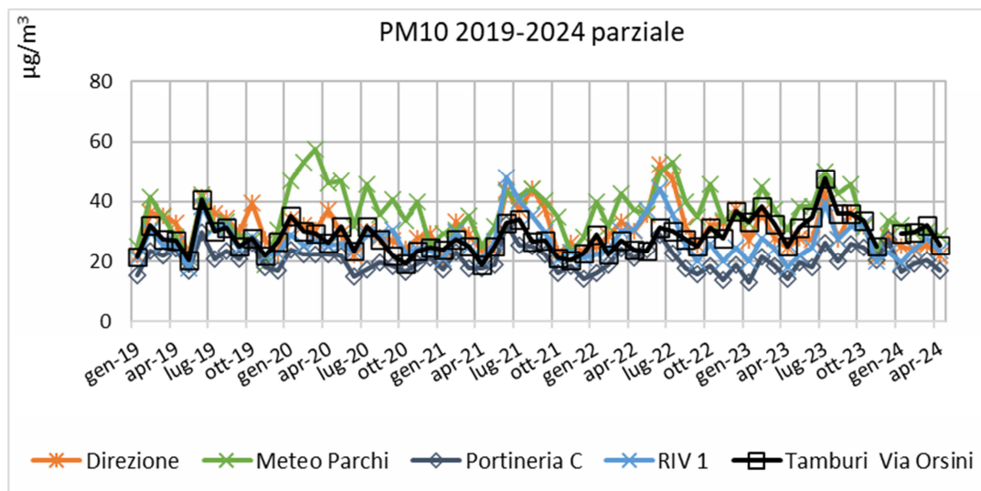
Figura 14 - Livelli medi mensili di concentrazione di PM10 2019÷aprile 2024 in µg/m 3 (Rete AdI senza Cokeria)
