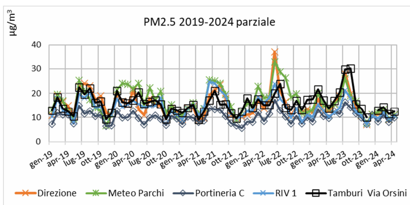
Figura 20 - Livelli medi mensili di concentrazione di PM2.5 2019÷ aprile 2024 in µg/m 3 (Rete AdI senza Cokeria)
