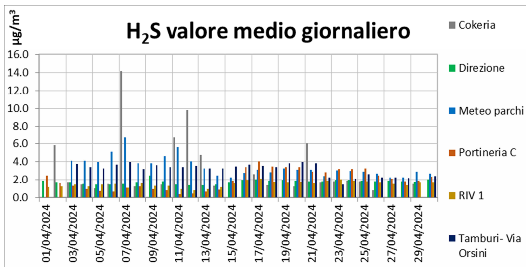
Figura 3 - Livelli medi giornalieri di concentrazione di H 2 S in \mu\text{g}/\text{m}^3 aprile 2024 (Rete AdI con Cokeria)
