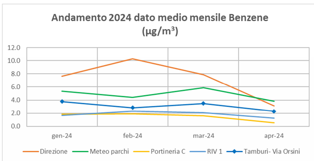
Figura 27 - Livelli di concentrazione medi mensili di Benzene in \mu\text{g}/\text{m}^3 (Rete AdI senza Cokeria)
