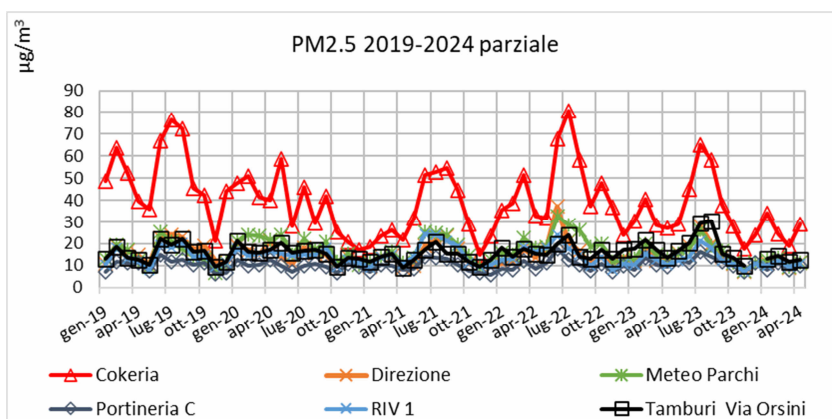
Figura 19 - Livelli medi mensili di concentrazione di PM2.5 2019÷aprile 2024 in µg/m 3 (Rete AdI con Cokeria)
