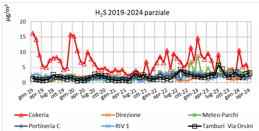
Figura 7 - Andamento dati medi mensili di H 2 S (µg/m 3 ) 2019÷aprile 2024 (Rete AdI con Cokeria)
