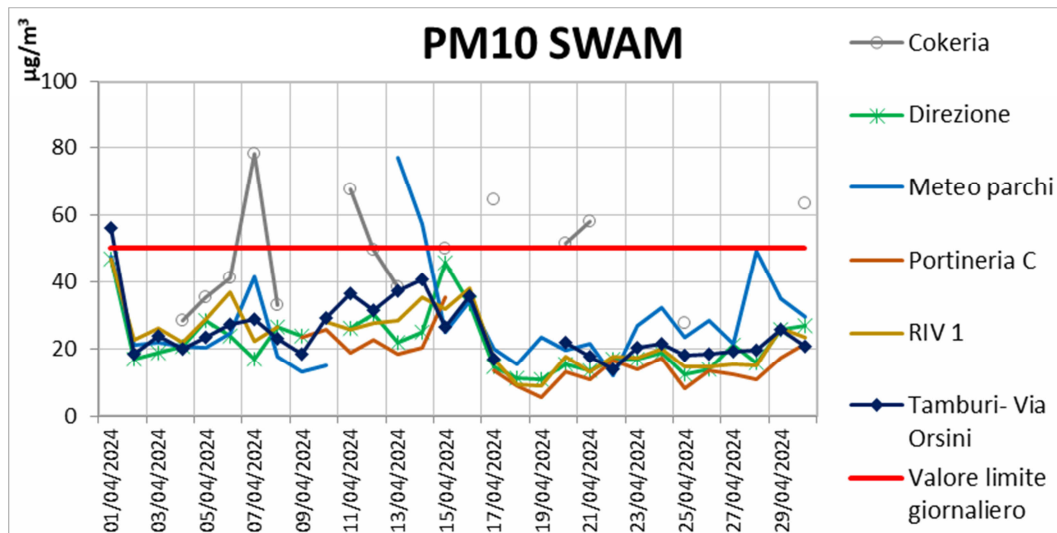
Figura 9 - Livelli di concentrazione aprile 2024 di PM10 (SWAM) in \mu\text{g}/\text{m}^3 (Rete AdI con Cokeria)
