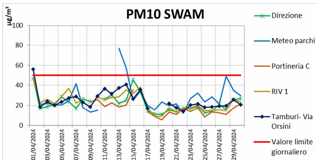
Figura 10 - Livelli di concentrazione aprile 2024 di PM10 (SWAM) in \mu\text{g}/\text{m}^3 (Rete AdI senza Cokeria)
