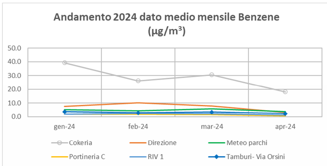
Figura 26 - Livelli di concentrazione medi mensili di Benzene in \mu\text{g}/\text{m}^3 (Rete AdI con Cokeria)
