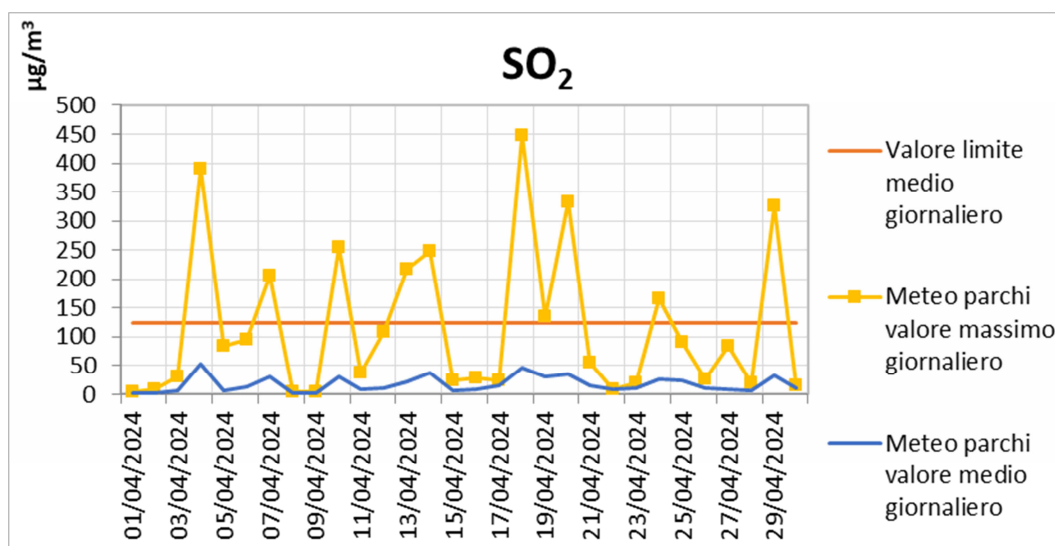
Figura 41 - Livelli di concentrazione di SO 2 in µg/m 3
