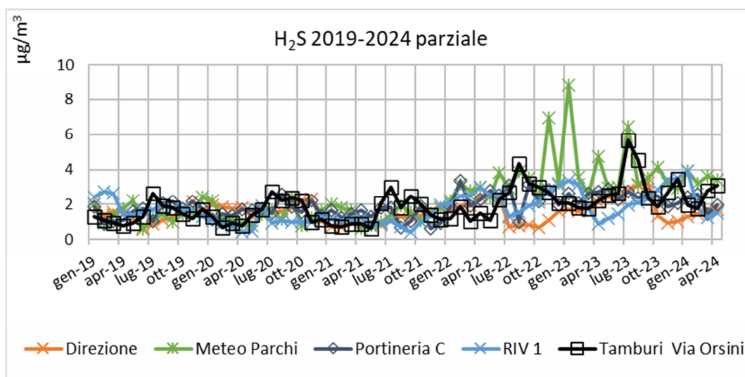
Figura 8 - Andamento dati medi mensili di H 2 S (µg/m 3 ) 2019÷ aprile 2024 (Rete AdI senza Cokeria)
