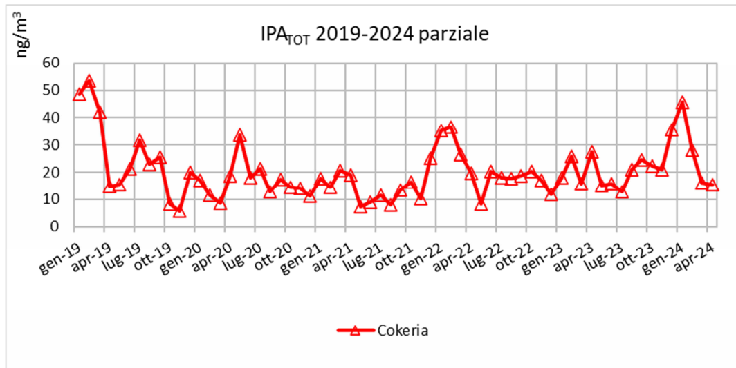
Figura 38 - Livelli medi mensili di concentrazione di IPA TOT 2019 ÷ aprile 2024 Cokeria in ng/m 3
