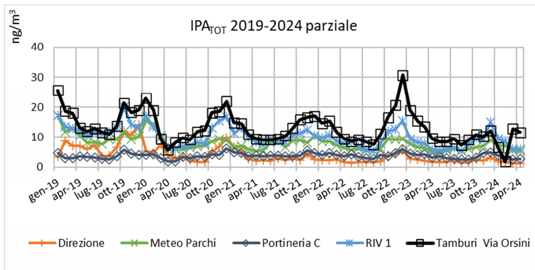
Figura 40 - Livelli medi mensili di concentrazione di IPA TOT 2019 ÷ aprile 2024 in ng/m 3 (Rete AdI senza Cokeria)
