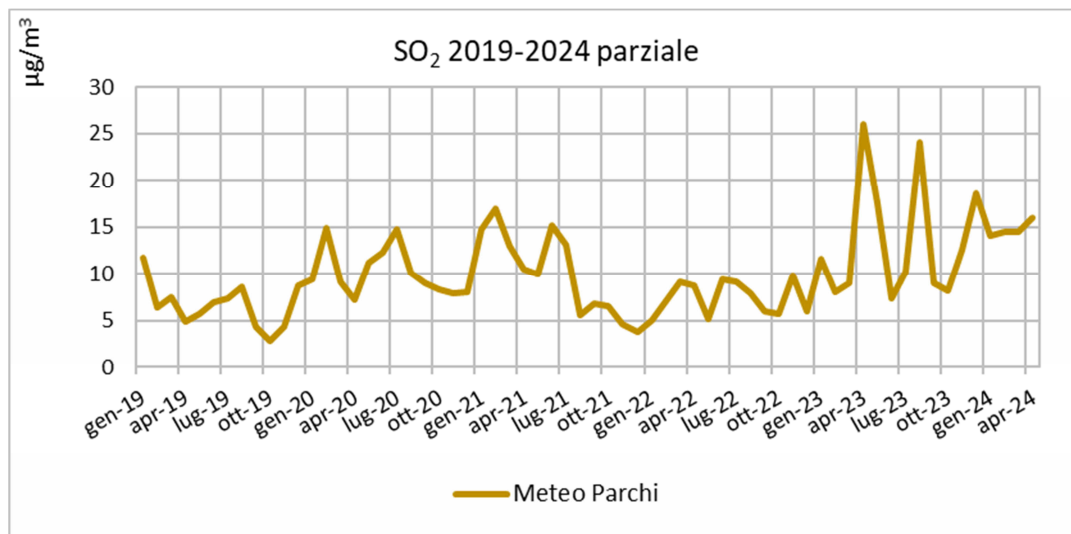
Figura 42 - Livelli medi mensili di concentrazione di SO 2 , 2019÷ 2024 (aprile) in µg/m 3
