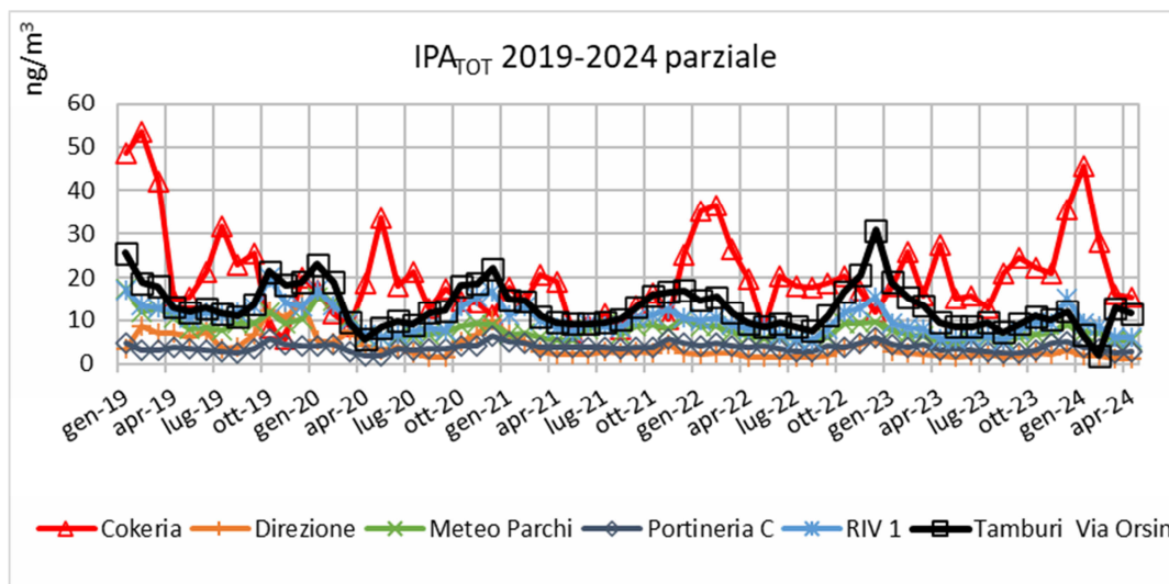
Figura 39 - Livelli medi mensili di concentrazione di IPA TOT 2019 ÷ aprile 2024 in ng/m 3 (Rete AdI con Cokeria)
