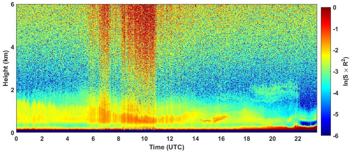
2024-03-30 RCS quick look CHM15k - ILVA LIDAR1 DIREZIONE
