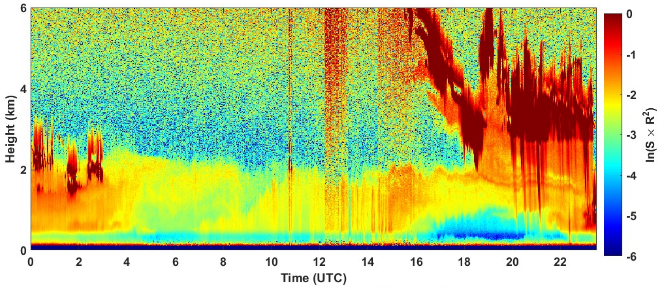
2024-03-26 RCS quick look CHM15k - ILVA LIDAR1 DIREZIONE
