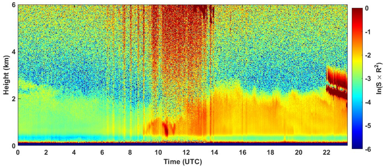
2024-03-24 RCS quick look CHM15k - ILVA LIDAR1 DIREZIONE
