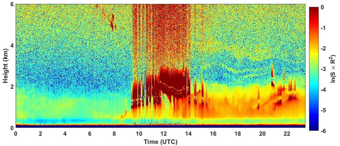
2024-03-06 RCS quick look CHM15k - ILVA LIDAR1 DIREZIONE
