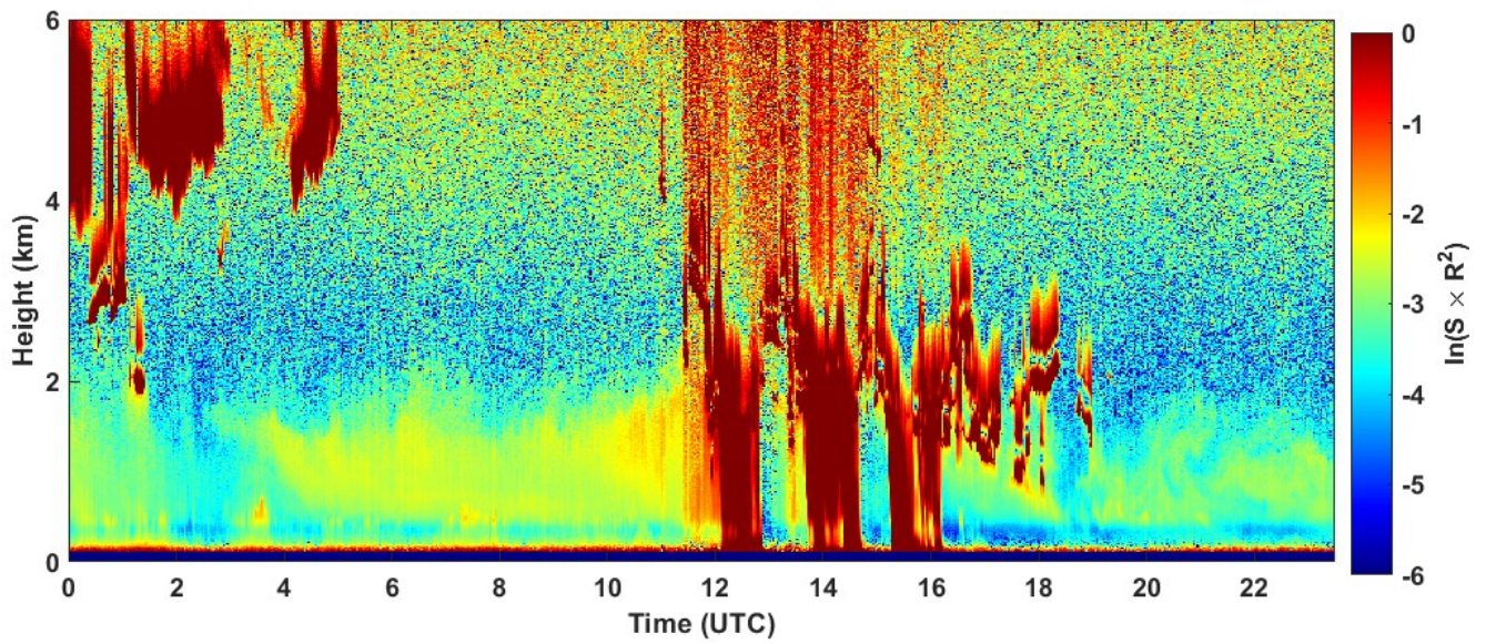
2024-03-12 RCS quick look CHM15k - ILVA LIDAR1 DIREZIONE
