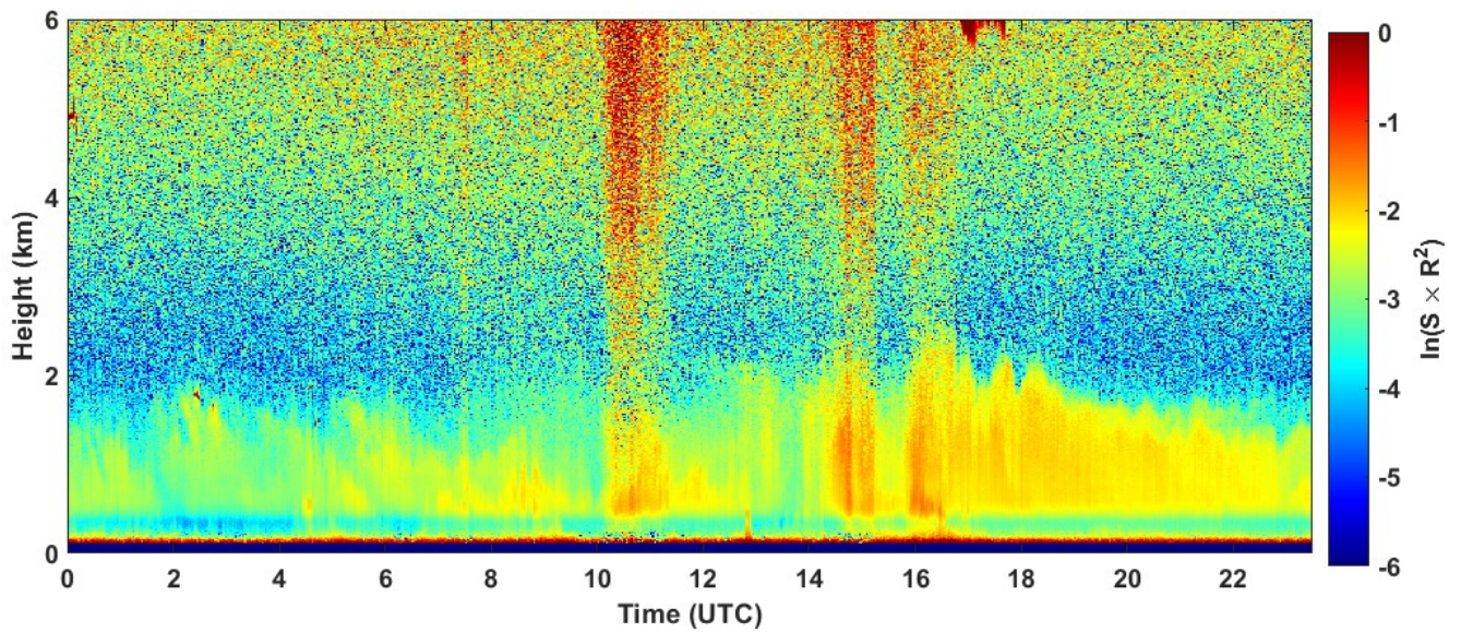
2024-03-28 RCS quick look CHM15k - ILVA LIDAR1 DIREZIONE
