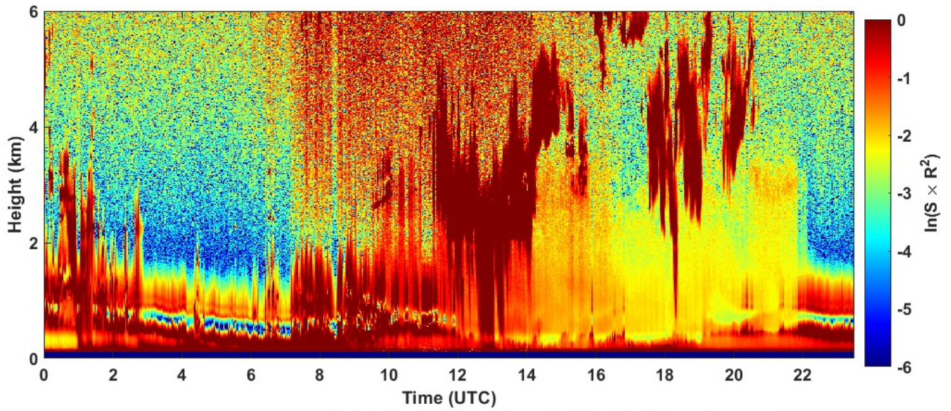
2024-03-10 RCS quick look CHM15k - ILVA LIDAR1 DIREZIONE
