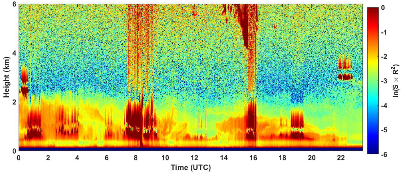
2024-03-02 RCS quick look CHM15k - ILVA LIDAR1 DIREZIONE
