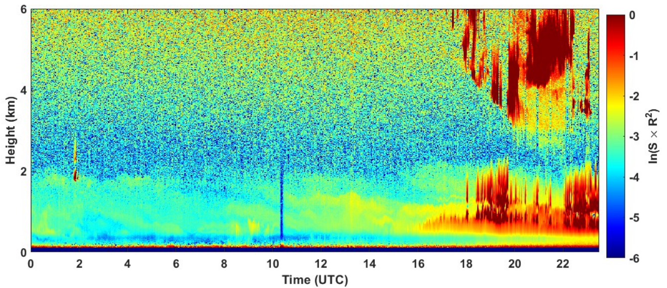
2024-03-08 RCS quick look CHM15k - ILVA LIDAR1 DIREZIONE
