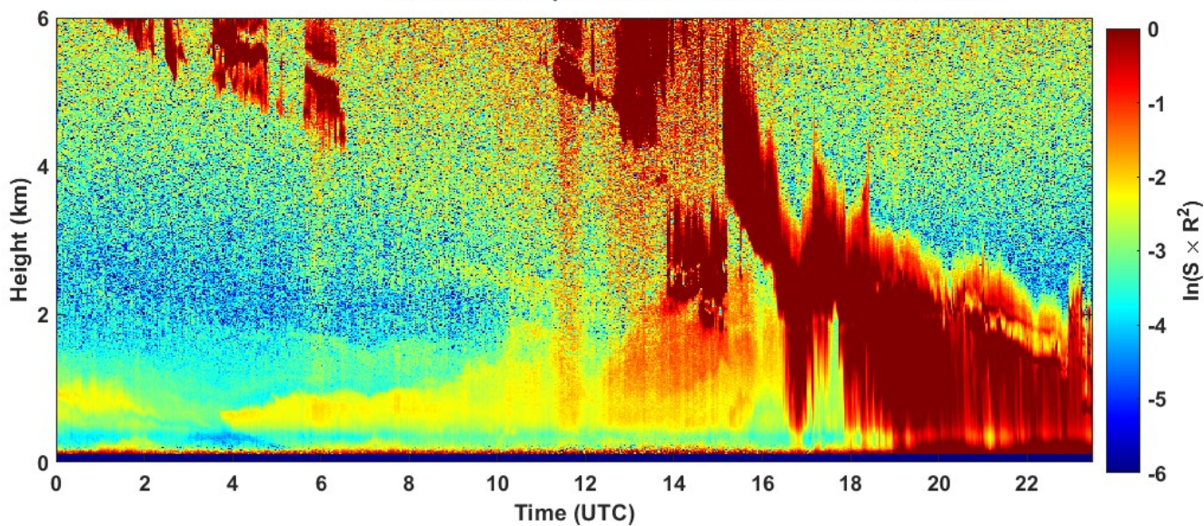
2024-03-18 RCS quick look CHM15k - ILVA LIDAR1 DIREZIONE
