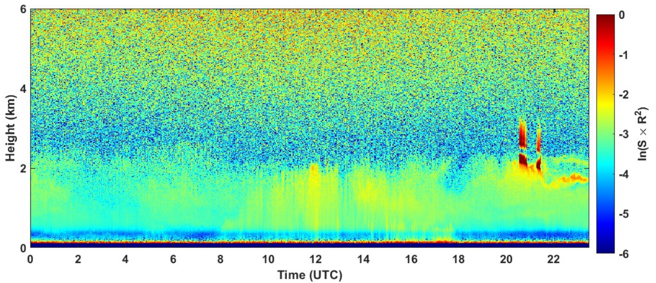
2024-03-14 RCS quick look CHM15k - ILVA LIDAR1 DIREZIONE
