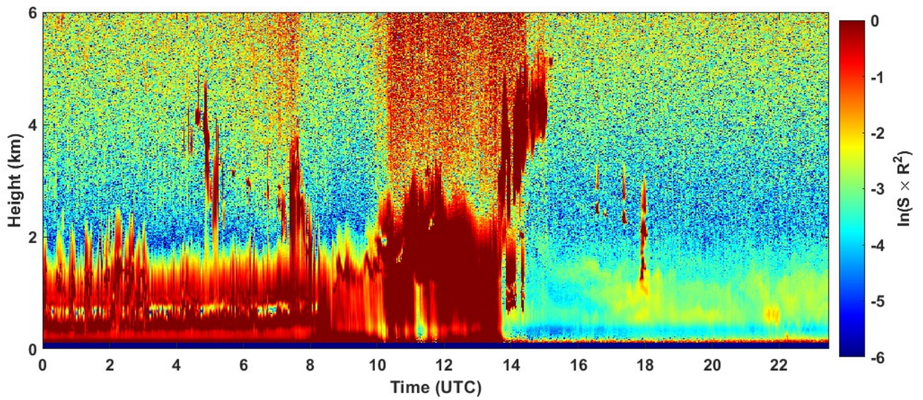
2024-03-04 RCS quick look CHM15k - ILVA LIDAR1 DIREZIONE
