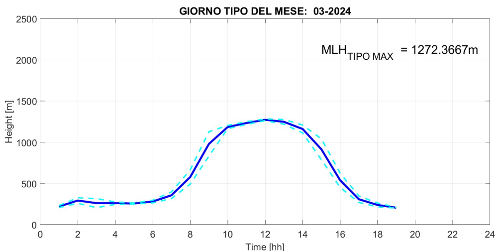
Fig. 2: Giorno tipo del parametro Mixing Layer Height nel mese di MARZO 2024, rappresentato mediante media oraria (linea blu continua) e deviazione standard (linee celesti tratteggiate).
