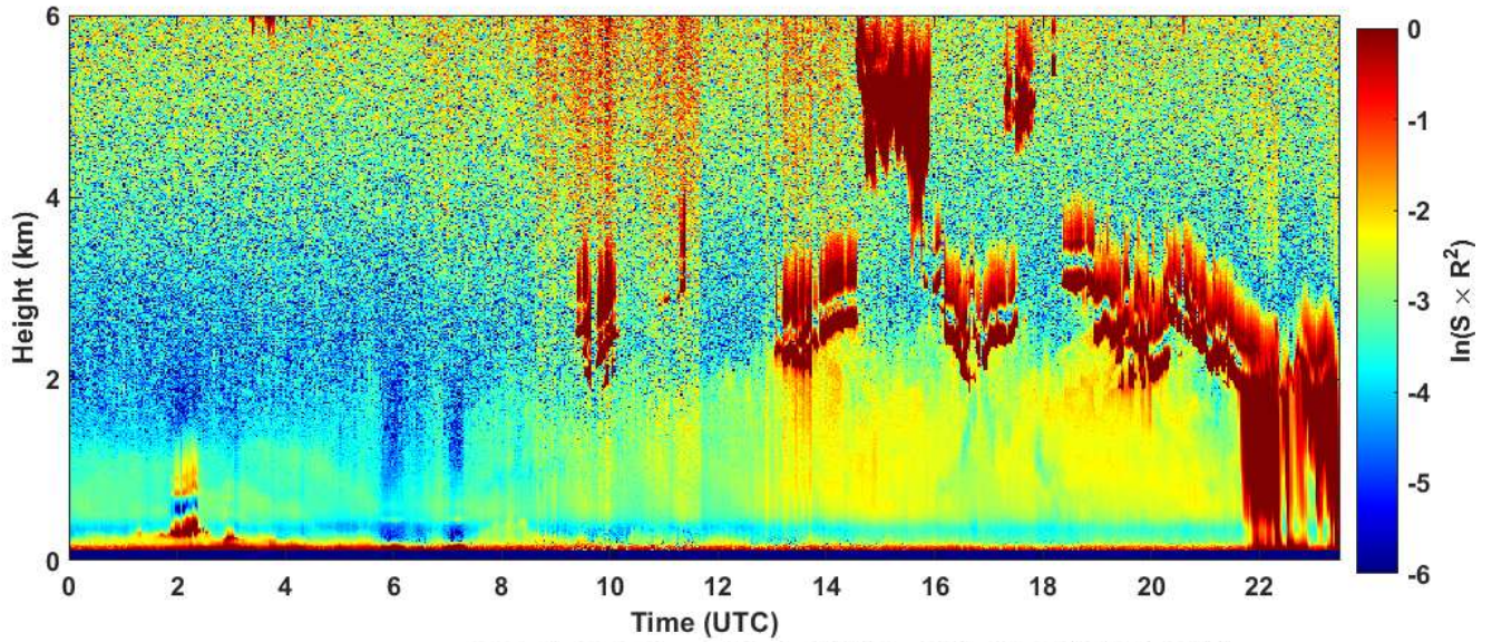
2024-01-02 RCS quick look CHM15k - ILVA LIDAR1 DIREZIONE
