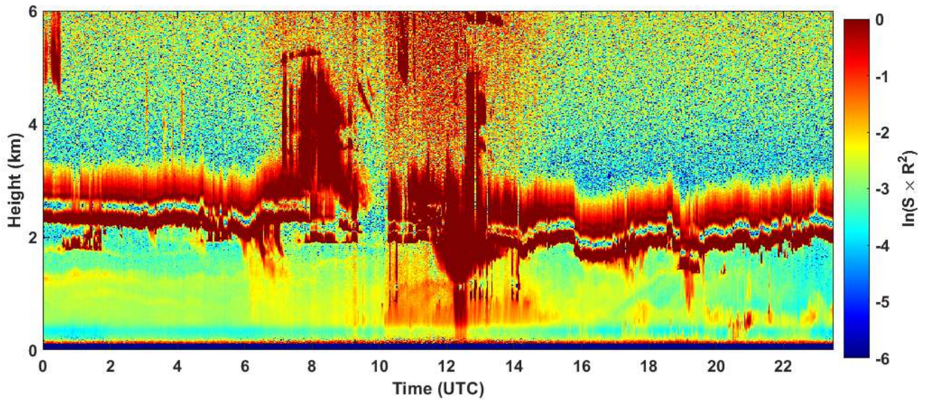
2024-01-12 RCS quick look CHM15k - ILVA LIDAR1 DIREZIONE
