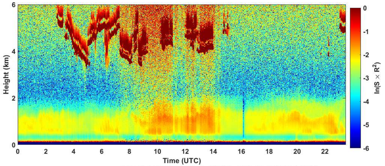
2024-01-04 RCS quick look CHM15k - ILVA LIDAR1 DIREZIONE
