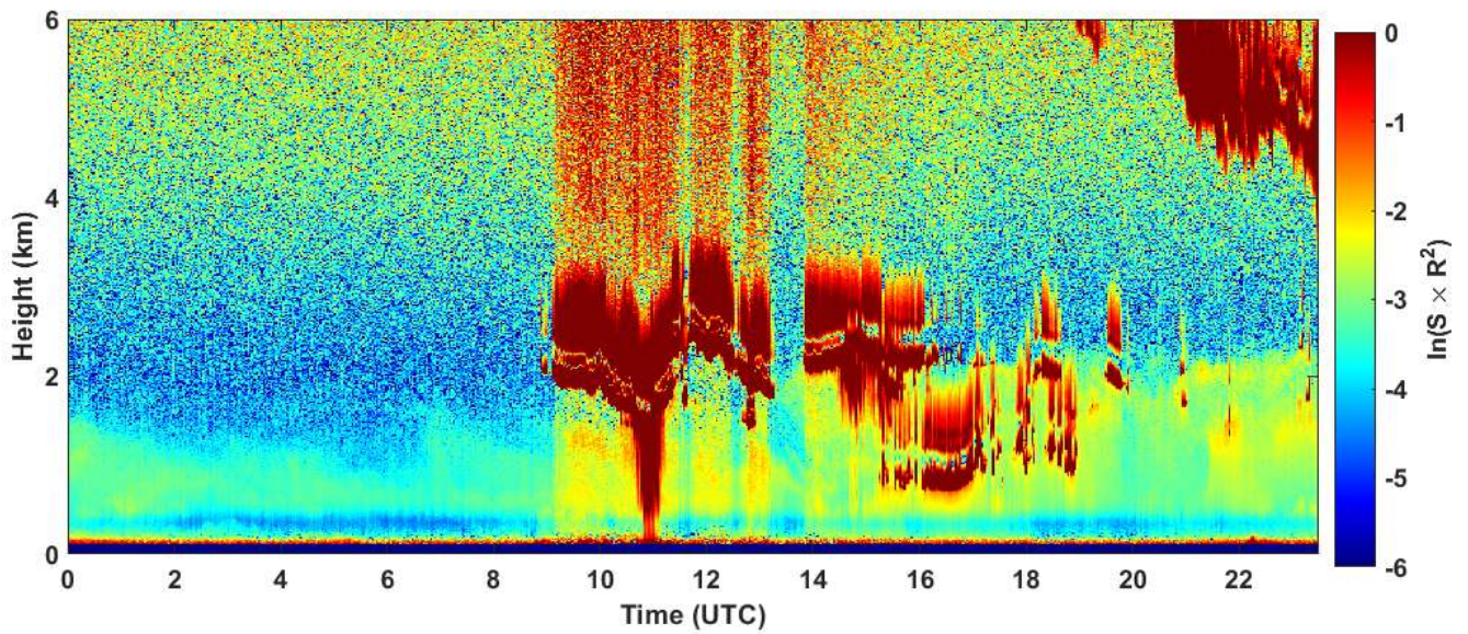
2024-01-14 RCS quick look CHM15k - ILVA LIDAR1 DIREZIONE
