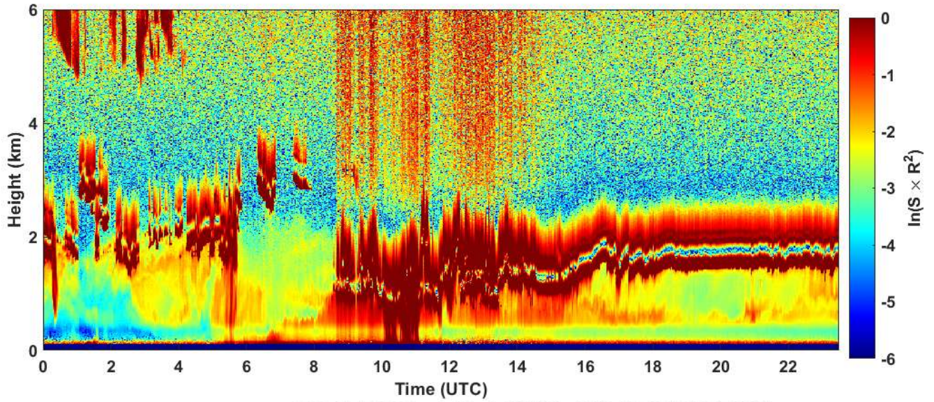
2024-01-10 RCS quick look CHM15k - ILVA LIDAR1 DIREZIONE
