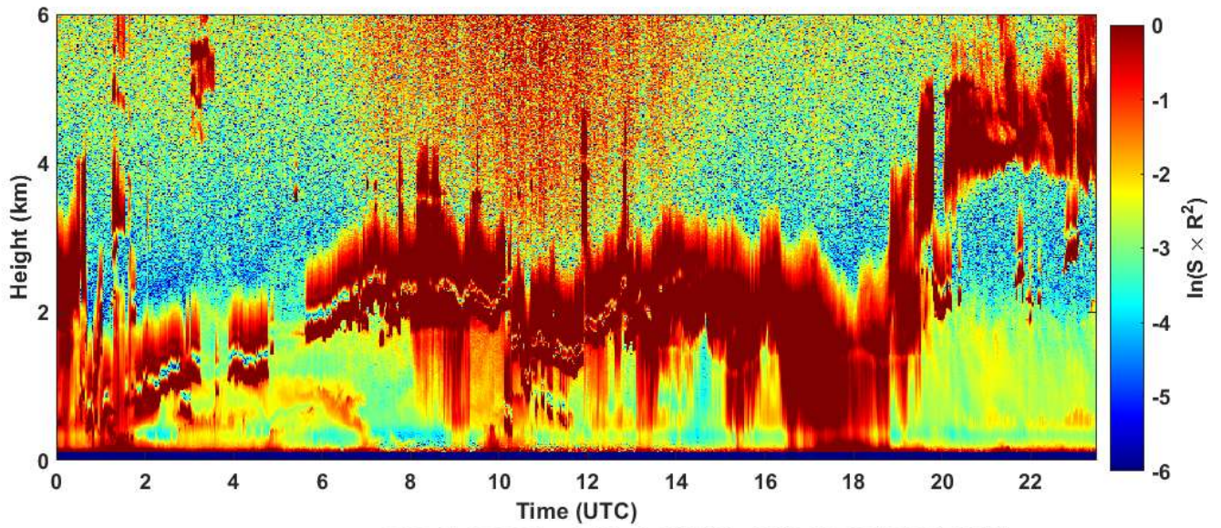
2024-01-08 RCS quick look CHM15k - ILVA LIDAR1 DIREZIONE
