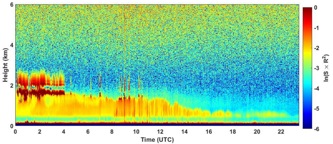
2024-01-30 RCS quick look CHM15k - ILVA LIDAR1 DIREZIONE
