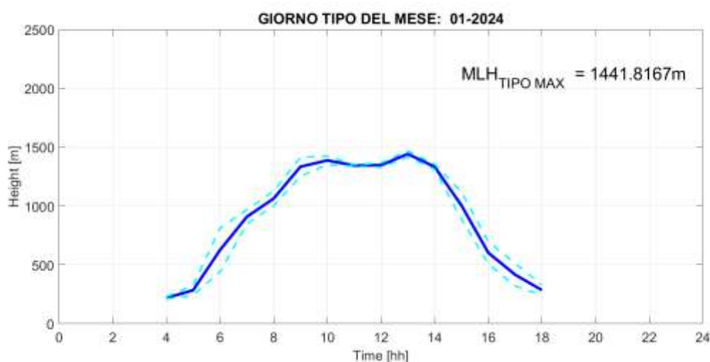
Fig. 2: Giorno tipo del parametro Mixing Layer Height nel mese di GENNAIO 2024, rappresentato mediante media oraria (linea blu continua) e deviazione standard (linee celesti tratteggiate).
