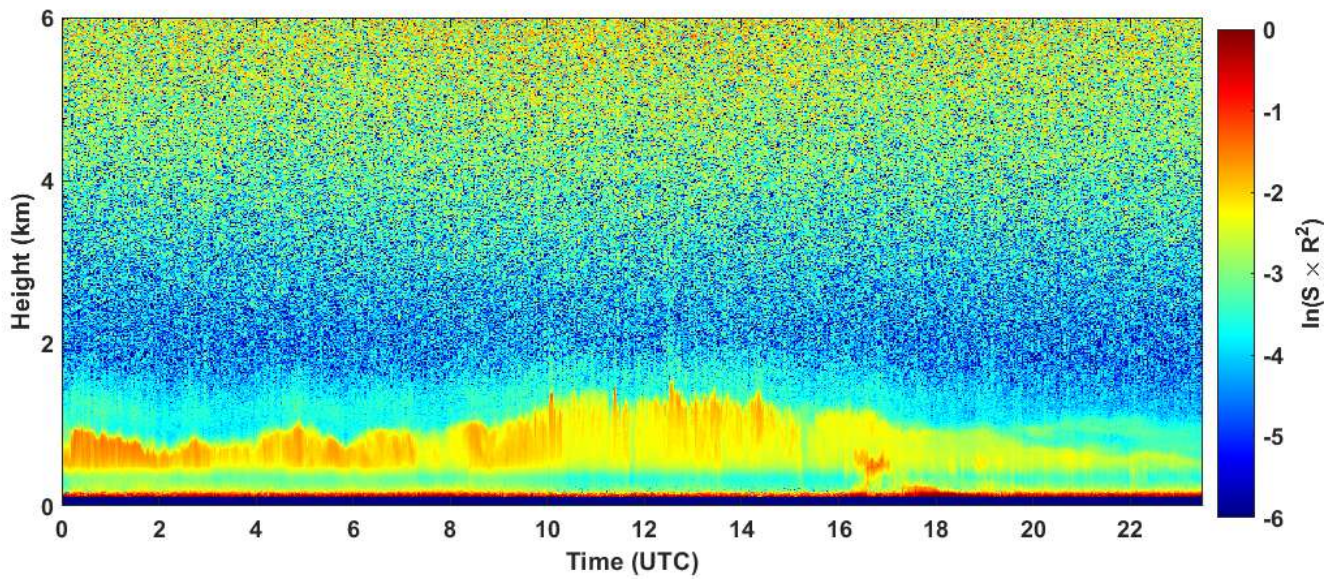
2024-01-22 RCS quick look CHM15k - ILVA LIDAR1 DIREZIONE
