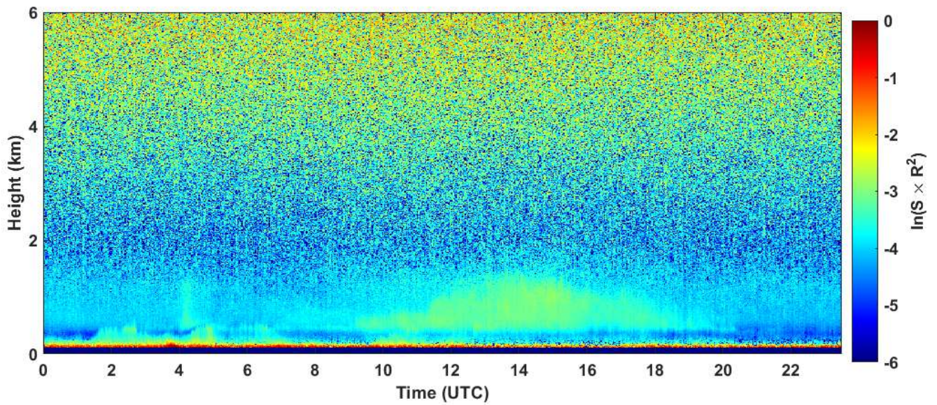
2024-01-26 RCS quick look CHM15k - ILVA LIDAR1 DIREZIONE
