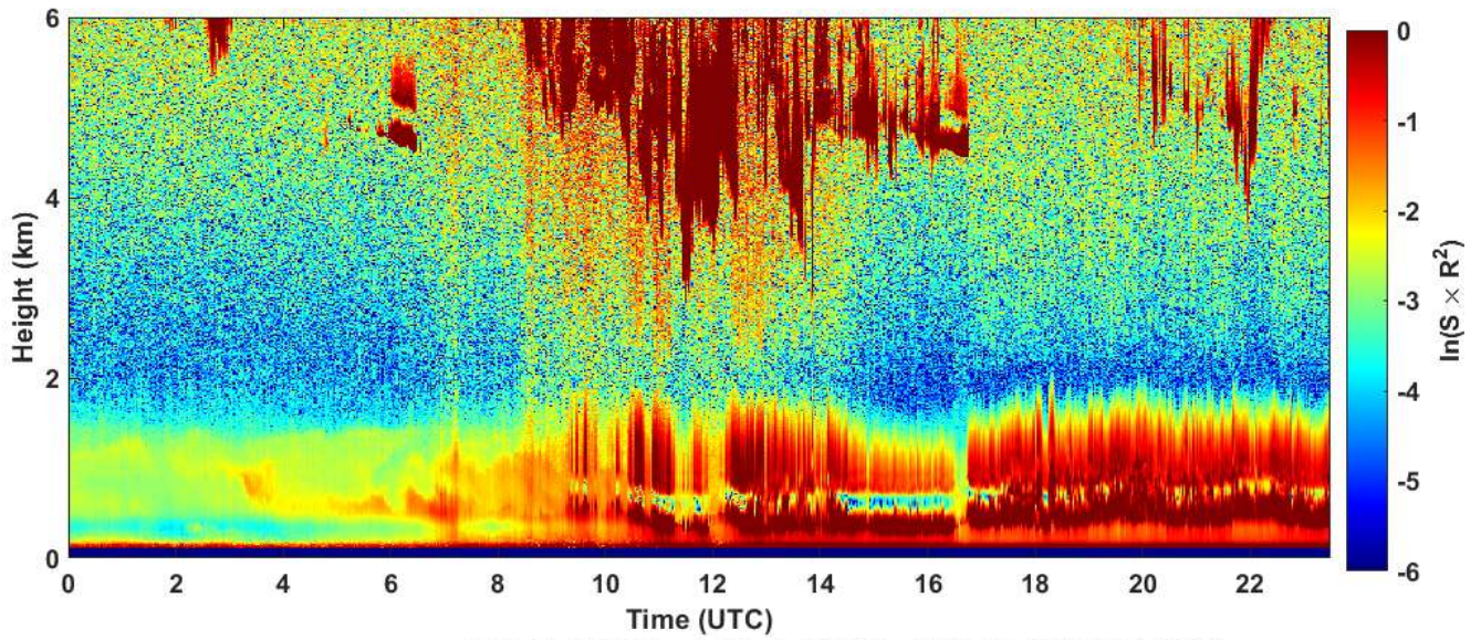
2024-01-06 RCS quick look CHM15k - ILVA LIDAR1 DIREZIONE
