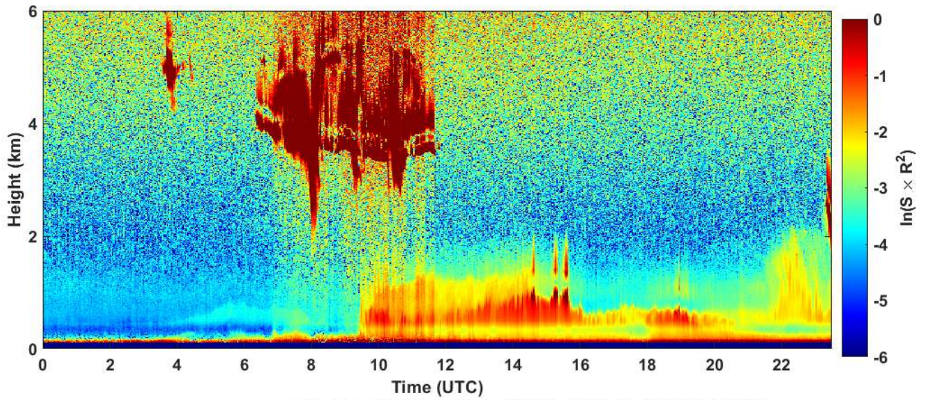
2024-01-28 RCS quick look CHM15k - ILVA LIDAR1 DIREZIONE
