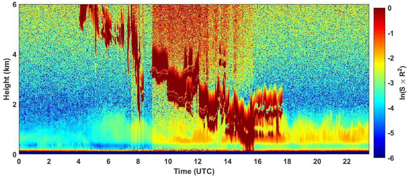
2024-01-24 RCS quick look CHM15k - ILVA LIDAR1 DIREZIONE
