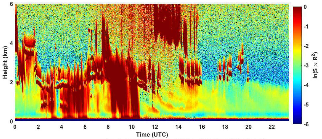
2024-01-16 RCS quick look CHM15k - ILVA LIDAR1 DIREZIONE
