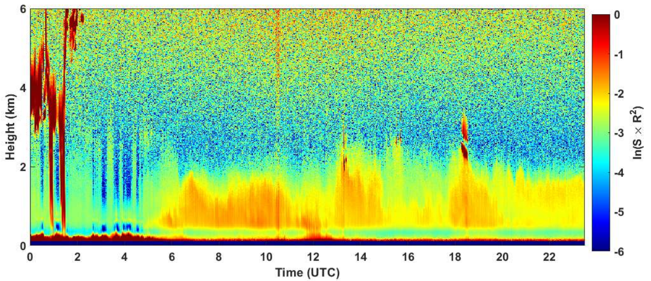
2024-01-18 RCS quick look CHM15k - ILVA LIDAR1 DIREZIONE
