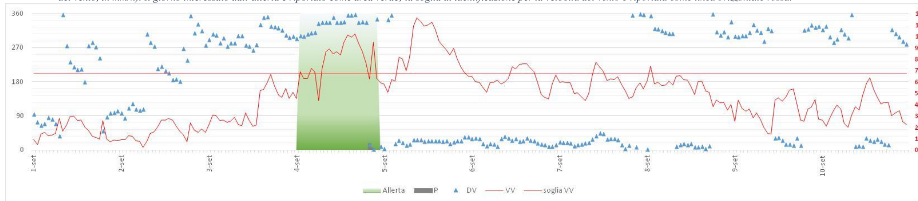
Figura 1: Velocità del vento (linea rossa, asse a destra, in m/s), direzione del vento (triangoli blu, asse a sinistra), precipitazione cumulata oraria (istogramma in grigio, stesso asse a destra della velocità del vento, in mm/h). Il giorno interessato dall'allerta è riportato come area verde; la soglia di identificazione per la velocità del vento è riportata come linea orizzontale rossa.
