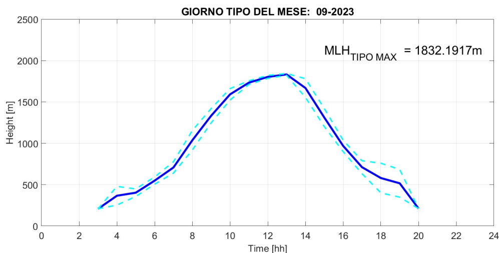
Fig. 2: Giorno tipo del parametro Mixing Layer Height nel mese di SETTEMBRE 2023, rappresentato mediante media oraria (linea blu continua) e deviazione standard (linee celesti tratteggiate).
