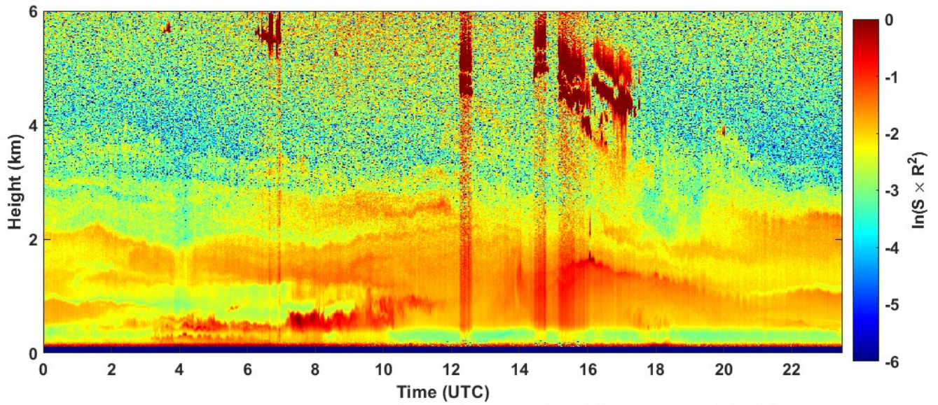
2023-09-16 RCS quick look CHM15k - ILVA LIDAR1 DIREZIONE
