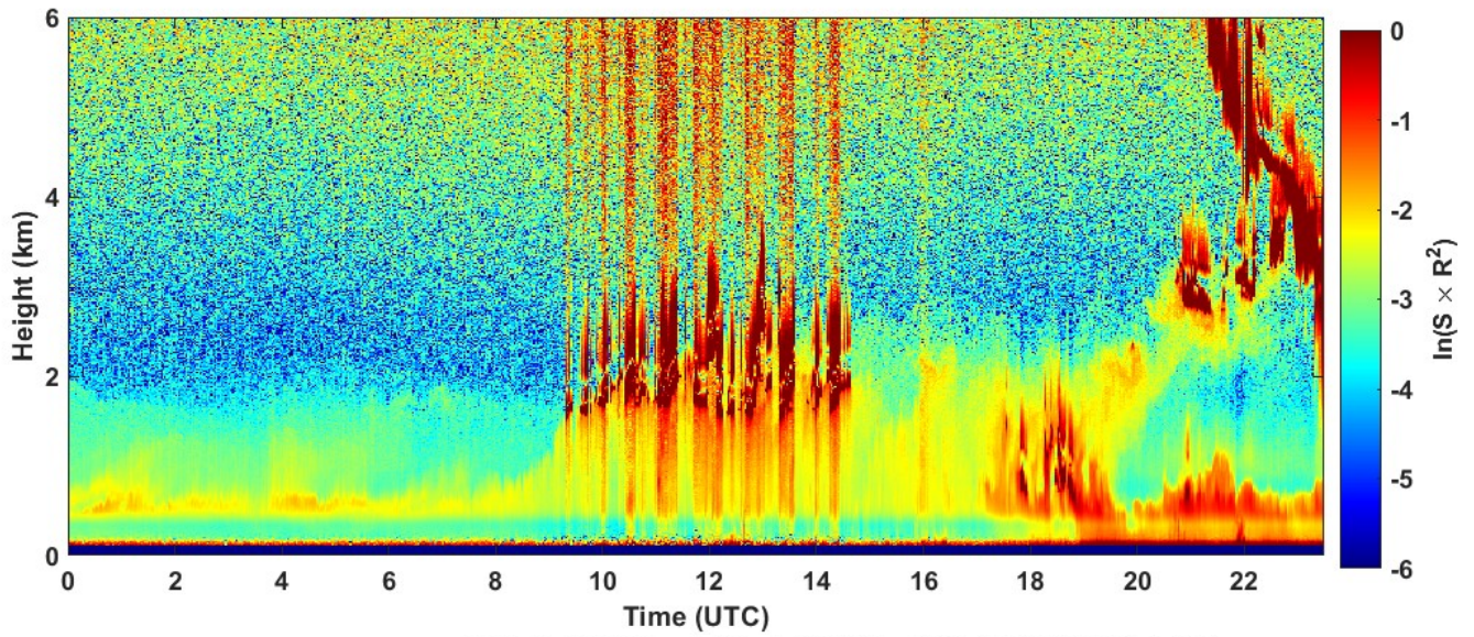
2023-09-26 RCS quick look CHM15k - ILVA LIDAR1 DIREZIONE
