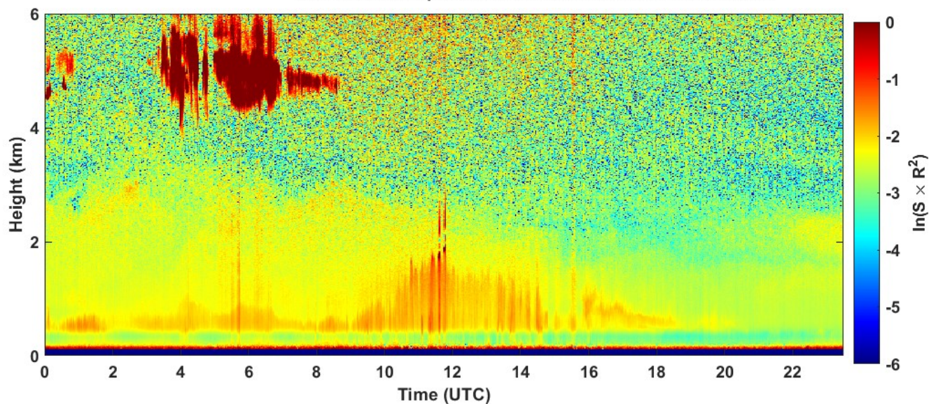
2023-09-28 RCS quick look CHM15k - ILVA LIDAR1 DIREZIONE
