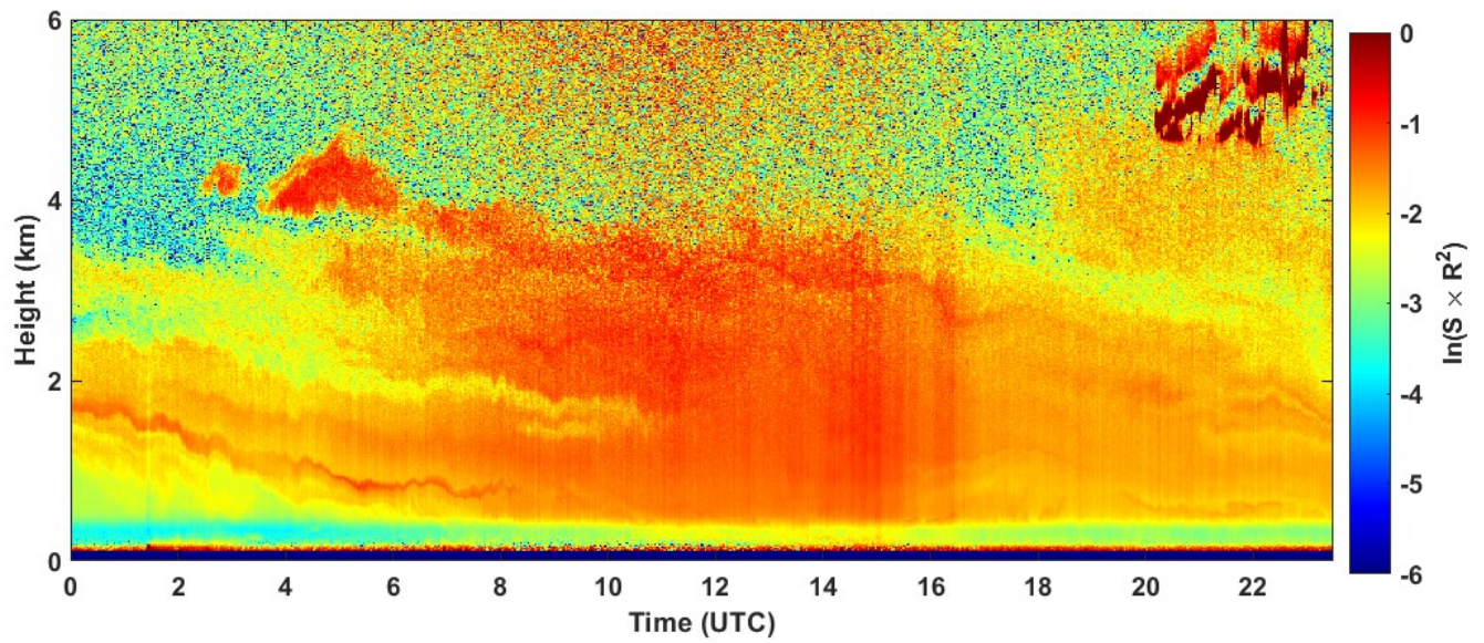
2023-09-18 RCS quick look CHM15k - ILVA LIDAR1 DIREZIONE
