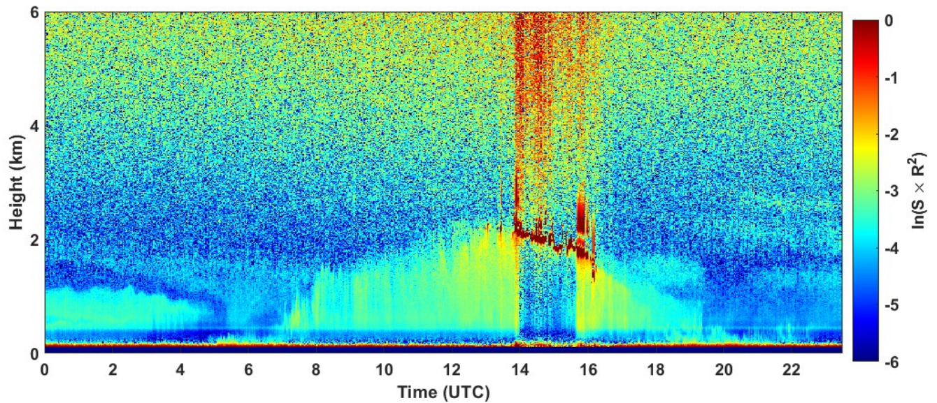
2023-09-02 RCS quick look CHM15k - ILVA LIDAR1 DIREZIONE
