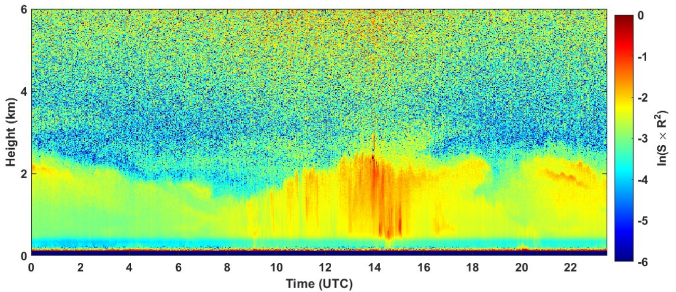
2023-08-16 RCS quick look CHM15k - ILVA LIDAR1 DIREZIONE
