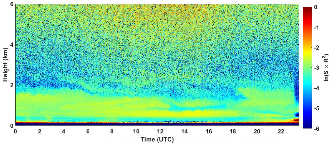
2023-08-28 RCS quick look CHM15k - ILVA LIDAR1 DIREZIONE
