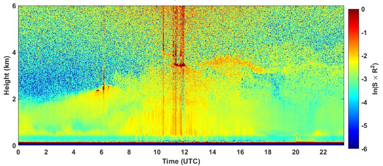
2023-08-20 RCS quick look CHM15k - ILVA LIDAR1 DIREZIONE
