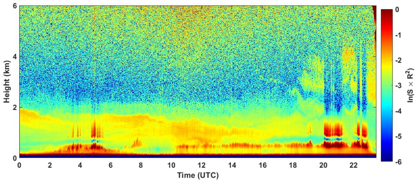
2023-08-04 RCS quick look CHM15k - ILVA LIDAR1 DIREZIONE
