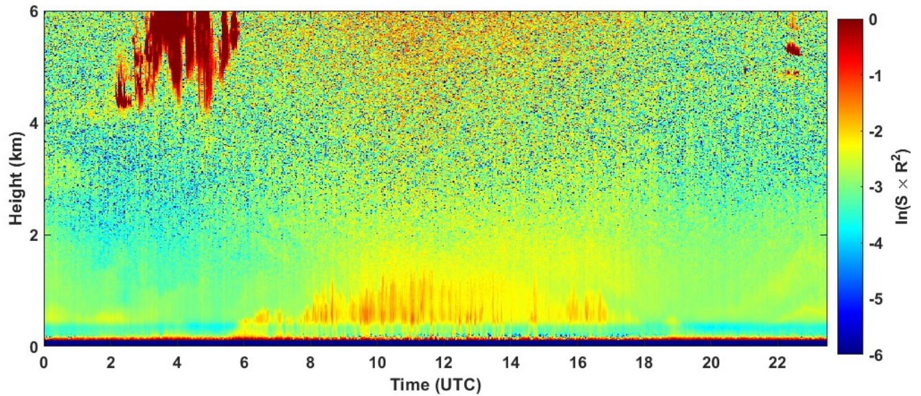
2023-08-22 RCS quick look CHM15k - ILVA LIDAR1 DIREZIONE
