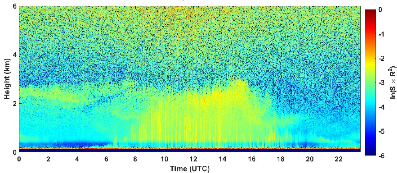
2023-08-10 RCS quick look CHM15k - ILVA LIDAR1 DIREZIONE
