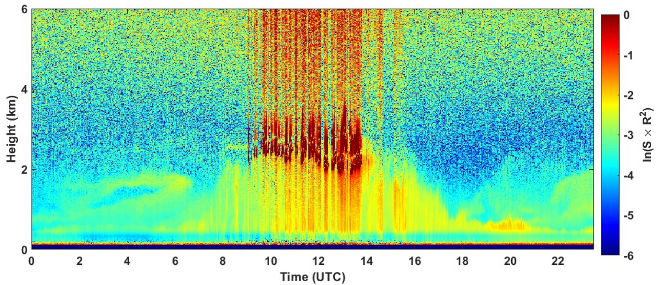
2023-08-12 RCS quick look CHM15k - ILVA LIDAR1 DIREZIONE
