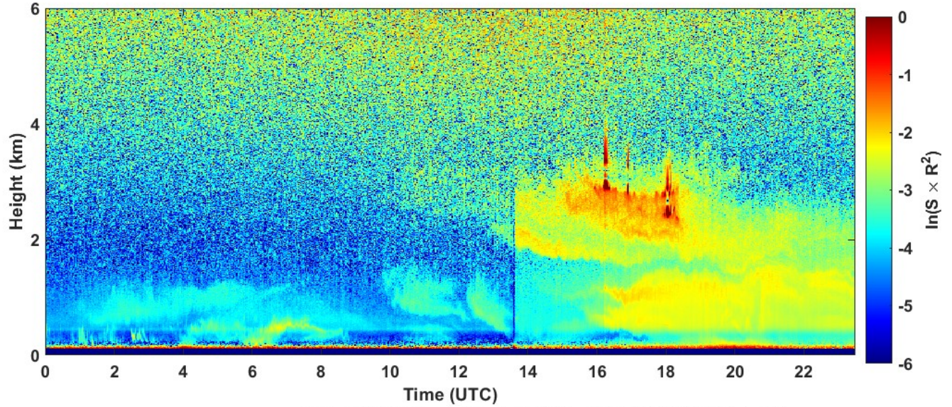
2023-08-02 RCS quick look CHM15k - ILVA LIDAR1 DIREZIONE
