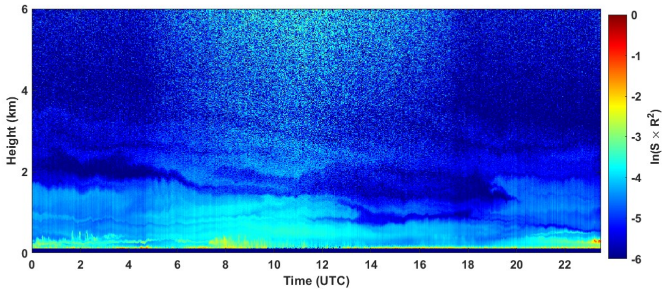
2023-08-28 RCS quick look CHM15k - ILVA LIDAR3 AGGLOMERATO
