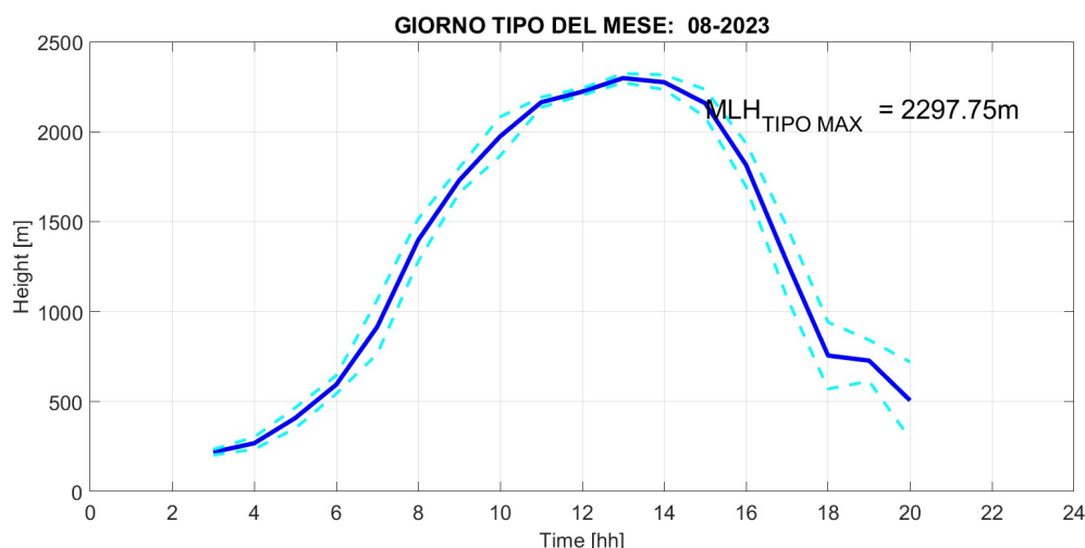
Fig. 2: Giorno tipo del parametro Mixing Layer Height nel mese di AGOSTO 2023, rappresentato mediante media oraria (linea blu continua) e deviazione standard (linee celesti tratteggiate).
