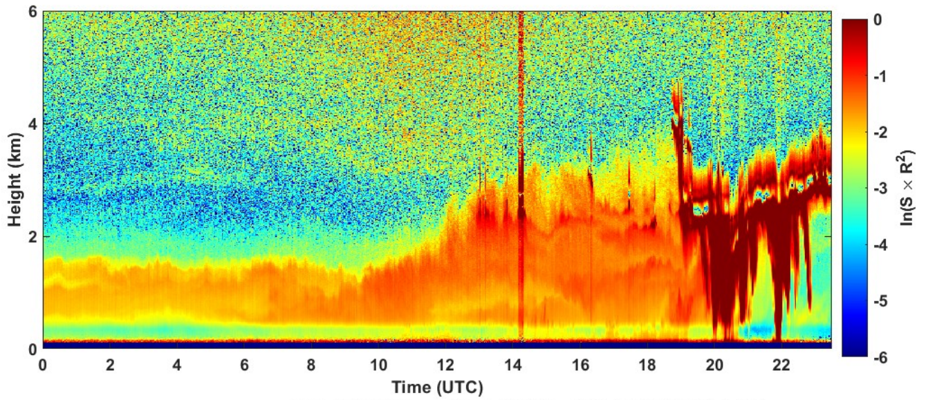
2023-08-08 RCS quick look CHM15k - ILVA LIDAR1 DIREZIONE
