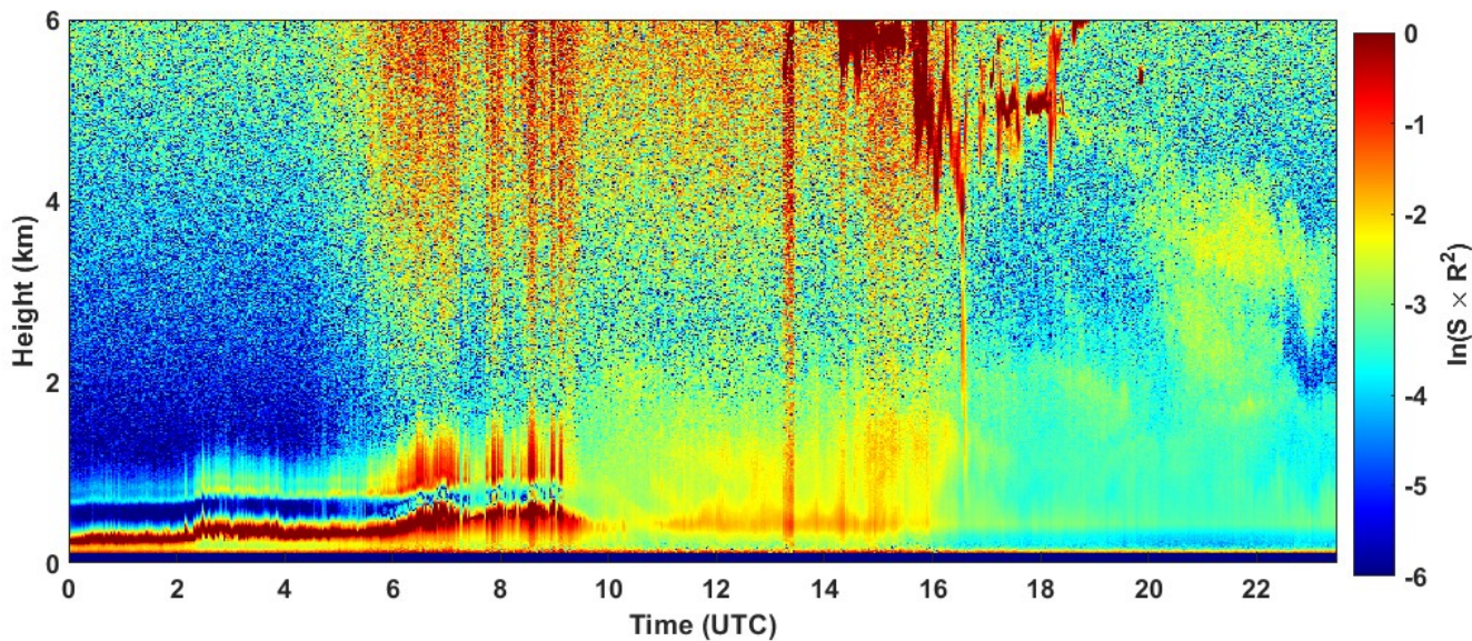
2023-08-28 RCS quick look CHM15k - ILVA LIDAR2 PARCHI
