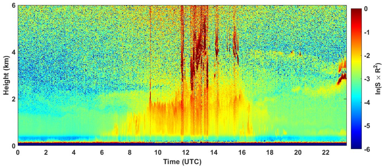
2023-08-14 RCS quick look CHM15k - ILVA LIDAR1 DIREZIONE
