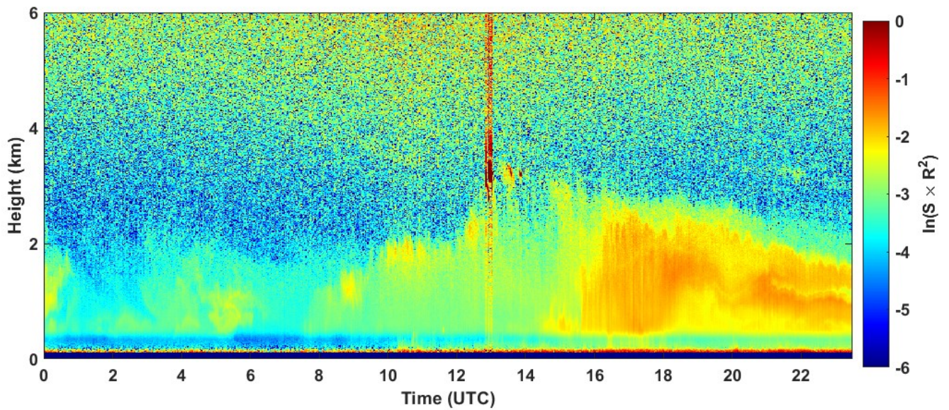
2023-08-06 RCS quick look CHM15k - ILVA LIDAR1 DIREZIONE
