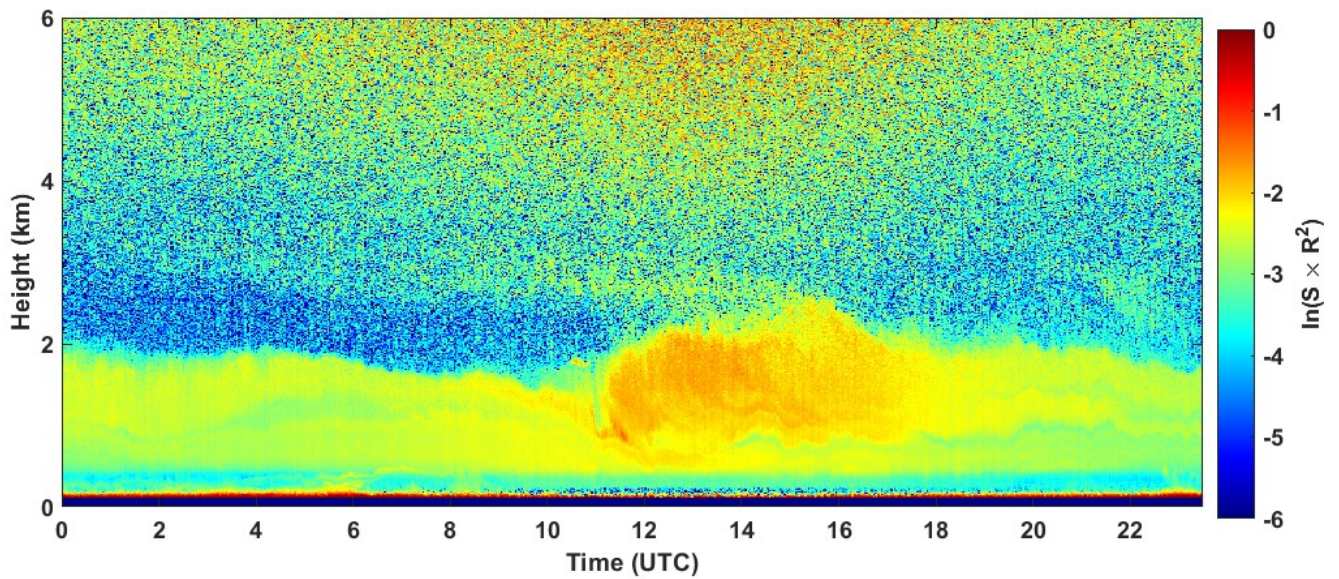
2023-08-26 RCS quick look CHM15k - ILVA LIDAR1 DIREZIONE
