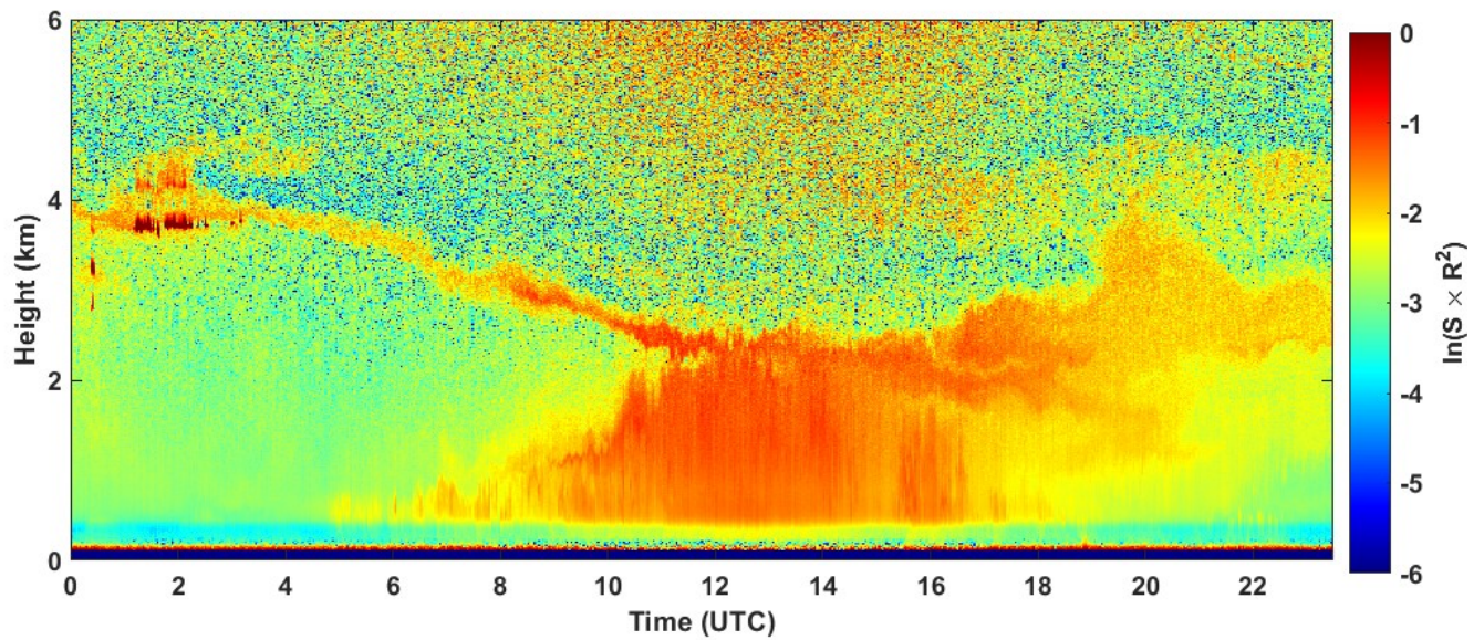
2023-08-24 RCS quick look CHM15k - ILVA LIDAR1 DIREZIONE
