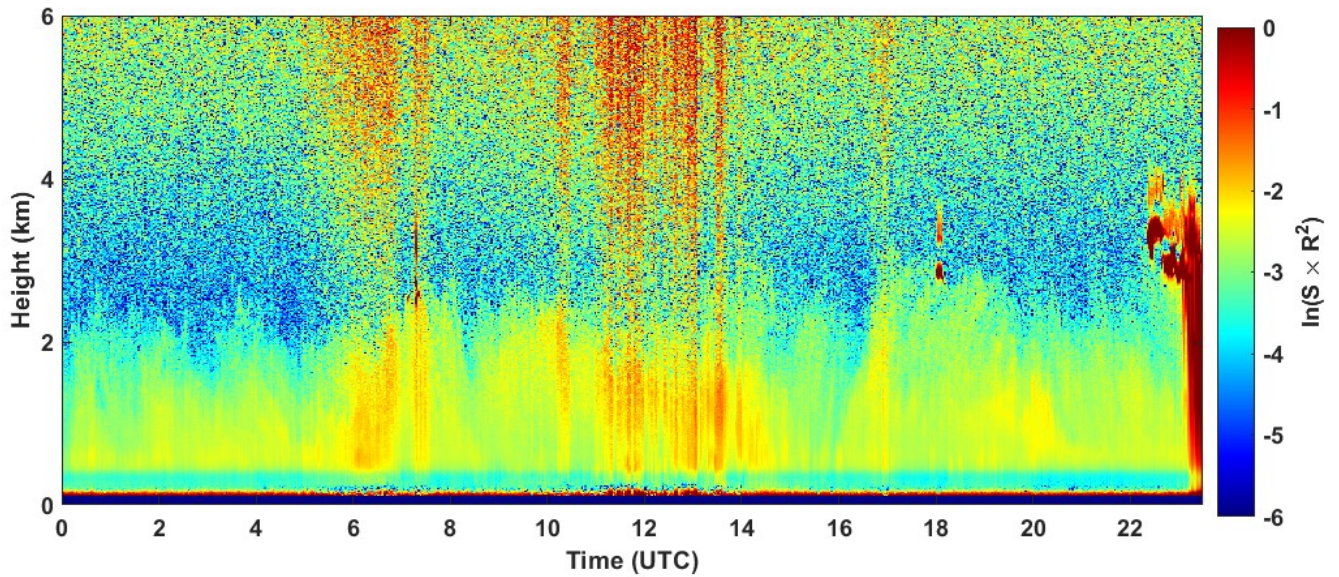
2023-08-30 RCS quick look CHM15k - ILVA LIDAR1 DIREZIONE
