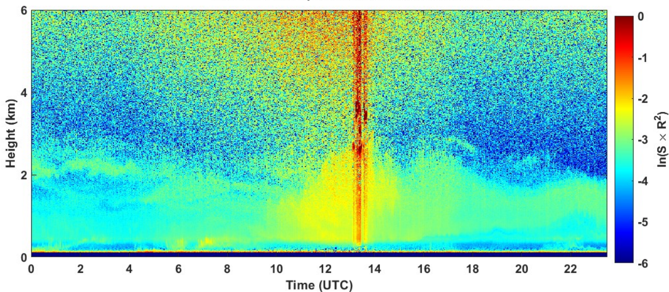
2023-08-26 RCS quick look CHM15k - ILVA LIDAR2 PARCHI
