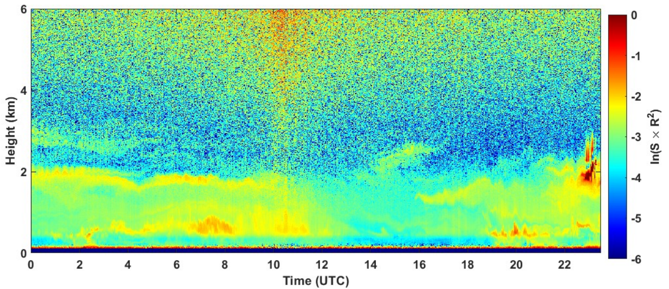
2023-07-04 RCS quick look CHM15k - ILVA LIDAR1 DIREZIONE
