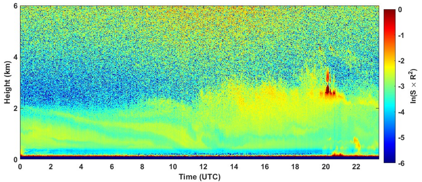
2023-07-30 RCS quick look CHM15k - ILVA LIDAR1 DIREZIONE
