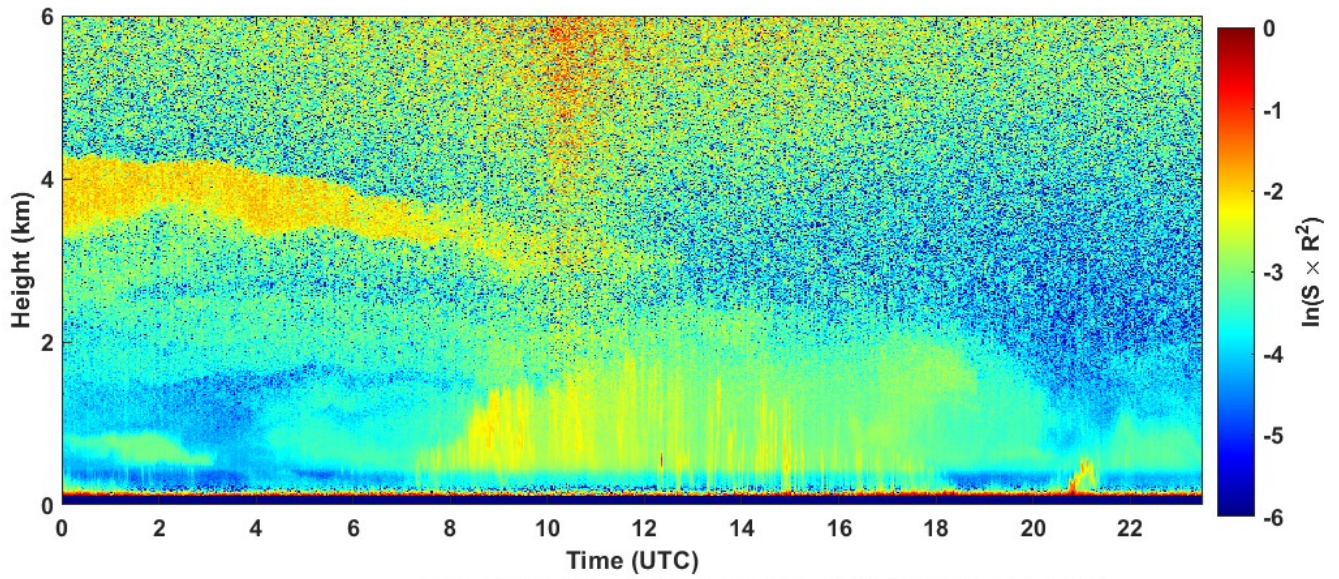
2023-07-10 RCS quick look CHM15k - ILVA LIDAR1 DIREZIONE
