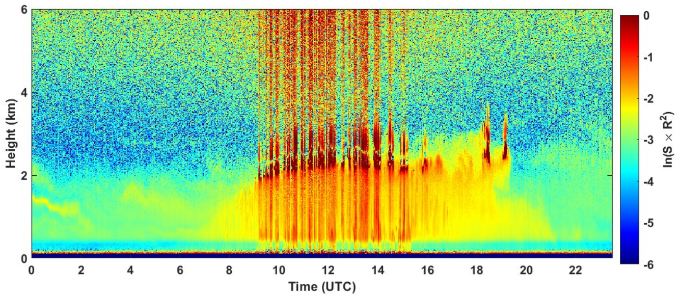
2023-07-06 RCS quick look CHM15k - ILVA LIDAR1 DIREZIONE
