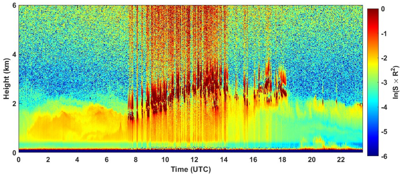
2023-07-02 RCS quick look CHM15k - ILVA LIDAR1 DIREZIONE
