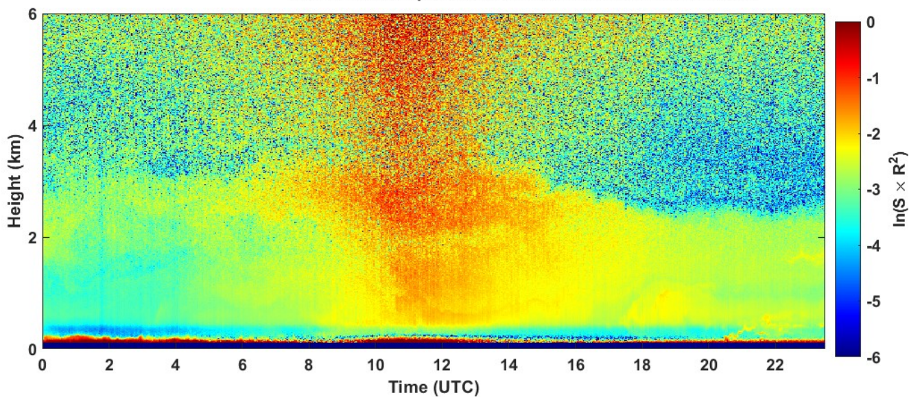
2023-07-14 RCS quick look CHM15k - ILVA LIDAR1 DIREZIONE
