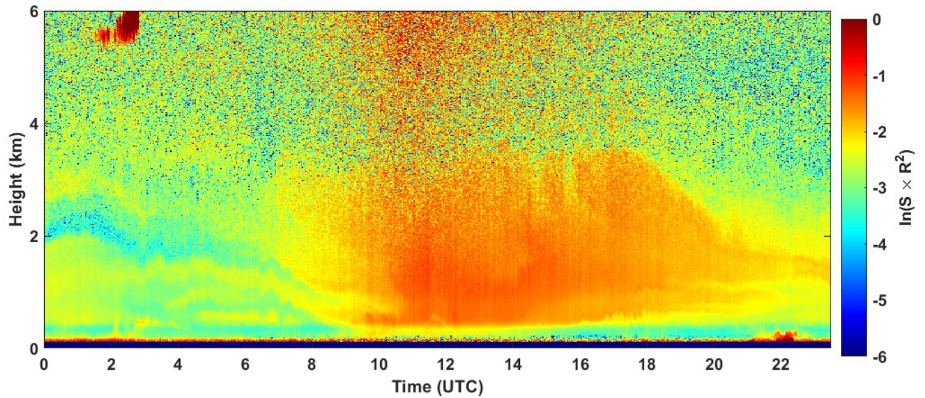
2023-07-20 RCS quick look CHM15k - ILVA LIDAR1 DIREZIONE
