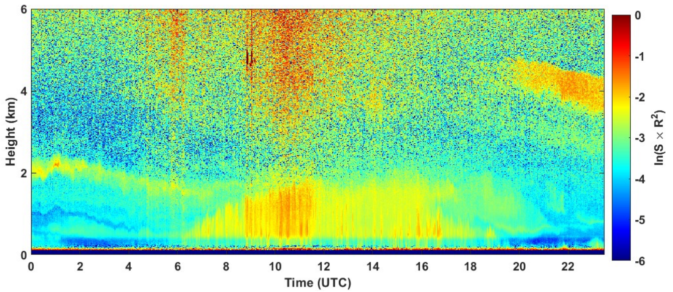
2023-07-08 RCS quick look CHM15k - ILVA LIDAR1 DIREZIONE
