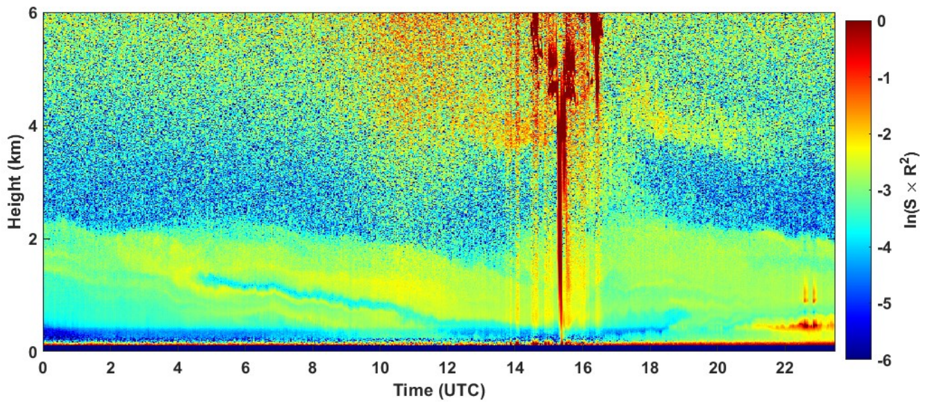
2023-07-28 RCS quick look CHM15k - ILVA LIDAR1 DIREZIONE
