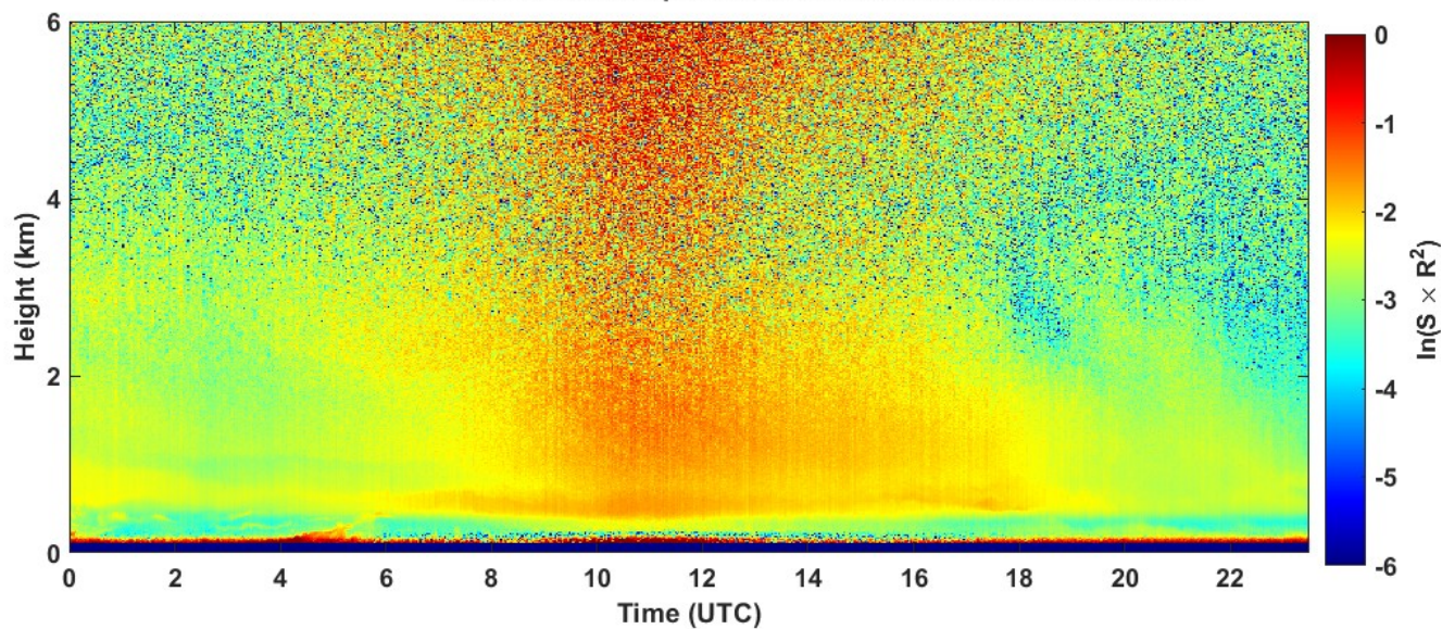
2023-07-24 RCS quick look CHM15k - ILVA LIDAR1 DIREZIONE
