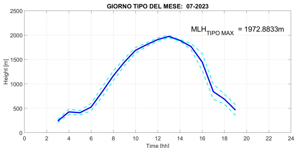
Fig. 2: Giorno tipo del parametro Mixing Layer Height nel mese di LUGLIO 2023, rappresentato mediante media oraria (linea blu continua) e deviazione standard (linee celesti tratteggiate).
