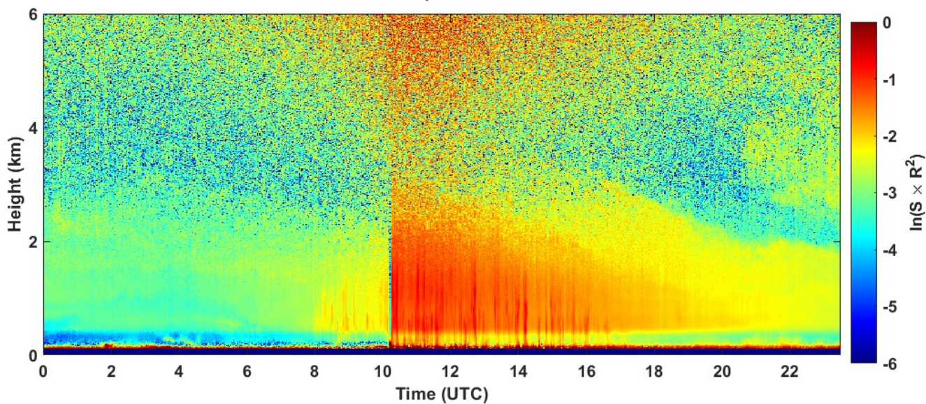
2023-07-18 RCS quick look CHM15k - ILVA LIDAR1 DIREZIONE
