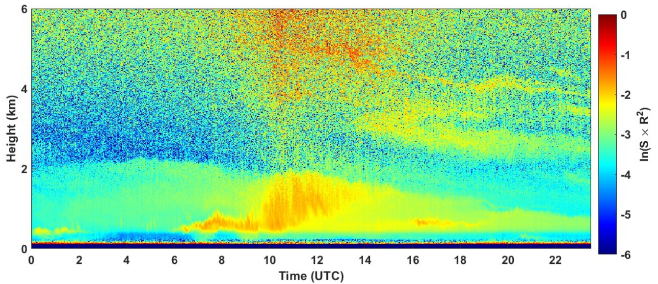
2023-07-12 RCS quick look CHM15k - ILVA LIDAR1 DIREZIONE
