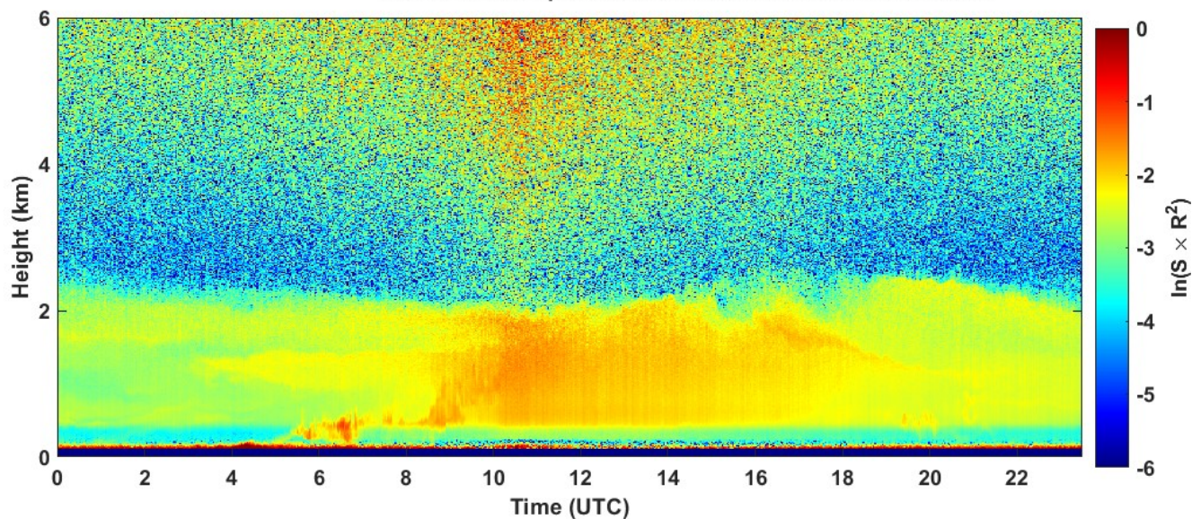
2023-07-16 RCS quick look CHM15k - ILVA LIDAR1 DIREZIONE
