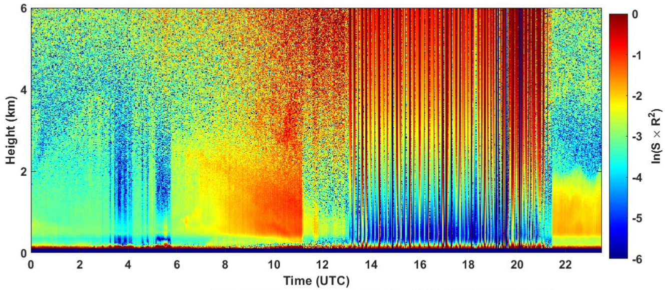
2023-07-26 RCS quick look CHM15k - ILVA LIDAR1 DIREZIONE
