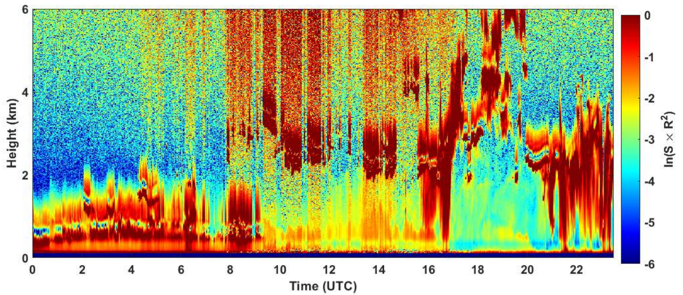
2023-05-16 RCS quick look CHM15k - ILVA LIDAR1 DIREZIONE
