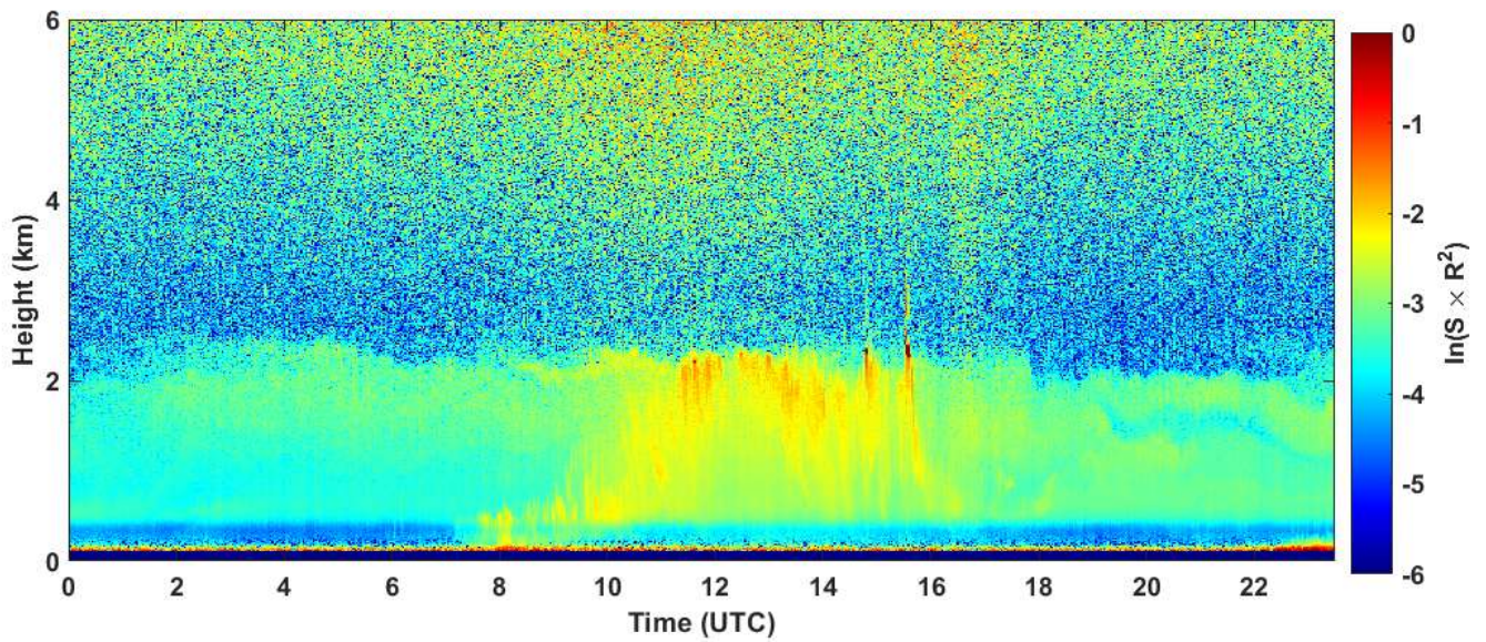
2023-05-06 RCS quick look CHM15k - ILVA LIDAR1 DIREZIONE
