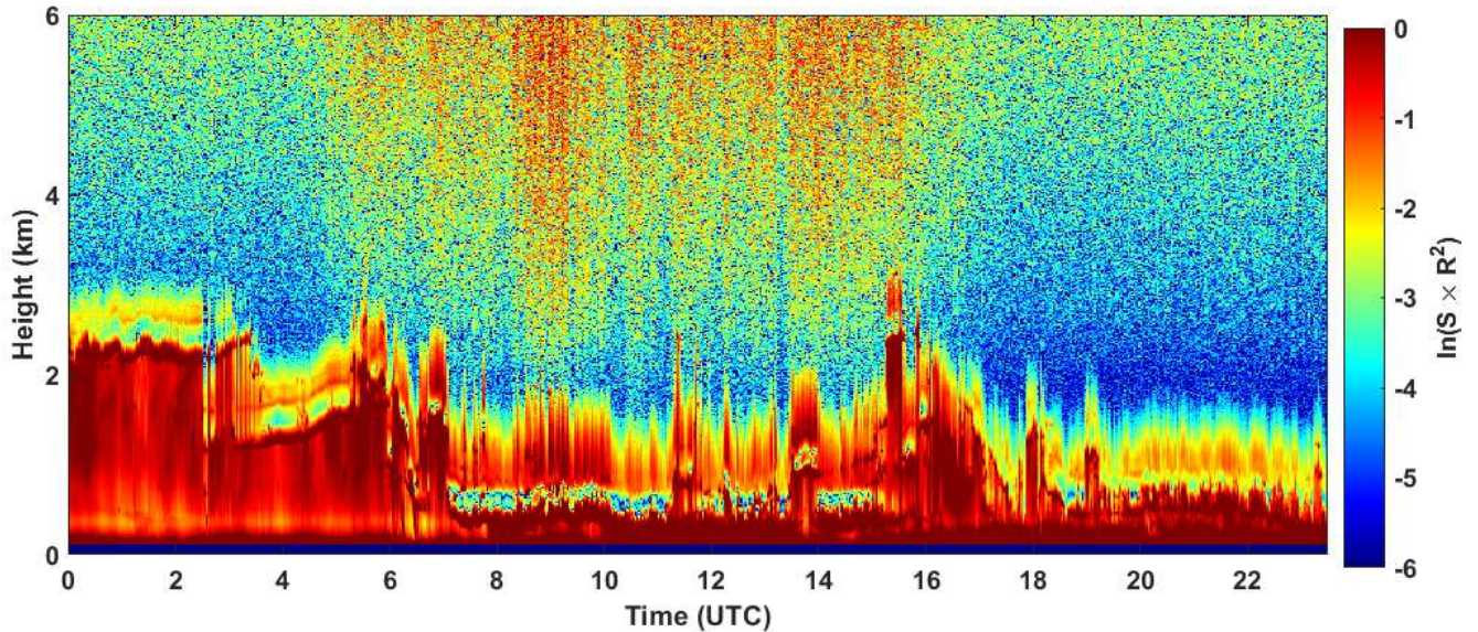
2023-05-02 RCS quick look CHM15k - ILVA LIDAR1 DIREZIONE
