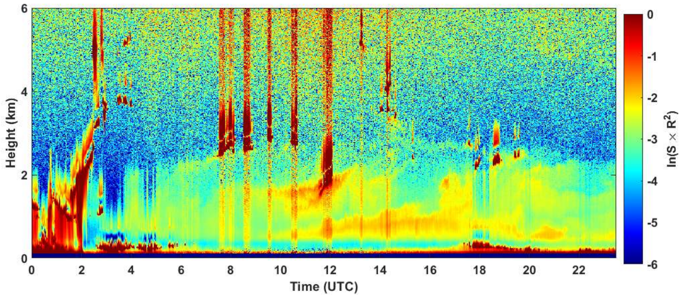
2023-05-12 RCS quick look CHM15k - ILVA LIDAR1 DIREZIONE
