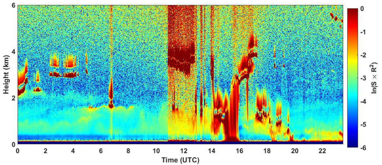
2023-05-18 RCS quick look CHM15k - ILVA LIDAR1 DIREZIONE
