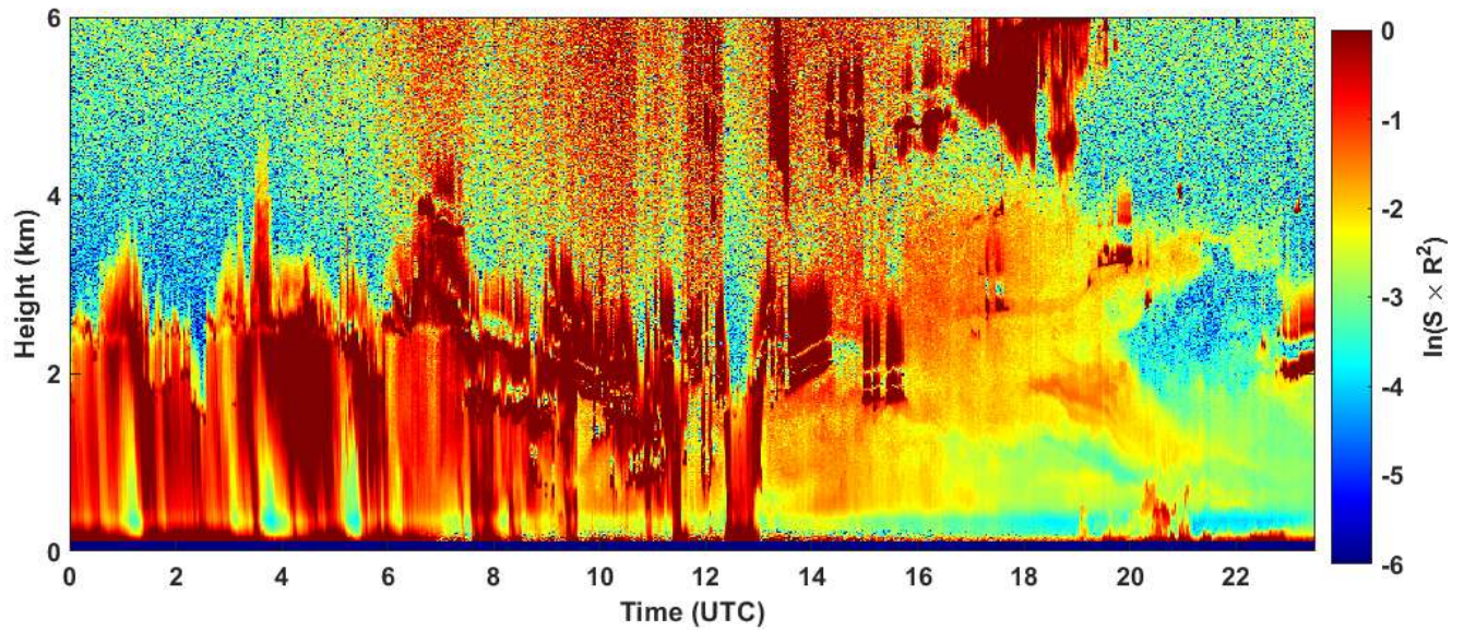
2023-05-22 RCS quick look CHM15k - ILVA LIDAR1 DIREZIONE
