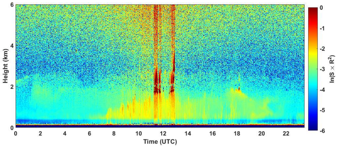
2023-05-28 RCS quick look CHM15k - ILVA LIDAR1 DIREZIONE
