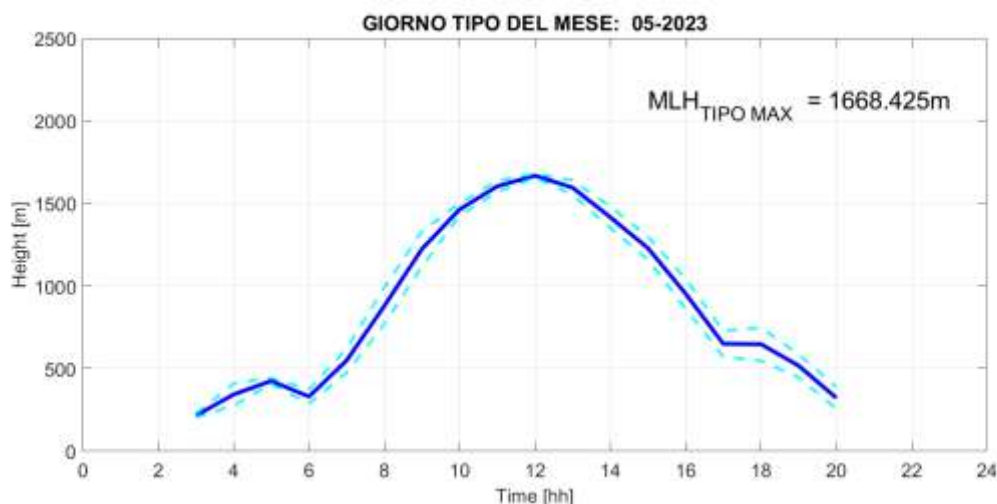
Fig. 2: Giorno tipo del parametro Mixing Layer Height nel mese di MAGGIO 2023, rappresentato mediante media oraria (linea blu continua) e deviazione standard (linee celesti tratteggiate).
