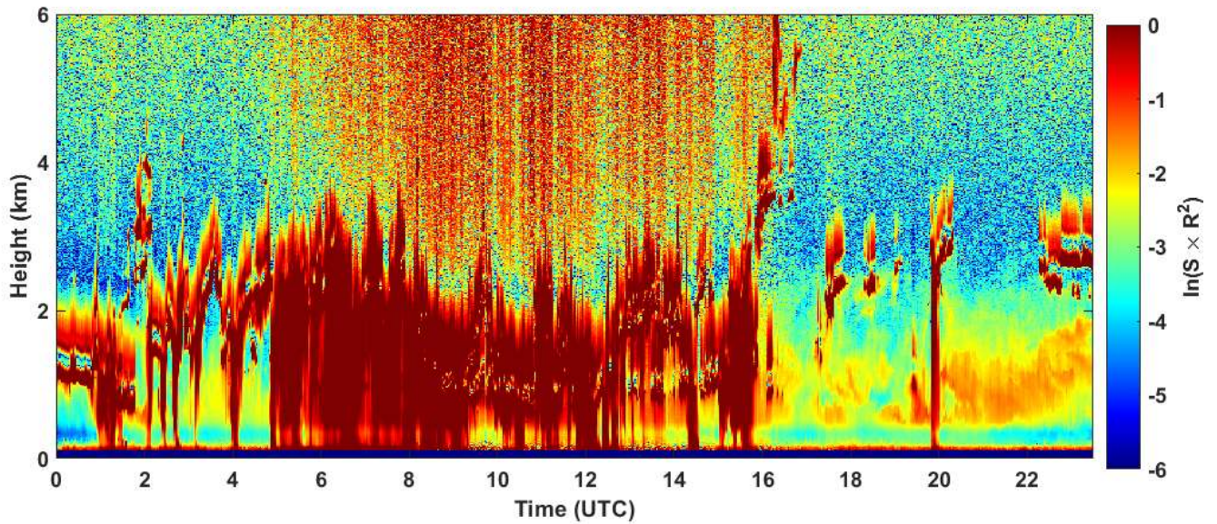
2023-05-04 RCS quick look CHM15k - ILVA LIDAR1 DIREZIONE
