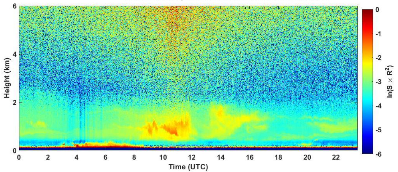
2023-05-24 RCS quick look CHM15k - ILVA LIDAR1 DIREZIONE
