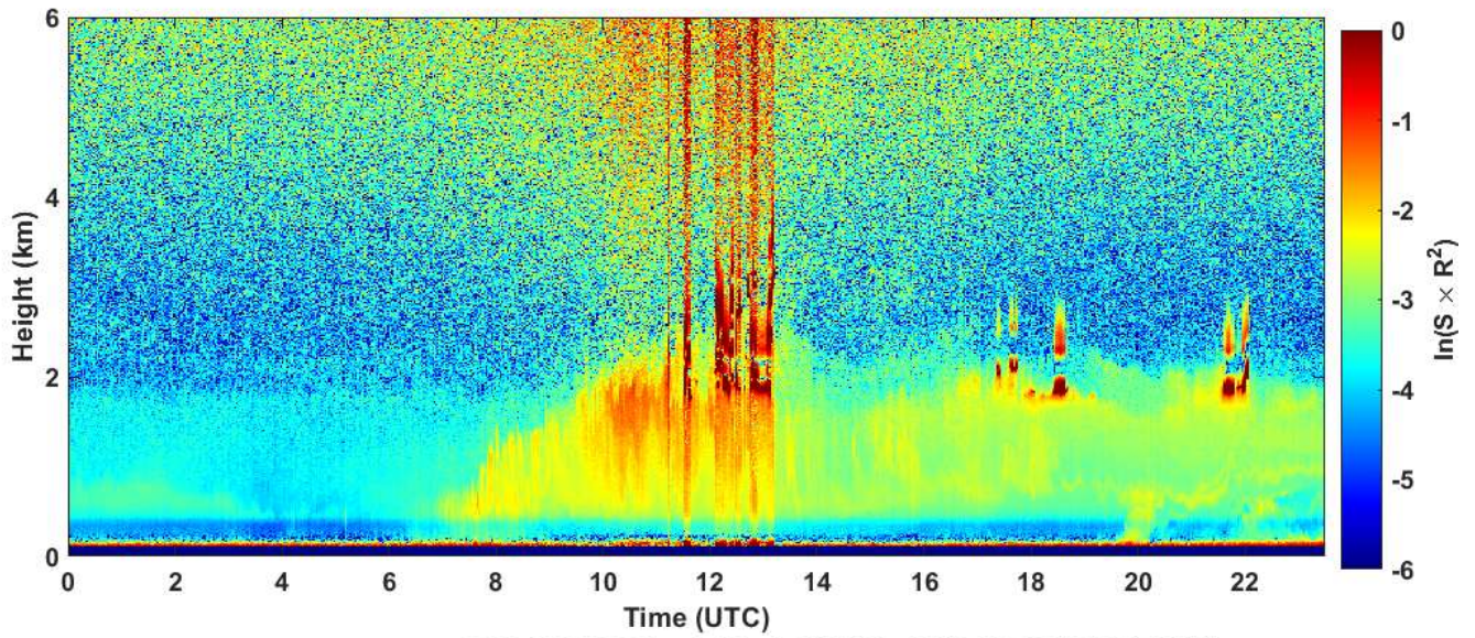
2023-05-30 RCS quick look CHM15k - ILVA LIDAR1 DIREZIONE
