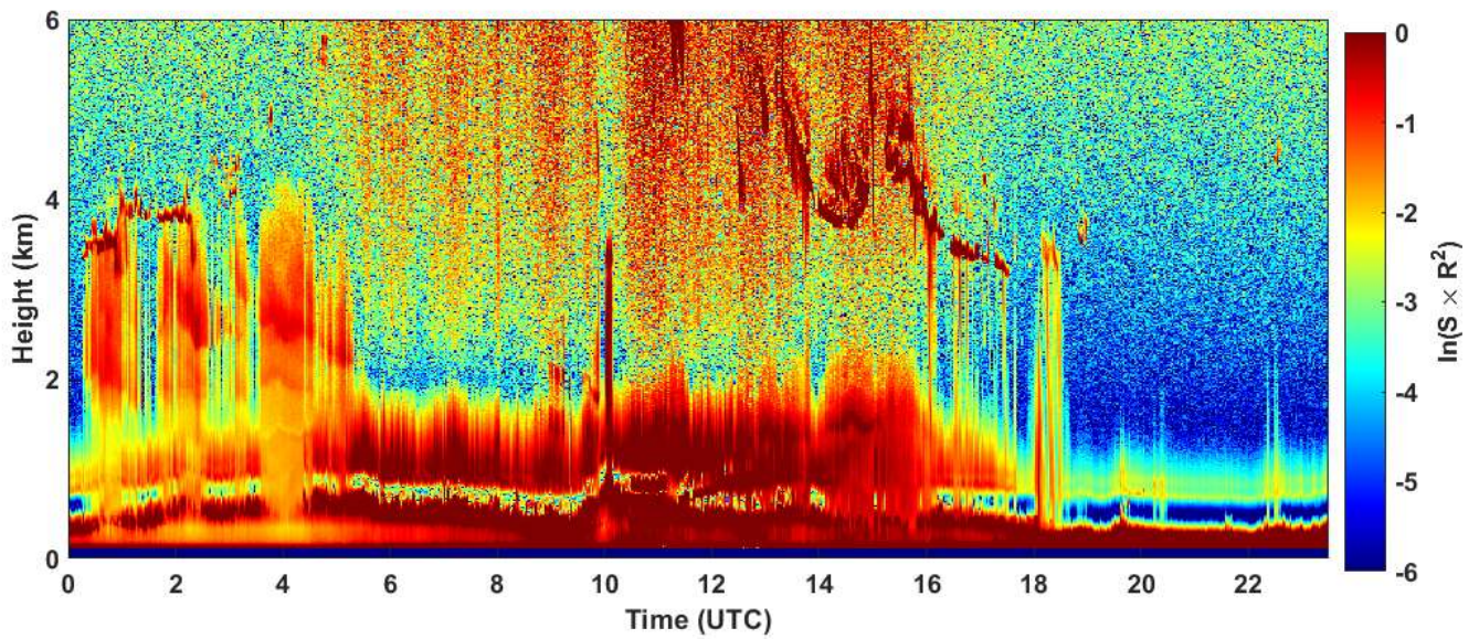
2023-05-14 RCS quick look CHM15k - ILVA LIDAR1 DIREZIONE
