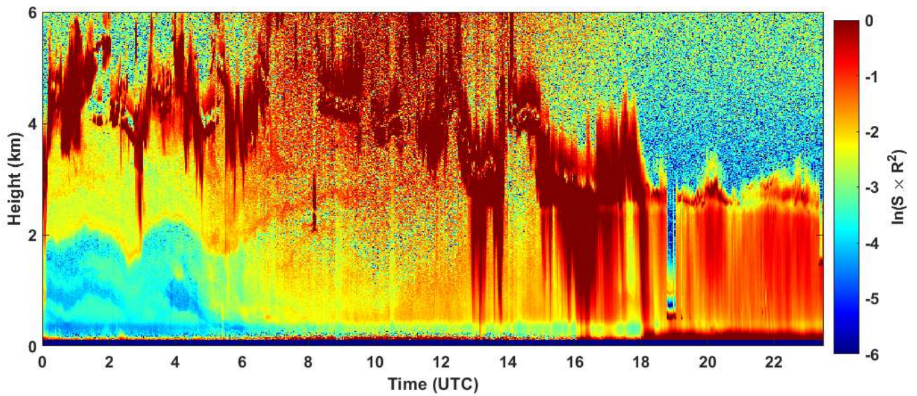
2023-05-20 RCS quick look CHM15k - ILVA LIDAR1 DIREZIONE
