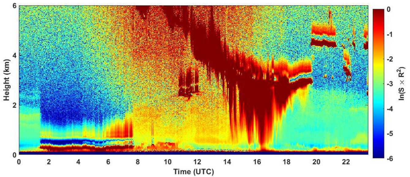
2023-05-08 RCS quick look CHM15k - ILVA LIDAR1 DIREZIONE
