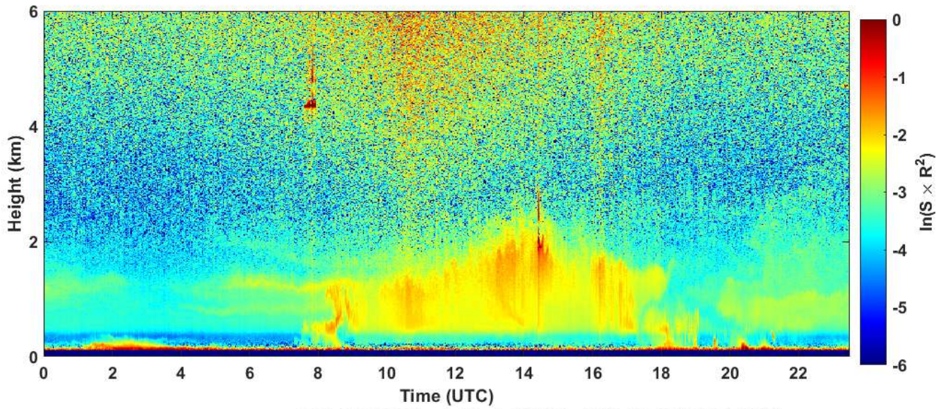
2023-05-26 RCS quick look CHM15k - ILVA LIDAR1 DIREZIONE
