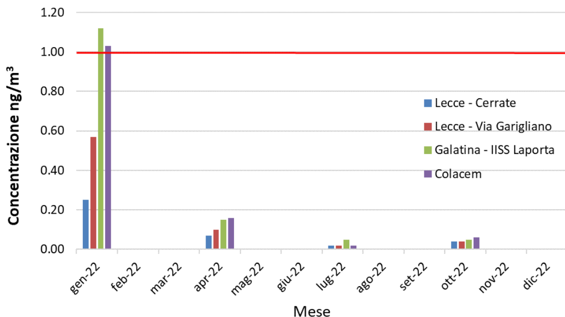
Figura 2: andamento delle concentrazioni di BaP durante le mensilità campionate.
