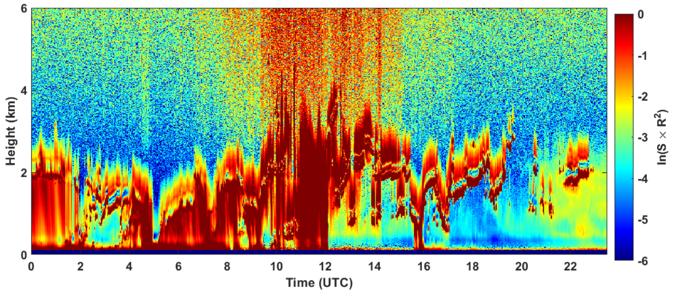
2023-03-22 RCS quick look CHM15k - ILVA LIDAR1 DIREZIONE
