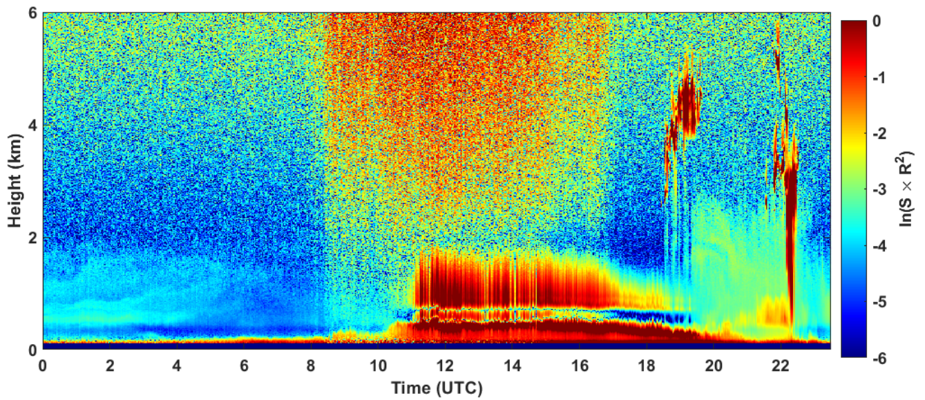
2023-03-14 RCS quick look CHM15k - ILVA LIDAR1 DIREZIONE
