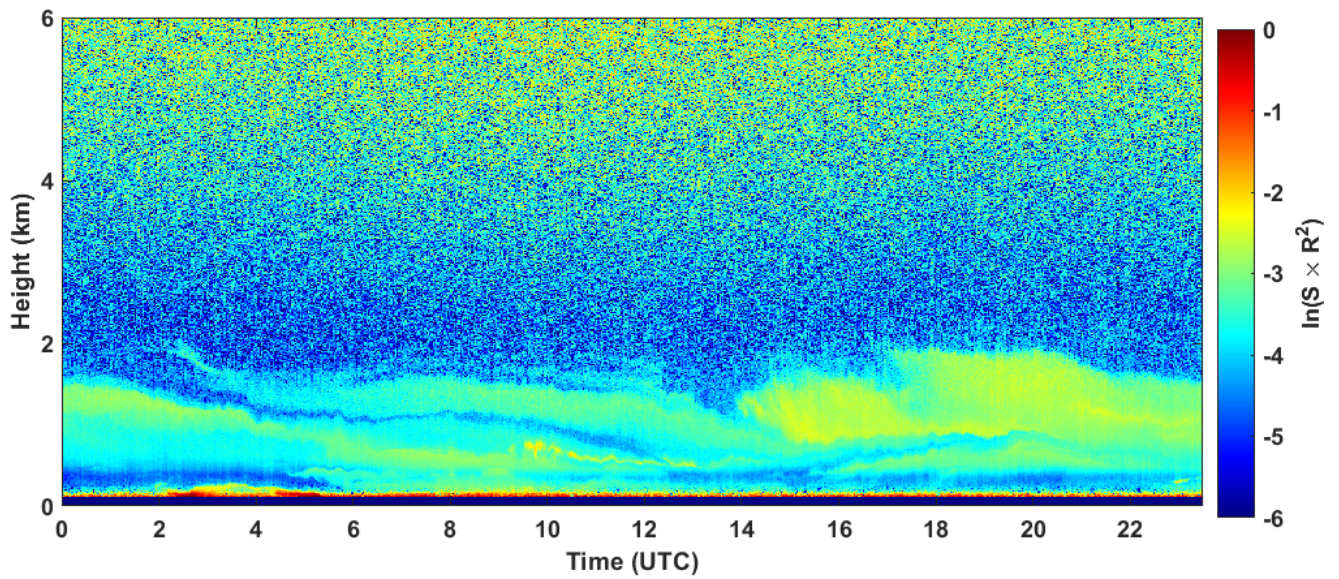
2023-03-24 RCS quick look CHM15k - ILVA LIDAR1 DIREZIONE
