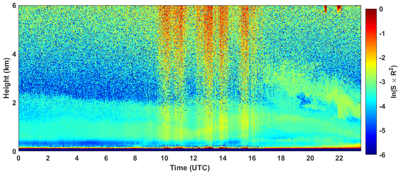
2023-03-30 RCS quick look CHM15k - ILVA LIDAR1 DIREZIONE
