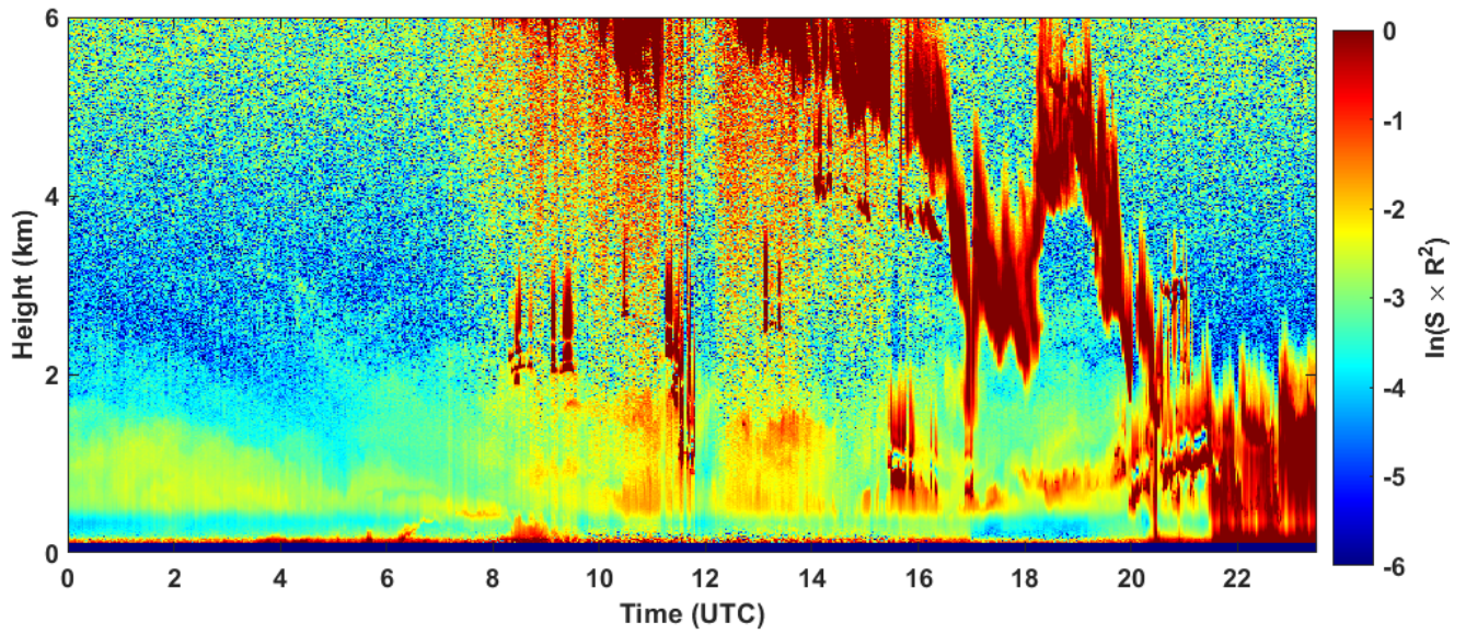
2023-03-04 RCS quick look CHM15k - ILVA LIDAR1 DIREZIONE
