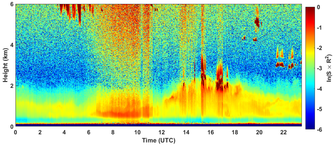
2023-03-12 RCS quick look CHM15k - ILVA LIDAR1 DIREZIONE
