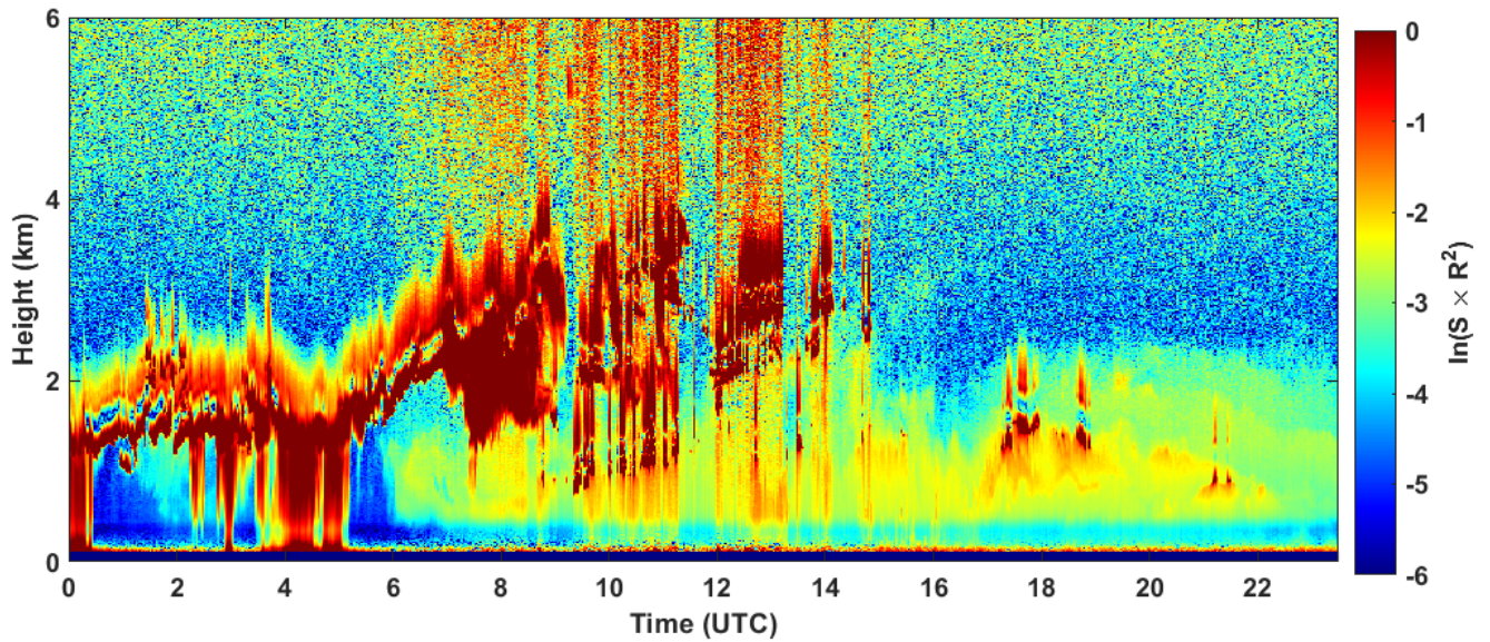
2023-03-06 RCS quick look CHM15k - ILVA LIDAR1 DIREZIONE
