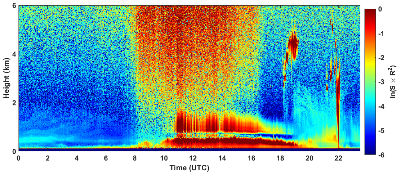
2023-03-14 RCS quick look CHM15k - ILVA LIDAR2 PARCHI
