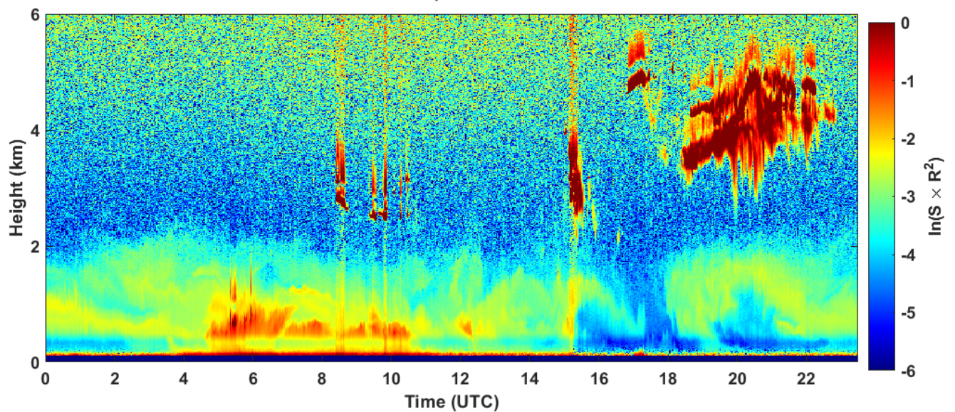
2023-03-02 RCS quick look CHM15k - ILVA LIDAR1 DIREZIONE
