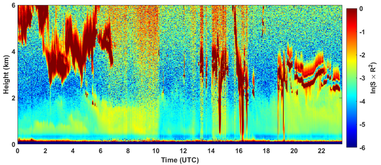
2023-03-10 RCS quick look CHM15k - ILVA LIDAR1 DIREZIONE
