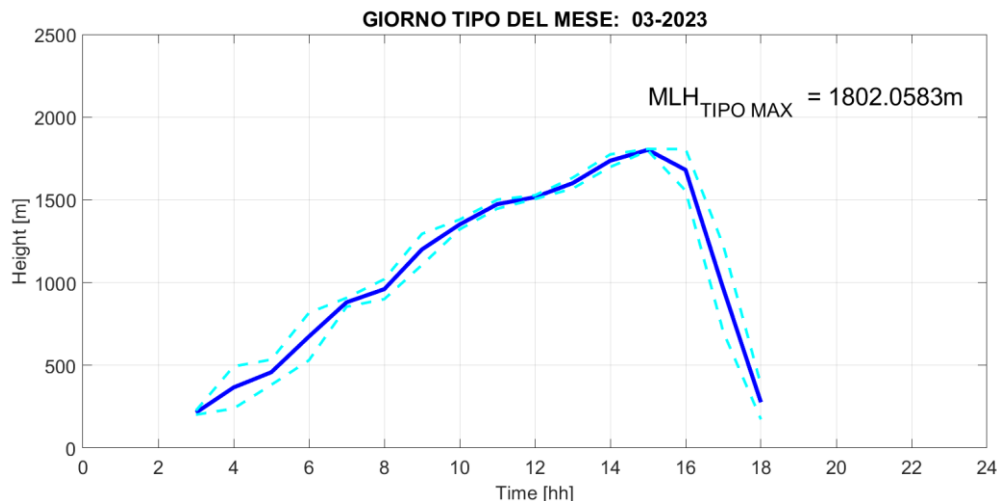
Fig. 2: Giorno tipo del parametro Mixing Layer Height nel mese di MARZO 2023, rappresentato mediante media oraria (linea blu continua) e deviazione standard (linee celesti tratteggiate).
