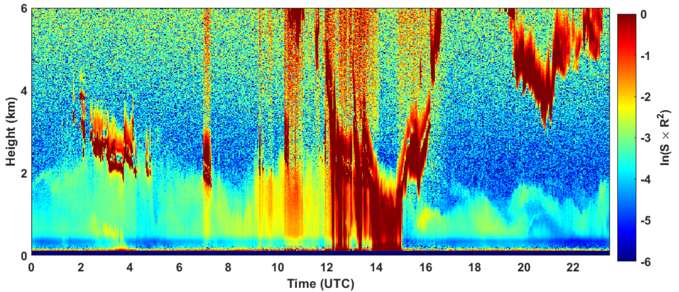
2023-03-28 RCS quick look CHM15k - ILVA LIDAR1 DIREZIONE
