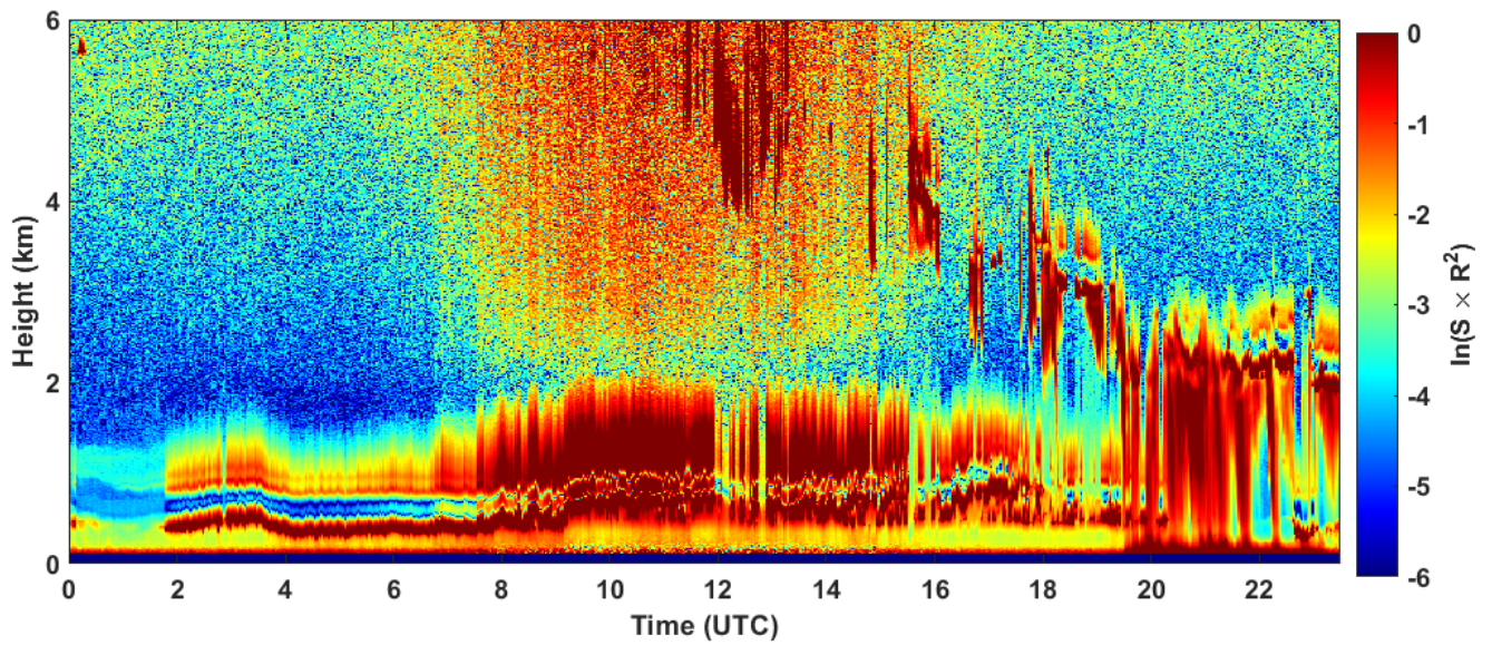
2023-03-20 RCS quick look CHM15k - ILVA LIDAR1 DIREZIONE
