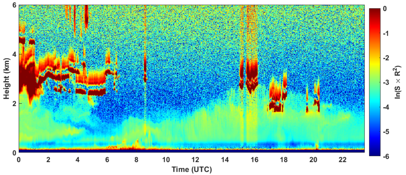
2023-03-08 RCS quick look CHM15k - ILVA LIDAR1 DIREZIONE
