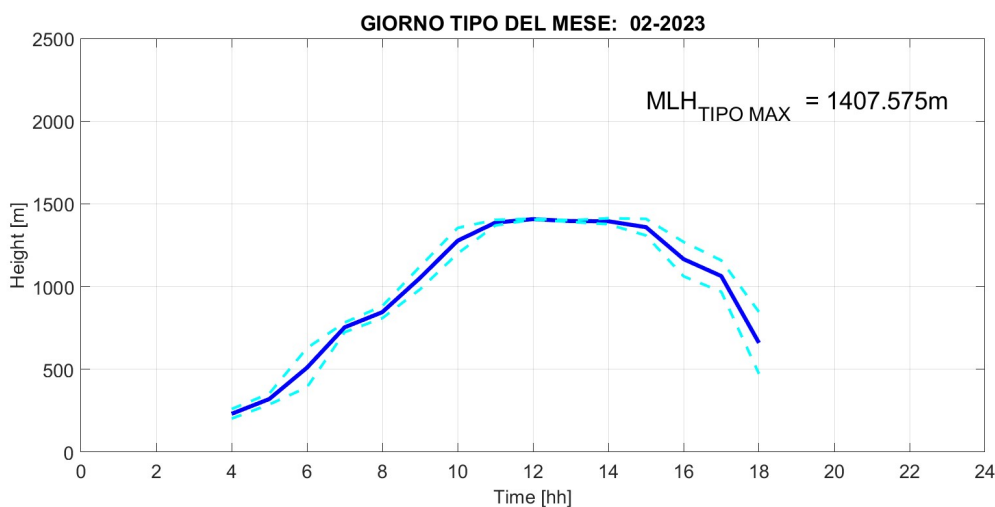
Fig. 2: Giorno tipo del parametro Mixing Layer Height nel mese di FEBBRAIO 2023, rappresentato mediante media oraria (linea blu continua) e deviazione standard (linee celesti tratteggiate).
