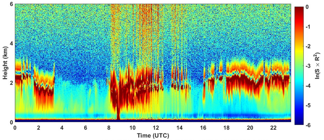
2023-02-08 RCS quick look CHM15k - ILVA LIDAR1 DIREZIONE
