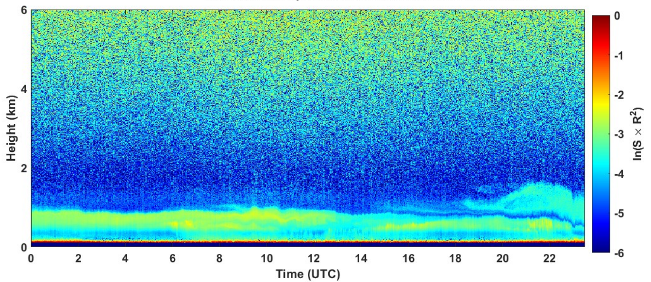
2023-02-16 RCS quick look CHM15k - ILVA LIDAR1 DIREZIONE
