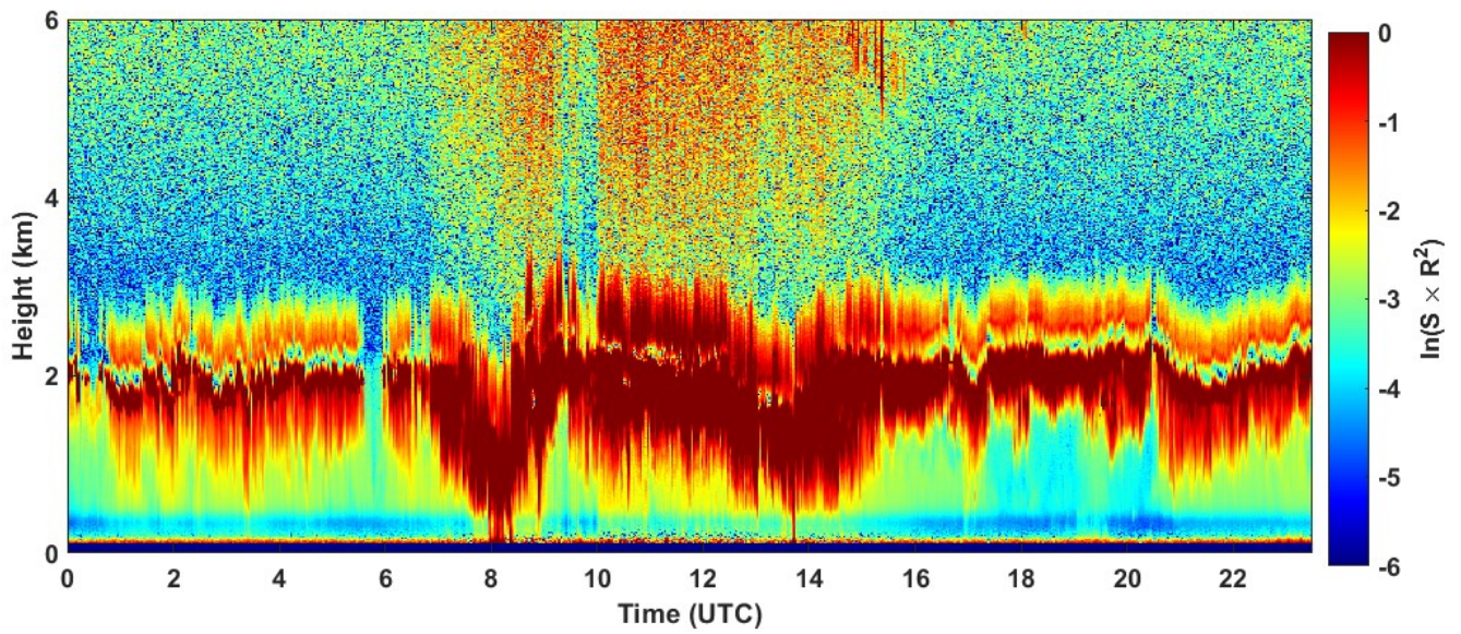
2023-02-06 RCS quick look CHM15k - ILVA LIDAR1 DIREZIONE
