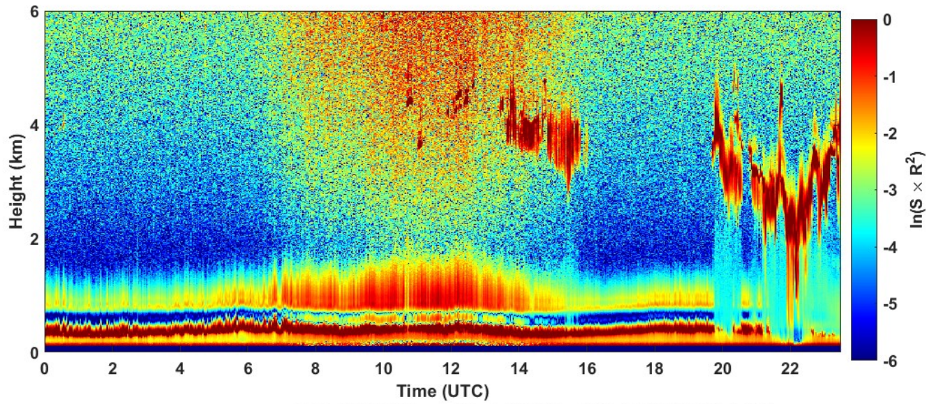
2023-02-26 RCS quick look CHM15k - ILVA LIDAR1 DIREZIONE
