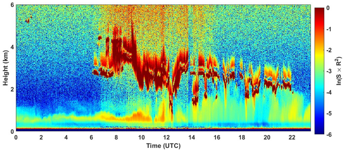
2023-02-12 RCS quick look CHM15k - ILVA LIDAR1 DIREZIONE
