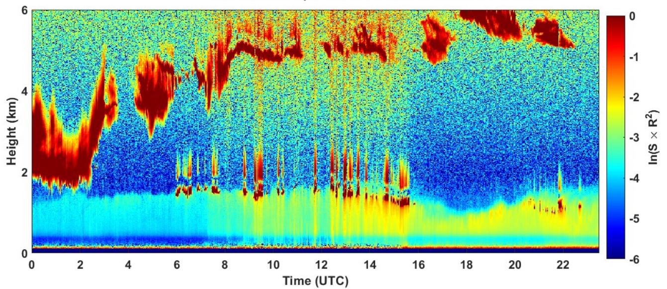
2023-02-10 RCS quick look CHM15k - ILVA LIDAR1 DIREZIONE
