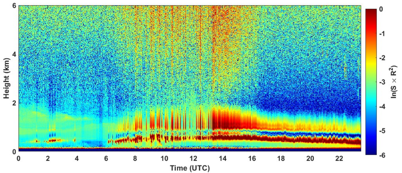
2023-02-24 RCS quick look CHM15k - ILVA LIDAR1 DIREZIONE
