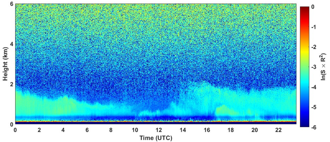
2023-02-02 RCS quick look CHM15k - ILVA LIDAR1 DIREZIONE
