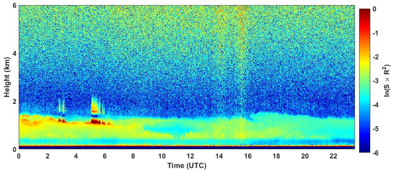
2023-02-18 RCS quick look CHM15k - ILVA LIDAR1 DIREZIONE
