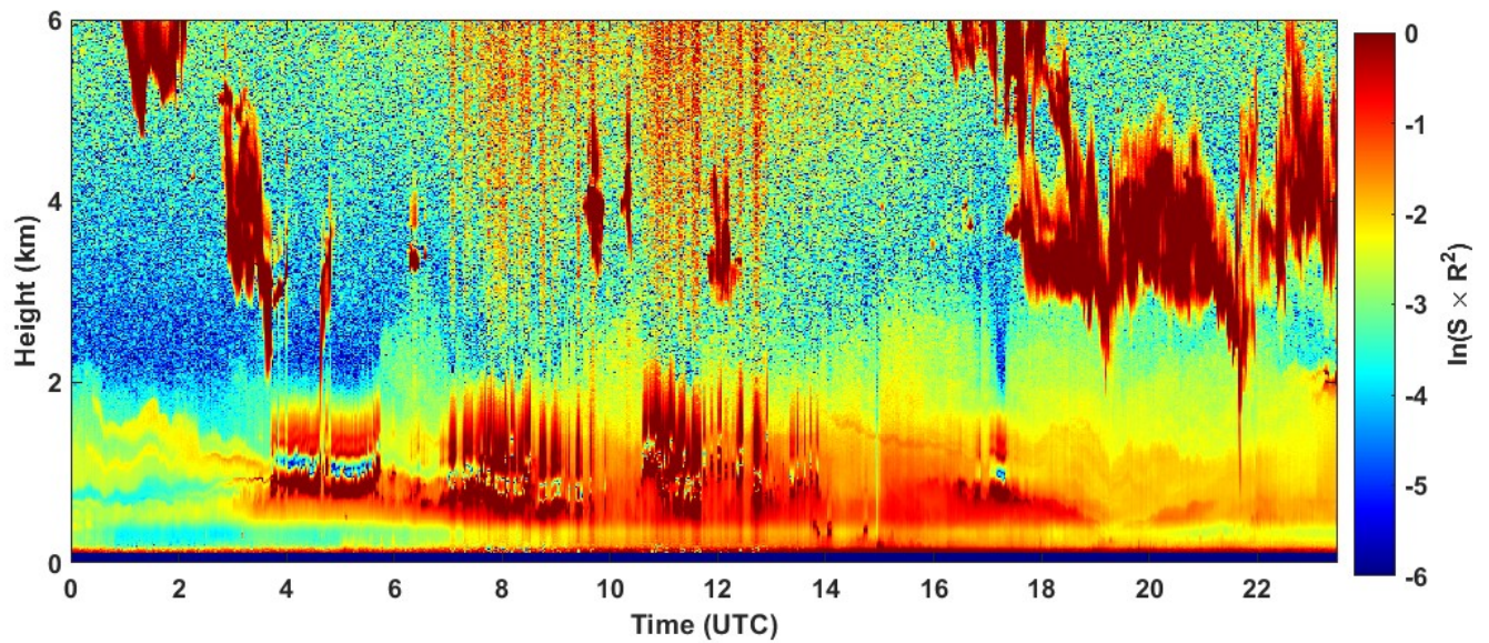
2023-02-28 RCS quick look CHM15k - ILVA LIDAR1 DIREZIONE
