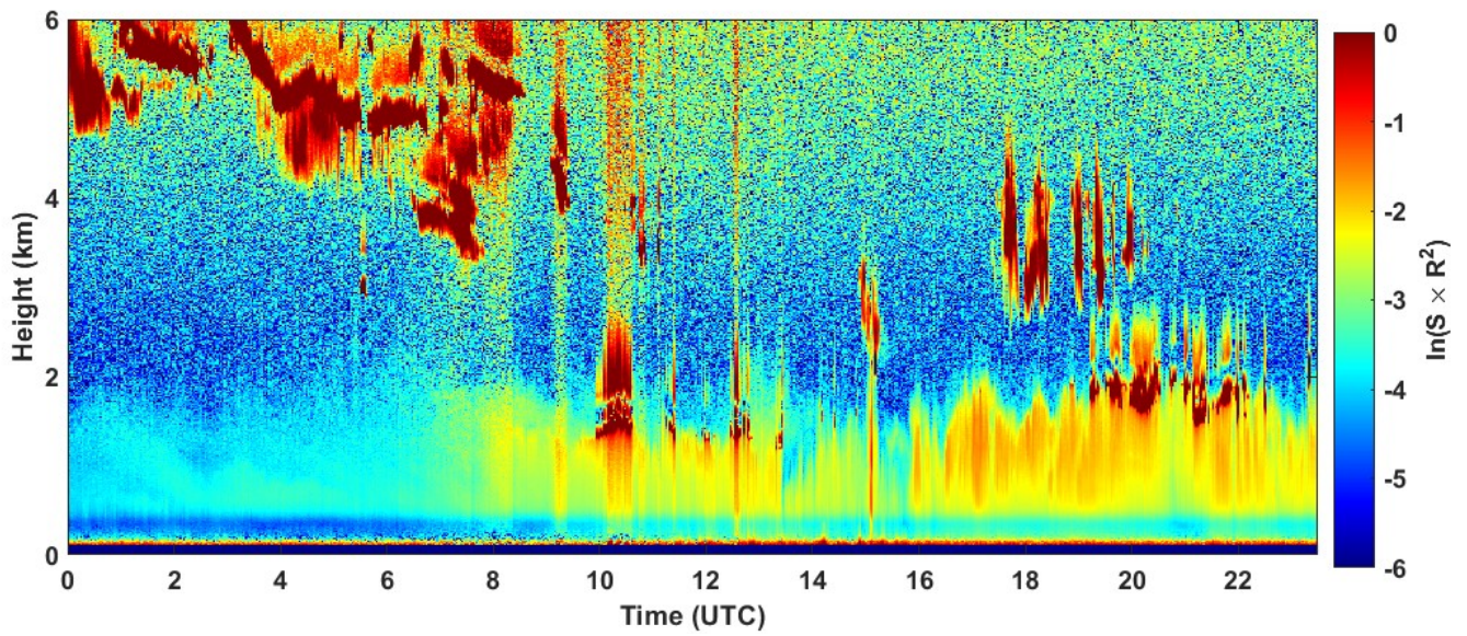
2023-02-04 RCS quick look CHM15k - ILVA LIDAR1 DIREZIONE
