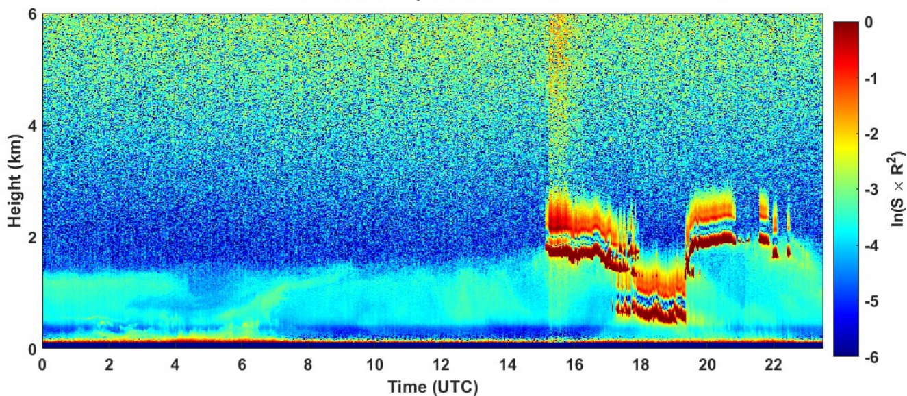
2023-02-20 RCS quick look CHM15k - ILVA LIDAR1 DIREZIONE
