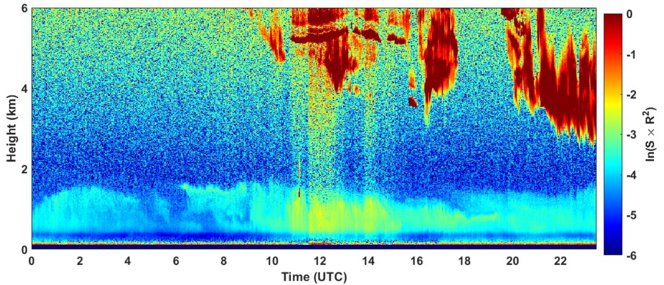
2023-01-14 RCS quick look CHM15k - ILVA LIDAR1 DIREZIONE
