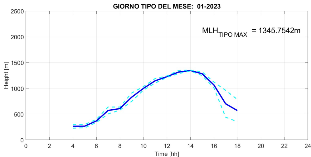
Fig. 2: Giorno tipo del parametro Mixing Layer Height nel mese di GENNAIO 2023, rappresentato mediante media oraria (linea blu continua) e deviazione standard (linee celesti tratteggiate).
