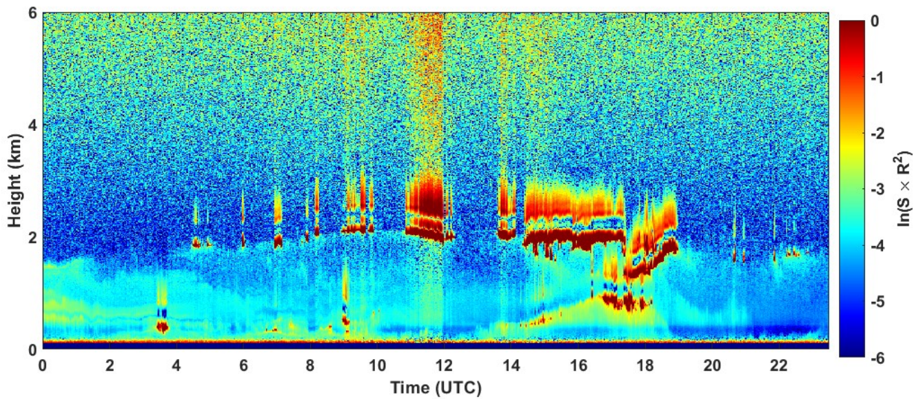
2023-01-08 RCS quick look CHM15k - ILVA LIDAR1 DIREZIONE
