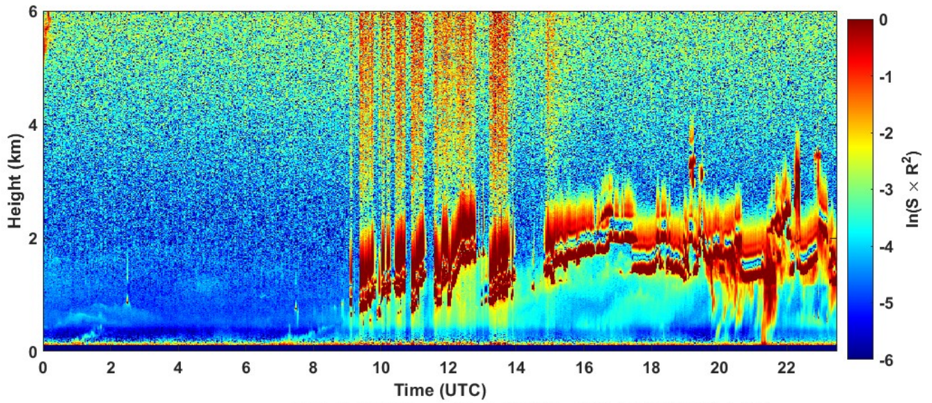
2023-01-28 RCS quick look CHM15k - ILVA LIDAR1 DIREZIONE
