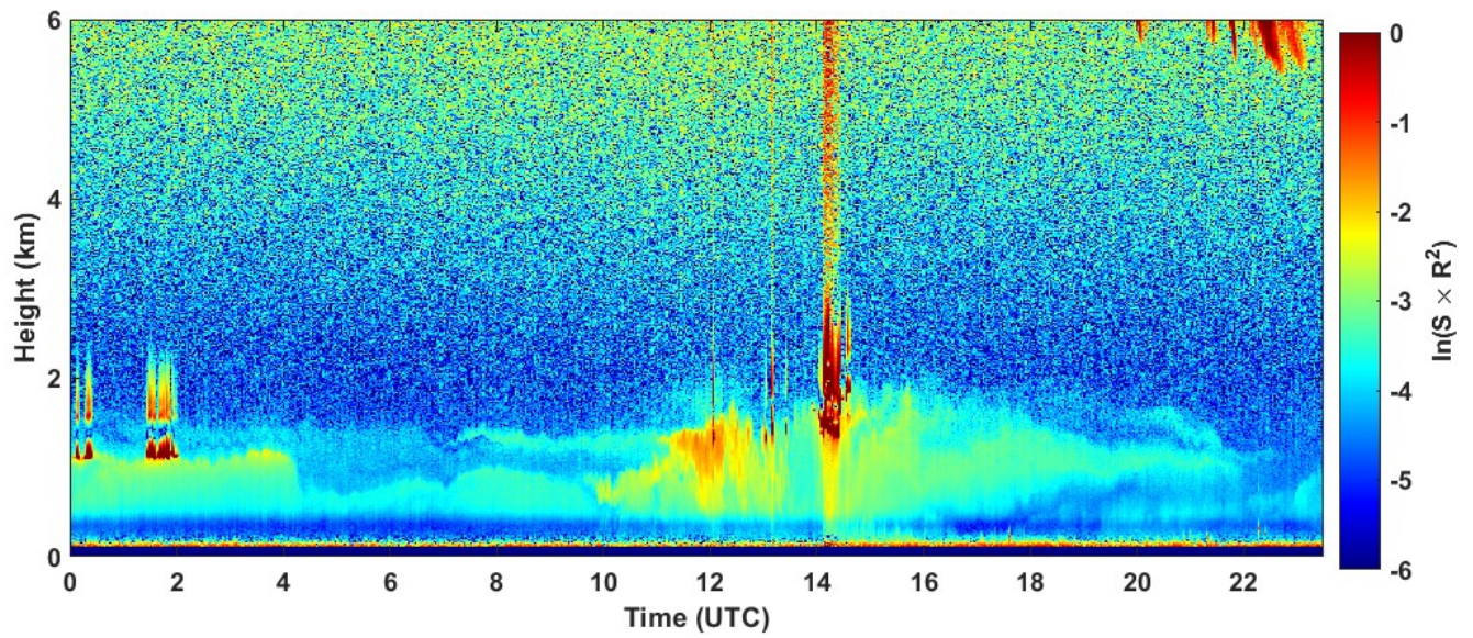
2023-01-24 RCS quick look CHM15k - ILVA LIDAR1 DIREZIONE
