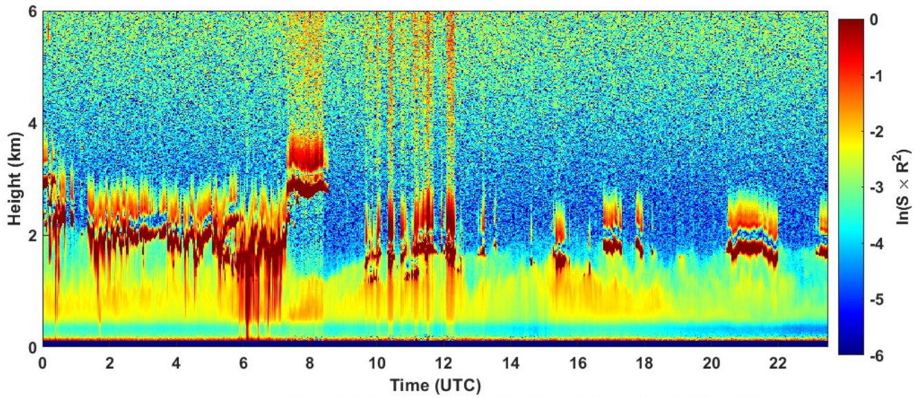
2023-01-12 RCS quick look CHM15k - ILVA LIDAR1 DIREZIONE
