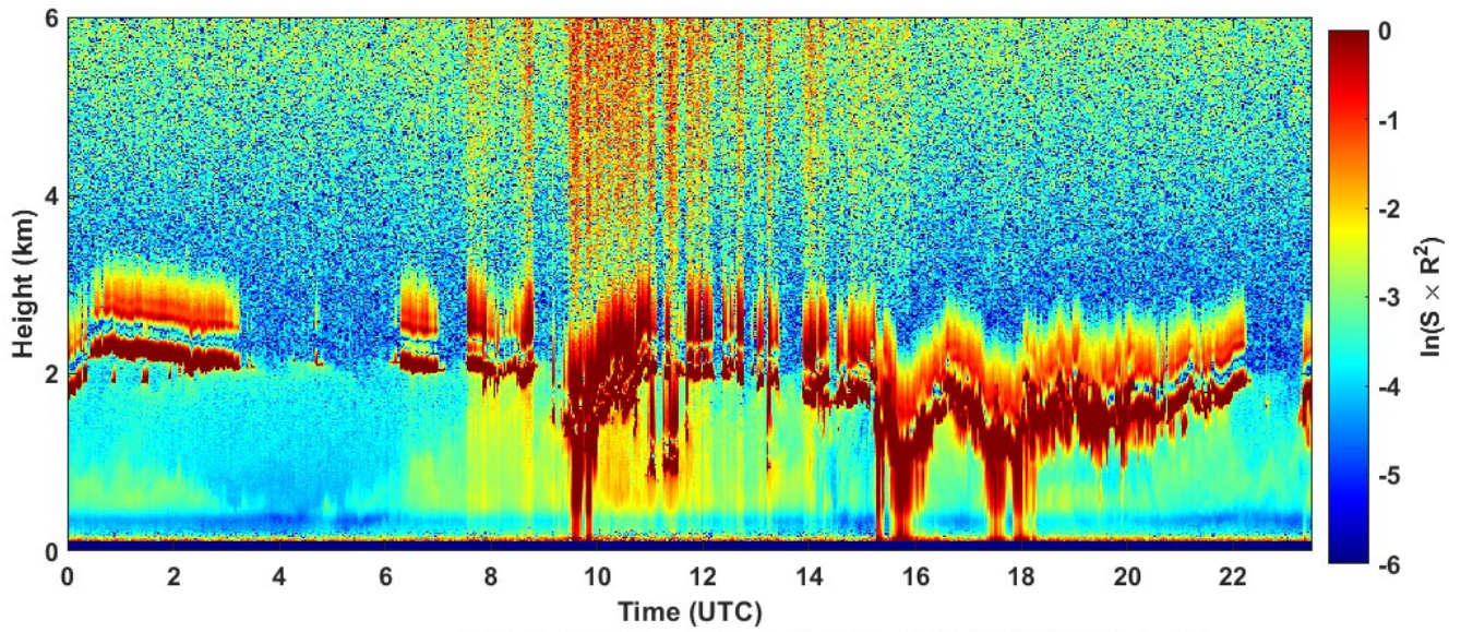
2023-01-30 RCS quick look CHM15k - ILVA LIDAR1 DIREZIONE
