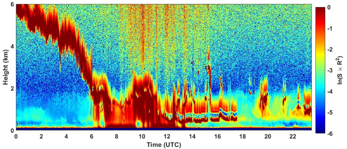
2023-01-26 RCS quick look CHM15k - ILVA LIDAR1 DIREZIONE
