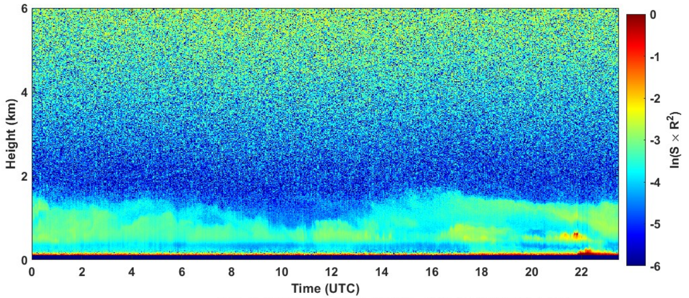
2023-01-06 RCS quick look CHM15k - ILVA LIDAR1 DIREZIONE
