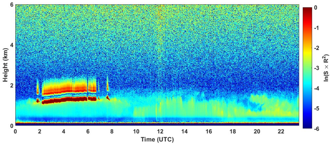
2023-01-04 RCS quick look CHM15k - ILVA LIDAR1 DIREZIONE
