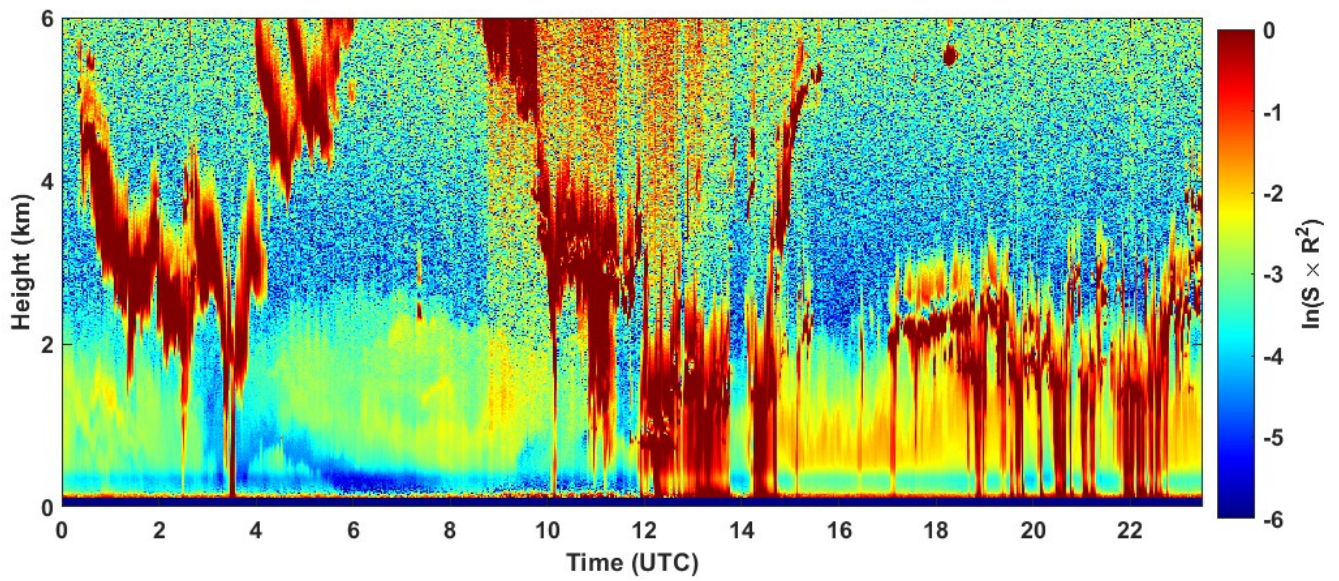
2023-01-10 RCS quick look CHM15k - ILVA LIDAR1 DIREZIONE
