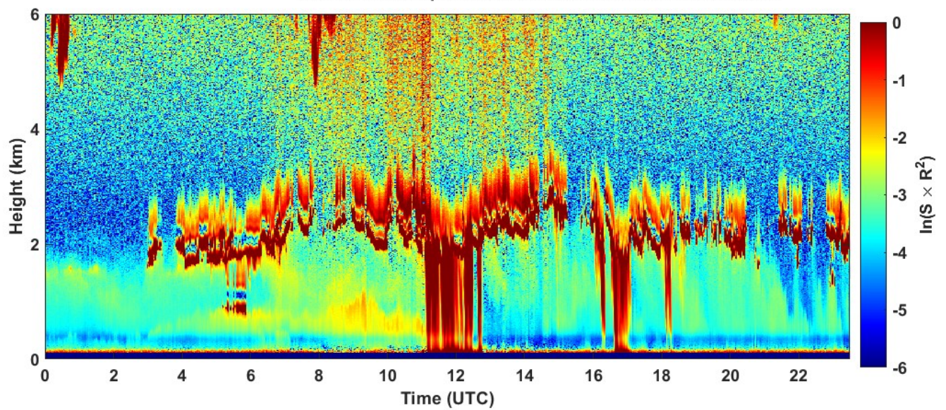
2023-01-16 RCS quick look CHM15k - ILVA LIDAR1 DIREZIONE
