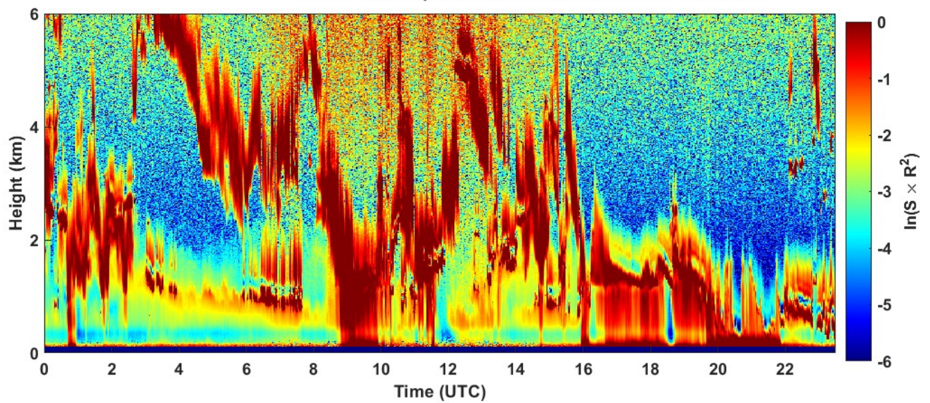
2023-01-22 RCS quick look CHM15k - ILVA LIDAR1 DIREZIONE
