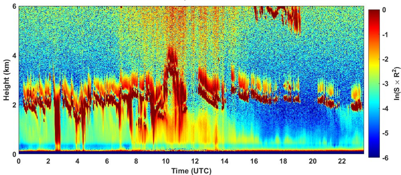
2023-01-18 RCS quick look CHM15k - ILVA LIDAR1 DIREZIONE
