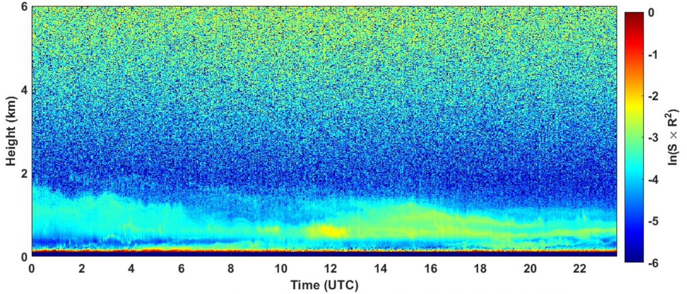
2023-01-02 RCS quick look CHM15k - ILVA LIDAR1 DIREZIONE
