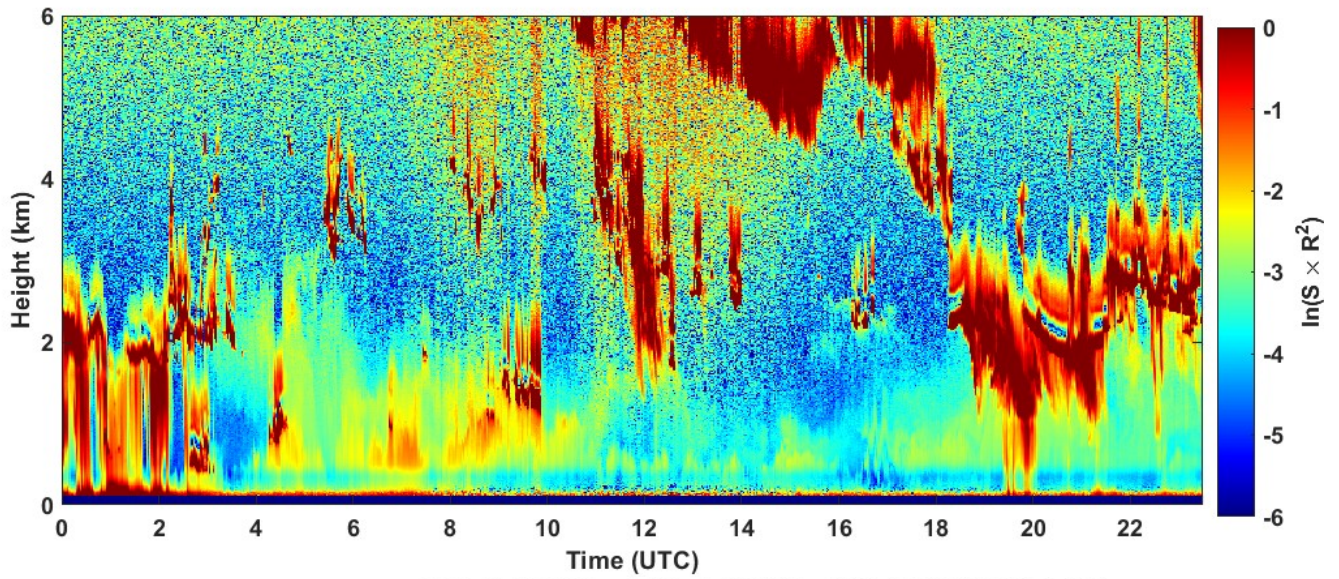
2023-01-20 RCS quick look CHM15k - ILVA LIDAR1 DIREZIONE
