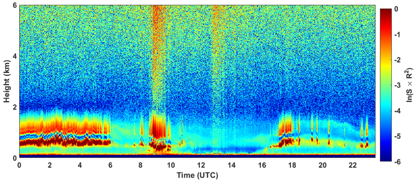
2022-12-30 RCS quick look CHM15k - ILVA LIDAR1 DIREZIONE
