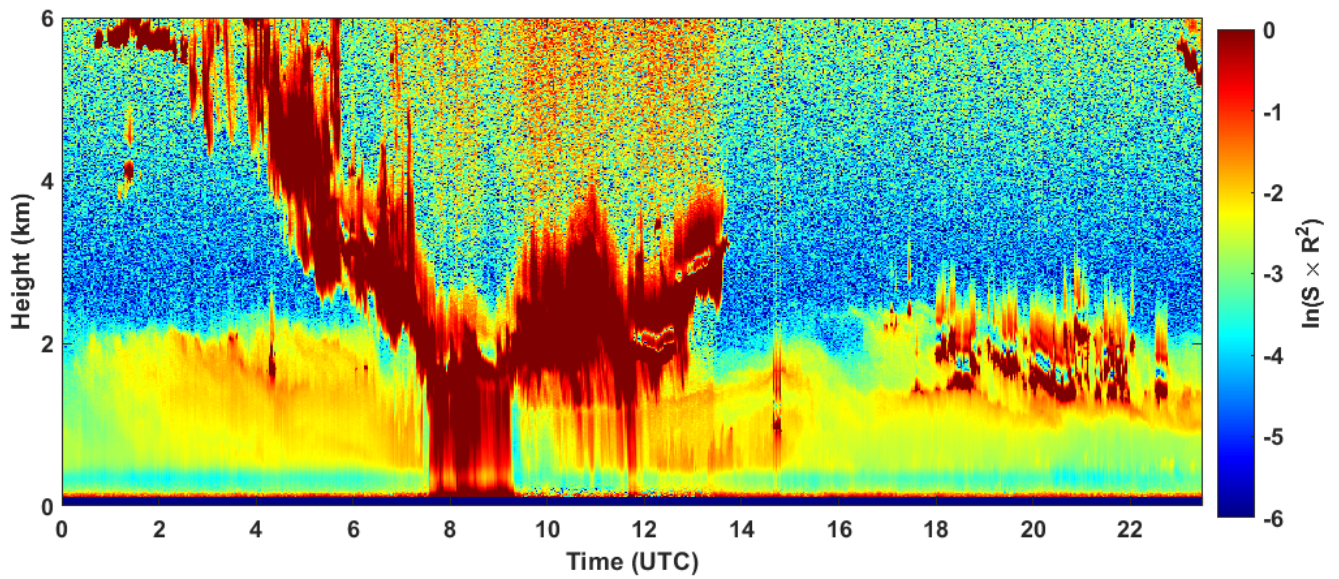
2022-12-12 RCS quick look CHM15k - ILVA LIDAR1 DIREZIONE
