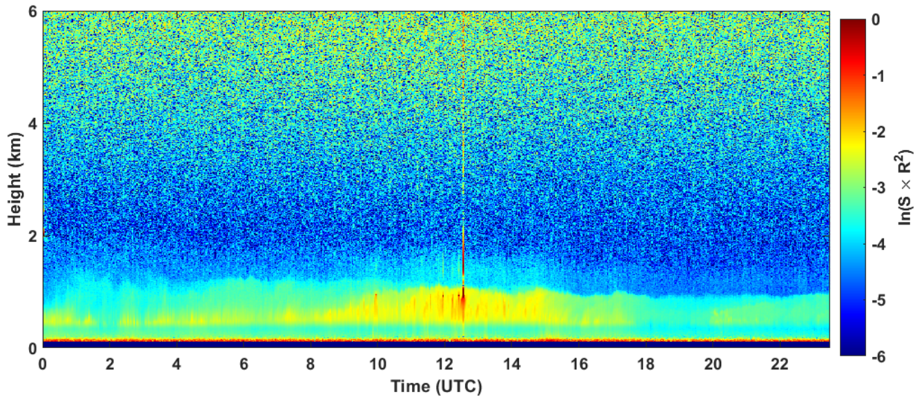
2022-12-20 RCS quick look CHM15k - ILVA LIDAR1 DIREZIONE
