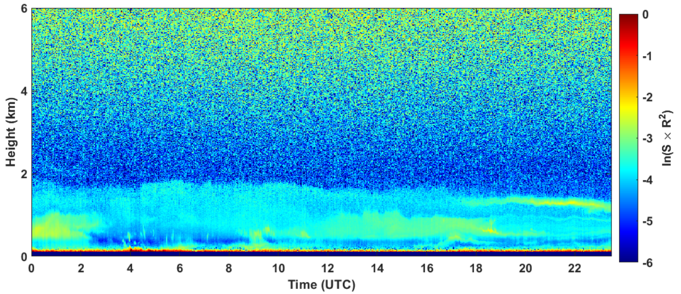
2022-12-26 RCS quick look CHM15k - ILVA LIDAR1 DIREZIONE
