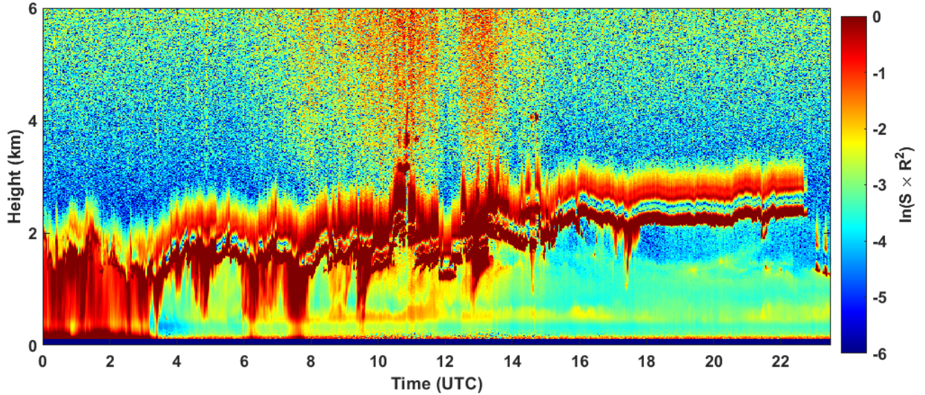
2022-12-02 RCS quick look CHM15k - ILVA LIDAR1 DIREZIONE
