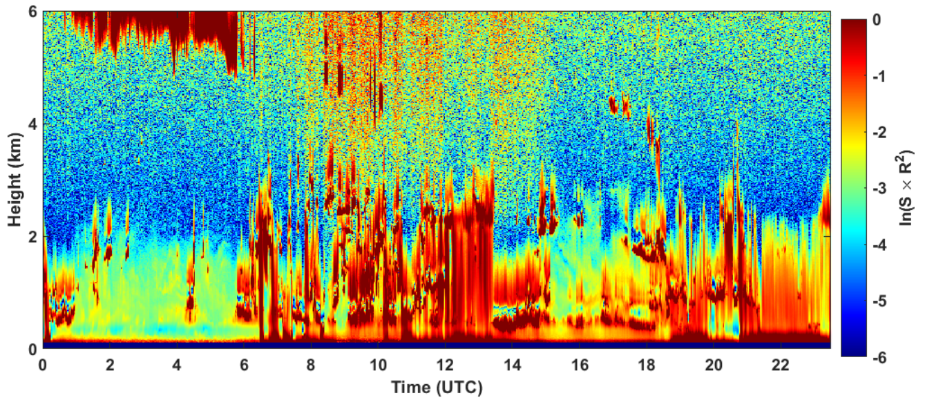
2022-12-04 RCS quick look CHM15k - ILVA LIDAR1 DIREZIONE
