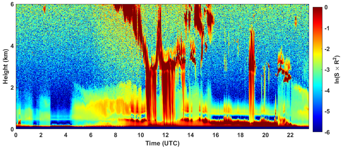
2022-12-10 RCS quick look CHM15k - ILVA LIDAR1 DIREZIONE
