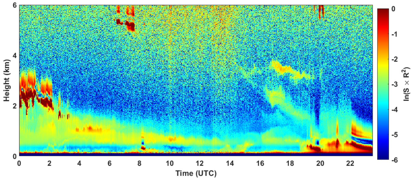
2022-12-16 RCS quick look CHM15k - ILVA LIDAR1 DIREZIONE
