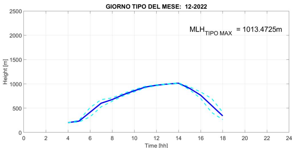
Fig. 2: Giorno tipo del parametro Mixing Layer Height nel mese di DICEMBRE 2022, rappresentato mediante media oraria (linea blu continua) e deviazione standard (linee celesti tratteggiate).
