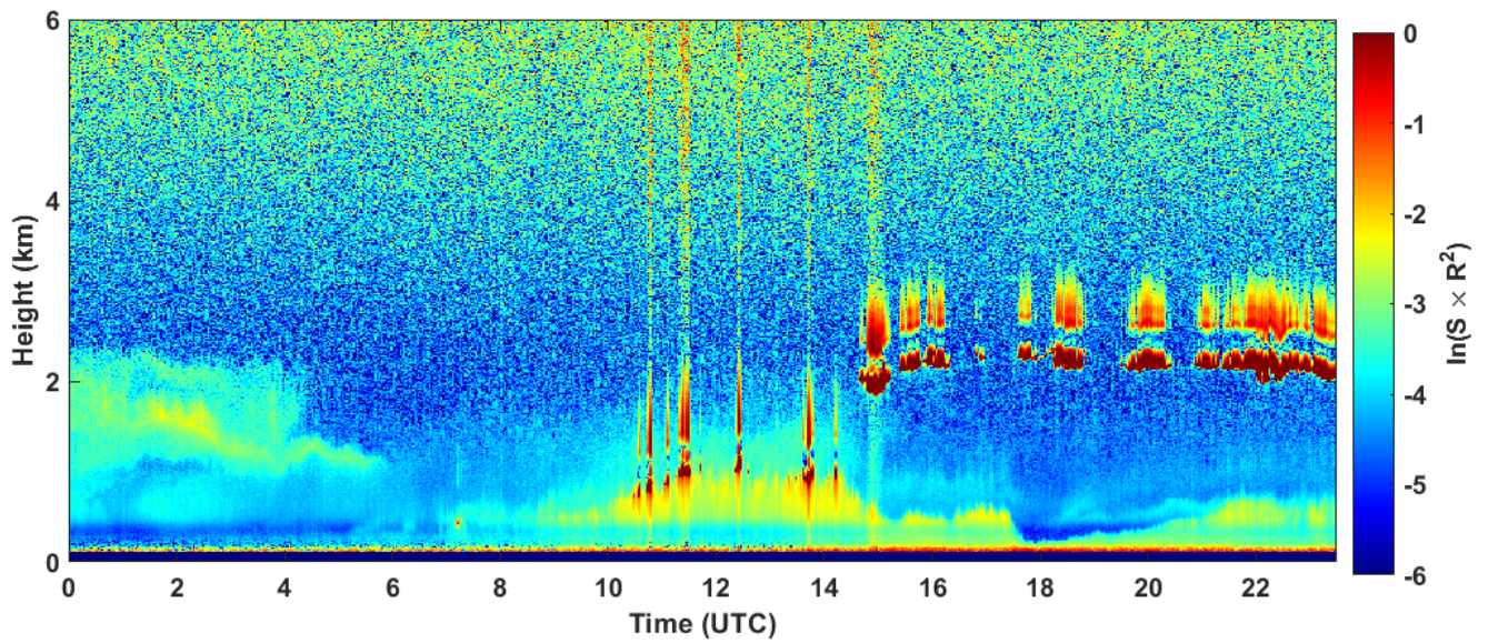
2022-12-18 RCS quick look CHM15k - ILVA LIDAR1 DIREZIONE
