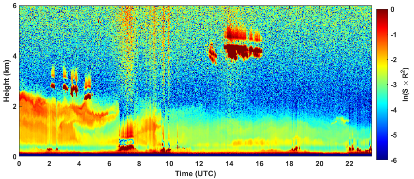
2022-12-08 RCS quick look CHM15k - ILVA LIDAR1 DIREZIONE
