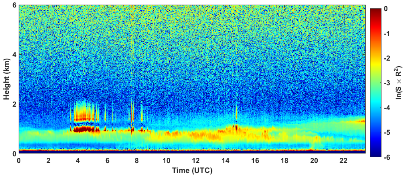
2022-12-22 RCS quick look CHM15k - ILVA LIDAR1 DIREZIONE
