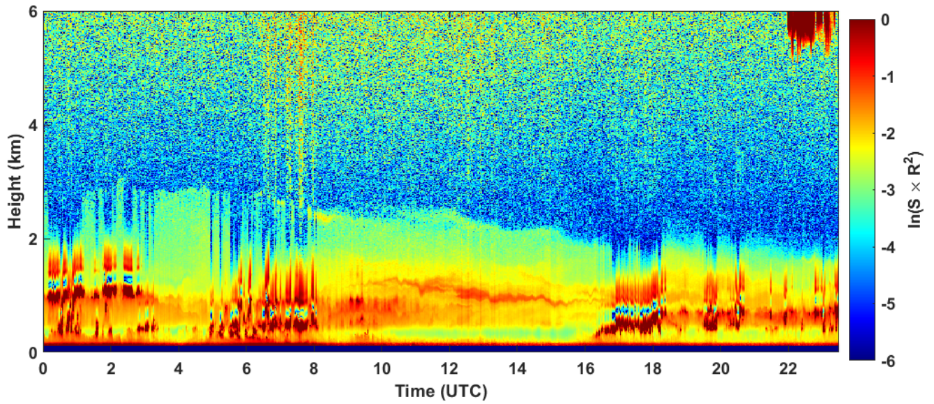
2022-12-06 RCS quick look CHM15k - ILVA LIDAR1 DIREZIONE
