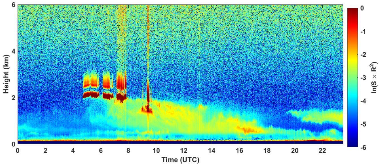
2022-12-24 RCS quick look CHM15k - ILVA LIDAR1 DIREZIONE
