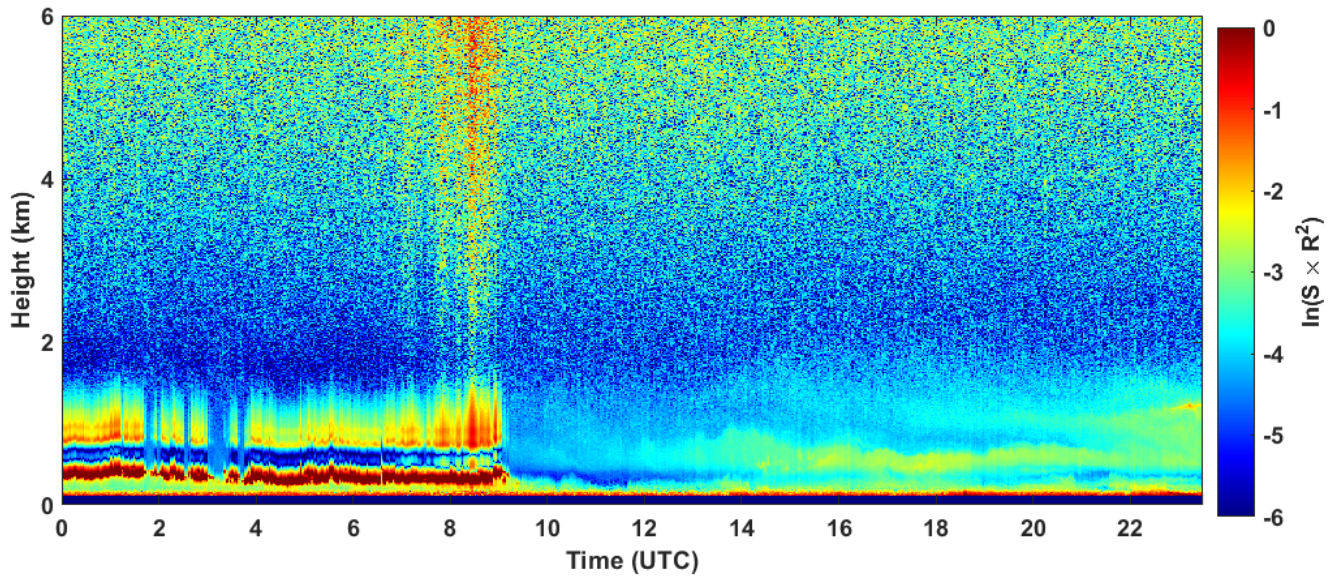
2022-12-28 RCS quick look CHM15k - ILVA LIDAR1 DIREZIONE
