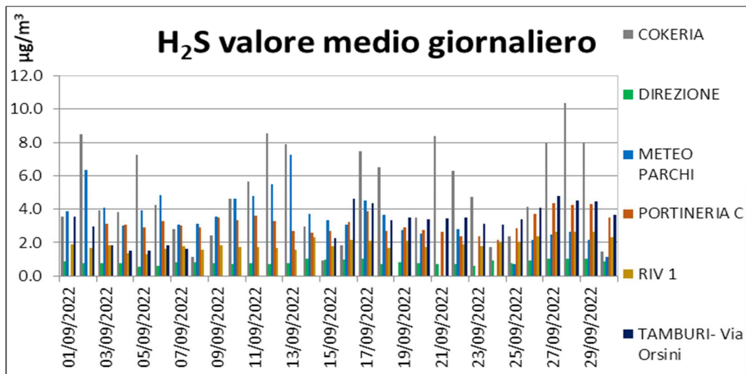
Figura 2 Livelli medi giornalieri di concentrazione di H 2 S in µg/m 3 Settembre 2022 (Rete AdI con Cokeria)
