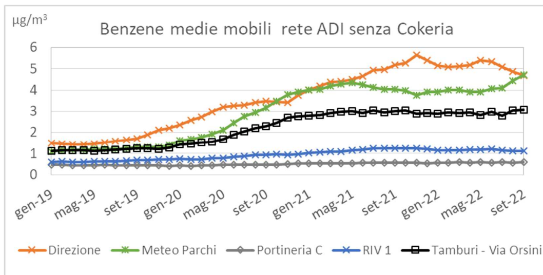
Figura 30 Medie mobili mensili di concentrazione di Benzene in \mu\text{g}/\text{m}^3
