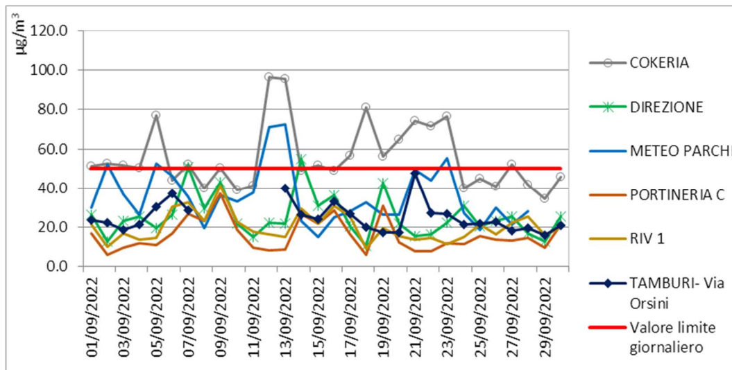
Figura 9 Livelli di concentrazione Settembre 2022 di PM 10 (SWAM) in µg/m 3
