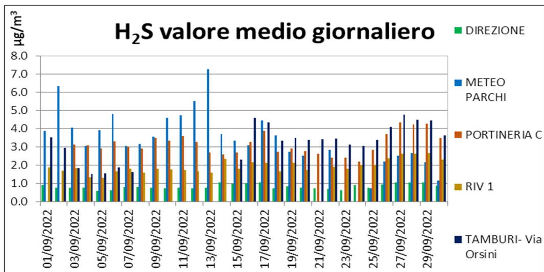
Figura 3 Livelli medi giornalieri di concentrazione di H 2 S in µg/m 3 Settembre 2022 (Rete AdI senza Cokeria)
