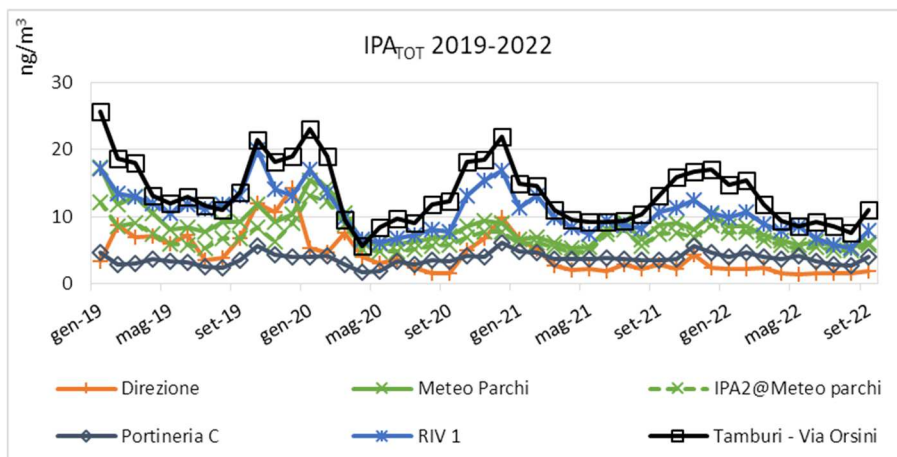
Figura 35 Livelli medi mensili di concentrazione di IPA TOT 2019 ÷ 2022 in ng/m 3 (Rete ADI senza Cokeria)
