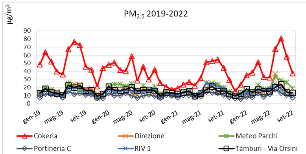
Figura 20 Livelli medi mensili di concentrazione di PM 2.5 2019÷2022 in µg/m 3 (Rete ADI con Cokeria)
