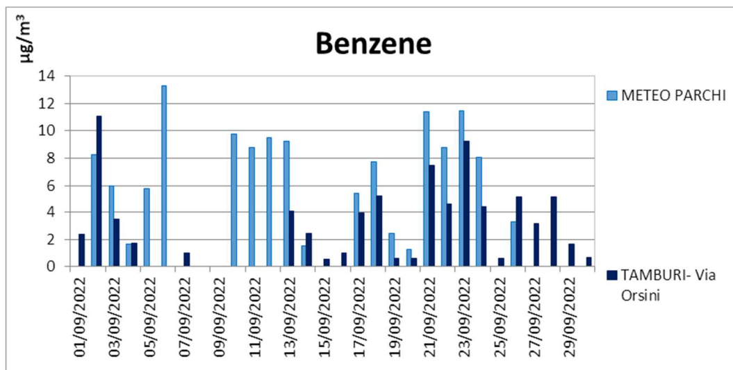
Figura 24a Confronto livelli di concentrazione di Benzene in \mu\text{g}/\text{m}^3 Tamburi - Via Orsini vs Meteo Parchi
