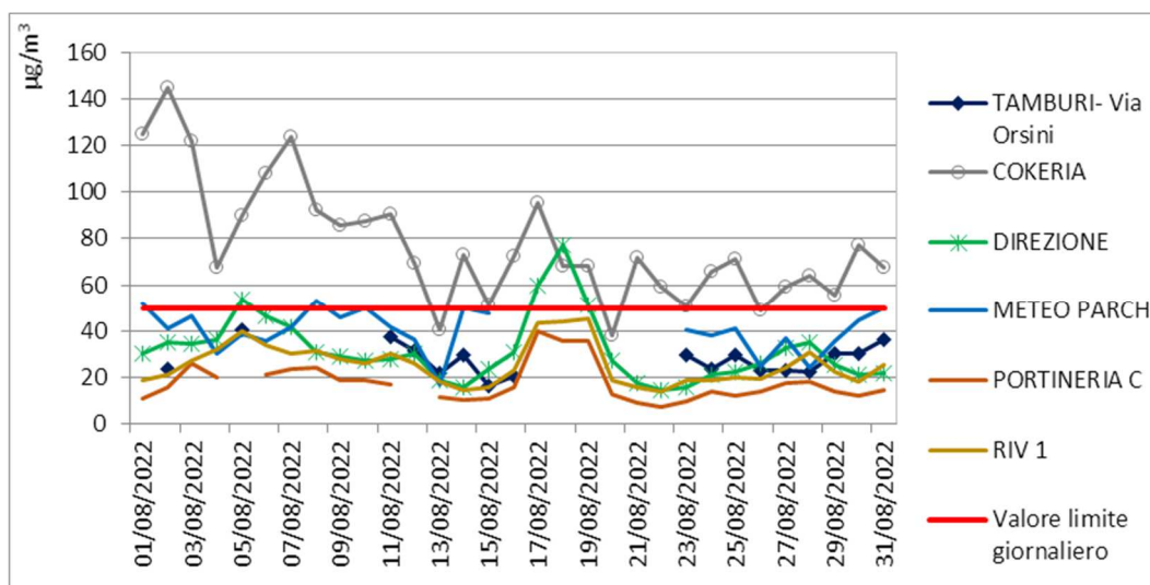
Figura 10 Livelli di concentrazione Agosto 2022 di PM 10 (SWAM) in µg/m 3
