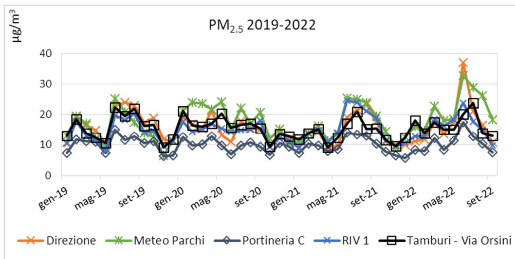
Figura 21 Livelli medi mensili di concentrazione di PM 2.5 2019÷2022 in µg/m 3 (Rete ADI senza Cokeria)
