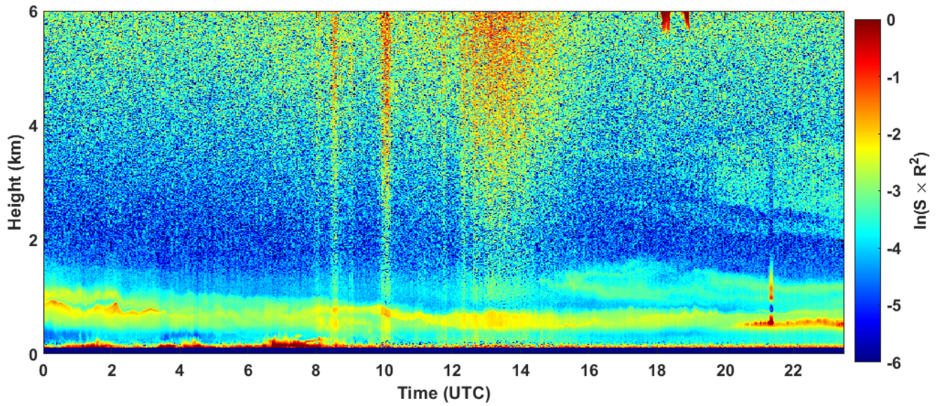
2022-10-22 RCS quick look CHM15k - ILVA LIDAR1 DIREZIONE
