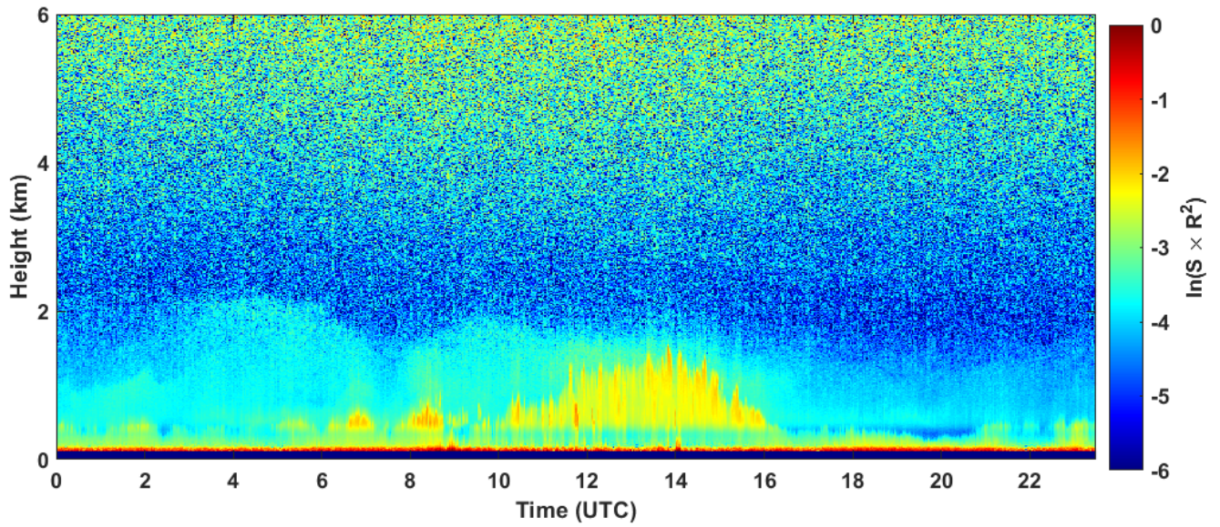
2022-10-30 RCS quick look CHM15k - ILVA LIDAR1 DIREZIONE
