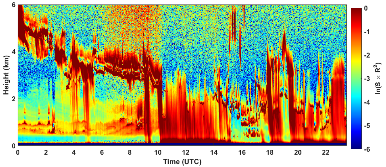
2022-10-14 RCS quick look CHM15k - ILVA LIDAR1 DIREZIONE
