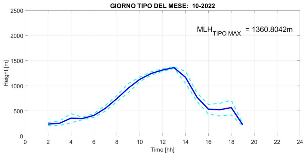
Fig. 2: Giorno tipo del parametro Mixing Layer Height nel mese di OTTOBRE 2022, rappresentato mediante media oraria (linea blu continua) e deviazione standard (linee celesti tratteggiate).
