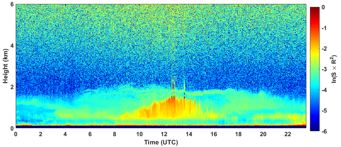
2022-10-18 RCS quick look CHM15k - ILVA LIDAR1 DIREZIONE
