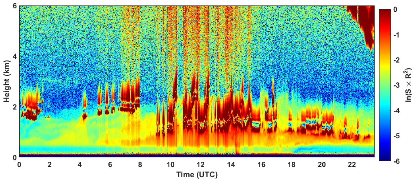
2022-10-12 RCS quick look CHM15k - ILVA LIDAR1 DIREZIONE
