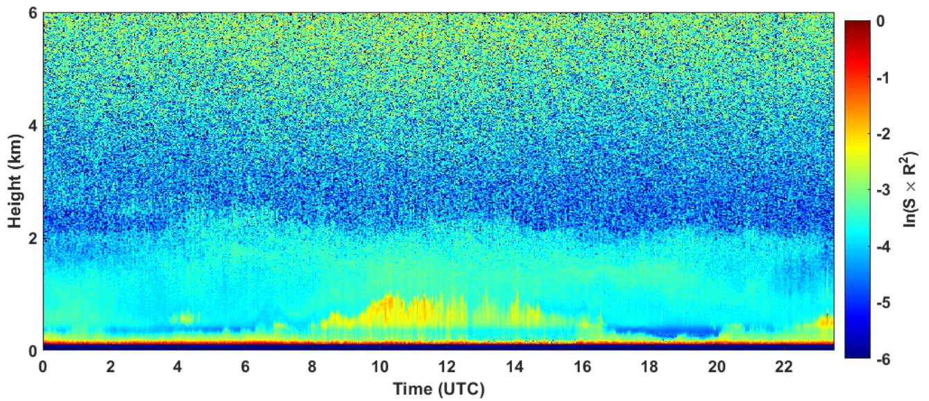
2022-10-28 RCS quick look CHM15k - ILVA LIDAR1 DIREZIONE
