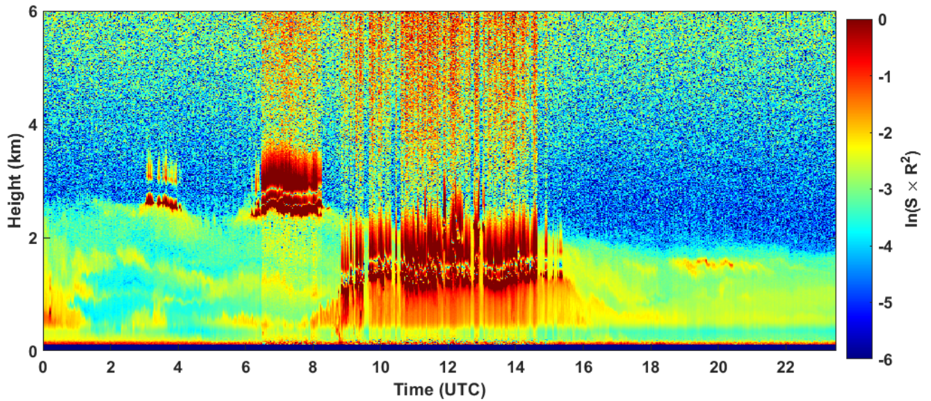
2022-10-16 RCS quick look CHM15k - ILVA LIDAR1 DIREZIONE
