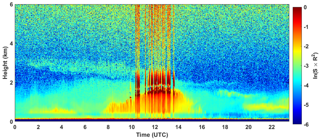
2022-10-20 RCS quick look CHM15k - ILVA LIDAR1 DIREZIONE
