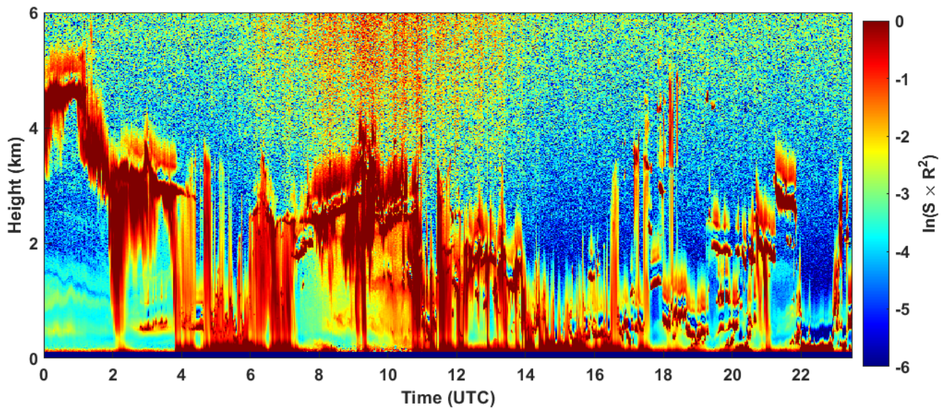
2022-10-10 RCS quick look CHM15k - ILVA LIDAR1 DIREZIONE
