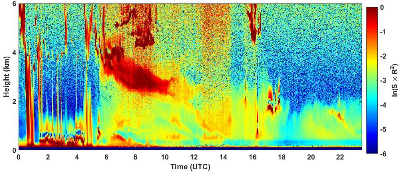
2022-10-02 RCS quick look CHM15k - ILVA LIDAR1 DIREZIONE
