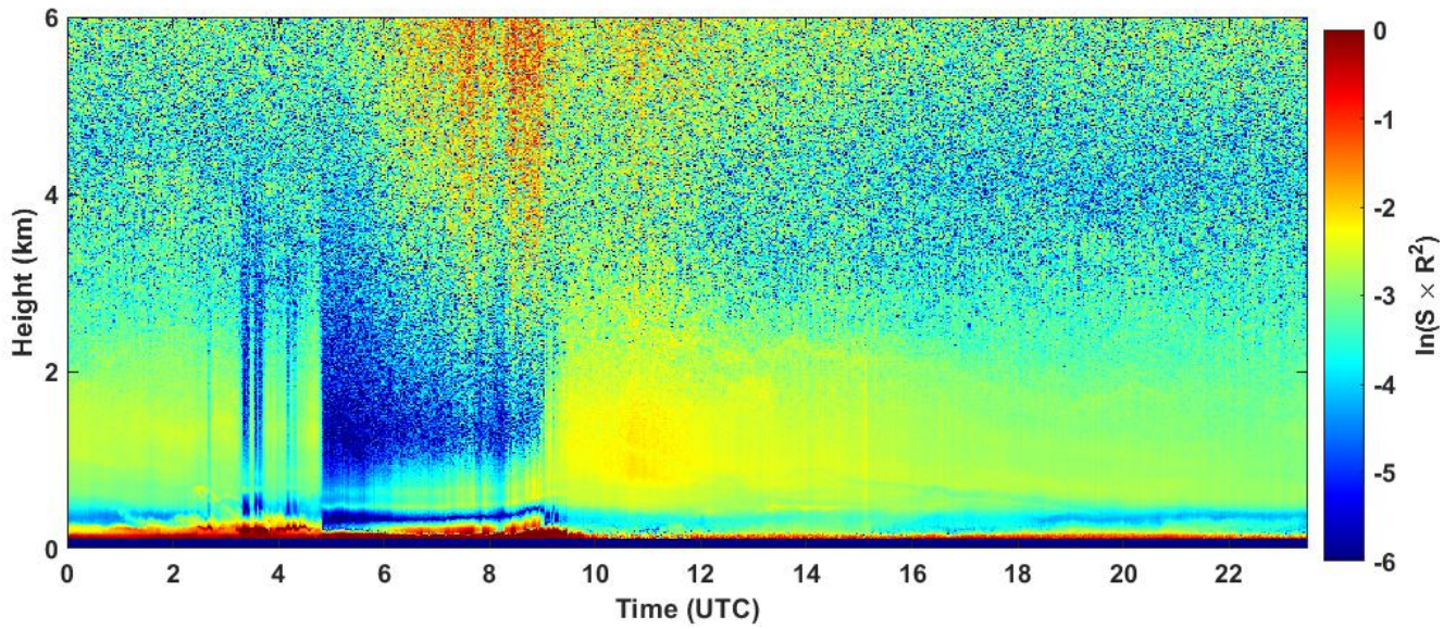
2022-10-24 RCS quick look CHM15k - ILVA LIDAR1 DIREZIONE
