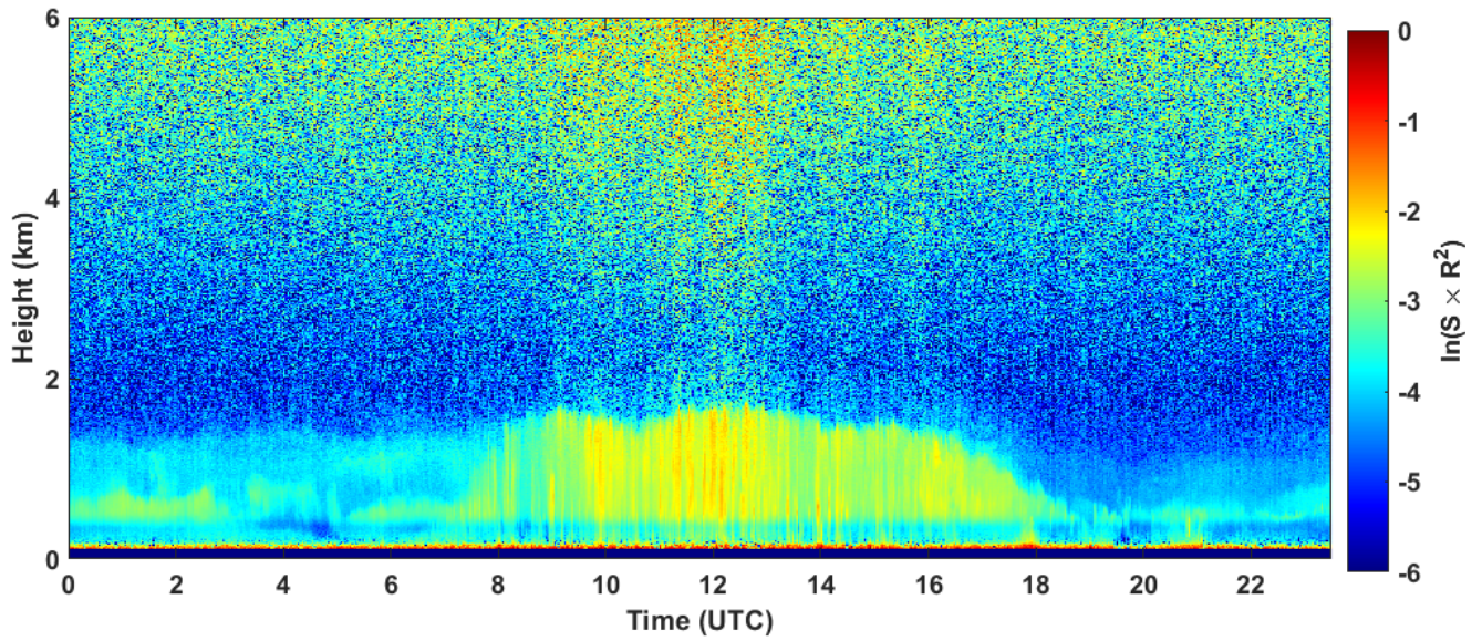
2022-10-06 RCS quick look CHM15k - ILVA LIDAR1 DIREZIONE
