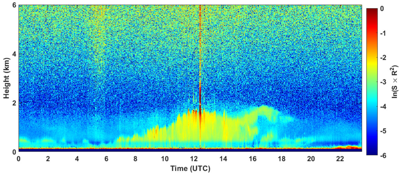
2022-10-08 RCS quick look CHM15k - ILVA LIDAR1 DIREZIONE
