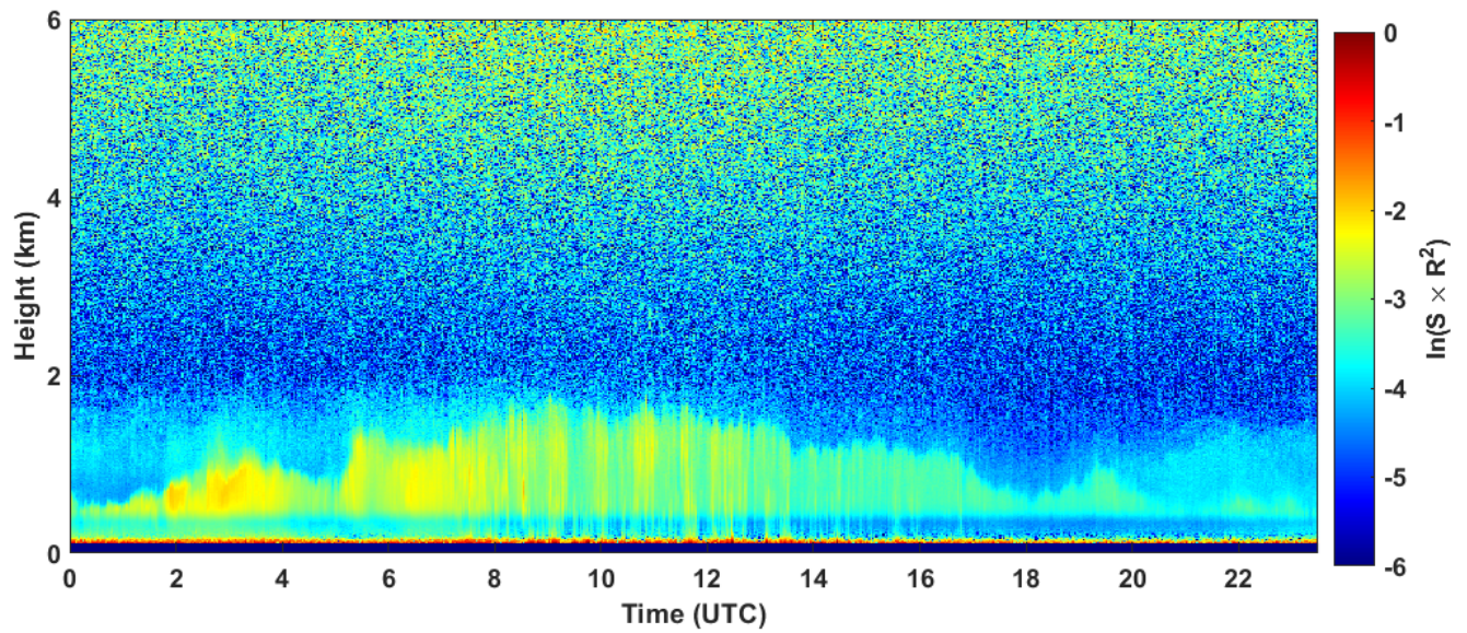
2022-10-04 RCS quick look CHM15k - ILVA LIDAR1 DIREZIONE
