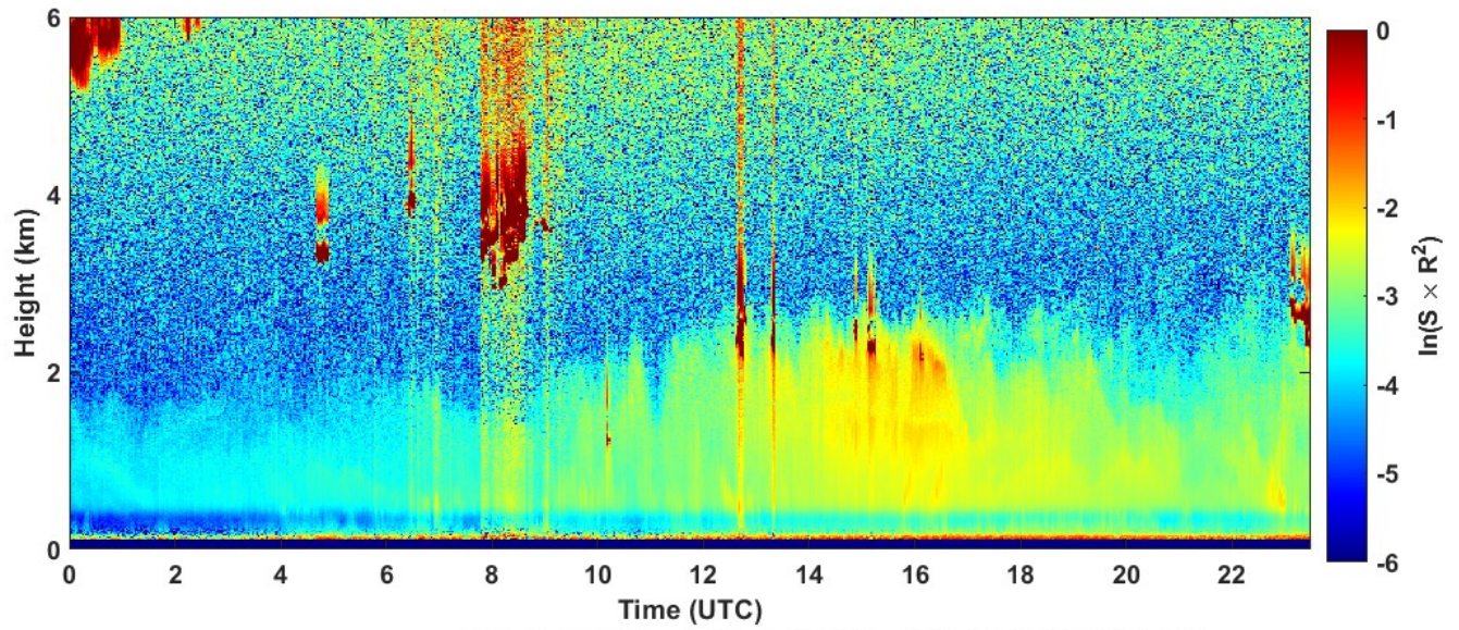
2022-09-28 RCS quick look CHM15k - ILVA LIDAR1 DIREZIONE
