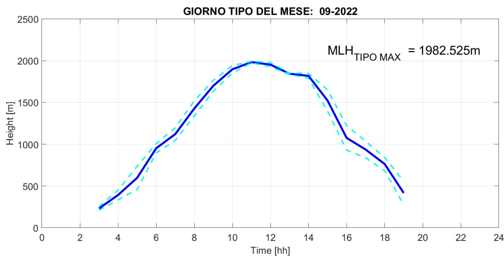
Fig. 2: Giorno tipo del parametro Mixing Layer Height nel mese di SETTEMBRE 2022, rappresentato mediante media oraria (linea blu continua) e deviazione standard (linee celesti tratteggiate).
