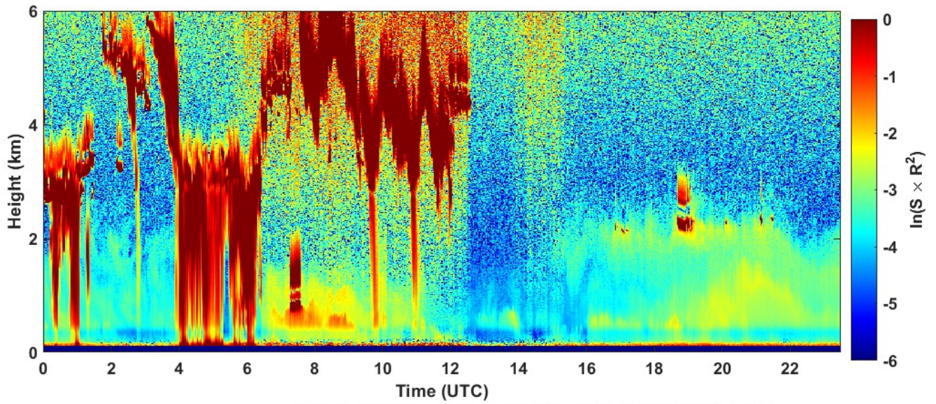
2022-09-30 RCS quick look CHM15k - ILVA LIDAR1 DIREZIONE
