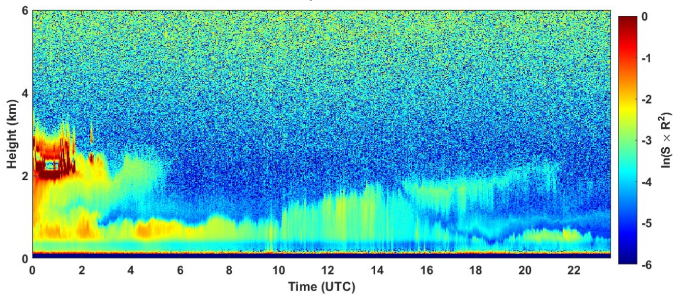
2022-09-18 RCS quick look CHM15k - ILVA LIDAR1 DIREZIONE
