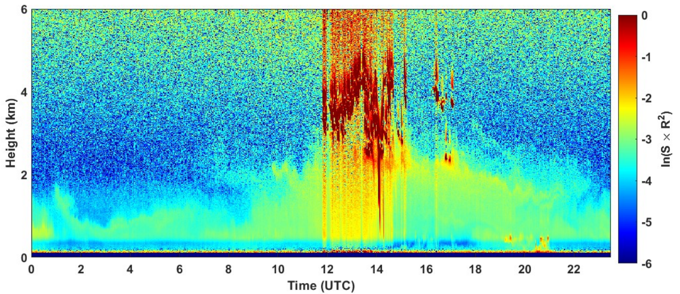
2022-09-10 RCS quick look CHM15k - ILVA LIDAR1 DIREZIONE
