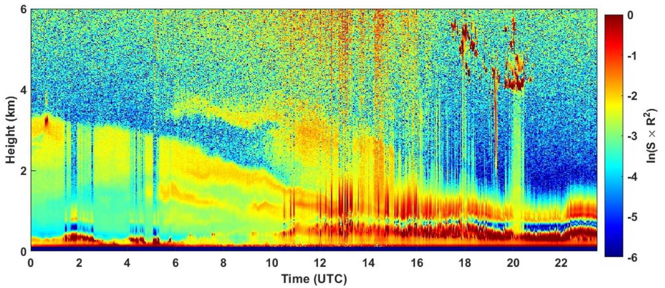
2022-09-08 RCS quick look CHM15k - ILVA LIDAR1 DIREZIONE
