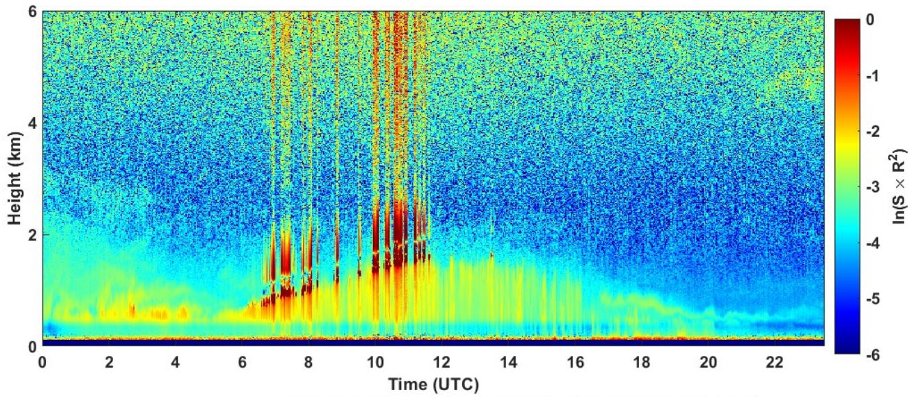
2022-09-06 RCS quick look CHM15k - ILVA LIDAR1 DIREZIONE
