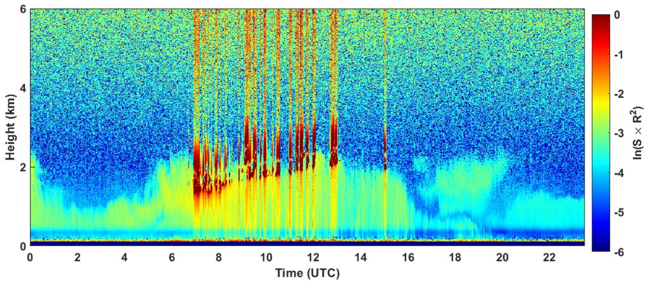
2022-09-22 RCS quick look CHM15k - ILVA LIDAR1 DIREZIONE
