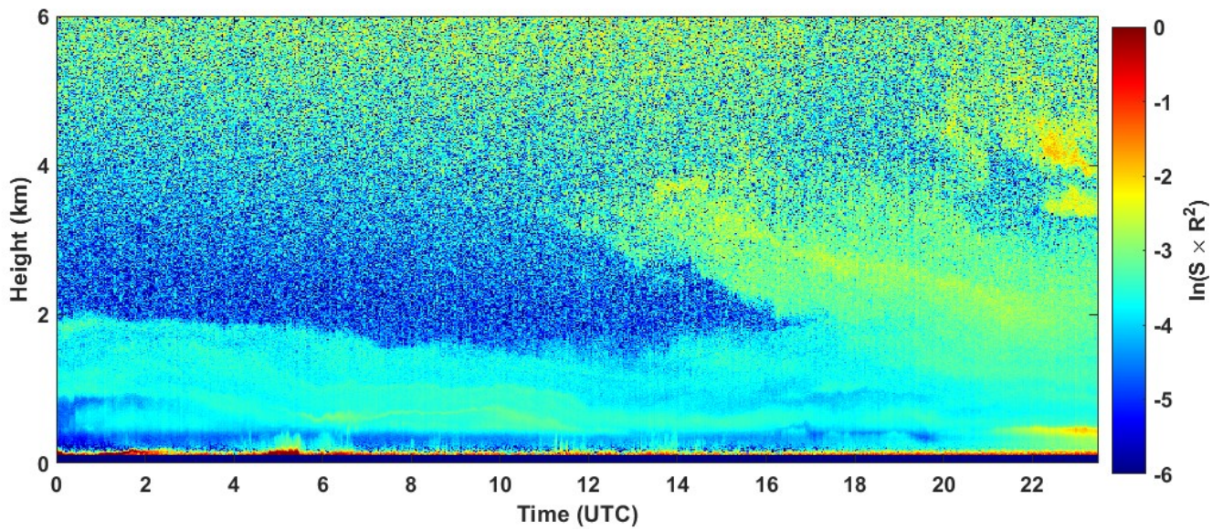
2022-09-14 RCS quick look CHM15k - ILVA LIDAR1 DIREZIONE
