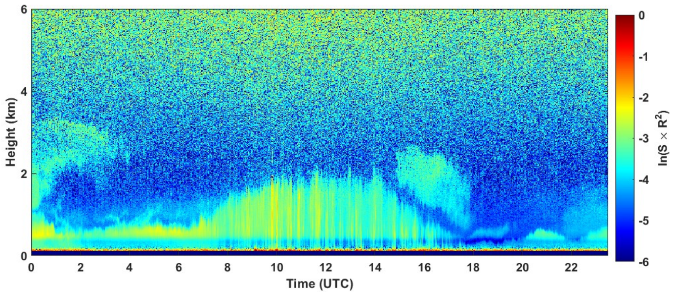
2022-09-12 RCS quick look CHM15k - ILVA LIDAR1 DIREZIONE
