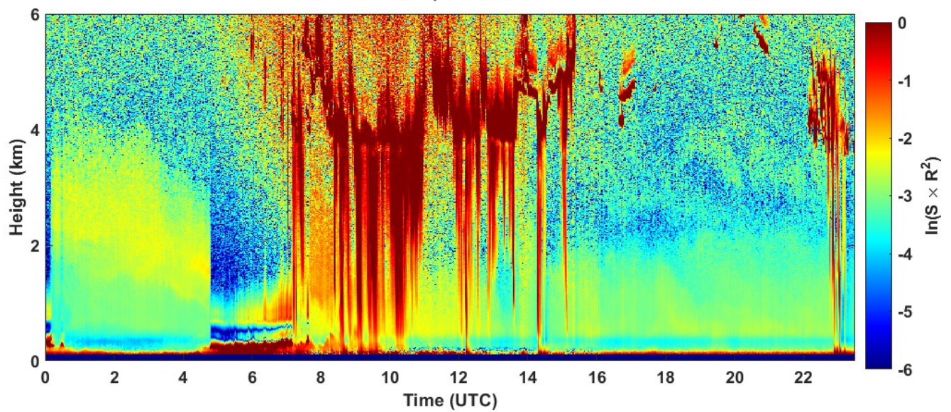
2022-09-16 RCS quick look CHM15k - ILVA LIDAR1 DIREZIONE
