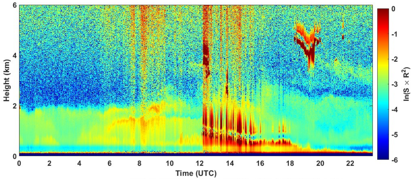
2022-09-26 RCS quick look CHM15k - ILVA LIDAR1 DIREZIONE
