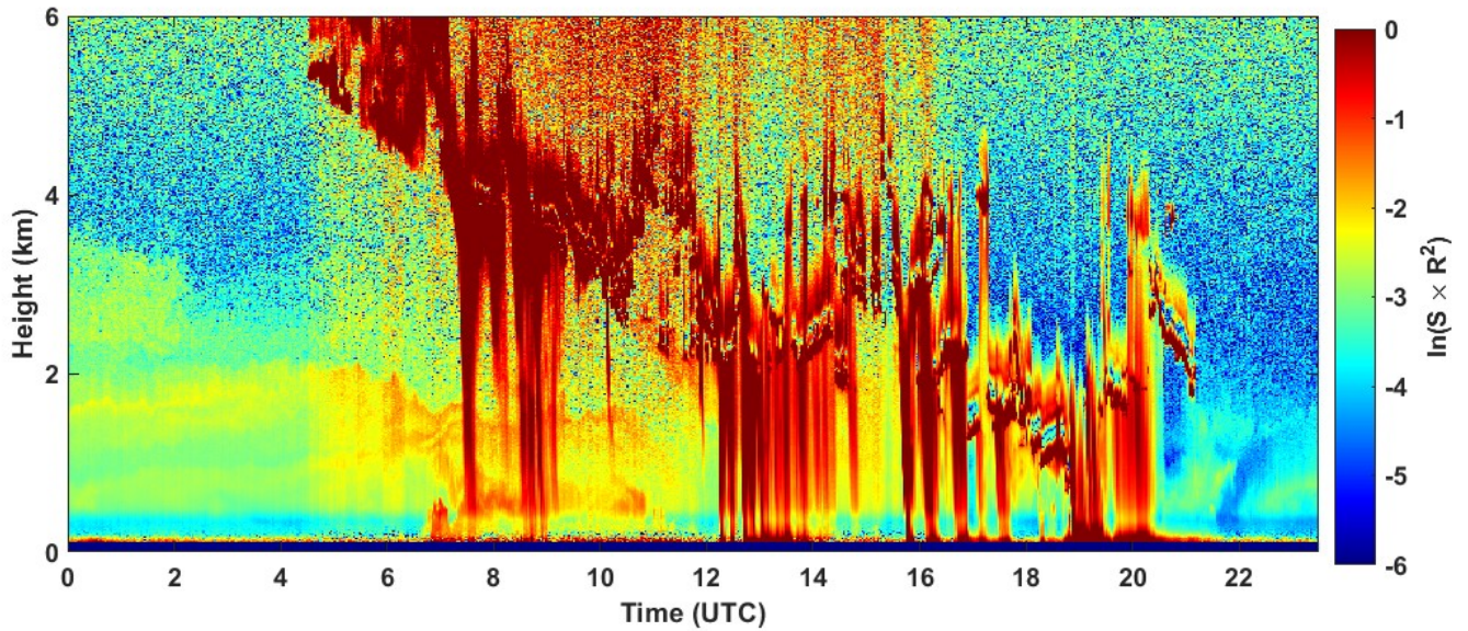
2022-09-02 RCS quick look CHM15k - ILVA LIDAR1 DIREZIONE
