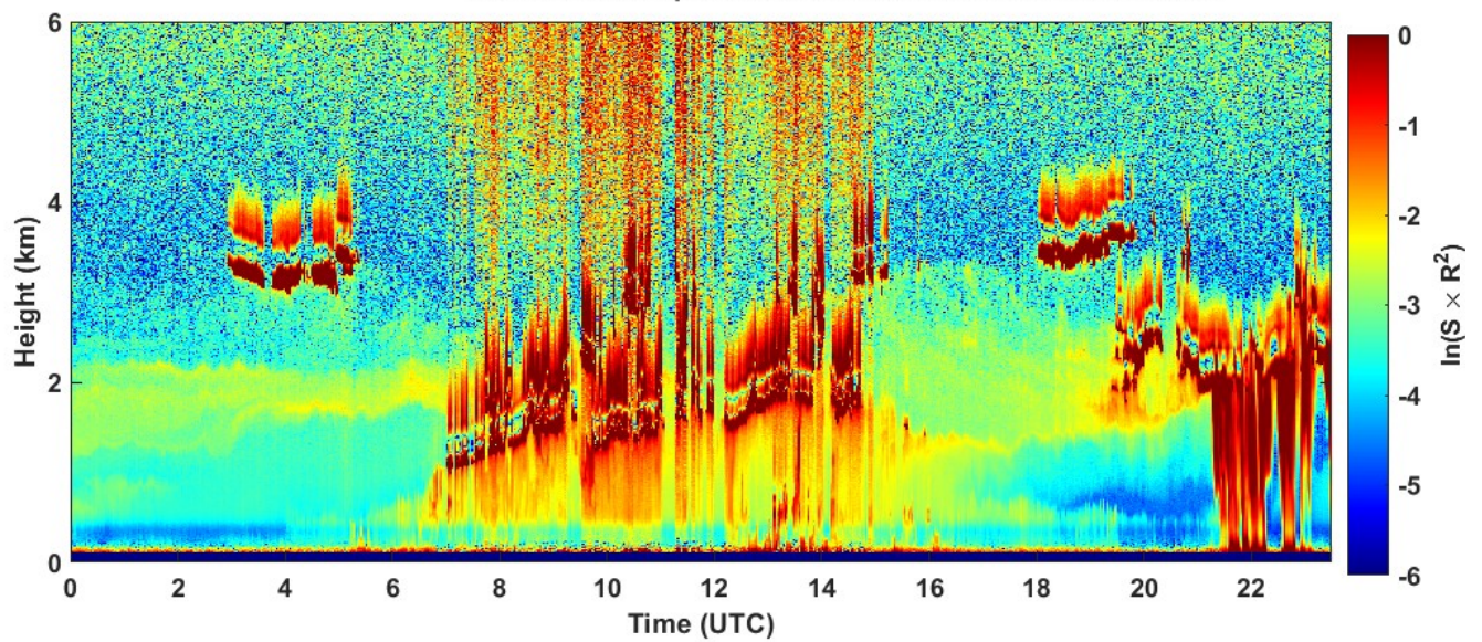
2022-09-20 RCS quick look CHM15k - ILVA LIDAR1 DIREZIONE
