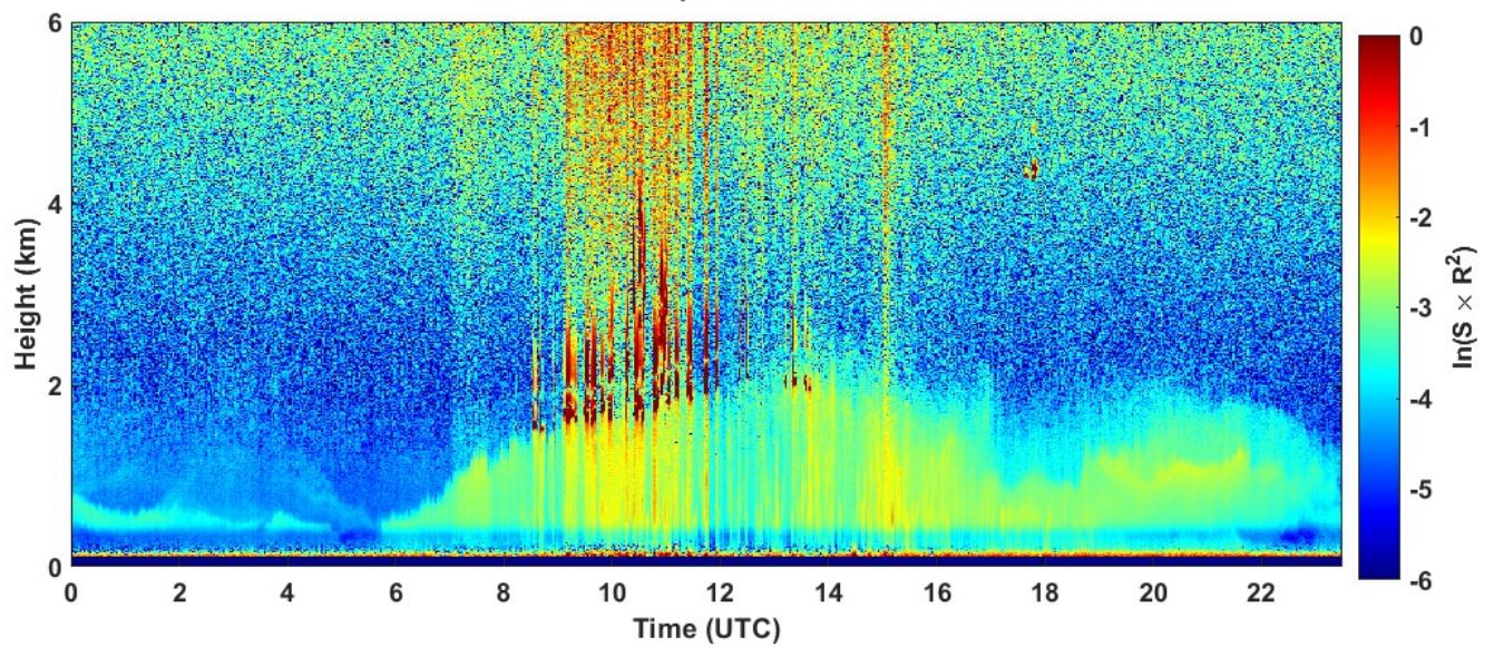
2022-08-22 RCS quick look CHM15k - ILVA LIDAR1 DIREZIONE
