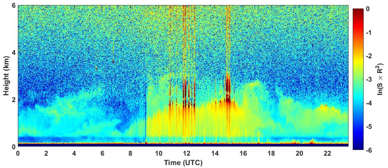
2022-08-30 RCS quick look CHM15k - ILVA LIDAR1 DIREZIONE
