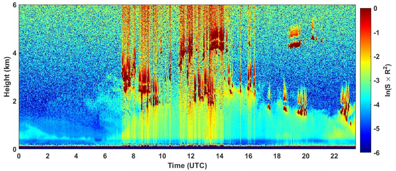
2022-08-24 RCS quick look CHM15k - ILVA LIDAR1 DIREZIONE
