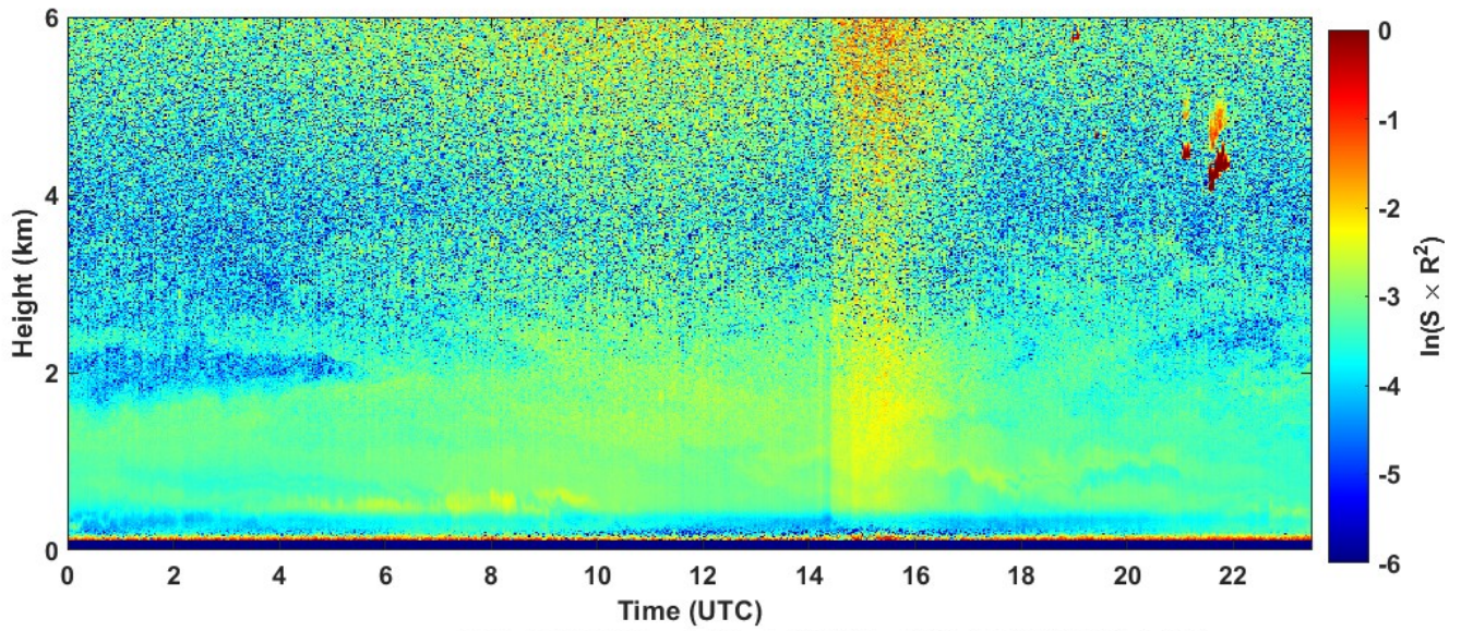
2022-08-28 RCS quick look CHM15k - ILVA LIDAR1 DIREZIONE
