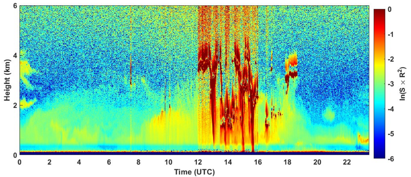
2022-08-20 RCS quick look CHM15k - ILVA LIDAR1 DIREZIONE
