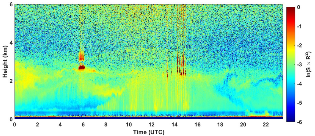
2022-08-26 RCS quick look CHM15k - ILVA LIDAR1 DIREZIONE
