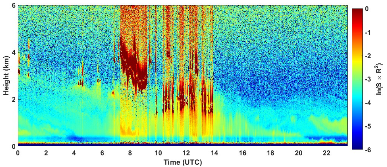
2022-08-14 RCS quick look CHM15k - ILVA LIDAR1 DIREZIONE
