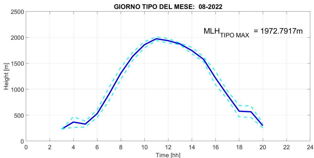
Fig. 2: Giorno tipo del parametro Mixing Layer Height nel mese di AGOSTO 2022, rappresentato mediante media oraria (linea blu continua) e deviazione standard (linee celesti tratteggiate).
