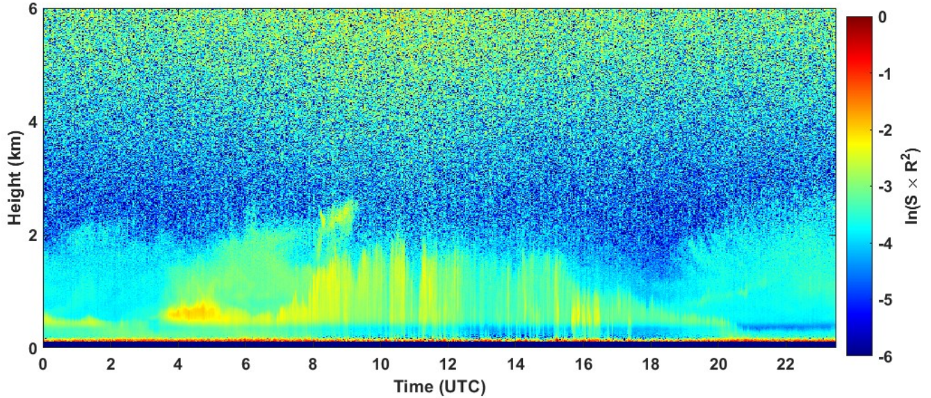
2022-08-02 RCS quick look CHM15k - ILVA LIDAR1 DIREZIONE
