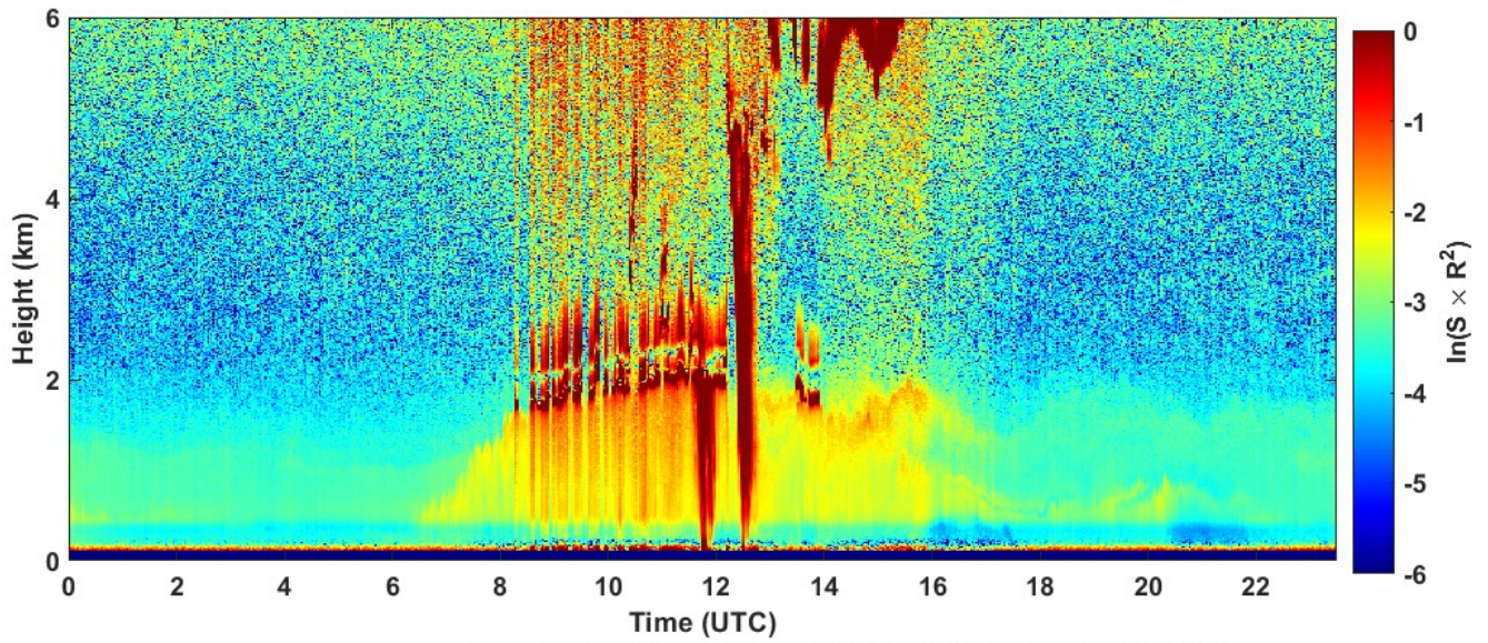
2022-08-10 RCS quick look CHM15k - ILVA LIDAR1 DIREZIONE
