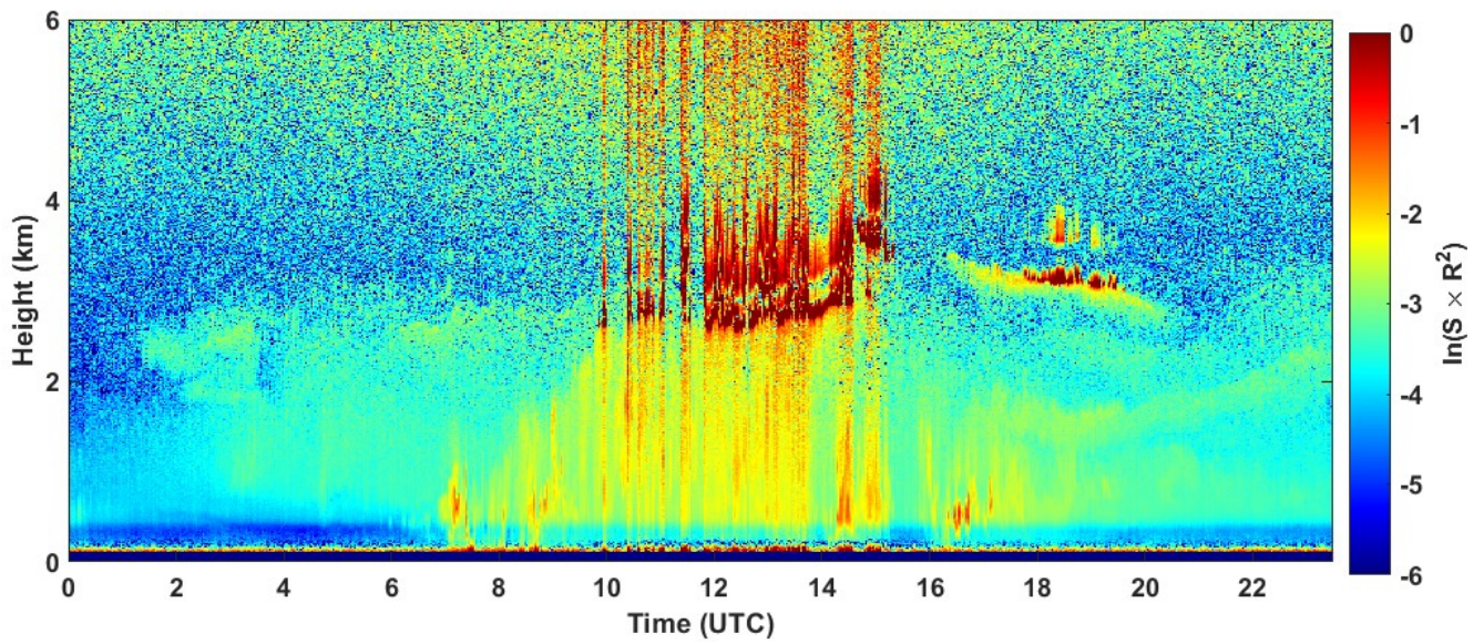
2022-08-04 RCS quick look CHM15k - ILVA LIDAR1 DIREZIONE
