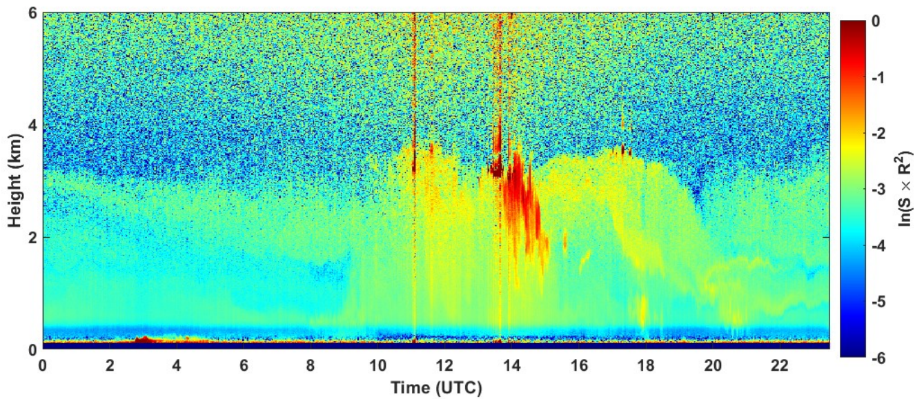
2022-08-06 RCS quick look CHM15k - ILVA LIDAR1 DIREZIONE
