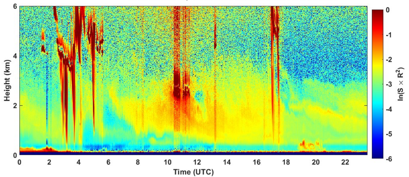
2022-08-16 RCS quick look CHM15k - ILVA LIDAR1 DIREZIONE
