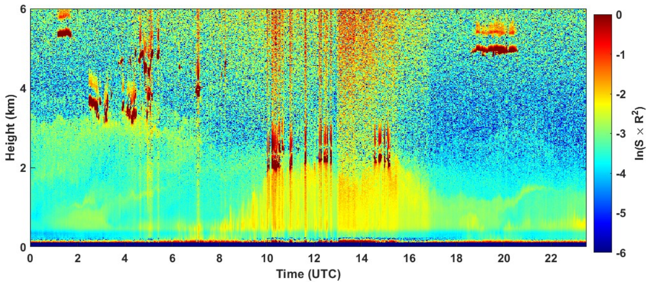
2022-08-08 RCS quick look CHM15k - ILVA LIDAR1 DIREZIONE
