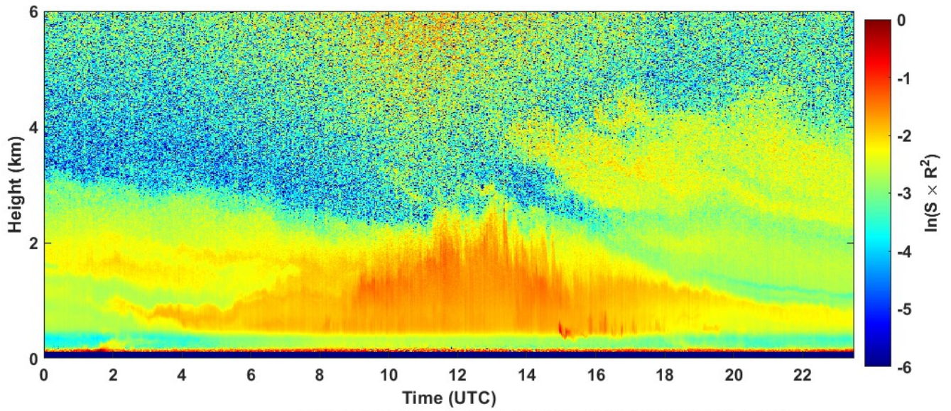
2022-08-18 RCS quick look CHM15k - ILVA LIDAR1 DIREZIONE
