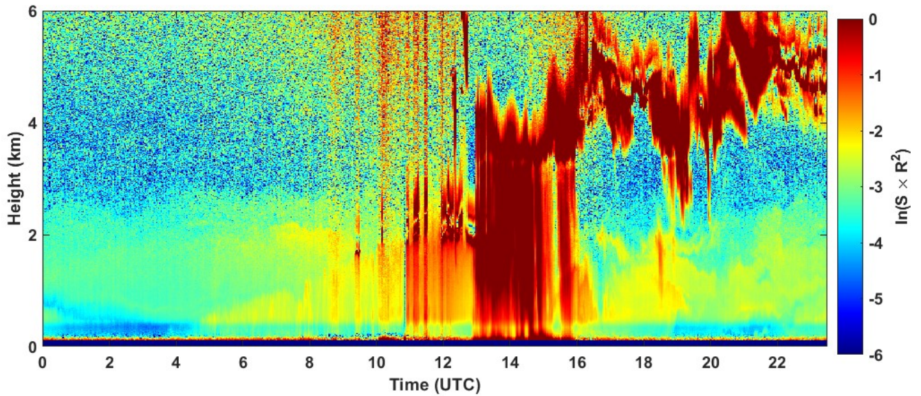
2022-08-12 RCS quick look CHM15k - ILVA LIDAR1 DIREZIONE
