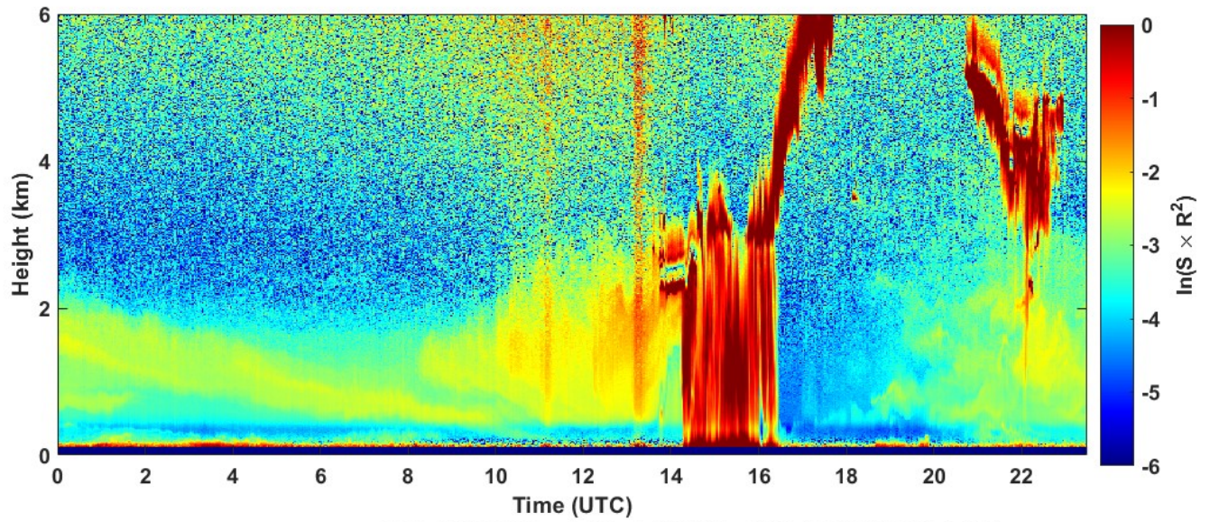
2022-05-18 RCS quick look CHM15k - ILVA LIDAR1 DIREZIONE
