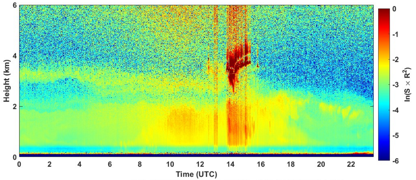
2022-05-12 RCS quick look CHM15k - ILVA LIDAR1 DIREZIONE
