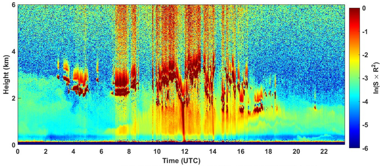
2022-05-04 RCS quick look CHM15k - ILVA LIDAR1 DIREZIONE
