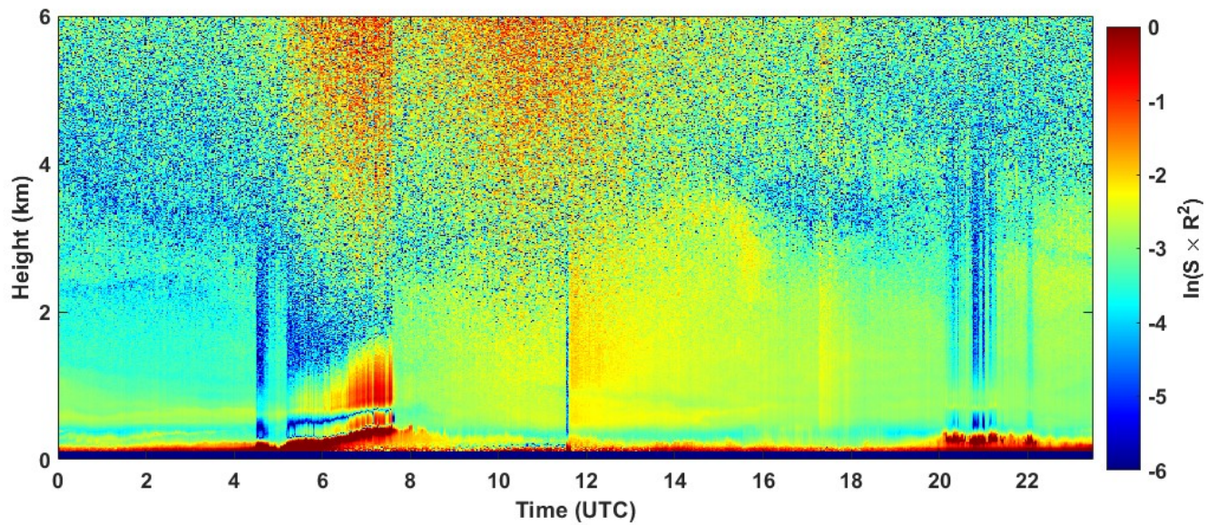
2022-05-24 RCS quick look CHM15k - ILVA LIDAR1 DIREZIONE
