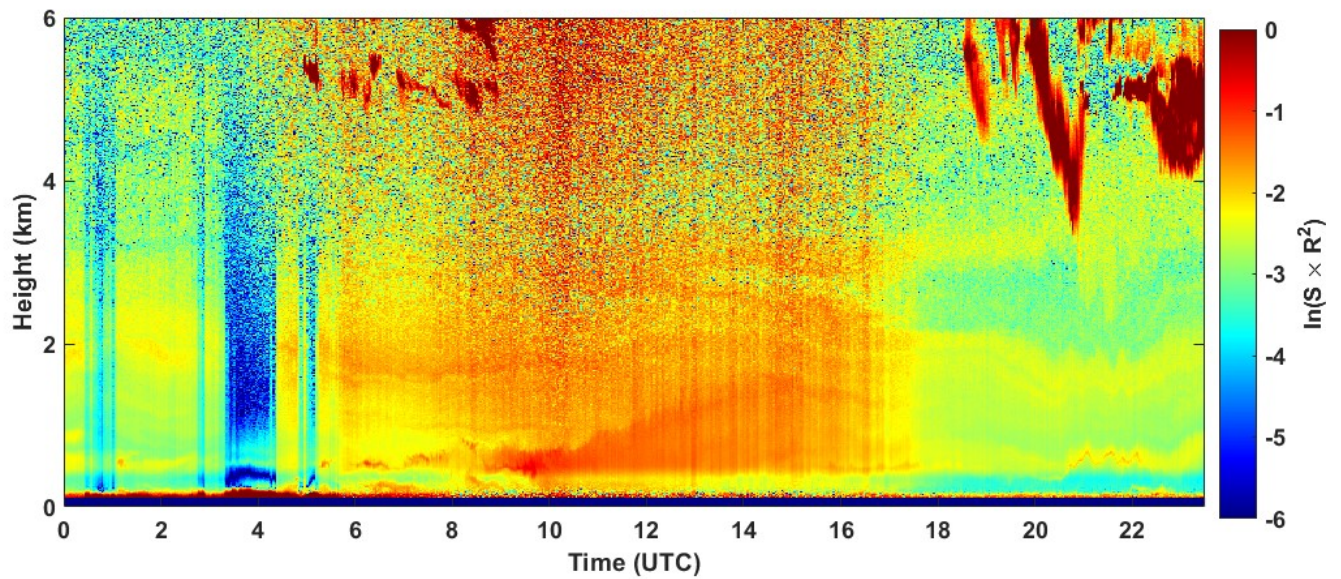
2022-05-28 RCS quick look CHM15k - ILVA LIDAR1 DIREZIONE
