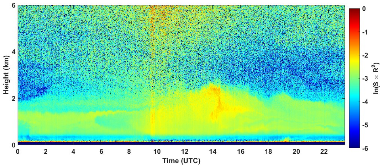
2022-05-22 RCS quick look CHM15k - ILVA LIDAR1 DIREZIONE
