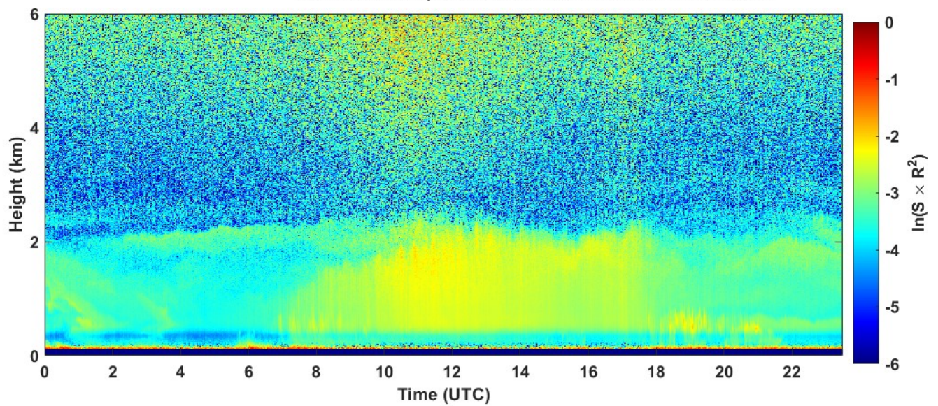
2022-05-14 RCS quick look CHM15k - ILVA LIDAR1 DIREZIONE
