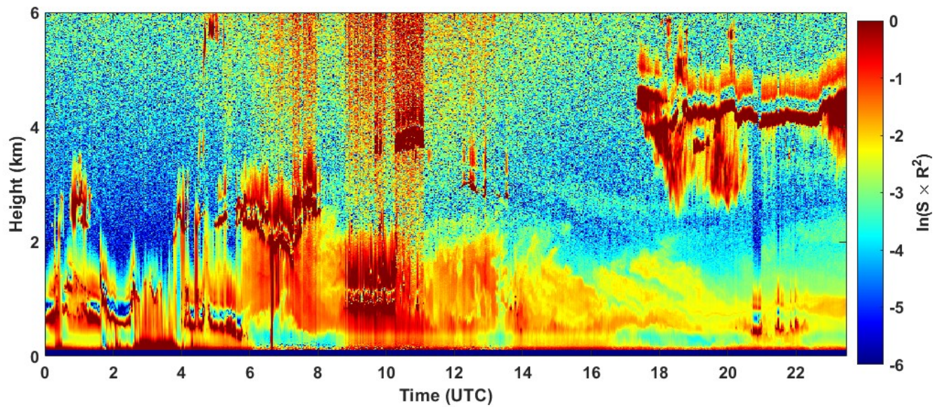
2022-05-08 RCS quick look CHM15k - ILVA LIDAR1 DIREZIONE
