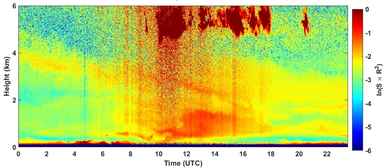
2022-05-26 RCS quick look CHM15k - ILVA LIDAR1 DIREZIONE
