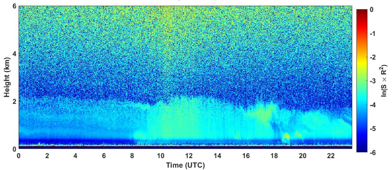
2022-05-20 RCS quick look CHM15k - ILVA LIDAR1 DIREZIONE
