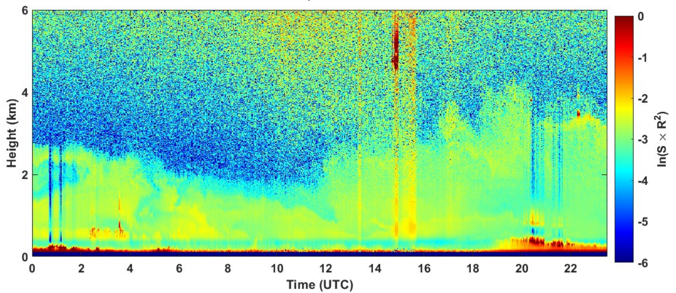
2022-05-30 RCS quick look CHM15k - ILVA LIDAR1 DIREZIONE
