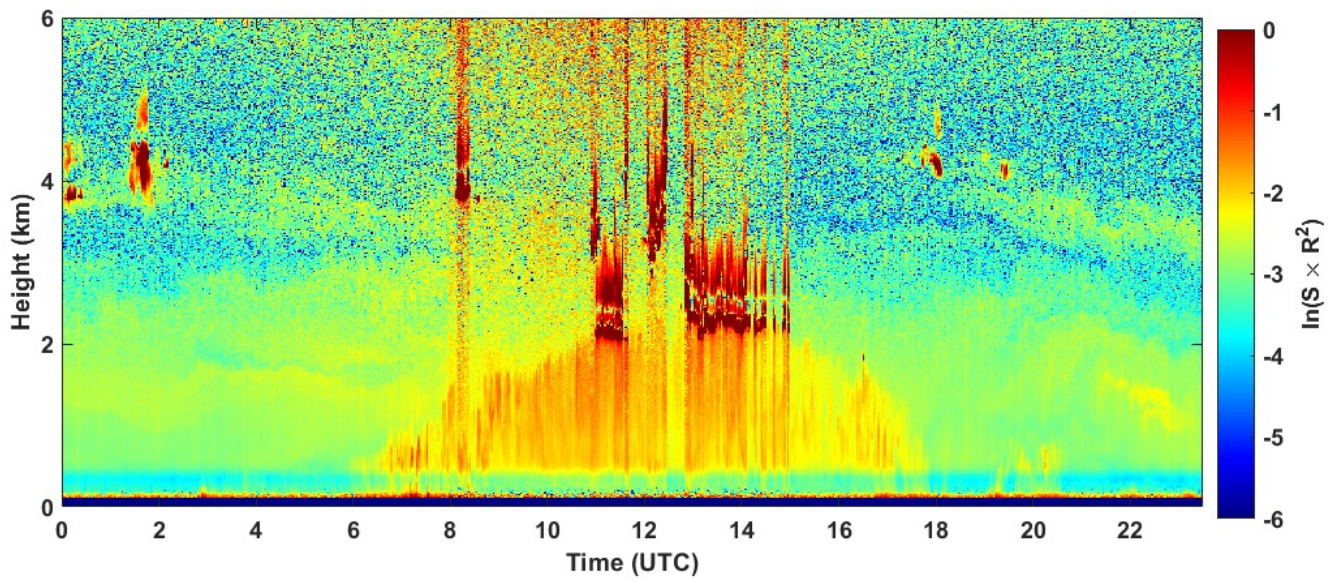
2022-05-10 RCS quick look CHM15k - ILVA LIDAR1 DIREZIONE
