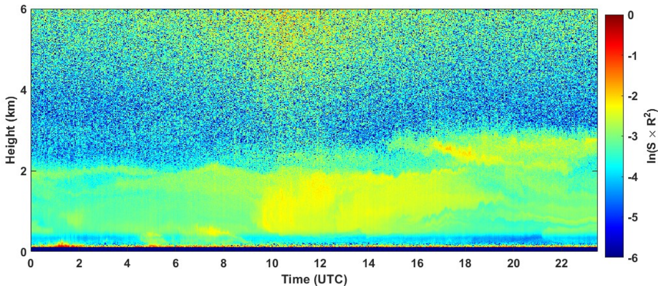
2022-05-16 RCS quick look CHM15k - ILVA LIDAR1 DIREZIONE
