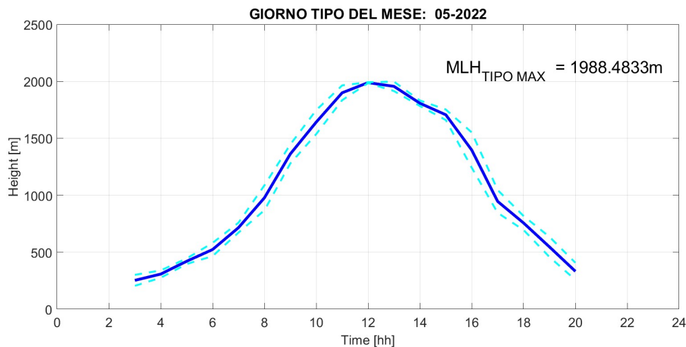
Fig. 2: Giorno tipo del parametro Mixing Layer Height nel mese di MAGGIO 2022, rappresentato mediante media oraria (linea blu continua) e deviazione standard (linee celesti tratteggiate).
