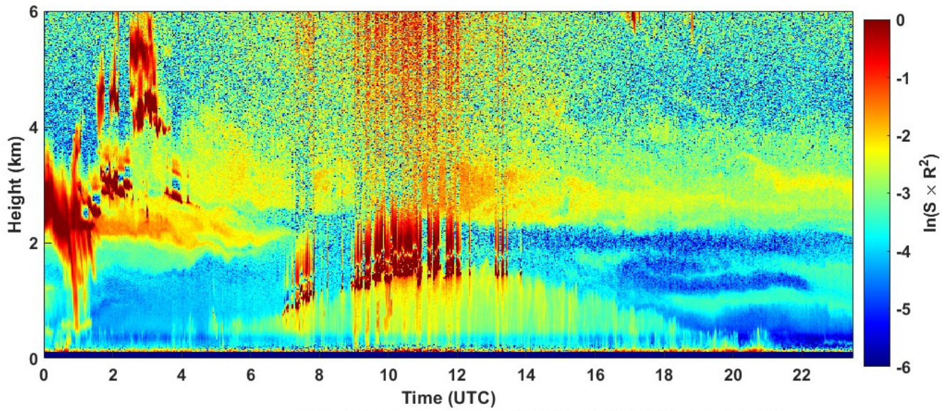
2022-04-06 RCS quick look CHM15k - ILVA LIDAR1 DIREZIONE
