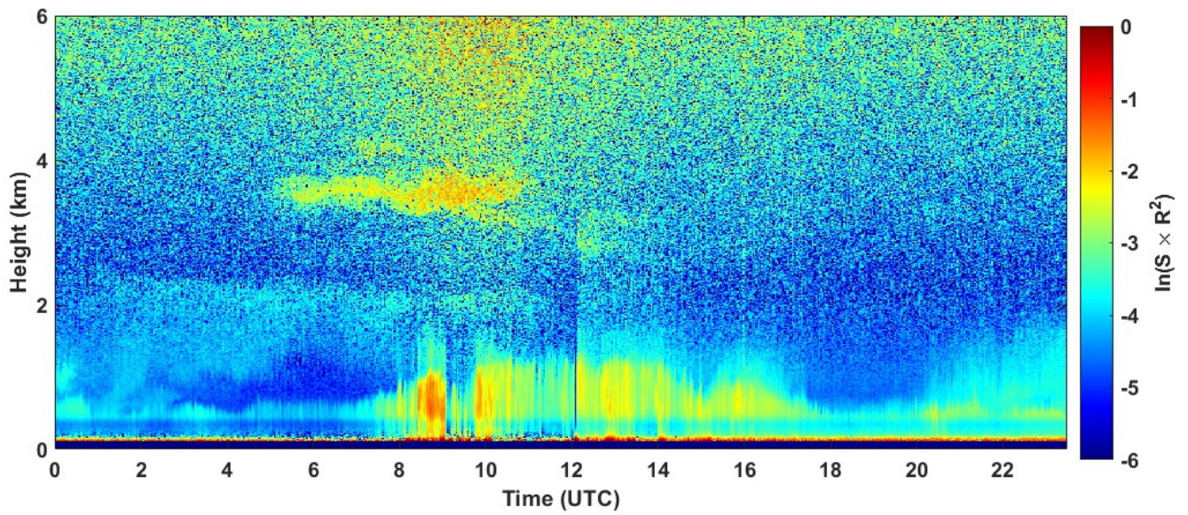
2022-04-28 RCS quick look CHM15k - ILVA LIDAR1 DIREZIONE
