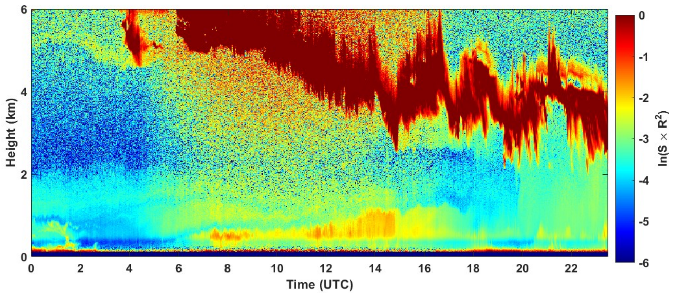
2022-04-16 RCS quick look CHM15k - ILVA LIDAR1 DIREZIONE
