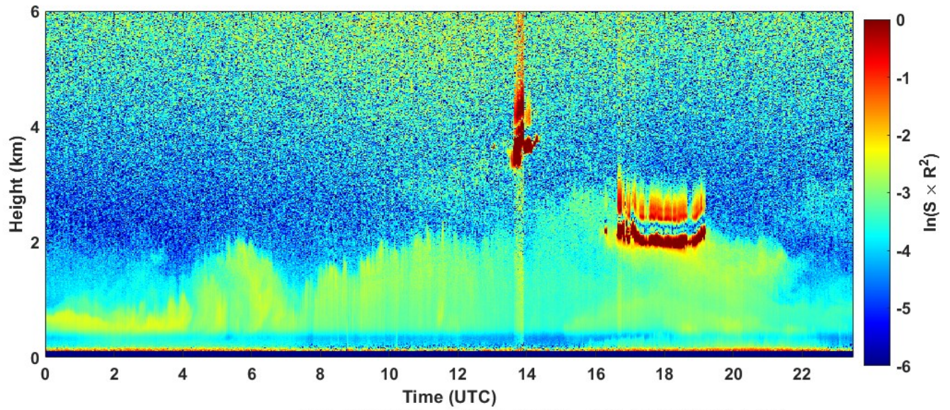
2022-04-20 RCS quick look CHM15k - ILVA LIDAR1 DIREZIONE
