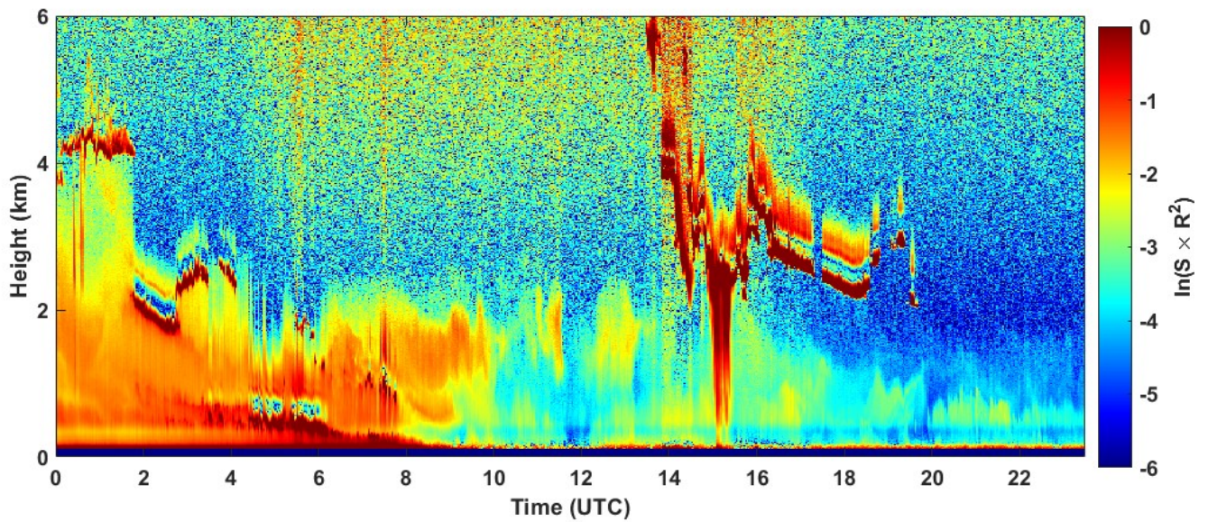
2022-04-22 RCS quick look CHM15k - ILVA LIDAR1 DIREZIONE
