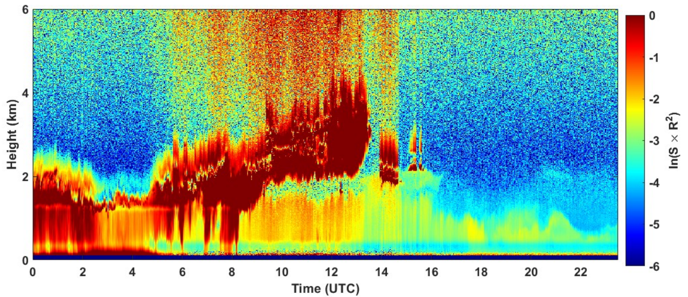
2022-04-18 RCS quick look CHM15k - ILVA LIDAR1 DIREZIONE
