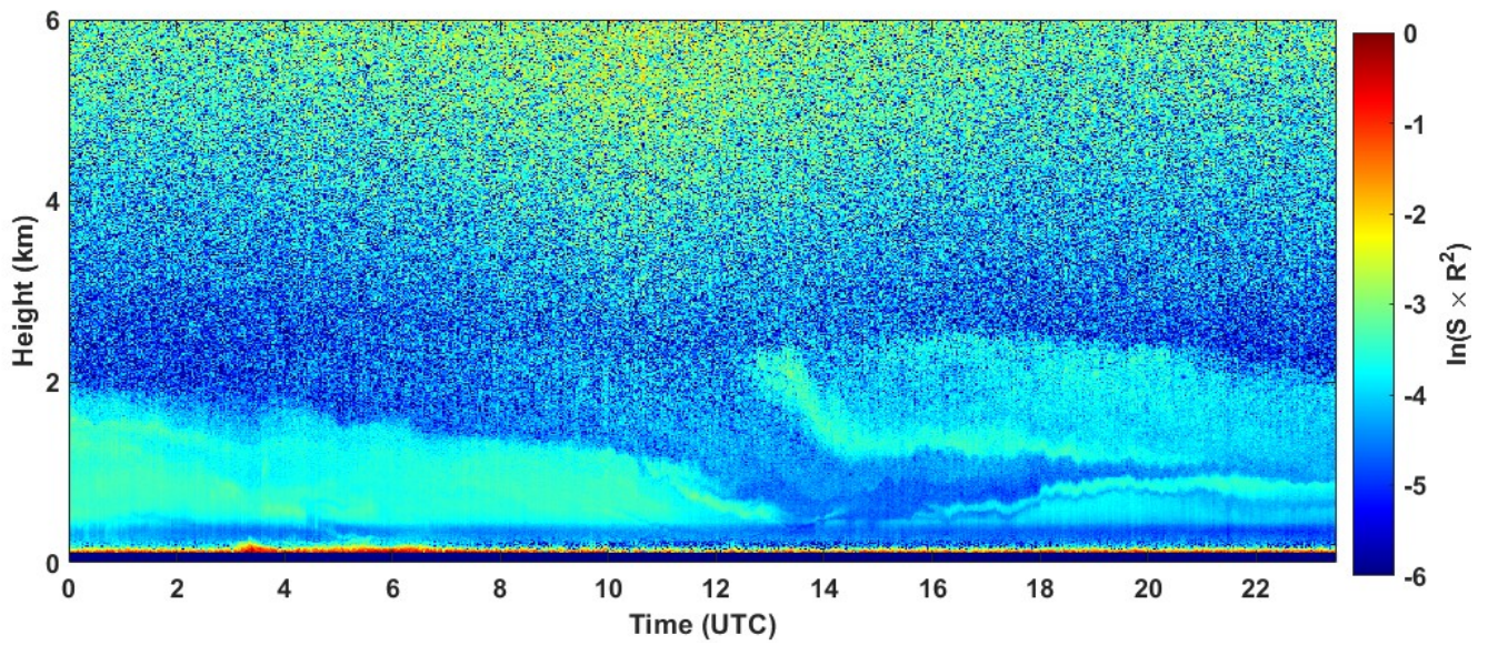
2022-04-26 RCS quick look CHM15k - ILVA LIDAR1 DIREZIONE
