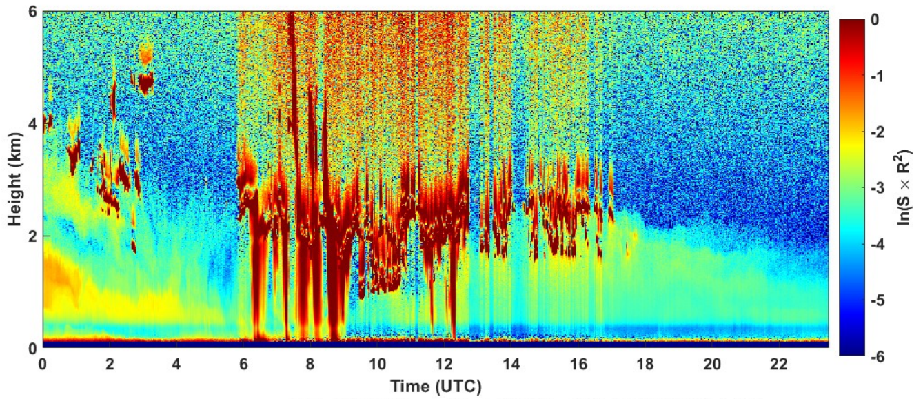
2022-04-08 RCS quick look CHM15k - ILVA LIDAR1 DIREZIONE
