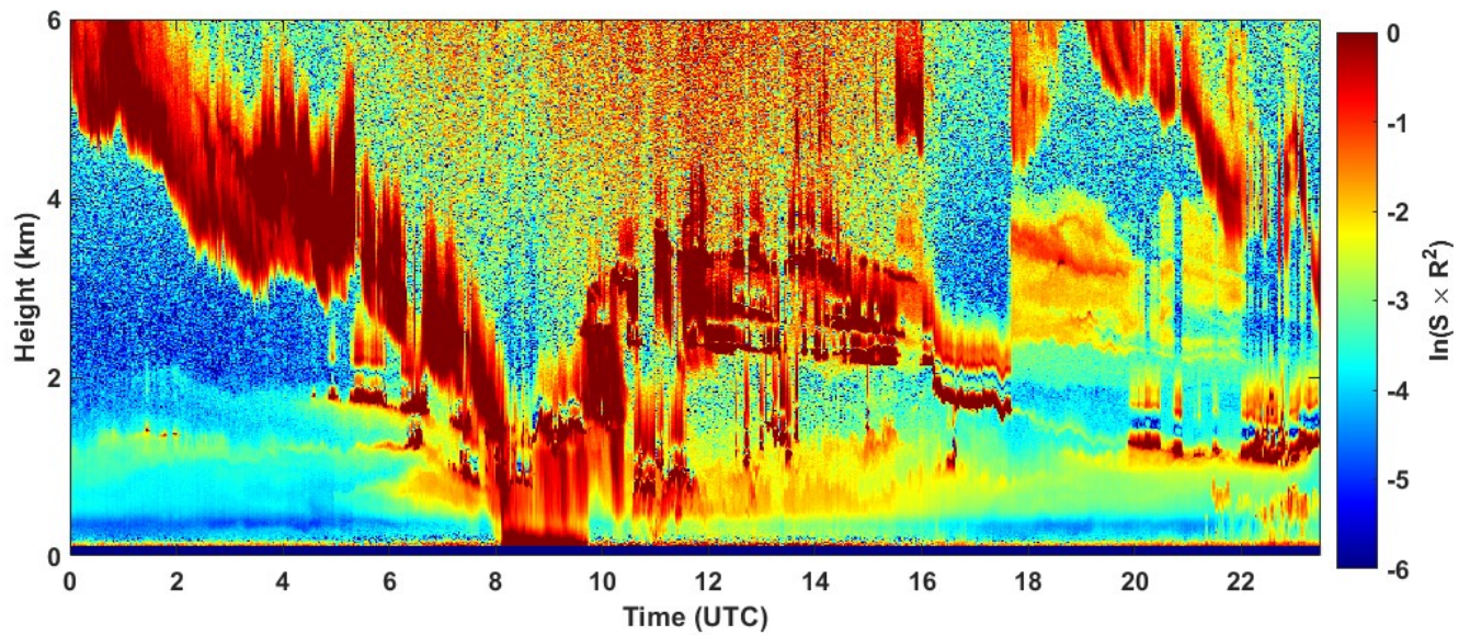
2022-04-04 RCS quick look CHM15k - ILVA LIDAR1 DIREZIONE
