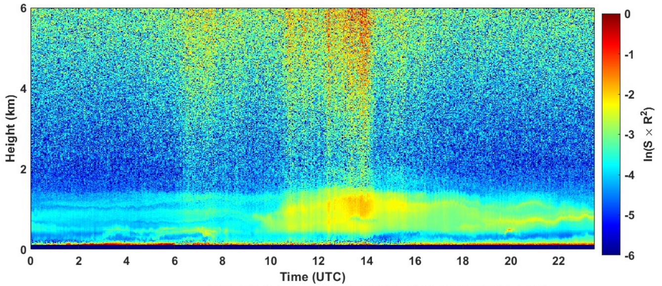
2022-04-14 RCS quick look CHM15k - ILVA LIDAR1 DIREZIONE
