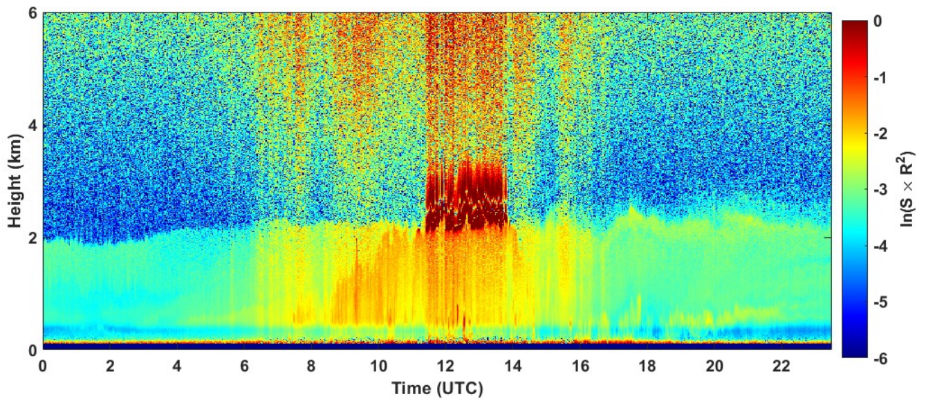
2022-04-30 RCS quick look CHM15k - ILVA LIDAR1 DIREZIONE
