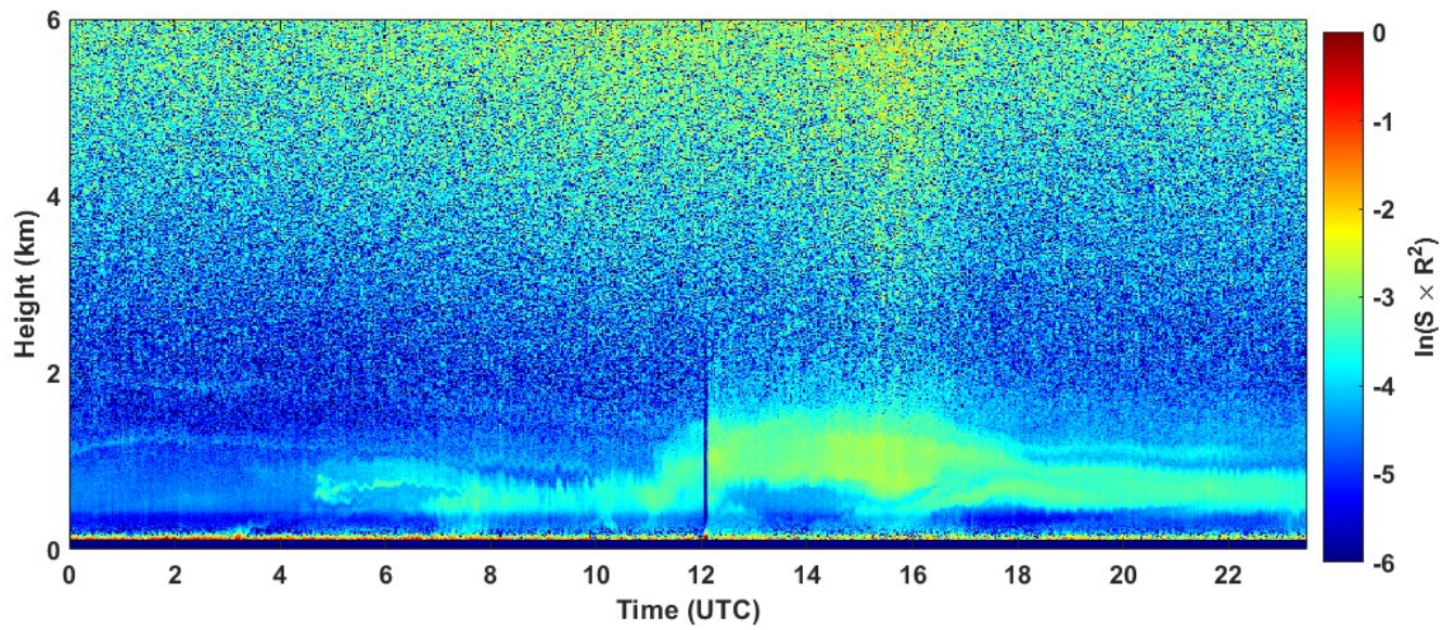
2022-04-12 RCS quick look CHM15k - ILVA LIDAR1 DIREZIONE
