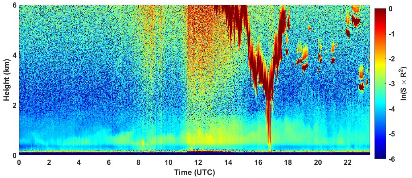
2022-04-10 RCS quick look CHM15k - ILVA LIDAR1 DIREZIONE
