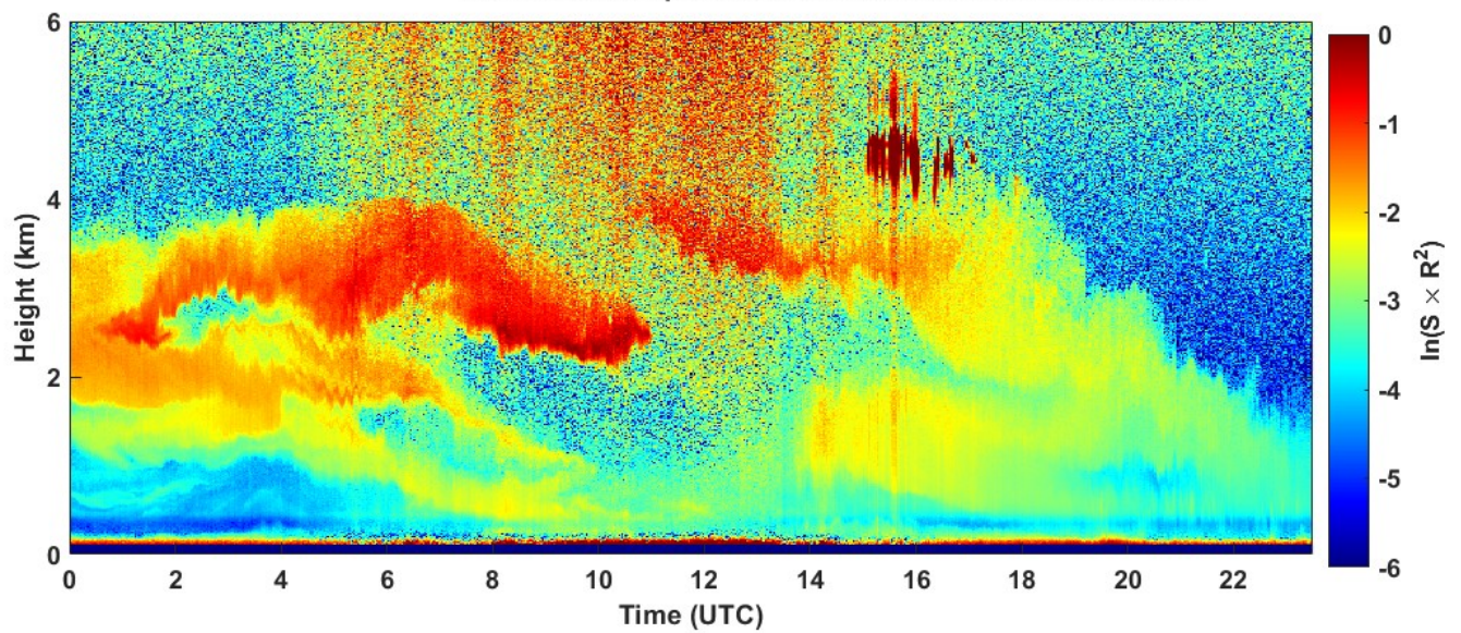
2022-04-24 RCS quick look CHM15k - ILVA LIDAR1 DIREZIONE
