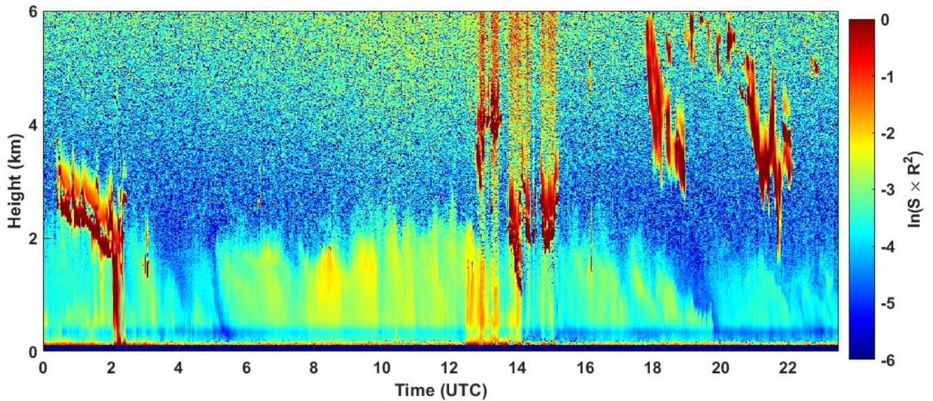
2022-04-02 RCS quick look CHM15k - ILVA LIDAR1 DIREZIONE
