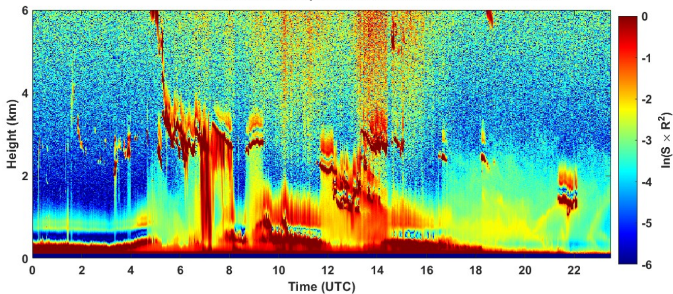
2022-03-31 RCS quick look CHM15k - ILVA LIDAR1 DIREZIONE
