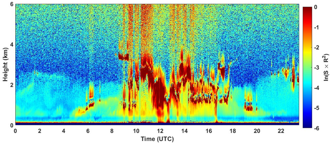
2022-03-21 RCS quick look CHM15k - ILVA LIDAR1 DIREZIONE
