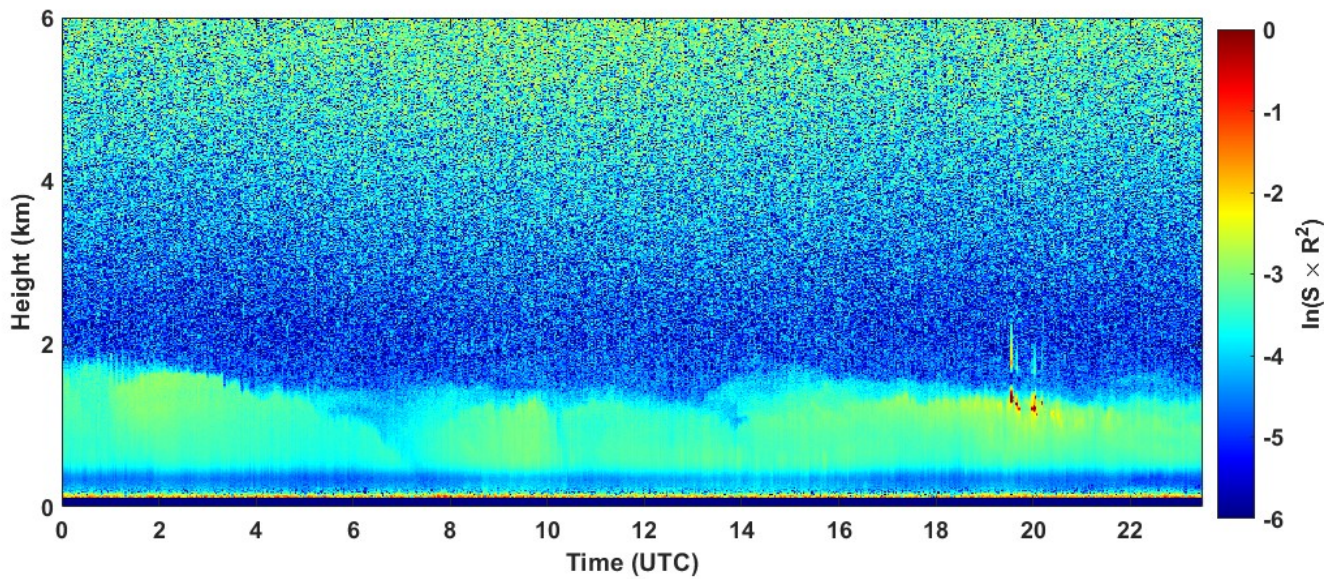
2022-03-13 RCS quick look CHM15k - ILVA LIDAR1 DIREZIONE
