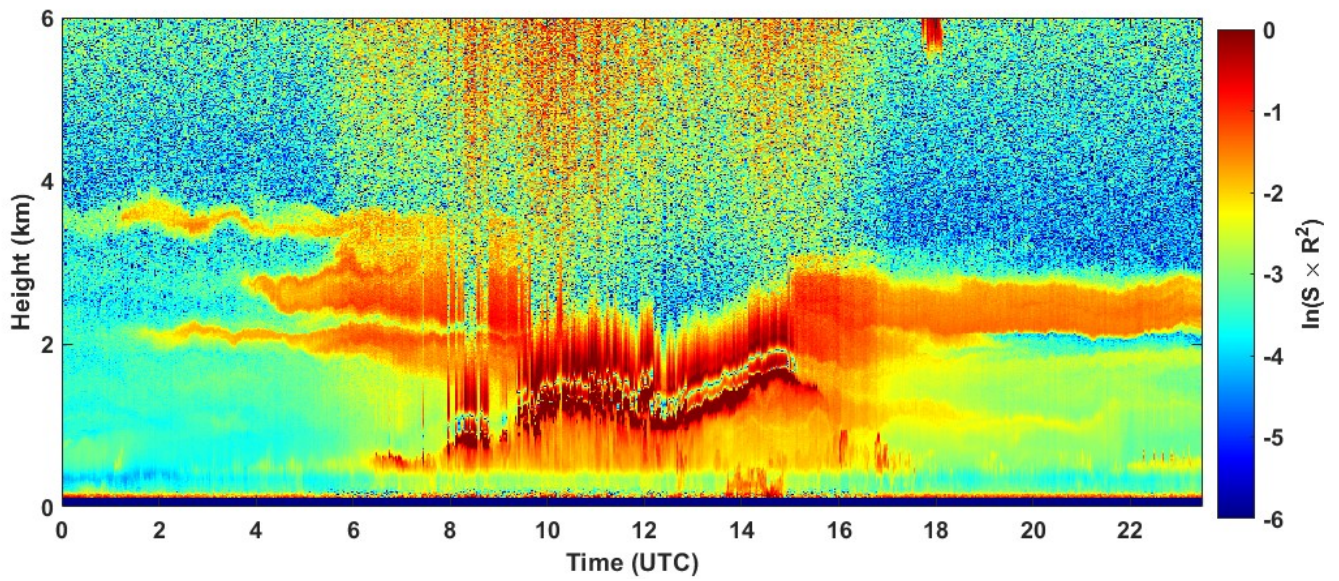
2022-03-17 RCS quick look CHM15k - ILVA LIDAR1 DIREZIONE
