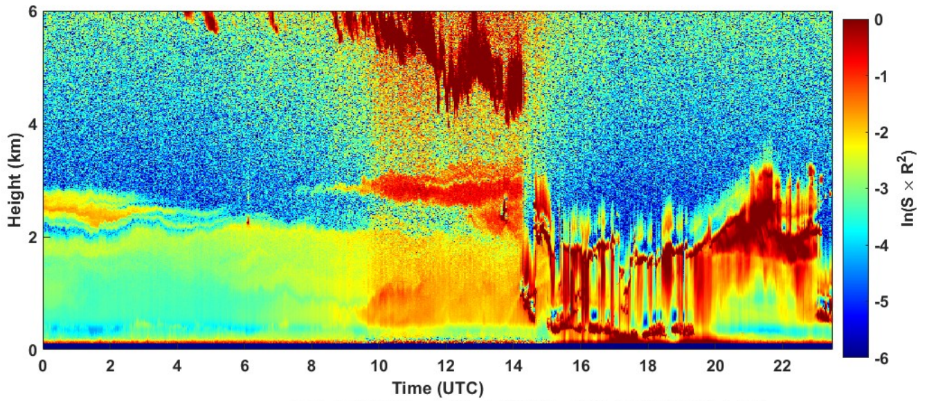
2022-03-19 RCS quick look CHM15k - ILVA LIDAR1 DIREZIONE
