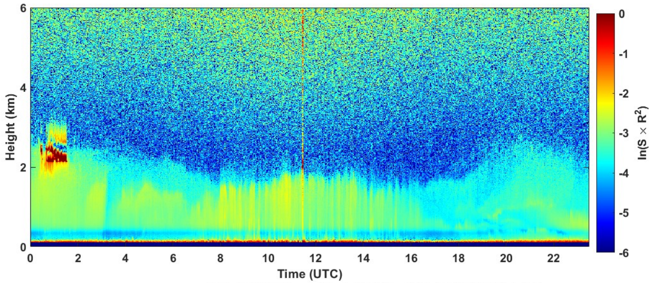
2022-03-23 RCS quick look CHM15k - ILVA LIDAR1 DIREZIONE
