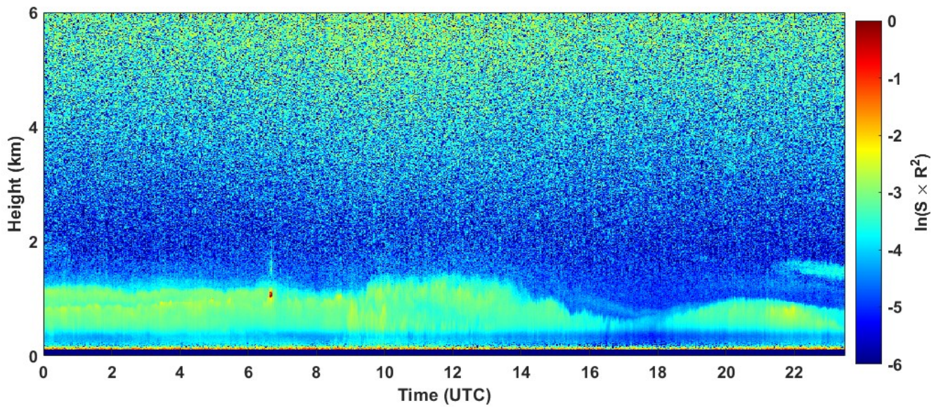
2022-03-15 RCS quick look CHM15k - ILVA LIDAR1 DIREZIONE
