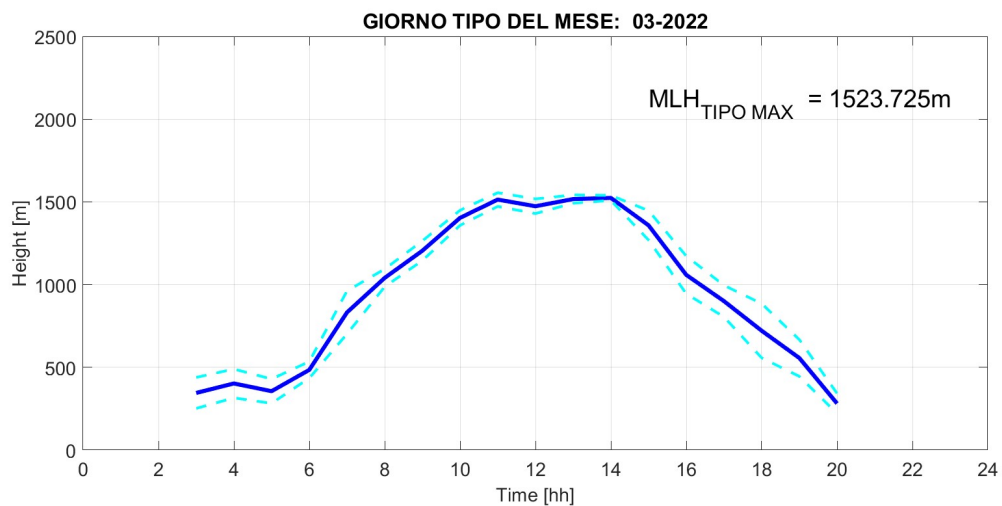
Fig. 2: Giorno tipo del parametro Mixing Layer Height nel mese di MARZO 2022, rappresentato mediante media oraria (linea blu continua) e deviazione standard (linee celesti tratteggiate).
