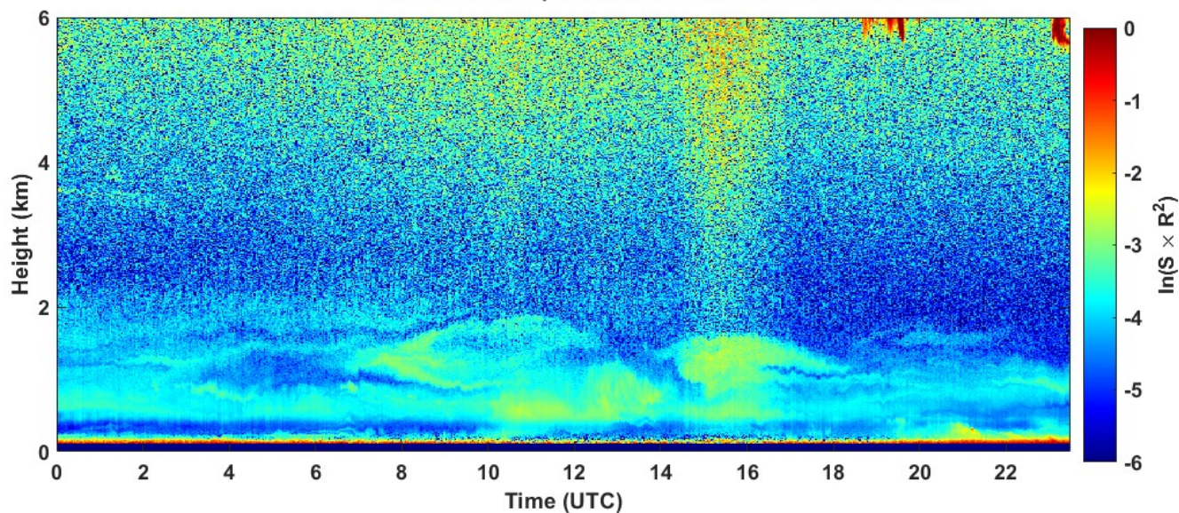
2022-03-27 RCS quick look CHM15k - ILVA LIDAR1 DIREZIONE
