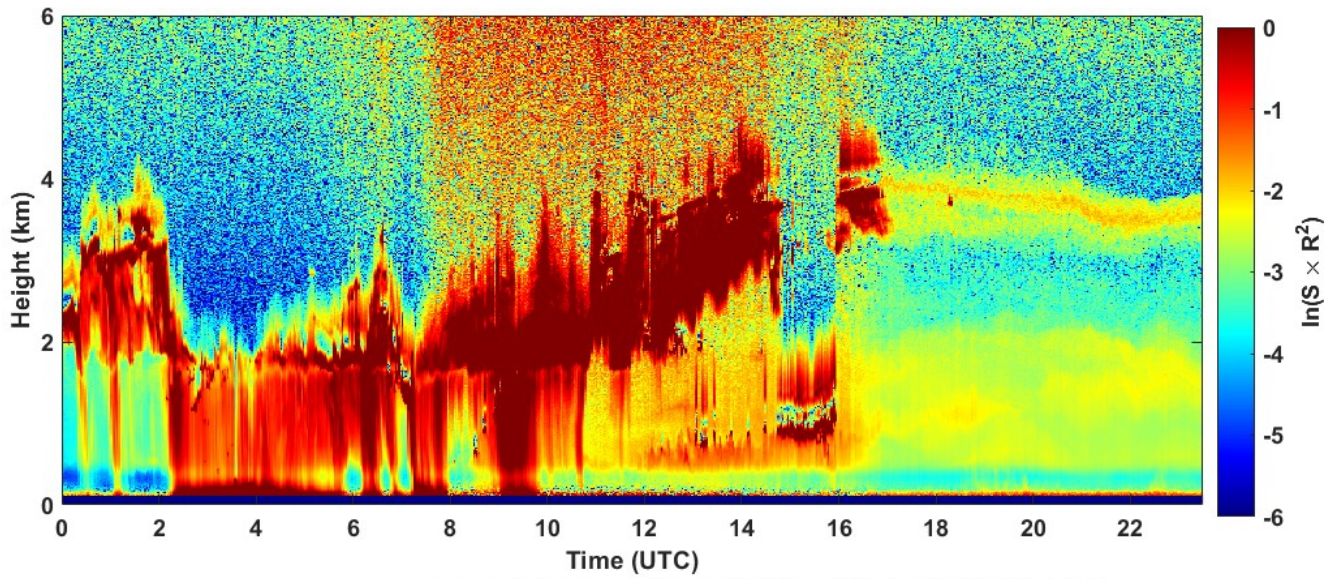
2022-03-29 RCS quick look CHM15k - ILVA LIDAR1 DIREZIONE
