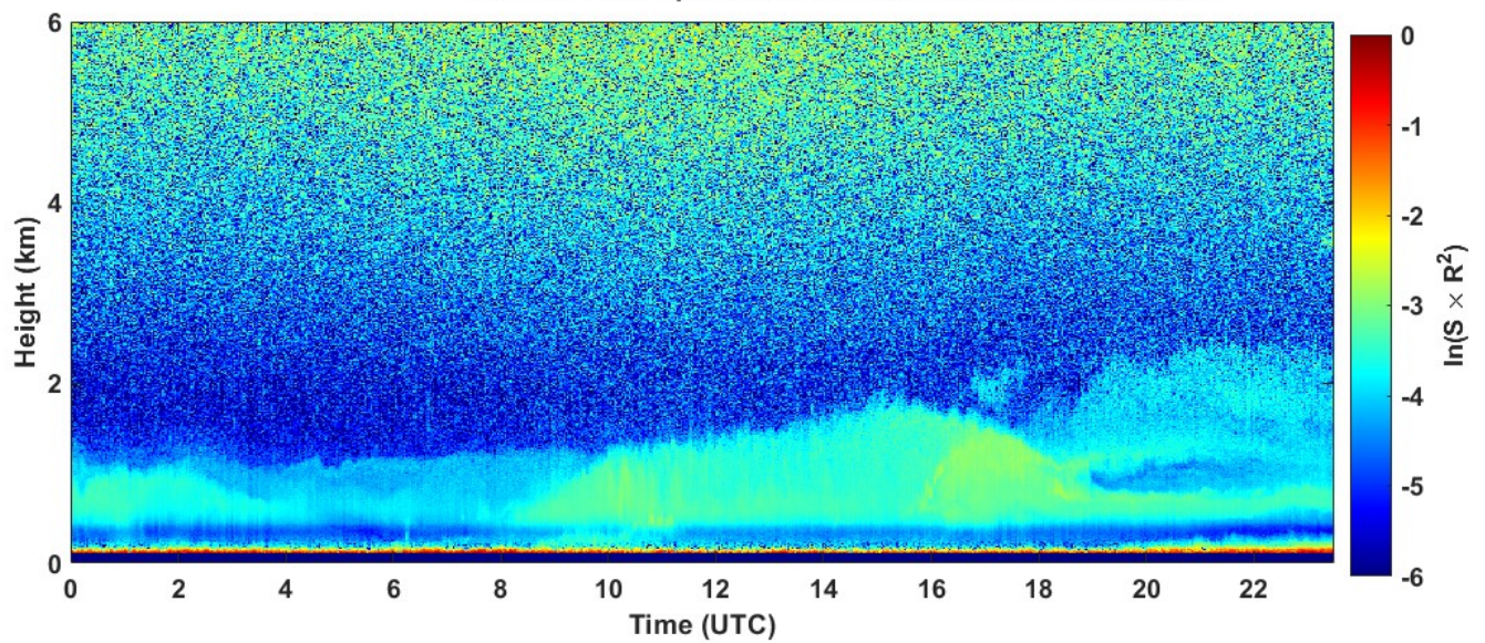
2022-03-25 RCS quick look CHM15k - ILVA LIDAR1 DIREZIONE
