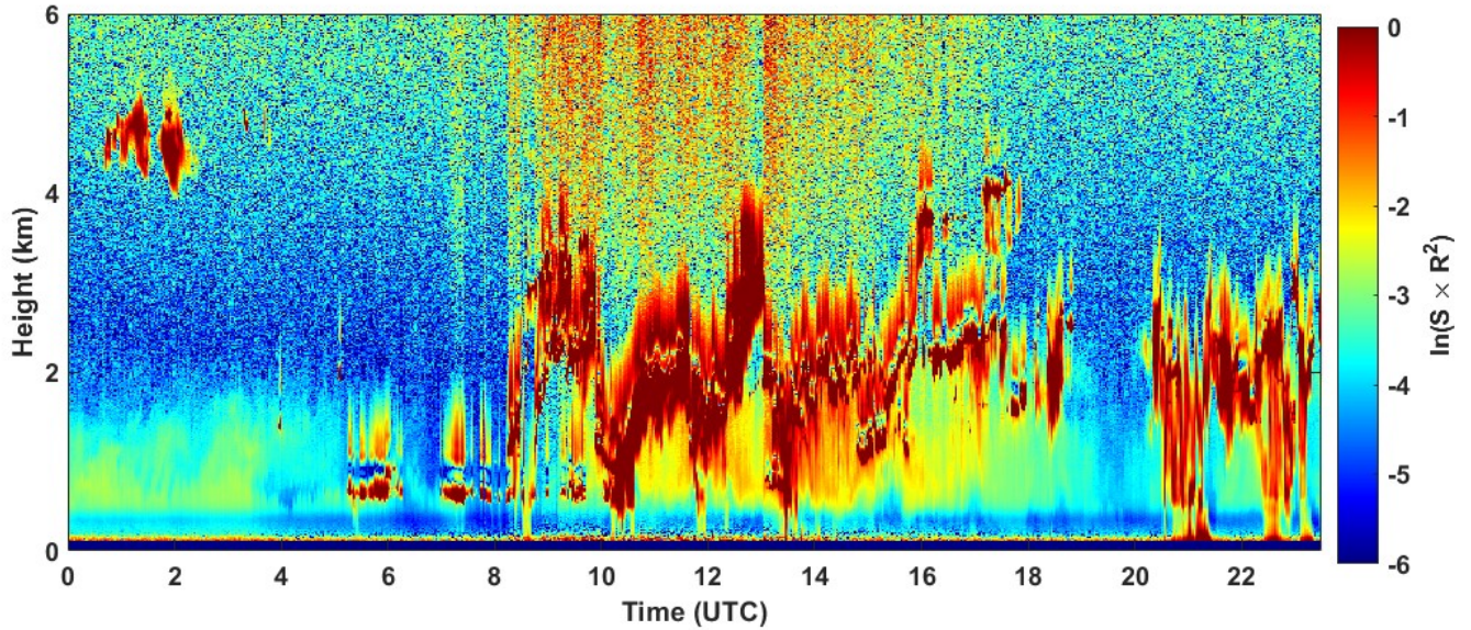
2022-03-04 RCS quick look CHM15k - ILVA LIDAR1 DIREZIONE
