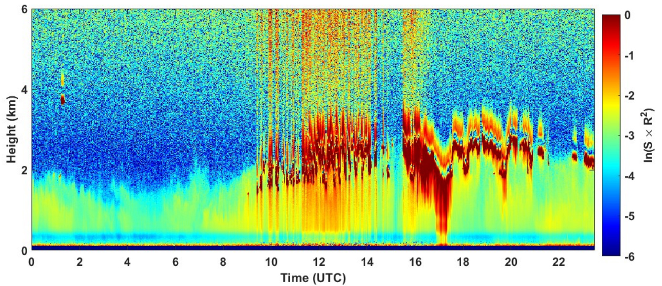
2022-03-11 RCS quick look CHM15k - ILVA LIDAR1 DIREZIONE
