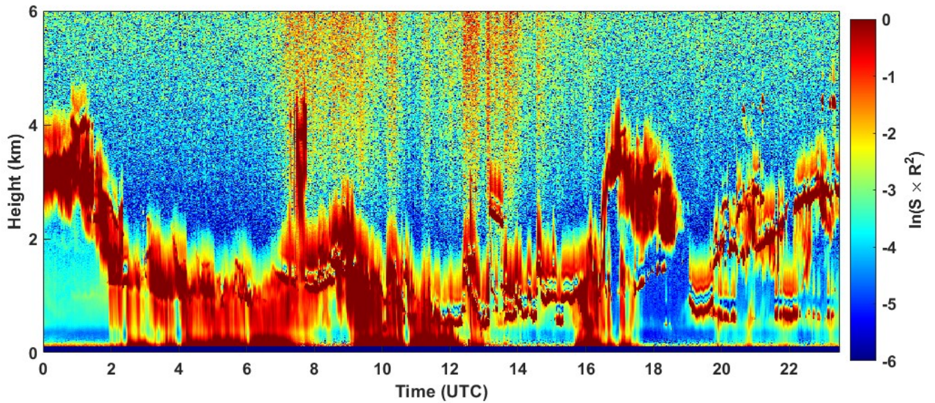
2022-03-06 RCS quick look CHM15k - ILVA LIDAR1 DIREZIONE
