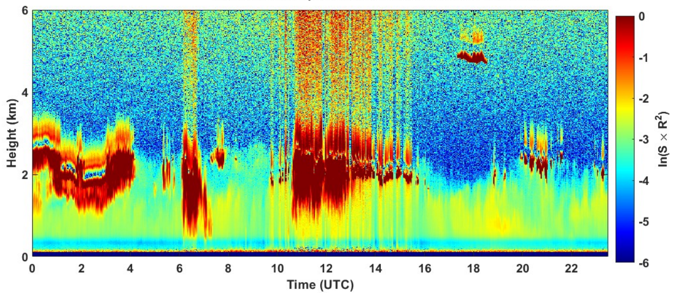
2022-03-09 RCS quick look CHM15k - ILVA LIDAR1 DIREZIONE
