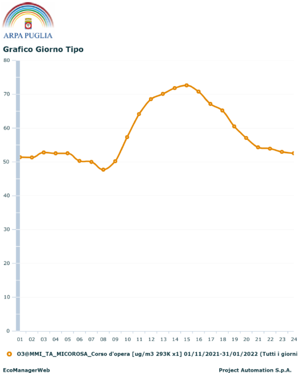
Figura 8: Grafico del giorno tipo per l'inquinante O 3 .
