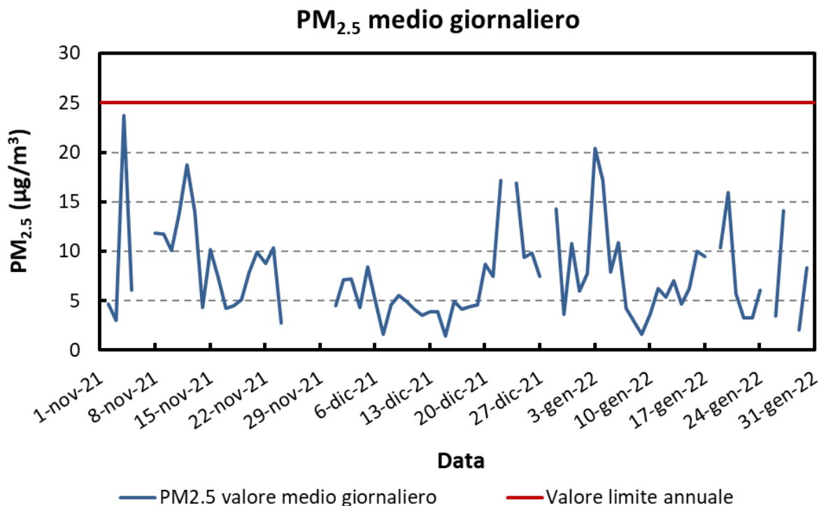
Figura 16: Andamento giornaliero del PM 2,5 (µg/m 3 ) misurato presso il sito oggetto della campagna.
