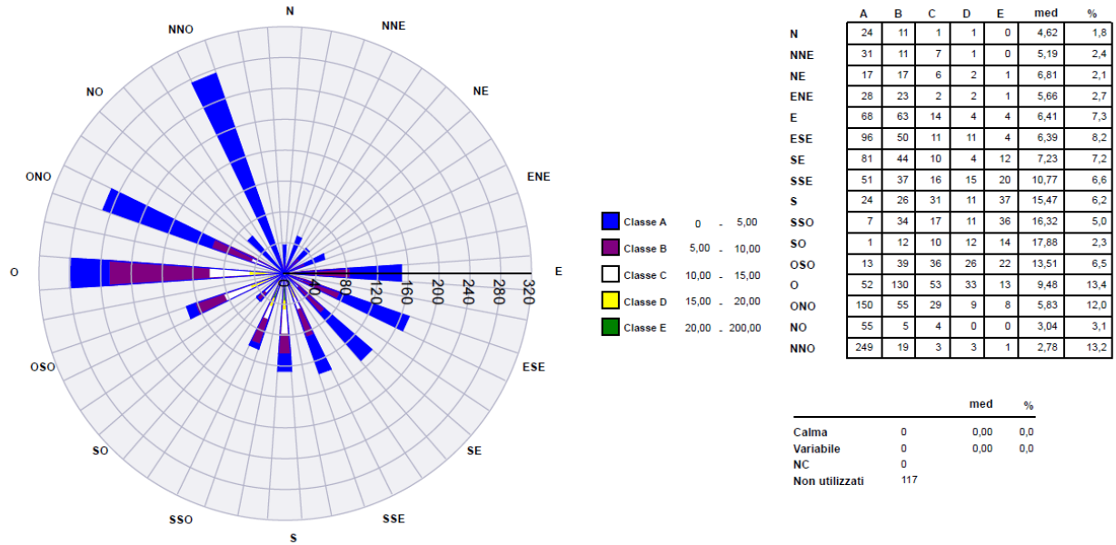
Figura 19: Rosa dell'inquinamento per l'inquinante biossido di azoto.
