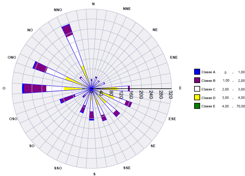
Figura 21: Rosa dell'inquinamento per l'inquinante biossido di zolfo.
