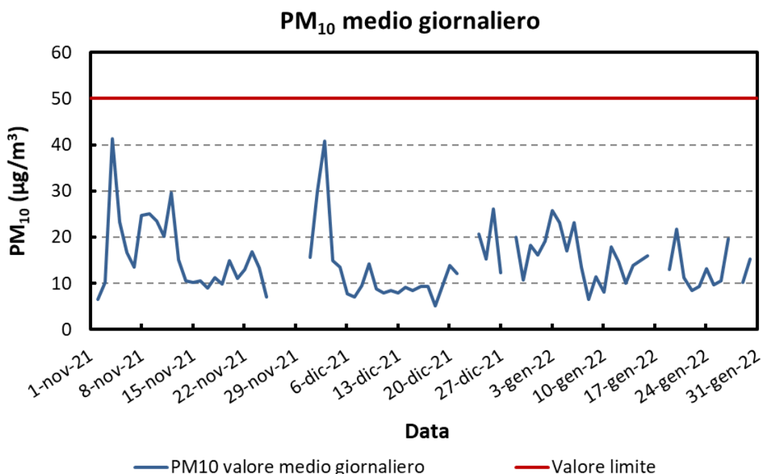
Figura 13: Andamento giornaliero del PM 10 (µg/m 3 ) misurato presso il sito oggetto della campagna.
