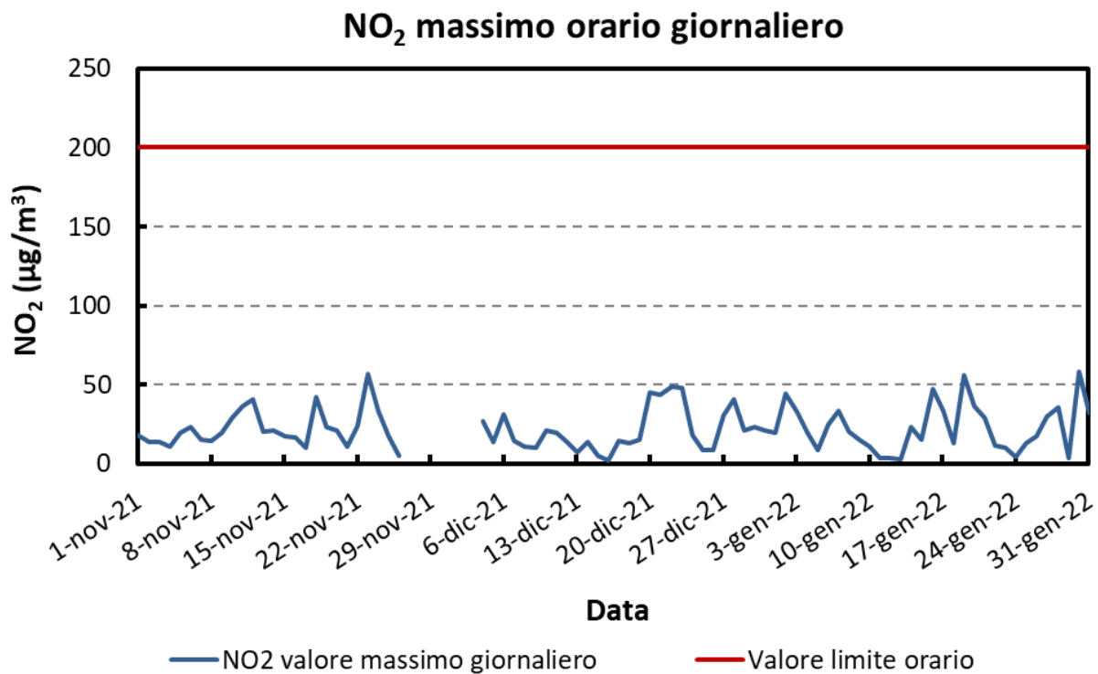
Figura 18: Andamento della concentrazione massima oraria giornaliera per il biossido di azoto (µg/m 3 ) misurata presso il sito oggetto della campagna.
