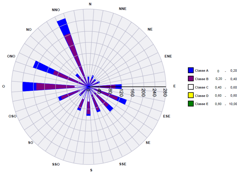
Figura 23: Rosa dell'inquinamento per l'inquinante monossido di carbonio.
