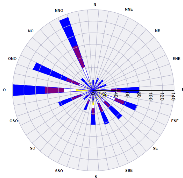
Figura 15: Rosa dell'inquinamento per il PM 10 .
