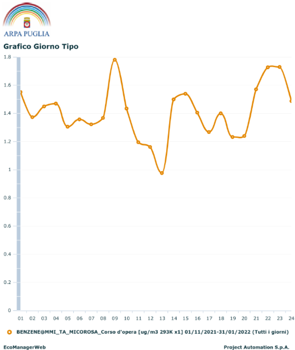
Figura 9: Grafico del giorno tipo per l'inquinante benzene.
