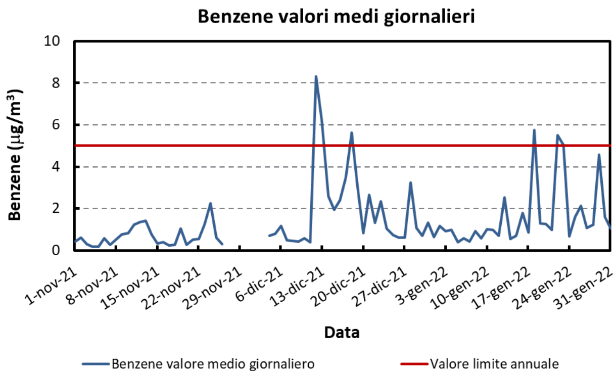
Figura 24: Andamento della concentrazione media giornaliera, per il benzene ( \mu\text{g}/\text{m}^3 ), misurata presso il sito oggetto della campagna.
