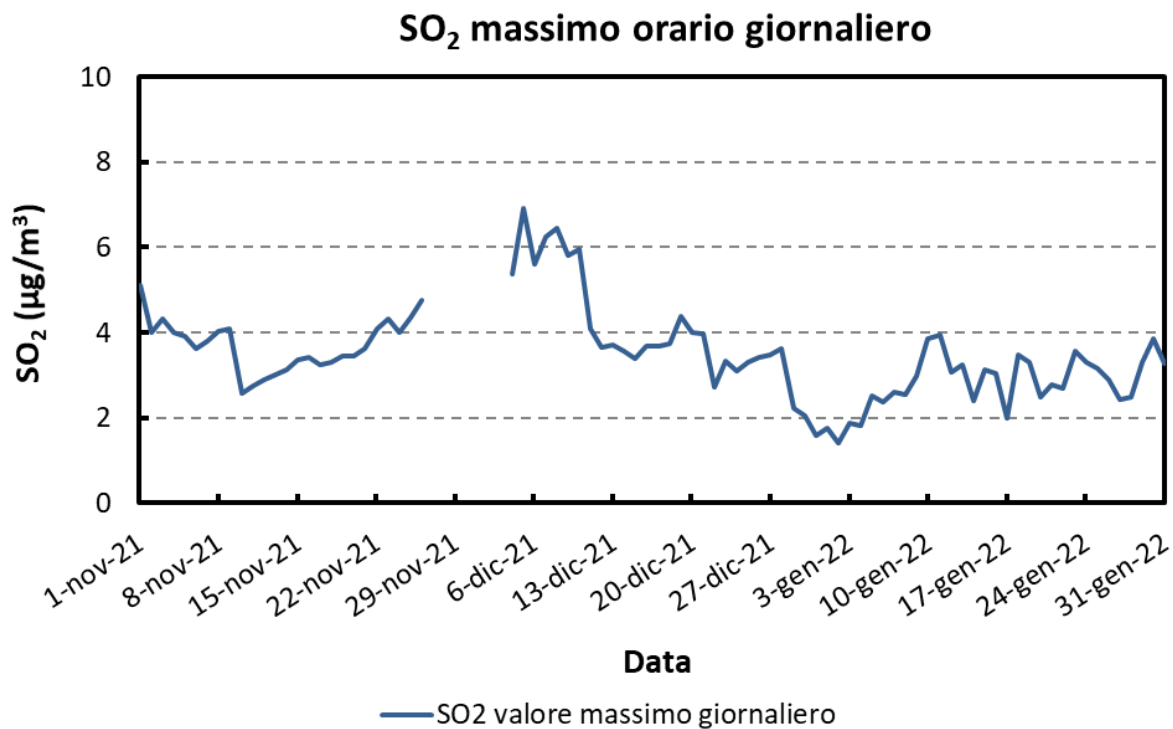
Figura 20: Andamento della concentrazione massima oraria giornaliera per il biossido di zolfo (µg/m 3 ) misurata presso il sito oggetto della campagna.
