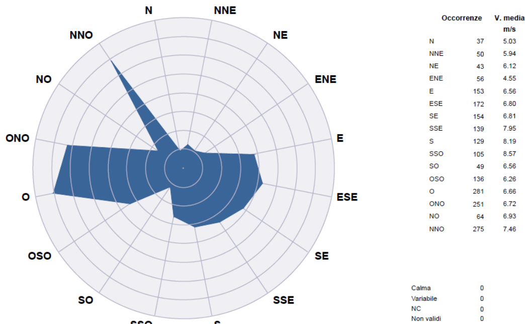
Figura 4: Rose dei venti per il periodo che va dal 01/11/2021 al 31/01/2022, corredato dalla tabella complessiva delle occorrenze.
