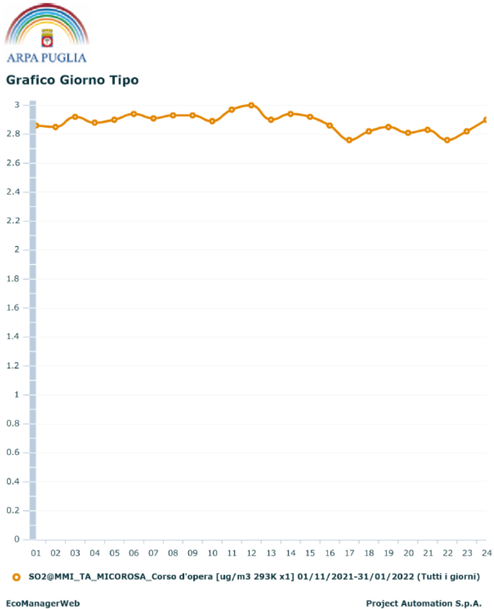
Figura 10: Grafico del giorno tipo per l'inquinante SO 2 .
