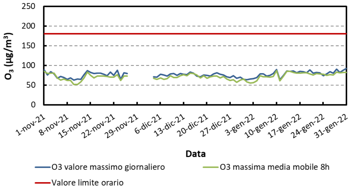
Figura 17: Andamento giornaliero del valore massimo e della massima media mobile misurata sulle 8 ore per l'inquinante ozono ( \mu\text{g}/\text{m}^3 ).
