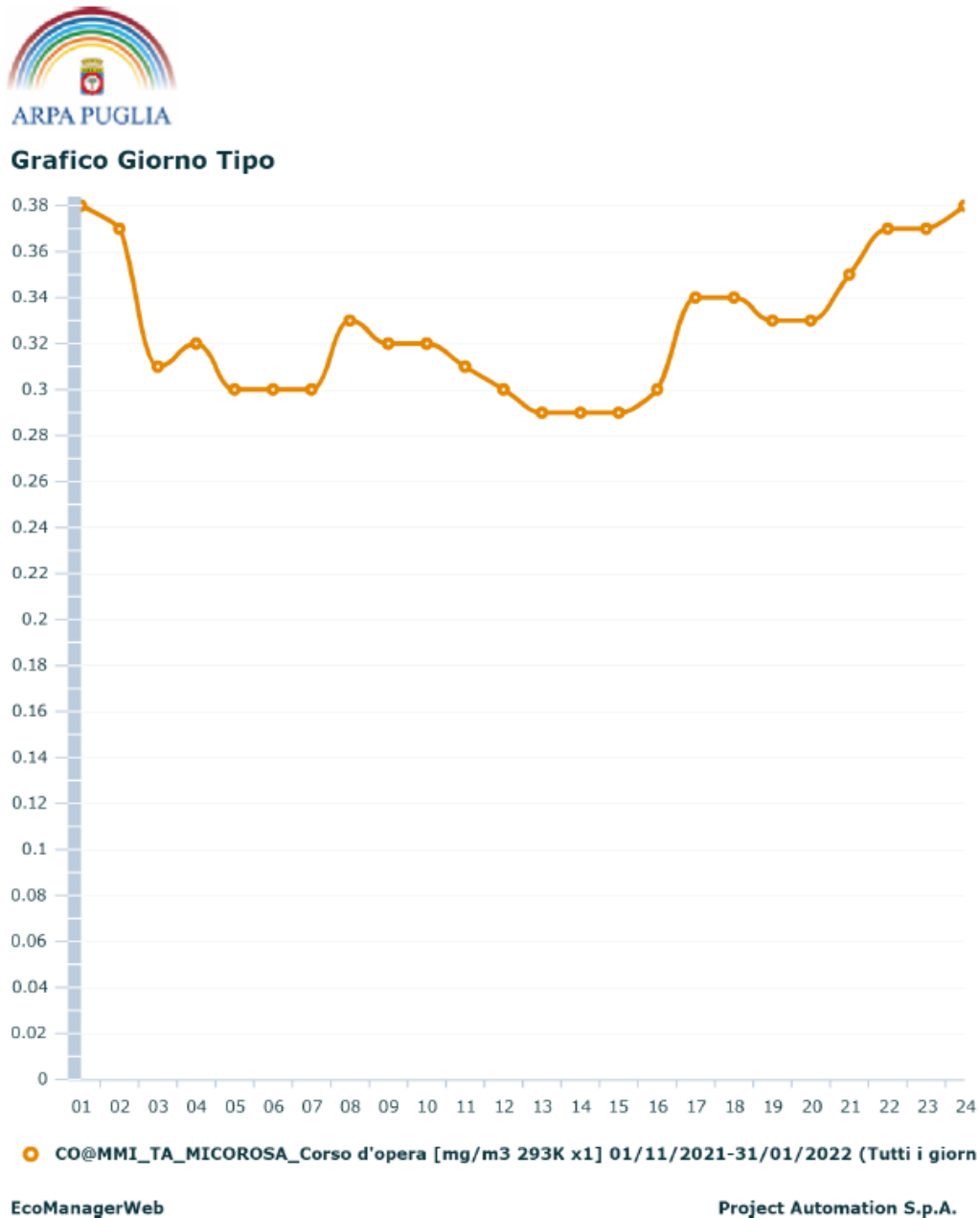
Figura 7: Grafico del giorno tipo per l'inquinante CO.
