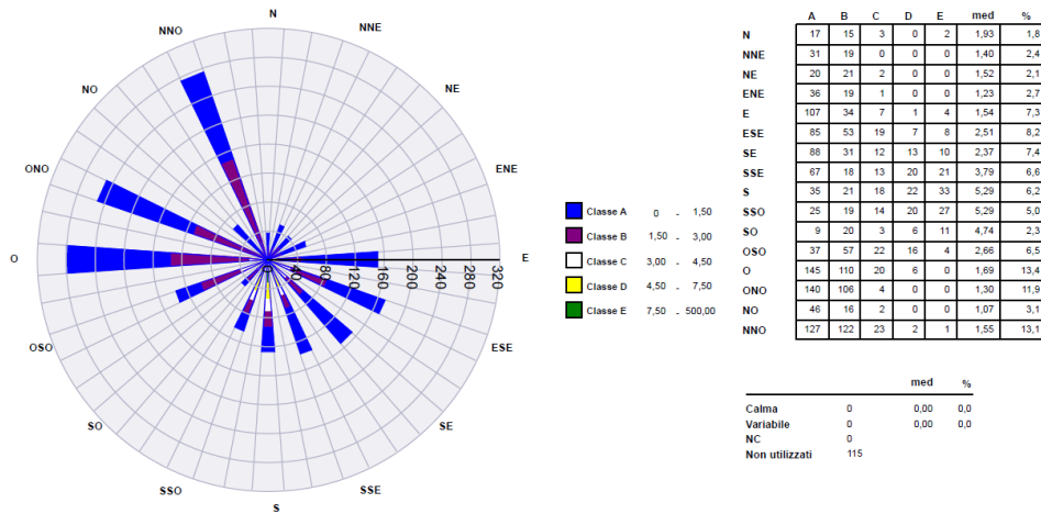
Figura 28: Rosa dell'inquinamento per gli idrocarburi policiclici aromatici.
