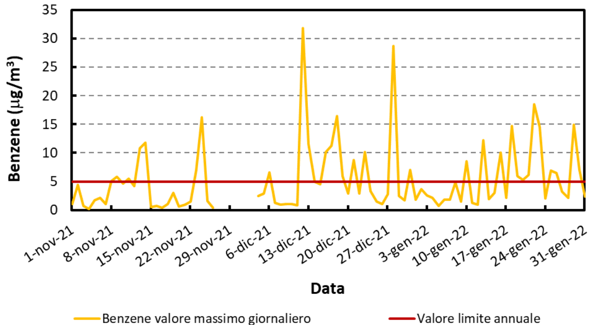
Figura 25: Andamento della concentrazione massima giornaliera, per il benzene ( \mu\text{g}/\text{m}^3 ), misurate presso il sito oggetto della campagna.
