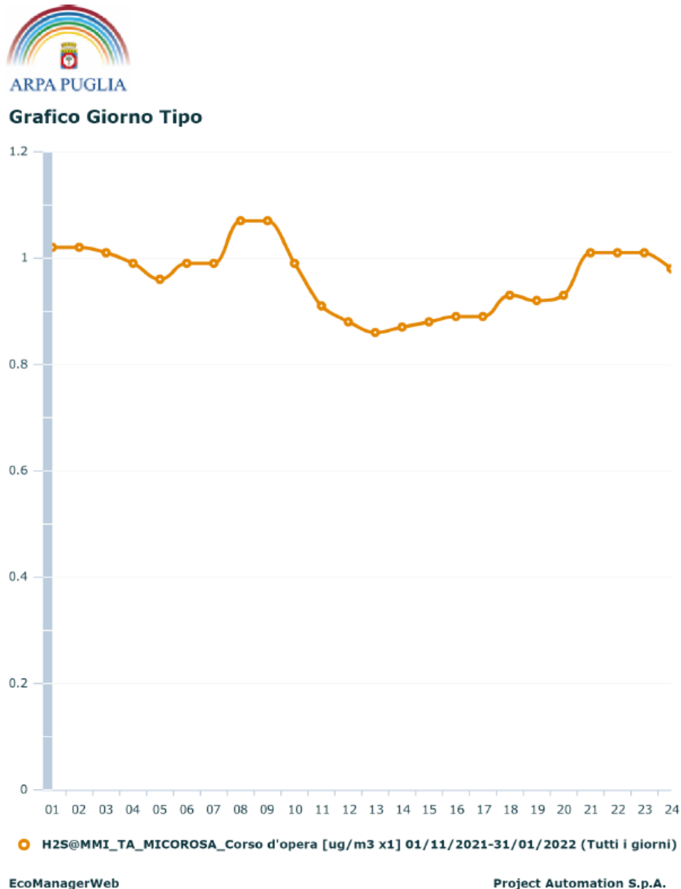
Figura 12: Grafico del giorno tipo per l'inquinante acido solfidrico.
