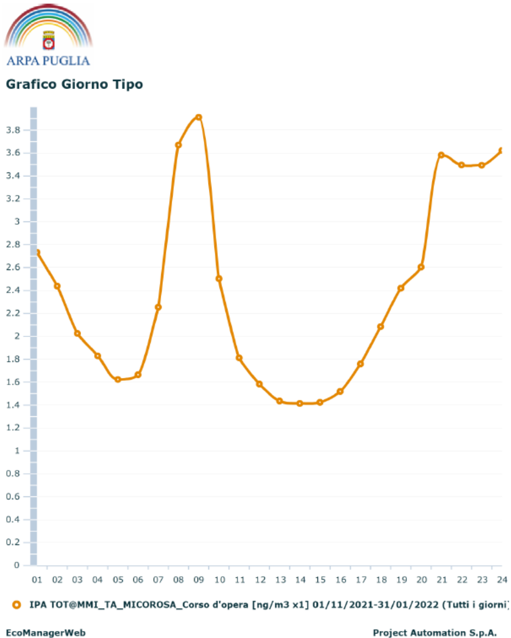
Figura 11: Grafico del giorno tipo per gli idrocarburi policiclici aromatici totali.
