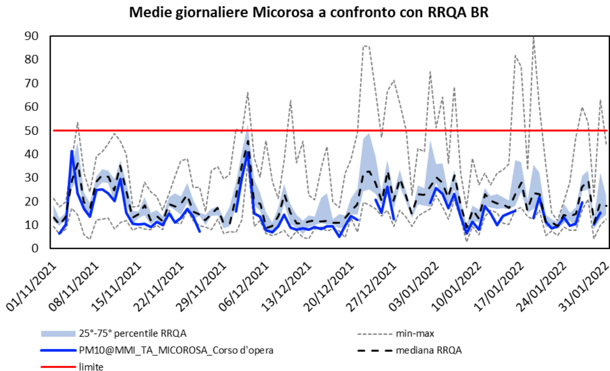
Figura 14: Andamento giornaliero del \text{PM}_{10} ( \mu\text{g}/\text{m}^3 ) misurato a Brindisi nel periodo oggetto della campagna.
