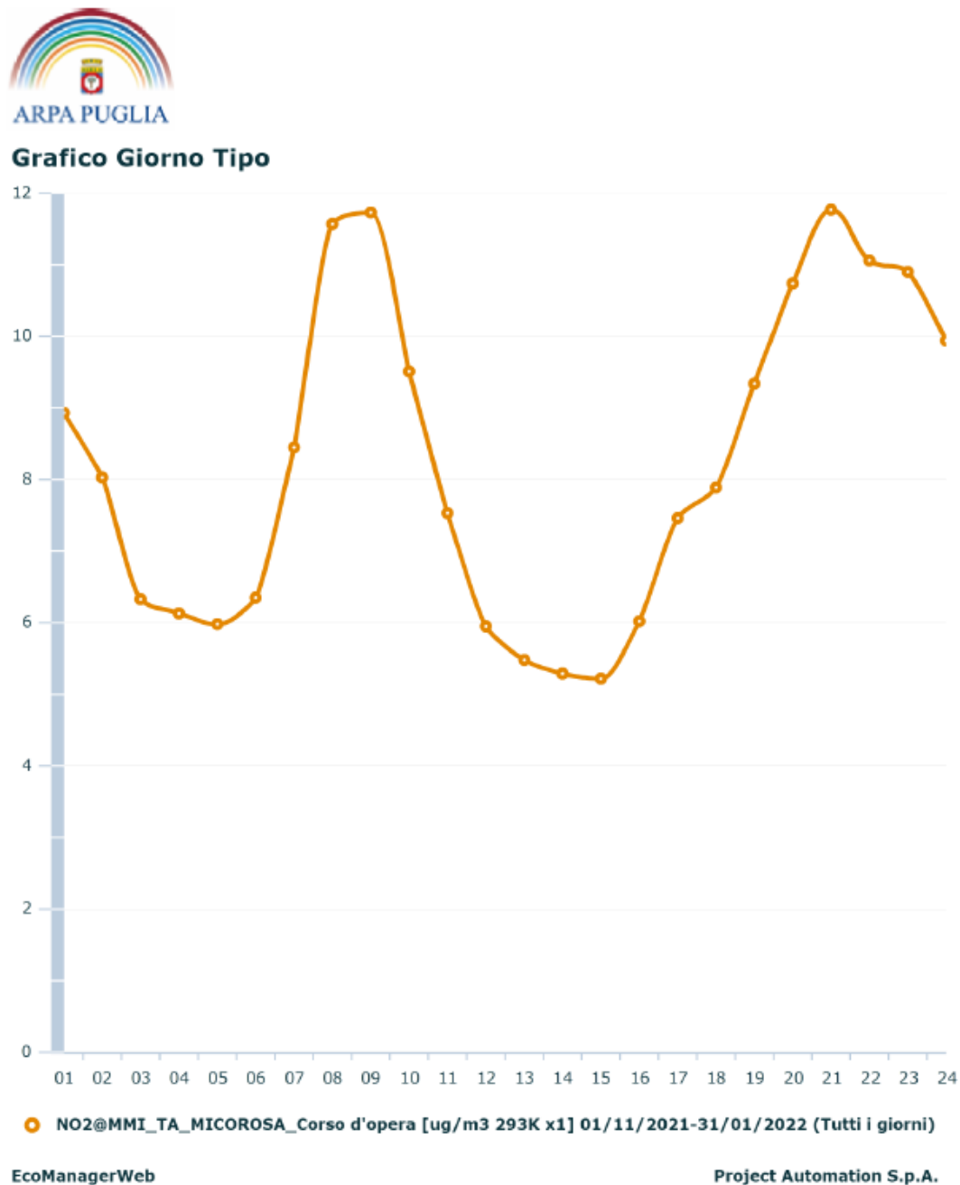
Figura 6: Grafico del giorno tipo per l'inquinante NO 2 .
