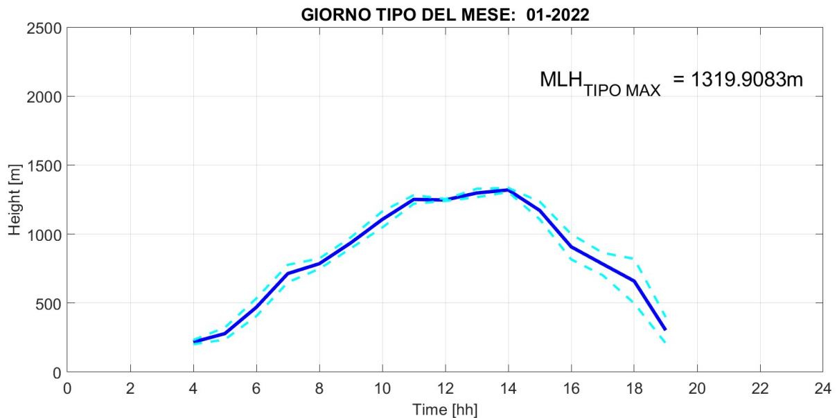
Fig. 2: Giorno tipo del parametro Mixing Layer Height nel mese di GENNAIO 2022, rappresentato mediante media oraria (linea blu continua) e deviazione standard (linee celesti tratteggiate).
