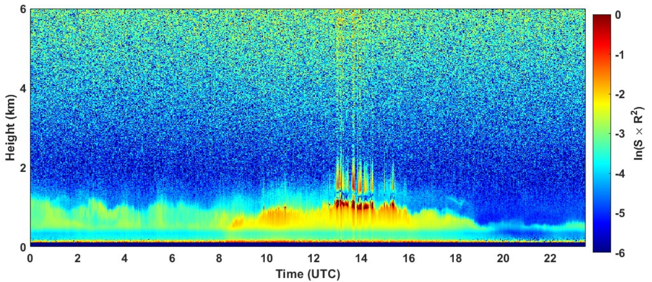
2022-01-14 RCS quick look CHM15k - ILVA LIDAR1 DIREZIONE
