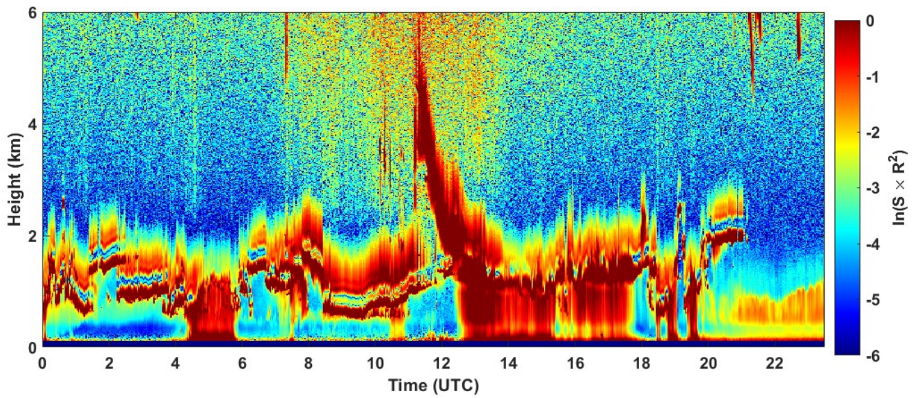
2022-01-10 RCS quick look CHM15k - ILVA LIDAR1 DIREZIONE
