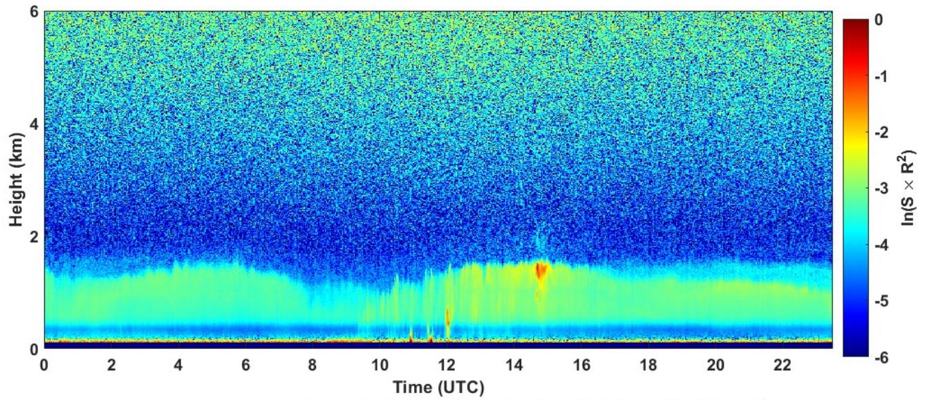
2022-01-20 RCS quick look CHM15k - ILVA LIDAR1 DIREZIONE
