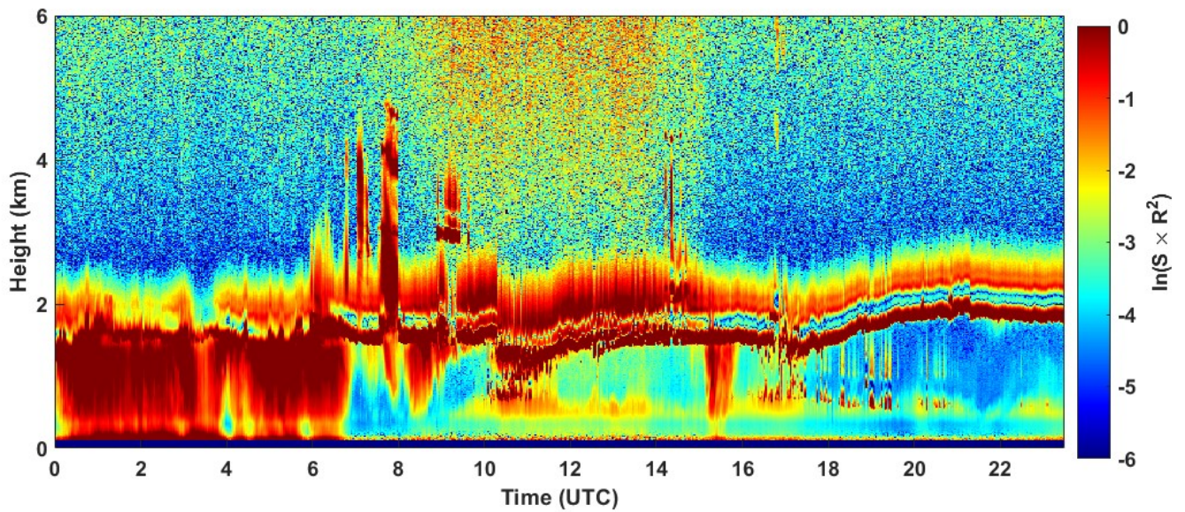
2022-01-08 RCS quick look CHM15k - ILVA LIDAR1 DIREZIONE
