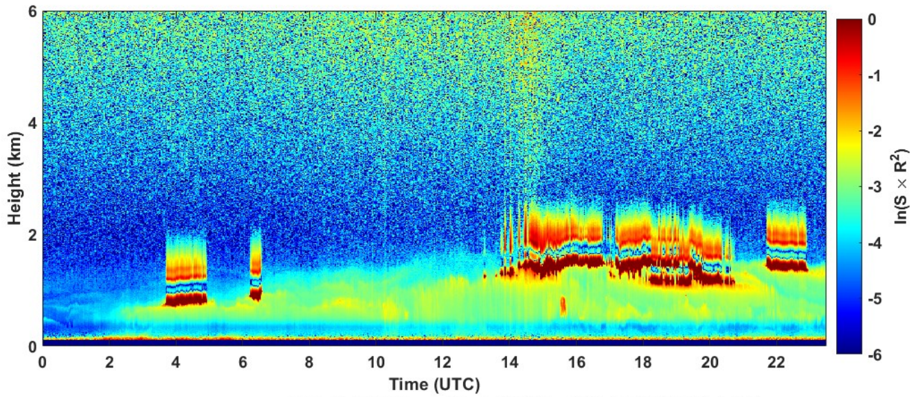
2022-01-04 RCS quick look CHM15k - ILVA LIDAR1 DIREZIONE
