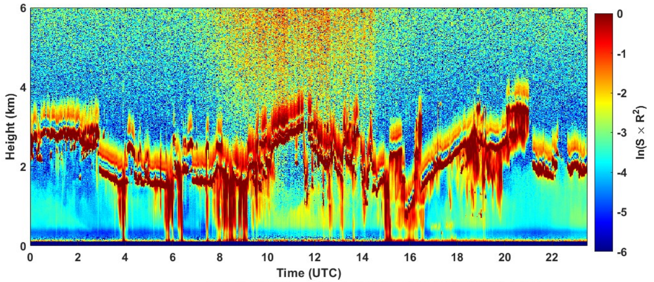
2022-01-22 RCS quick look CHM15k - ILVA LIDAR1 DIREZIONE
