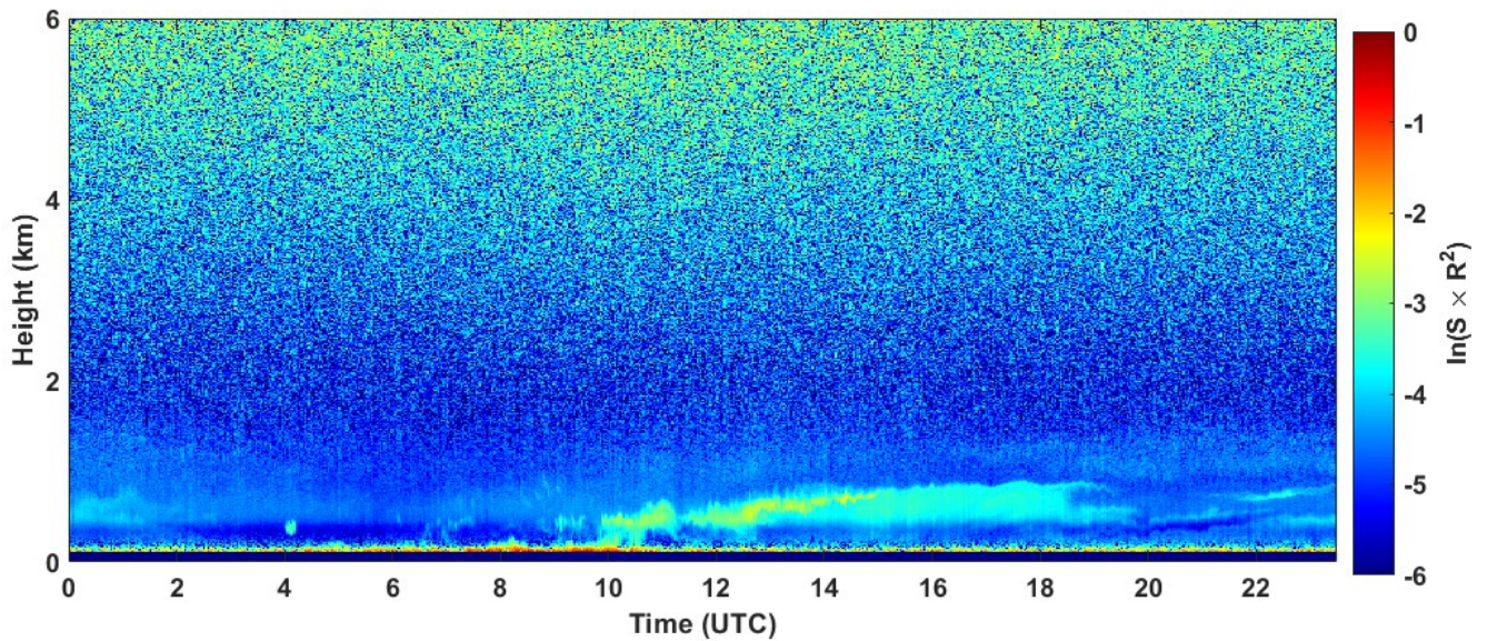
2022-01-02 RCS quick look CHM15k - ILVA LIDAR1 DIREZIONE
