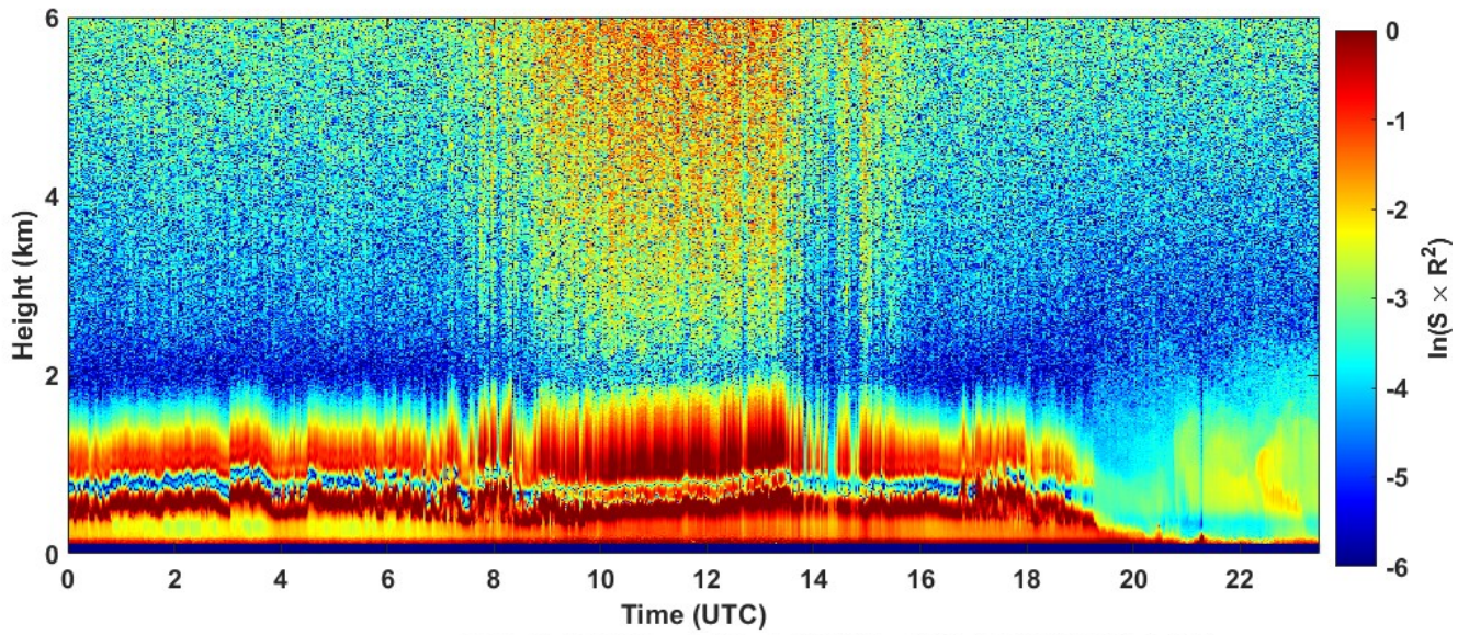
2022-01-06 RCS quick look CHM15k - ILVA LIDAR1 DIREZIONE
