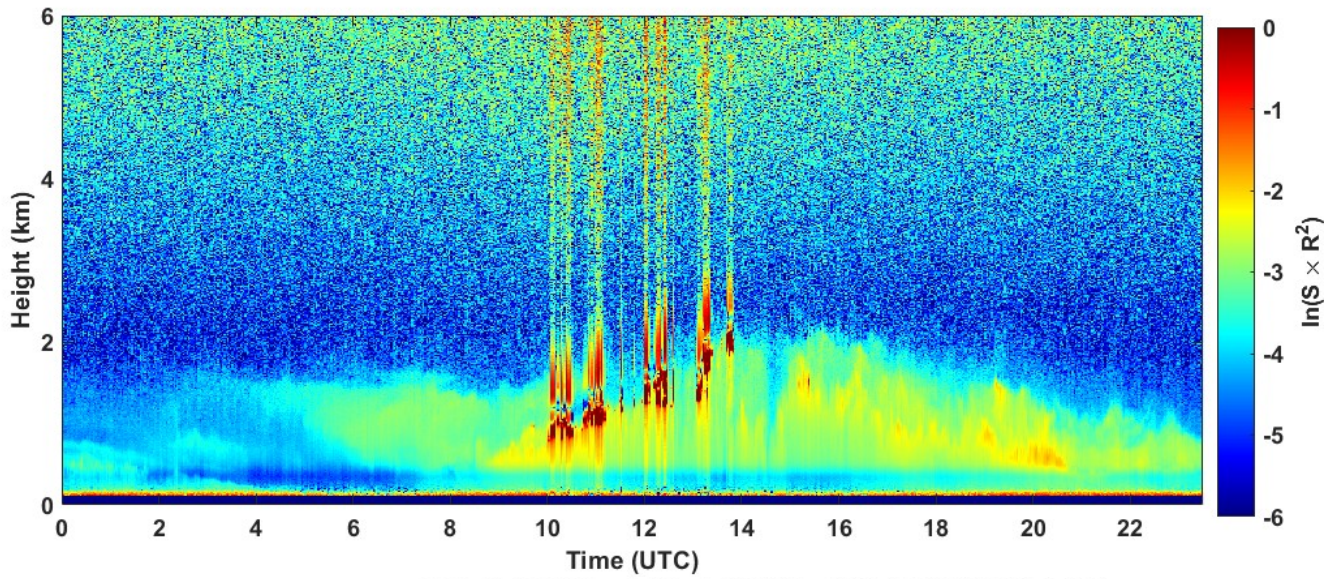
2022-01-18 RCS quick look CHM15k - ILVA LIDAR1 DIREZIONE
