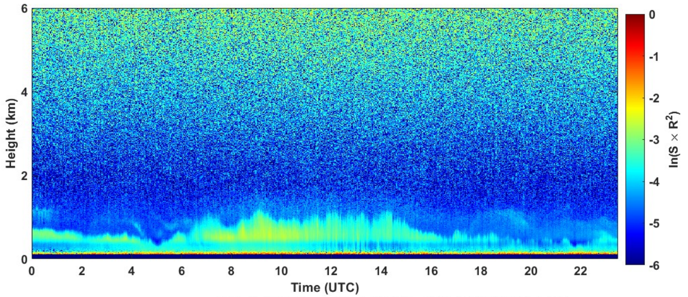
2022-01-16 RCS quick look CHM15k - ILVA LIDAR1 DIREZIONE
