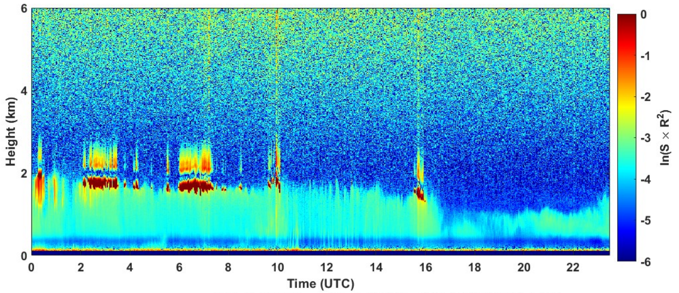
2022-01-26 RCS quick look CHM15k - ILVA LIDAR1 DIREZIONE
