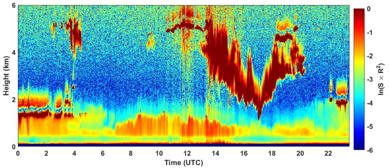
2022-01-12 RCS quick look CHM15k - ILVA LIDAR1 DIREZIONE
