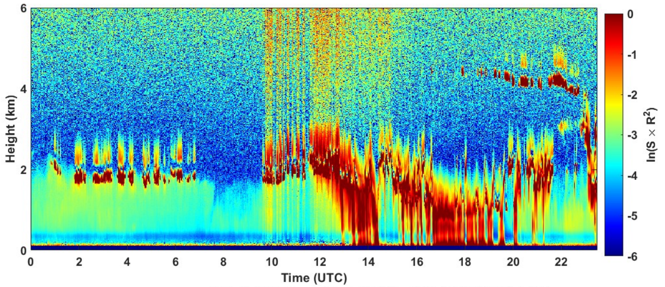
2022-01-24 RCS quick look CHM15k - ILVA LIDAR1 DIREZIONE
