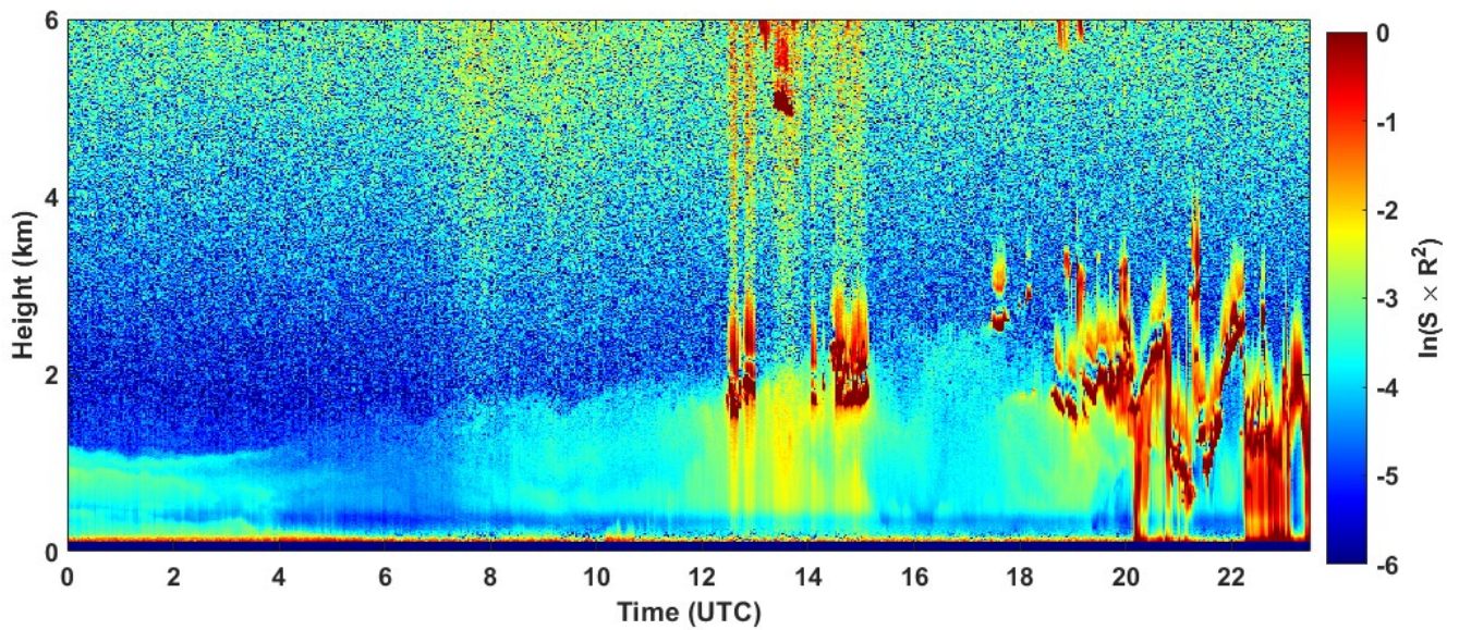
2022-01-28 RCS quick look CHM15k - ILVA LIDAR1 DIREZIONE
