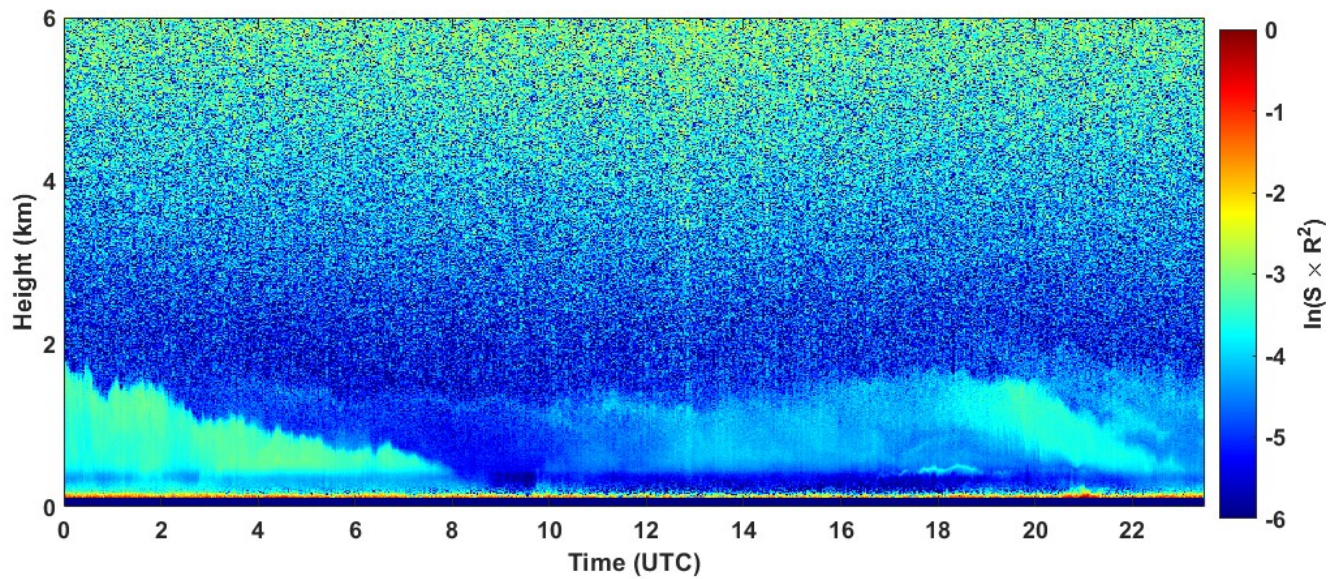
2022-01-30 RCS quick look CHM15k - ILVA LIDAR1 DIREZIONE
