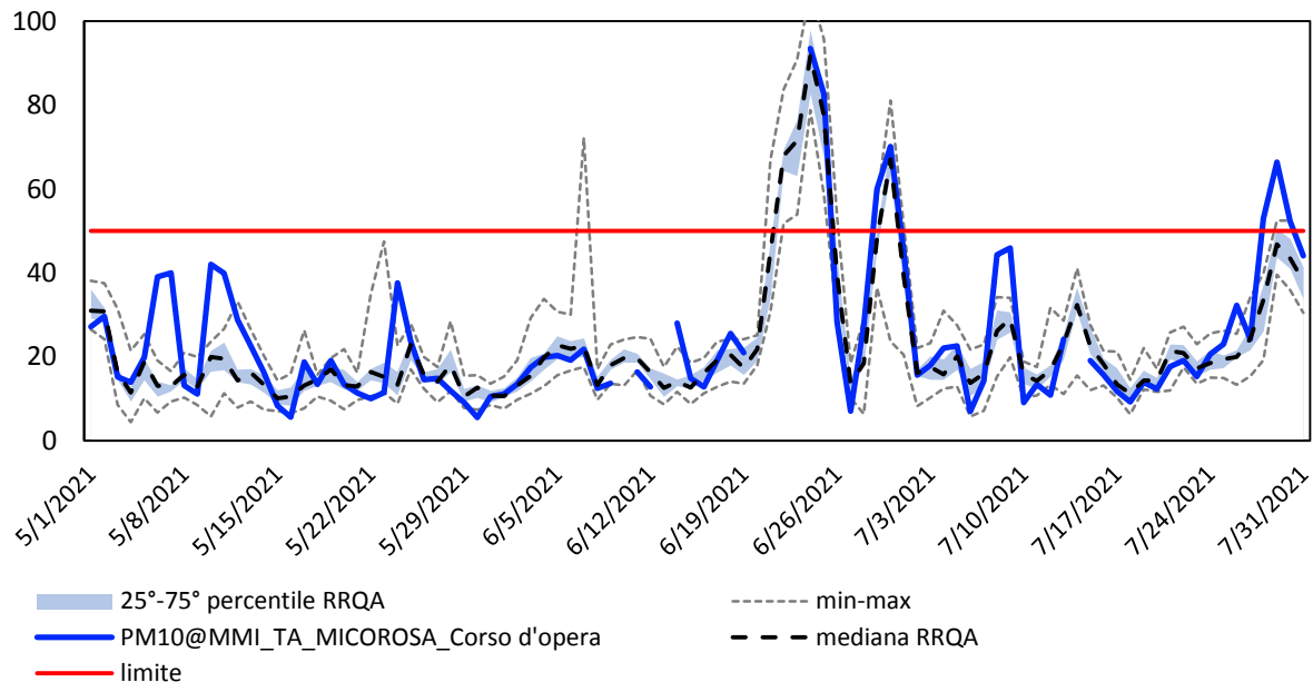
Figura 14: Andamento giornaliero del PM 10 (µg/m 3 ) misurato a Brindisi nel periodo oggetto della campagna.
