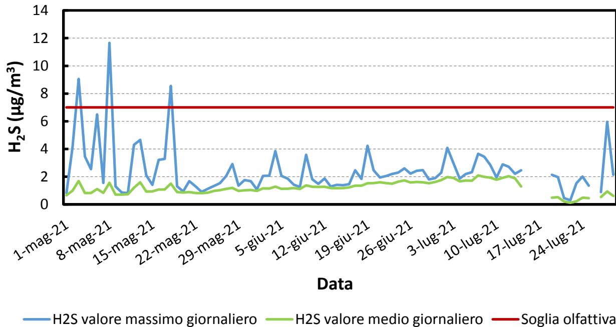
Figura 27: Andamento della concentrazione massima oraria e media giornaliera di H 2 S (µg/m 3 ), misurata presso il sito oggetto della campagna.
