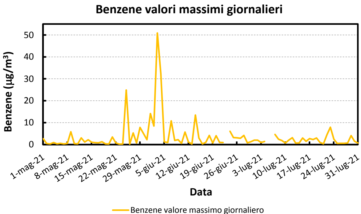
Figura 25: Andamento della concentrazione media e massima giornaliera, per il benzene ( \mu\text{g}/\text{m}^3 ), misurate presso il sito oggetto della campagna.
