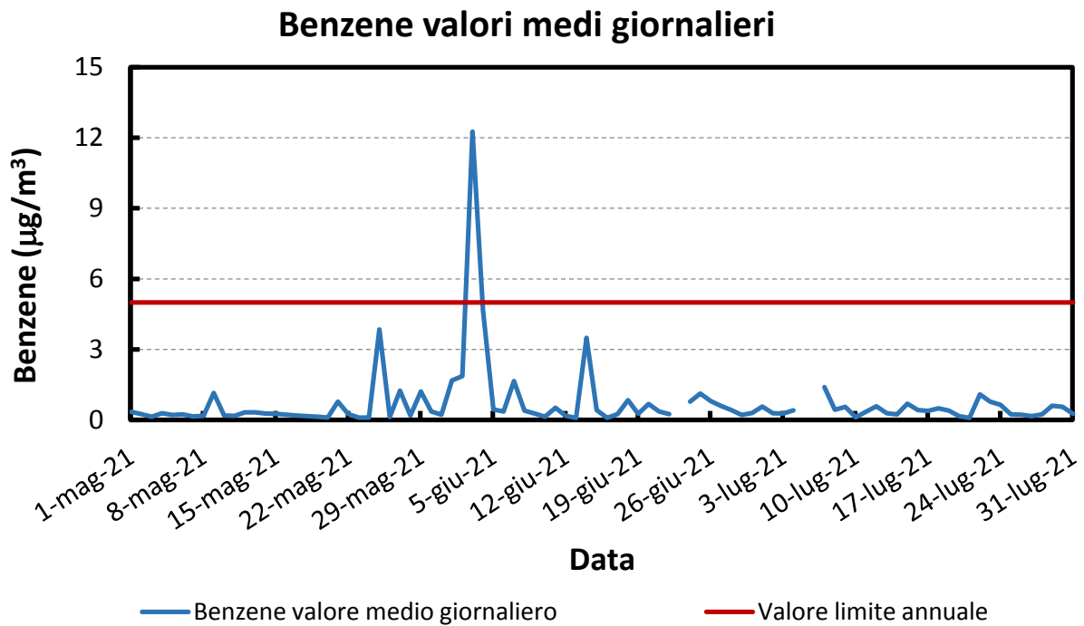
Figura 24: Andamento della concentrazione media e massima giornaliera, per il benzene ( \mu\text{g}/\text{m}^3 ), misurate presso il sito oggetto della campagna.
