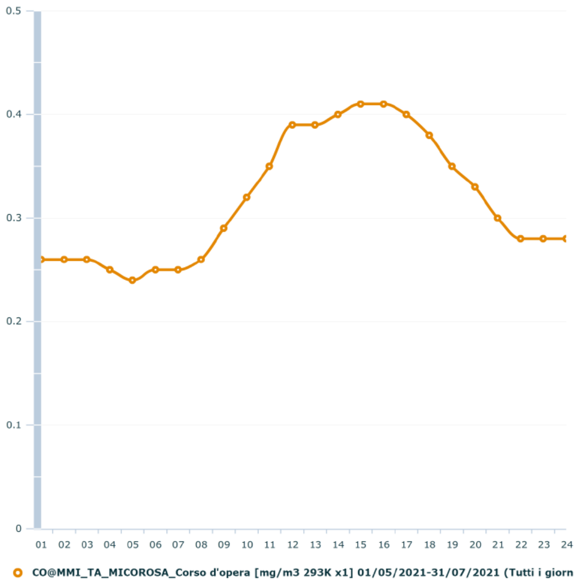
Figura 7: Grafico del giorno tipo per l'inquinante CO.
