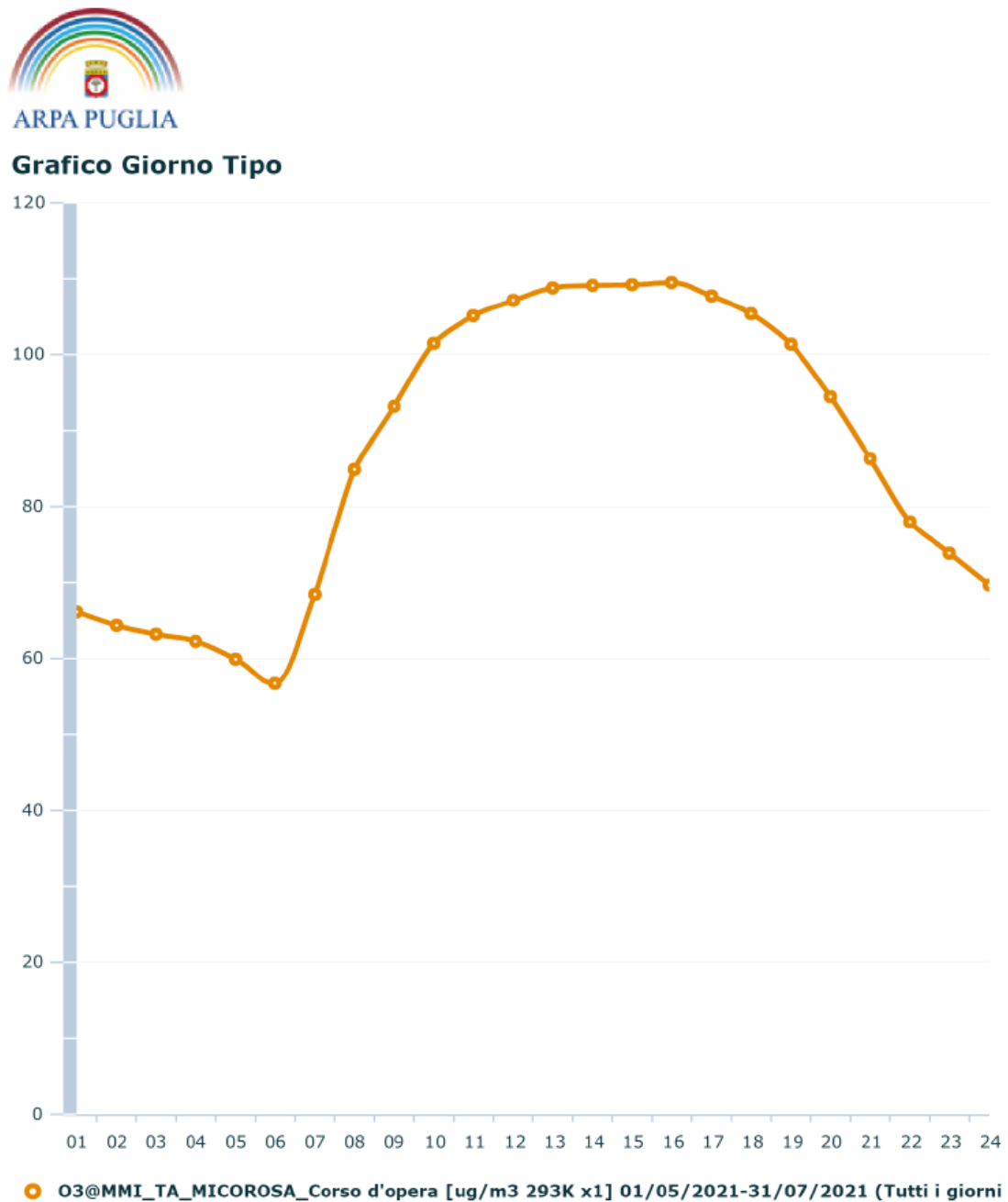
Figura 8: Grafico del giorno tipo per l'inquinante O 3 .
