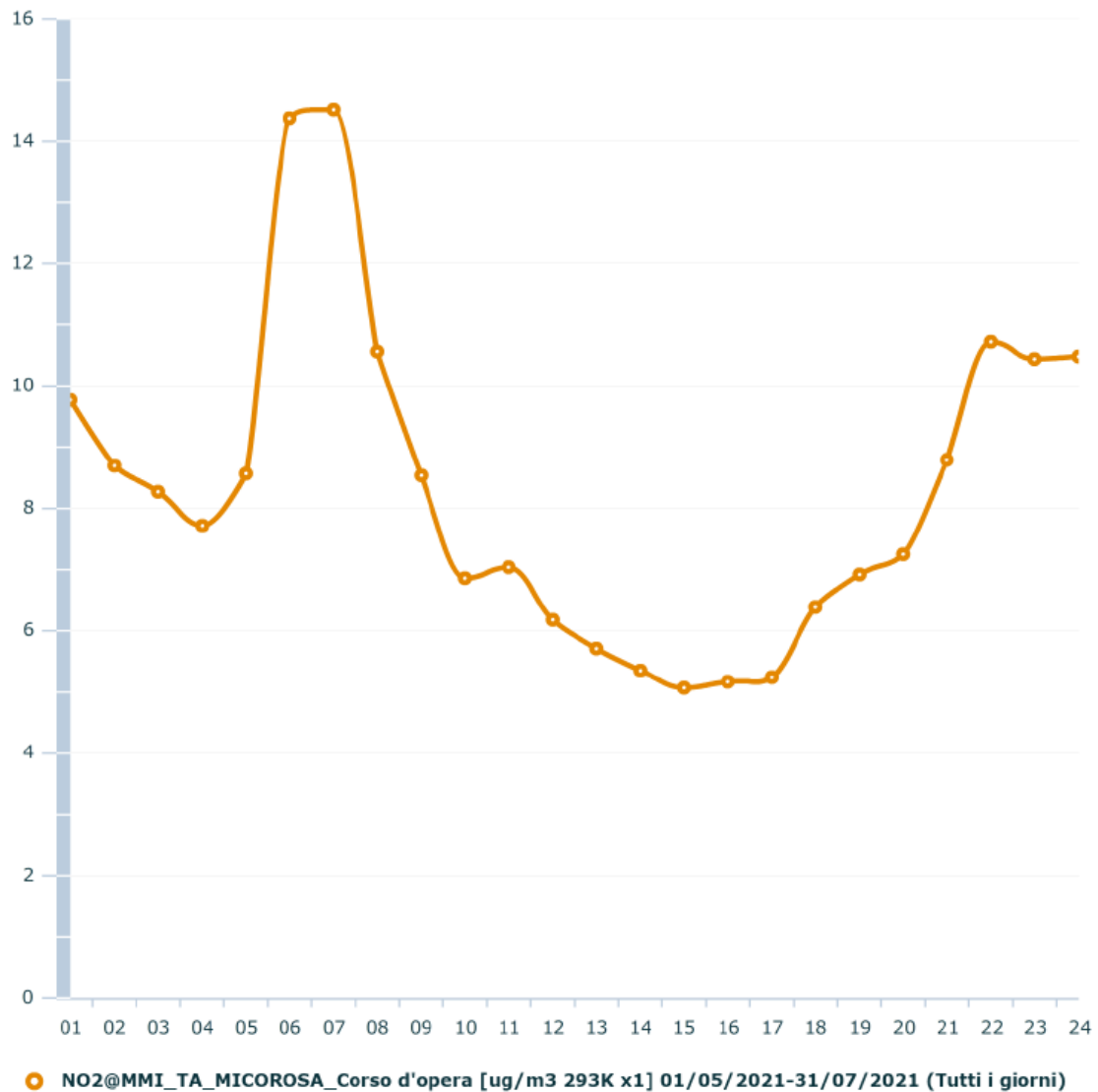
Figura 6: Grafico del giorno tipo per l'inquinante NO 2 .
