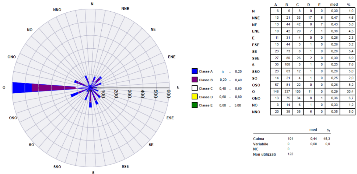
Figura 23: Rosa dell'inquinamento per l'inquinante monossido di carbonio.
