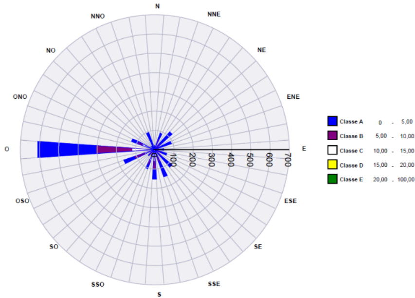
Figura 19: Rosa dell'inquinamento per l'inquinante biossido di azoto.
