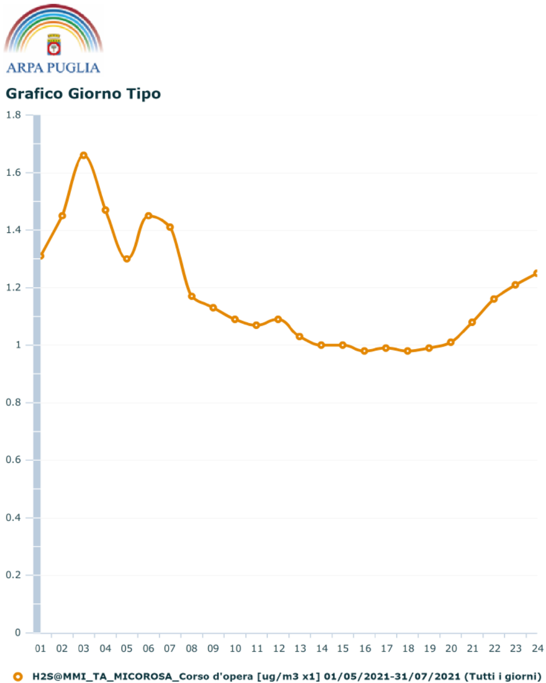
Figura 12: Grafico del giorno tipo per l'inquinante acido solfidrico.
