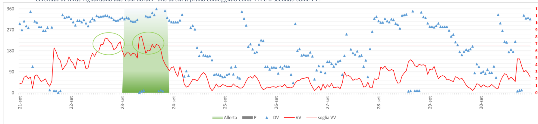
Figura 4: Velocità del vento (linea rossa, asse a destra, in m/s), direzione del vento (triangoli blu, asse a sinistra), precipitazione cumulata oraria (istogramma in grigio, stesso asse a destra della velocità del vento, in mm/h). Il giorno interessato dall'allerta è riportato come area verde; la soglia di identificazione per la velocità del vento è riportata come linea orizzontale rossa.
