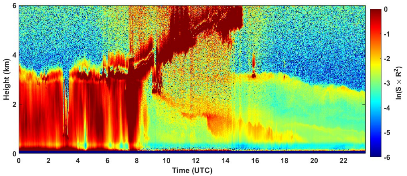
2021-09-12 RCS quick look CHM15k - ILVA LIDAR1 DIREZIONE
