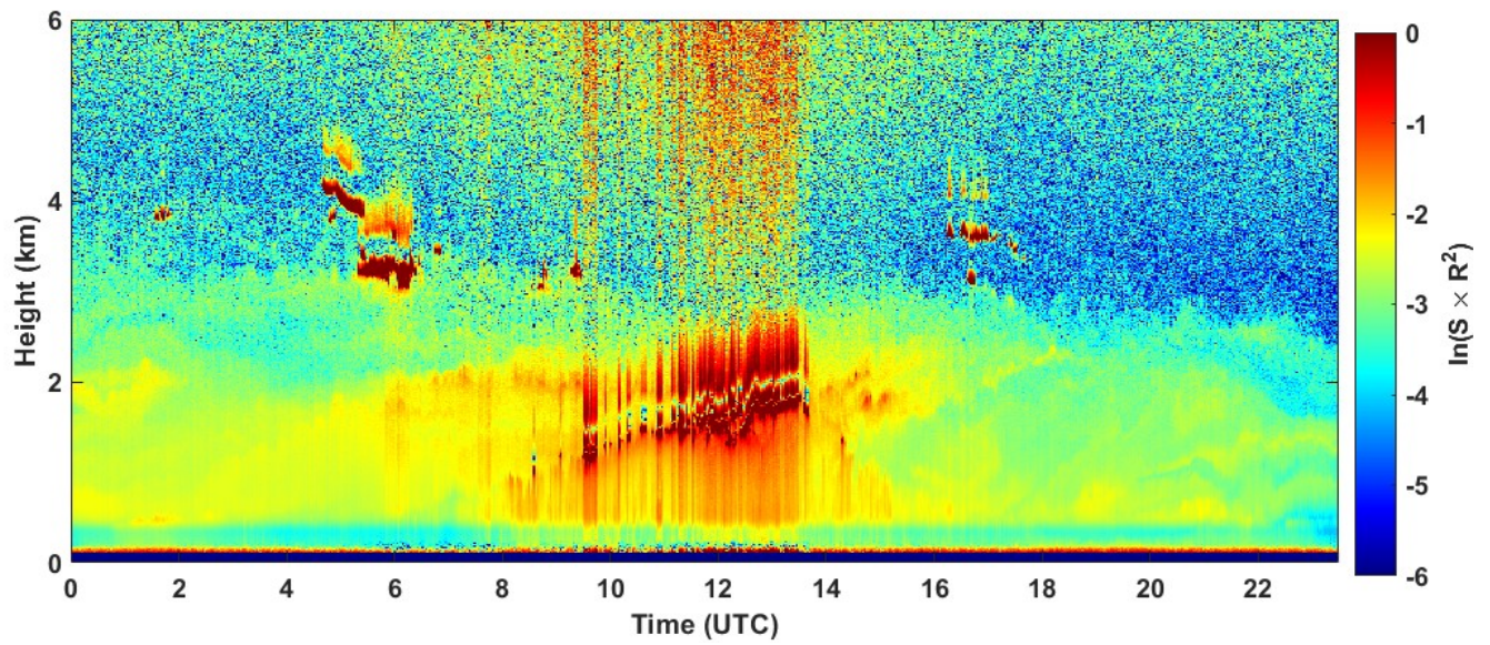
2021-09-28 RCS quick look CHM15k - ILVA LIDAR1 DIREZIONE
