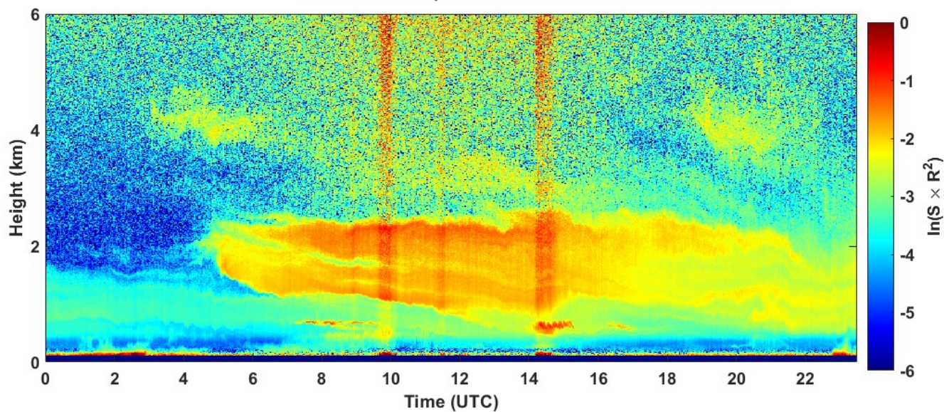
2021-09-26 RCS quick look CHM15k - ILVA LIDAR1 DIREZIONE
