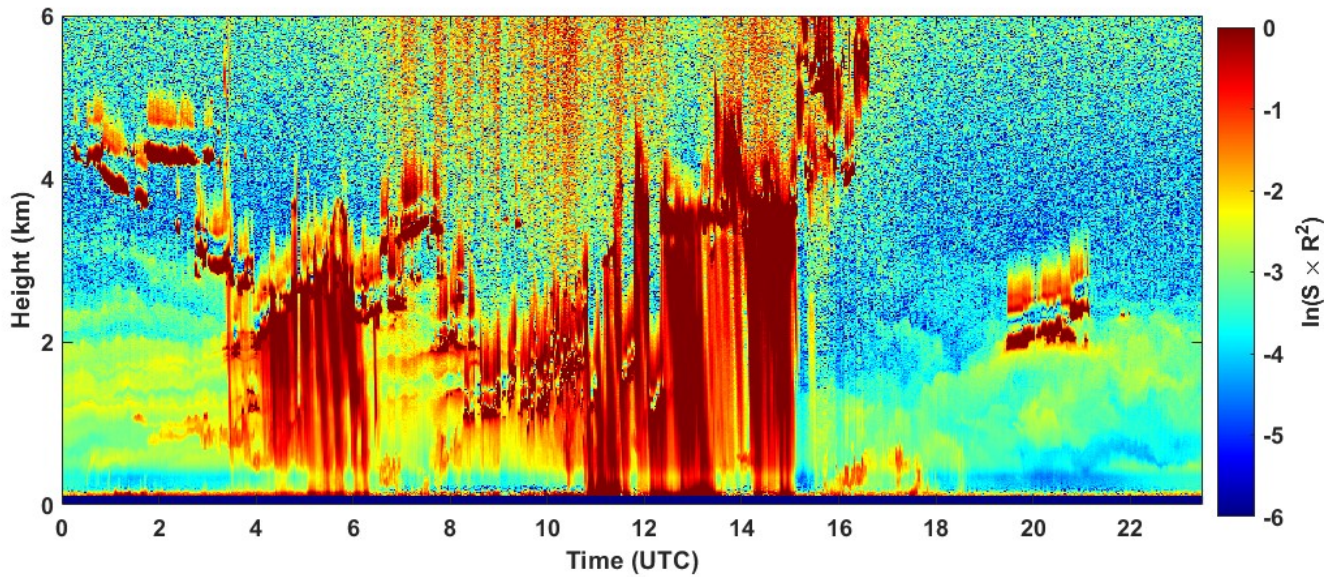
2021-09-06 RCS quick look CHM15k - ILVA LIDAR1 DIREZIONE
