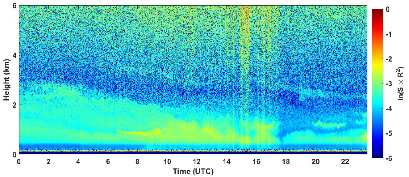
2021-09-10 RCS quick look CHM15k - ILVA LIDAR1 DIREZIONE
