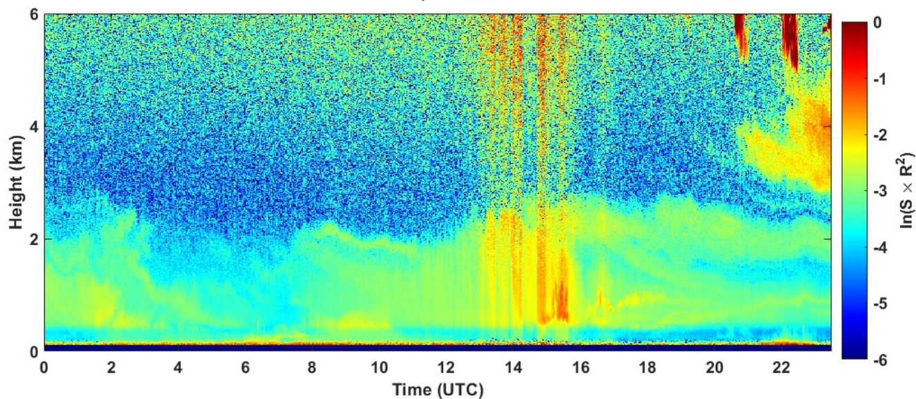
2021-09-16 RCS quick look CHM15k - ILVA LIDAR1 DIREZIONE
