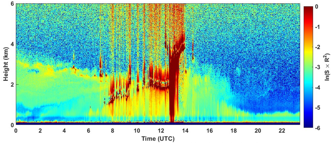
2021-09-02 RCS quick look CHM15k - ILVA LIDAR1 DIREZIONE
