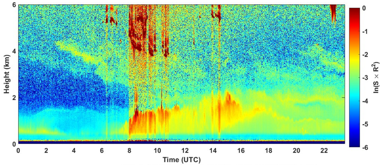
2021-09-04 RCS quick look CHM15k - ILVA LIDAR1 DIREZIONE
