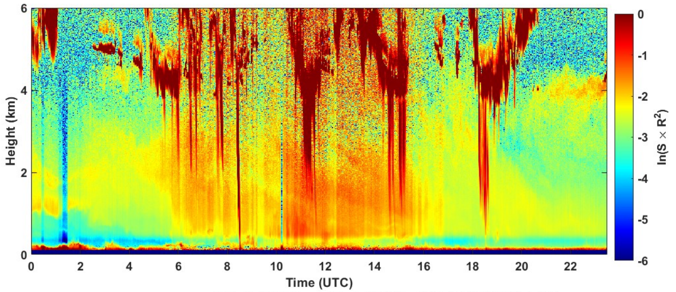
2021-09-18 RCS quick look CHM15k - ILVA LIDAR1 DIREZIONE
