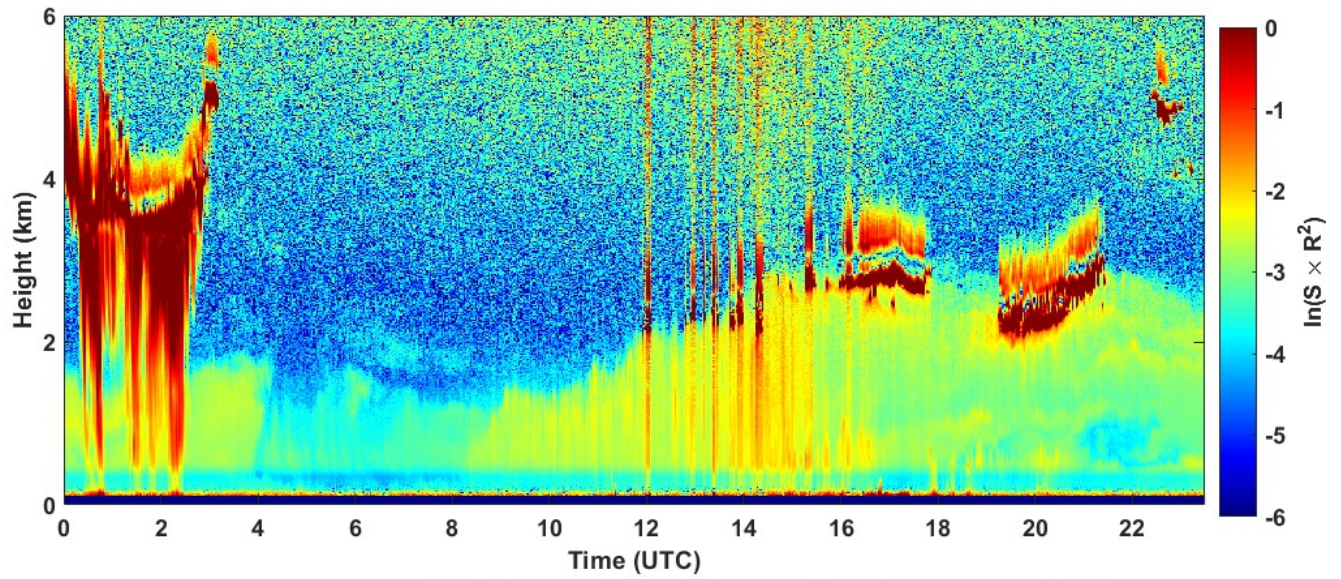
2021-09-22 RCS quick look CHM15k - ILVA LIDAR1 DIREZIONE
