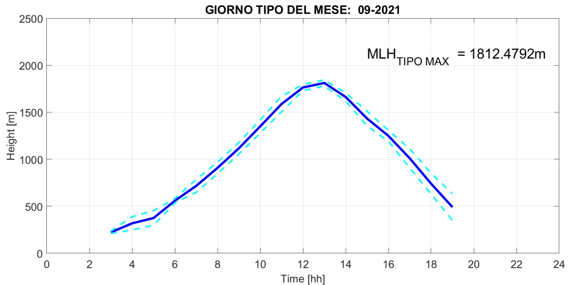
Fig. 2: Giorno tipo del parametro Mixing Layer Height nel mese di SETTEMBRE 2021, rappresentato mediante media oraria (linea blu continua) e deviazione standard (linee celesti tratteggiate).
