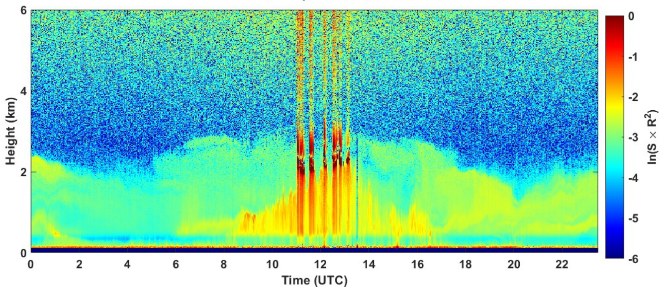
2021-09-14 RCS quick look CHM15k - ILVA LIDAR1 DIREZIONE
