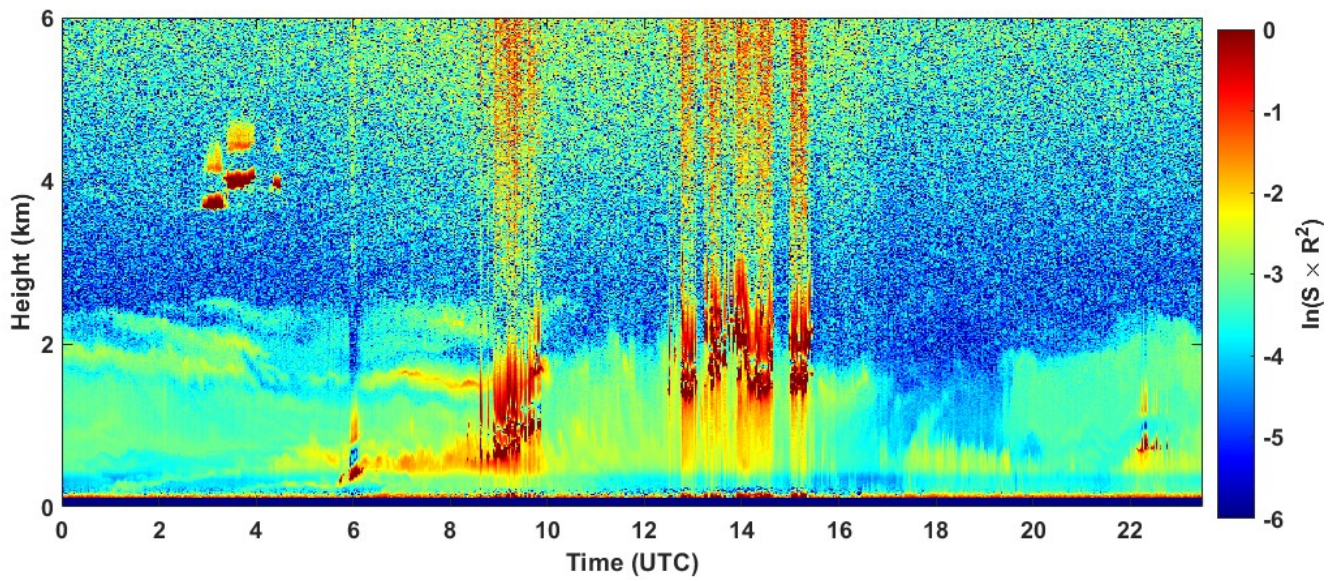
2021-09-30 RCS quick look CHM15k - ILVA LIDAR1 DIREZIONE
