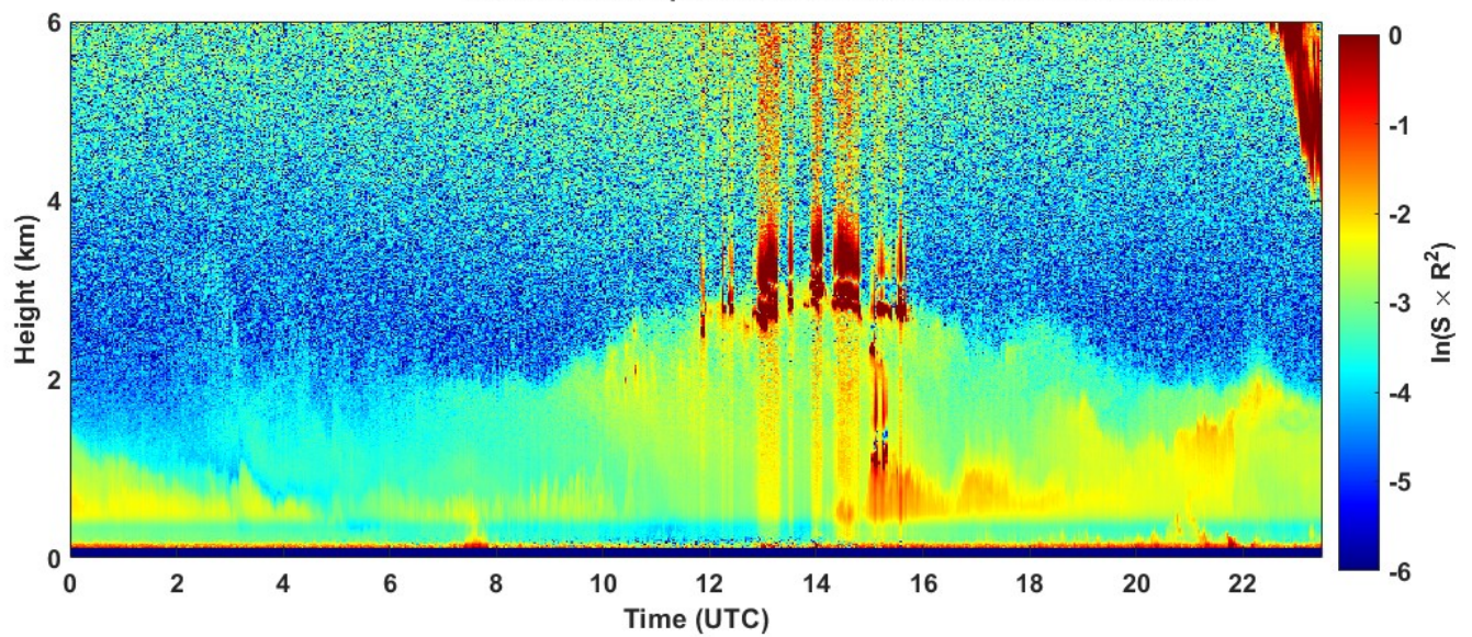
2021-09-20 RCS quick look CHM15k - ILVA LIDAR1 DIREZIONE
