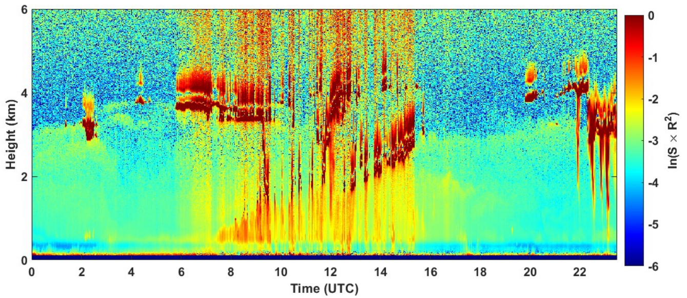
2021-09-08 RCS quick look CHM15k - ILVA LIDAR1 DIREZIONE
