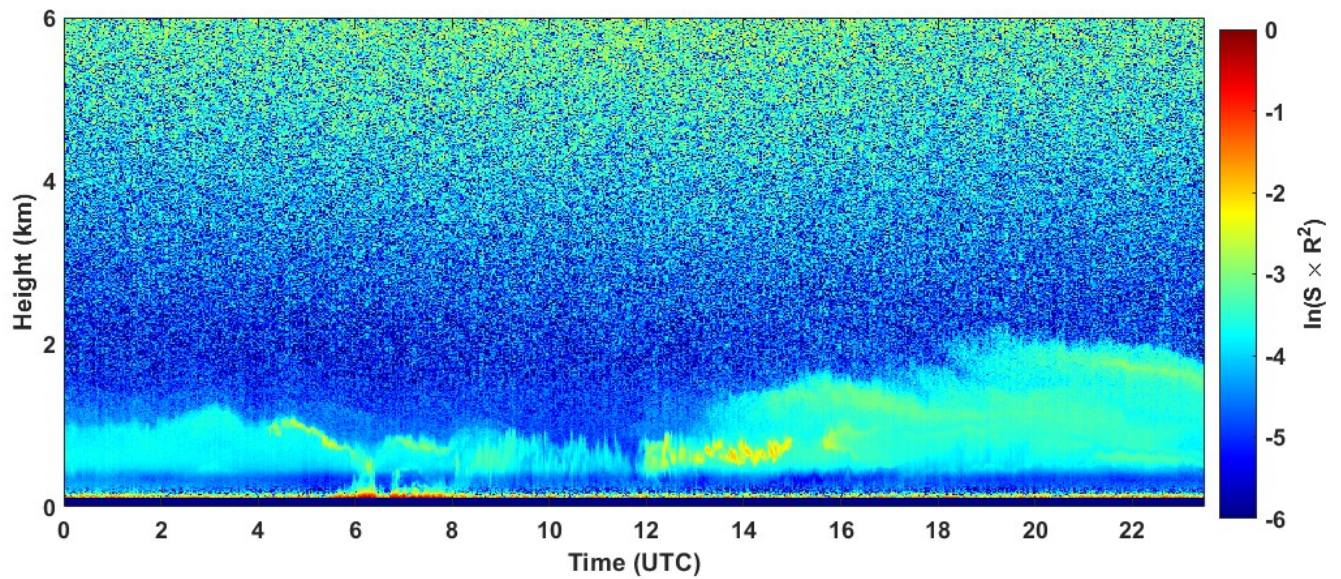
2021-09-24 RCS quick look CHM15k - ILVA LIDAR1 DIREZIONE
