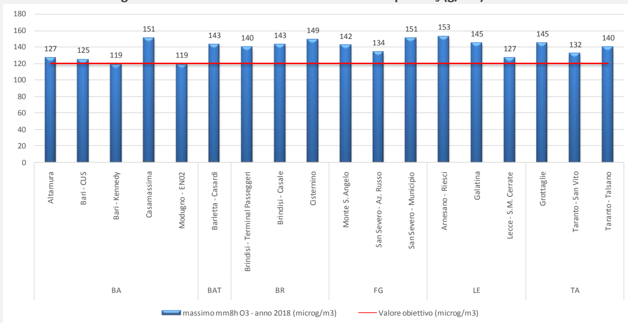
Fig. 1 - Massimo della media mobile sulle 8 ore per l'O 3 (g/m 3 ) - 2018
