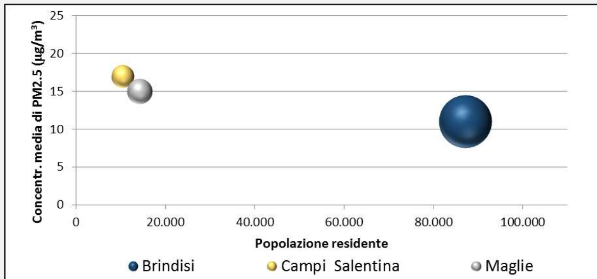
Fig. 1 - Esposizione della popolazione al PM 2.5 (µg/m 3 ) nei comuni coperti dall'indagine. Anno 2018
