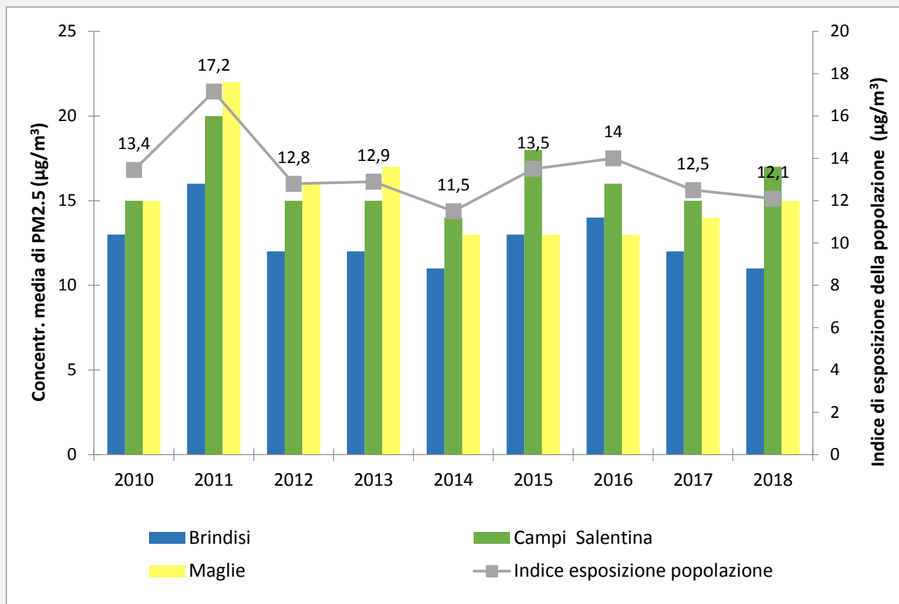
Fig. 2 - Concentrazione media di PM 2.5 (µg/m 3 ) nei comuni coperti dall'indagine e Indice di esposizione della popolazione generale. Anni 2010-2018
