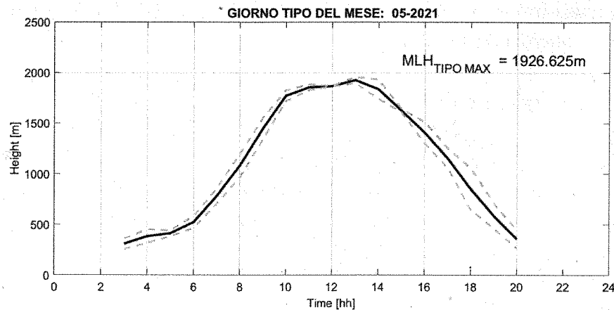
Fig. 2: Giorno tipo del parametro Mixing Layer Height nel mese di MAGGIO 2021, rappresentato mediante media oraria (linea blu continua) e deviazione standard (linee celesti tratteggiate).
