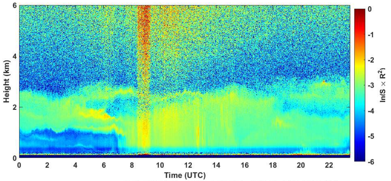
2021-05-30 RCS quick look CHM15k - ILVA LIDAR1 DIREZIONE
