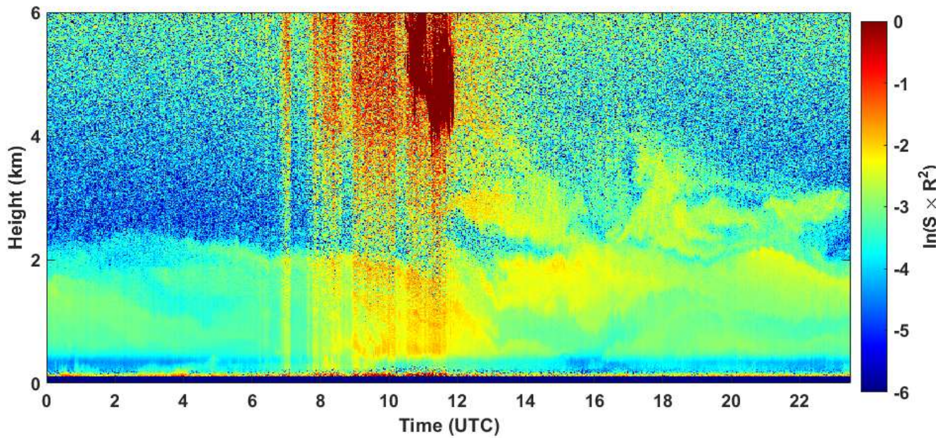
2021-05-28 RCS quick look CHM15k - ILVA LIDAR1 DIREZIONE
