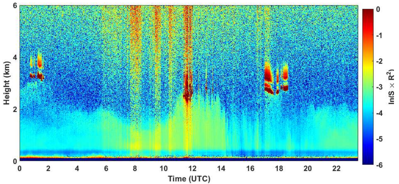
2021-05-18 RCS quick look CHM15k - ILVA LIDAR1 DIREZIONE
