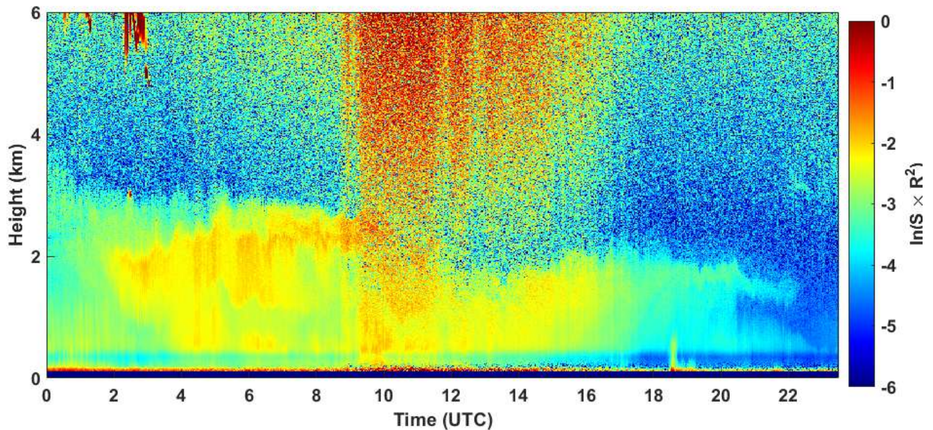
2021-05-02 RCS quick look CHM15k - ILVA LIDAR1 DIREZIONE
