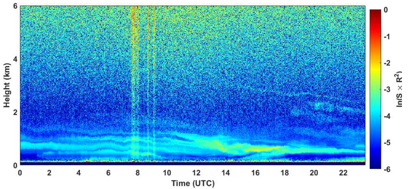
2021-05-10 RCS quick look CHM15k - ILVA LIDAR1 DIREZIONE
