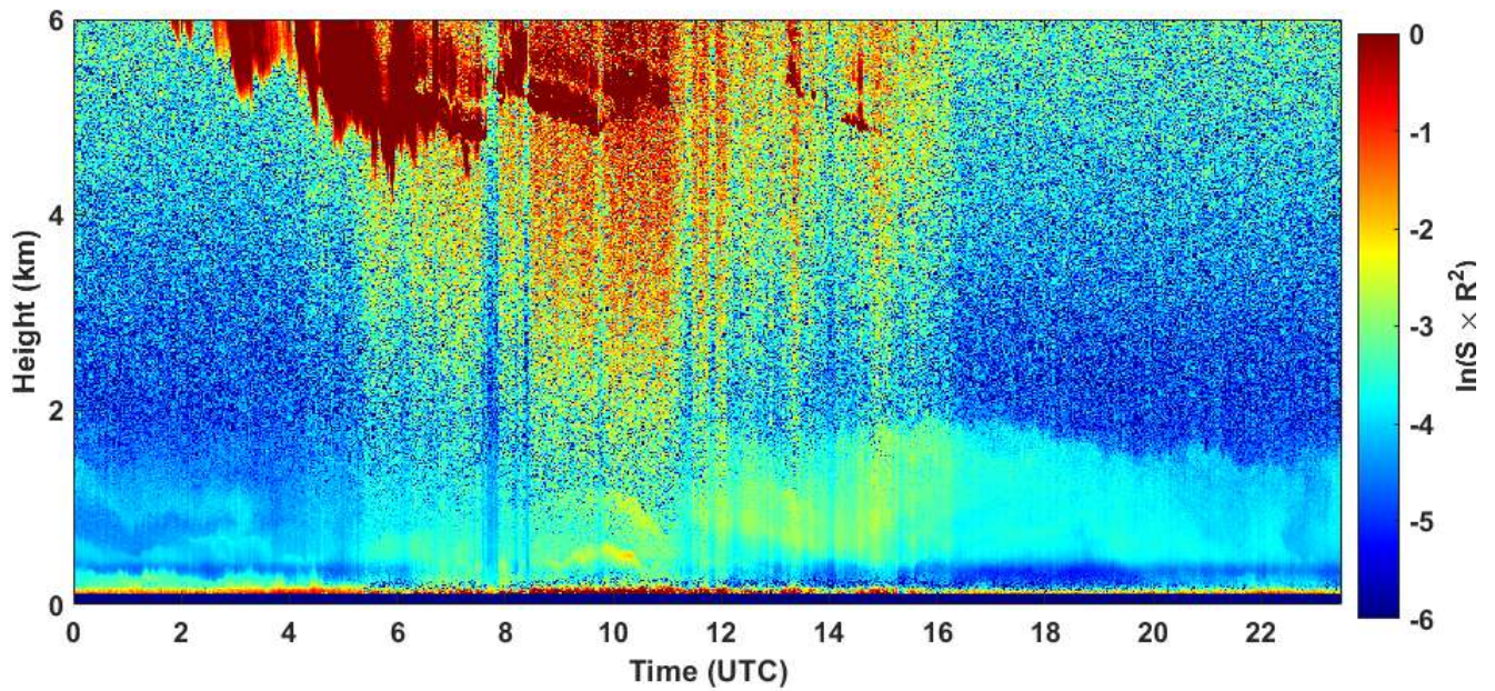
2021-05-08 RCS quick look CHM15k - ILVA LIDAR1 DIREZIONE
