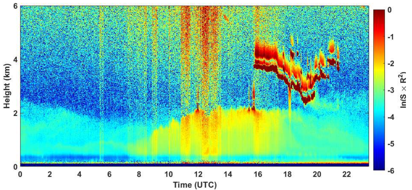
2021-05-16 RCS quick look CHM15k - ILVA LIDAR1 DIREZIONE
