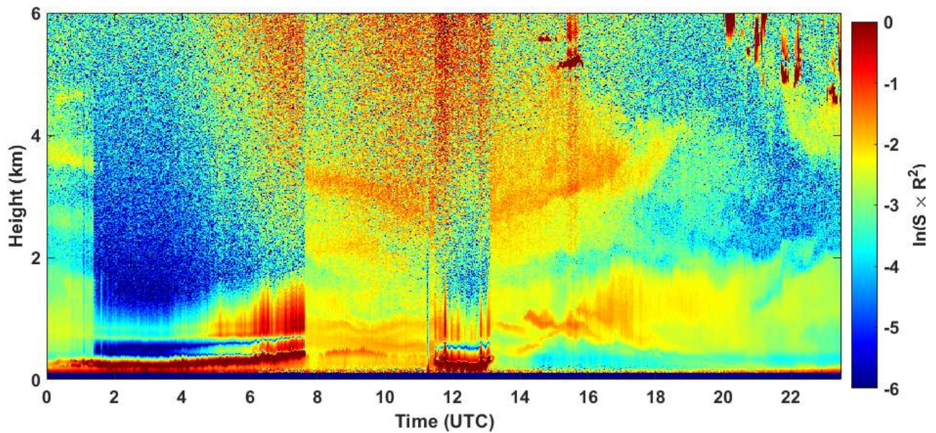
2021-05-24 RCS quick look CHM15k - ILVA LIDAR1 DIREZIONE
