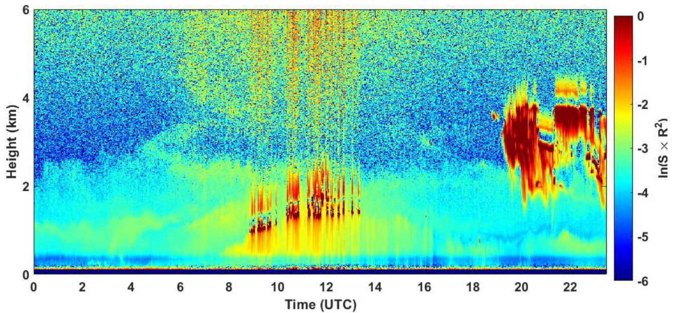
2021-03-06 RCS quick look CHM15k - ILVA LIDAR1 DIREZIONE
