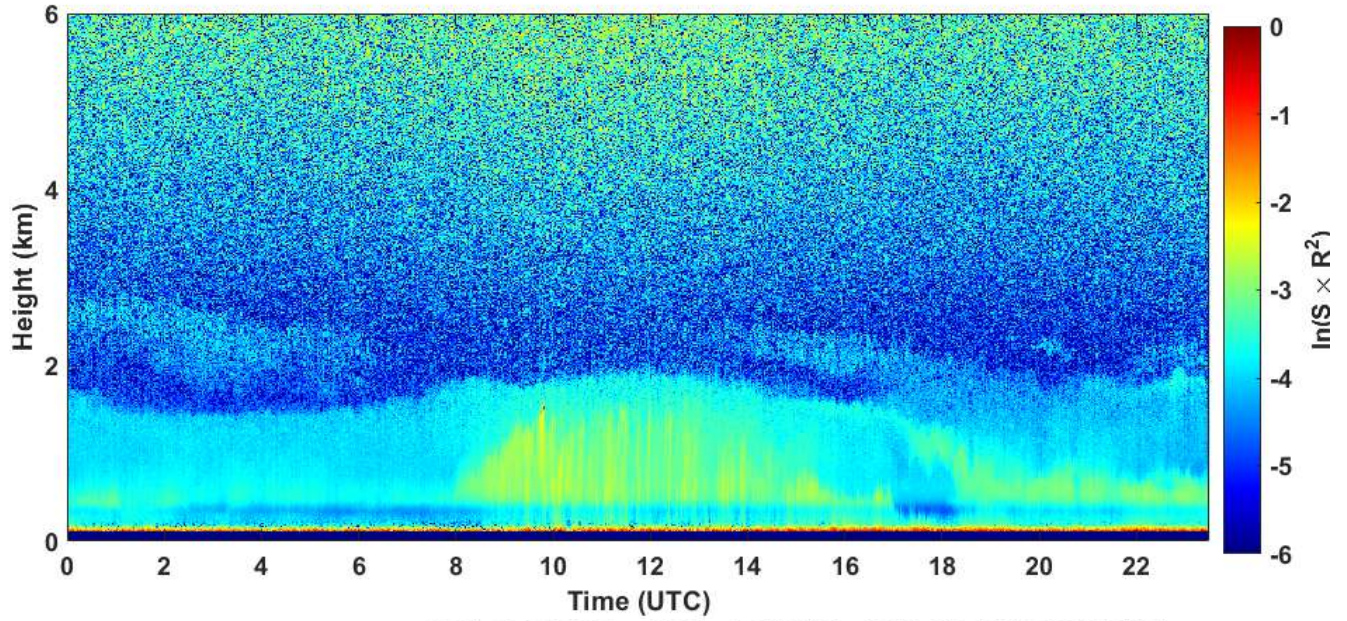
2021-03-02 RCS quick look CHM15k - ILVA LIDAR1 DIREZIONE
