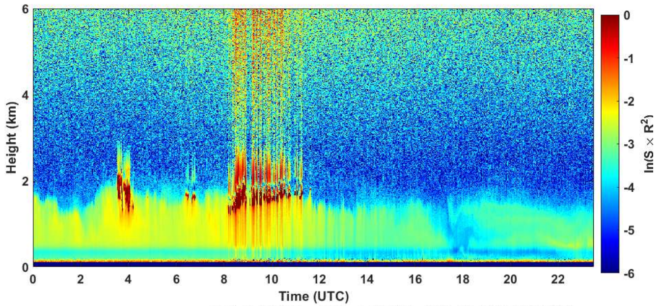
2021-03-12 RCS quick look CHM15k - ILVA LIDAR1 DIREZIONE
