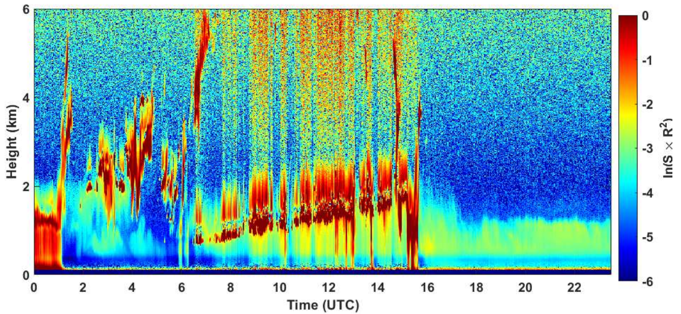
2021-03-16 RCS quick look CHM15k - ILVA LIDAR1 DIREZIONE
