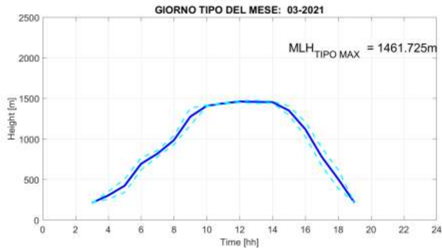
Fig. 2: Giorno tipo del parametro Mixing Layer Height nel mese di MARZO 2021, rappresentato mediante media oraria (linea blu continua) e deviazione standard (linee celesti tratteggiate).
