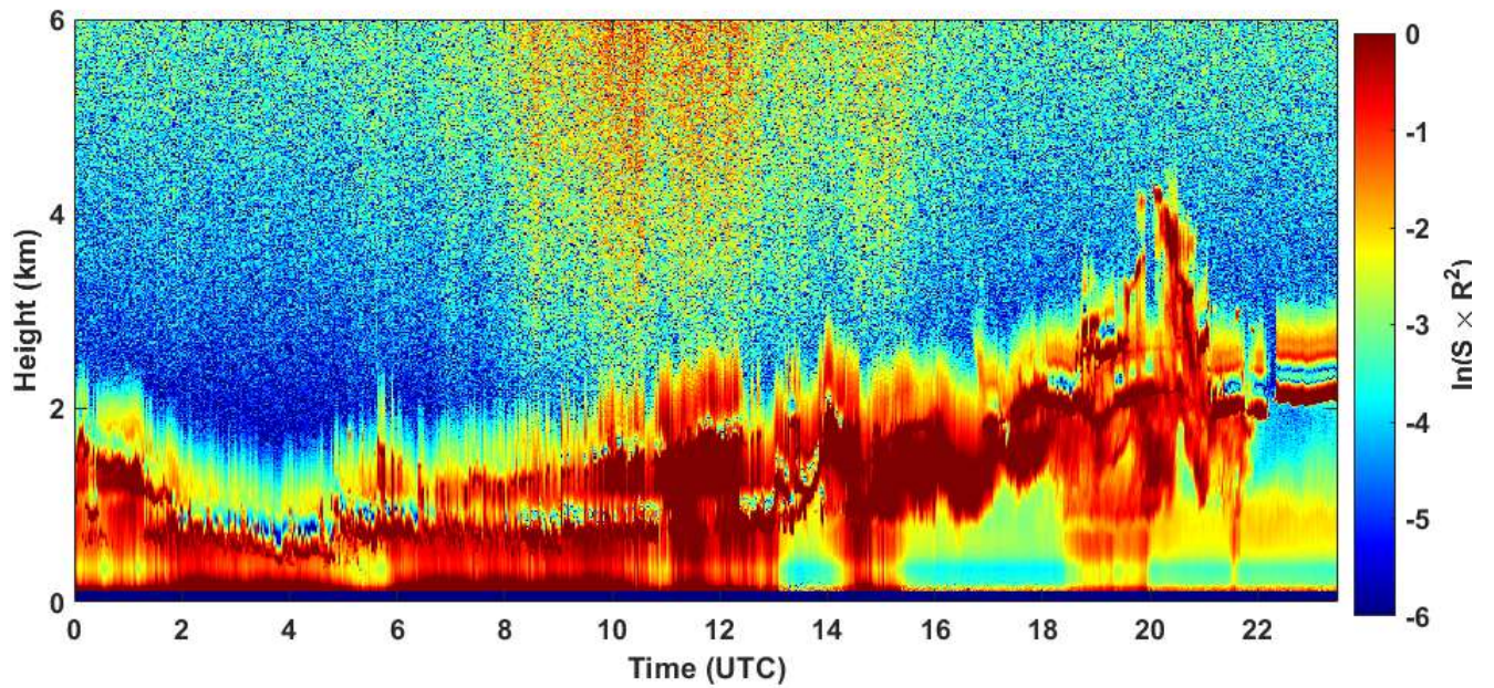
2021-03-22 RCS quick look CHM15k - ILVA LIDAR1 DIREZIONE
