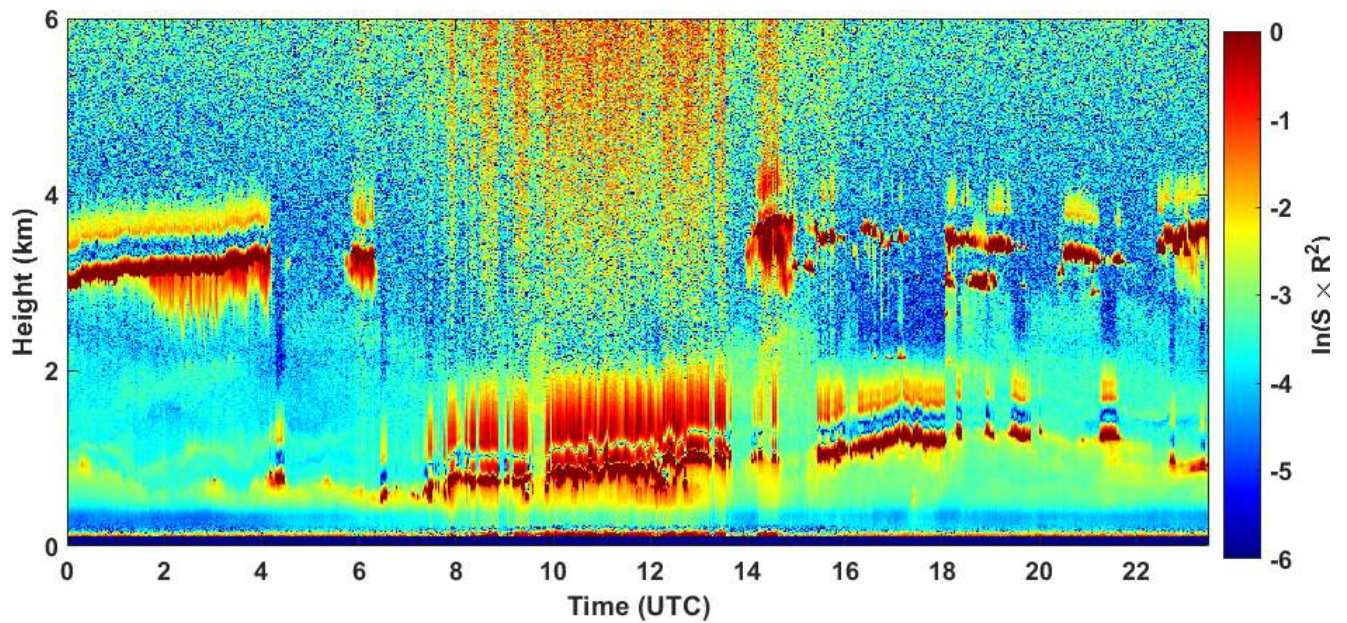
2021-03-08 RCS quick look CHM15k - ILVA LIDAR1 DIREZIONE
