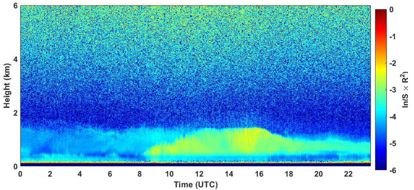
2021-03-04 RCS quick look CHM15k - ILVA LIDAR1 DIREZIONE
