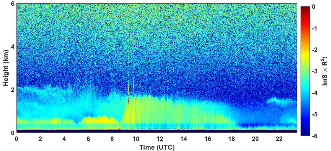
2021-03-02 RCS quick look CHM15k - ILVA LIDAR1 DIREZIONE
