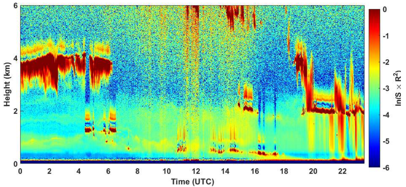
2021-03-10 RCS quick look CHM15k - ILVA LIDAR1 DIREZIONE
