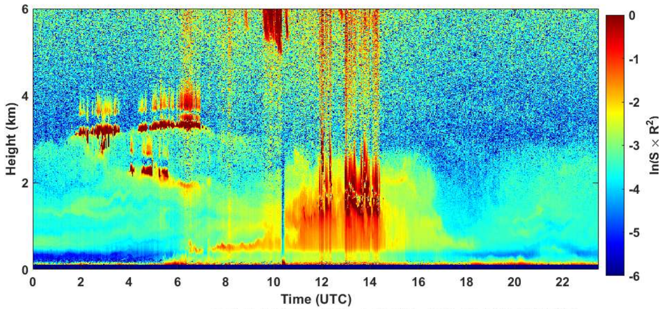
2021-03-30 RCS quick look CHM15k - ILVA LIDAR1 DIREZIONE
