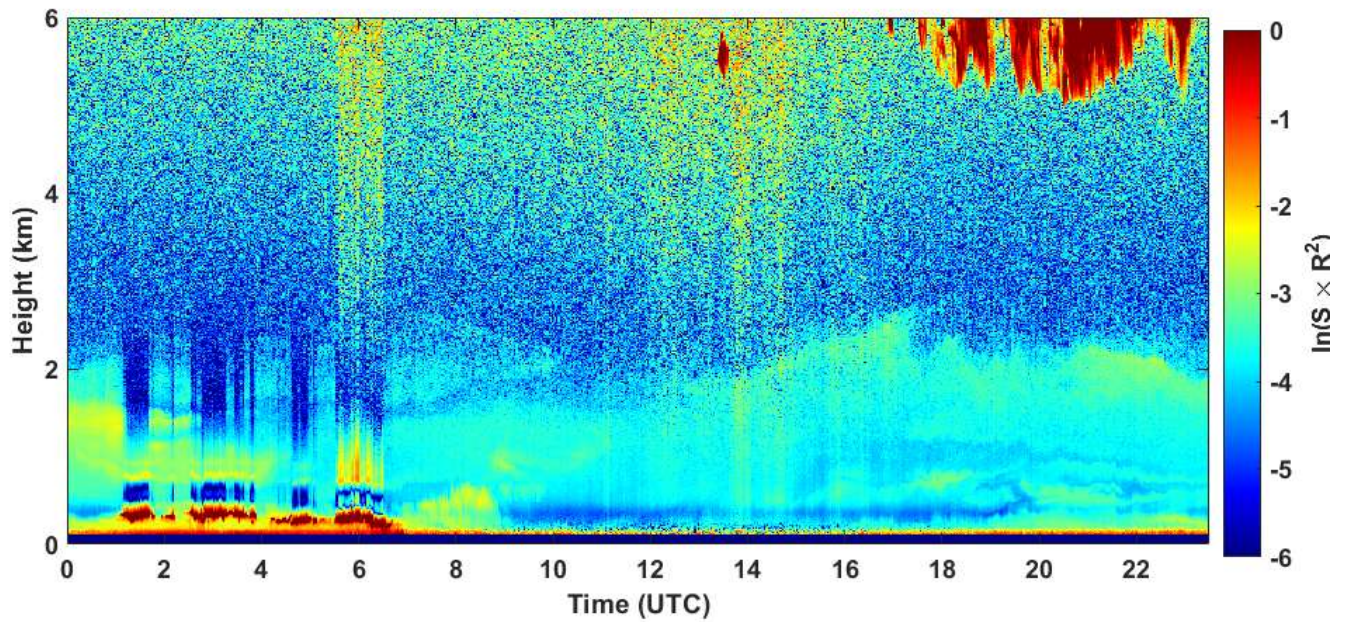
2021-03-28 RCS quick look CHM15k - ILVA LIDAR1 DIREZIONE
