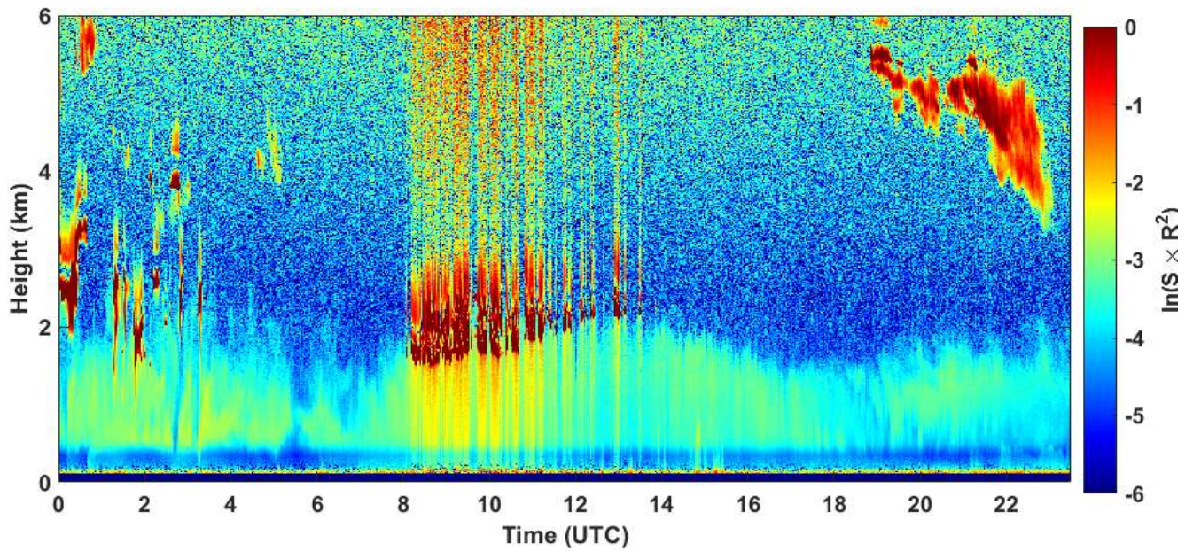
2021-03-18 RCS quick look CHM15k - ILVA LIDAR1 DIREZIONE
