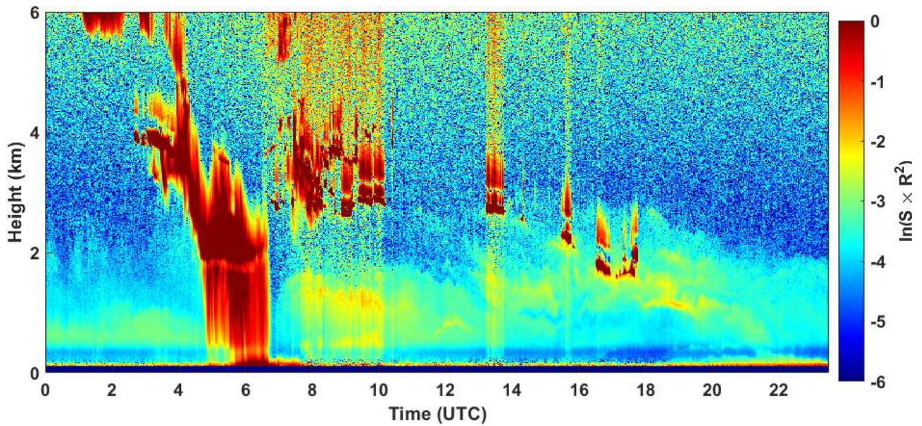
2021-03-14 RCS quick look CHM15k - ILVA LIDAR1 DIREZIONE
