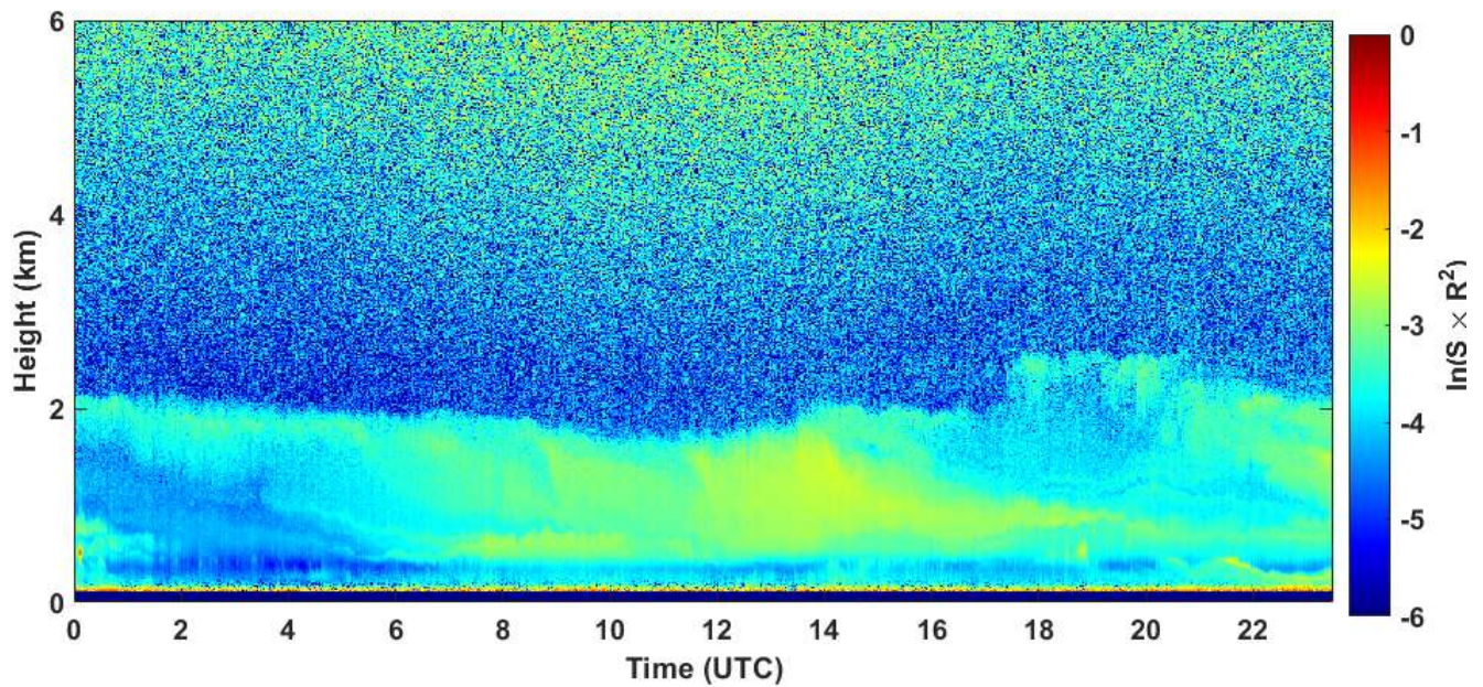
2021-03-26 RCS quick look CHM15k - ILVA LIDAR1 DIREZIONE
