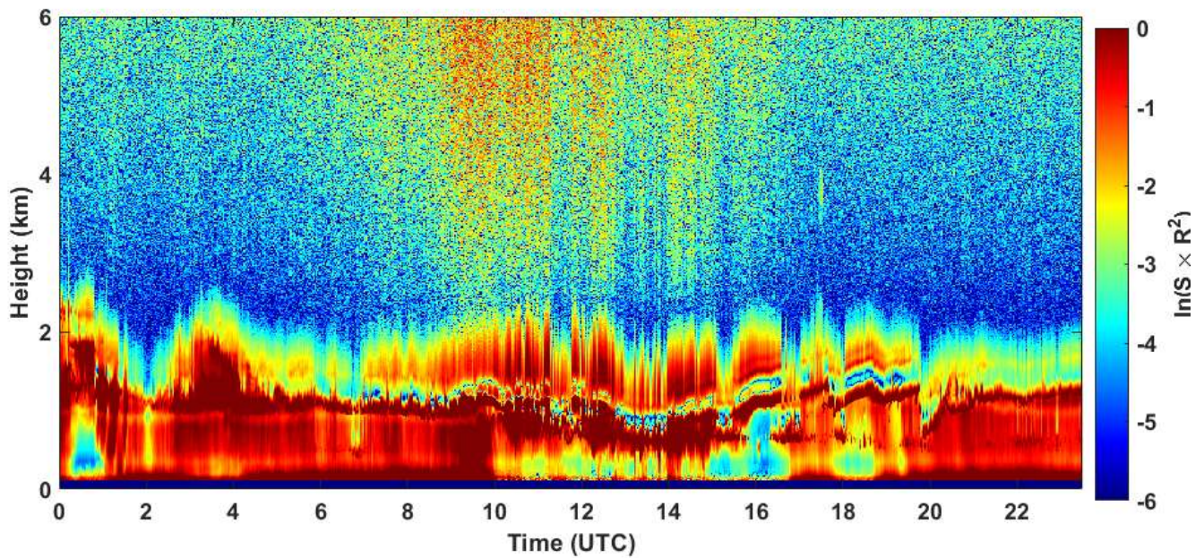
2021-03-20 RCS quick look CHM15k - ILVA LIDAR1 DIREZIONE
