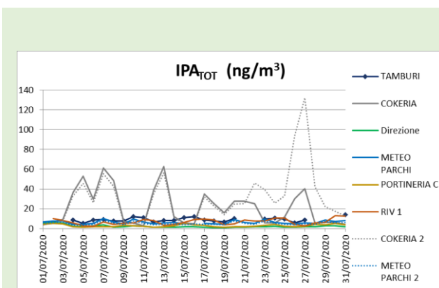
Fig. 16 - Livelli di concentrazione di IPA TOT
