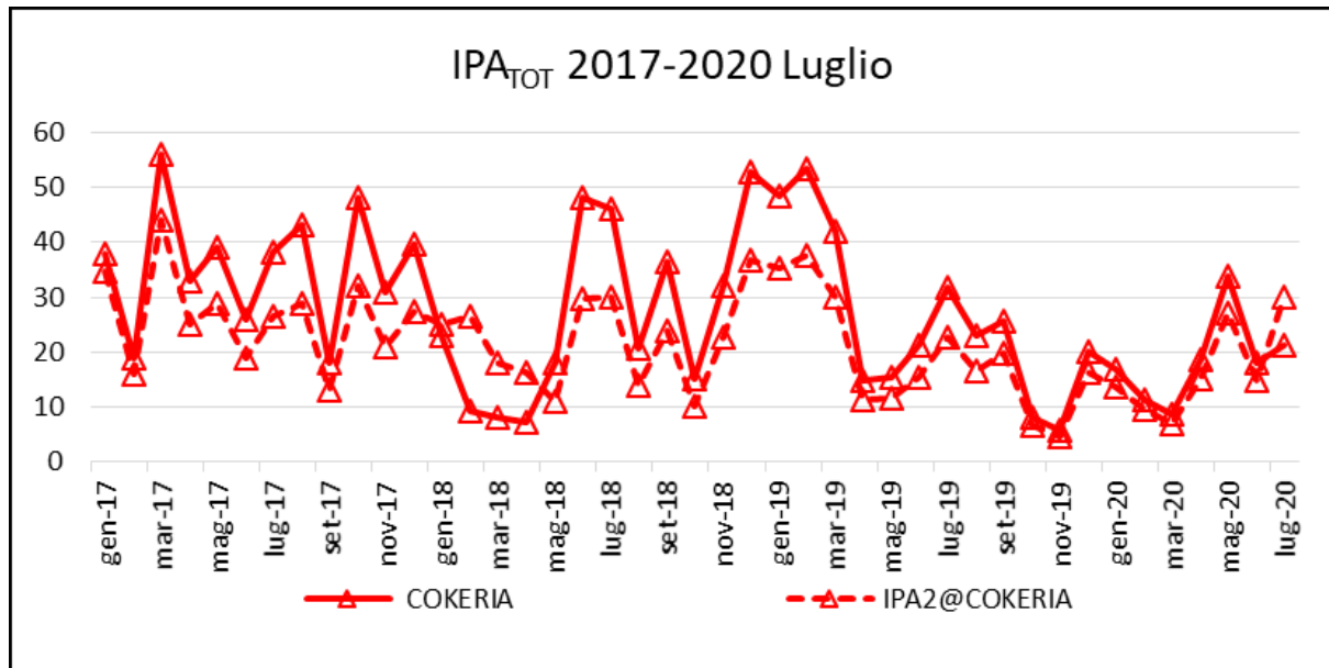
Fig. 17d - Livelli medi mensili di concentrazione di IPA TOT Cokeria (ng/m 3 )
