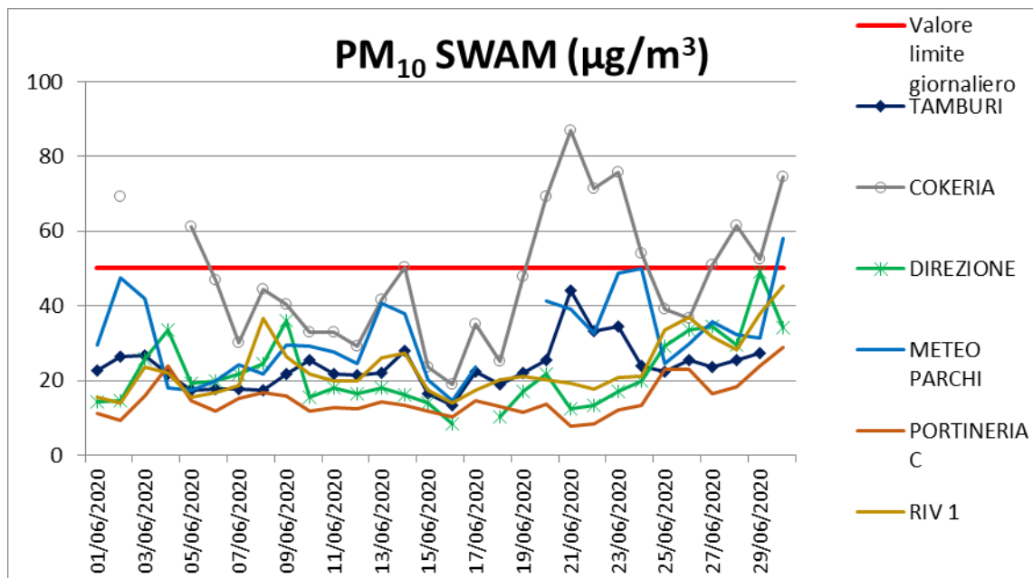
Fig.5b - Livelli di concentrazione Giugno 2020 di PM 10 (SWAM) in µg/m 3
