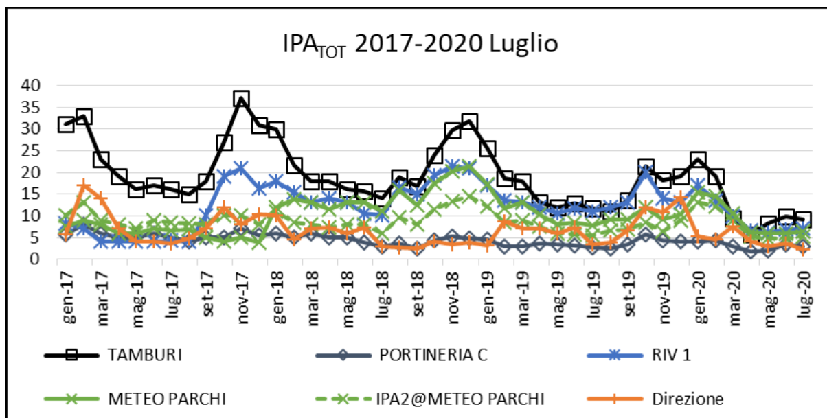
Fig. 17c - Livelli medi mensili di concentrazione di IPA TOT (ng/m 3 ) (senza Cokeria)
