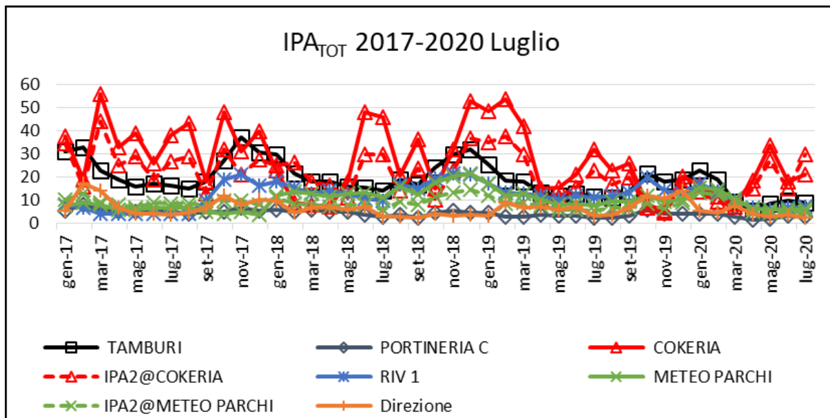
Fig. 17b - Livelli medi mensili di concentrazione di IPA TOT (ng/m 3 )
