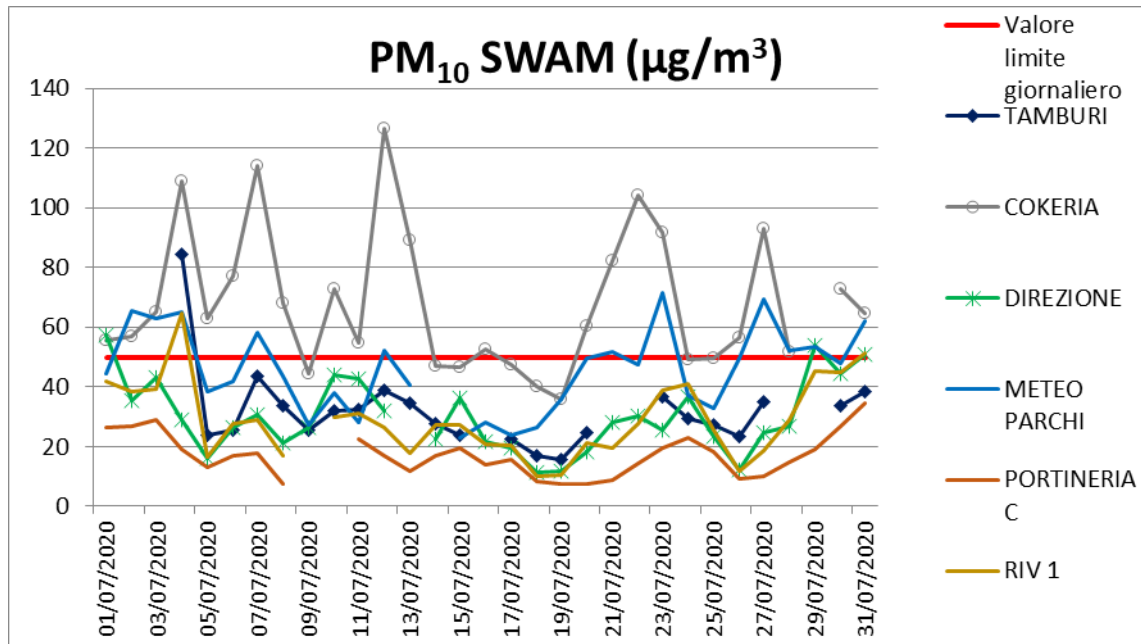
Fig.5a - Livelli di concentrazione Luglio 2020 di PM 10 (SWAM) in µg/m 3
