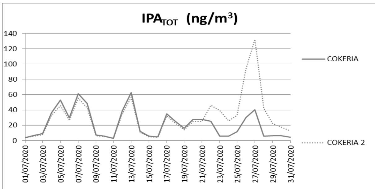
Fig. 17e – Valori medi giornalieri di IPA TOT Cokeria (ng/m 3 )
