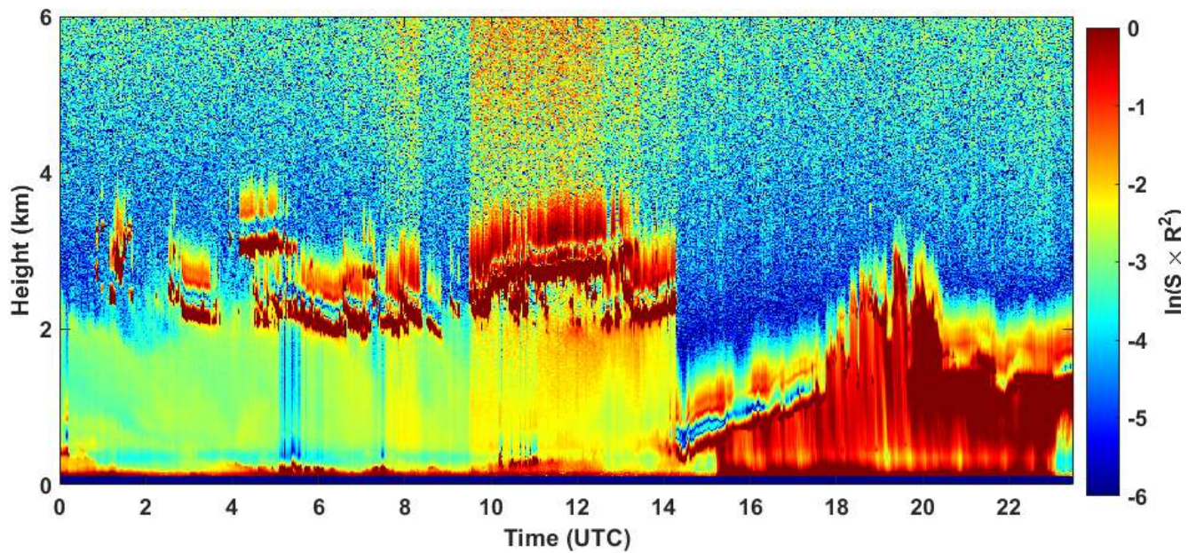
2021-01-08 RCS quick look CHM15k - ILVA LIDAR1 DIREZIONE
