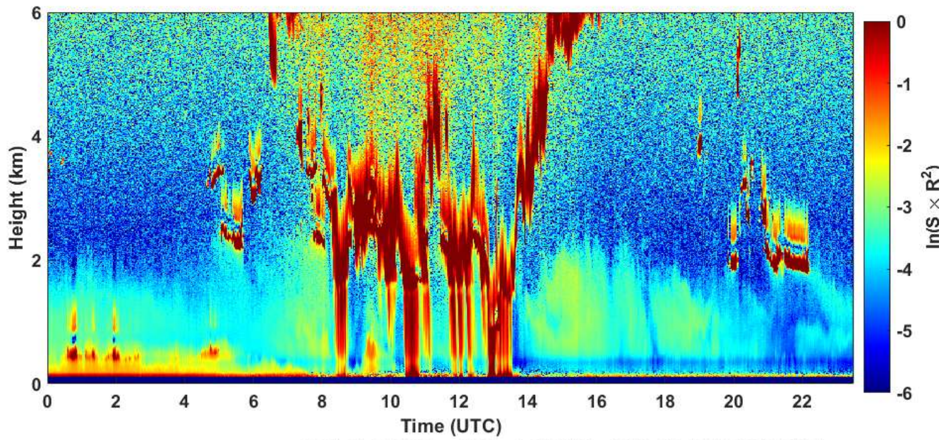
2021-01-24 RCS quick look CHM15k - ILVA LIDAR1 DIREZIONE
