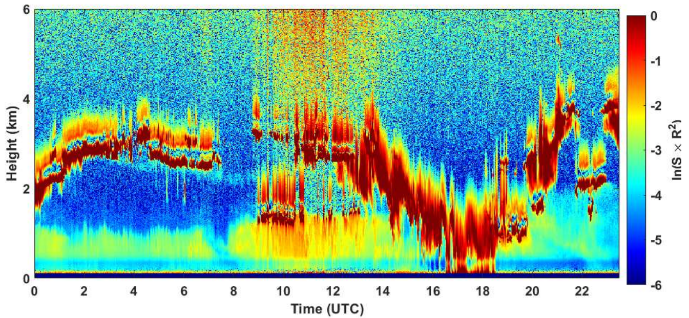
2021-01-16 RCS quick look CHM15k - ILVA LIDAR1 DIREZIONE
