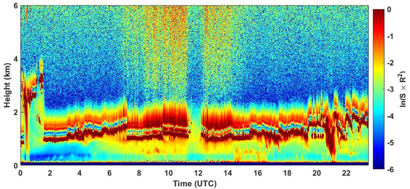
2021-01-12 RCS quick look CHM15k - ILVA LIDAR1 DIREZIONE
