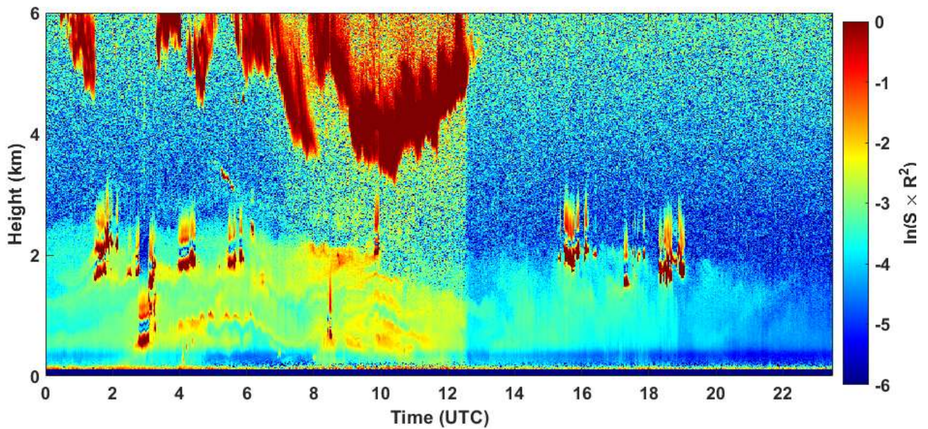
2021-01-04 RCS quick look CHM15k - ILVA LIDAR1 DIREZIONE
