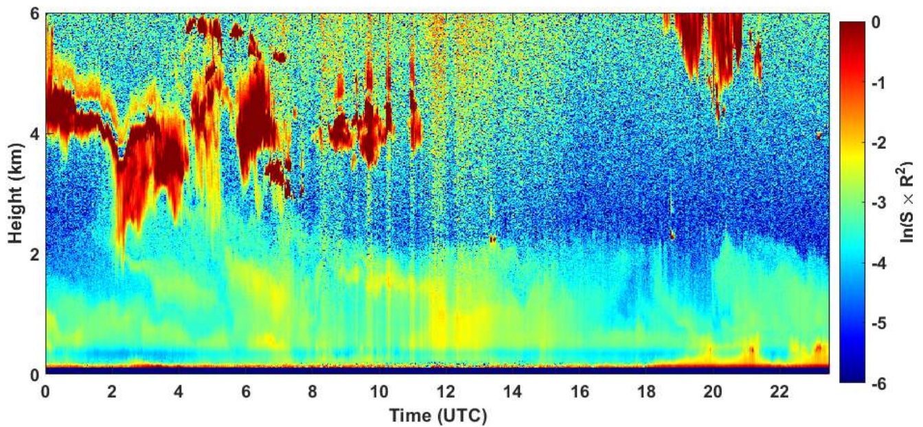
2021-01-22 RCS quick look CHM15k - ILVA LIDAR1 DIREZIONE
