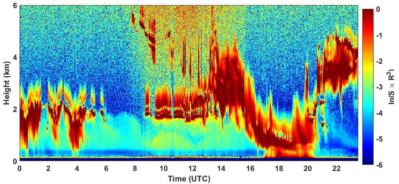
2021-01-18 RCS quick look CHM15k - ILVA LIDAR1 DIREZIONE
