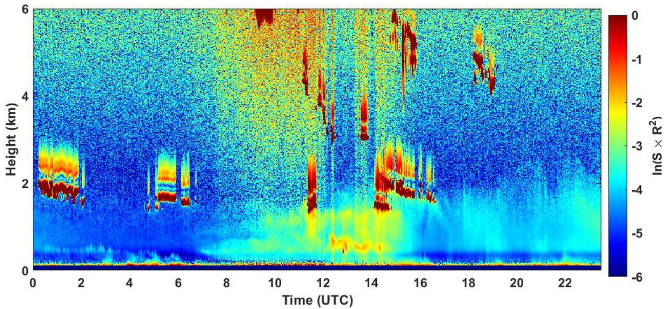
2021-01-30 RCS quick look CHM15k - ILVA LIDAR1 DIREZIONE
