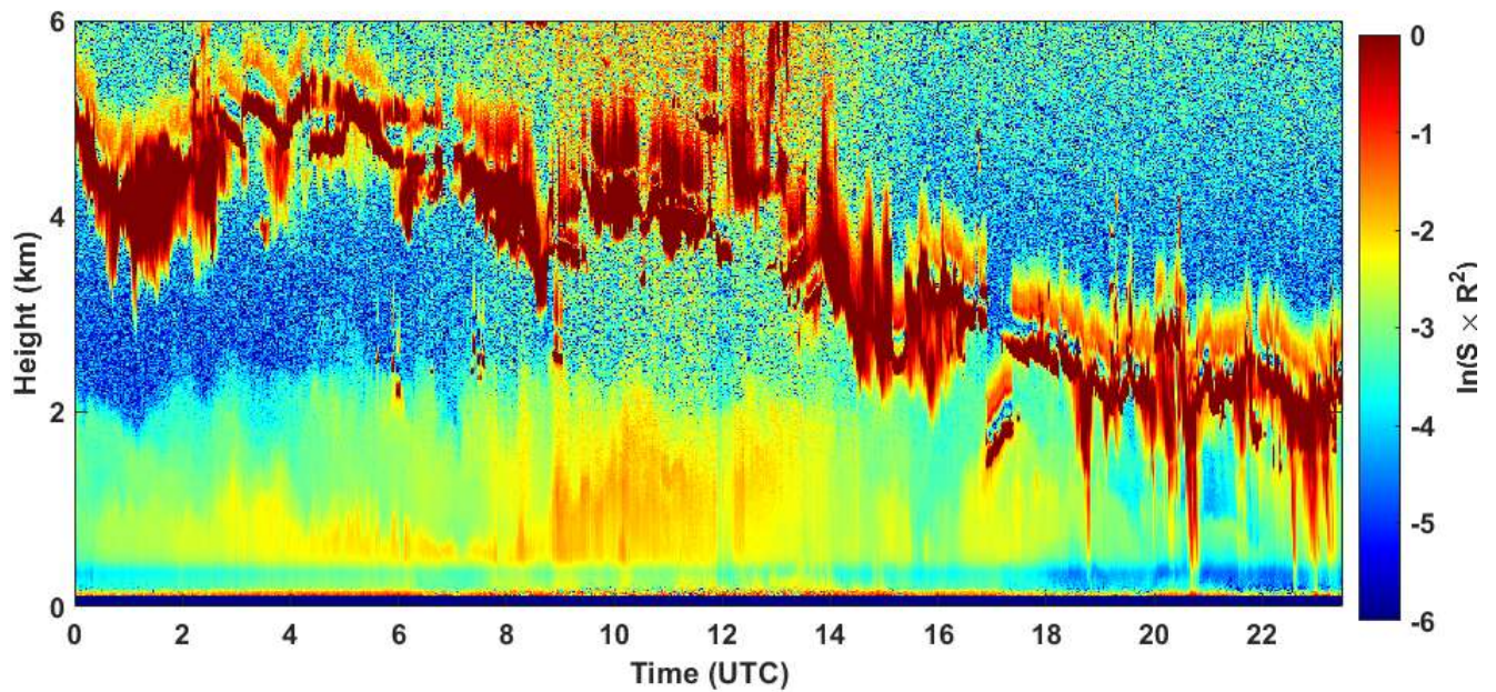
2021-01-06 RCS quick look CHM15k - ILVA LIDAR1 DIREZIONE
