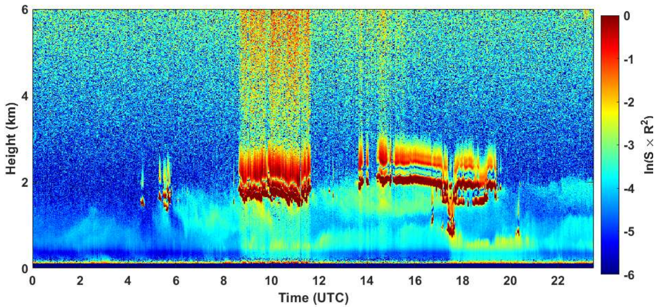
2021-01-20 RCS quick look CHM15k - ILVA LIDAR1 DIREZIONE
