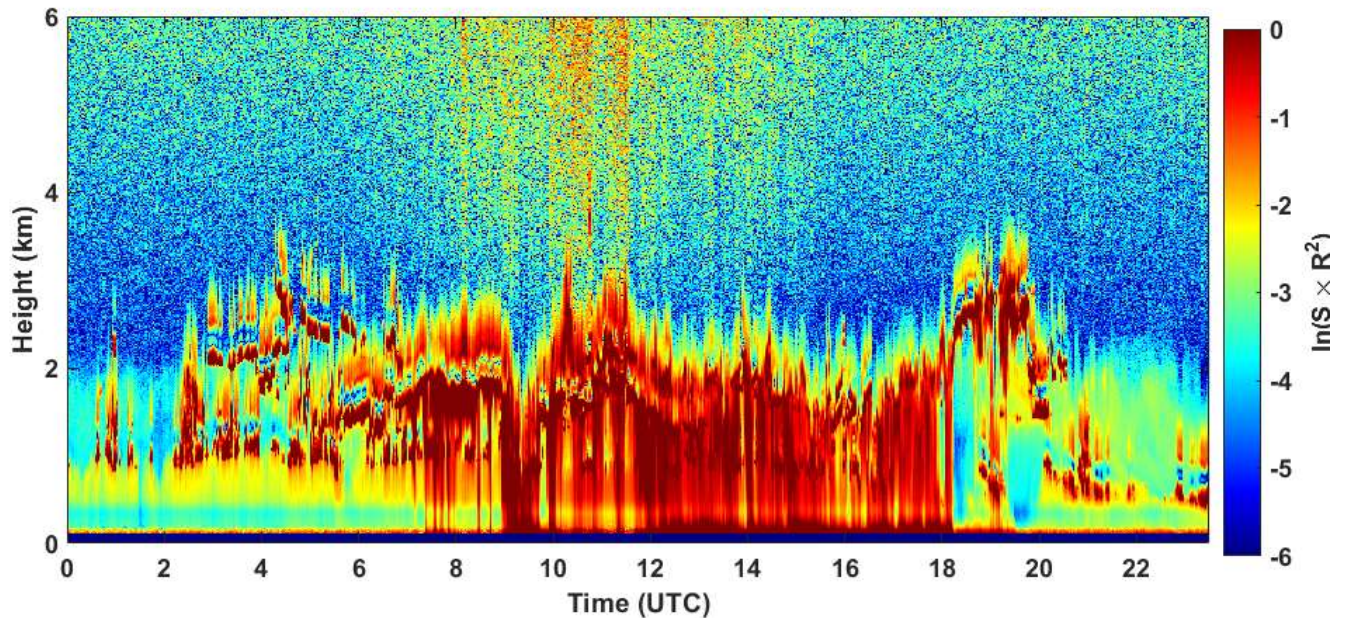
2021-01-02 RCS quick look CHM15k - ILVA LIDAR1 DIREZIONE
