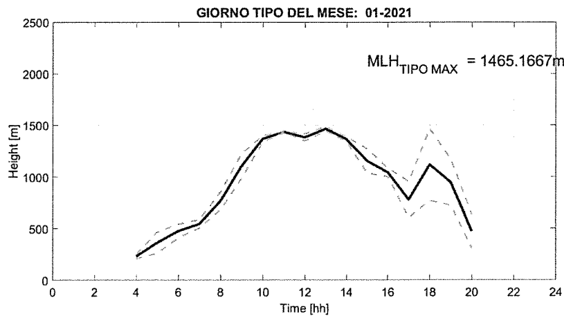
Fig. 2: Giorno tipo del parametro Mixing Layer Height nel mese di GENNAIO 2021, rappresentato mediante media oraria (linea blu continua) e deviazione standard (linee celesti tratteggiate).
