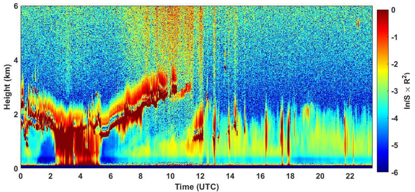
2021-01-26 RCS quick look CHM15k - ILVA LIDAR1 DIREZIONE
