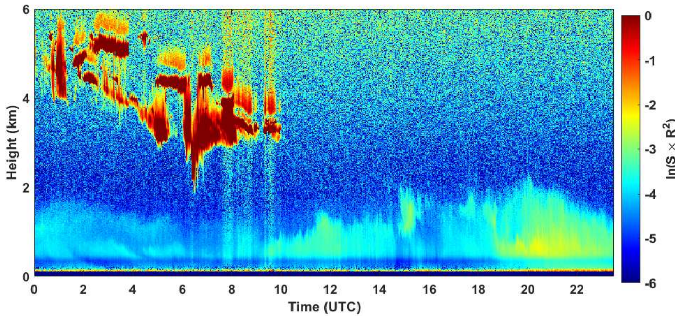
2021-01-14 RCS quick look CHM15k - ILVA LIDAR1 DIREZIONE
