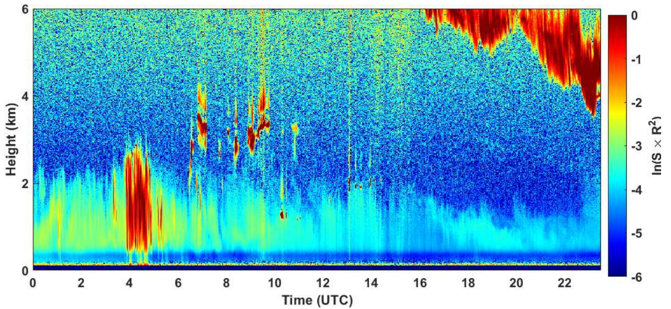
2021-01-28 RCS quick look CHM15k - ILVA LIDAR1 DIREZIONE
