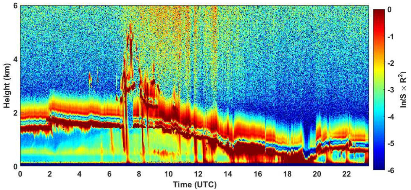
2021-01-10 RCS quick look CHM15k - ILVA LIDAR1 DIREZIONE
