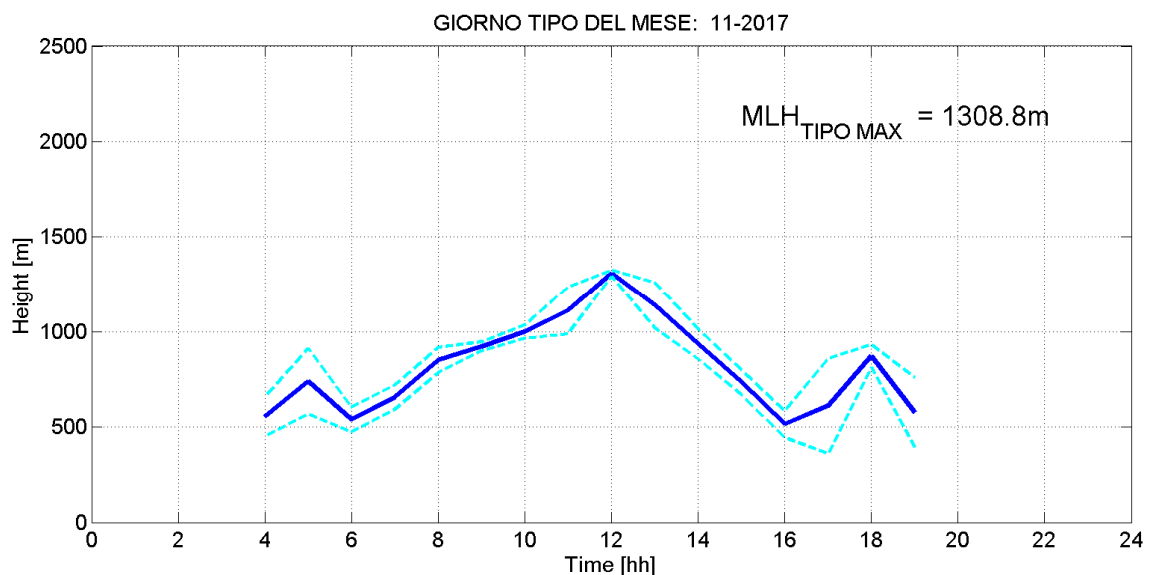
Fig. 2: Giorno tipo del parametro Mixing Layer Height nel mese di NOVEMBRE 2017, rappresentato mediante media oraria (linea blu continua), e quartili corrispondenti ad una deviazione standard (linee celesti tratteggiate).
