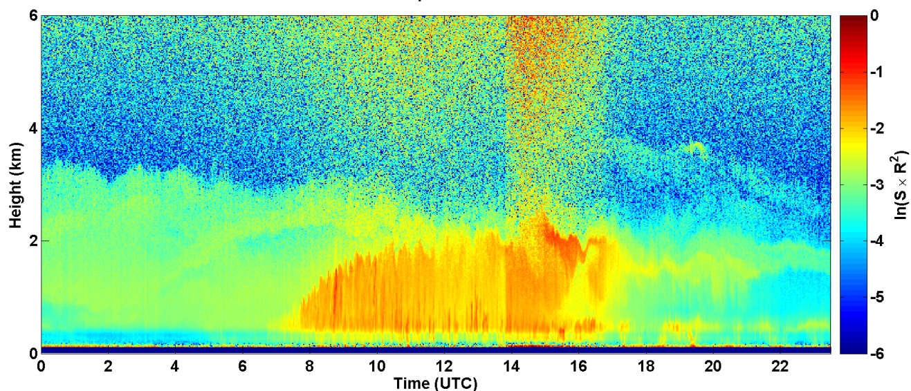
2017-08-08 RCS quick look CHM15k - ILVA LIDAR1 DIREZIONE
