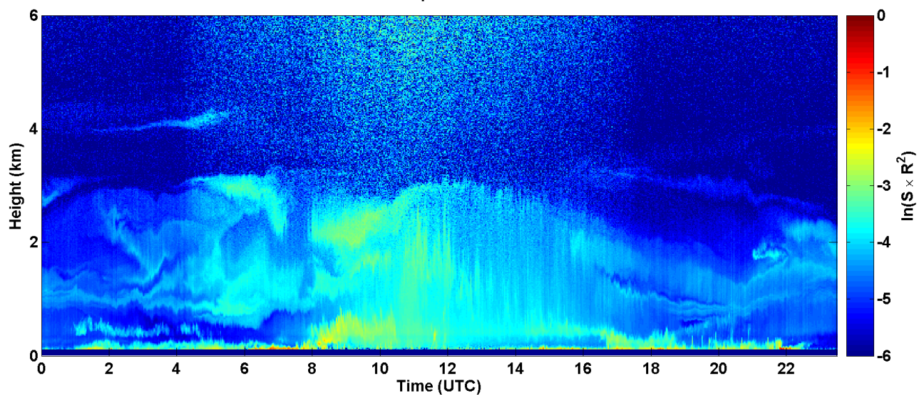
2017-08-26 RCS quick look CHM15k - ILVA LIDAR3 AGGLOMERATO
