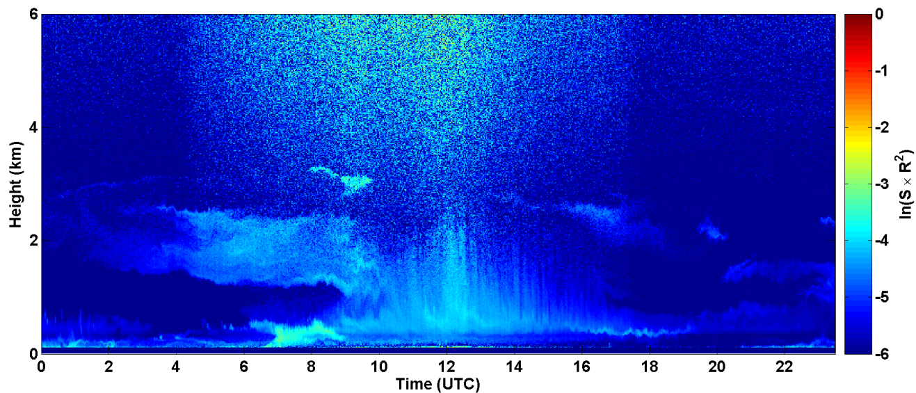
2017-08-25 RCS quick look CHM15k - ILVA LIDAR2 PARCHI
