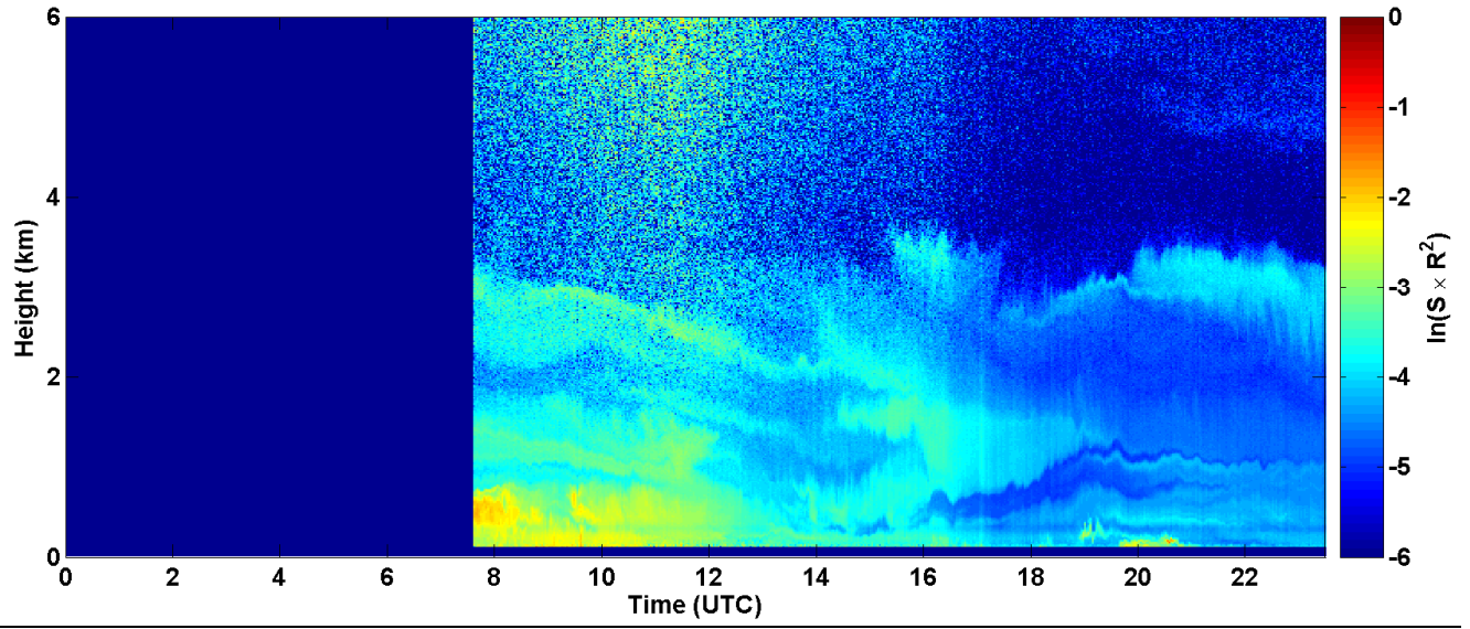
2017-08-09 RCS quick look CHM15k - ILVA LIDAR2 PARCHI
