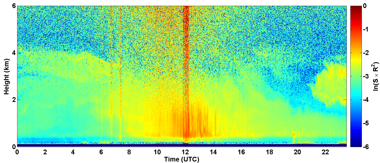
2017-08-04 RCS quick look CHM15k - ILVA LIDAR1 DIREZIONE
