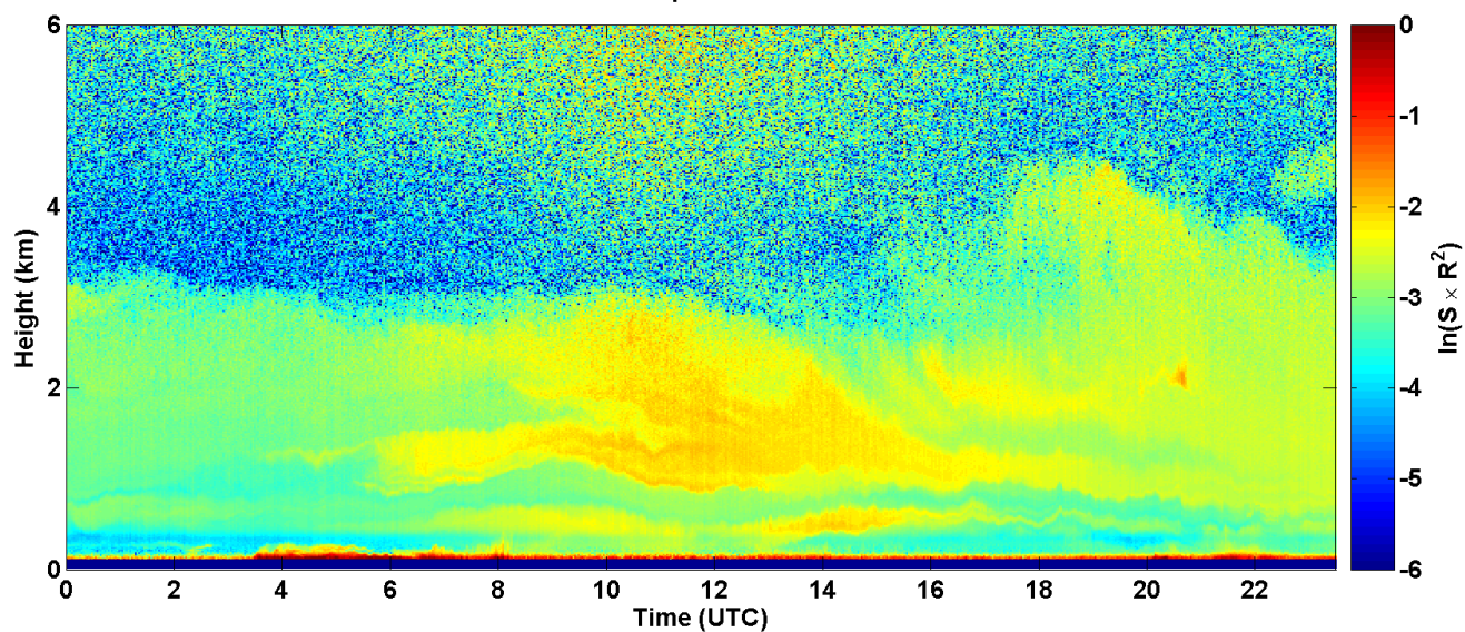
2017-08-11 RCS quick look CHM15k - ILVA LIDAR1 DIREZIONE
