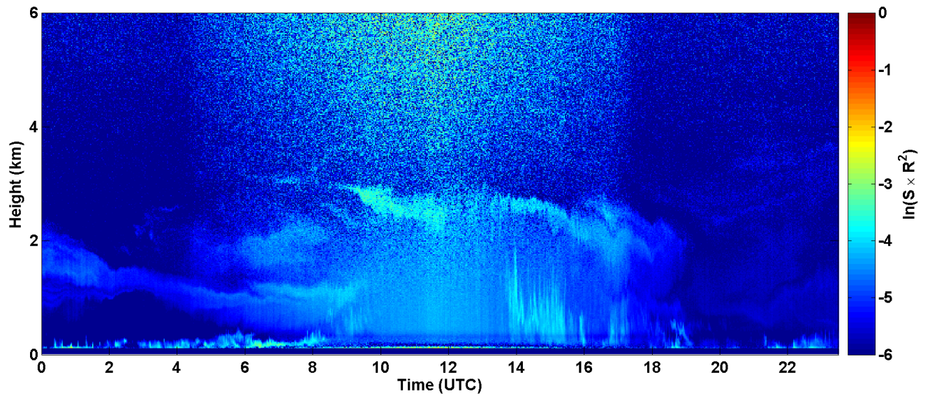
2017-08-28 RCS quick look CHM15k - ILVA LIDAR2 PARCHI
