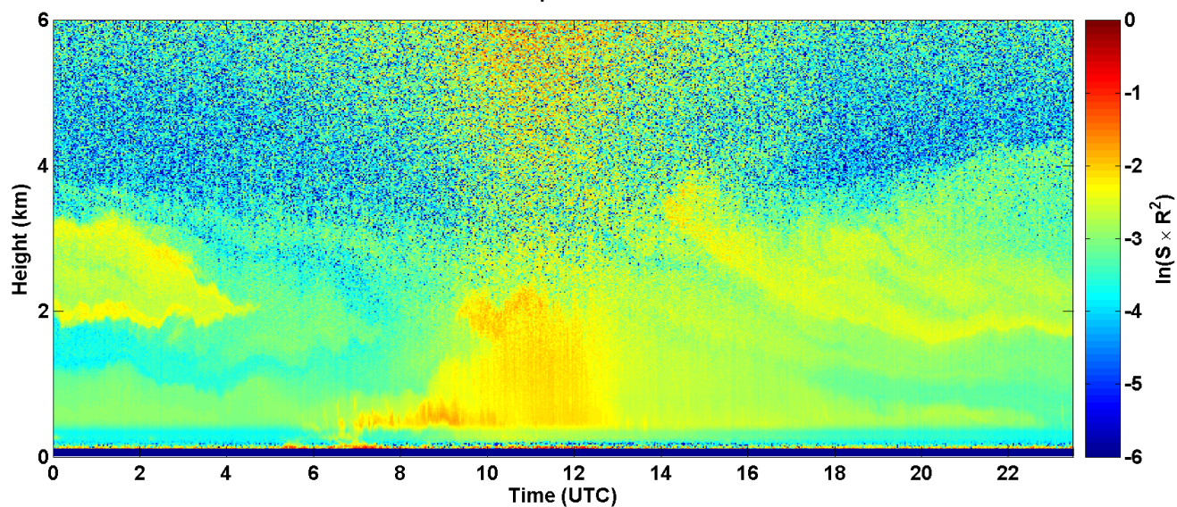
2017-08-05 RCS quick look CHM15k - ILVA LIDAR1 DIREZIONE
