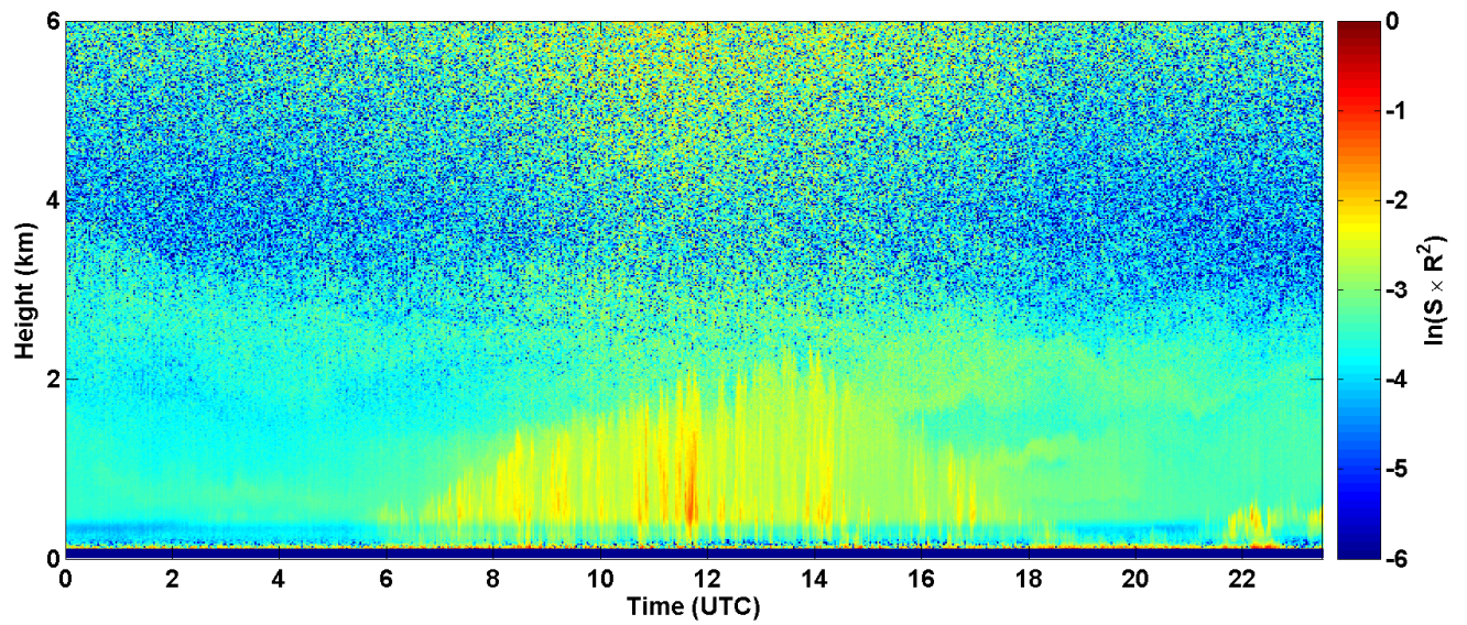
2017-08-02 RCS quick look CHM15k - ILVA LIDAR1 DIREZIONE
