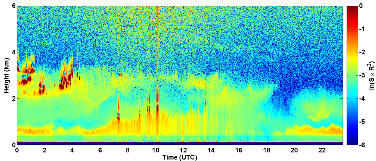
2017-08-22 RCS quick look CHM15k - ILVA LIDAR1 DIREZIONE
