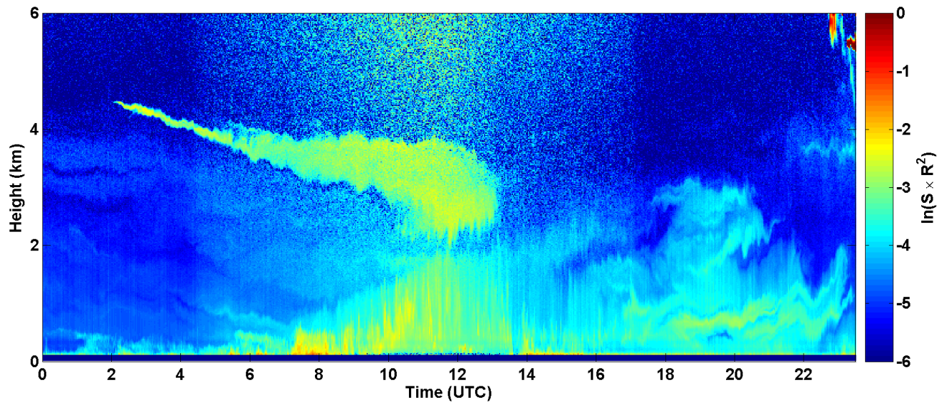
2017-08-28 RCS quick look CHM15k - ILVA LIDAR3 AGGLOMERATO
