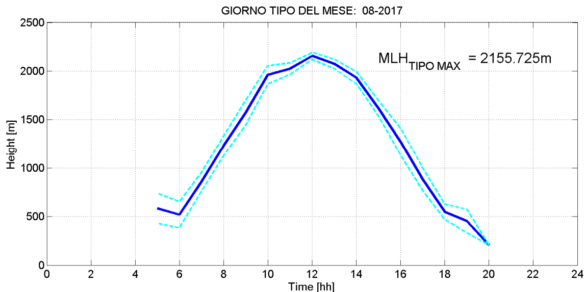
Fig. 2: Giorno tipo del parametro Mixing Layer Height nel mese di AGOSTO 2017, rappresentato mediante media oraria (linea blu continua), e quartili corrispondenti ad una deviazione standard (linee celesti tratteggiate).
