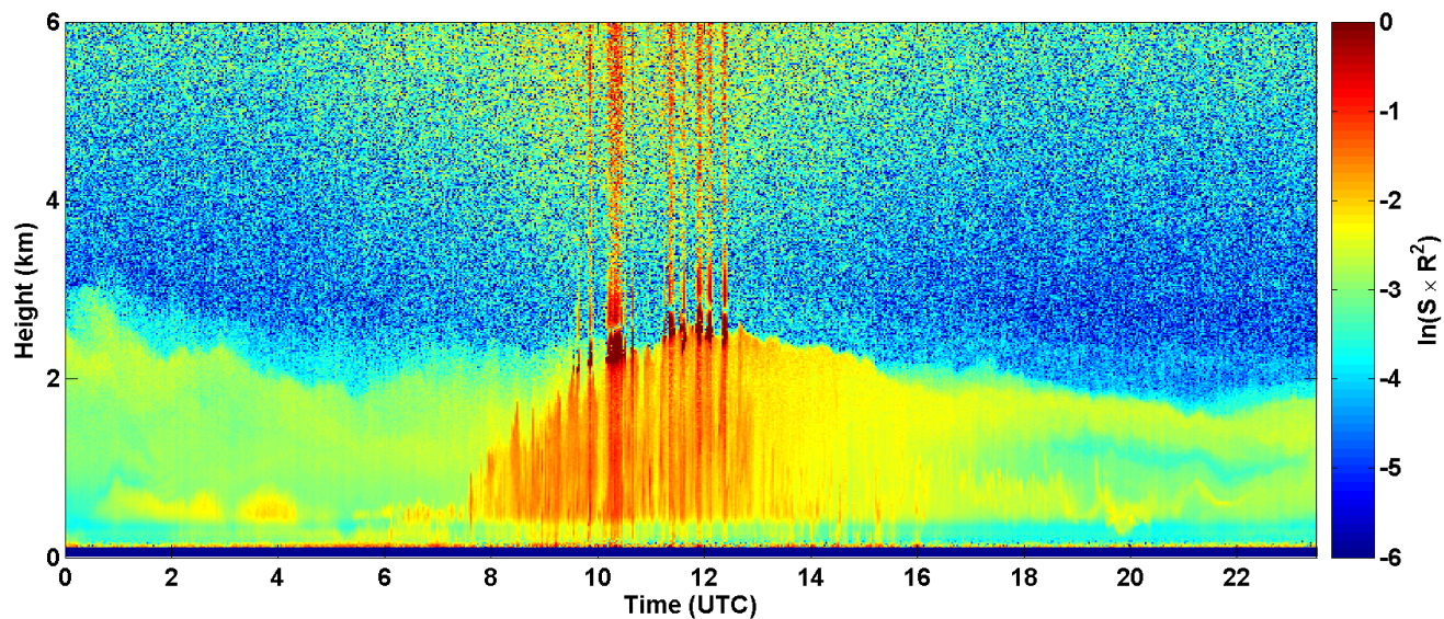
2017-08-30 RCS quick look CHM15k - ILVA LIDAR1 DIREZIONE
