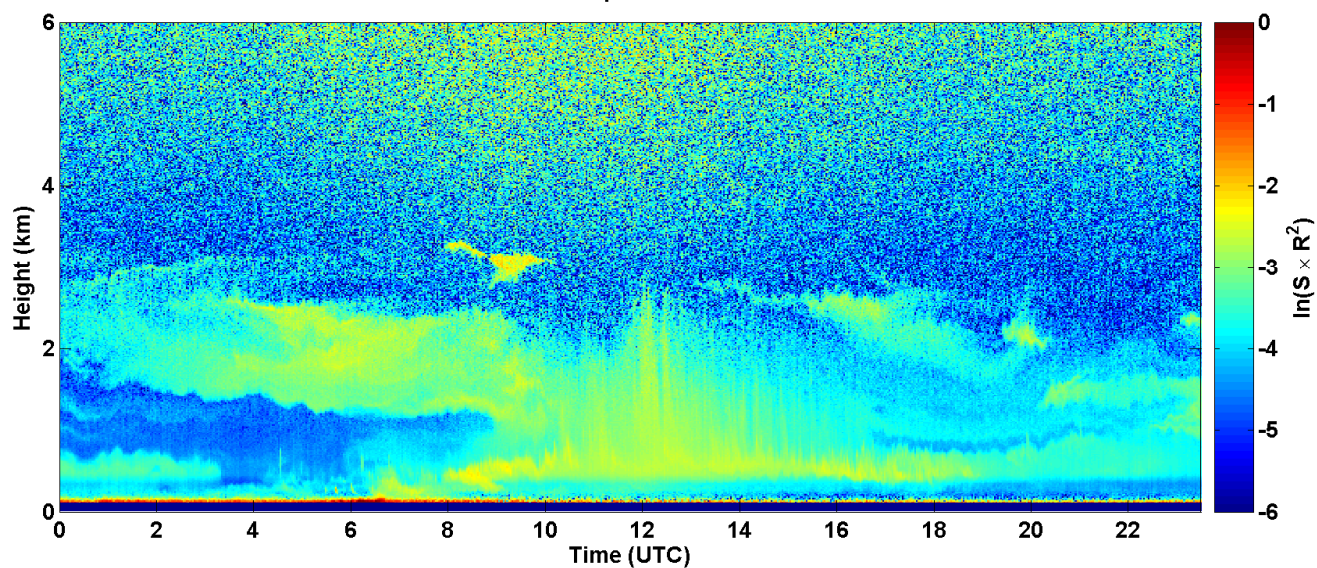
2017-08-26 RCS quick look CHM15k - ILVA LIDAR1 DIREZIONE
