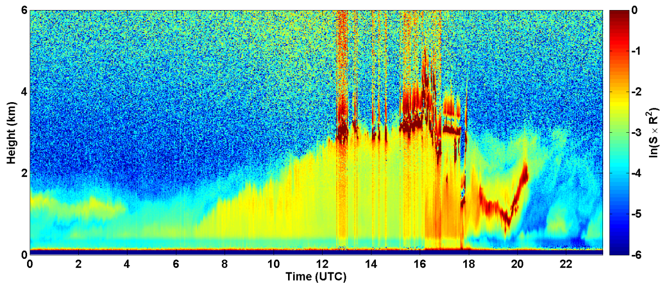
2017-08-13 RCS quick look CHM15k - ILVA LIDAR1 DIREZIONE
