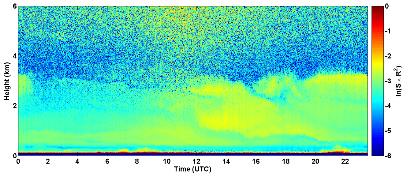
2017-08-10 RCS quick look CHM15k - ILVA LIDAR1 DIREZIONE
