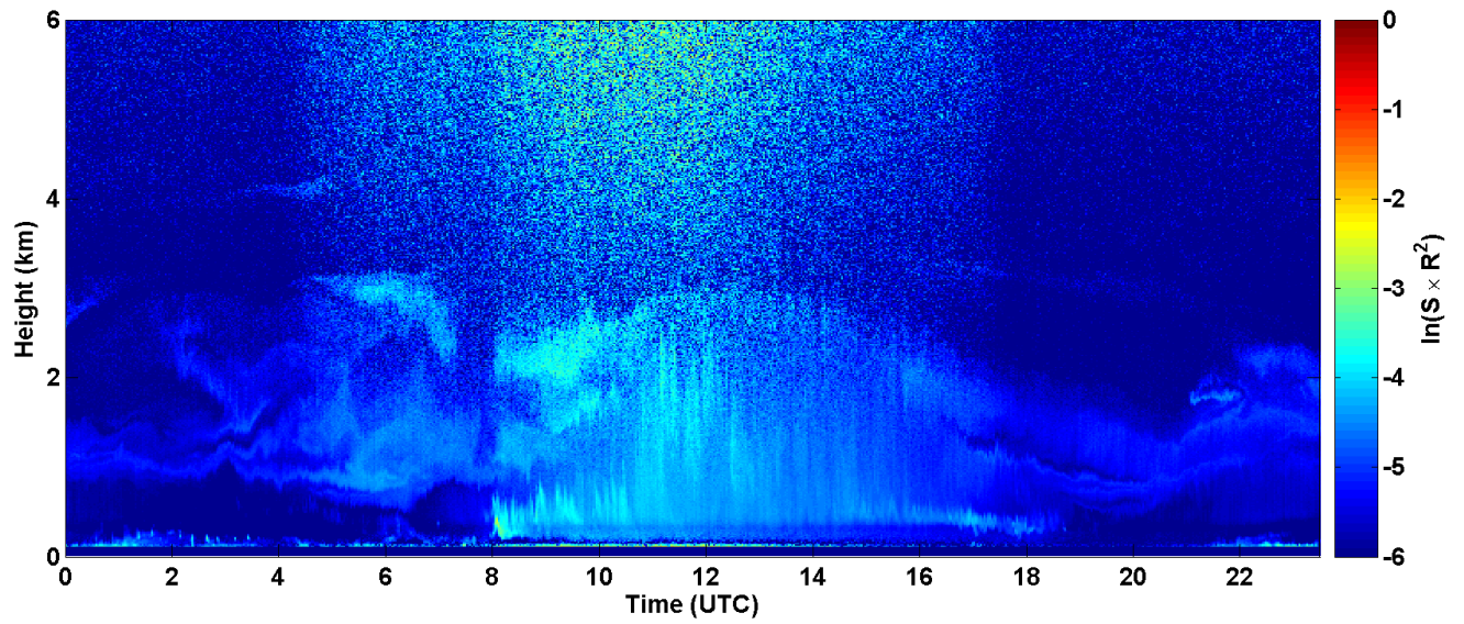
2017-08-27 RCS quick look CHM15k - ILVA LIDAR2 PARCHI
