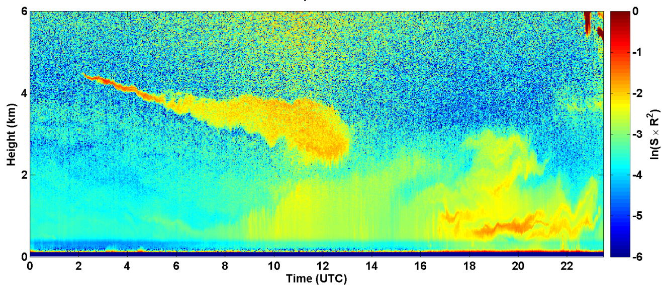
2017-08-29 RCS quick look CHM15k - ILVA LIDAR1 DIREZIONE
