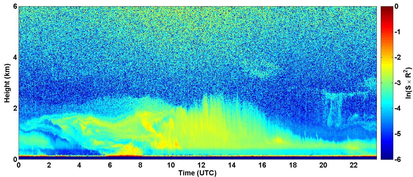
2017-08-25 RCS quick look CHM15k - ILVA LIDAR1 DIREZIONE
