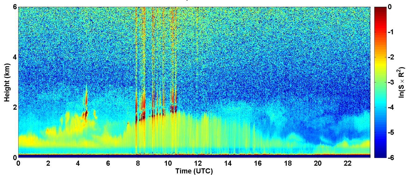
2017-08-14 RCS quick look CHM15k - ILVA LIDAR1 DIREZIONE
