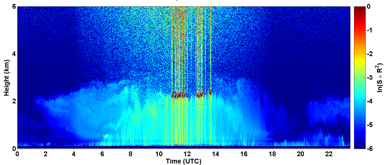
2017-08-16 RCS quick look CHM15k - ILVA LIDAR2 PARCHI
