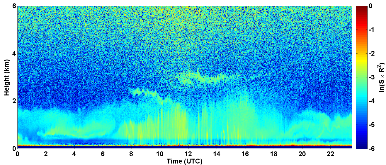
2017-08-16 RCS quick look CHM15k - ILVA LIDAR1 DIREZIONE
