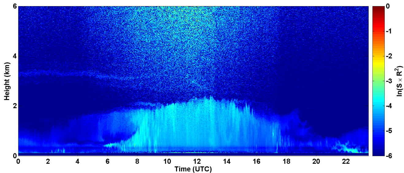
2017-08-24 RCS quick look CHM15k - ILVA LIDAR2 PARCHI
