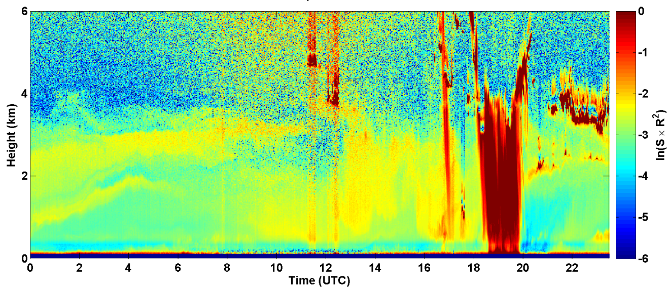
2017-08-20 RCS quick look CHM15k - ILVA LIDAR1 DIREZIONE
