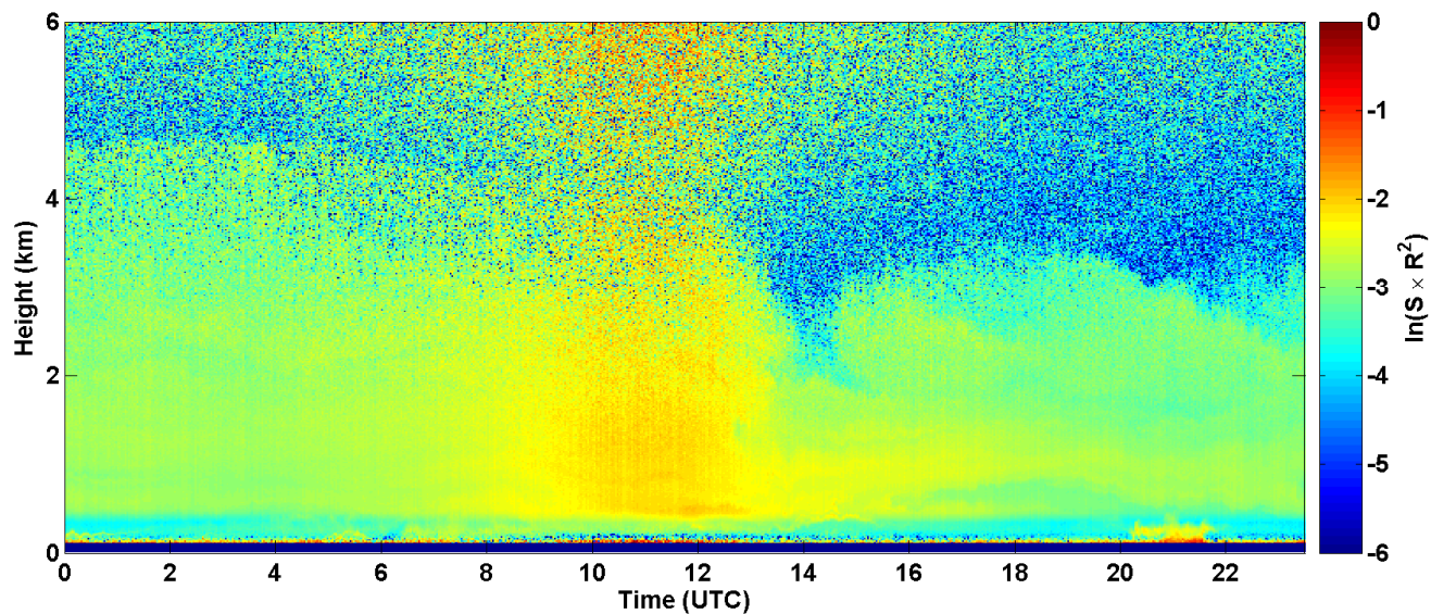
2017-08-07 RCS quick look CHM15k - ILVA LIDAR1 DIREZIONE
