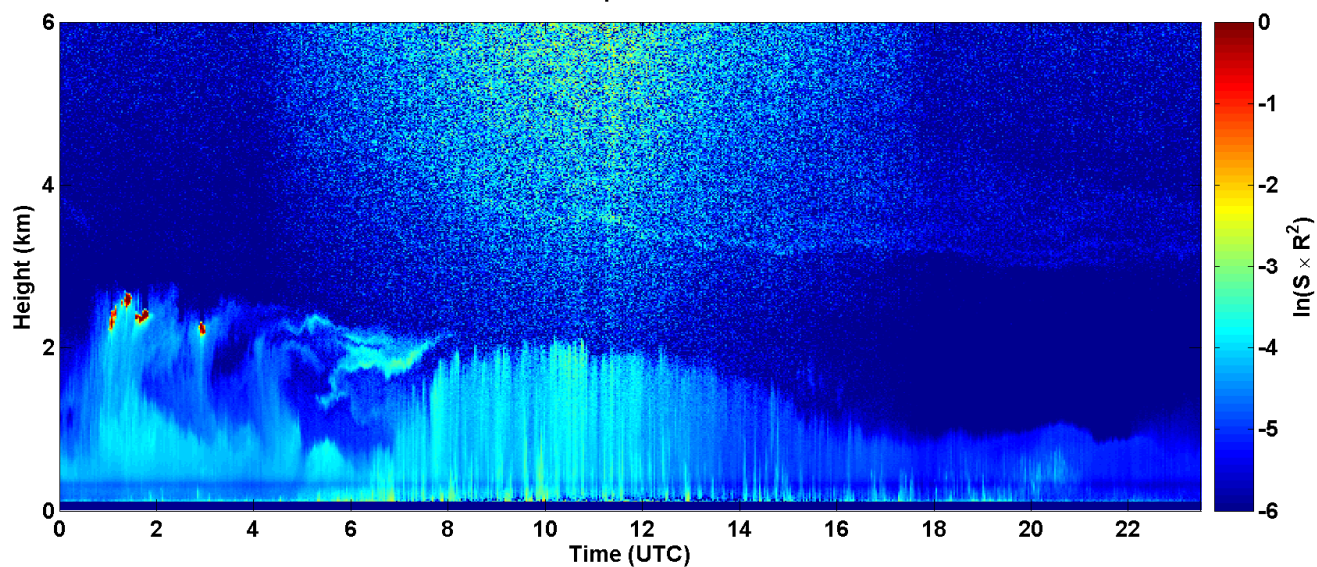
2017-08-22 RCS quick look CHM15k - ILVA LIDAR2 PARCHI
