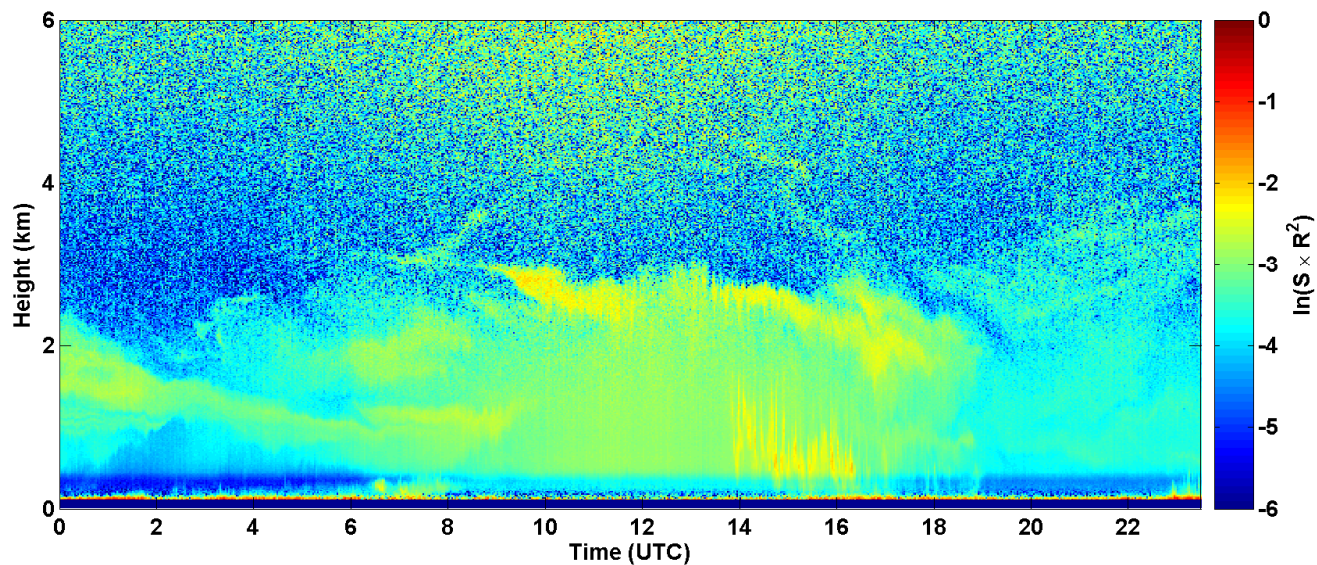
2017-08-28 RCS quick look CHM15k - ILVA LIDAR1 DIREZIONE
