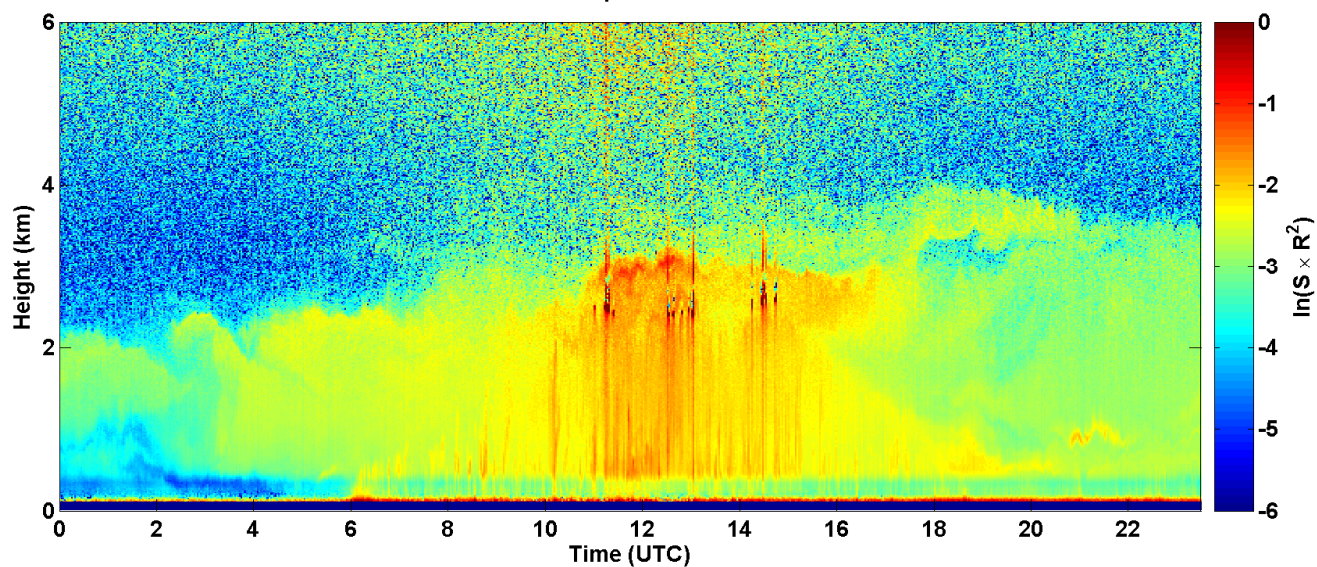
2017-08-17 RCS quick look CHM15k - ILVA LIDAR1 DIREZIONE
