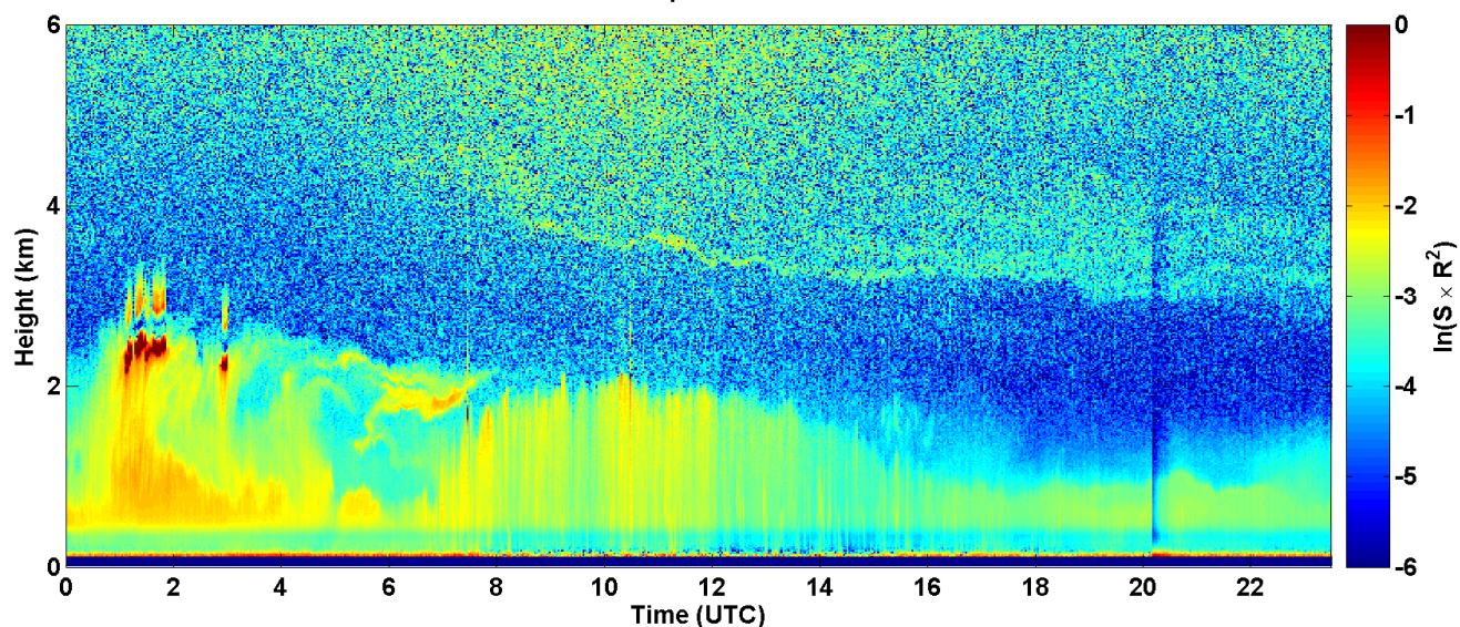
2017-08-23 RCS quick look CHM15k - ILVA LIDAR1 DIREZIONE
