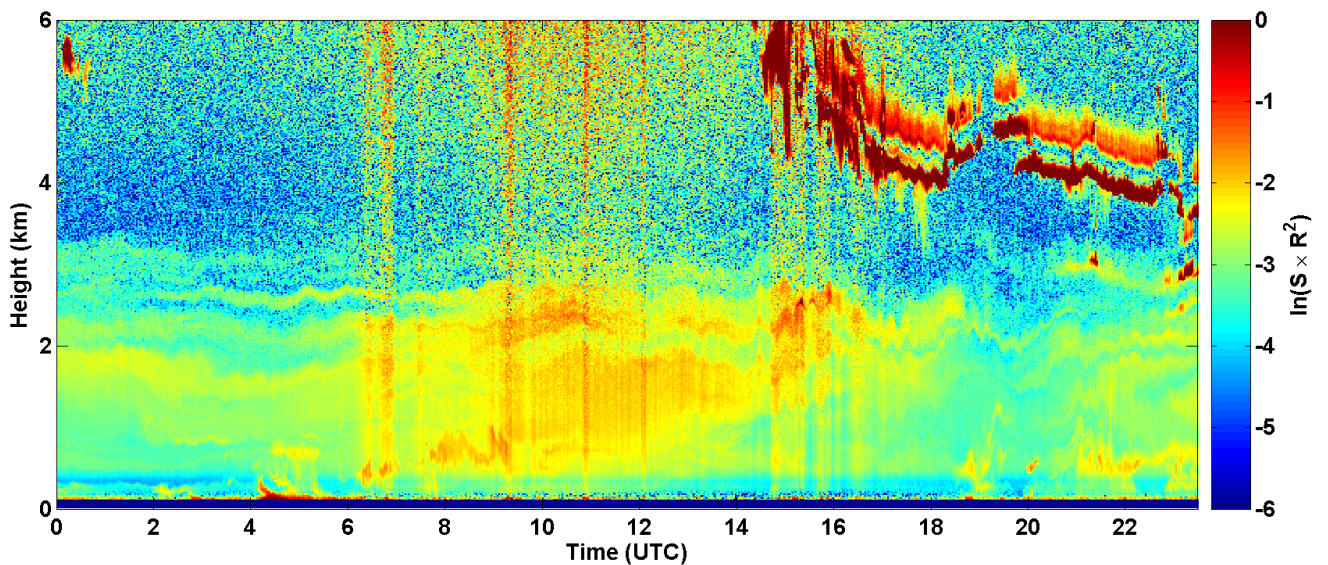
2017-06-02 RCS quick look CHM15k - ILVA LIDAR1 DIREZIONE
