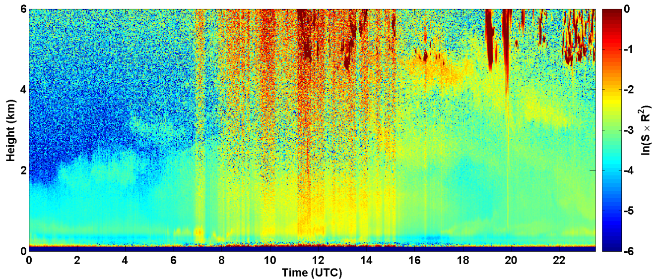
2017-06-29 RCS quick look CHM15k - ILVA LIDAR1 DIREZIONE
