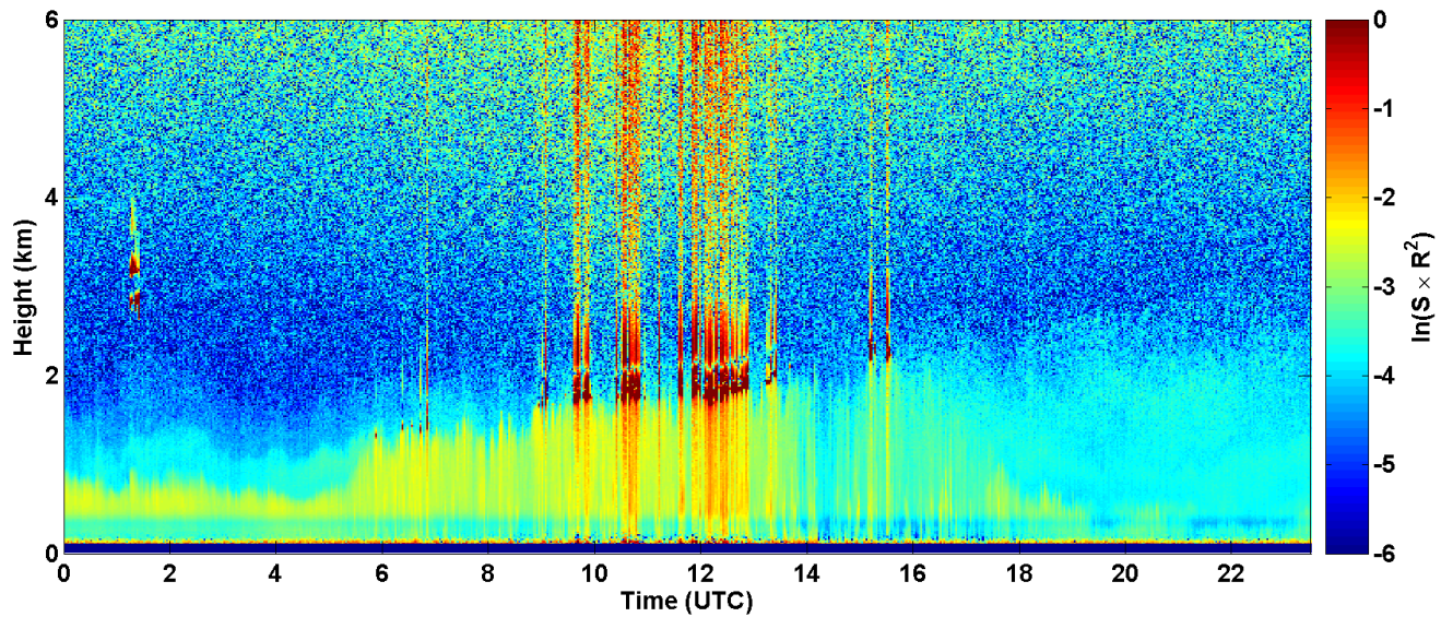
2017-06-20 RCS quick look CHM15k - ILVA LIDAR1 DIREZIONE
