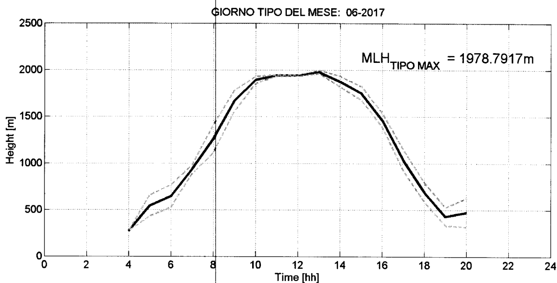
Fig. 2: Giorno tipo del parametro Mixing Layer Height nel mese di GIUGNO 2017, rappresentato mediante media oraria (linea blu continua), e quartili corrispondenti ad una deviazione standard (linee celesti tratteggiate).
