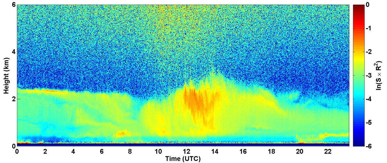
2017-06-22 RCS quick look CHM15k - ILVA LIDAR1 DIREZIONE
