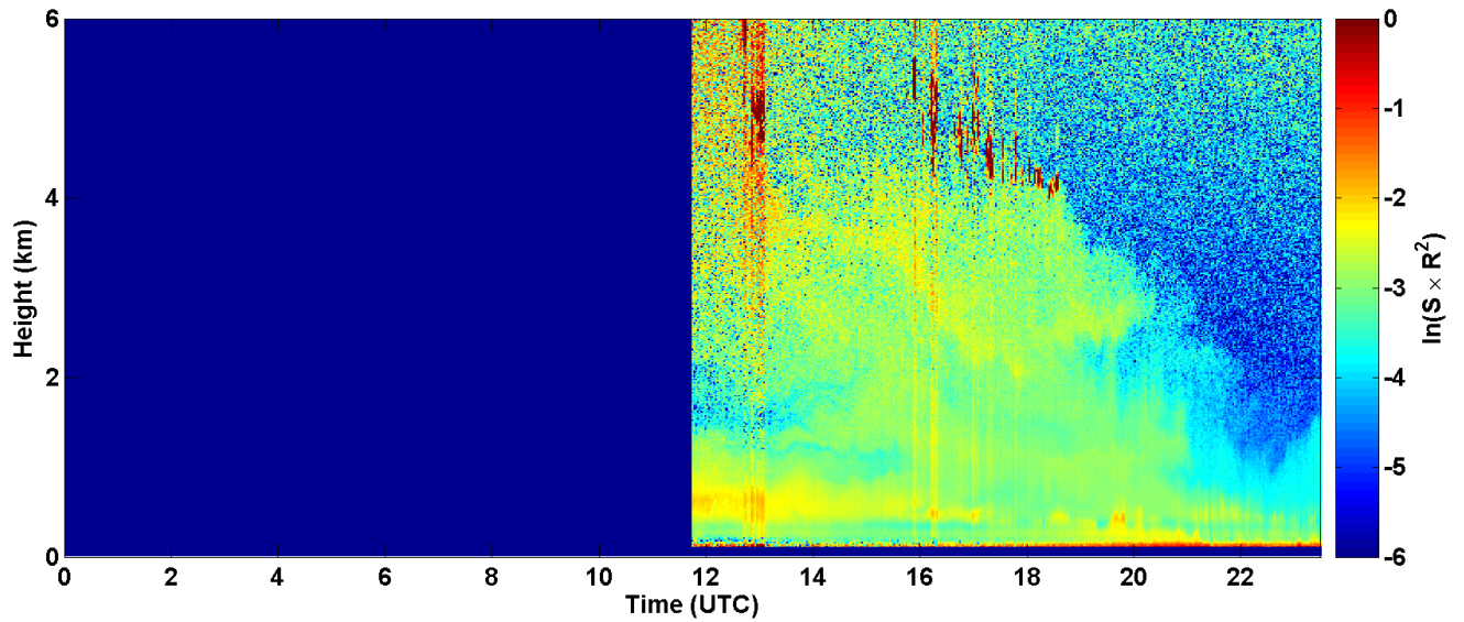
2017-06-27 RCS quick look CHM15k - ILVA LIDAR1 DIREZIONE
