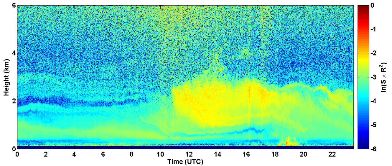
2017-06-24 RCS quick look CHM15k - ILVA LIDAR1 DIREZIONE
