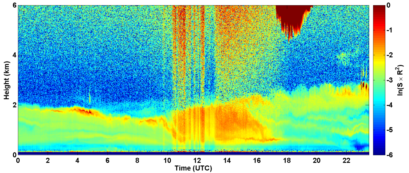
2017-06-10 RCS quick look CHM15k - ILVA LIDAR1 DIREZIONE
