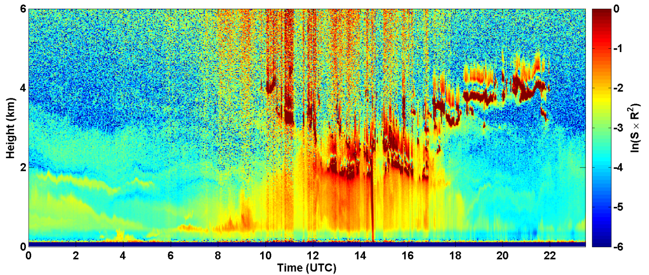
2017-06-18 RCS quick look CHM15k - ILVA LIDAR1 DIREZIONE
