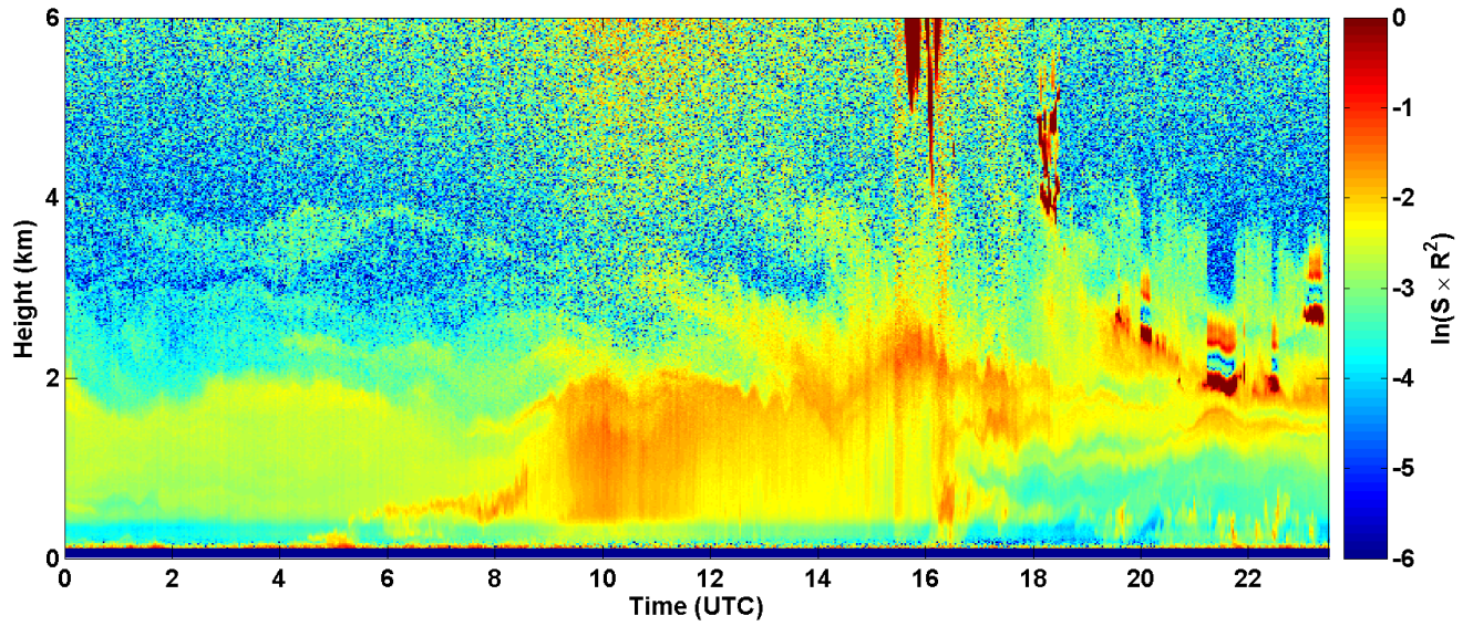
2017-06-16 RCS quick look CHM15k - ILVA LIDAR1 DIREZIONE
