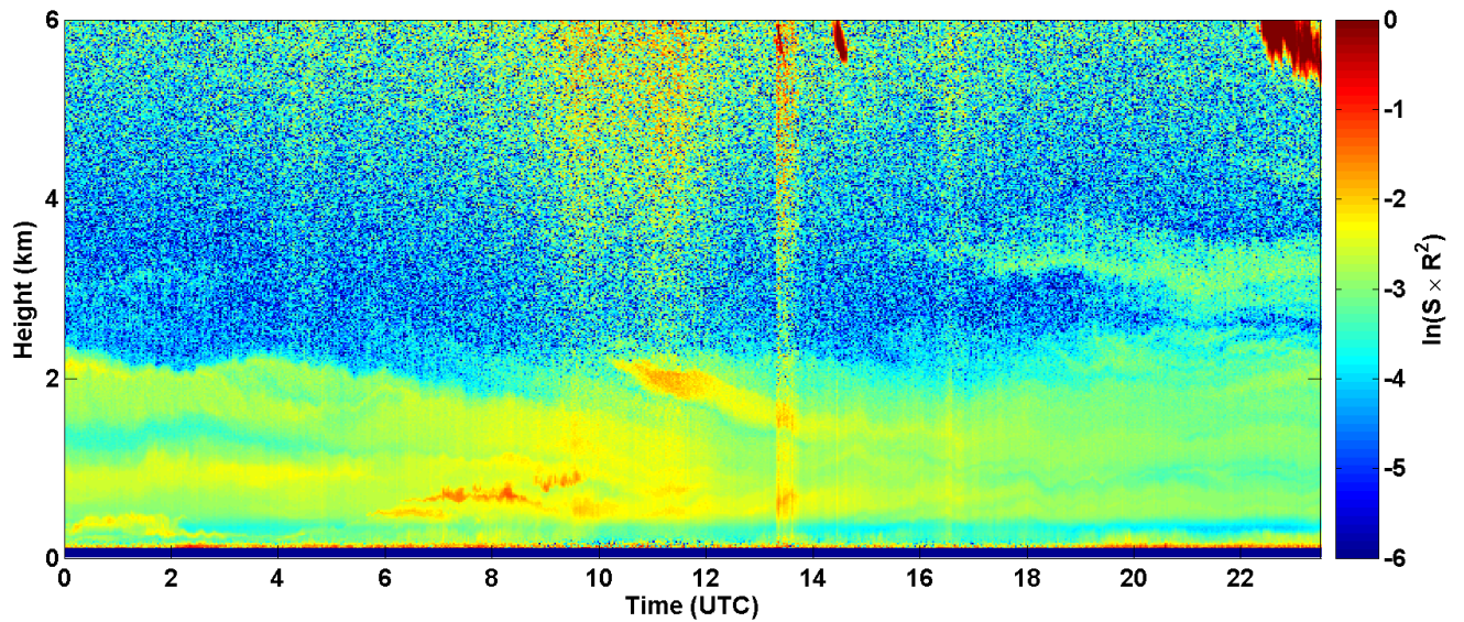
2017-06-06 RCS quick look CHM15k - ILVA LIDAR1 DIREZIONE
