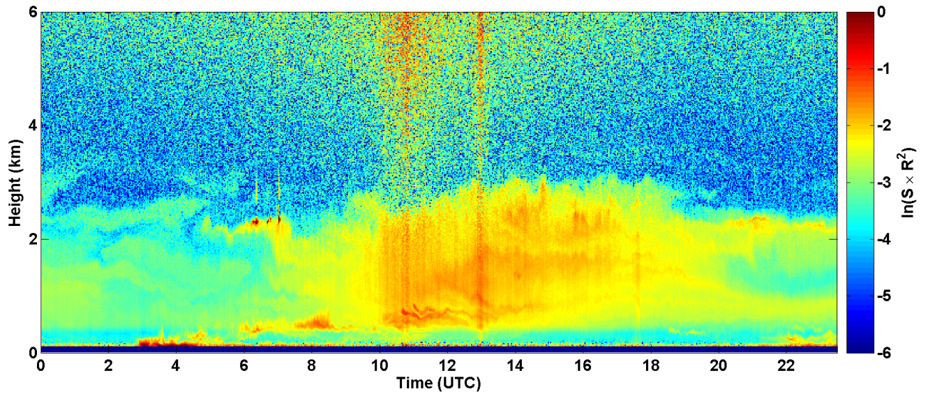
2017-06-04 RCS quick look CHM15k - ILVA LIDAR1 DIREZIONE
