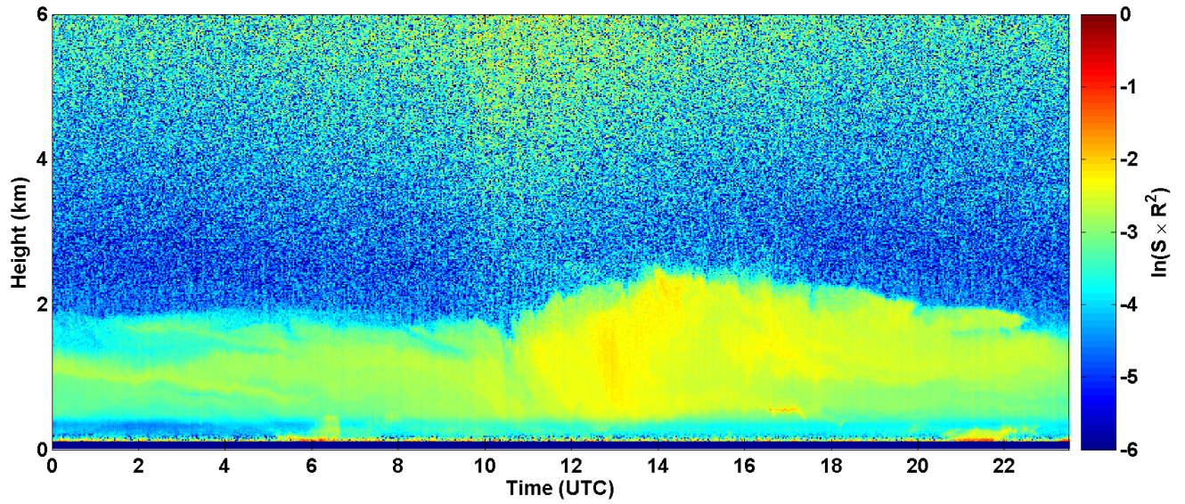
2017-06-14 RCS quick look CHM15k - ILVA LIDAR1 DIREZIONE
