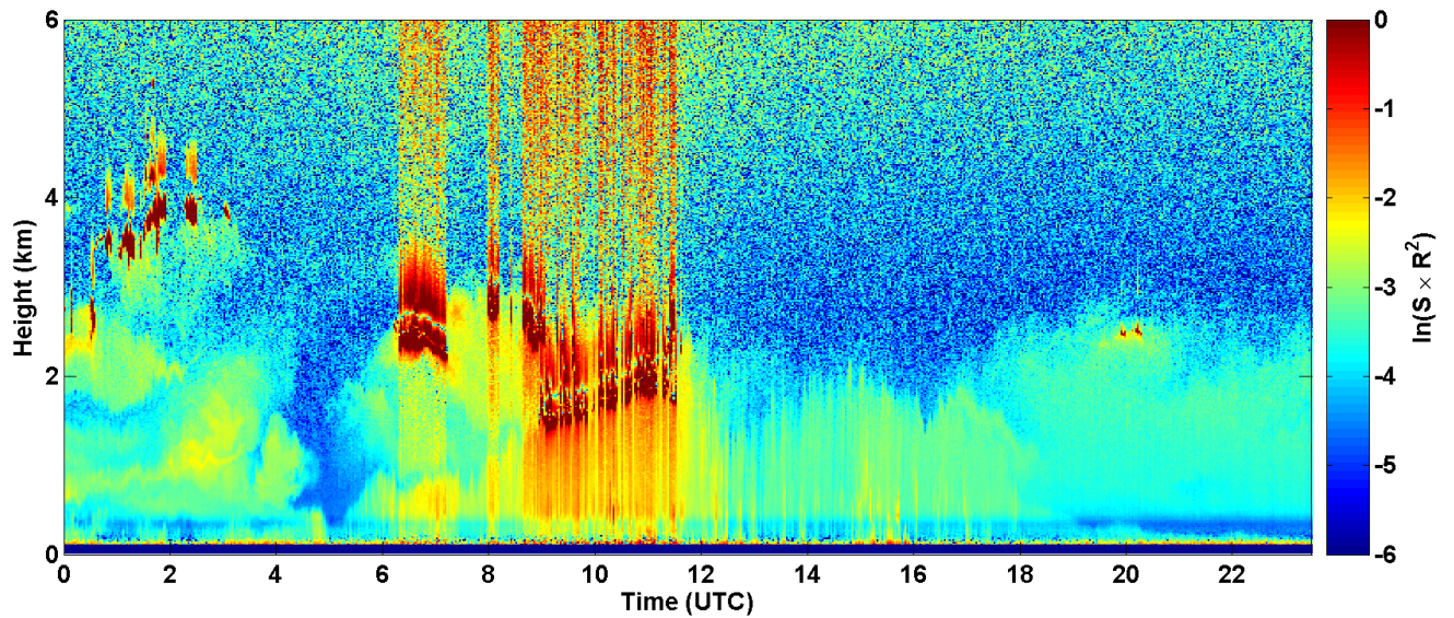
2017-06-12 RCS quick look CHM15k - ILVA LIDAR1 DIREZIONE
