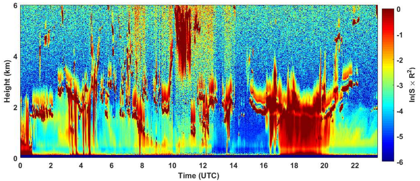
2018-11-28 RCS quick look CHM15k - ILVA LIDAR1 DIREZIONE
