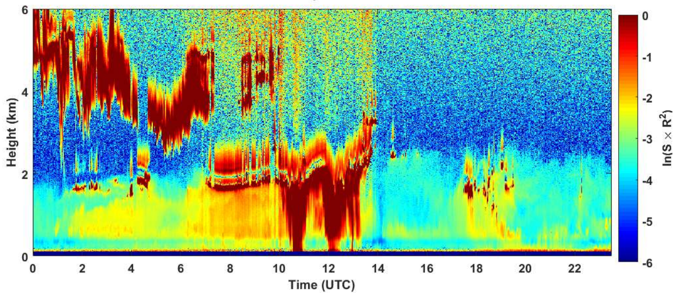
2018-11-16 RCS quick look CHM15k - ILVA LIDAR1 DIREZIONE
