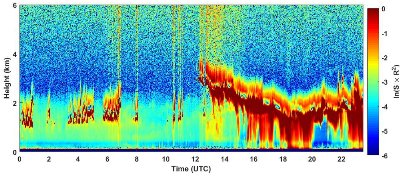
2018-11-18 RCS quick look CHM15k - ILVA LIDAR1 DIREZIONE
