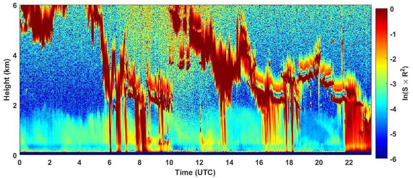
2018-11-26 RCS quick look CHM15k - ILVA LIDAR1 DIREZIONE
