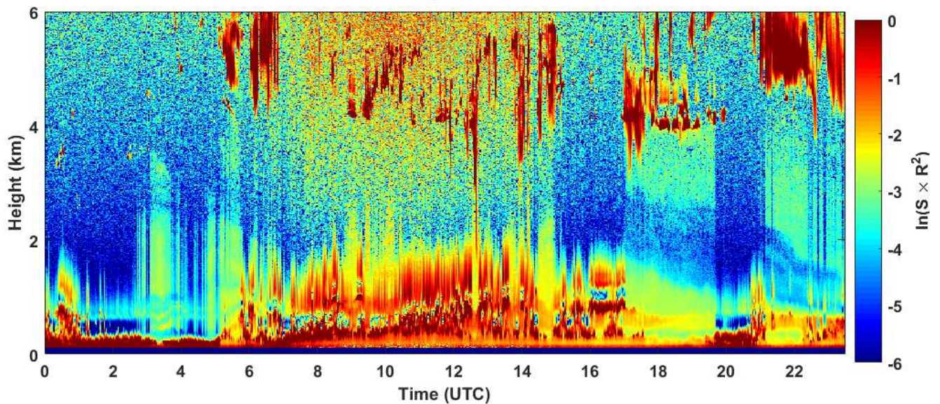
2018-11-02 RCS quick look CHM15k - ILVA LIDAR1 DIREZIONE
