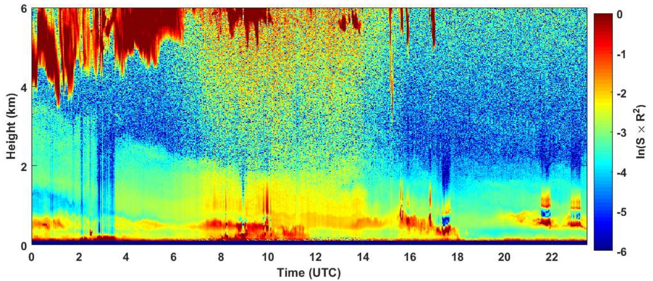
2018-11-04 RCS quick look CHM15k - ILVA LIDAR1 DIREZIONE
