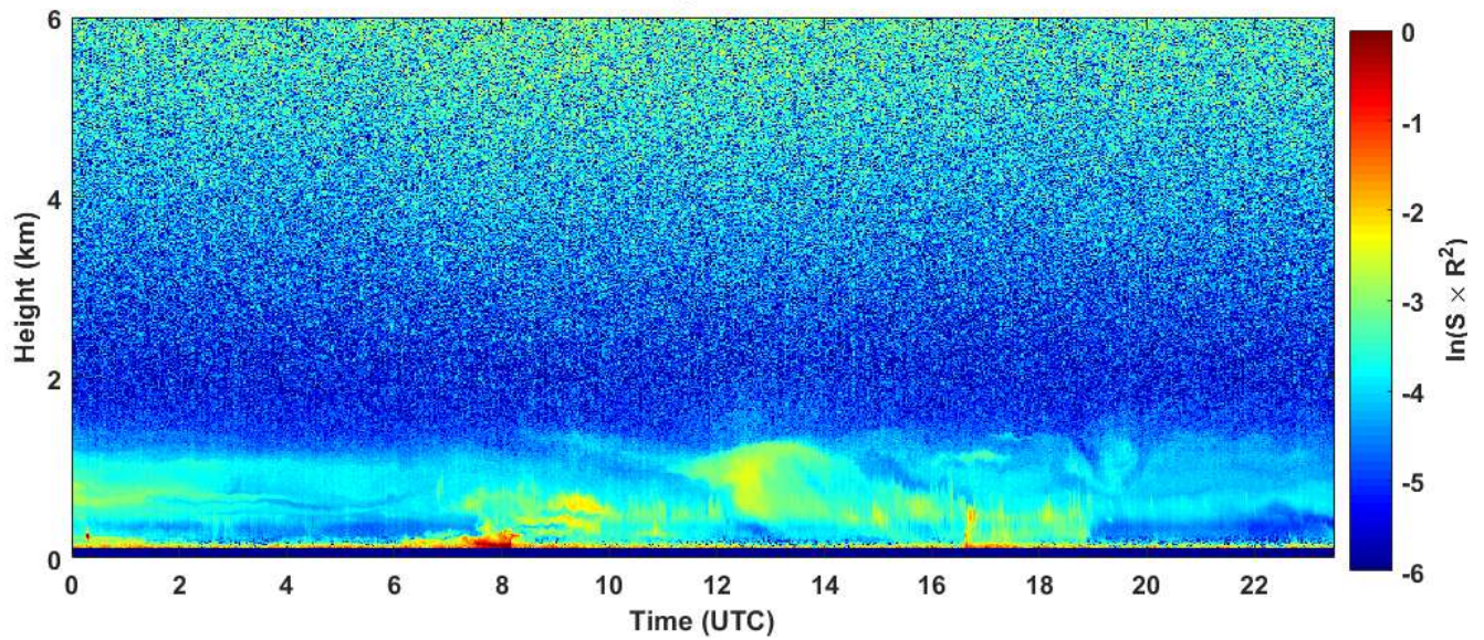
2018-11-14 RCS quick look CHM15k - ILVA LIDAR1 DIREZIONE
