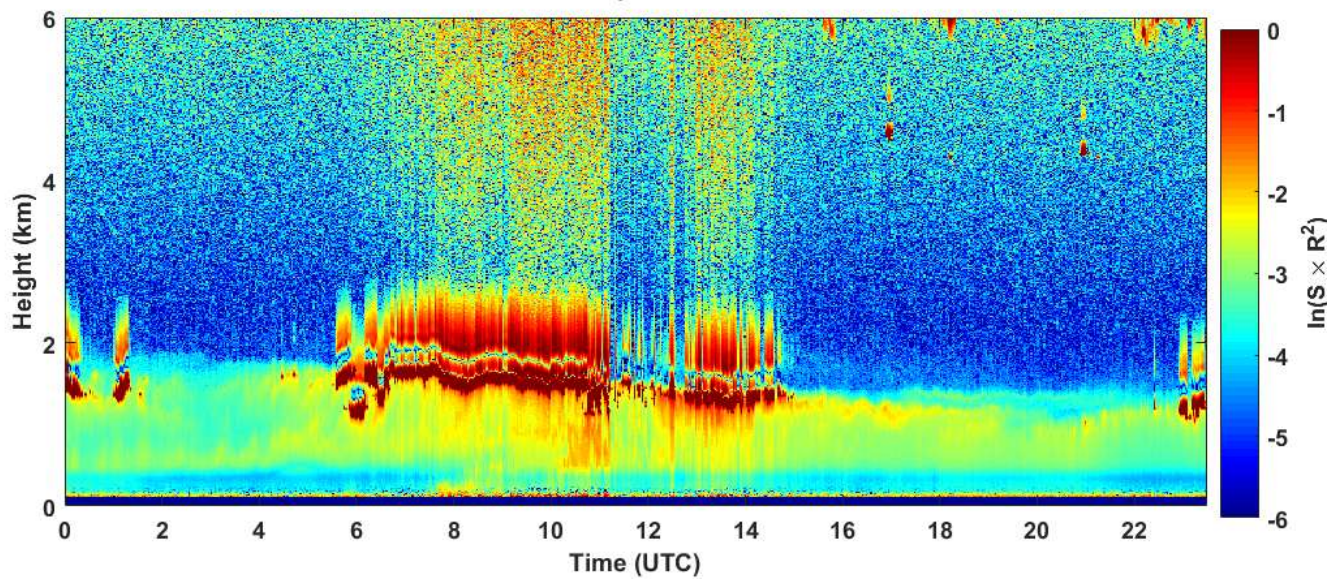
2018-11-30 RCS quick look CHM15k - ILVA LIDAR1 DIREZIONE
