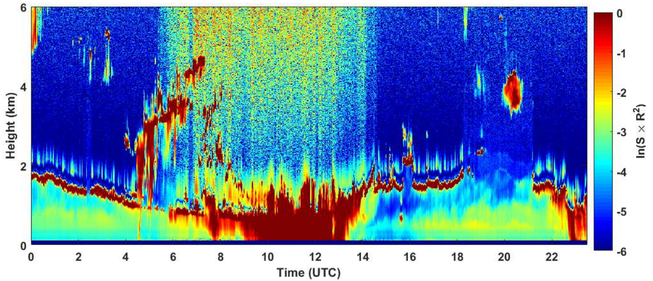
2018-11-29 RCS quick look CHM15k - ILVA LIDAR2 PARCHI
