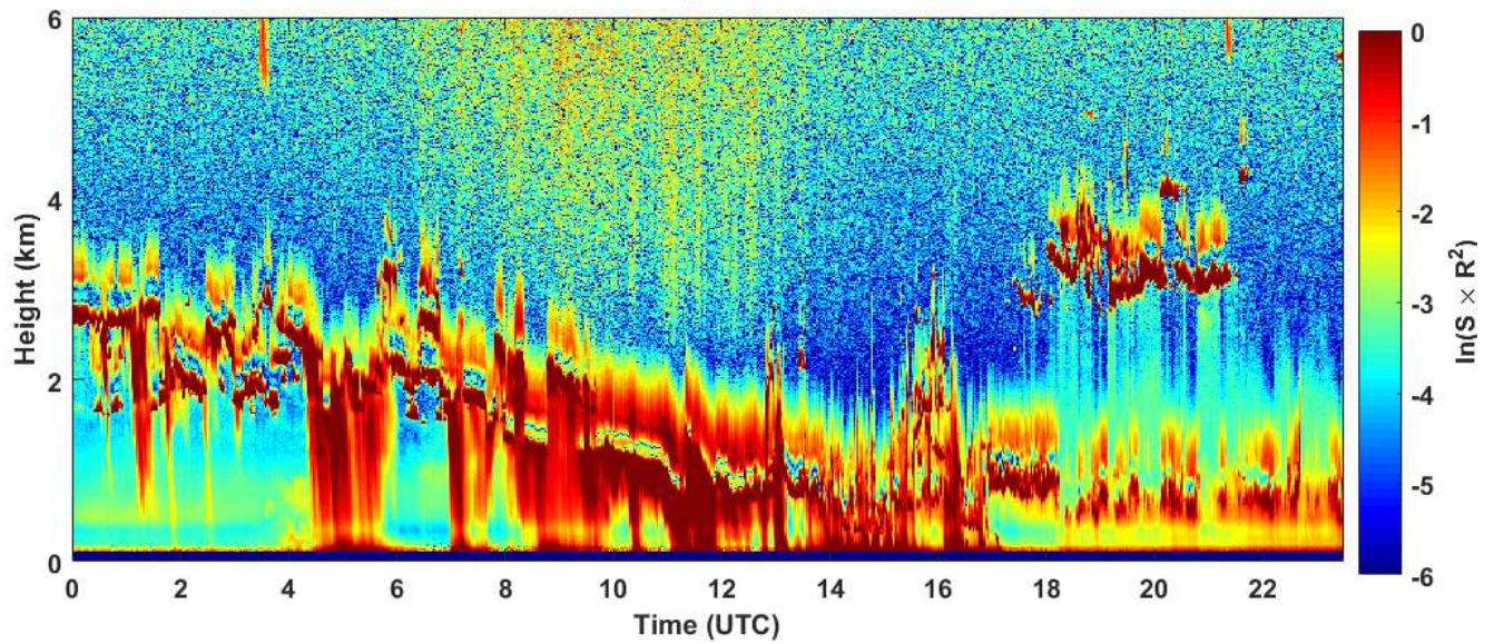
2018-11-20 RCS quick look CHM15k - ILVA LIDAR1 DIREZIONE
