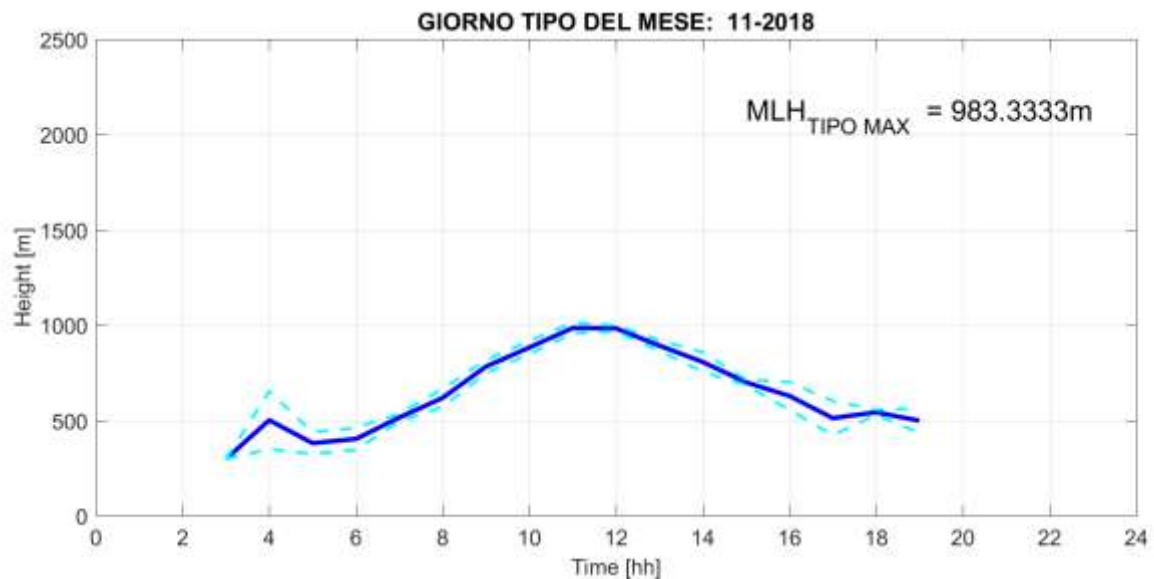
Fig. 2: Giorno tipo del parametro Mixing Layer Height nel mese di NOVEMBRE 2018, rappresentato mediante media oraria (linea blu continua) e deviazione standard (linee celesti tratteggiate).
