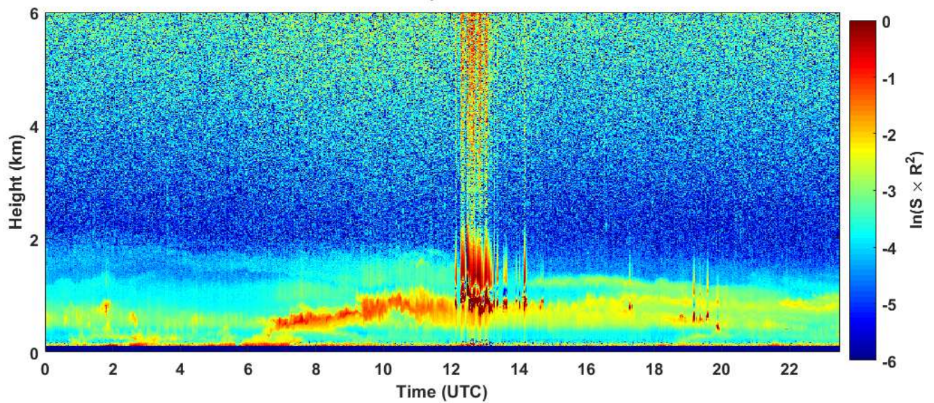
2018-11-12 RCS quick look CHM15k - ILVA LIDAR1 DIREZIONE
