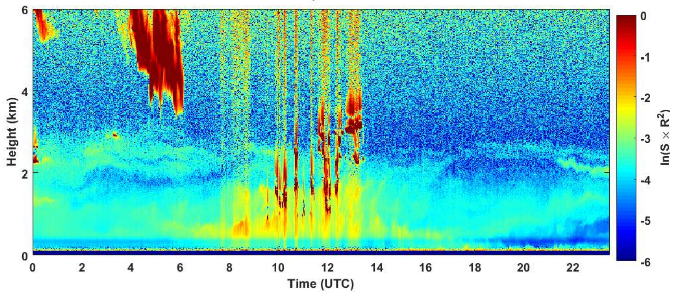
2018-11-08 RCS quick look CHM15k - ILVA LIDAR1 DIREZIONE
