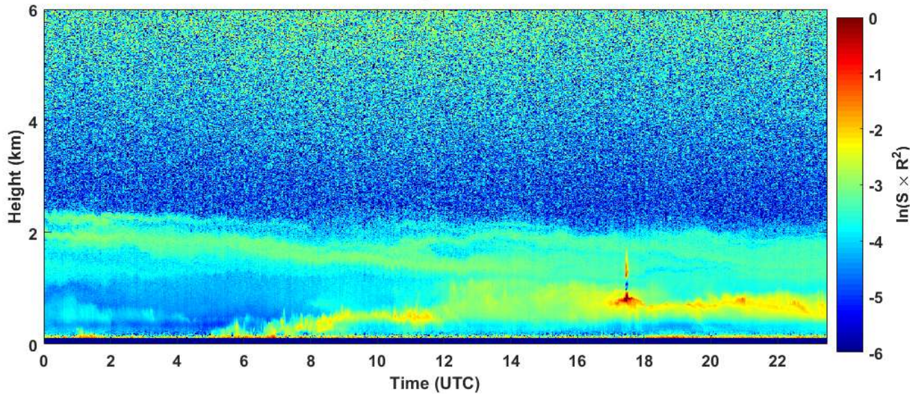
2018-11-10 RCS quick look CHM15k - ILVA LIDAR1 DIREZIONE
