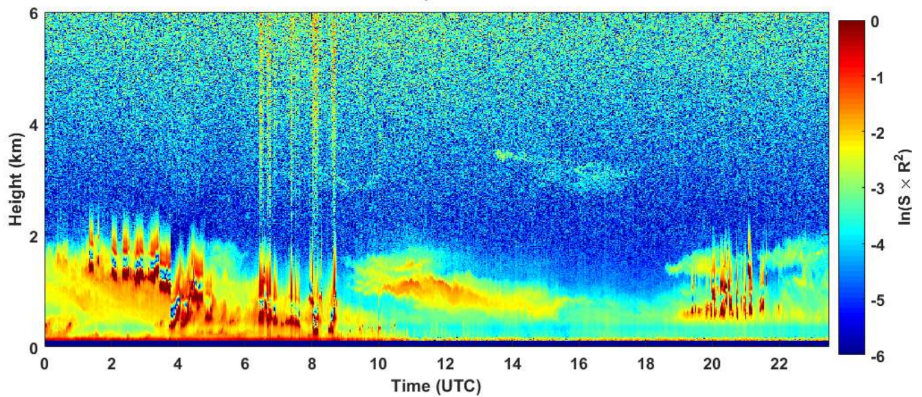
2018-11-06 RCS quick look CHM15k - ILVA LIDAR1 DIREZIONE
