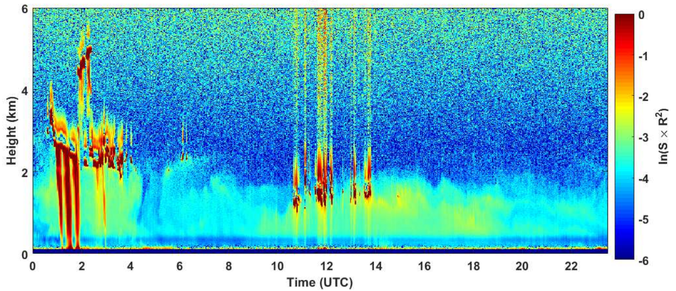
2018-11-22 RCS quick look CHM15k - ILVA LIDAR1 DIREZIONE
