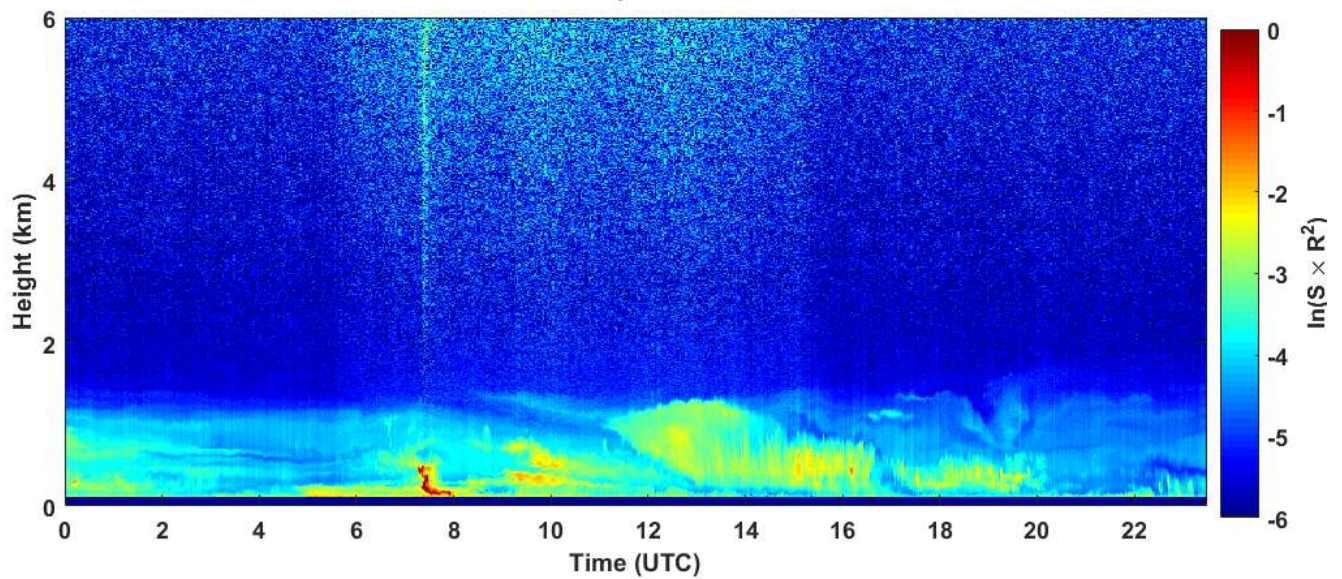
2018-11-13 RCS quick look CHM15k - ILVA LIDAR2 PARCHI
