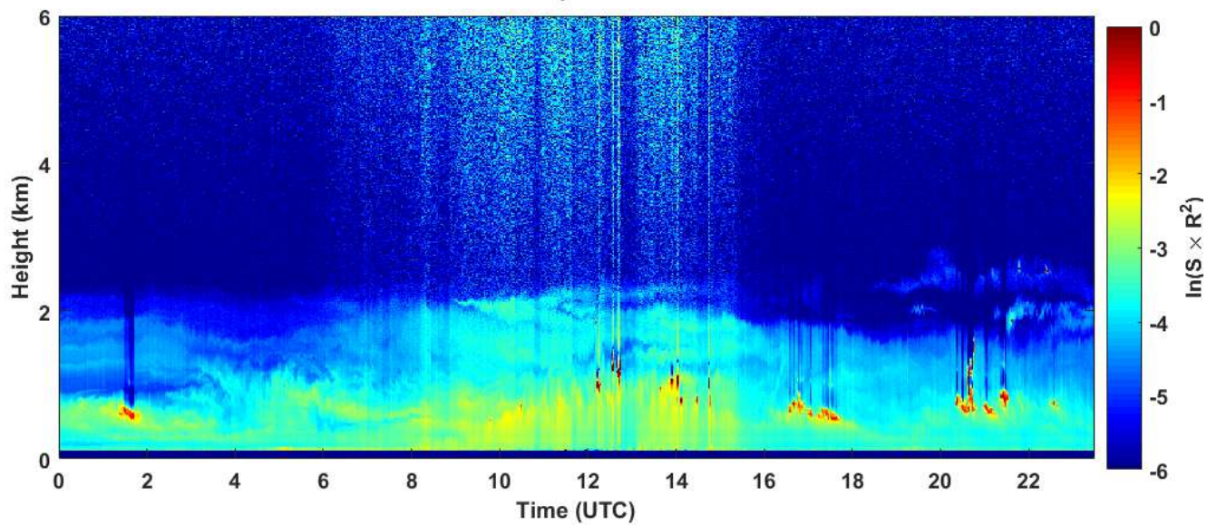
2018-11-10 RCS quick look CHM15k - ILVA LIDAR3 AGGLOMERATO
