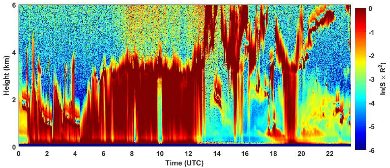
2018-10-06 RCS quick look CHM15k - ILVA LIDAR1 DIREZIONE
