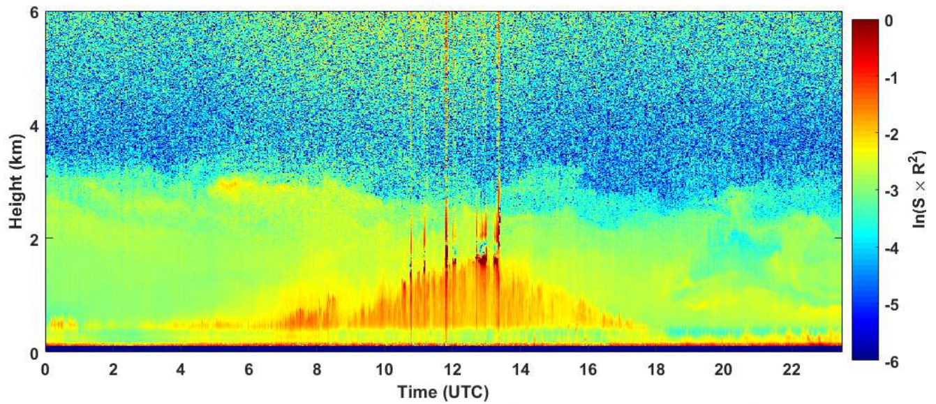
2018-10-14 RCS quick look CHM15k - ILVA LIDAR1 DIREZIONE
