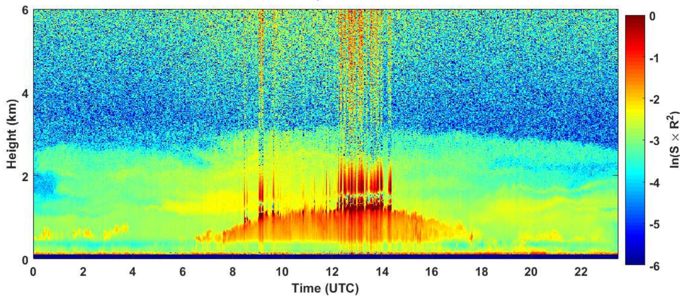
2018-10-10 RCS quick look CHM15k - ILVA LIDAR1 DIREZIONE
