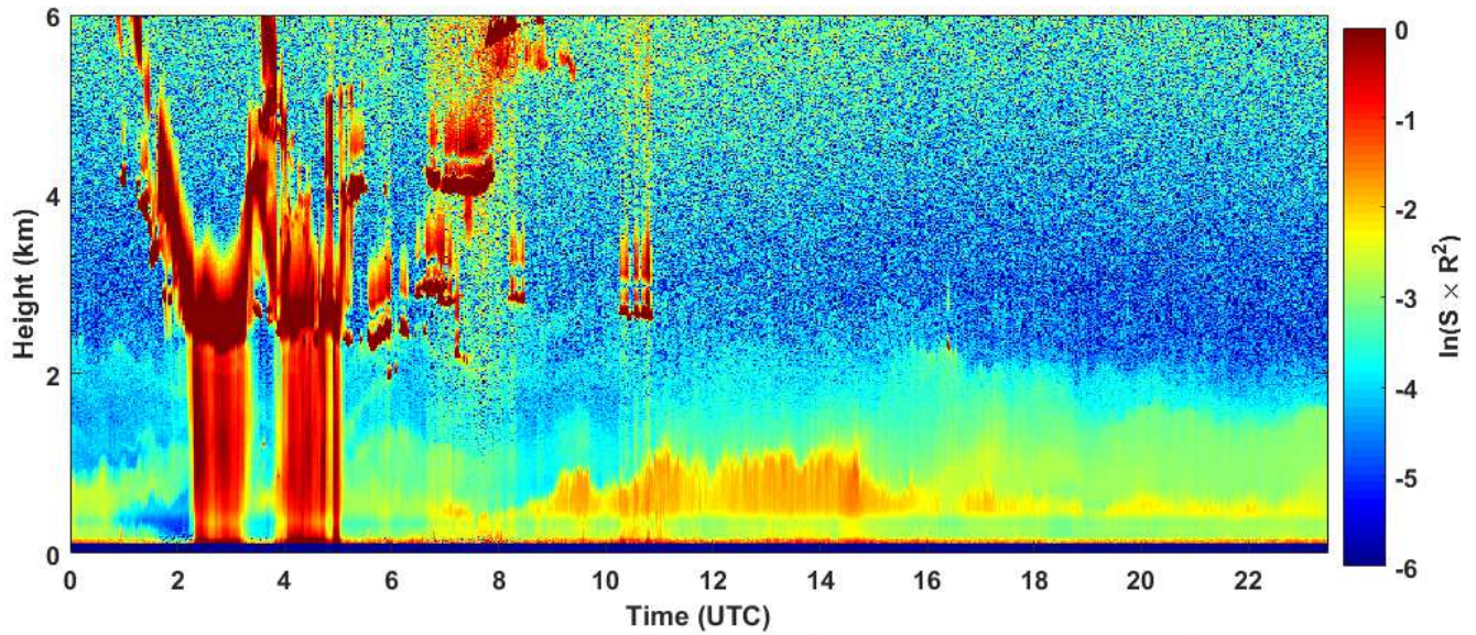
2018-10-24 RCS quick look CHM15k - ILVA LIDAR1 DIREZIONE
