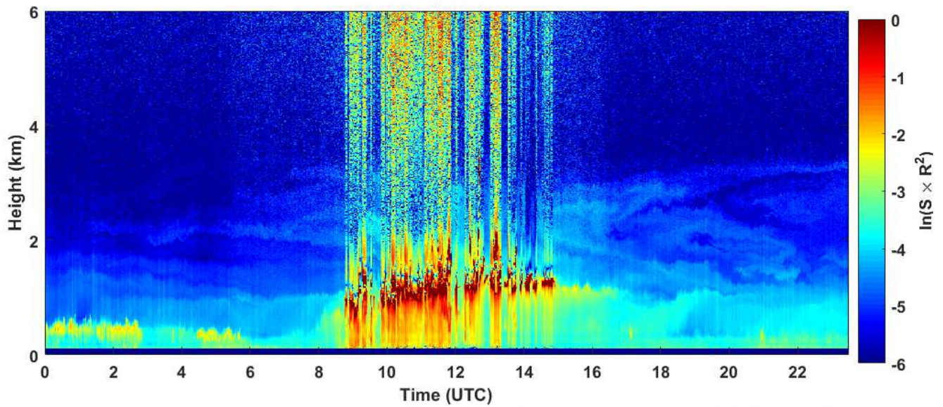
2018-10-10 RCS quick look CHM15k - ILVA LIDAR3 AGGLOMERATO
