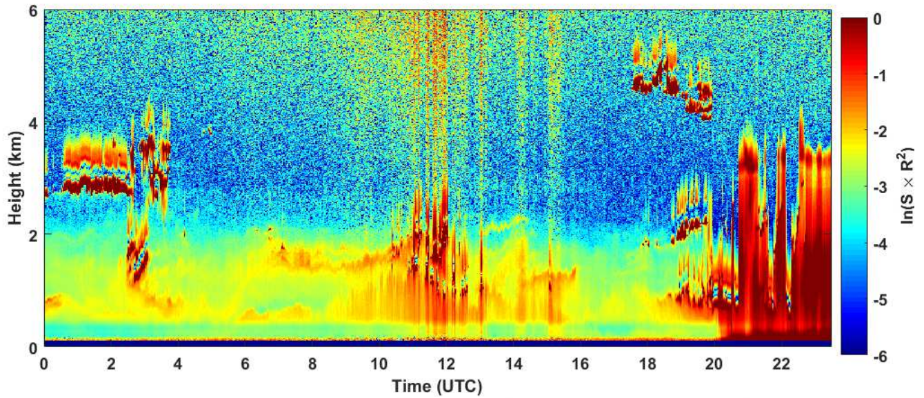
2018-10-16 RCS quick look CHM15k - ILVA LIDAR1 DIREZIONE
