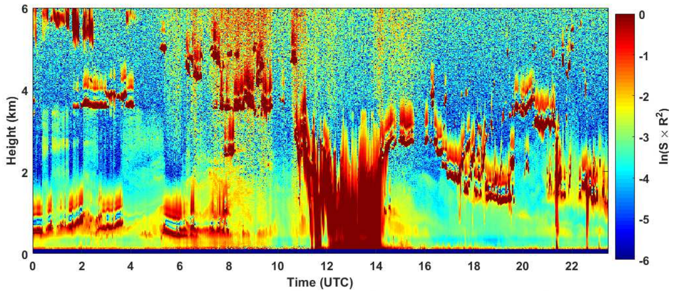
2018-10-04 RCS quick look CHM15k - ILVA LIDAR1 DIREZIONE
