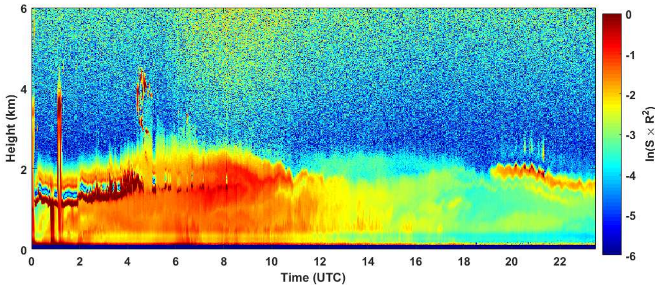
2018-10-30 RCS quick look CHM15k - ILVA LIDAR1 DIREZIONE
