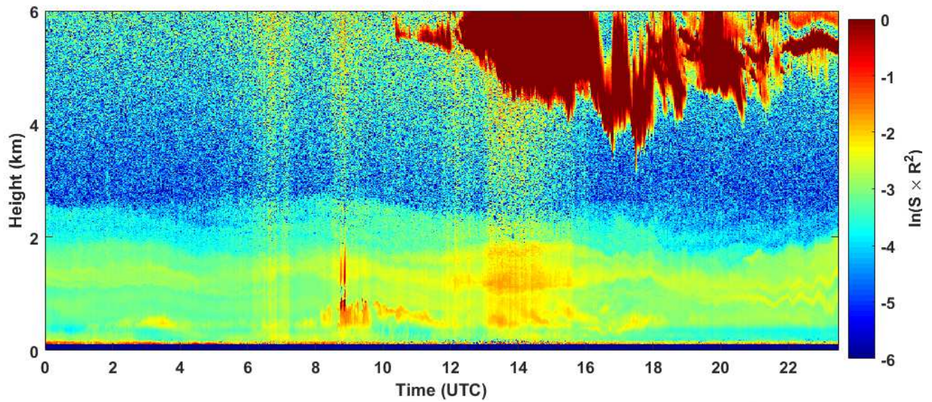
2018-10-12 RCS quick look CHM15k - ILVA LIDAR1 DIREZIONE
