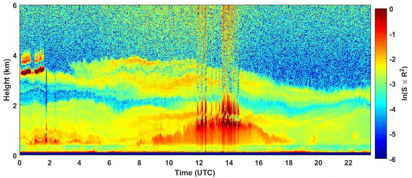
2018-10-20 RCS quick look CHM15k - ILVA LIDAR1 DIREZIONE
