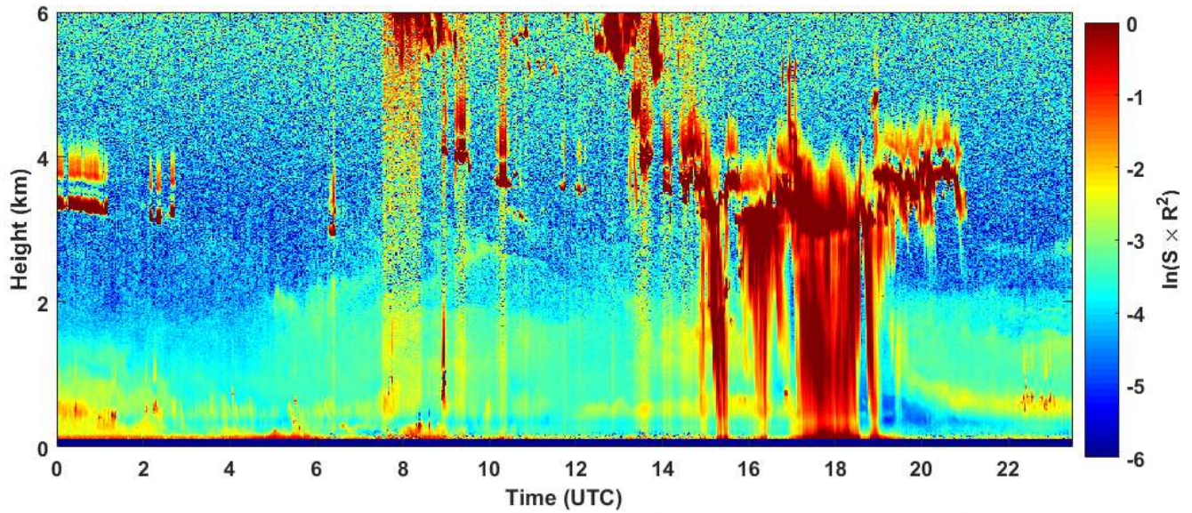
2018-10-08 RCS quick look CHM15k - ILVA LIDAR1 DIREZIONE
