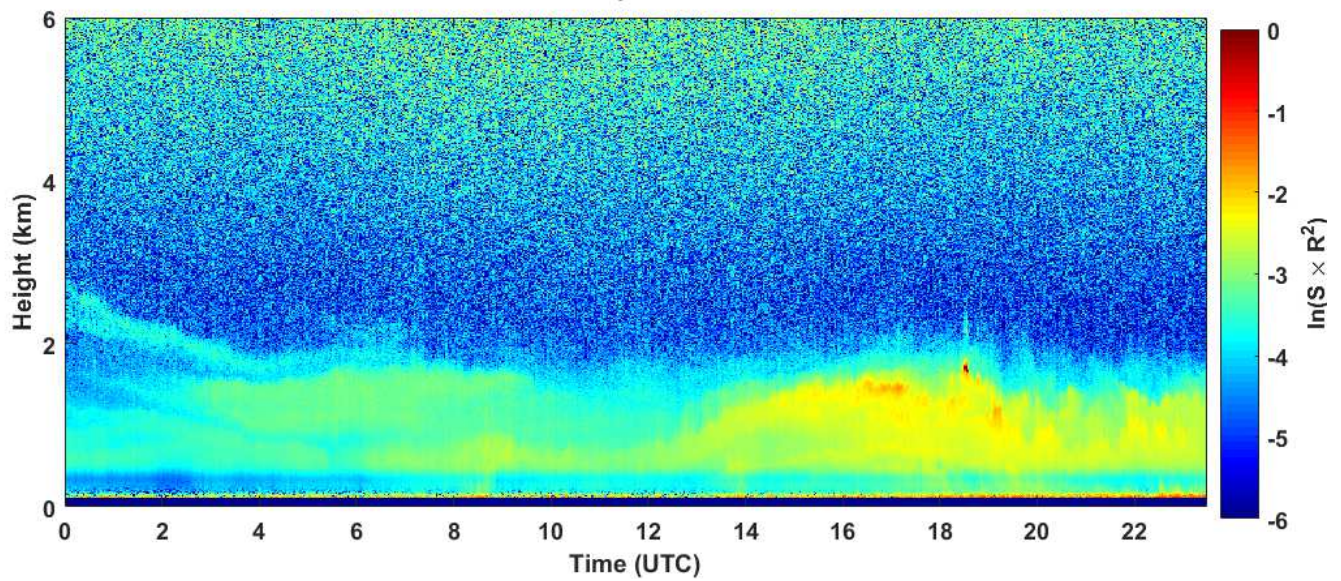
2018-10-26 RCS quick look CHM15k - ILVA LIDAR1 DIREZIONE
