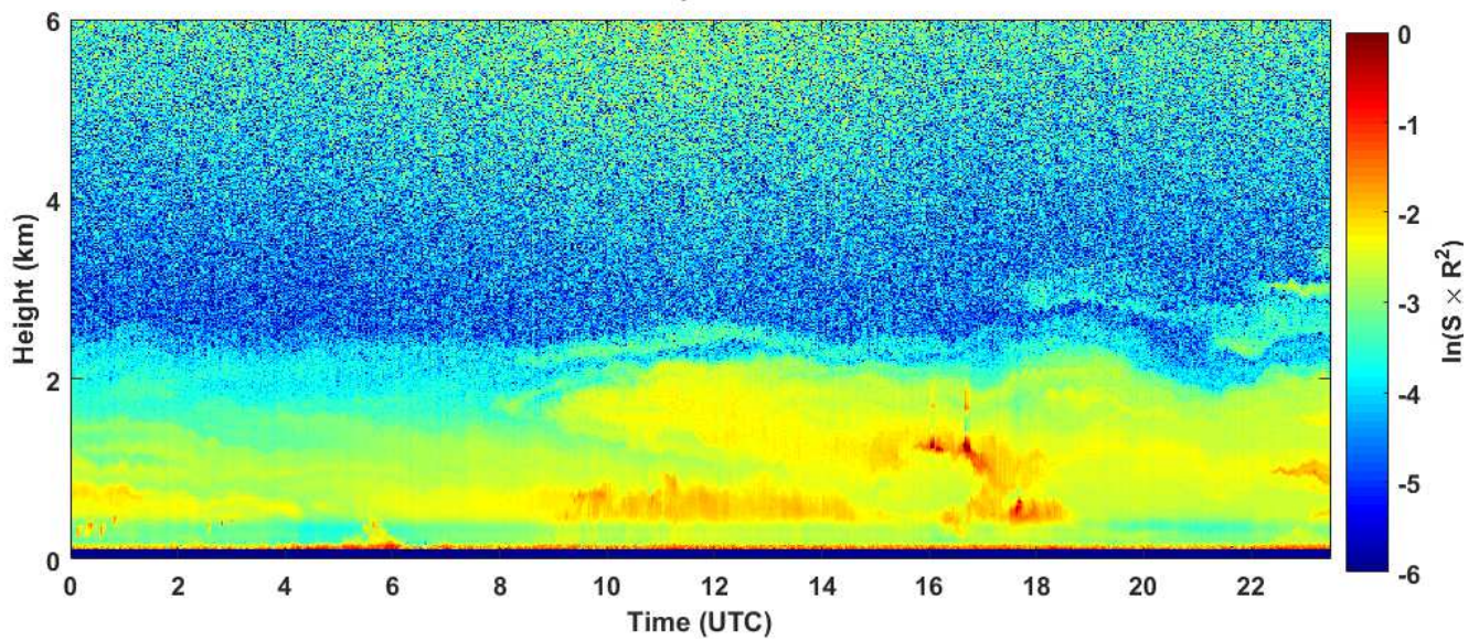
2018-10-18 RCS quick look CHM15k - ILVA LIDAR1 DIREZIONE
