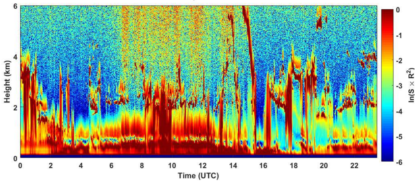
2018-10-28 RCS quick look CHM15k - ILVA LIDAR1 DIREZIONE
