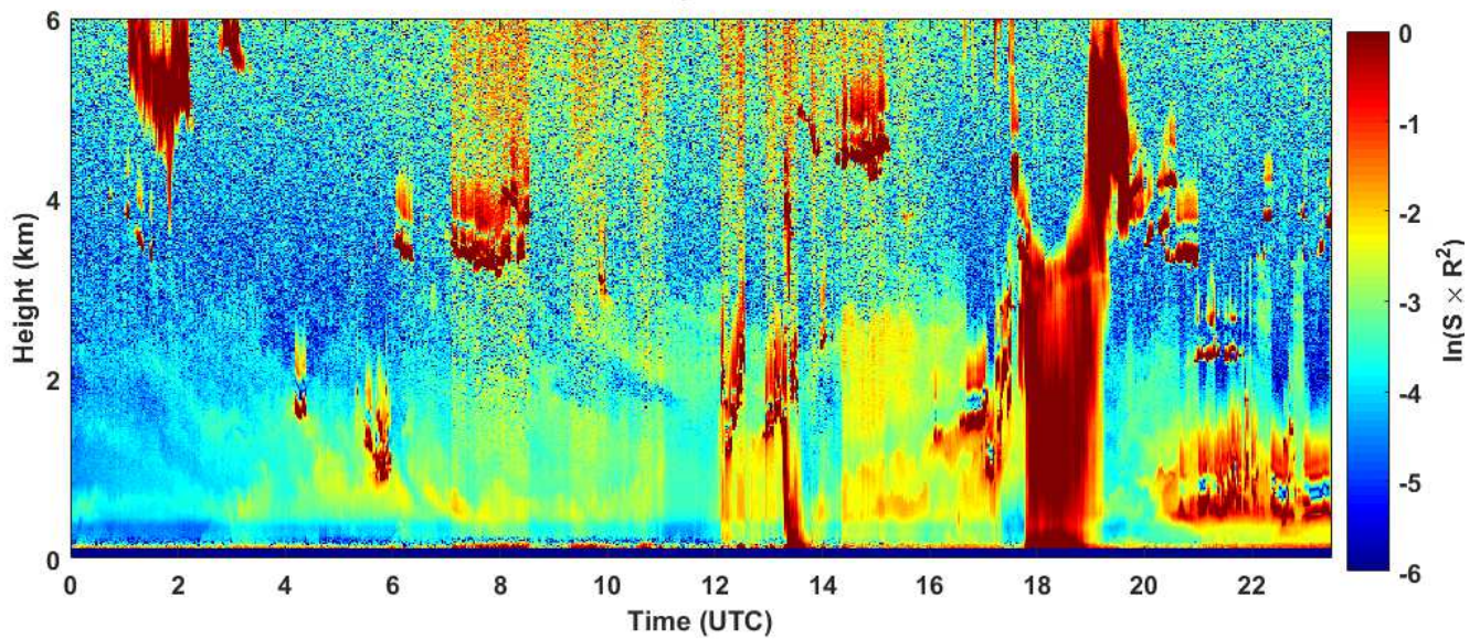
2018-10-02 RCS quick look CHM15k - ILVA LIDAR1 DIREZIONE
