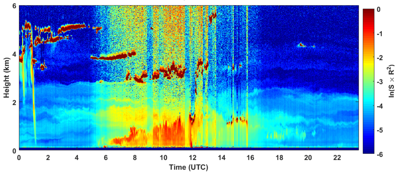
2018-09-20 RCS quick look CHM15k - ILVA LIDAR3 AGGLOMERATO
