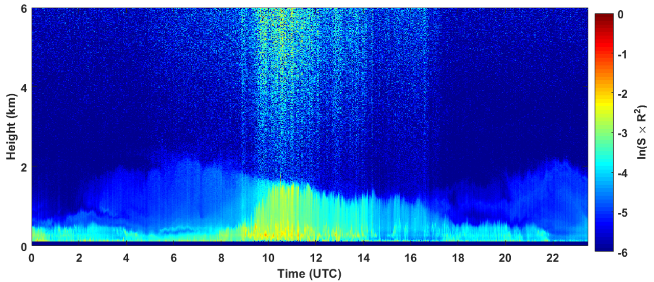
2018-09-12 RCS quick look CHM15k - ILVA LIDAR3 AGGLOMERATO
