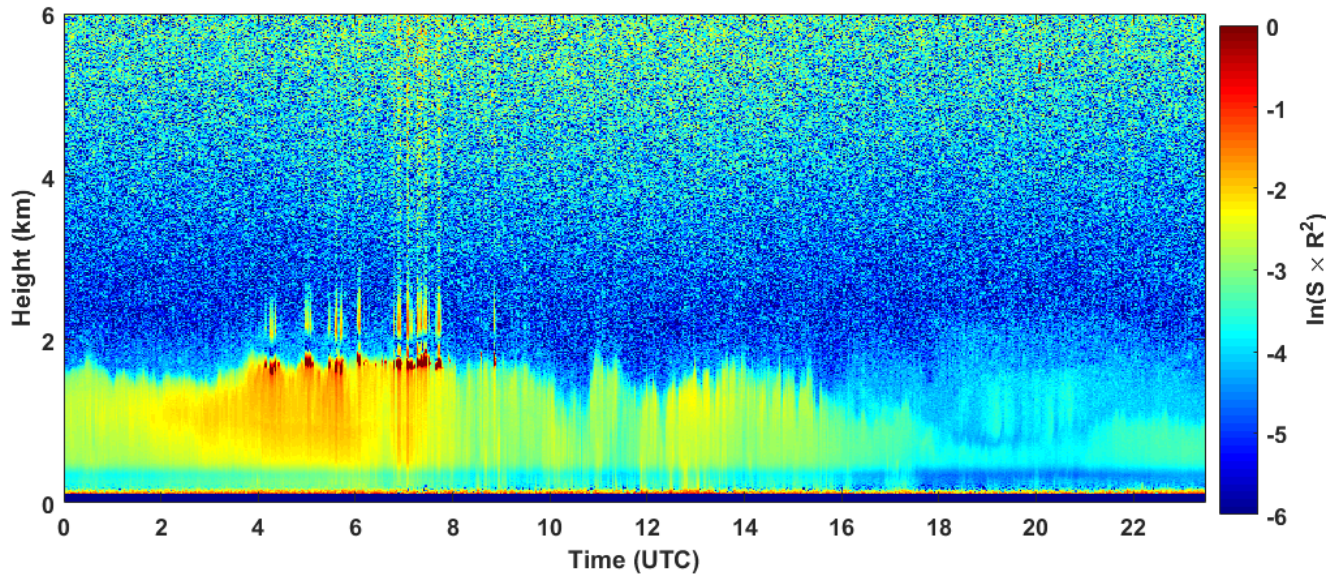
2018-09-28 RCS quick look CHM15k - ILVA LIDAR1 DIREZIONE
