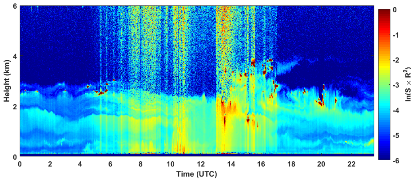
2018-09-14 RCS quick look CHM15k - ILVA LIDAR3 AGGLOMERATO
