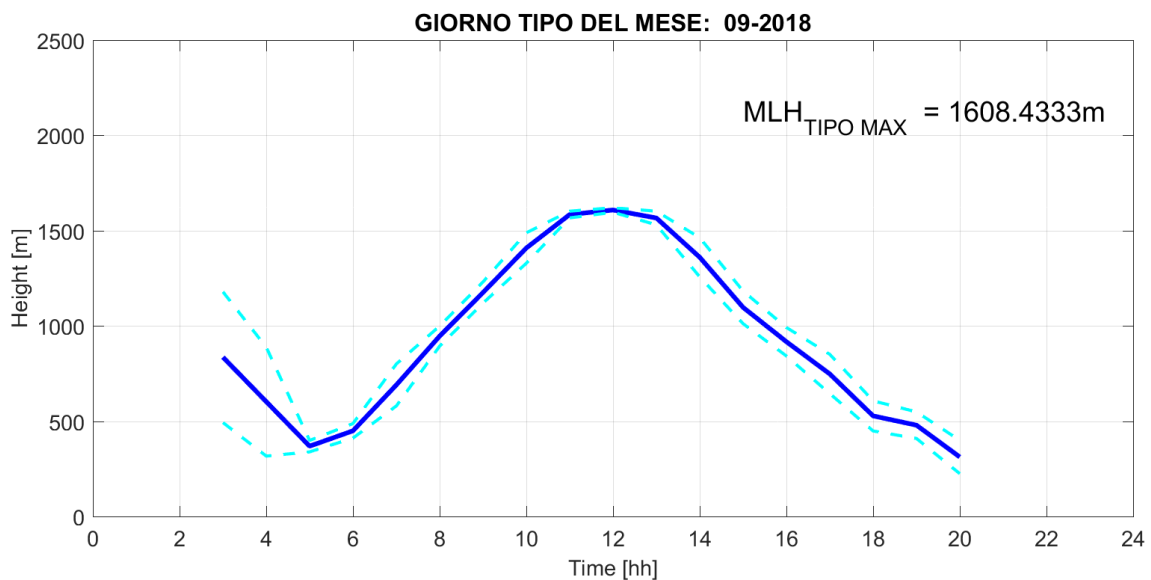
Fig. 2: Giorno tipo del parametro Mixing Layer Height nel mese di SETTEMBRE 2018, rappresentato mediante media oraria (linea blu continua) e deviazione standard (linee celesti tratteggiate).
