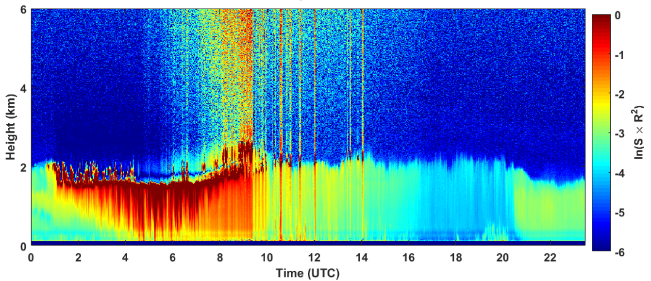
2018-09-26 RCS quick look CHM15k - ILVA LIDAR2 PARCHI
