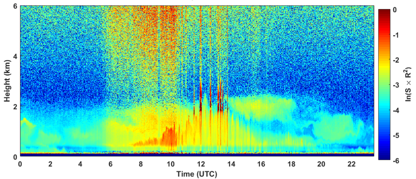
2018-09-10 RCS quick look CHM15k - ILVA LIDAR1 DIREZIONE
