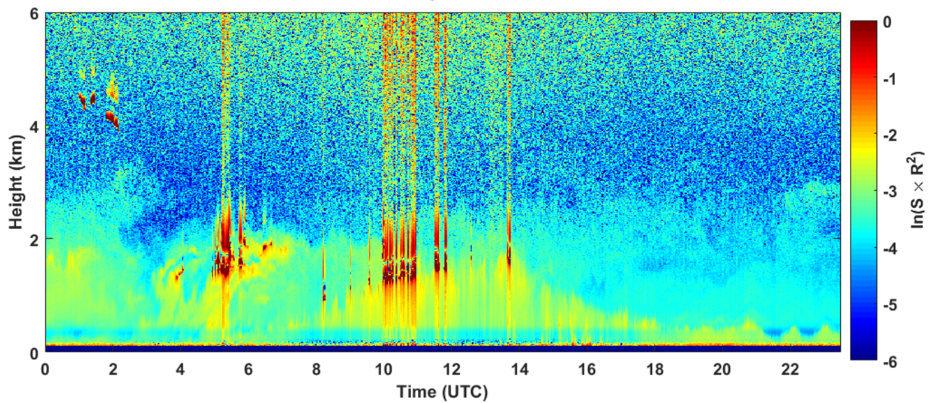
2018-09-08 RCS quick look CHM15k - ILVA LIDAR1 DIREZIONE
