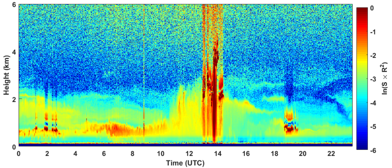
2018-09-16 RCS quick look CHM15k - ILVA LIDAR1 DIREZIONE
