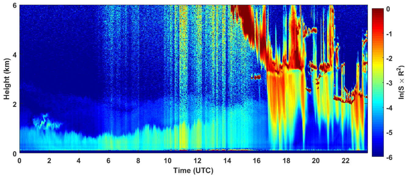
2018-09-28 RCS quick look CHM15k - ILVA LIDAR3 AGGLOMERATO
