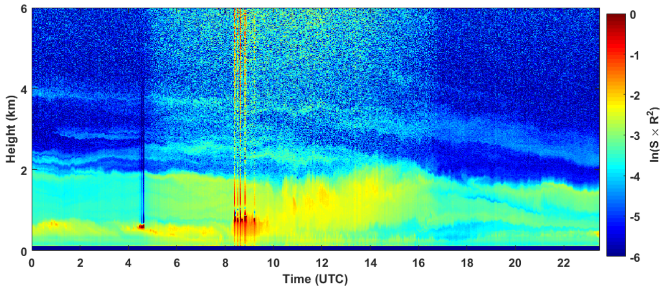
2018-09-22 RCS quick look CHM15k - ILVA LIDAR2 PARCHI
