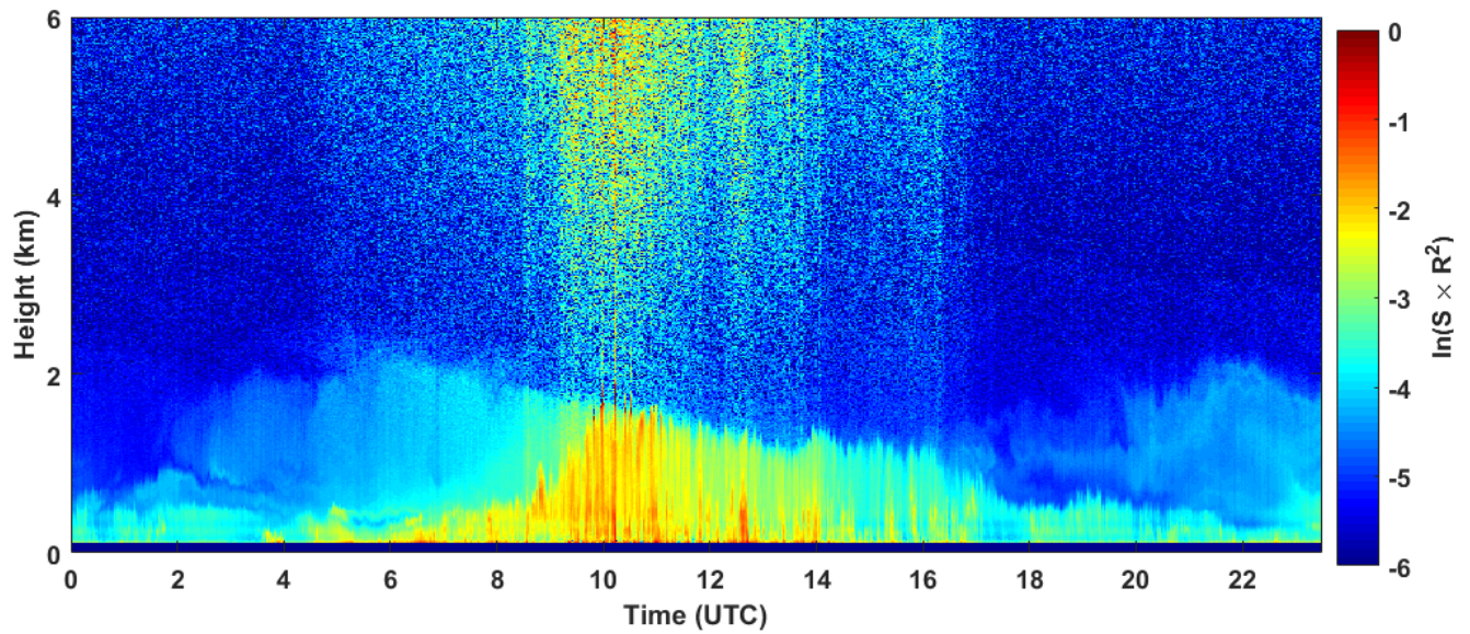
2018-09-12 RCS quick look CHM15k - ILVA LIDAR2 PARCHI
