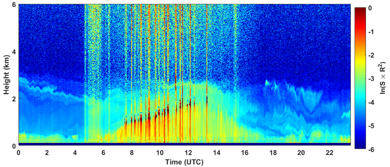
2018-09-10 RCS quick look CHM15k - ILVA LIDAR2 PARCHI
