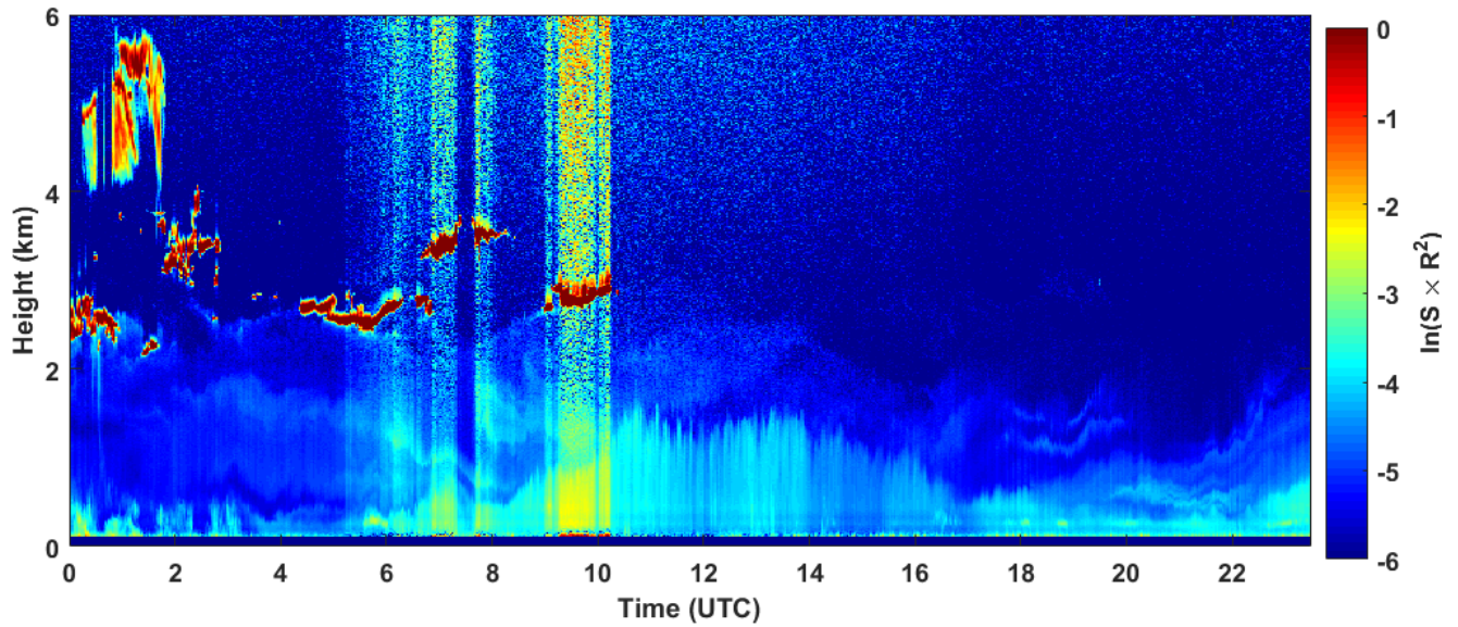
2018-09-30 RCS quick look CHM15k - ILVA LIDAR3 AGGLOMERATO
