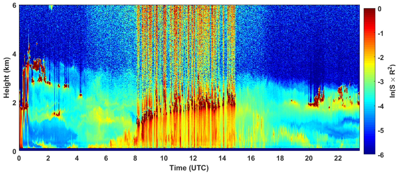
2018-09-06 RCS quick look CHM15k - ILVA LIDAR2 PARCHI
