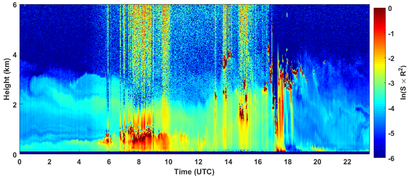
2018-09-08 RCS quick look CHM15k - ILVA LIDAR3 AGGLOMERATO
