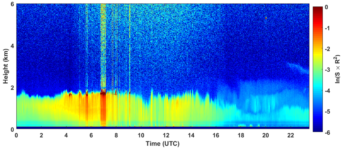
2018-09-28 RCS quick look CHM15k - ILVA LIDAR2 PARCHI
