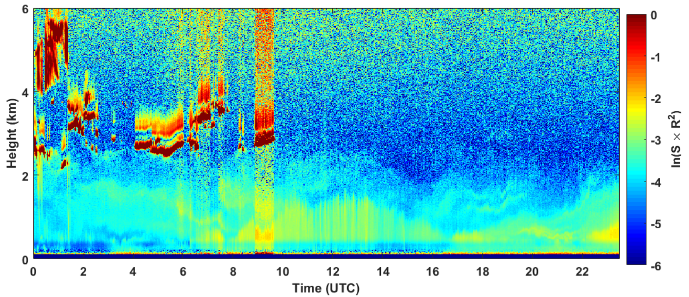
2018-09-30 RCS quick look CHM15k - ILVA LIDAR1 DIREZIONE
