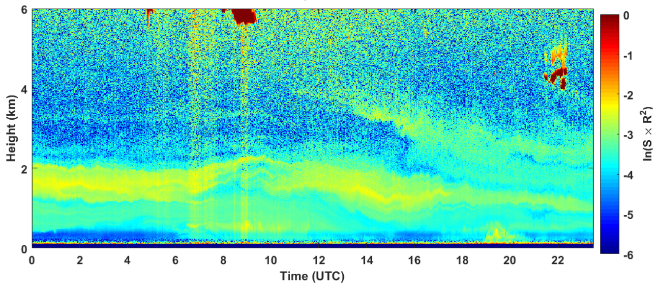
2018-09-18 RCS quick look CHM15k - ILVA LIDAR1 DIREZIONE
