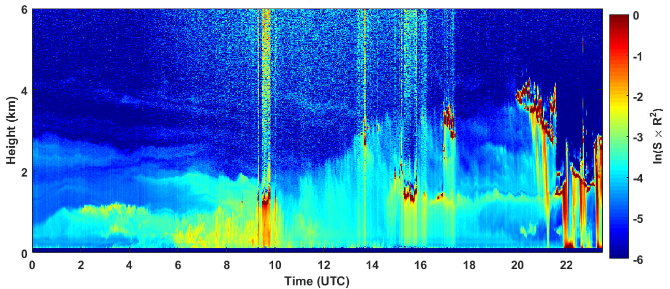
2018-09-04 RCS quick look CHM15k - ILVA LIDAR3 AGGLOMERATO
