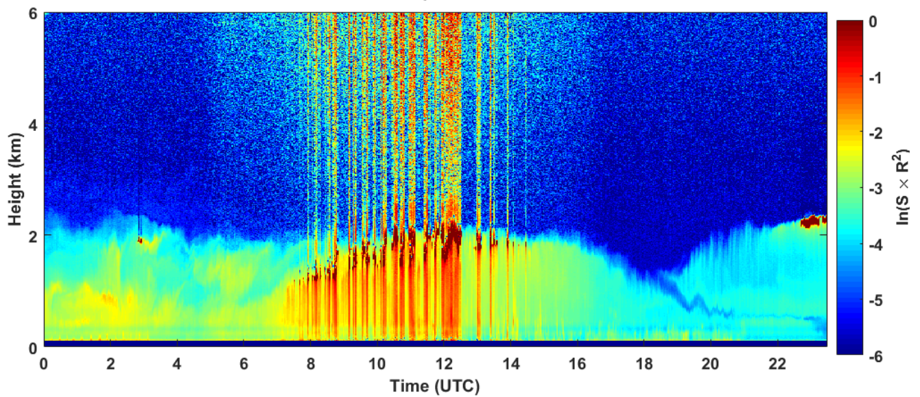
2018-09-30 RCS quick look CHM15k - ILVA LIDAR2 PARCHI
