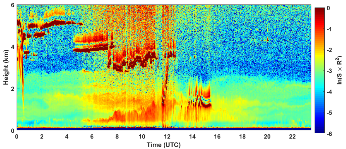
2018-09-20 RCS quick look CHM15k - ILVA LIDAR1 DIREZIONE
