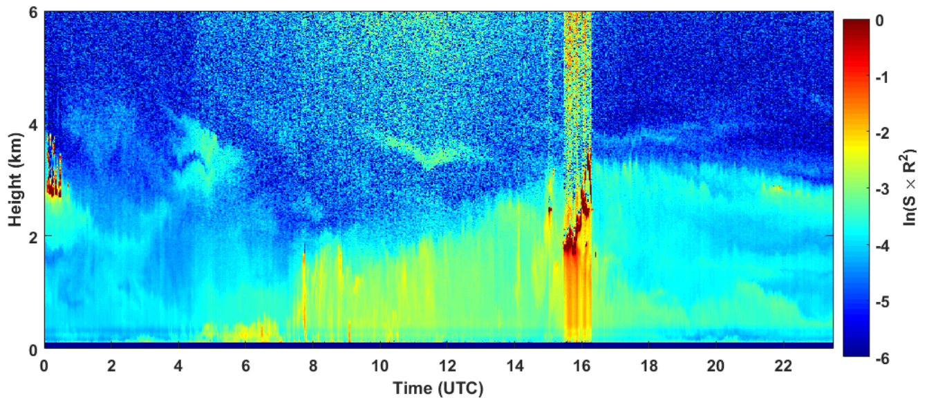
2018-09-04 RCS quick look CHM15k - ILVA LIDAR2 PARCHI
