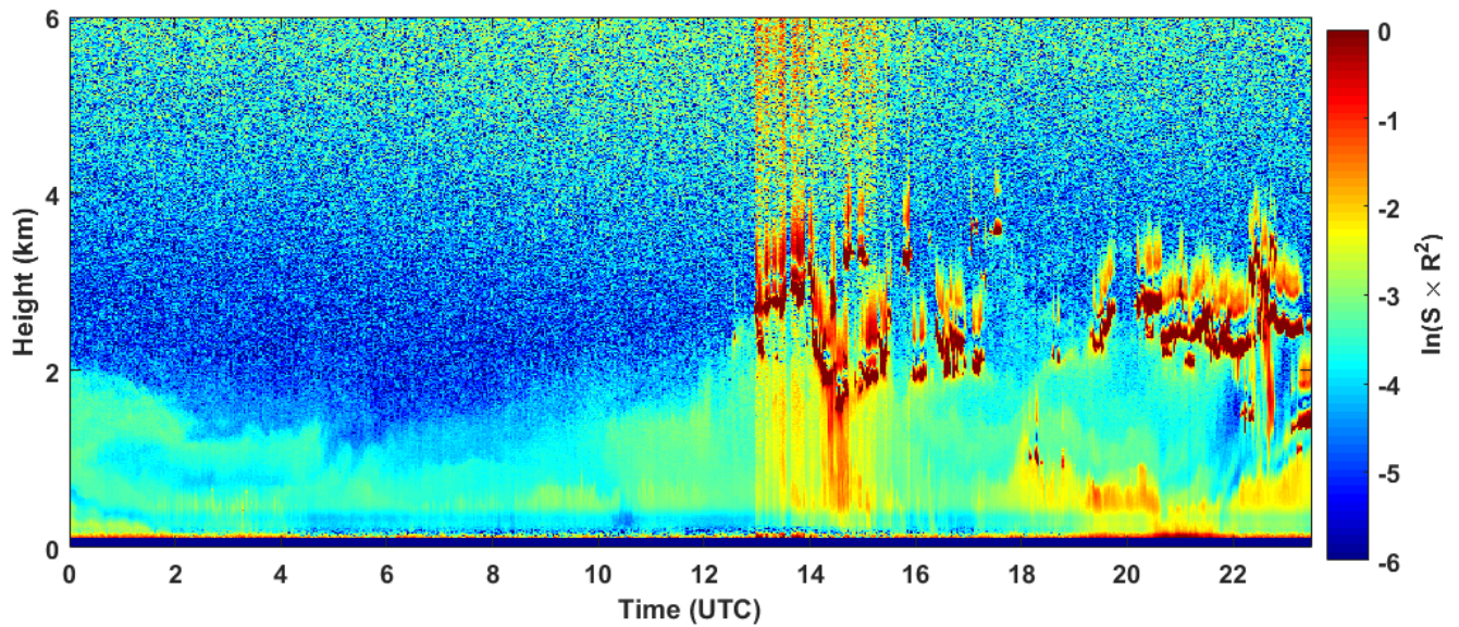
2018-09-24 RCS quick look CHM15k - ILVA LIDAR1 DIREZIONE
