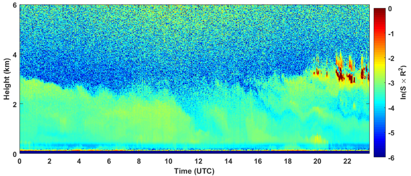
2018-09-02 RCS quick look CHM15k - ILVA LIDAR1 DIREZIONE
