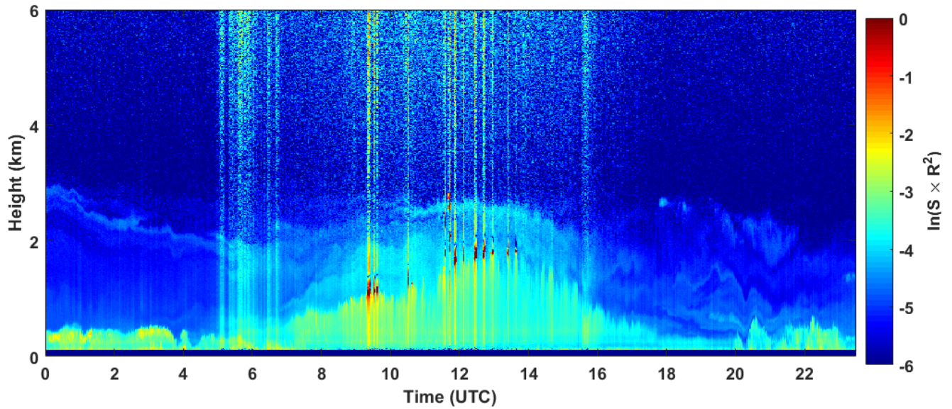
2018-09-10 RCS quick look CHM15k - ILVA LIDAR3 AGGLOMERATO
