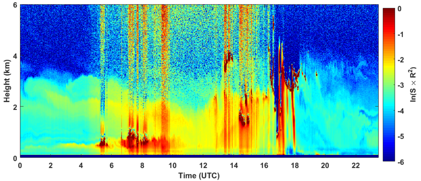
2018-09-08 RCS quick look CHM15k - ILVA LIDAR2 PARCHI
