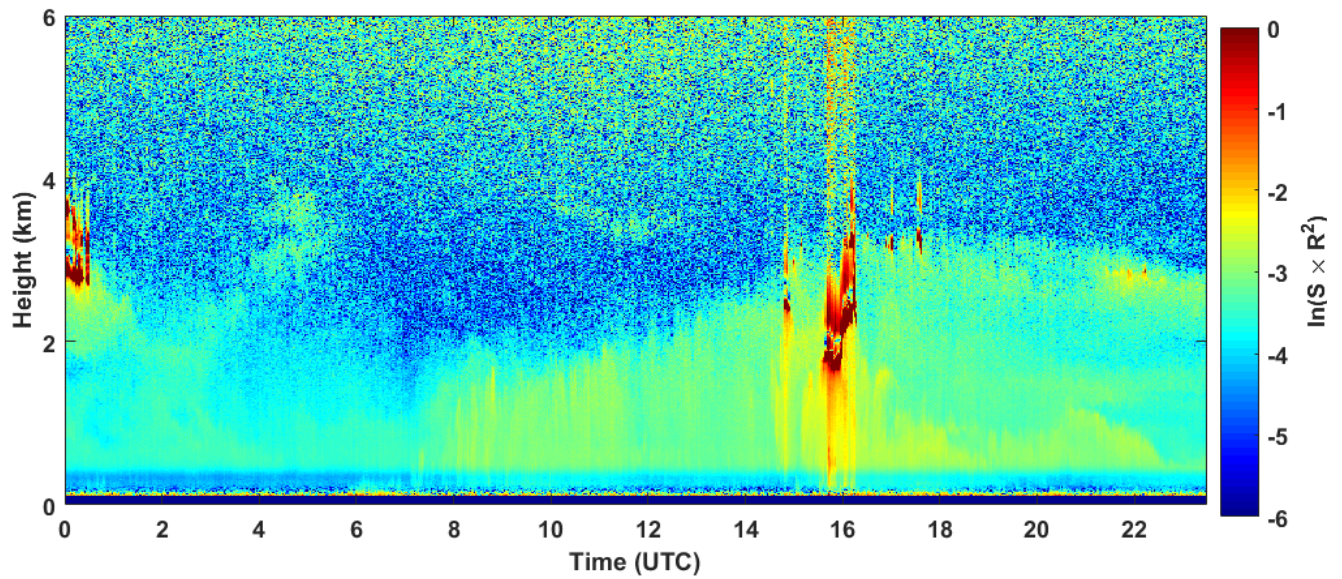
2018-09-04 RCS quick look CHM15k - ILVA LIDAR1 DIREZIONE
