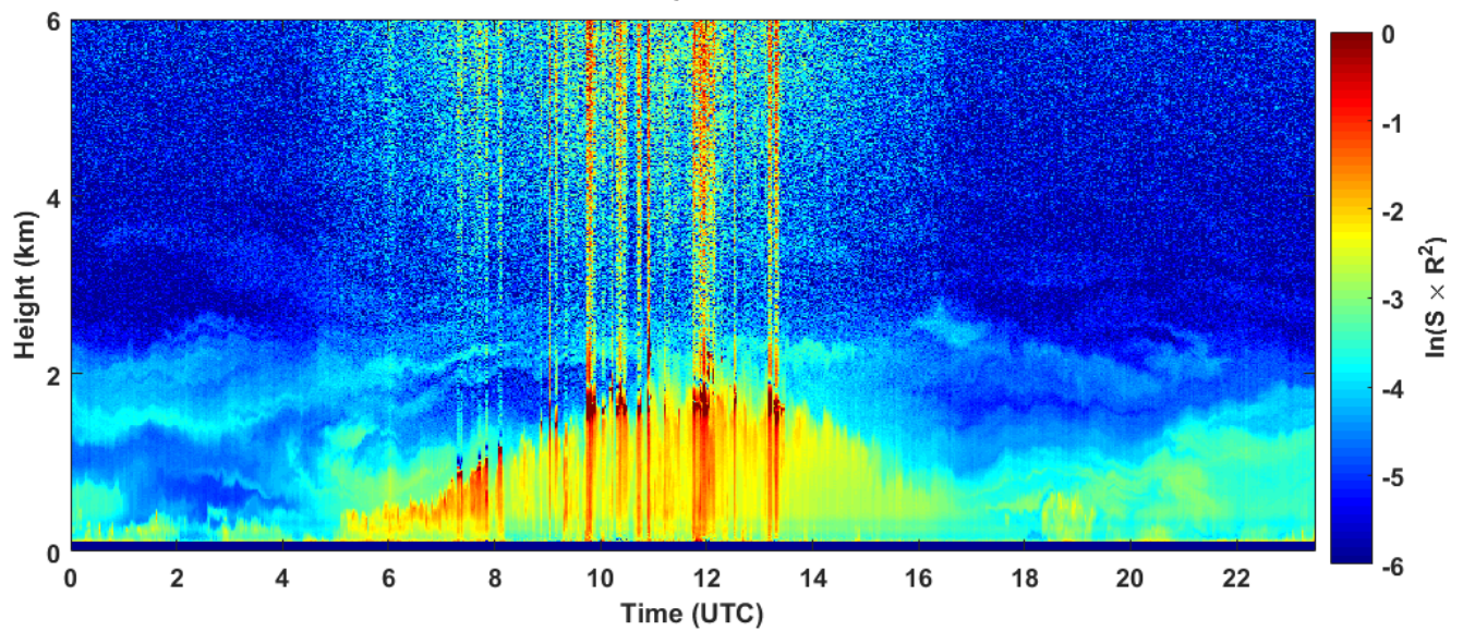
2018-09-16 RCS quick look CHM15k - ILVA LIDAR2 PARCHI
