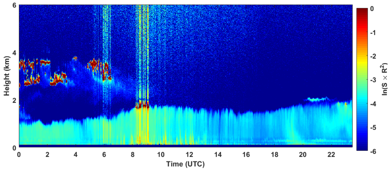
2018-09-26 RCS quick look CHM15k - ILVA LIDAR3 AGGLOMERATO
