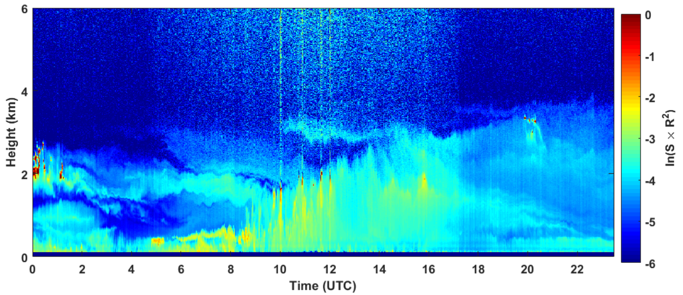
2018-09-06 RCS quick look CHM15k - ILVA LIDAR3 AGGLOMERATO
