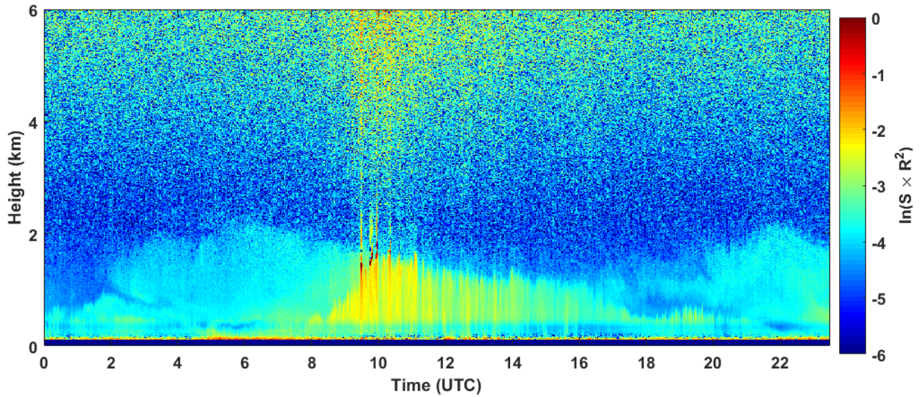
2018-09-12 RCS quick look CHM15k - ILVA LIDAR1 DIREZIONE
