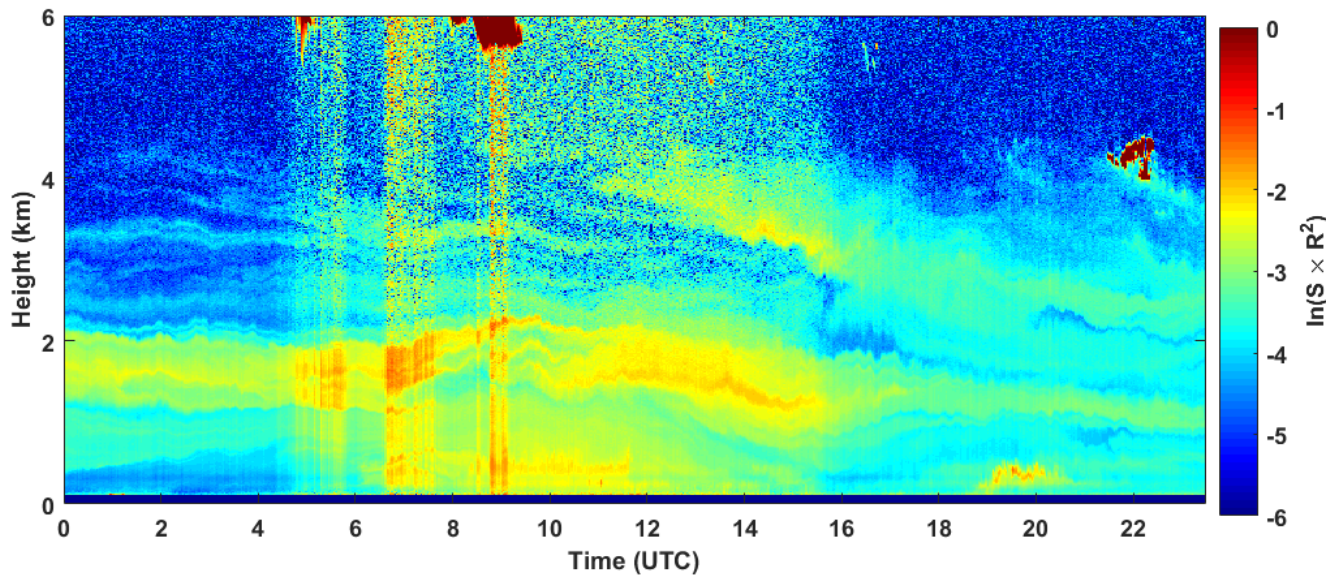
2018-09-18 RCS quick look CHM15k - ILVA LIDAR2 PARCHI
