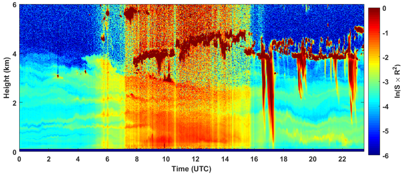
2018-09-20 RCS quick look CHM15k - ILVA LIDAR2 PARCHI
