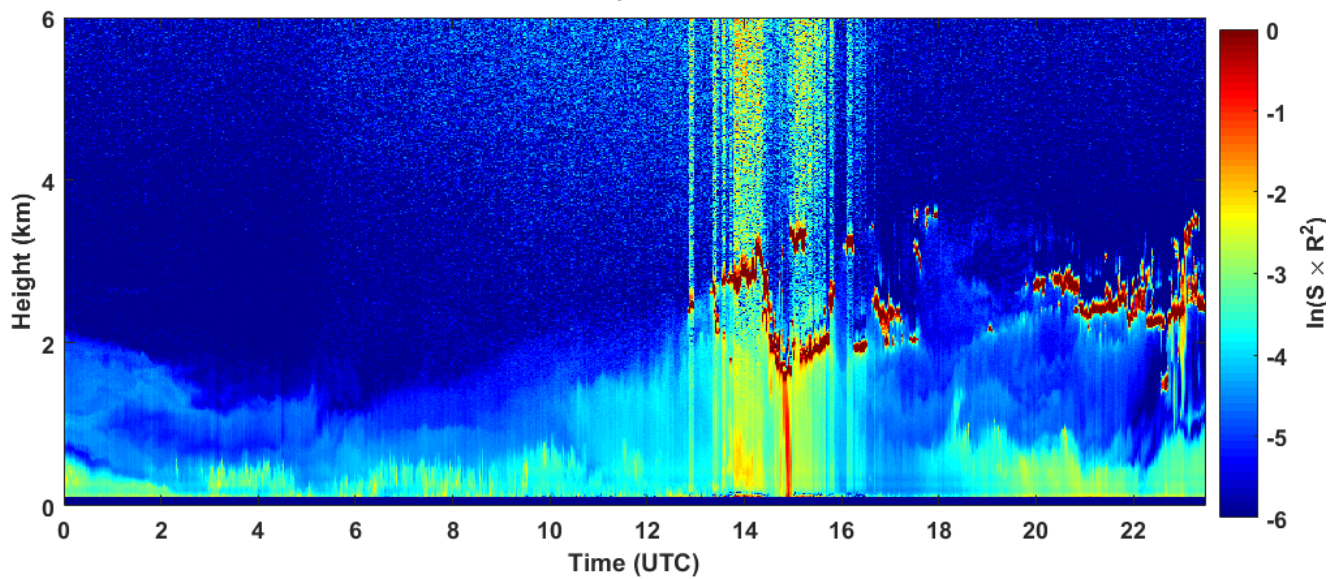
2018-09-24 RCS quick look CHM15k - ILVA LIDAR3 AGGLOMERATO
