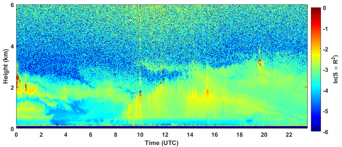
2018-09-06 RCS quick look CHM15k - ILVA LIDAR1 DIREZIONE
