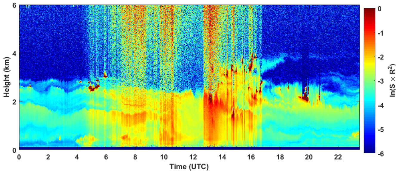
2018-09-14 RCS quick look CHM15k - ILVA LIDAR2 PARCHI
