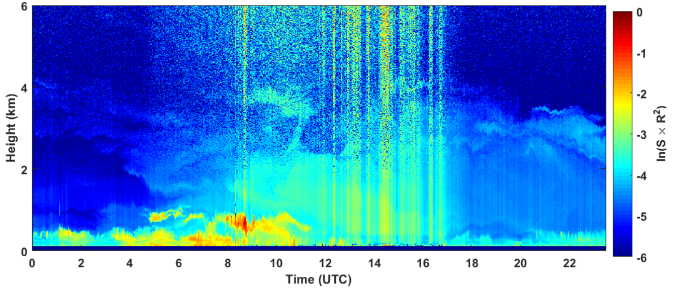
2018-09-02 RCS quick look CHM15k - ILVA LIDAR3 AGGLOMERATO
