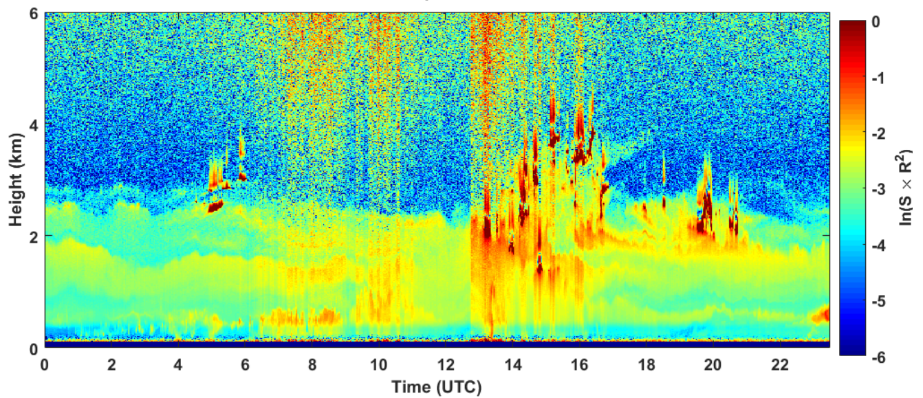
2018-09-14 RCS quick look CHM15k - ILVA LIDAR1 DIREZIONE
