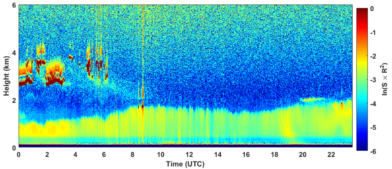
2018-09-26 RCS quick look CHM15k - ILVA LIDAR1 DIREZIONE
