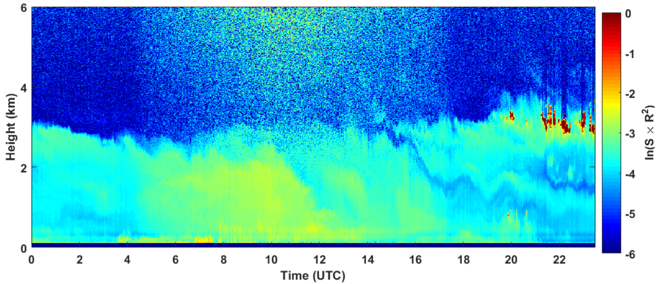
2018-09-02 RCS quick look CHM15k - ILVA LIDAR2 PARCHI
