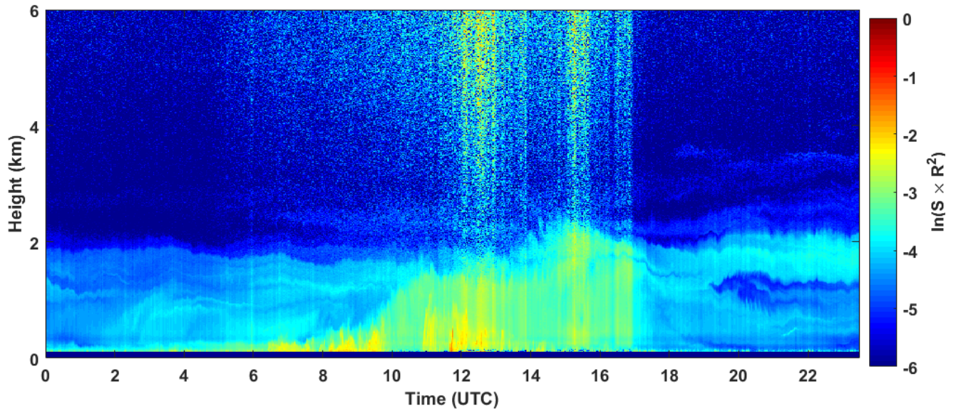
2018-09-18 RCS quick look CHM15k - ILVA LIDAR3 AGGLOMERATO
