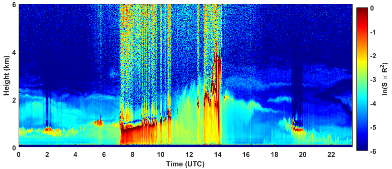
2018-09-16 RCS quick look CHM15k - ILVA LIDAR3 AGGLOMERATO
