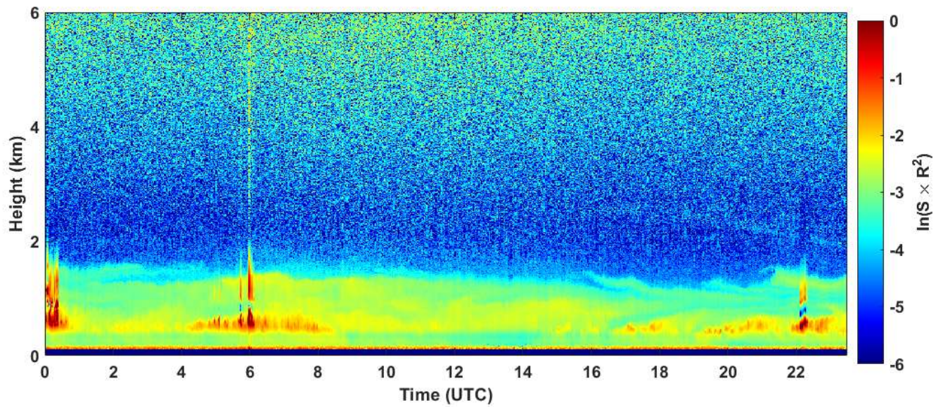
2019-10-20 RCS quick look CHM15k - ILVA LIDAR1 DIREZIONE
