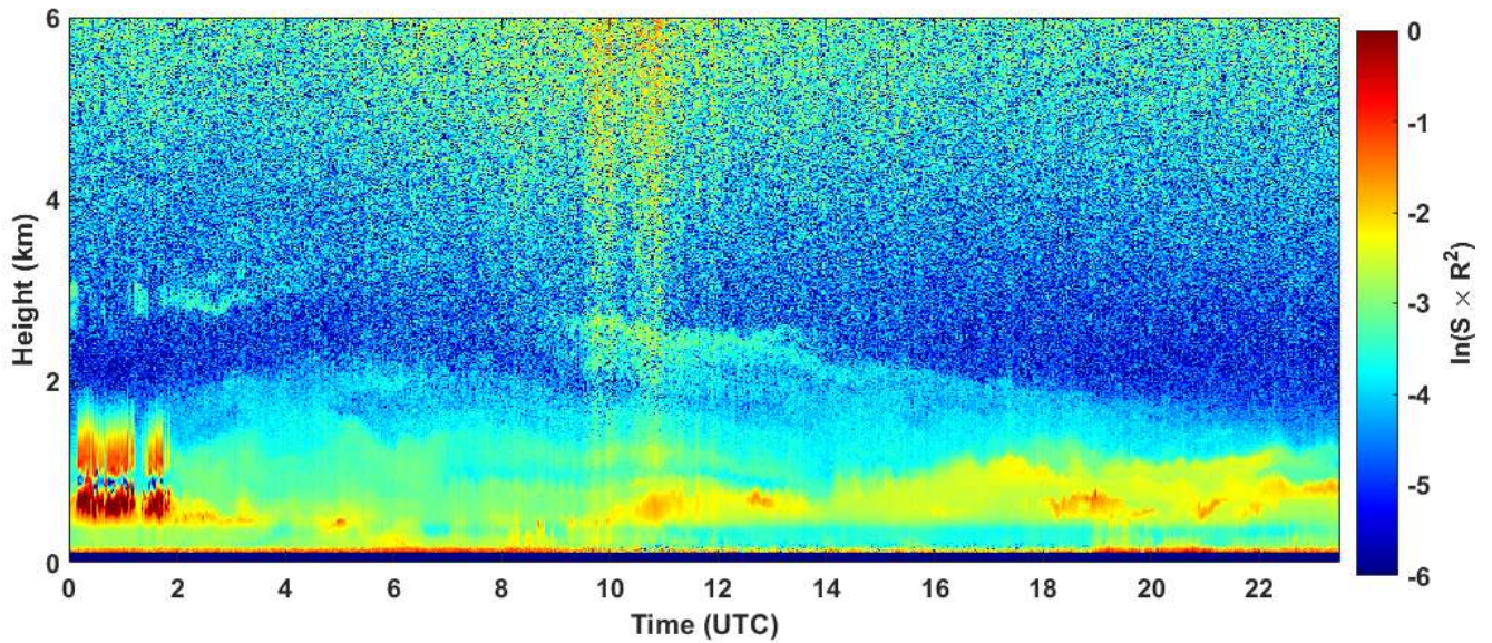
2019-10-26 RCS quick look CHM15k - ILVA LIDAR1 DIREZIONE
