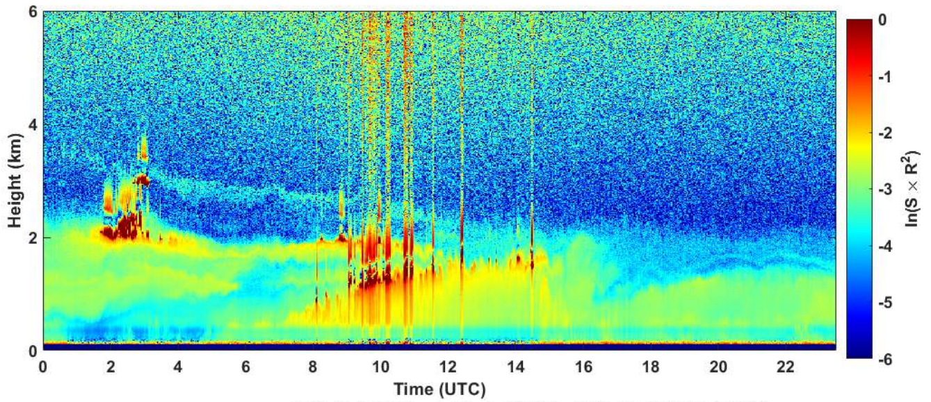
2019-10-12 RCS quick look CHM15k - ILVA LIDAR1 DIREZIONE
