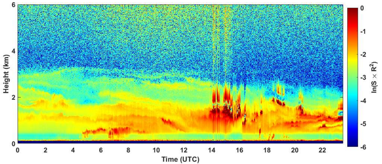
2019-10-18 RCS quick look CHM15k - ILVA LIDAR1 DIREZIONE
