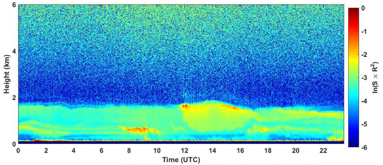
2019-10-14 RCS quick look CHM15k - ILVA LIDAR1 DIREZIONE
