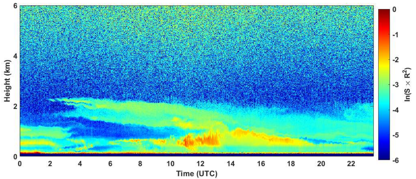
2019-10-22 RCS quick look CHM15k - ILVA LIDAR1 DIREZIONE
