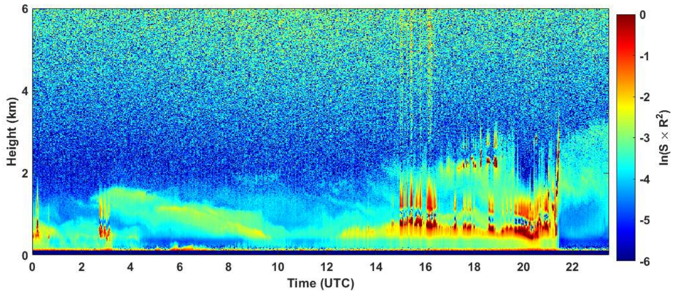
2019-10-02 RCS quick look CHM15k - ILVA LIDAR1 DIREZIONE
