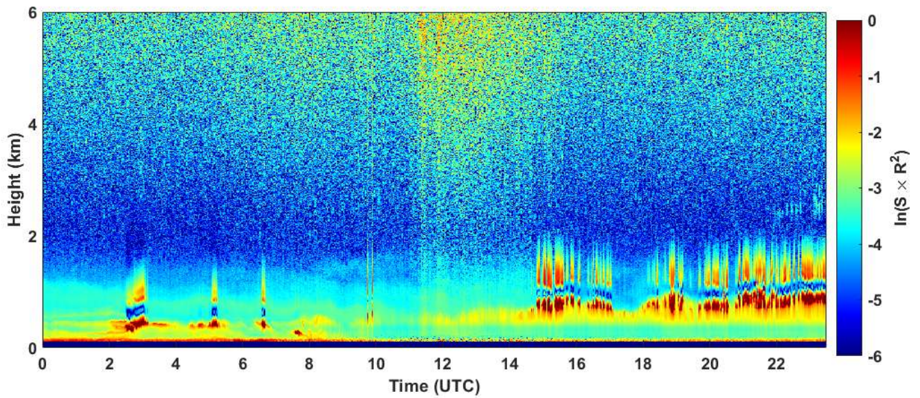
2019-10-24 RCS quick look CHM15k - ILVA LIDAR1 DIREZIONE
