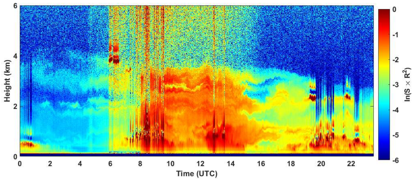
2019-10-10 RCS quick look CHM15k - ILVA LIDAR2 PARCHI
