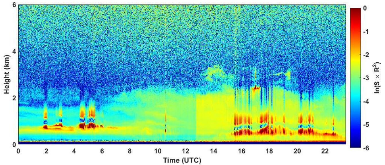
2019-10-16 RCS quick look CHM15k - ILVA LIDAR1 DIREZIONE
