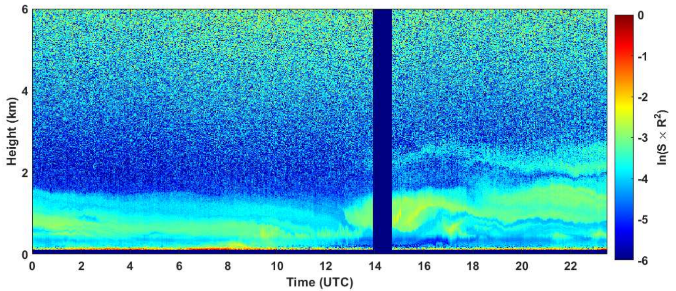
2019-10-28 RCS quick look CHM15k - ILVA LIDAR1 DIREZIONE
