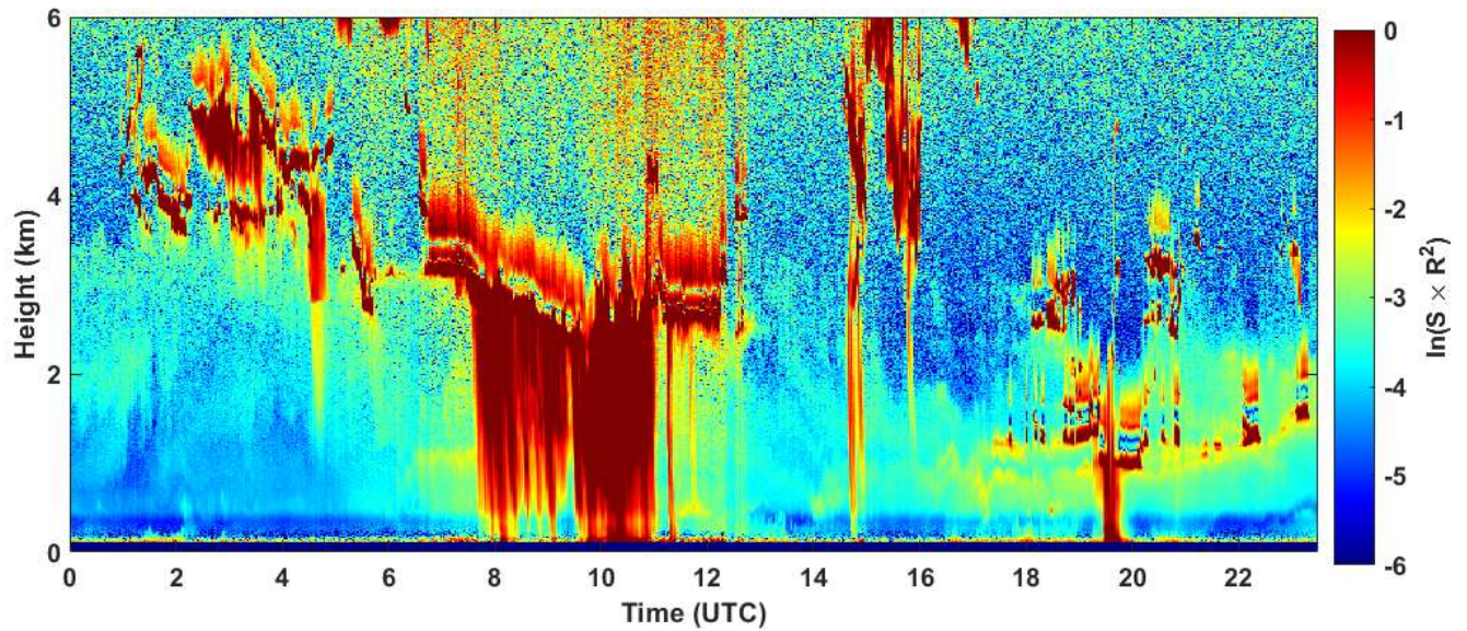
2019-10-04 RCS quick look CHM15k - ILVA LIDAR1 DIREZIONE
