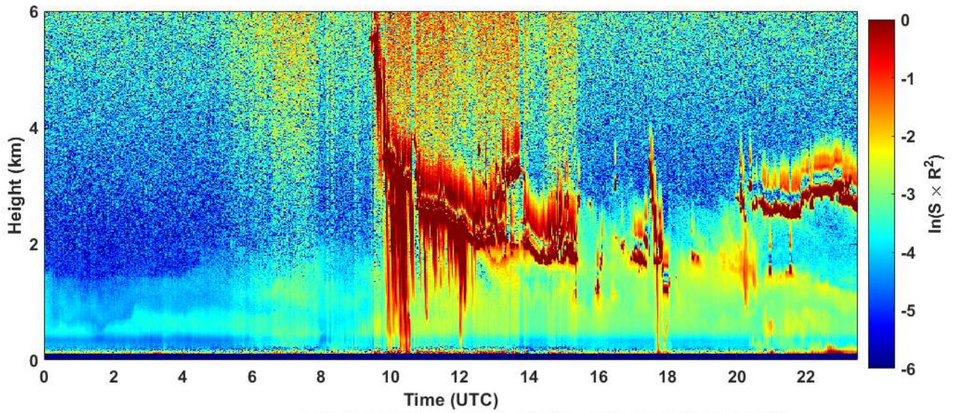
2019-10-06 RCS quick look CHM15k - ILVA LIDAR1 DIREZIONE
