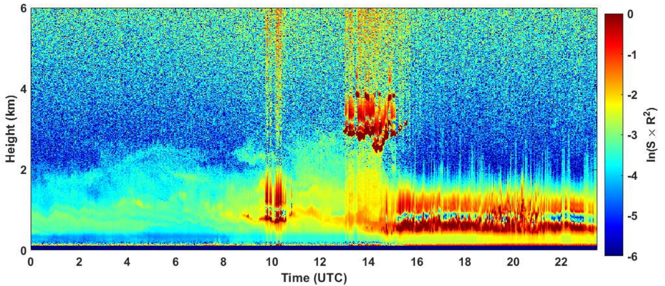
2019-10-10 RCS quick look CHM15k - ILVA LIDAR1 DIREZIONE
