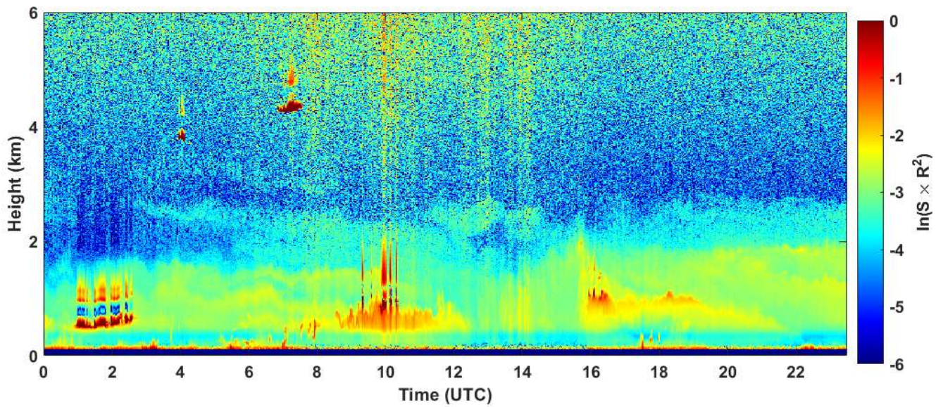
2019-10-30 RCS quick look CHM15k - ILVA LIDAR1 DIREZIONE
