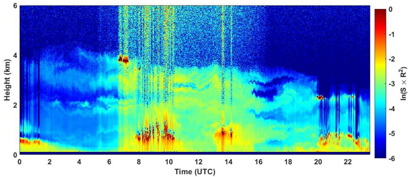
2019-10-10 RCS quick look CHM15k - ILVA LIDAR3 AGGLOMERATO
