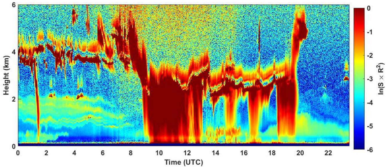
2019-10-08 RCS quick look CHM15k - ILVA LIDAR1 DIREZIONE
