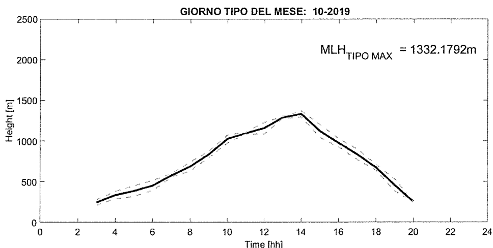
Fig. 2: Giorno tipo del parametro Mixing Layer Height nel mese di OTTOBRE 2019, rappresentato mediante media oraria (linea blu continua) e deviazione standard (linee celesti tratteggiate).
