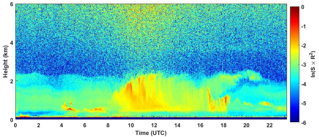
2019-07-20 RCS quick look CHM15k - ILVA LIDAR1 DIREZIONE
