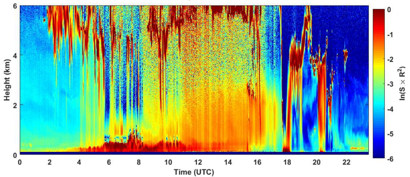
2019-07-10 RCS quick look CHM15k - ILVA LIDAR3 AGGLOMERATO
