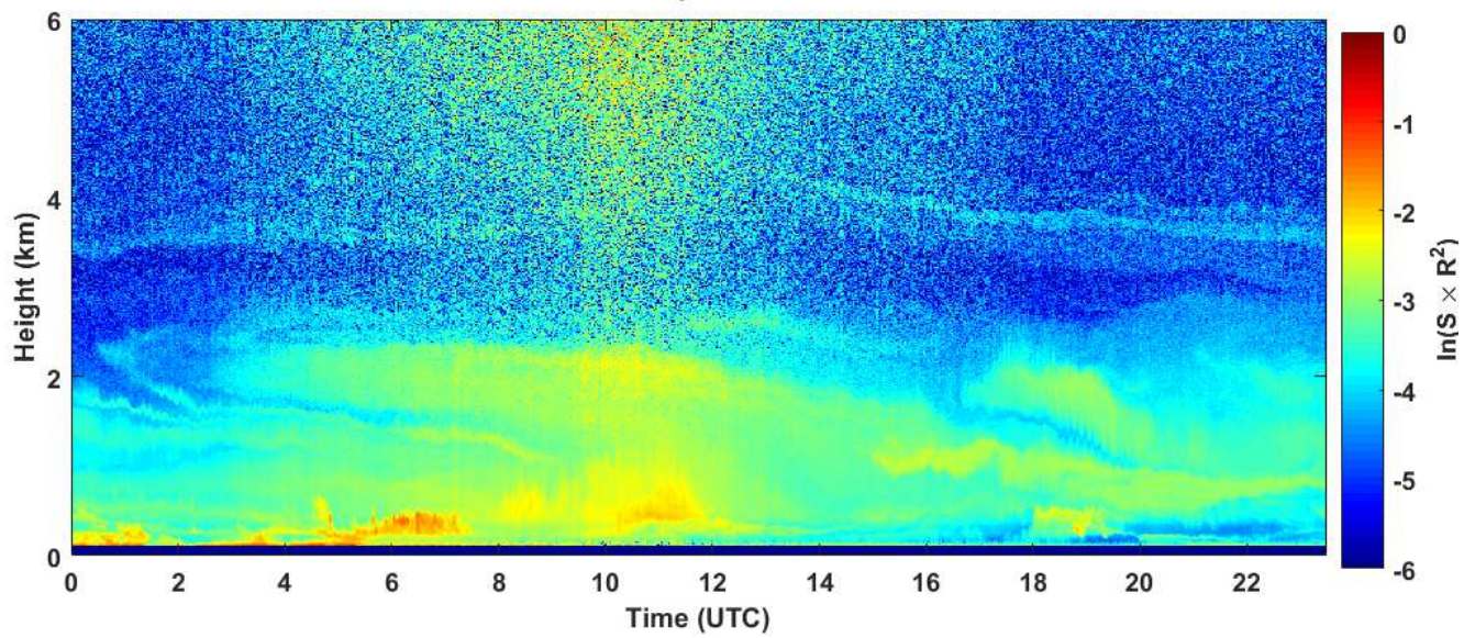
2019-07-20 RCS quick look CHM15k - ILVA LIDAR2 PARCHI
