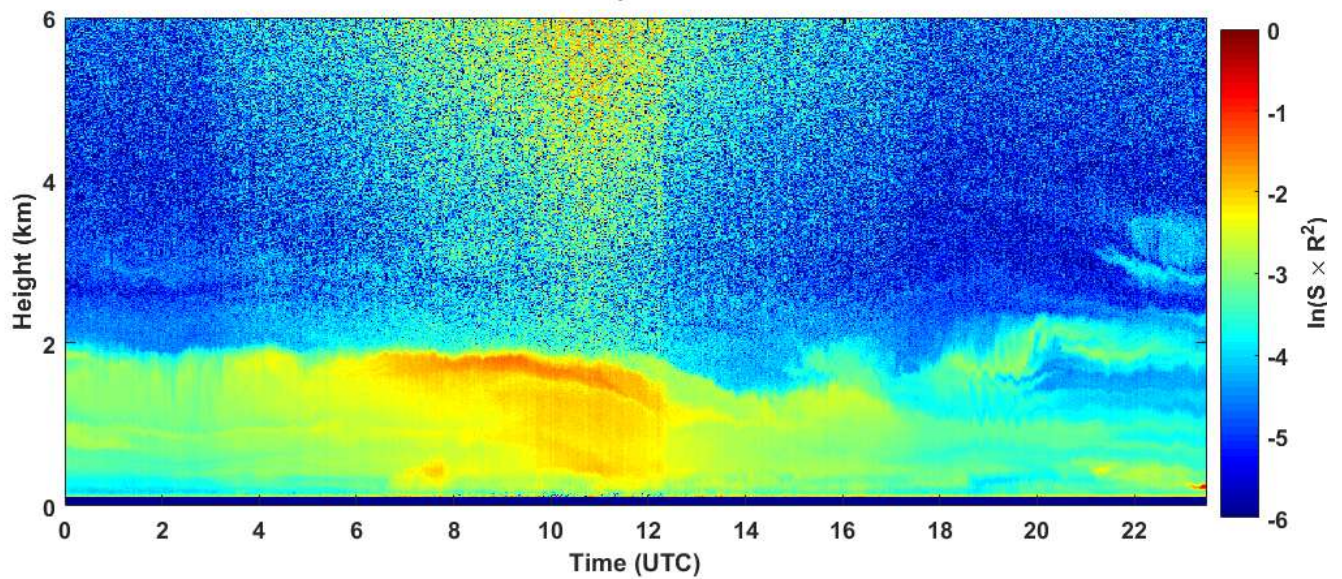
2019-07-26 RCS quick look CHM15k - ILVA LIDAR2 PARCHI
