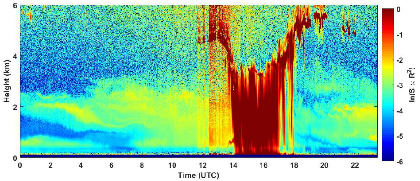
2019-07-12 RCS quick look CHM15k - ILVA LIDAR1 DIREZIONE
