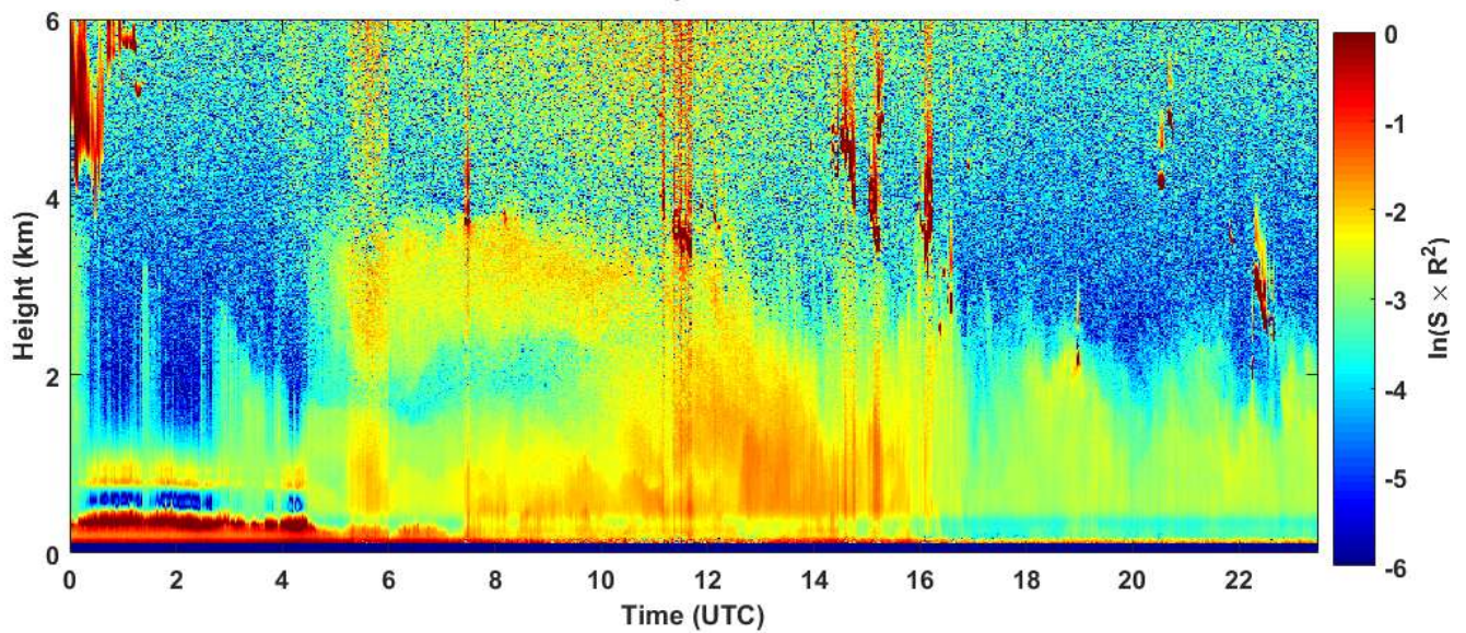
2019-07-28 RCS quick look CHM15k - ILVA LIDAR1 DIREZIONE
