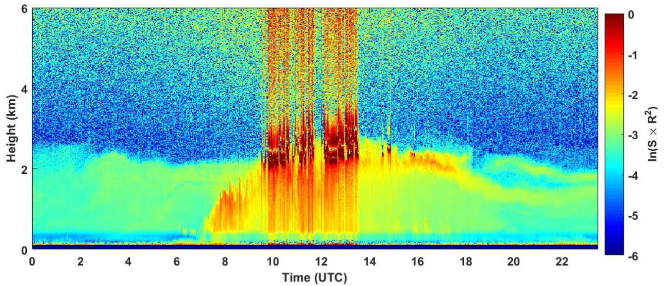
2019-07-26 RCS quick look CHM15k - ILVA LIDAR1 DIREZIONE
