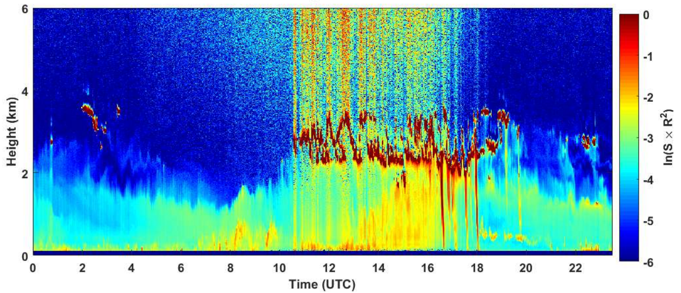
2019-07-30 RCS quick look CHM15k - ILVA LIDAR3 AGGLOMERATO
