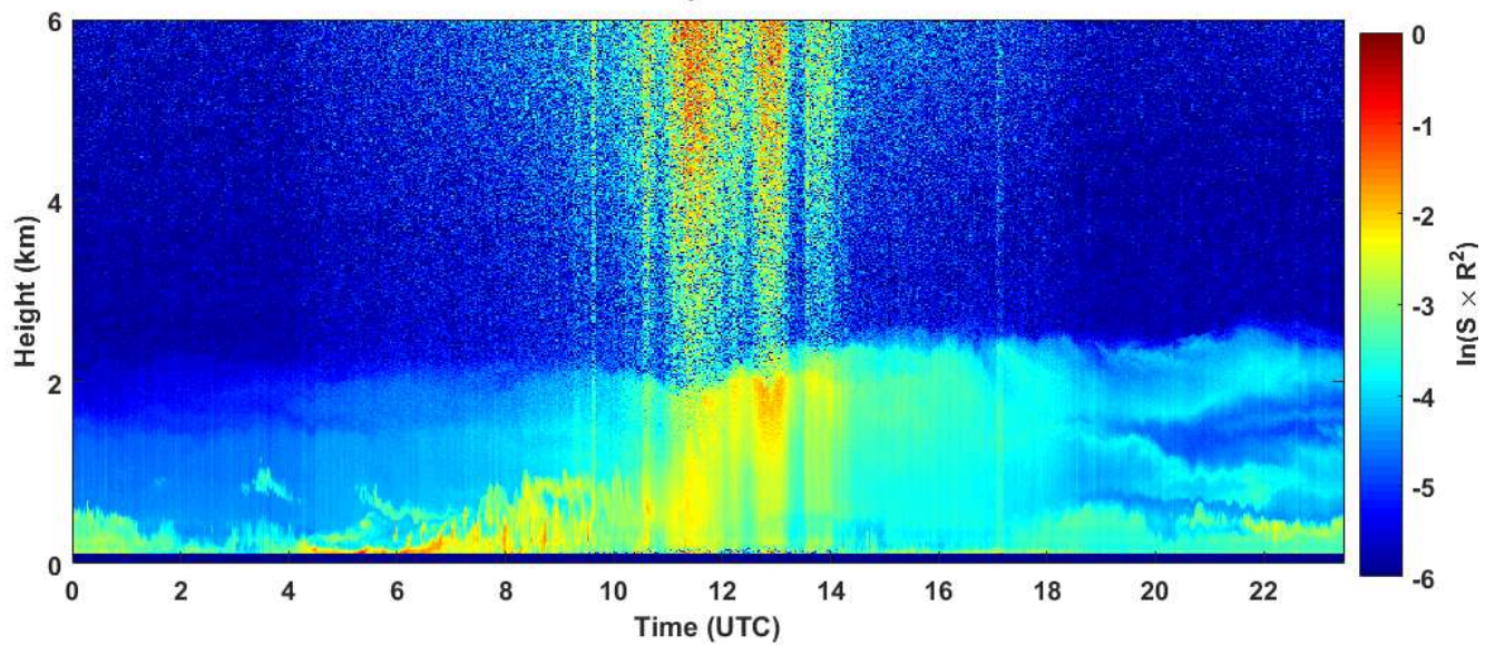
2019-07-18 RCS quick look CHM15k - ILVA LIDAR3 AGGLOMERATO
