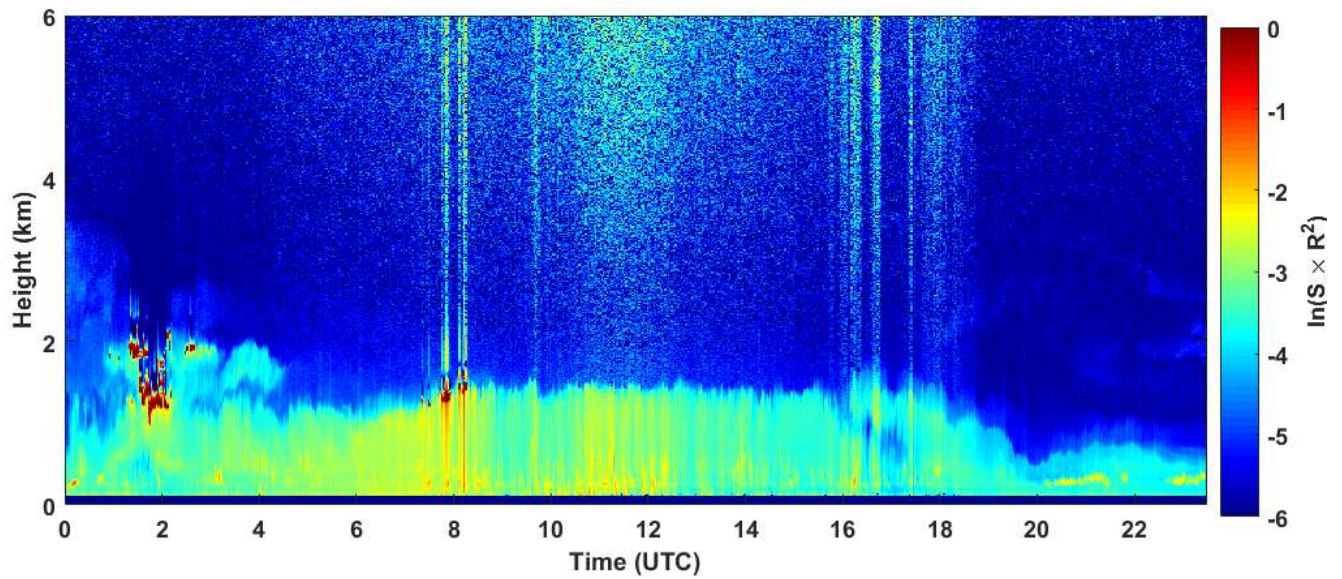
2019-07-12 RCS quick look CHM15k - ILVA LIDAR3 AGGLOMERATO
