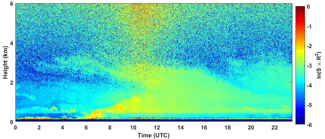
2019-07-02 RCS quick look CHM15k - ILVA LIDAR1 DIREZIONE
