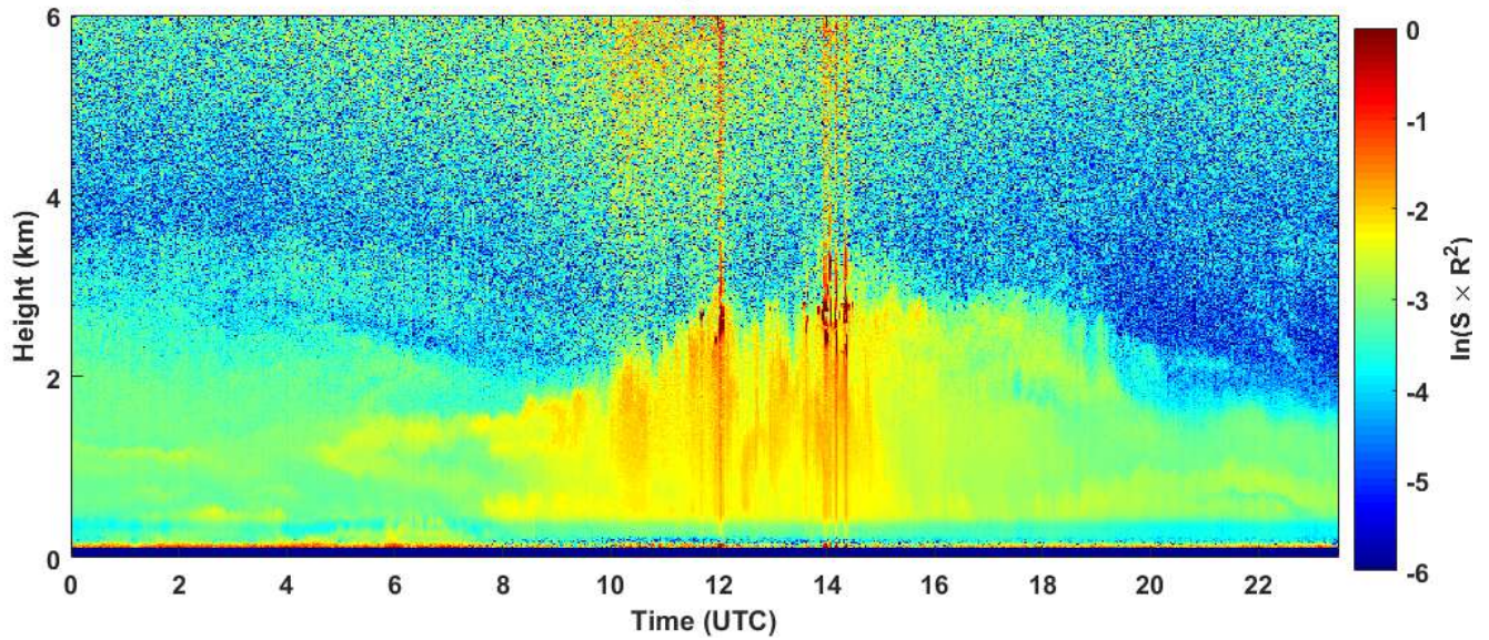
2019-07-06 RCS quick look CHM15k - ILVA LIDAR1 DIREZIONE
