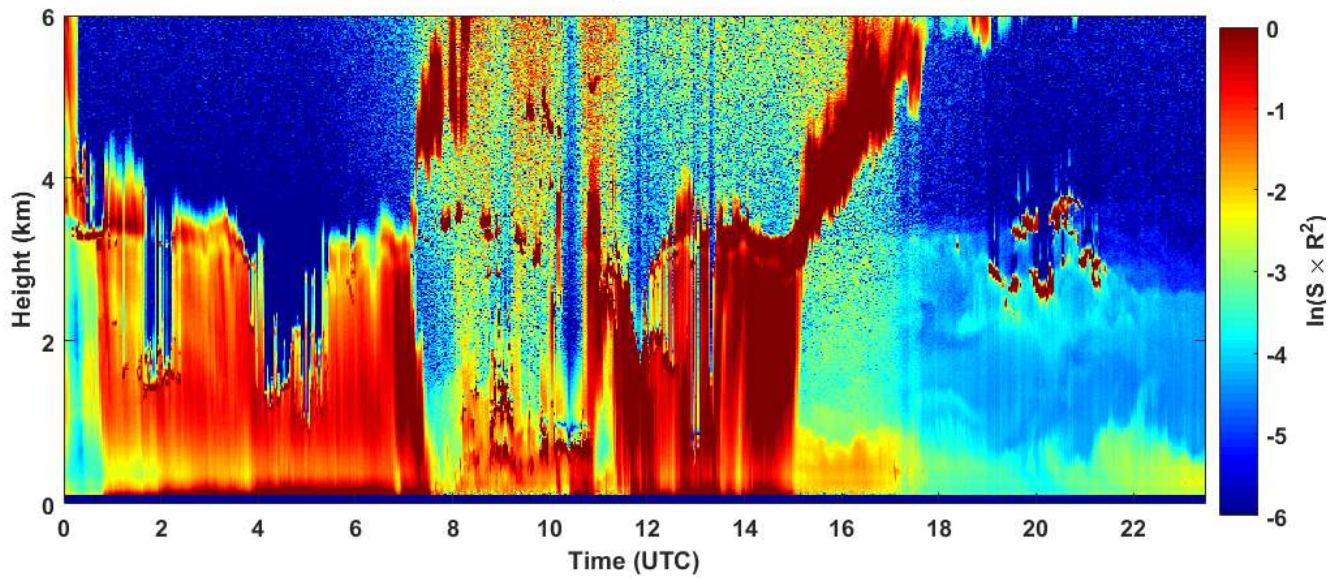
2019-07-16 RCS quick look CHM15k - ILVA LIDAR3 AGGLOMERATO
