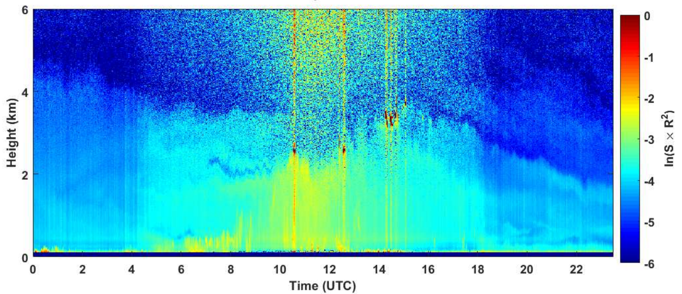
2019-07-08 RCS quick look CHM15k - ILVA LIDAR3 AGGLOMERATO
