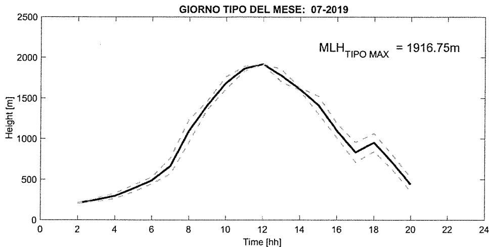
Fig. 2: Giorno tipo del parametro Mixing Layer Height nel mese di LUGLIO 2019, rappresentato mediante media oraria (linea blu continua) e deviazione standard (linee celesti tratteggiate).
