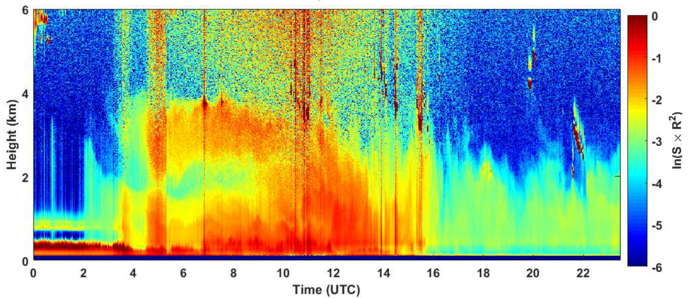
2019-07-28 RCS quick look CHM15k - ILVA LIDAR2 PARCHI
