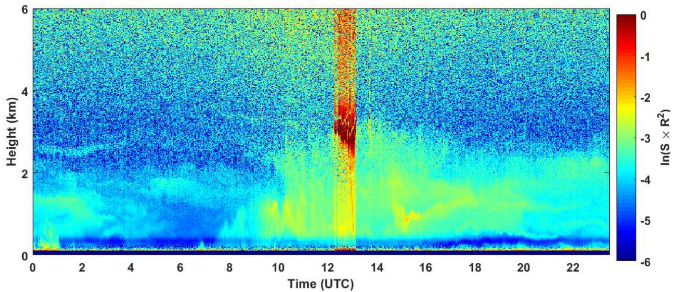
2019-05-02 RCS quick look CHM15k - ILVA LIDAR1 DIREZIONE
