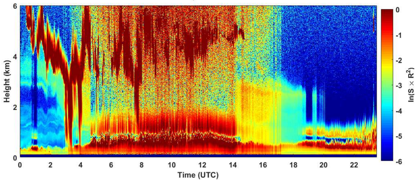
2019-05-18 RCS quick look CHM15k - ILVA LIDAR2 PARCHI
