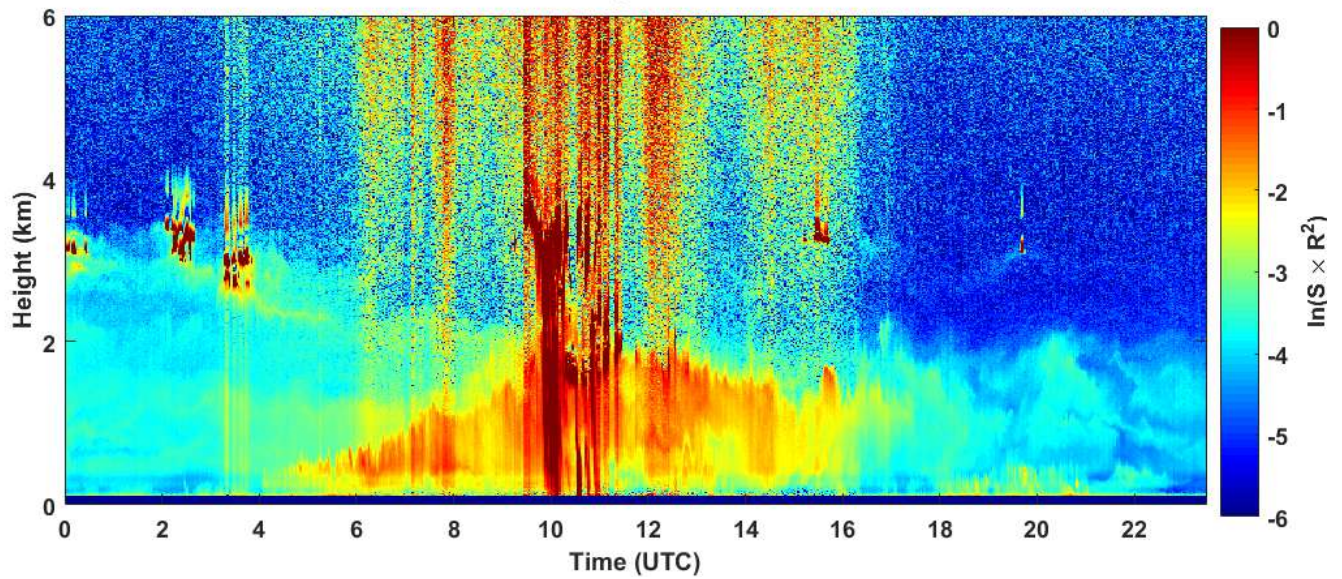
2019-05-24 RCS quick look CHM15k - ILVA LIDAR2 PARCHI
