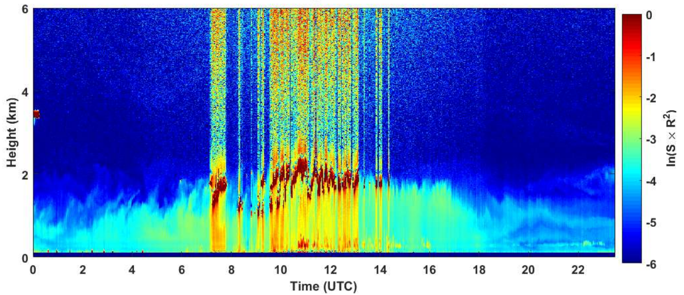
2019-05-08 RCS quick look CHM15k - ILVA LIDAR3 AGGLOMERATO
