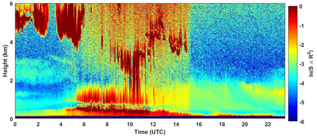
2019-05-10 RCS quick look CHM15k - ILVA LIDAR1 DIREZIONE
