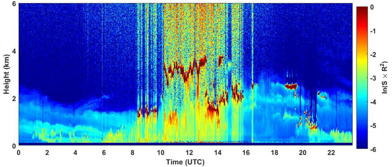
2019-05-02 RCS quick look CHM15k - ILVA LIDAR3 AGGLOMERATO
