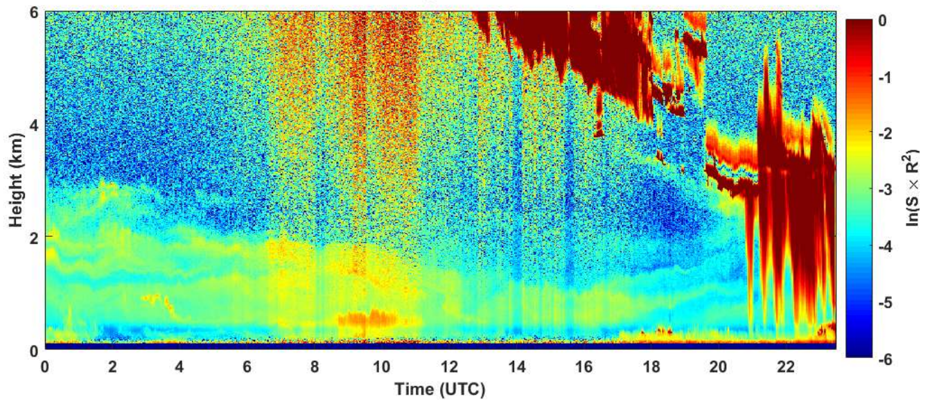
2019-05-26 RCS quick look CHM15k - ILVA LIDAR1 DIREZIONE
