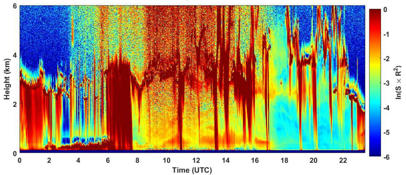
2019-05-26 RCS quick look CHM15k - ILVA LIDAR2 PARCHI
