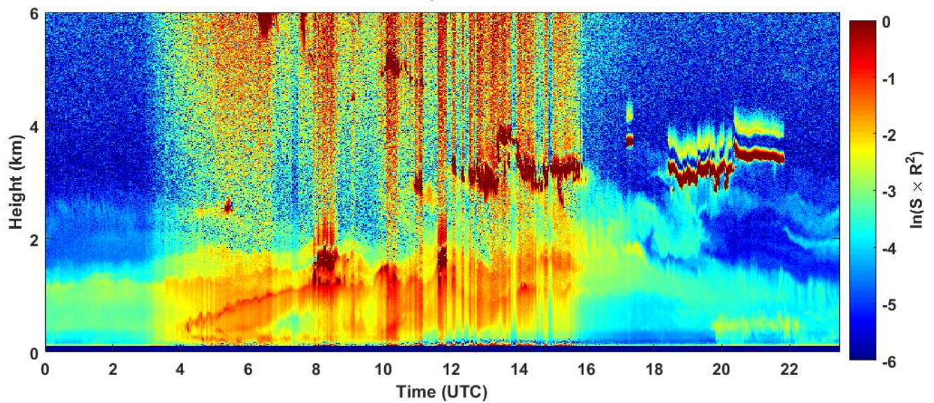
2019-05-10 RCS quick look CHM15k - ILVA LIDAR2 PARCHI
