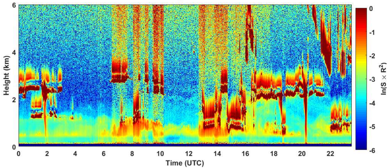
2019-05-16 RCS quick look CHM15k - ILVA LIDAR1 DIREZIONE
