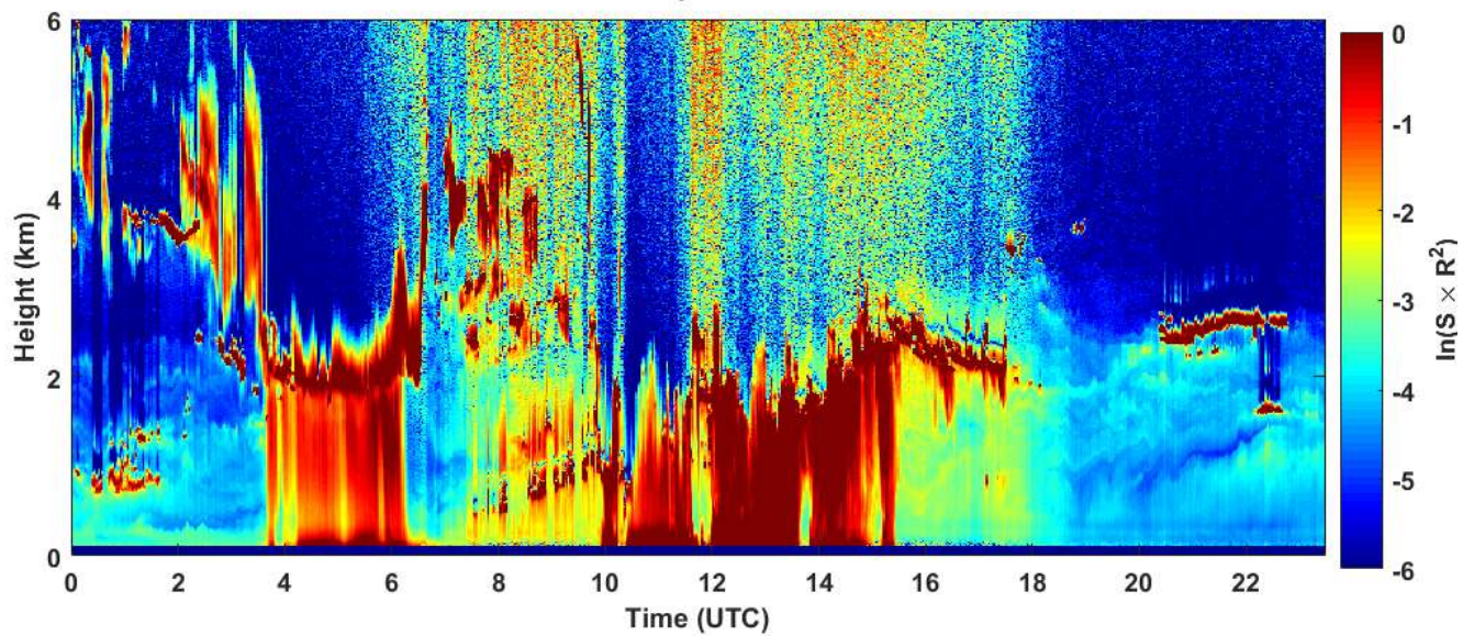
2019-05-16 RCS quick look CHM15k - ILVA LIDAR3 AGGLOMERATO
