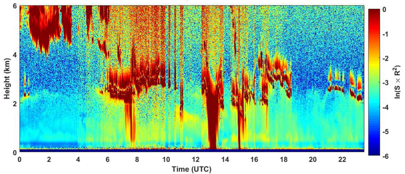
2019-05-20 RCS quick look CHM15k - ILVA LIDAR1 DIREZIONE
