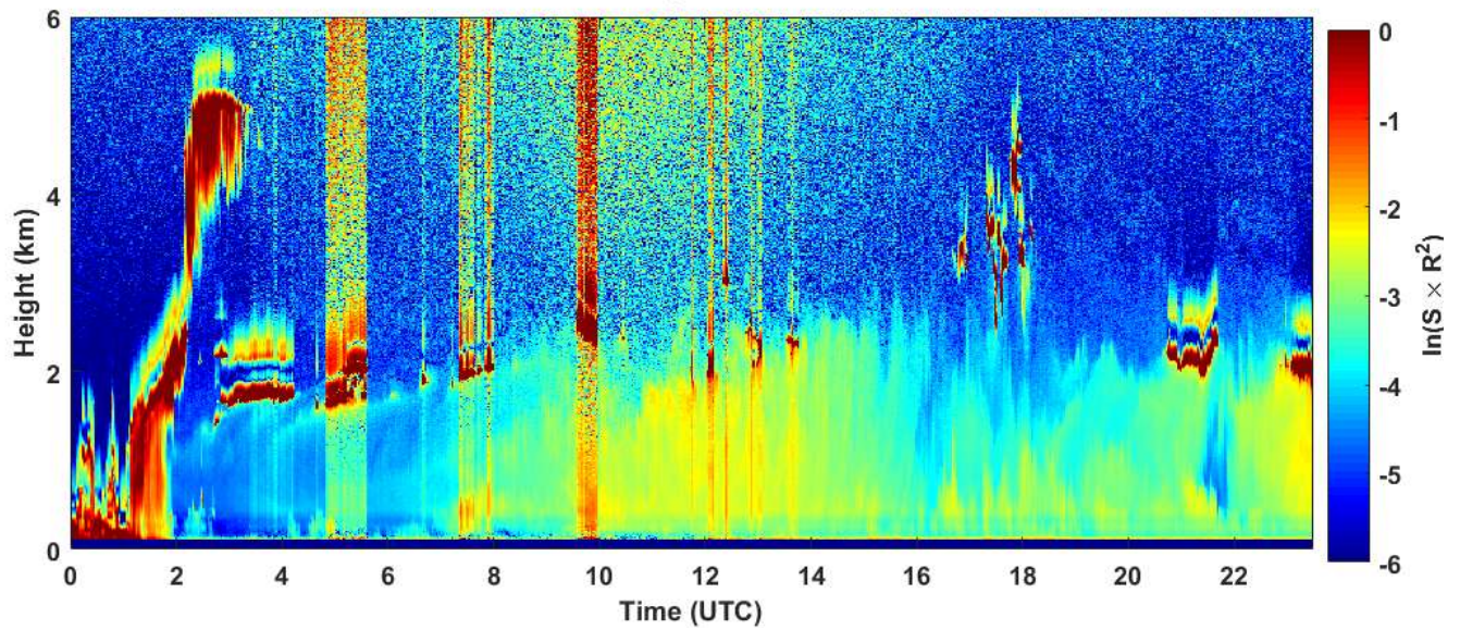
2019-05-06 RCS quick look CHM15k - ILVA LIDAR2 PARCHI
