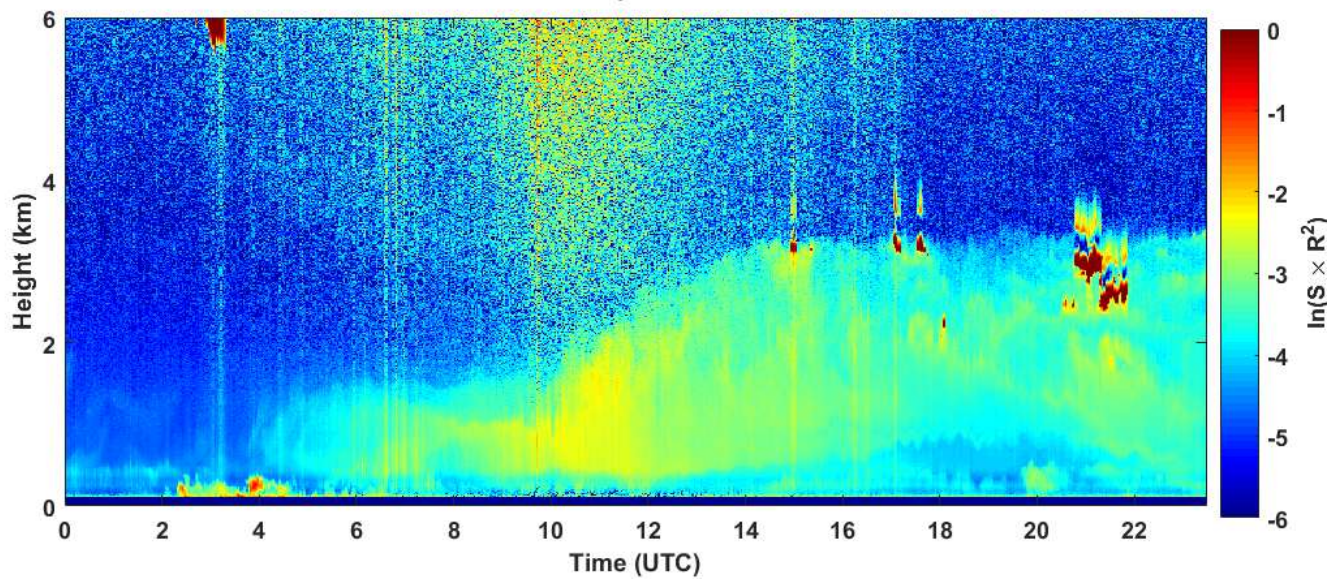
2019-05-22 RCS quick look CHM15k - ILVA LIDAR2 PARCHI
