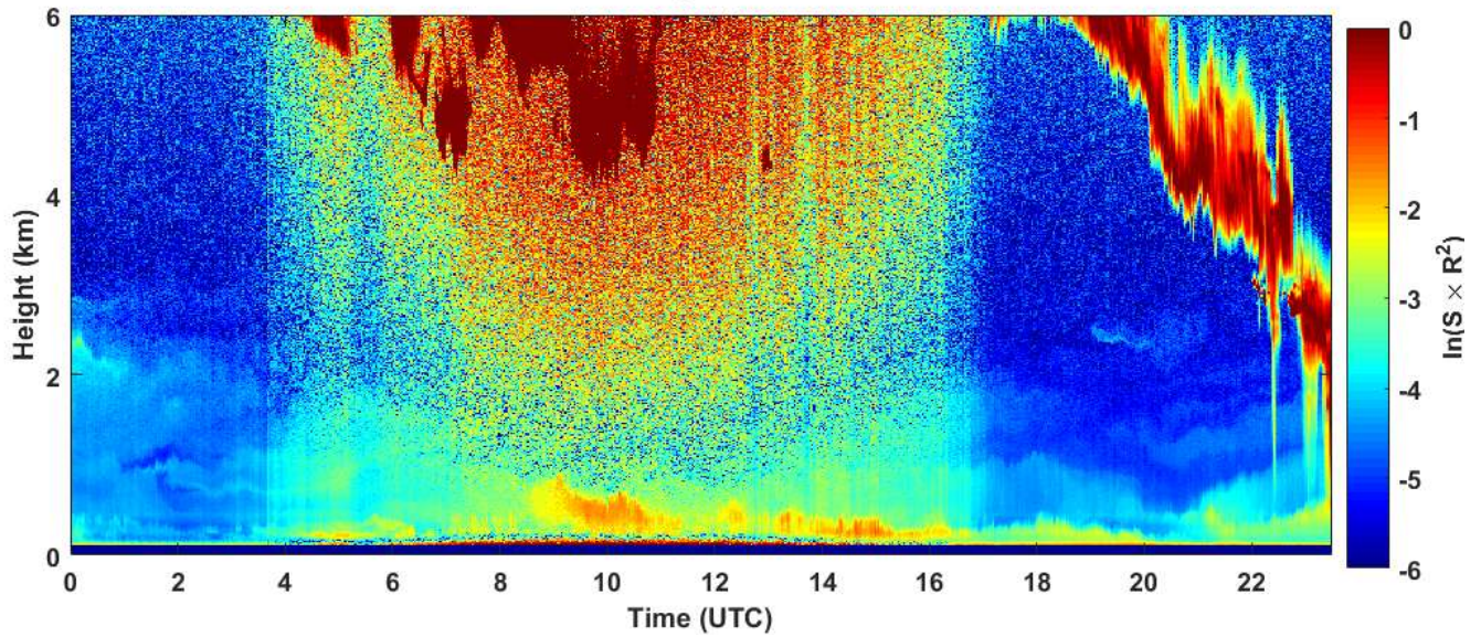
2019-05-04 RCS quick look CHM15k - ILVA LIDAR2 PARCHI
