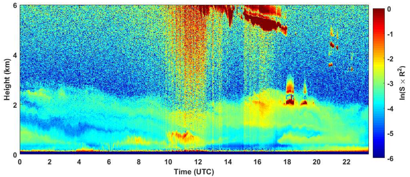
2019-05-12 RCS quick look CHM15k - ILVA LIDAR1 DIREZIONE
