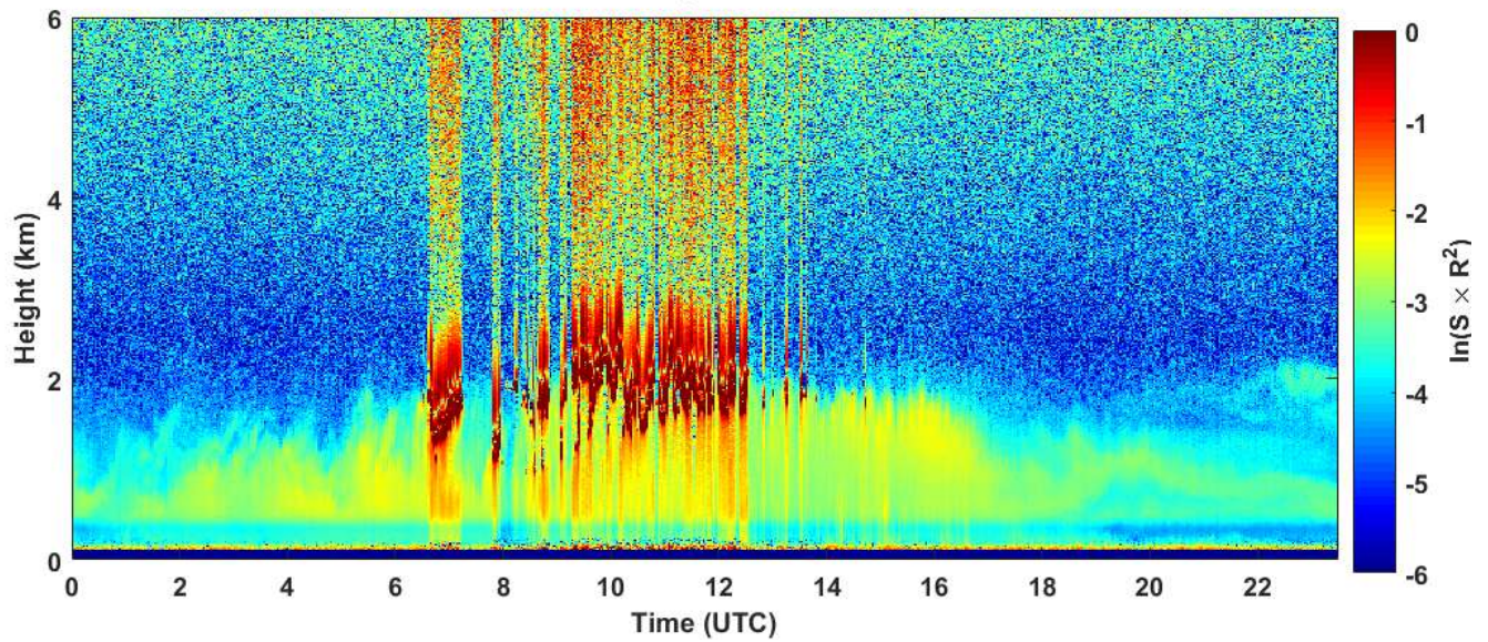
2019-05-08 RCS quick look CHM15k - ILVA LIDAR1 DIREZIONE
