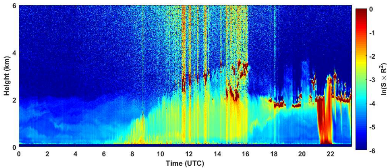
2019-05-24 RCS quick look CHM15k - ILVA LIDAR3 AGGLOMERATO
