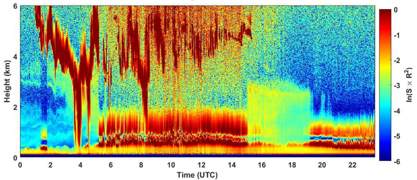
2019-05-18 RCS quick look CHM15k - ILVA LIDAR1 DIREZIONE
