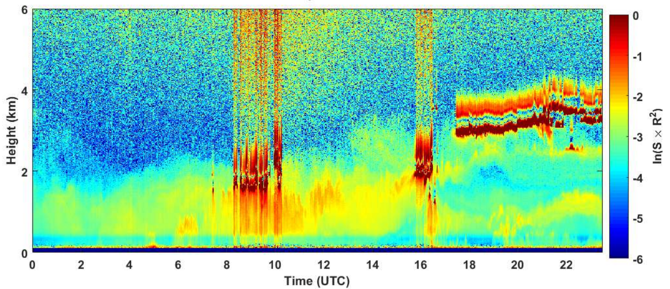
2019-05-30 RCS quick look CHM15k - ILVA LIDAR1 DIREZIONE
