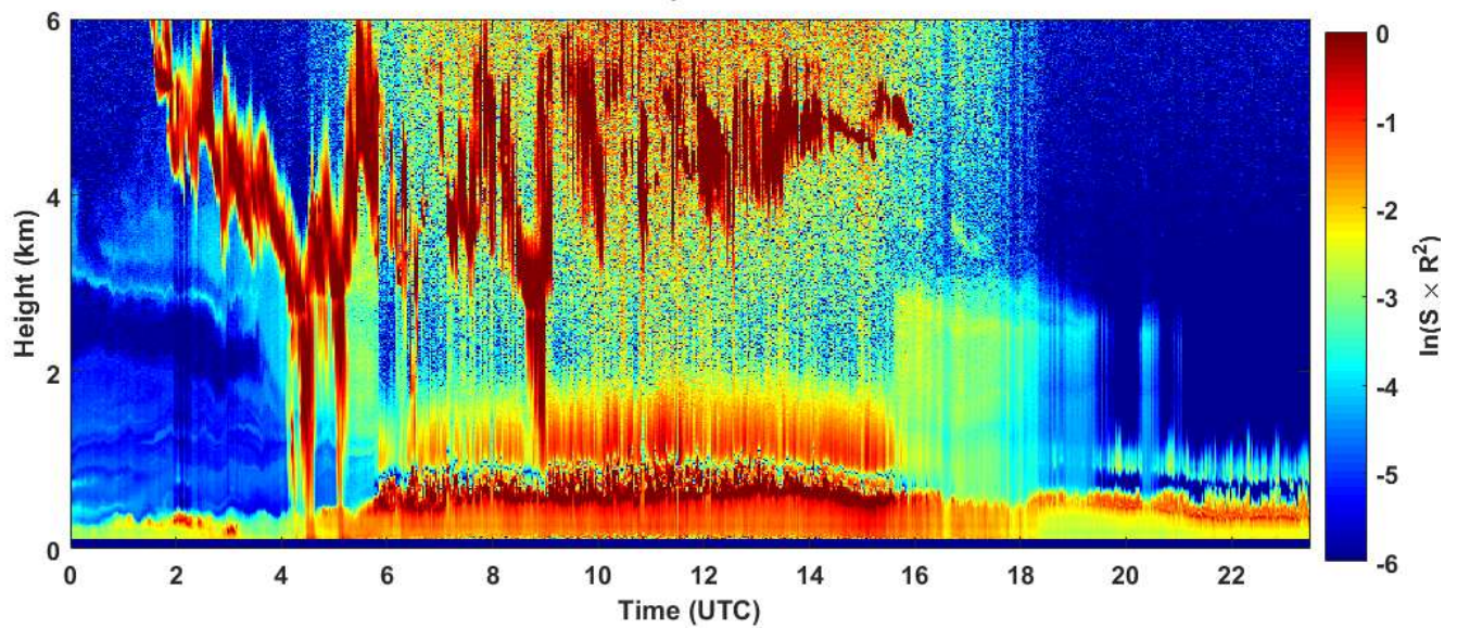
2019-05-18 RCS quick look CHM15k - ILVA LIDAR3 AGGLOMERATO
