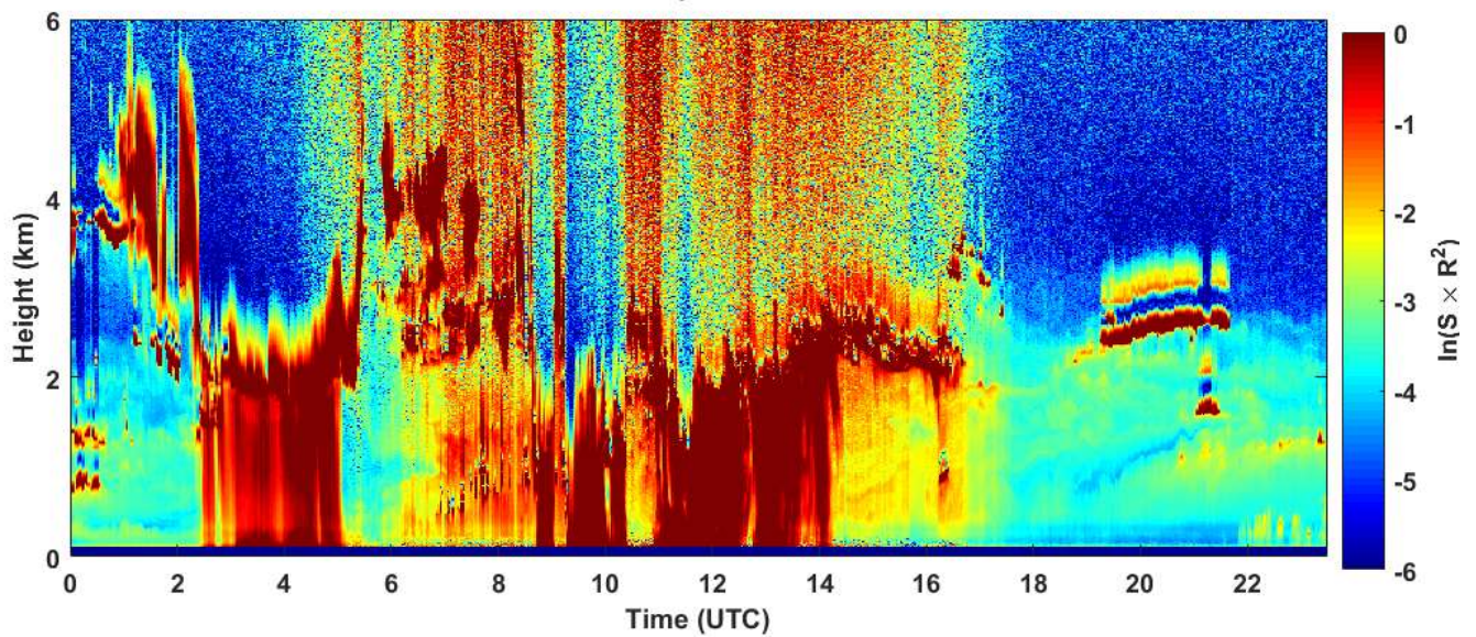
2019-05-16 RCS quick look CHM15k - ILVA LIDAR2 PARCHI
