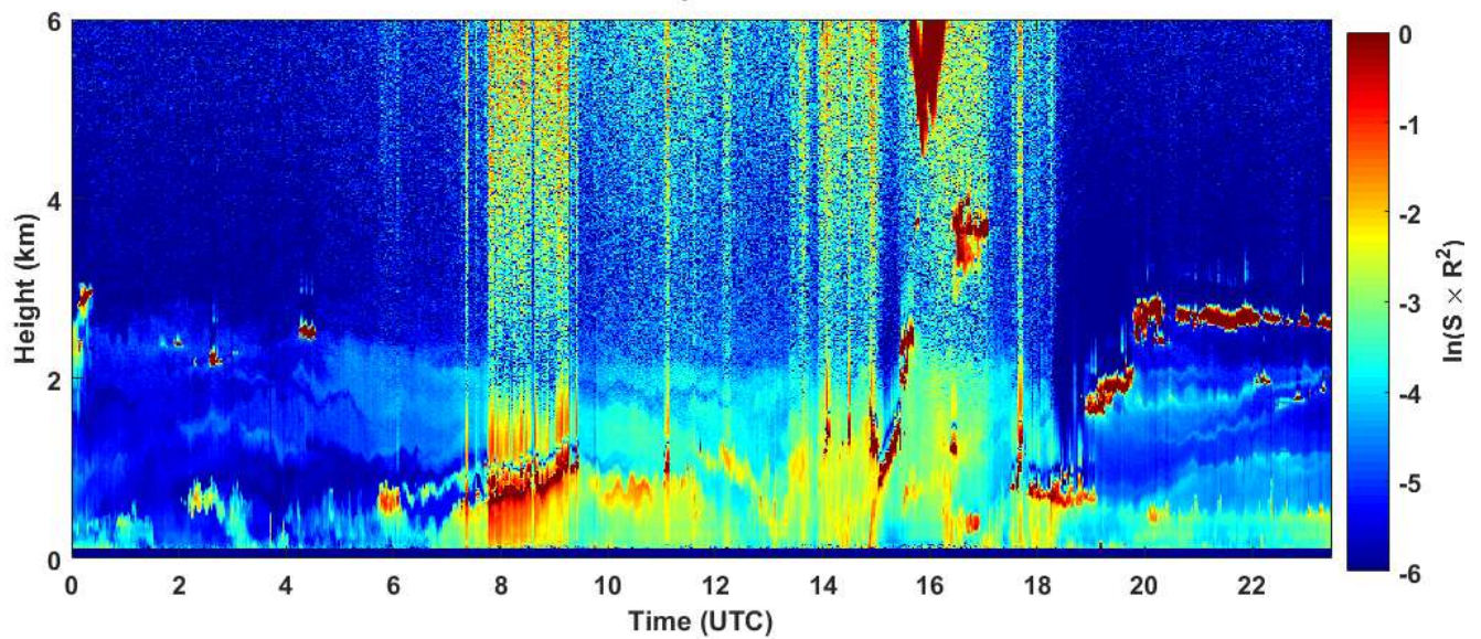
2019-05-14 RCS quick look CHM15k - ILVA LIDAR3 AGGLOMERATO
