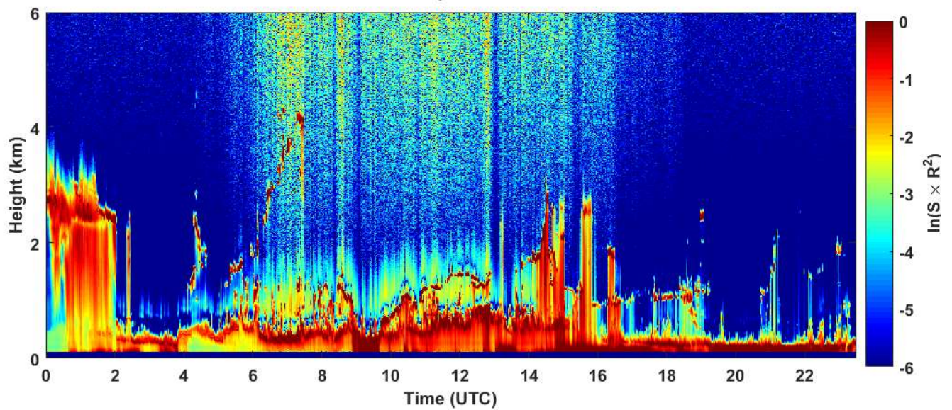
2019-05-04 RCS quick look CHM15k - ILVA LIDAR3 AGGLOMERATO
