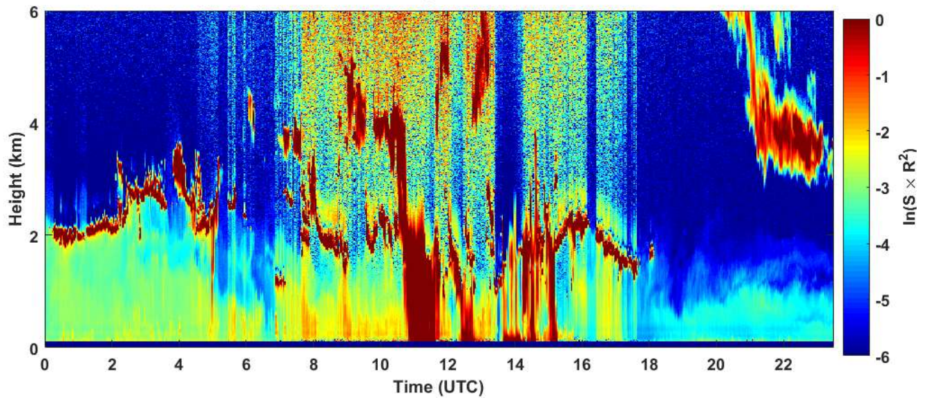
2019-05-06 RCS quick look CHM15k - ILVA LIDAR3 AGGLOMERATO
