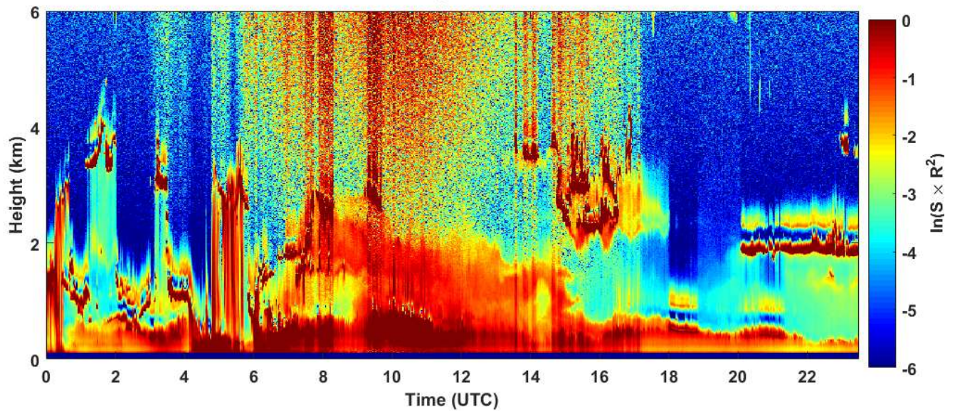
2019-05-28 RCS quick look CHM15k - ILVA LIDAR2 PARCHI
