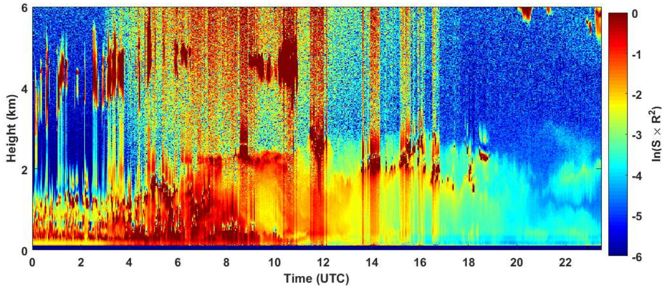
2019-05-20 RCS quick look CHM15k - ILVA LIDAR2 PARCHI
