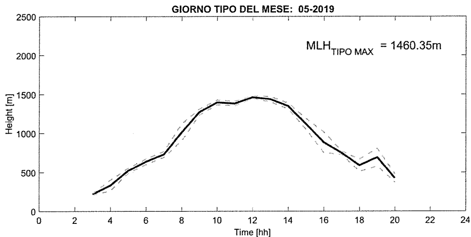
Fig. 2: Giorno tipo del parametro Mixing Layer Height nel mese di MAGGIO 2019, rappresentato mediante media oraria (linea blu continua) e deviazione standard (linee celesti tratteggiate).
