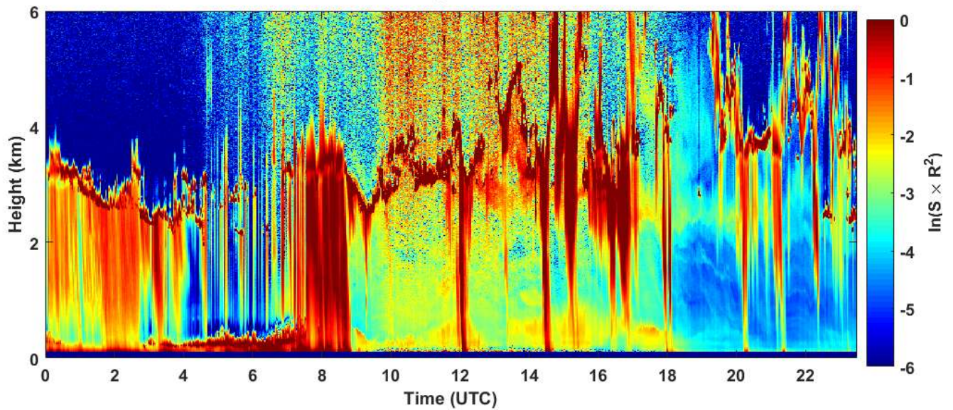
2019-05-26 RCS quick look CHM15k - ILVA LIDAR3 AGGLOMERATO
