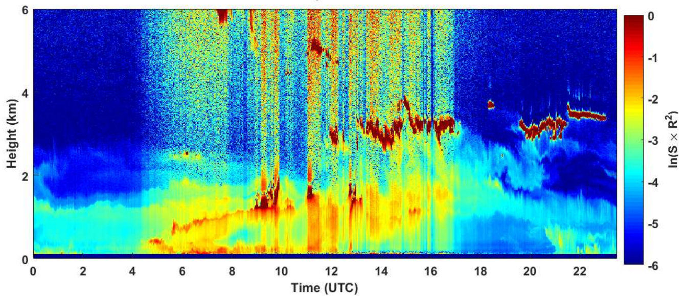
2019-05-10 RCS quick look CHM15k - ILVA LIDAR3 AGGLOMERATO
