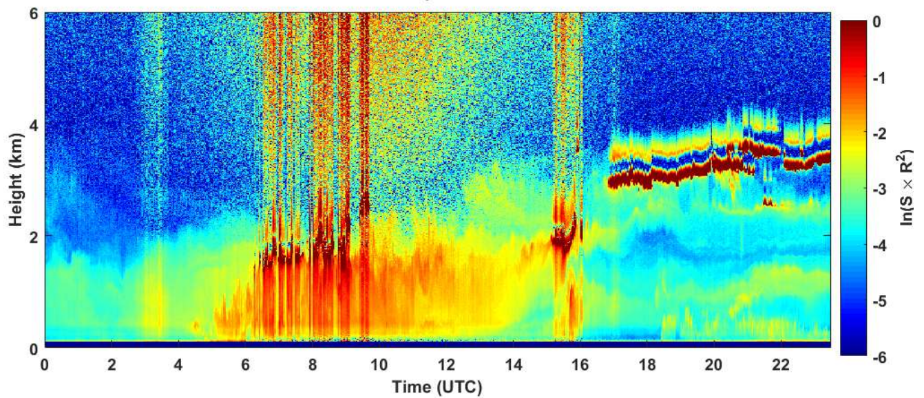
2019-05-30 RCS quick look CHM15k - ILVA LIDAR2 PARCHI
