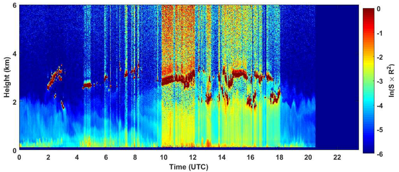
2019-05-22 RCS quick look CHM15k - ILVA LIDAR3 AGGLOMERATO
