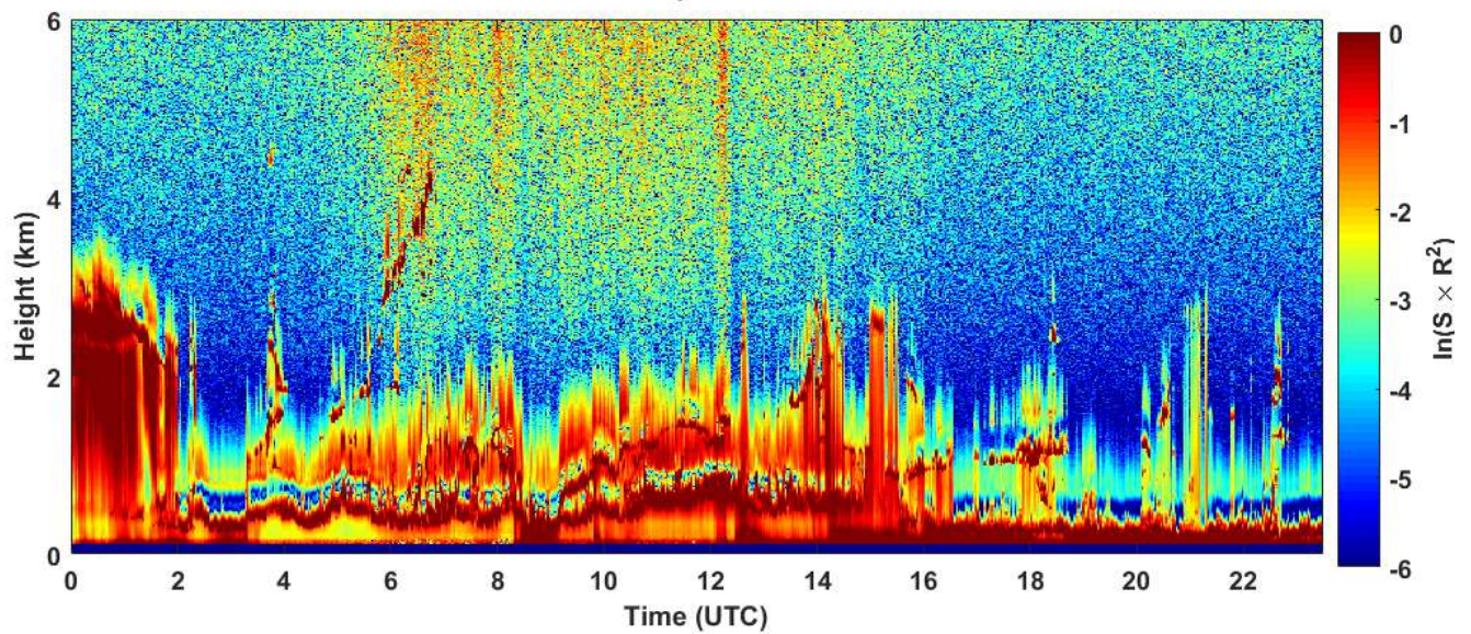
2019-05-04 RCS quick look CHM15k - ILVA LIDAR1 DIREZIONE
