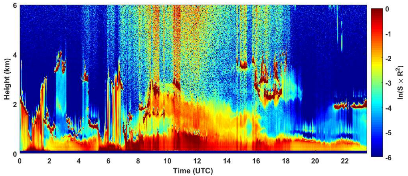
2019-05-28 RCS quick look CHM15k - ILVA LIDAR3 AGGLOMERATO
