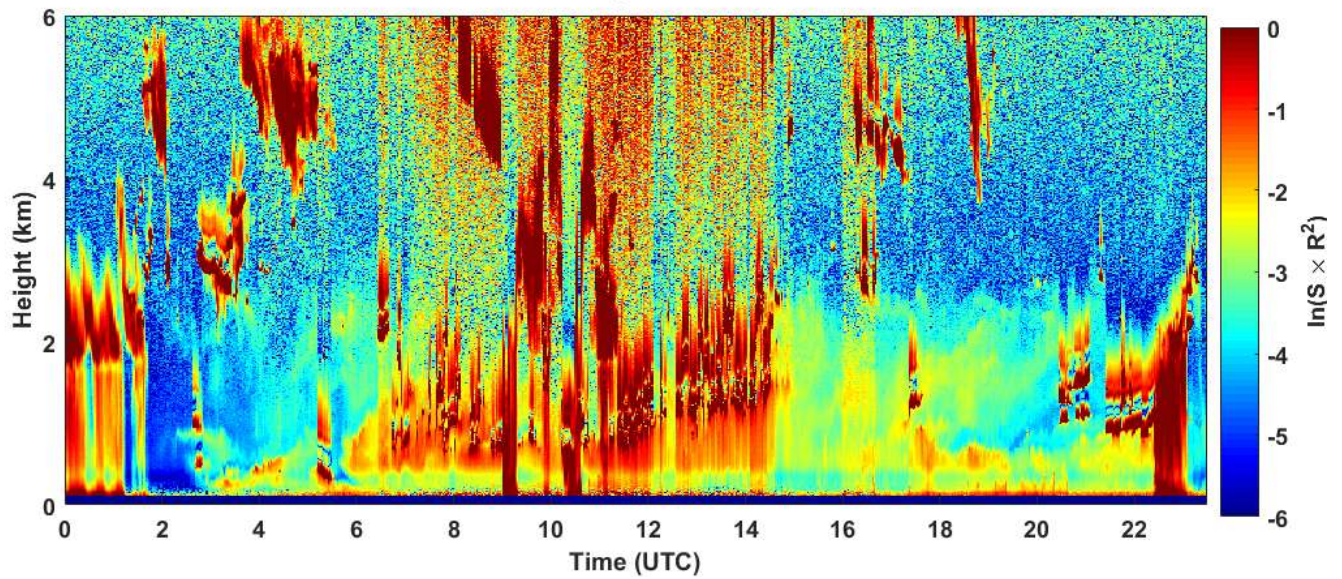
2019-05-14 RCS quick look CHM15k - ILVA LIDAR1 DIREZIONE
