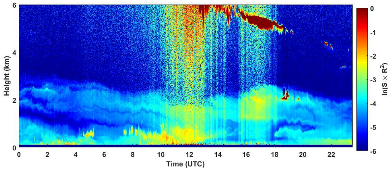
2019-05-12 RCS quick look CHM15k - ILVA LIDAR3 AGGLOMERATO
