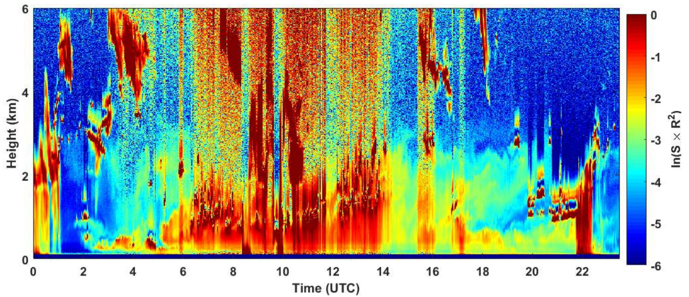
2019-05-14 RCS quick look CHM15k - ILVA LIDAR2 PARCHI
