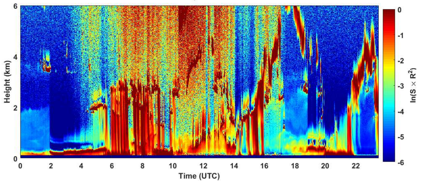
2019-05-12 RCS quick look CHM15k - ILVA LIDAR2 PARCHI
