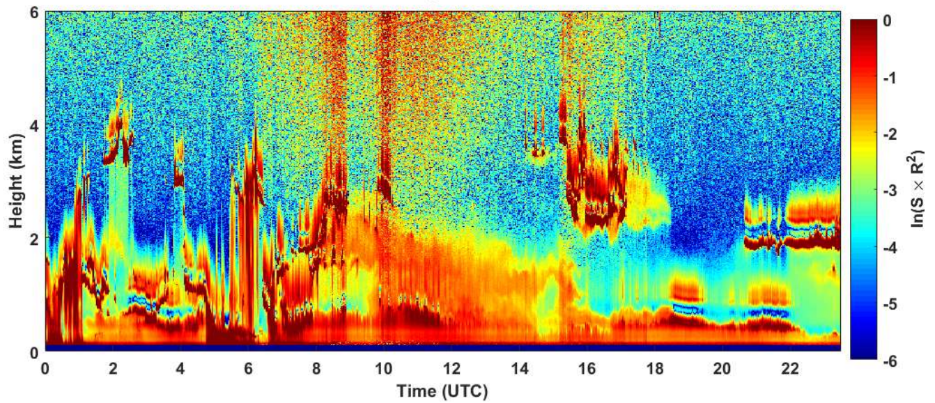
2019-05-28 RCS quick look CHM15k - ILVA LIDAR1 DIREZIONE
