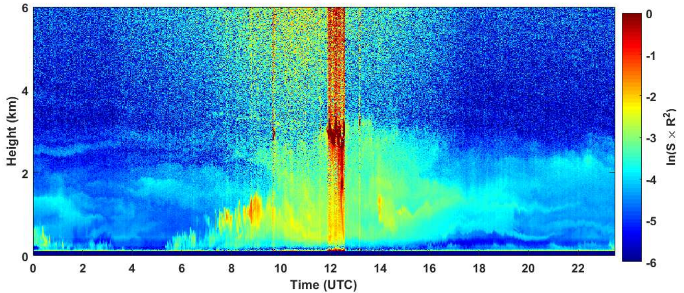
2019-05-02 RCS quick look CHM15k - ILVA LIDAR2 PARCHI
