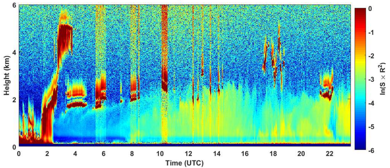
2019-05-06 RCS quick look CHM15k - ILVA LIDAR1 DIREZIONE
