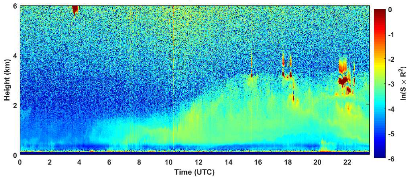
2019-05-22 RCS quick look CHM15k - ILVA LIDAR1 DIREZIONE
