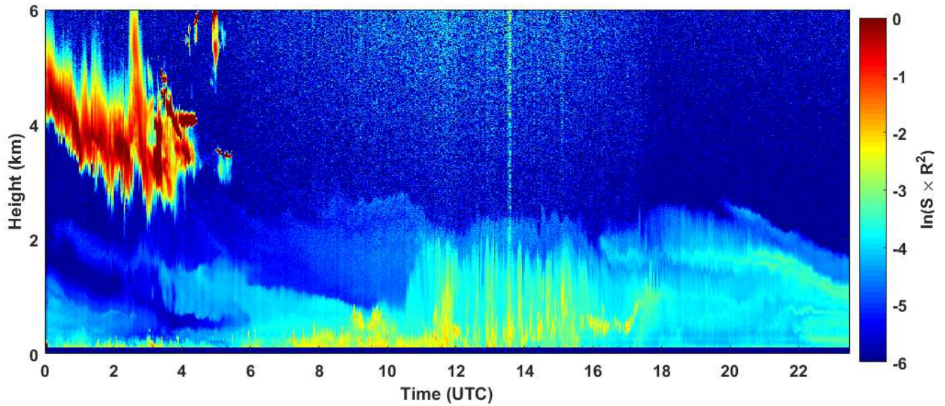
2019-03-16 RCS quick look CHM15k - ILVA LIDAR3 AGGLOMERATO
