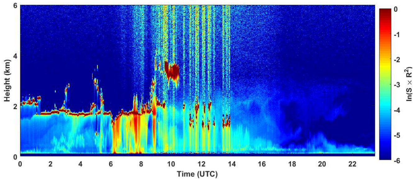
2019-03-02 RCS quick look CHM15k - ILVA LIDAR3 AGGLOMERATO
