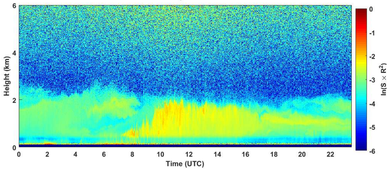
2019-03-24 RCS quick look CHM15k - ILVA LIDAR1 DIREZIONE
