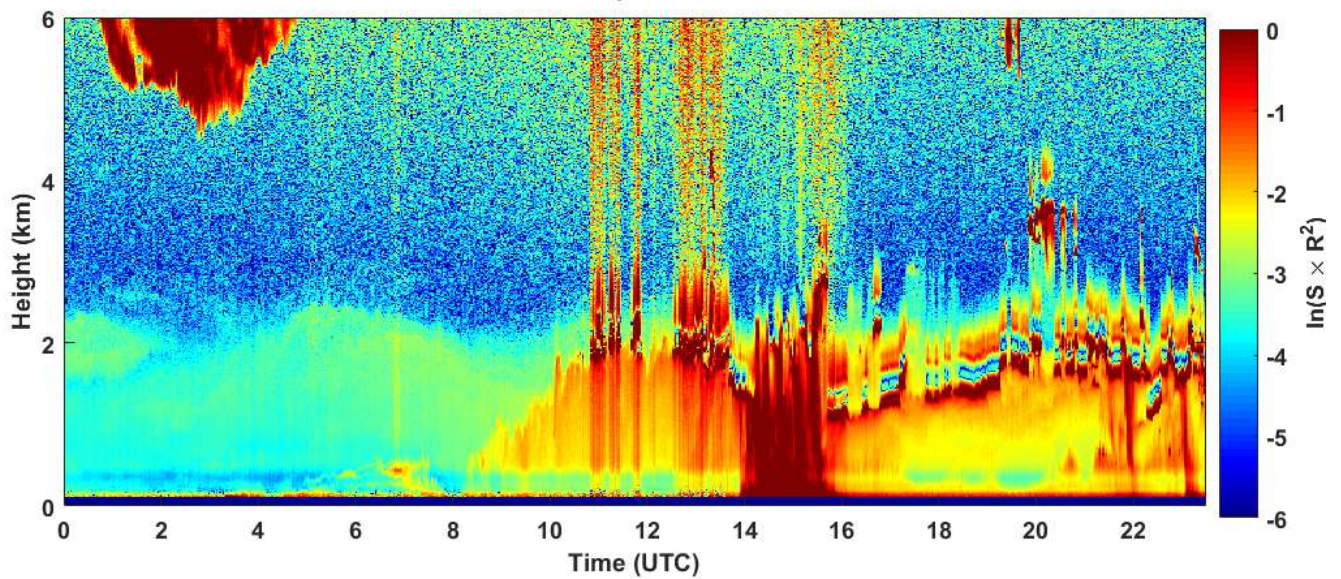
2019-03-26 RCS quick look CHM15k - ILVA LIDAR1 DIREZIONE
