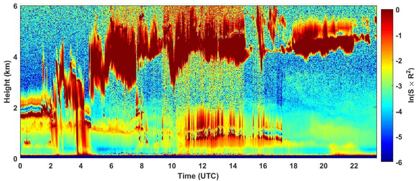
2019-03-20 RCS quick look CHM15k - ILVA LIDAR1 DIREZIONE
