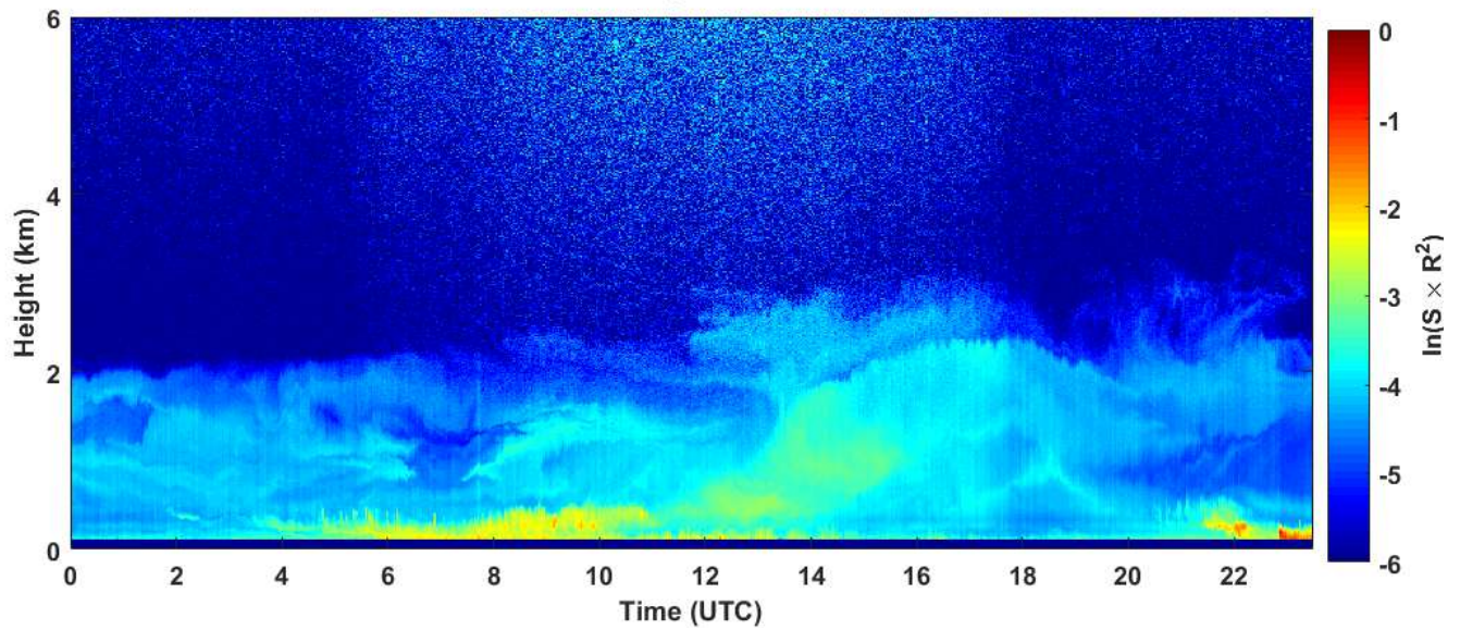
2019-03-26 RCS quick look CHM15k - ILVA LIDAR3 AGGLOMERATO
