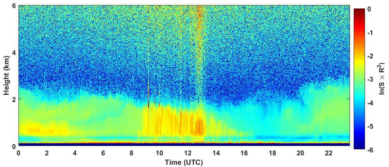
2019-03-30 RCS quick look CHM15k - ILVA LIDAR1 DIREZIONE
