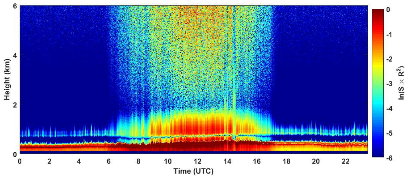
2019-03-08 RCS quick look CHM15k - ILVA LIDAR3 AGGLOMERATO
