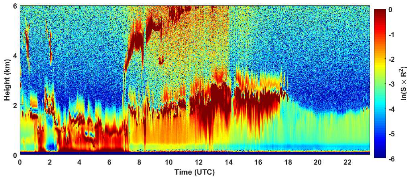
2019-03-12 RCS quick look CHM15k - ILVA LIDAR1 DIREZIONE
