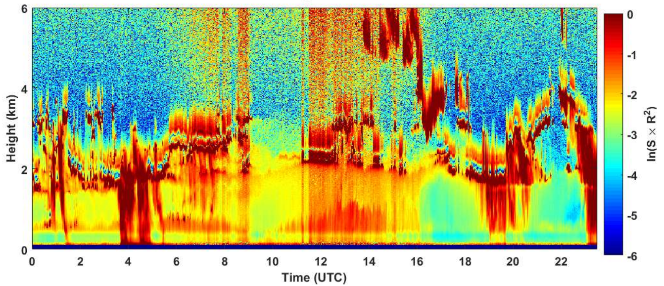
2019-03-28 RCS quick look CHM15k - ILVA LIDAR1 DIREZIONE
