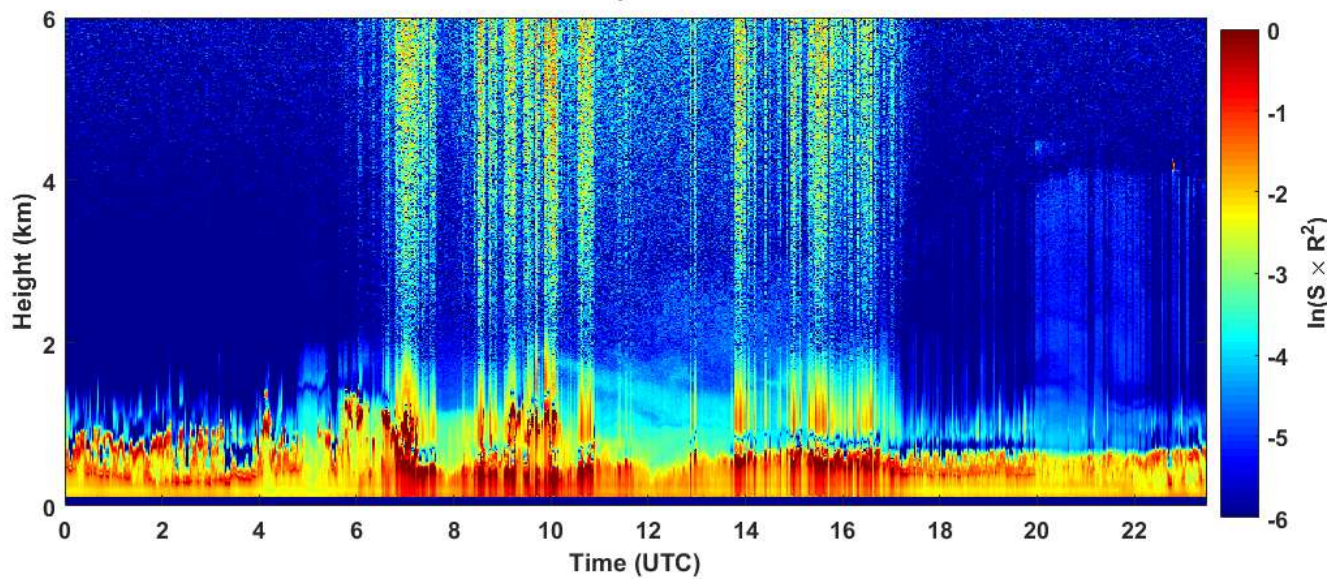
2019-03-18 RCS quick look CHM15k - ILVA LIDAR3 AGGLOMERATO
