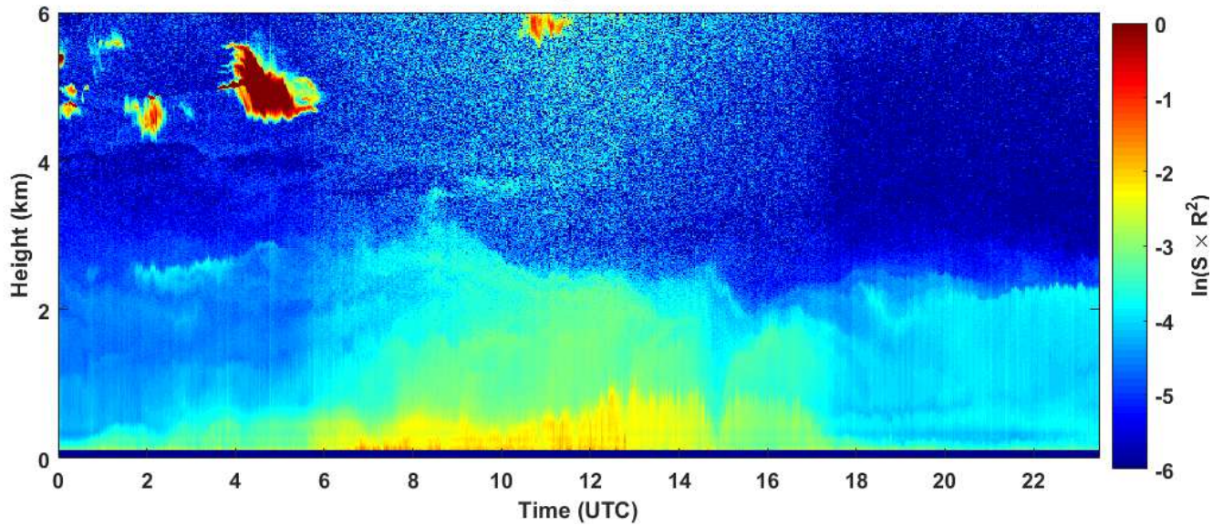
2019-03-22 RCS quick look CHM15k - ILVA LIDAR3 AGGLOMERATO
