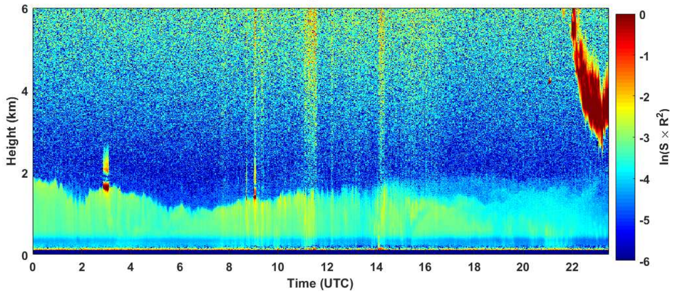
2019-03-14 RCS quick look CHM15k - ILVA LIDAR1 DIREZIONE
