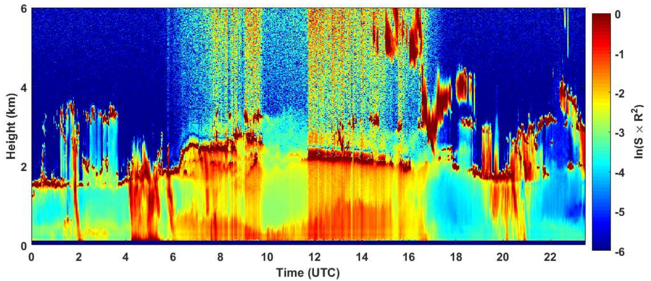
2019-03-28 RCS quick look CHM15k - ILVA LIDAR3 AGGLOMERATO
