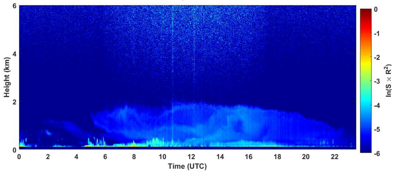
2019-03-04 RCS quick look CHM15k - ILVA LIDAR3 AGGLOMERATO
