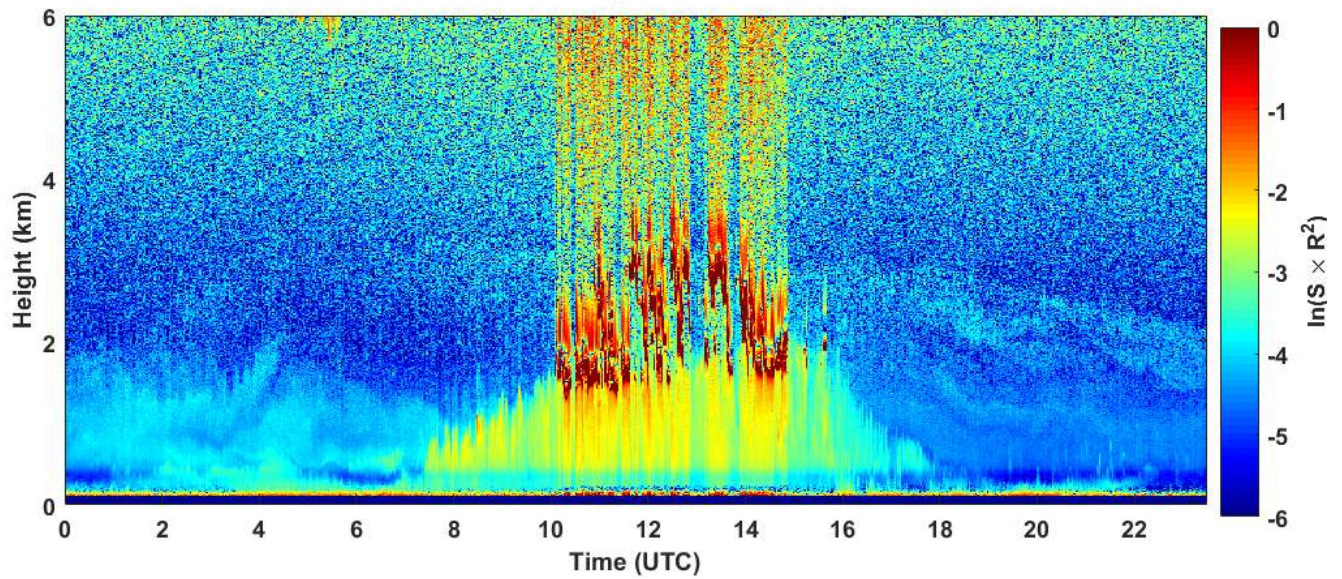
2019-03-04 RCS quick look CHM15k - ILVA LIDAR1 DIREZIONE
