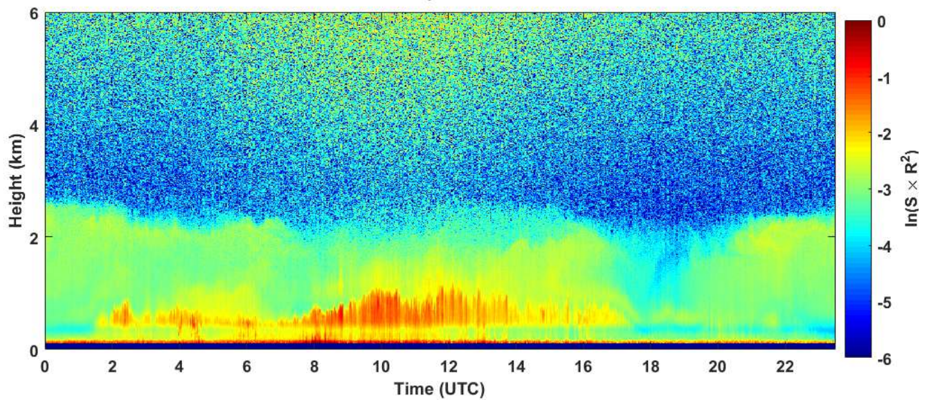
2019-03-22 RCS quick look CHM15k - ILVA LIDAR1 DIREZIONE
