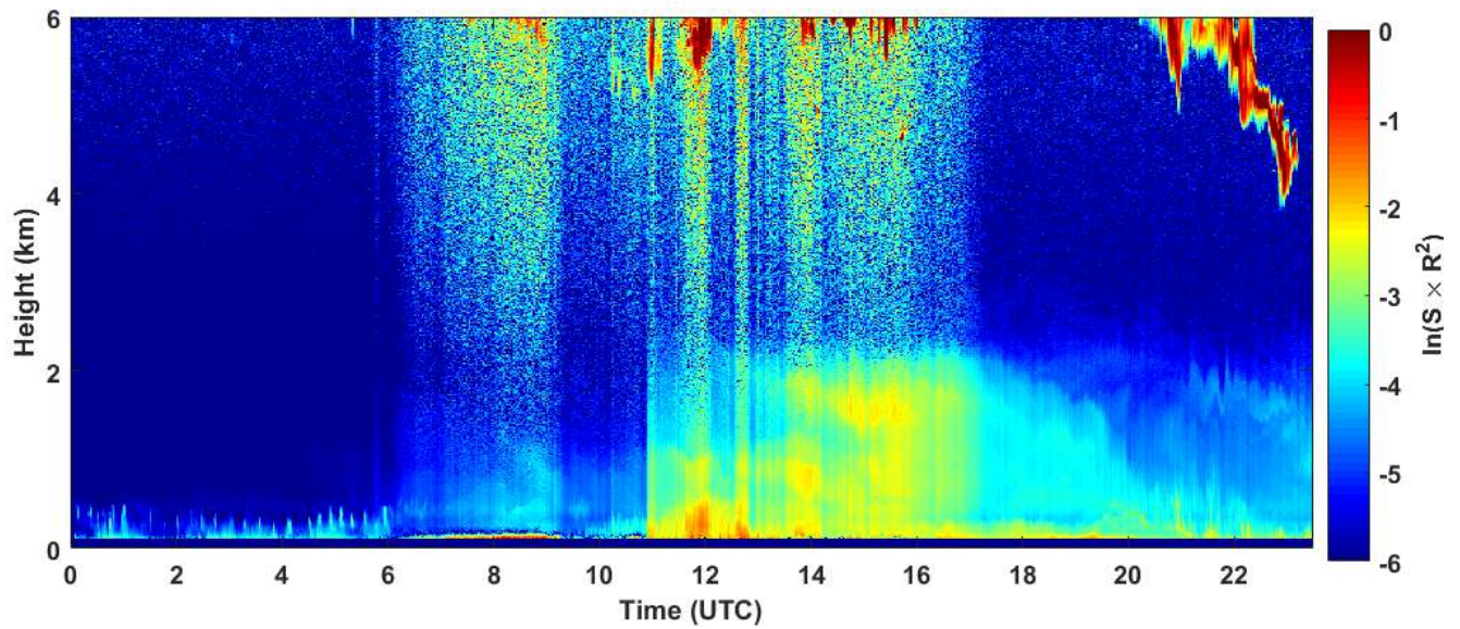
2019-03-06 RCS quick look CHM15k - ILVA LIDAR3 AGGLOMERATO
