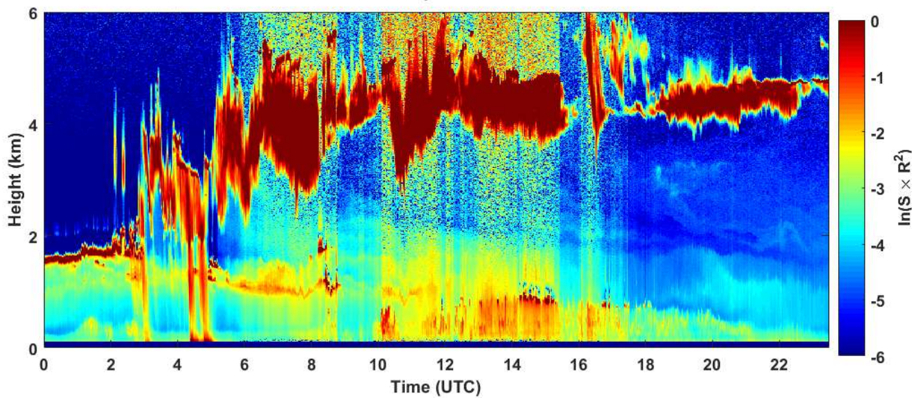
2019-03-20 RCS quick look CHM15k - ILVA LIDAR3 AGGLOMERATO
