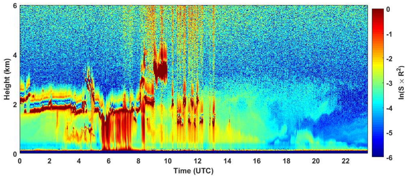
2019-03-02 RCS quick look CHM15k - ILVA LIDAR1 DIREZIONE
