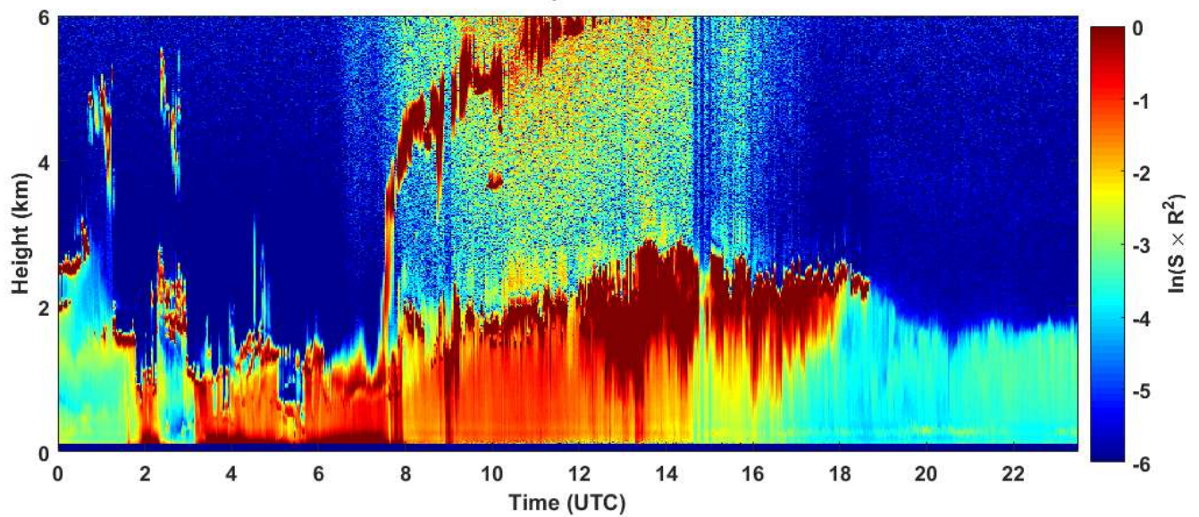
2019-03-12 RCS quick look CHM15k - ILVA LIDAR3 AGGLOMERATO
