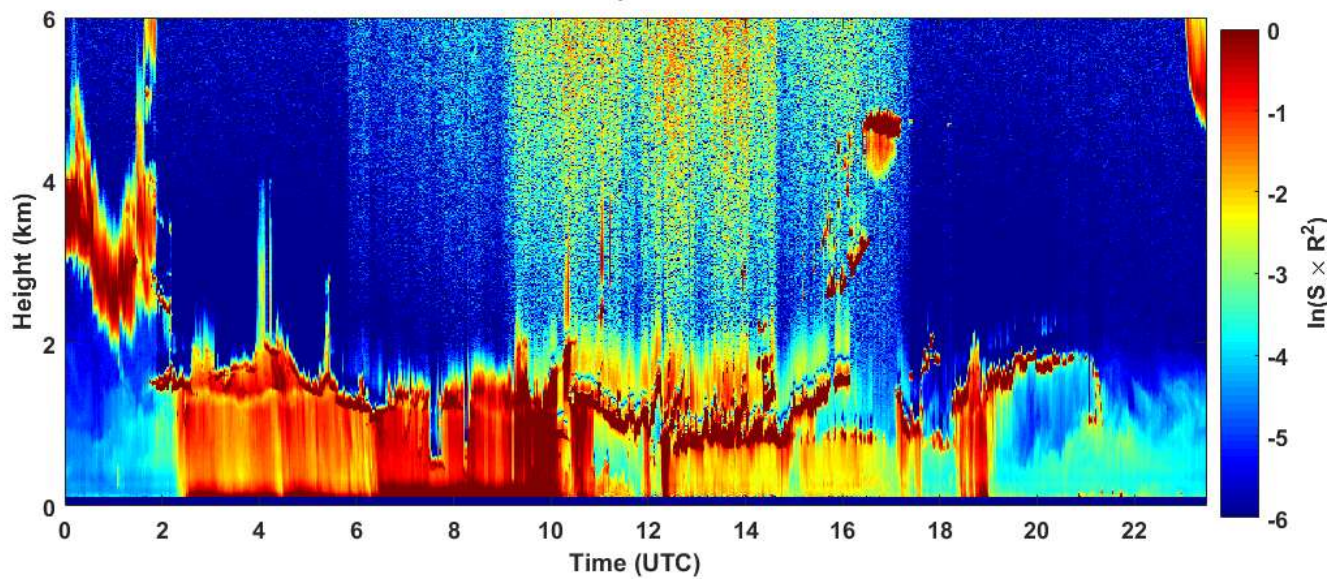
2019-03-14 RCS quick look CHM15k - ILVA LIDAR3 AGGLOMERATO
