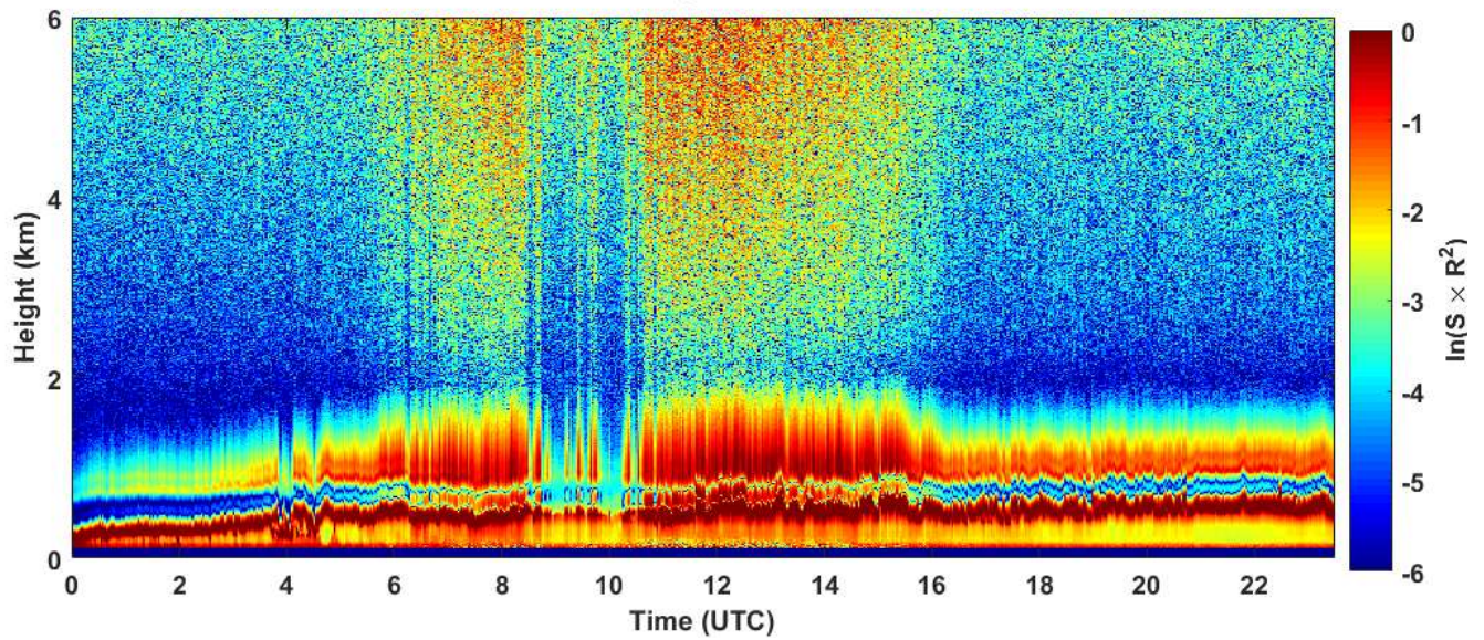
2019-03-18 RCS quick look CHM15k - ILVA LIDAR1 DIREZIONE
