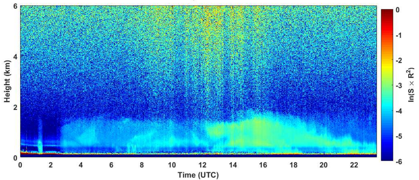
2019-03-10 RCS quick look CHM15k - ILVA LIDAR1 DIREZIONE
