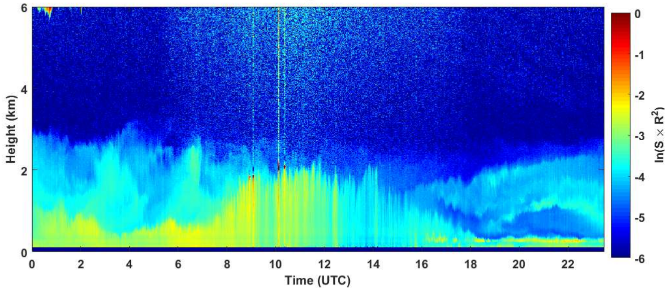
2019-03-30 RCS quick look CHM15k - ILVA LIDAR3 AGGLOMERATO
