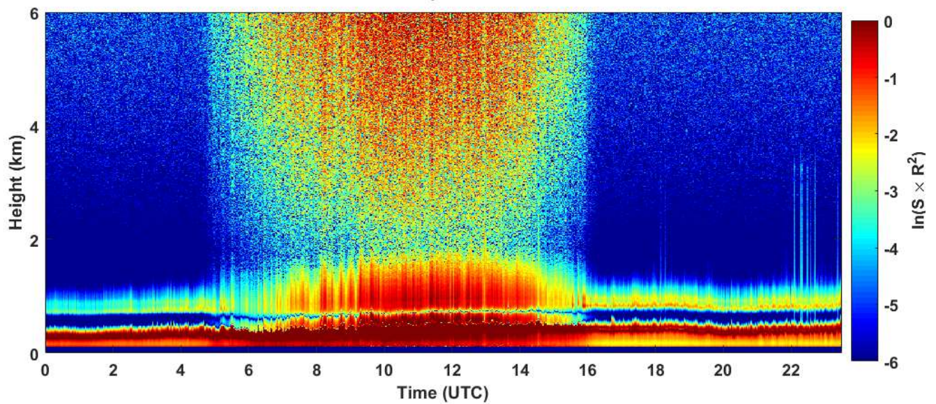
2019-03-08 RCS quick look CHM15k - ILVA LIDAR2 PARCHI
