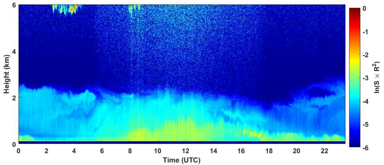
2019-03-24 RCS quick look CHM15k - ILVA LIDAR3 AGGLOMERATO
