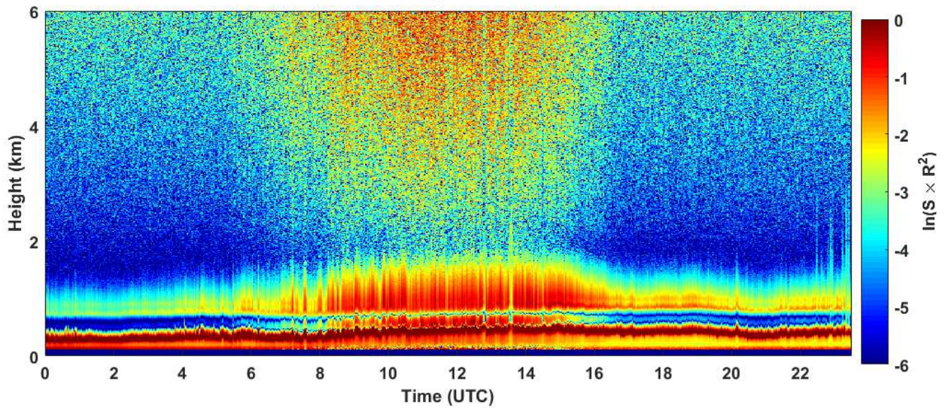
2019-03-08 RCS quick look CHM15k - ILVA LIDAR1 DIREZIONE
