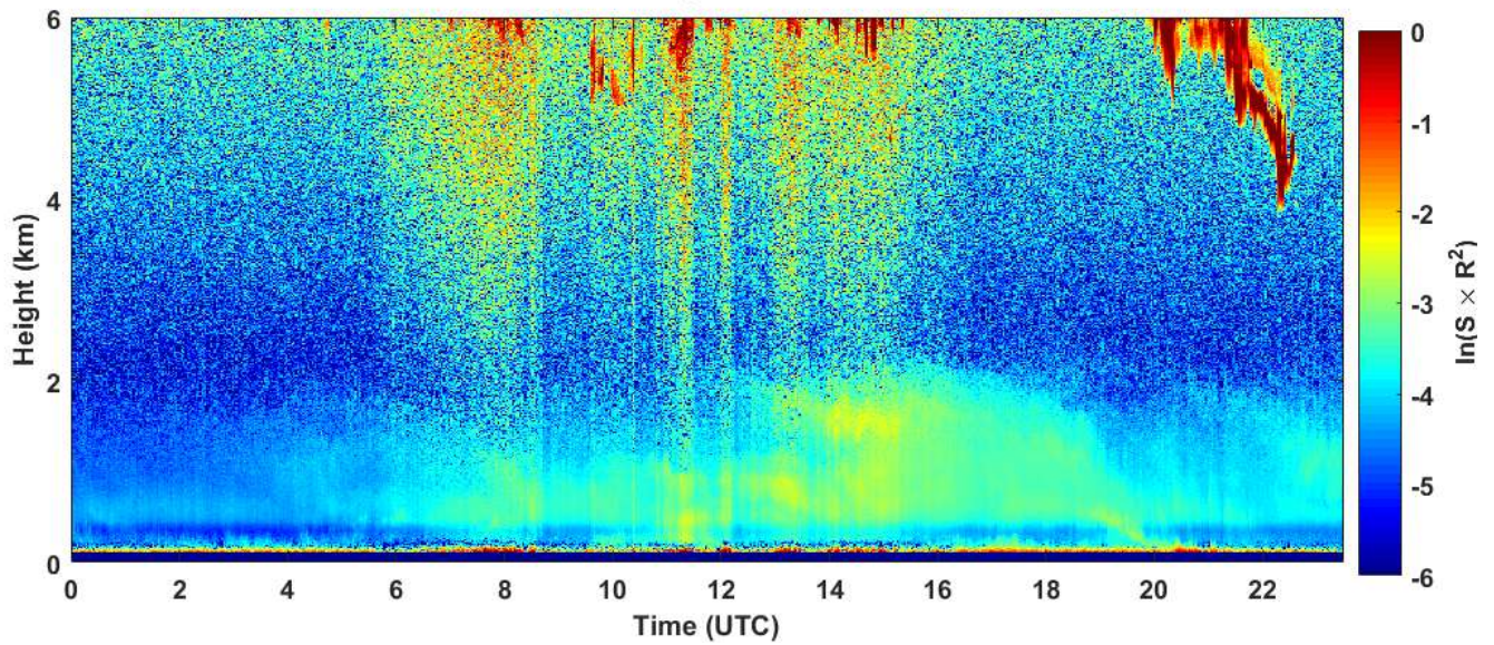
2019-03-06 RCS quick look CHM15k - ILVA LIDAR1 DIREZIONE
