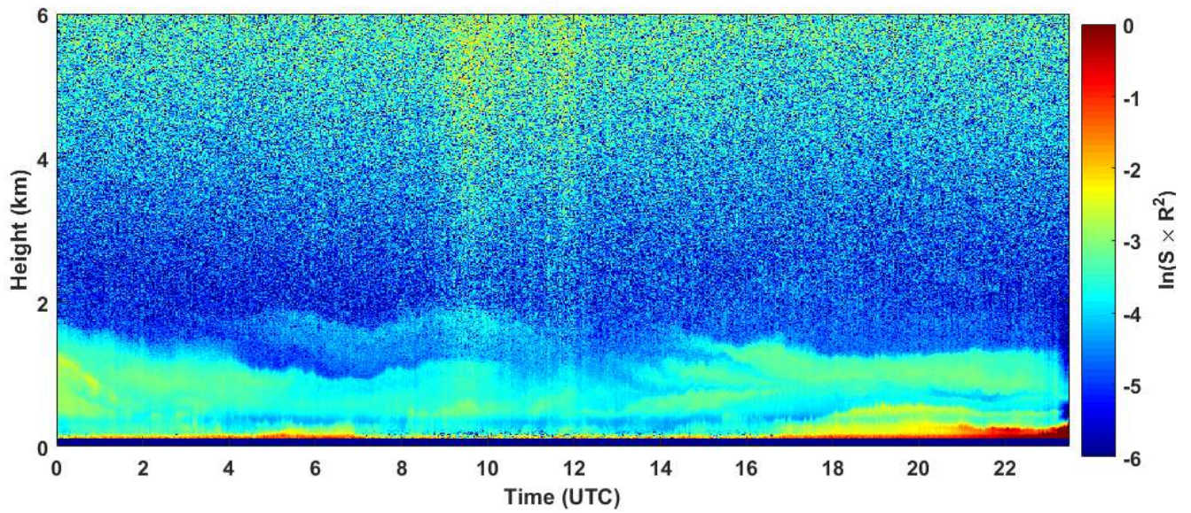
2019-03-16 RCS quick look CHM15k - ILVA LIDAR1 DIREZIONE
