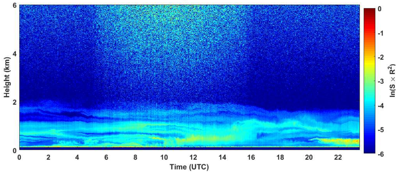
2019-02-20 RCS quick look CHM15k - ILVA LIDAR2 PARCHI
