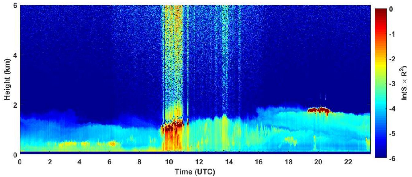
2019-02-10 RCS quick look CHM15k - ILVA LIDAR3 AGGLOMERATO
