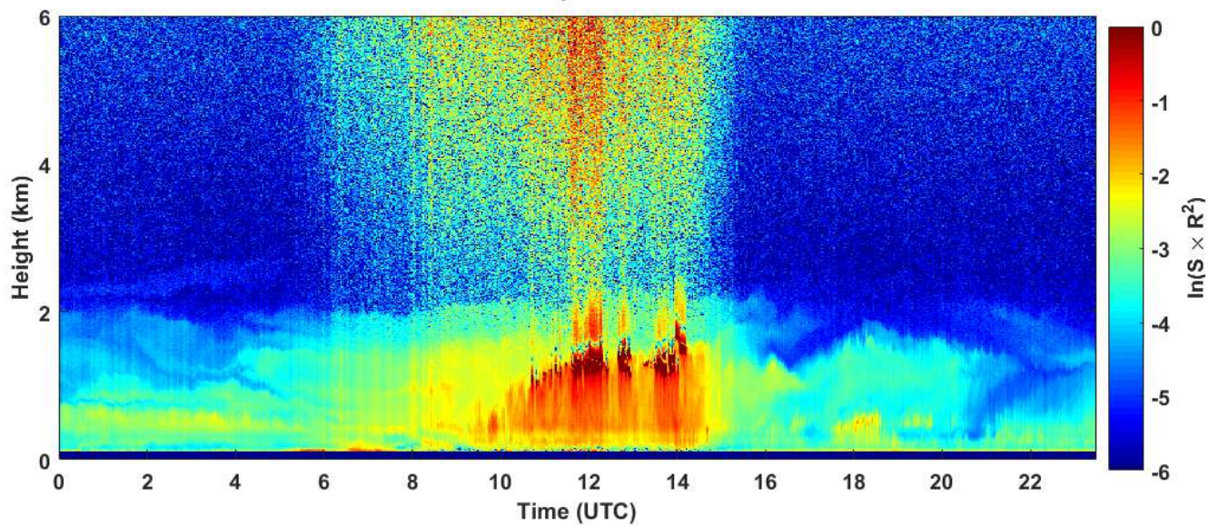
2019-02-08 RCS quick look CHM15k - ILVA LIDAR2 PARCHI
