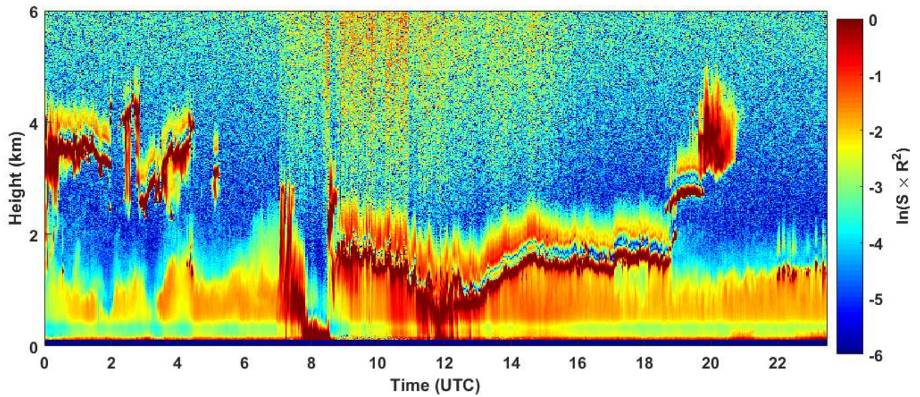
2019-02-24 RCS quick look CHM15k - ILVA LIDAR1 DIREZIONE
