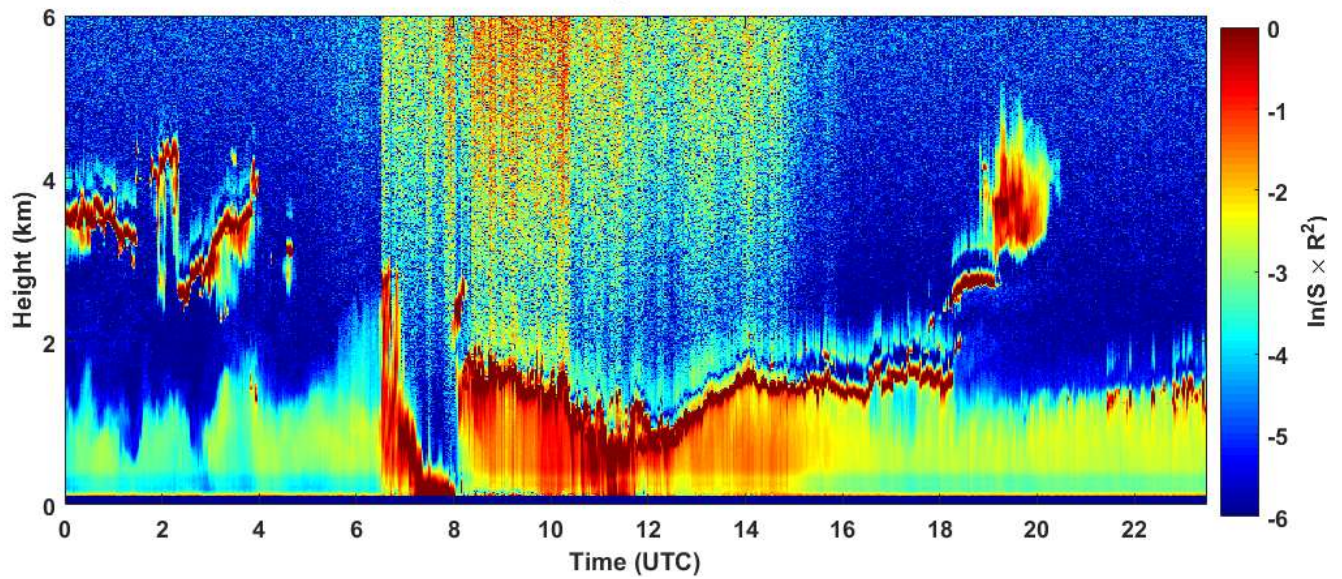
2019-02-24 RCS quick look CHM15k - ILVA LIDAR2 PARCHI
