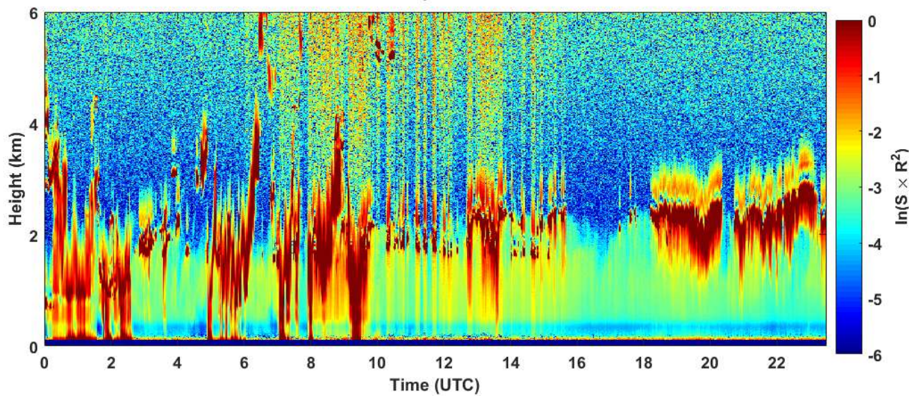
2019-02-12 RCS quick look CHM15k - ILVA LIDAR1 DIREZIONE
