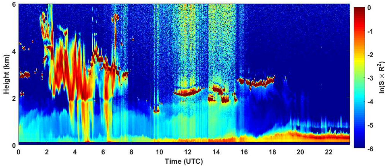
2019-02-02 RCS quick look CHM15k - ILVA LIDAR3 AGGLOMERATO
