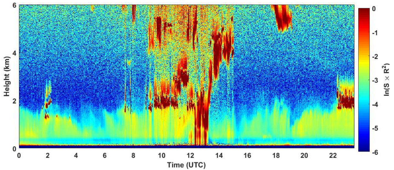
2019-02-16 RCS quick look CHM15k - ILVA LIDAR1 DIREZIONE
