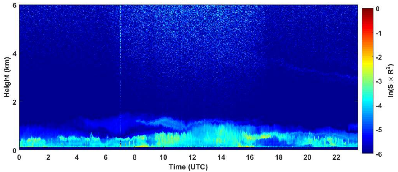
2019-02-18 RCS quick look CHM15k - ILVA LIDAR3 AGGLOMERATO
