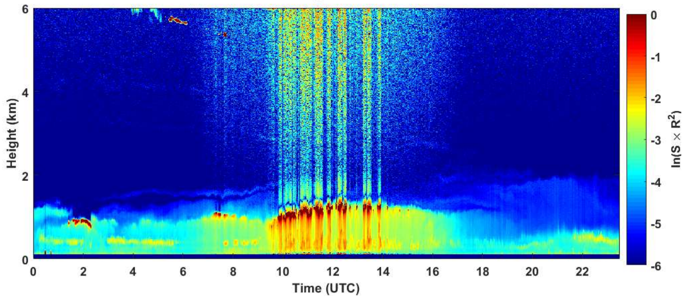
2019-02-22 RCS quick look CHM15k - ILVA LIDAR3 AGGLOMERATO
