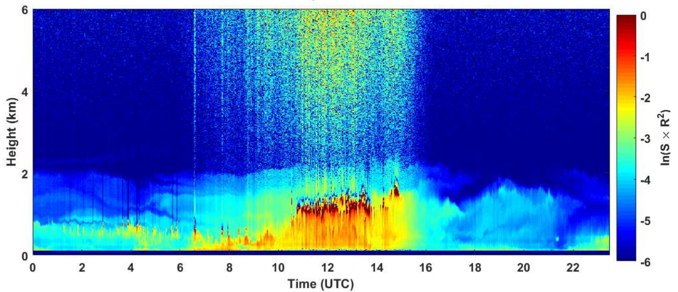
2019-02-08 RCS quick look CHM15k - ILVA LIDAR3 AGGLOMERATO
