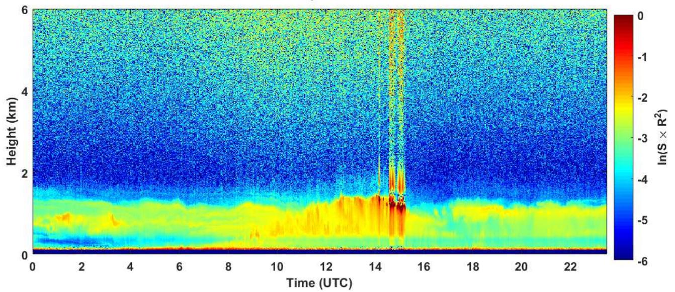
2019-02-20 RCS quick look CHM15k - ILVA LIDAR1 DIREZIONE
