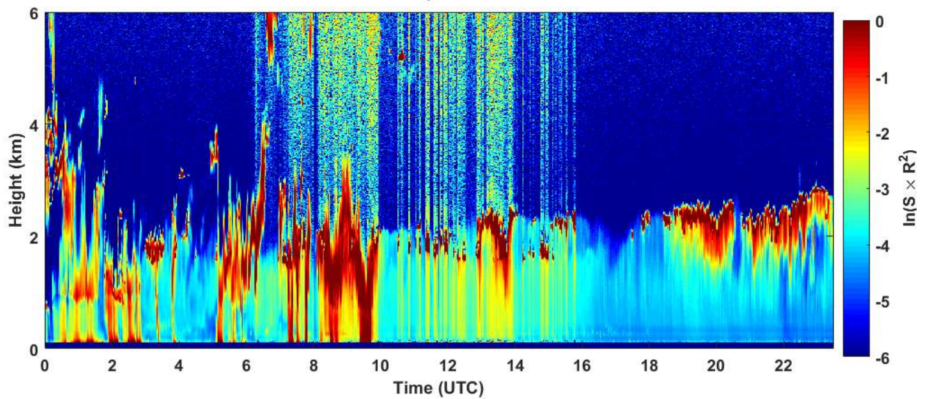
2019-02-12 RCS quick look CHM15k - ILVA LIDAR3 AGGLOMERATO
