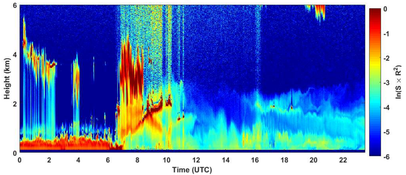
2019-02-04 RCS quick look CHM15k - ILVA LIDAR3 AGGLOMERATO
