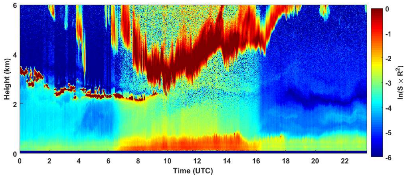
2019-02-06 RCS quick look CHM15k - ILVA LIDAR3 AGGLOMERATO
