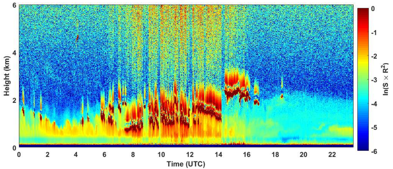
2019-02-08 RCS quick look CHM15k - ILVA LIDAR1 DIREZIONE
