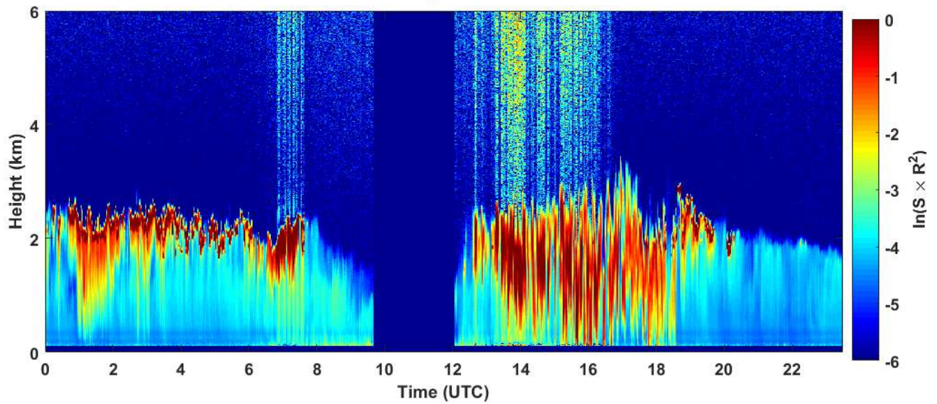
2019-02-14 RCS quick look CHM15k - ILVA LIDAR3 AGGLOMERATO
