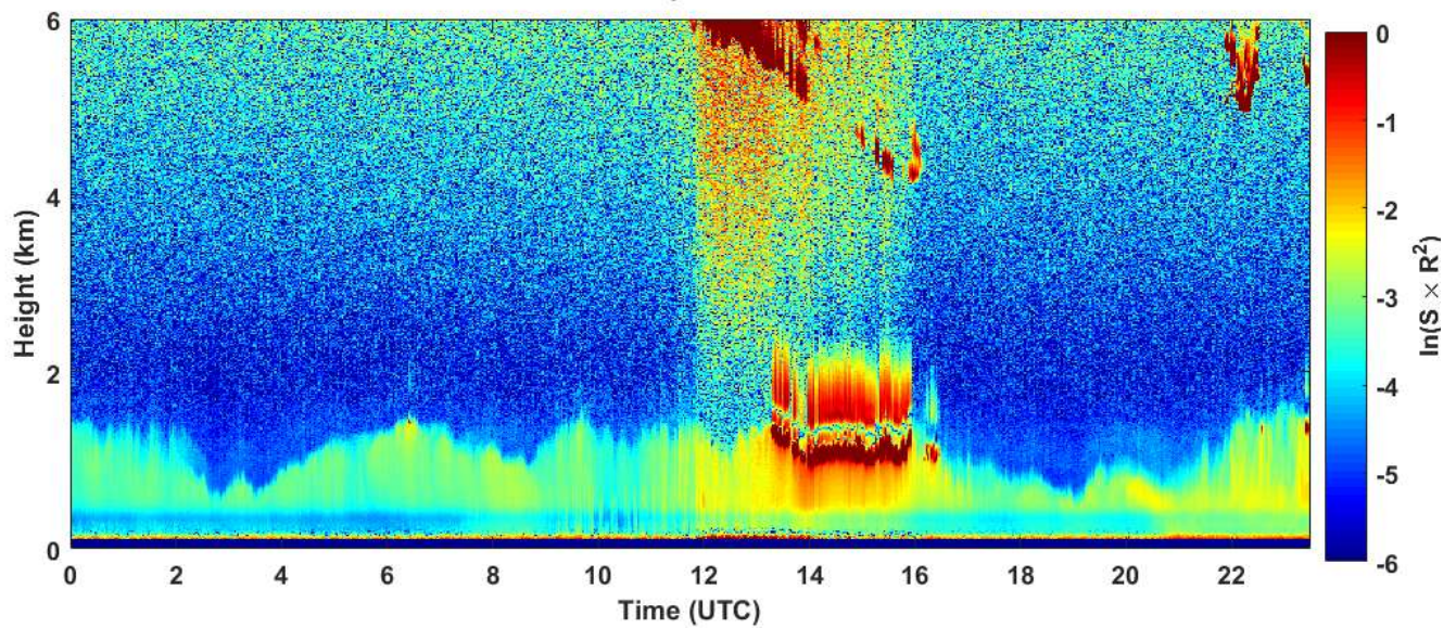
2019-02-14 RCS quick look CHM15k - ILVA LIDAR1 DIREZIONE
