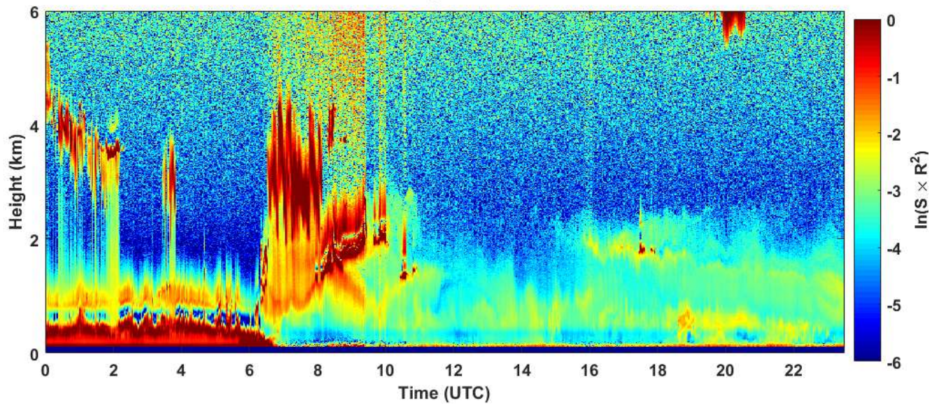
2019-02-04 RCS quick look CHM15k - ILVA LIDAR1 DIREZIONE
