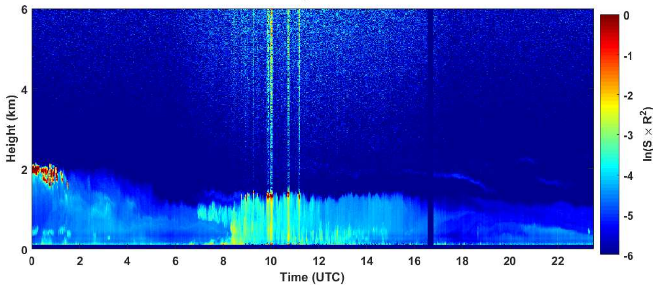
2019-02-28 RCS quick look CHM15k - ILVA LIDAR3 AGGLOMERATO
