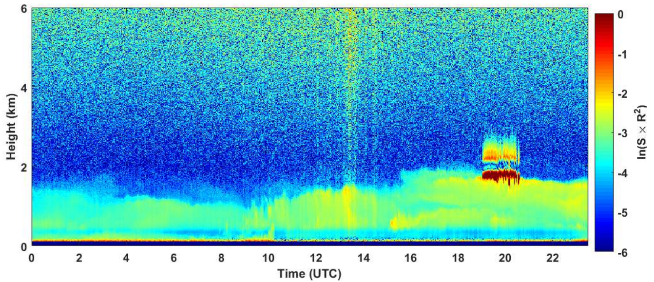
2019-02-10 RCS quick look CHM15k - ILVA LIDAR1 DIREZIONE
