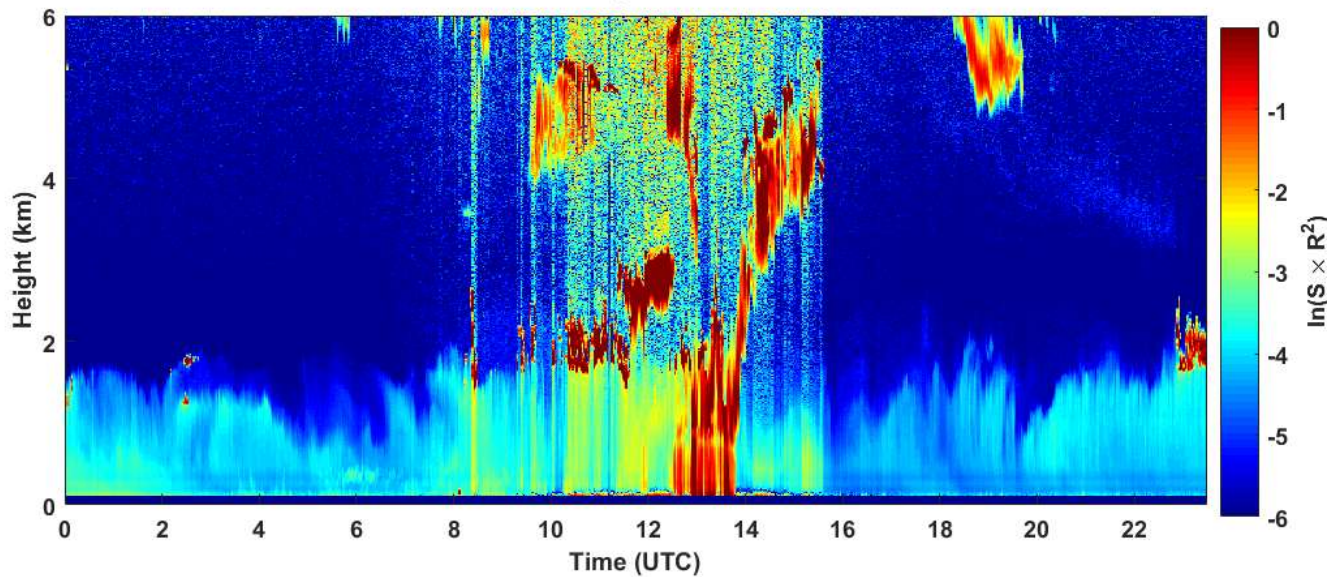
2019-02-16 RCS quick look CHM15k - ILVA LIDAR3 AGGLOMERATO
