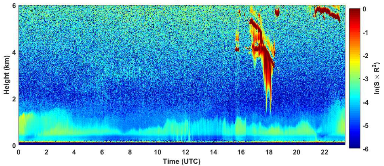
2019-02-26 RCS quick look CHM15k - ILVA LIDAR1 DIREZIONE
