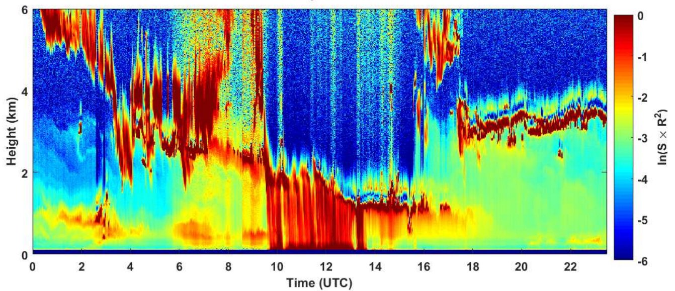
2019-02-04 RCS quick look CHM15k - ILVA LIDAR2 PARCHI
