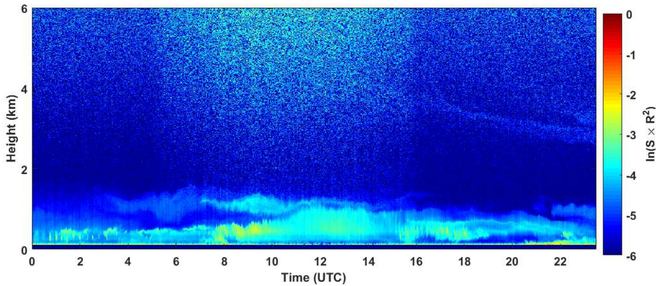
2019-02-18 RCS quick look CHM15k - ILVA LIDAR2 PARCHI
