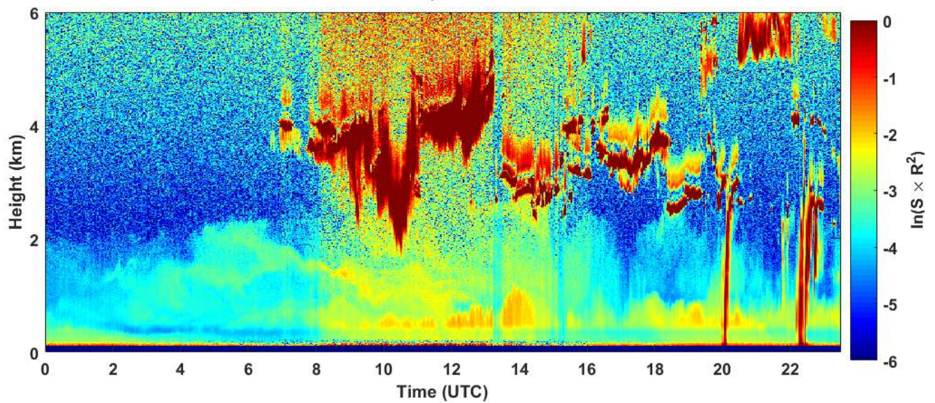
2019-02-22 RCS quick look CHM15k - ILVA LIDAR1 DIREZIONE
