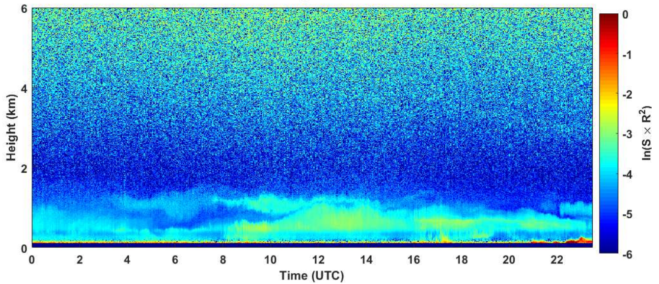
2019-02-18 RCS quick look CHM15k - ILVA LIDAR1 DIREZIONE
