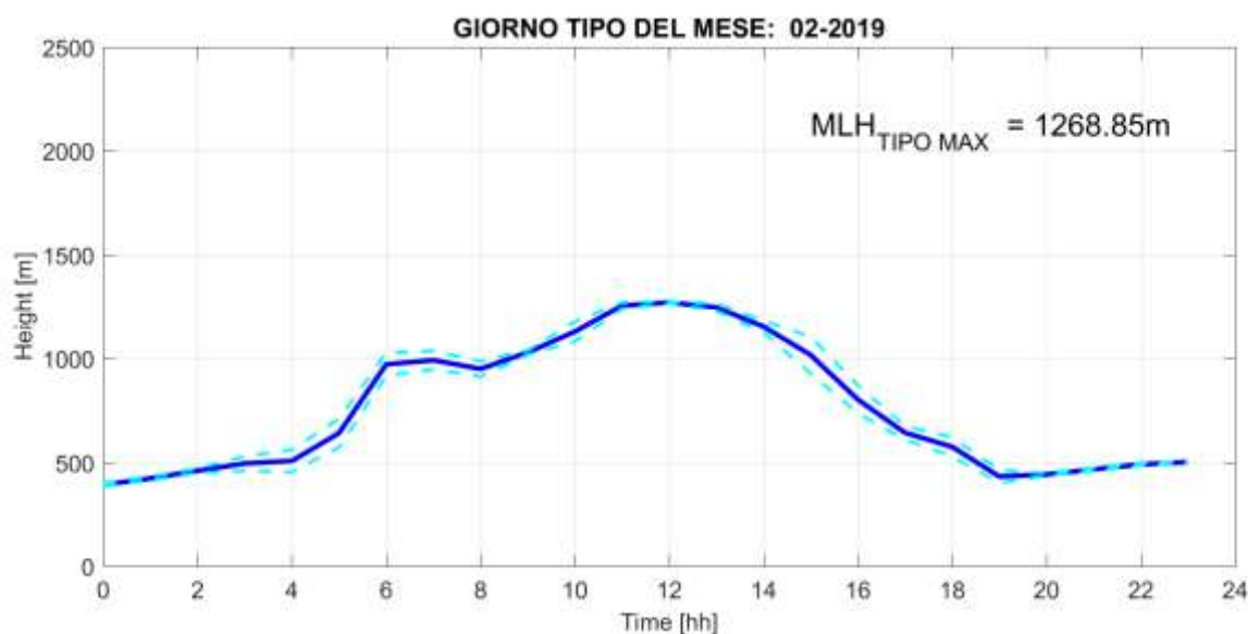
Fig. 2: Giorno tipo del parametro Mixing Layer Height nel mese di FEBBRAIO 2019, rappresentato mediante media oraria (linea blu continua) e deviazione standard (linee celesti tratteggiate).
