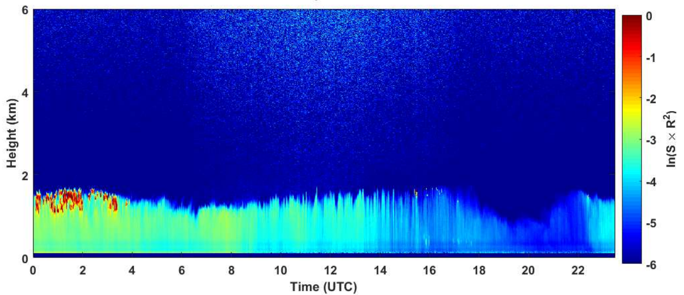
2019-02-24 RCS quick look CHM15k - ILVA LIDAR3 AGGLOMERATO
