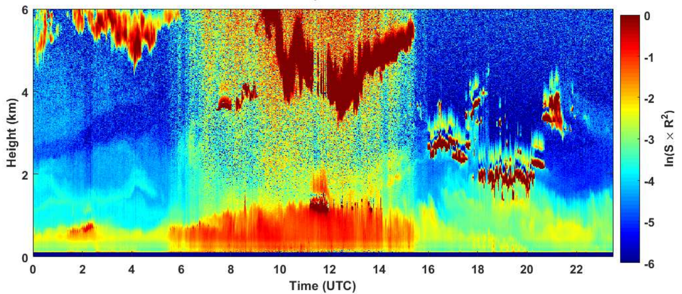
2019-02-06 RCS quick look CHM15k - ILVA LIDAR2 PARCHI
