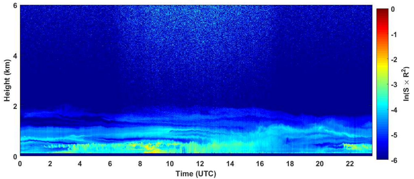
2019-02-20 RCS quick look CHM15k - ILVA LIDAR3 AGGLOMERATO
