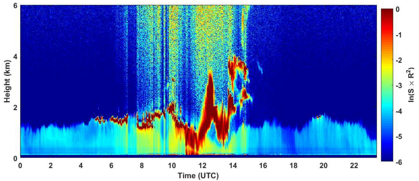
2019-02-26 RCS quick look CHM15k - ILVA LIDAR3 AGGLOMERATO
