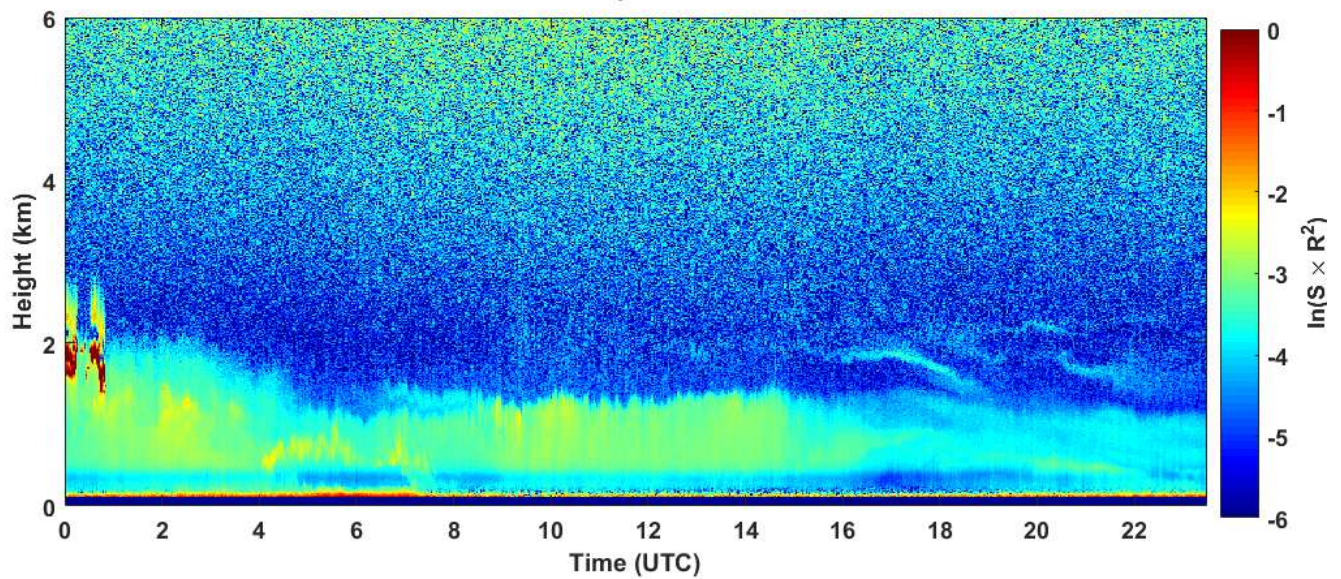
2019-02-28 RCS quick look CHM15k - ILVA LIDAR1 DIREZIONE
