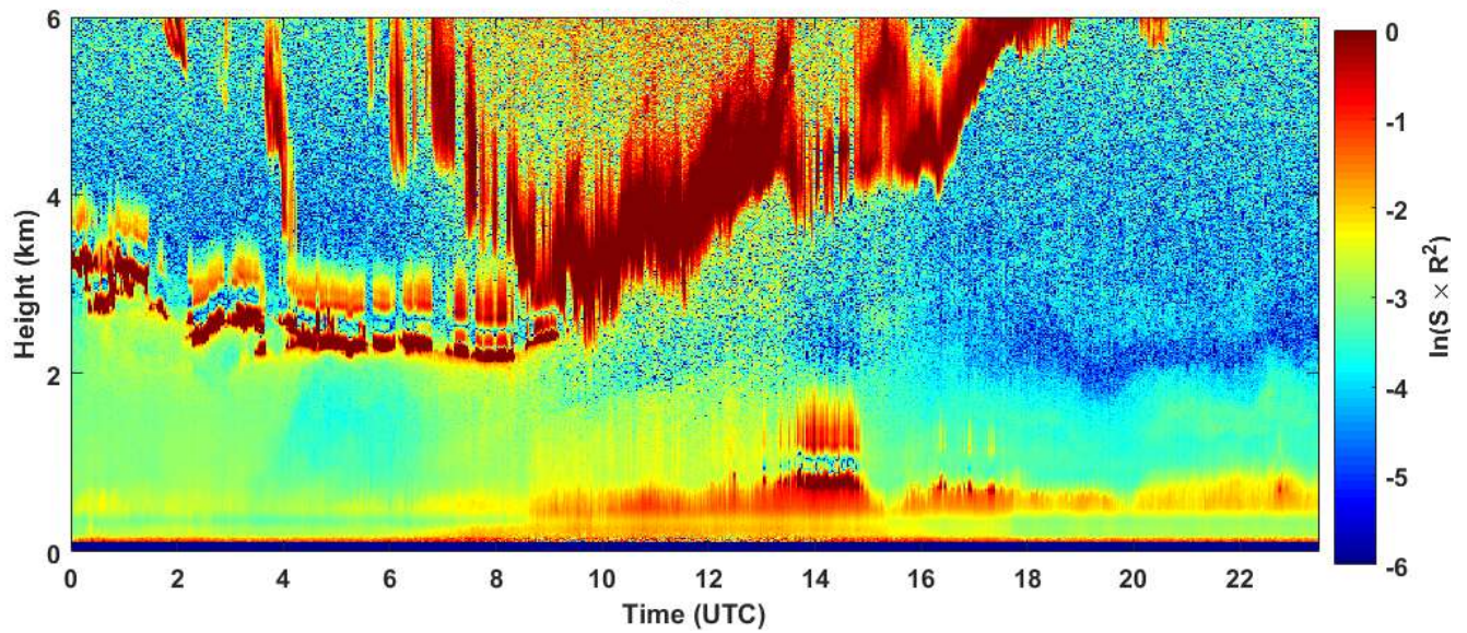
2019-02-06 RCS quick look CHM15k - ILVA LIDAR1 DIREZIONE
