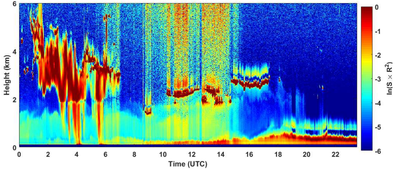
2019-02-02 RCS quick look CHM15k - ILVA LIDAR2 PARCHI
