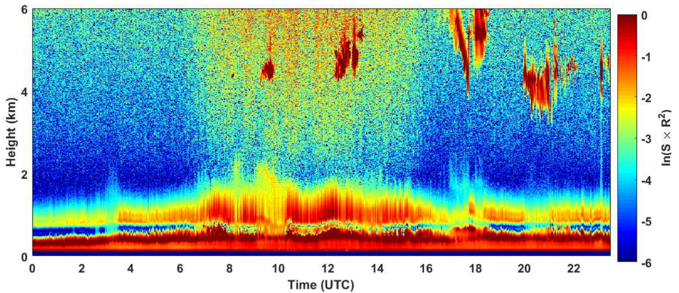
2019-02-02 RCS quick look CHM15k - ILVA LIDAR1 DIREZIONE
