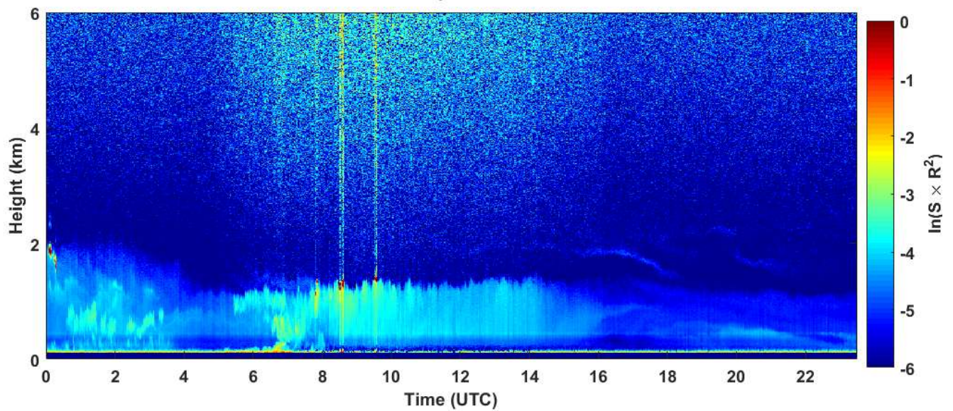
2019-02-28 RCS quick look CHM15k - ILVA LIDAR2 PARCHI
