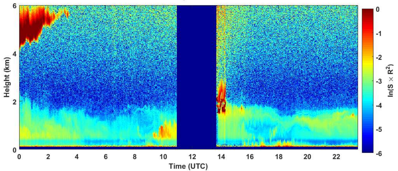
2019-01-29 RCS quick look CHM15k - ILVA LIDAR1 DIREZIONE
