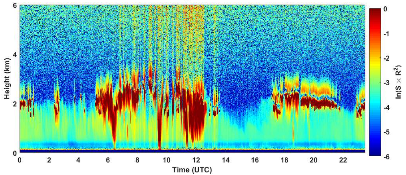
2019-01-08 RCS quick look CHM15k - ILVA LIDAR1 DIREZIONE
