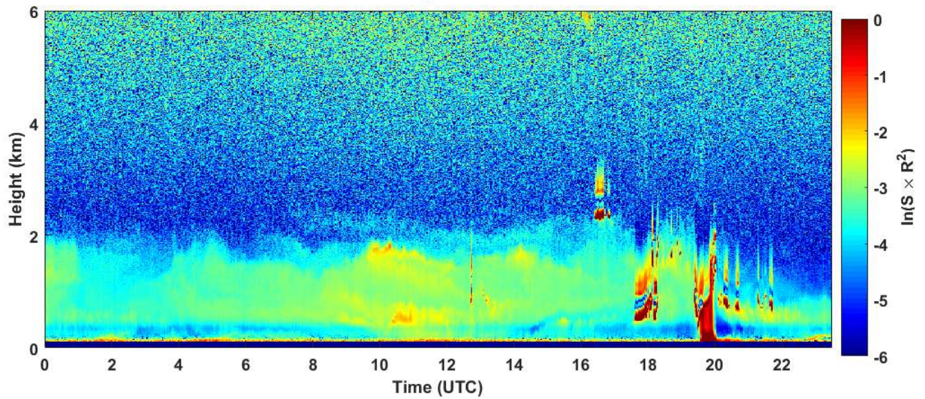
2019-01-20 RCS quick look CHM15k - ILVA LIDAR1 DIREZIONE
