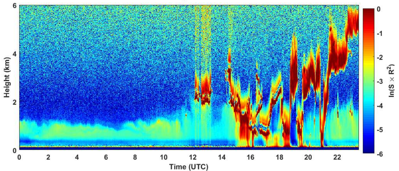
2019-01-02 RCS quick look CHM15k - ILVA LIDAR1 DIREZIONE
