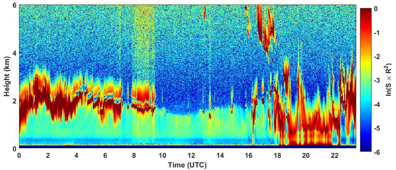
2019-01-06 RCS quick look CHM15k - ILVA LIDAR1 DIREZIONE
