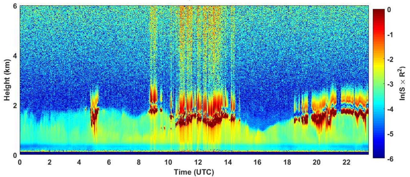
2019-01-12 RCS quick look CHM15k - ILVA LIDAR1 DIREZIONE
