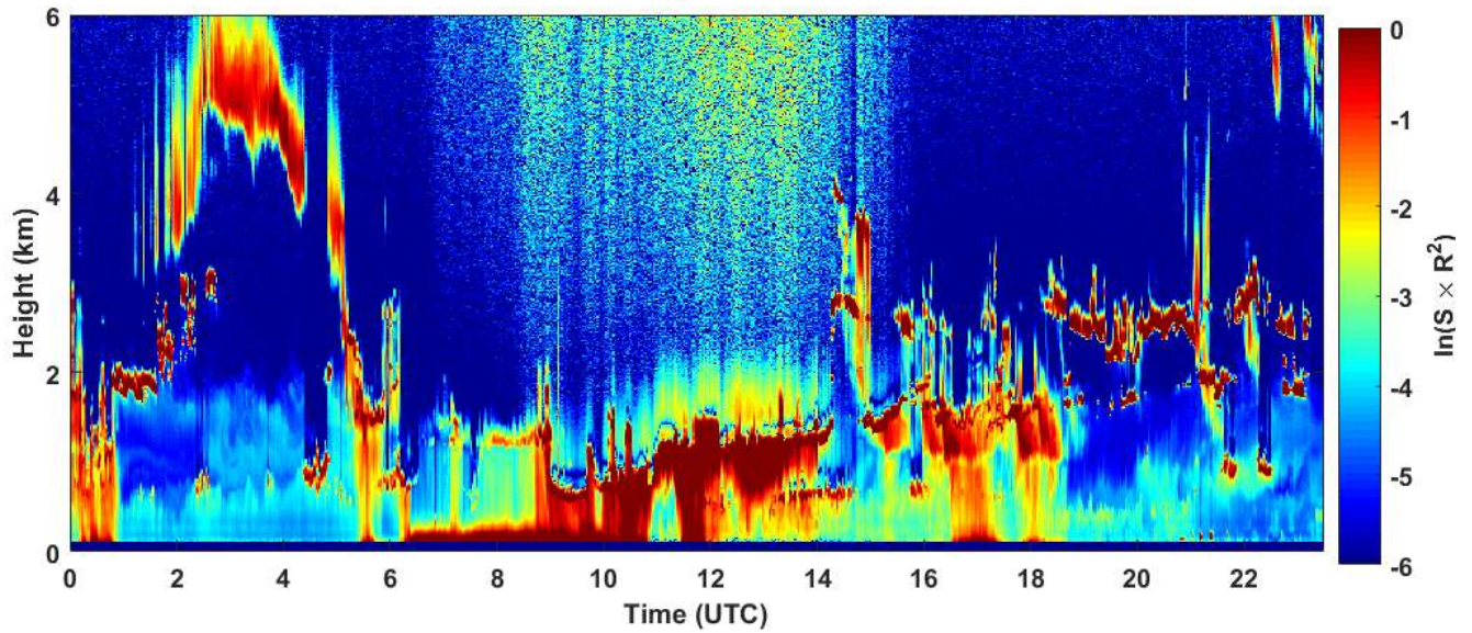
2019-01-10 RCS quick look CHM15k - ILVA LIDAR3 AGGLOMERATO
