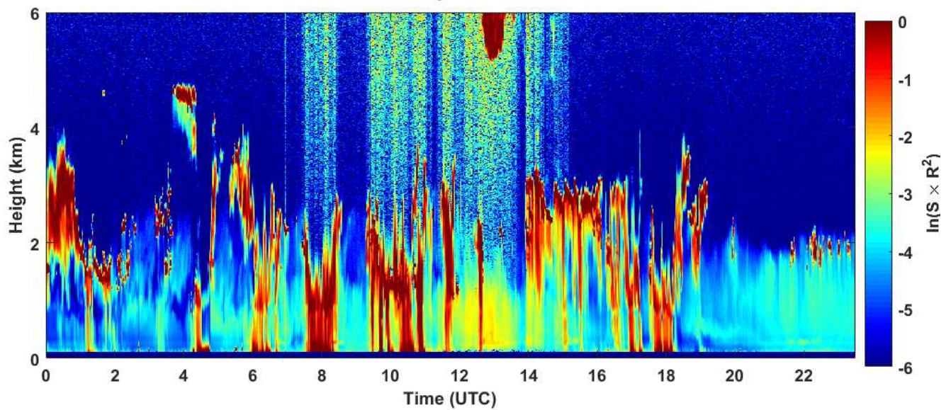
2019-01-06 RCS quick look CHM15k - ILVA LIDAR3 AGGLOMERATO
