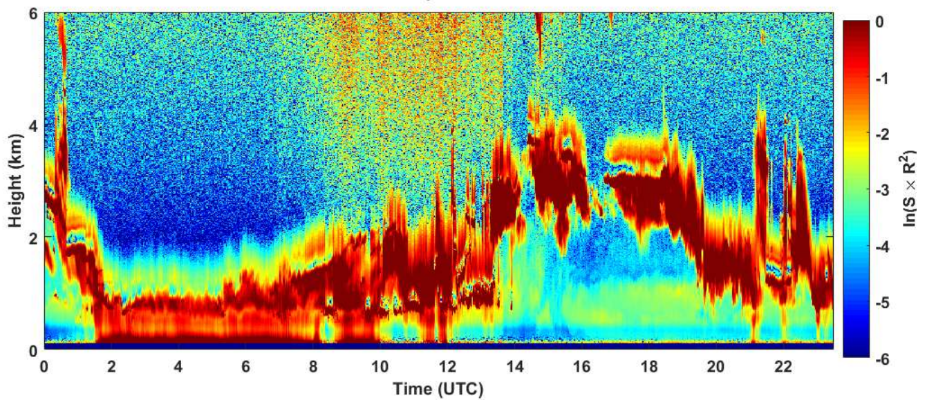
2019-01-10 RCS quick look CHM15k - ILVA LIDAR1 DIREZIONE
