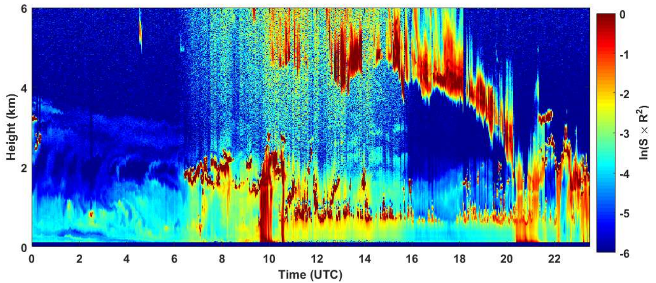
2019-01-22 RCS quick look CHM15k - ILVA LIDAR3 AGGLOMERATO
