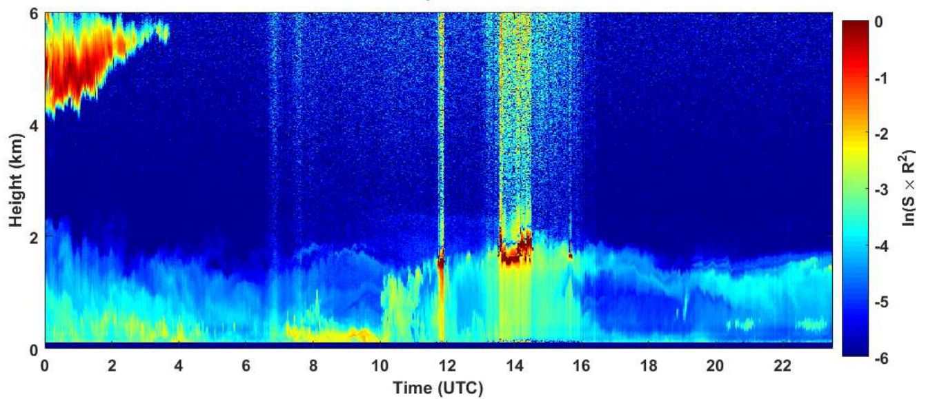
2019-01-29 RCS quick look CHM15k - ILVA LIDAR3 AGGLOMERATO
