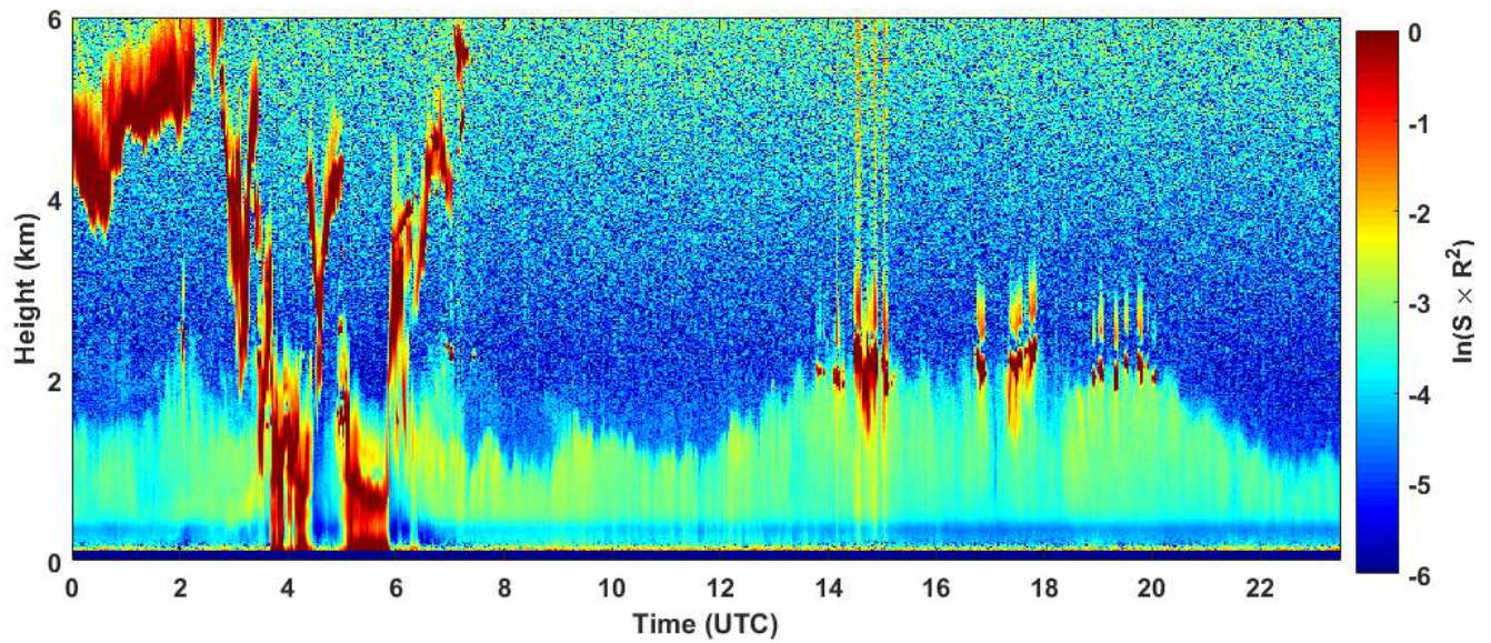
2019-01-16 RCS quick look CHM15k - ILVA LIDAR1 DIREZIONE
