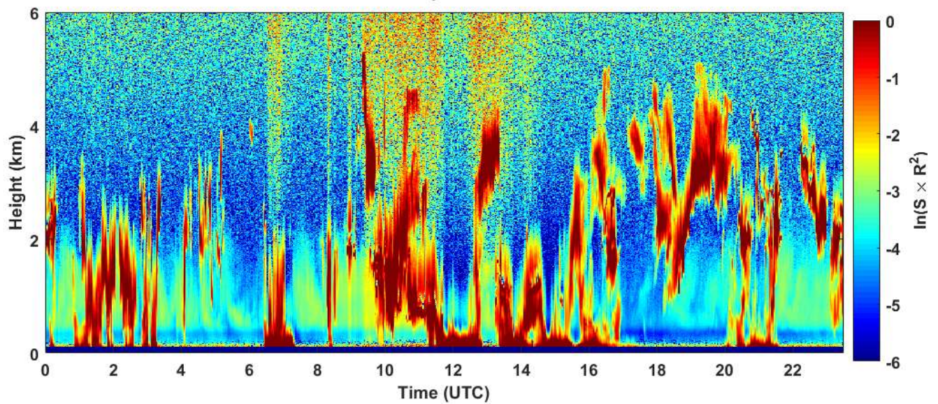
2019-01-04 RCS quick look CHM15k - ILVA LIDAR1 DIREZIONE
