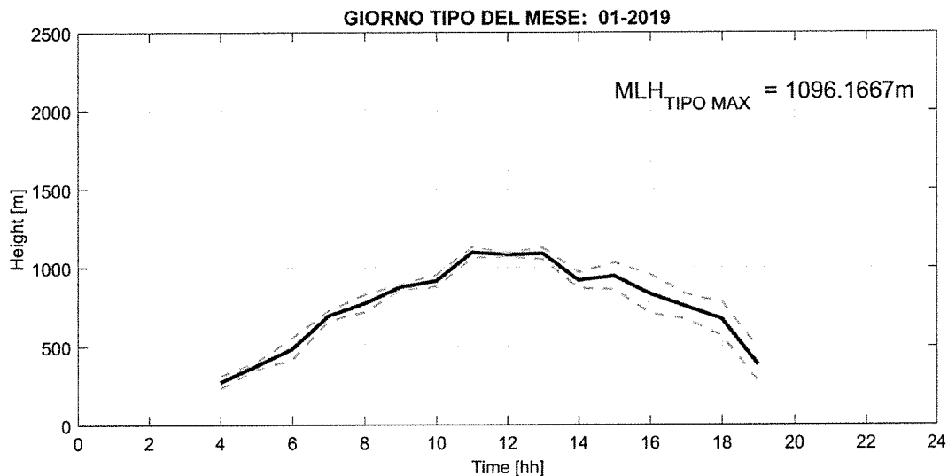
Fig. 2: Giorno tipo del parametro Mixing Layer Height nel mese di GENNAIO 2019, rappresentato mediante media oraria (linea blu continua) e deviazione standard (linee celesti tratteggiate).
