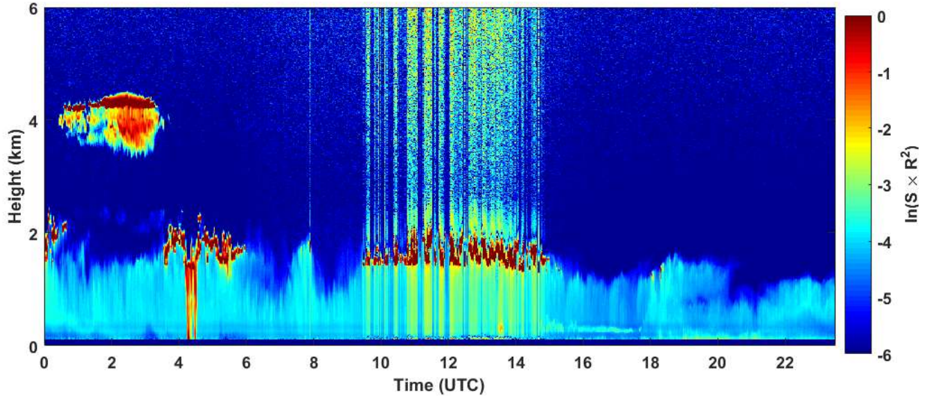
2019-01-02 RCS quick look CHM15k - ILVA LIDAR3 AGGLOMERATO
