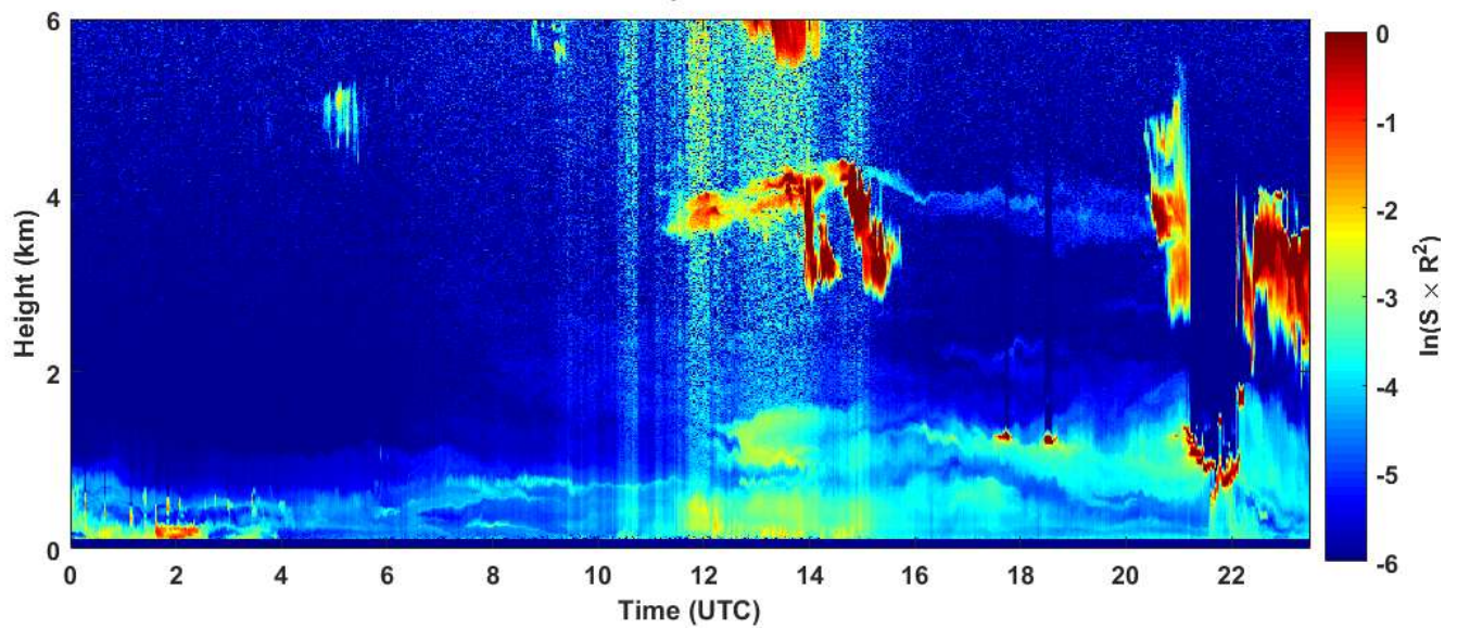
2019-01-20 RCS quick look CHM15k - ILVA LIDAR3 AGGLOMERATO
