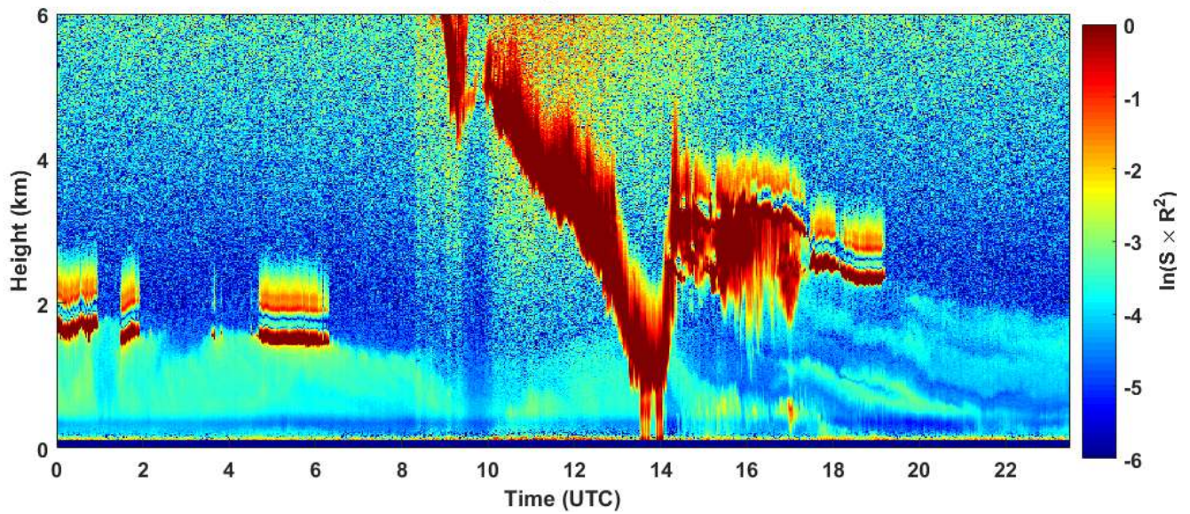
2019-01-14 RCS quick look CHM15k - ILVA LIDAR1 DIREZIONE
