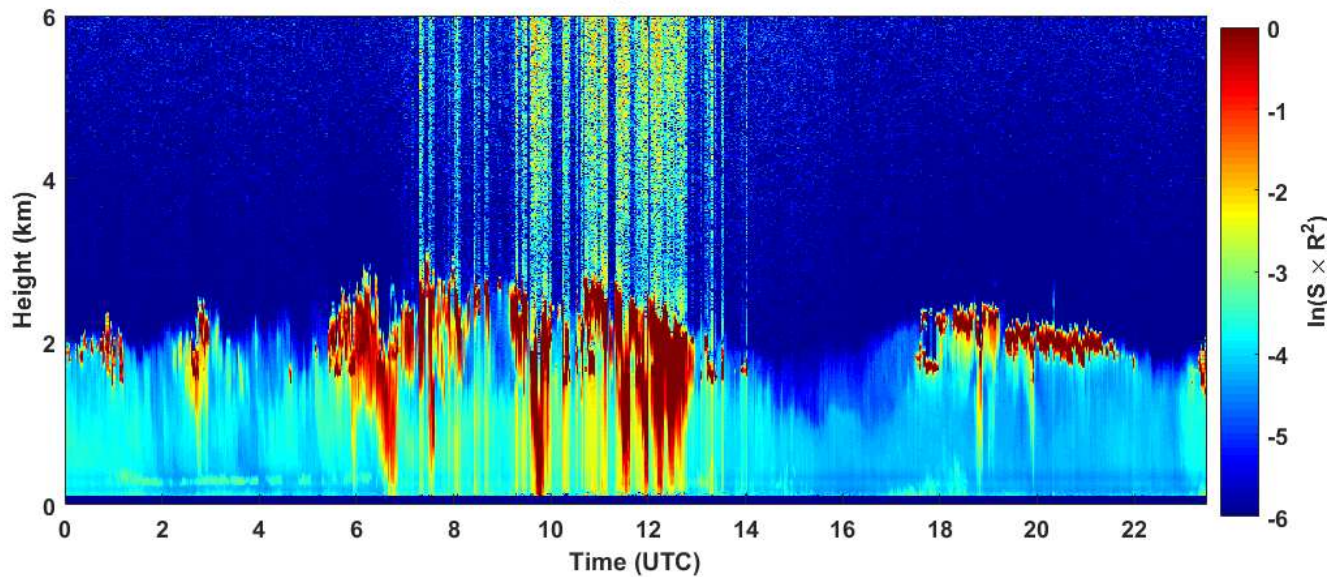
2019-01-08 RCS quick look CHM15k - ILVA LIDAR3 AGGLOMERATO
