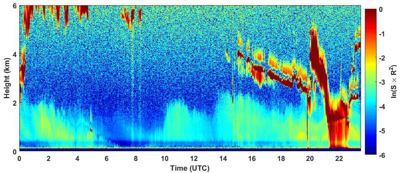
2019-01-31 RCS quick look CHM15k - ILVA LIDAR1 DIREZIONE
