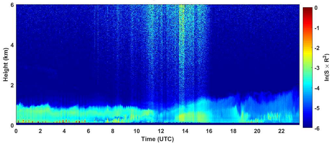
2019-01-27 RCS quick look CHM15k - ILVA LIDAR3 AGGLOMERATO
