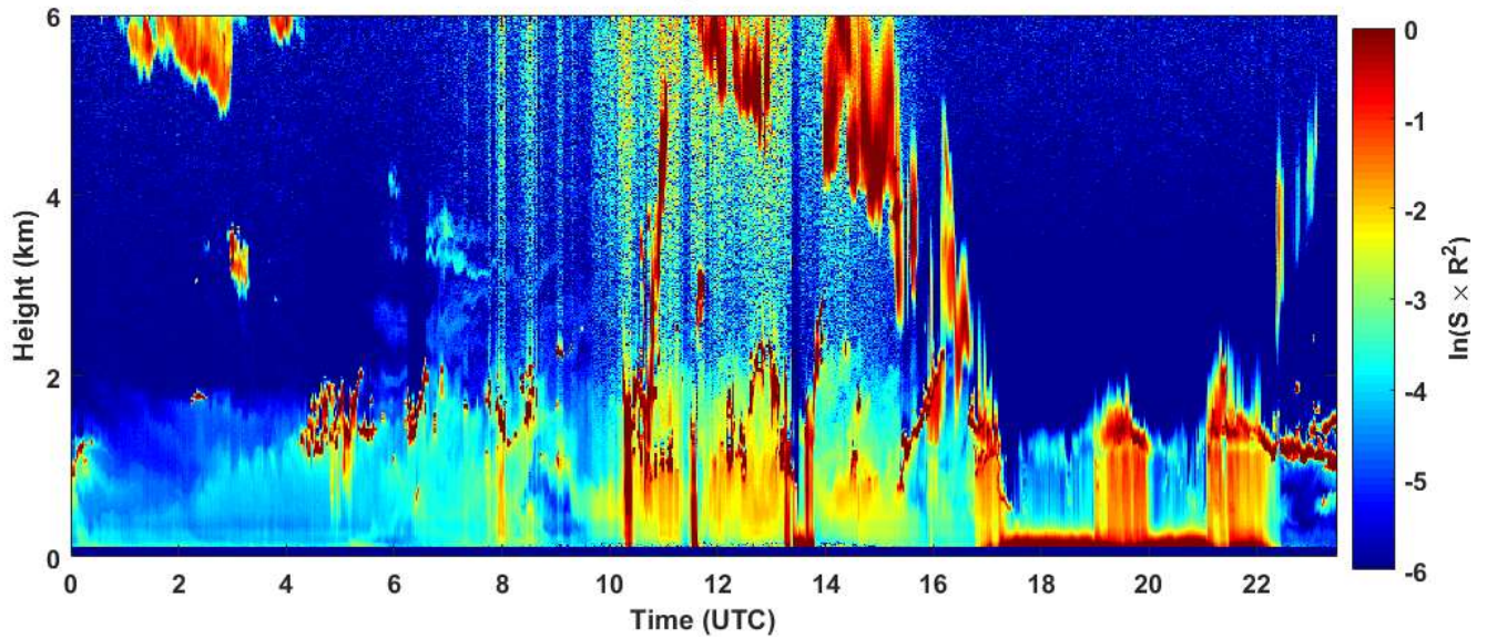
2019-01-25 RCS quick look CHM15k - ILVA LIDAR3 AGGLOMERATO
