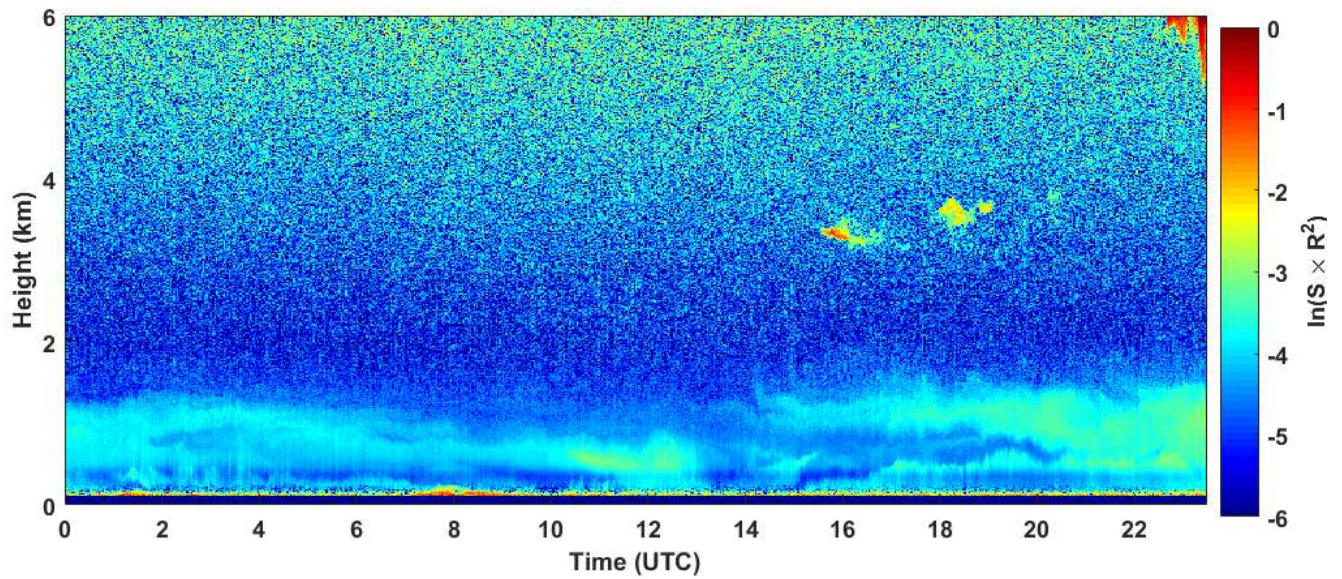
2019-01-18 RCS quick look CHM15k - ILVA LIDAR1 DIREZIONE
