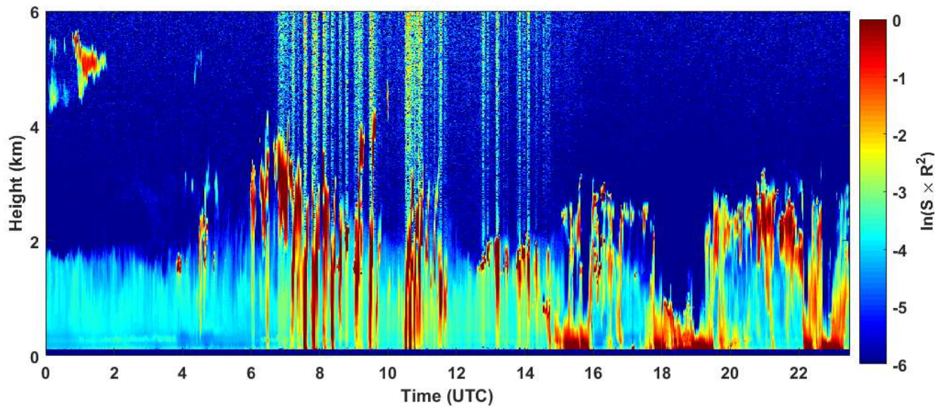
2019-01-04 RCS quick look CHM15k - ILVA LIDAR3 AGGLOMERATO
