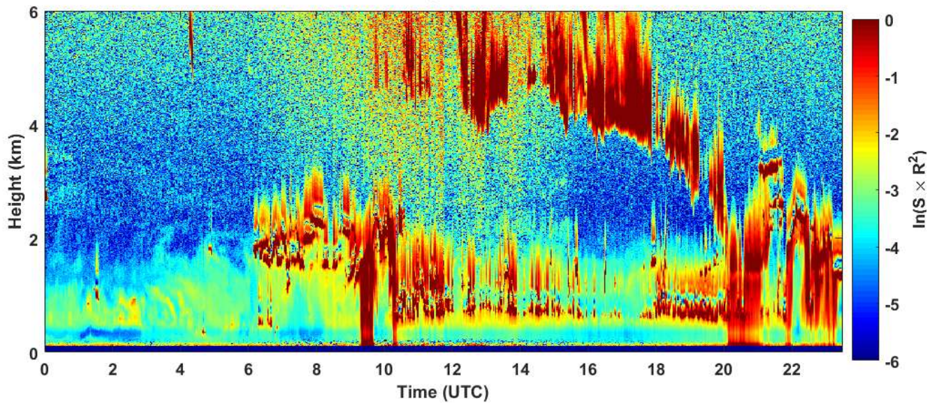
2019-01-22 RCS quick look CHM15k - ILVA LIDAR1 DIREZIONE
