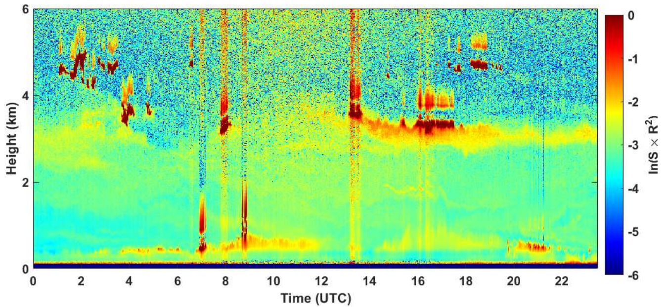
2020-09-08 RCS quick look CHM15k - ILVA LIDAR1 DIREZIONE
