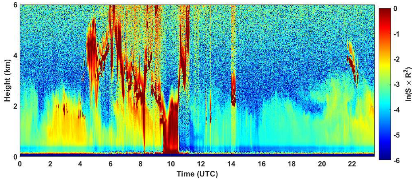
2020-09-26 RCS quick look CHM15k - ILVA LIDAR1 DIREZIONE
