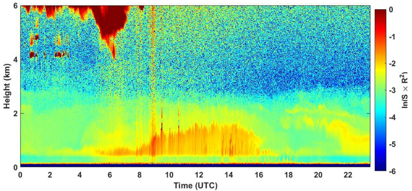
2020-09-20 RCS quick look CHM15k - ILVA LIDAR1 DIREZIONE
