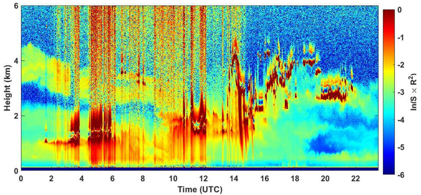
2020-09-04 RCS quick look CHM15k - ILVA LIDAR2 PARCHI
