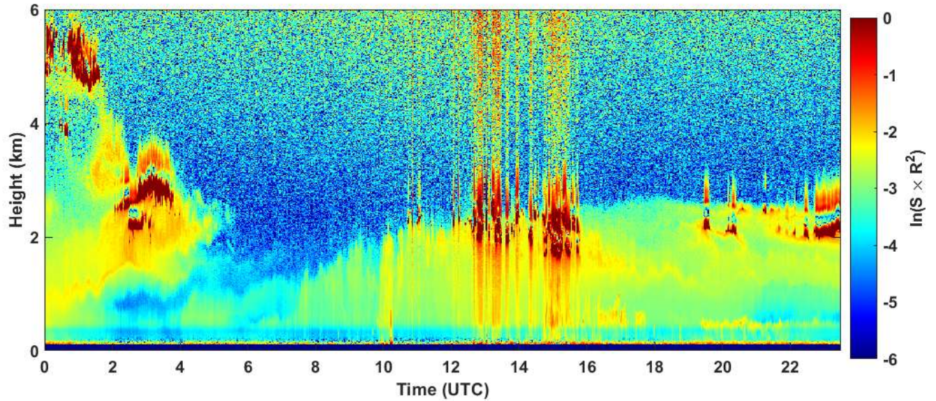
2020-09-02 RCS quick look CHM15k - ILVA LIDAR1 DIREZIONE
