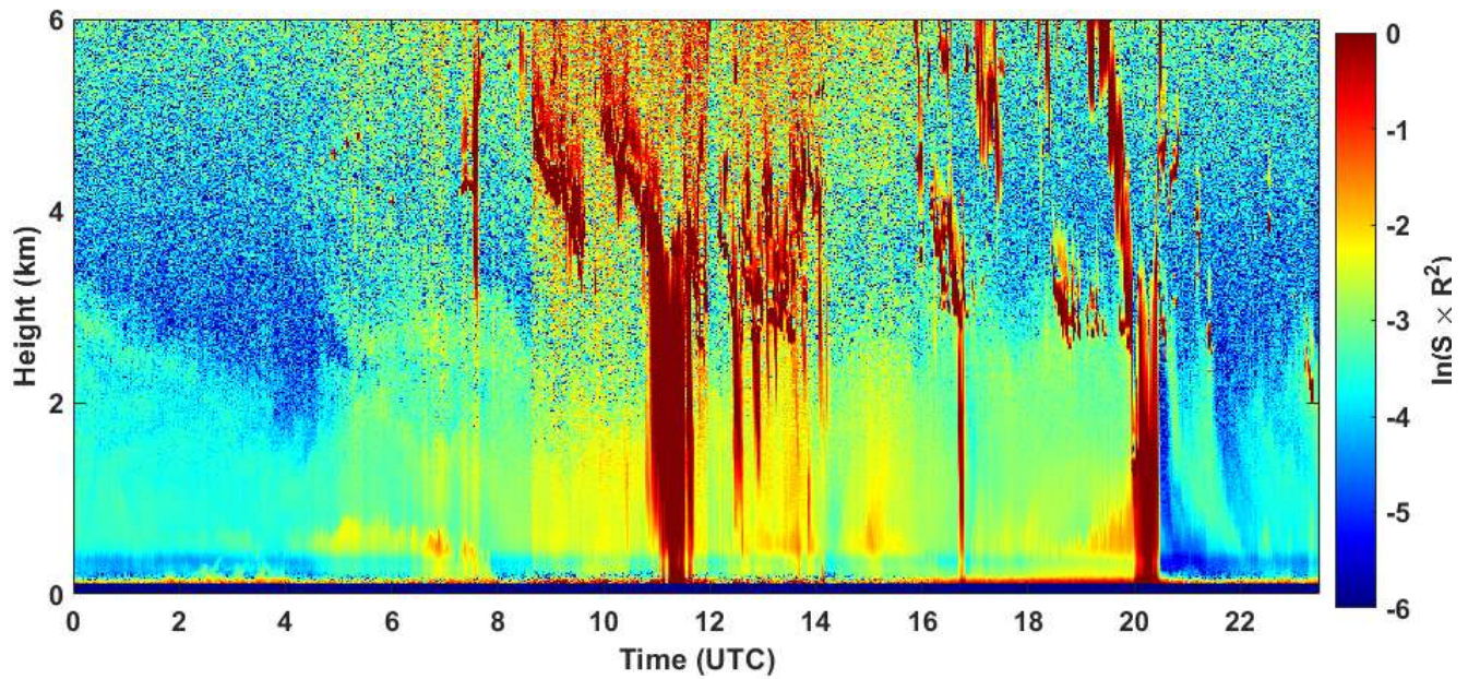
2020-09-26 RCS quick look CHM15k - ILVA LIDAR1 DIREZIONE
