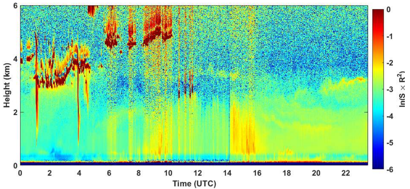
2020-09-16 RCS quick look CHM15k - ILVA LIDAR1 DIREZIONE
