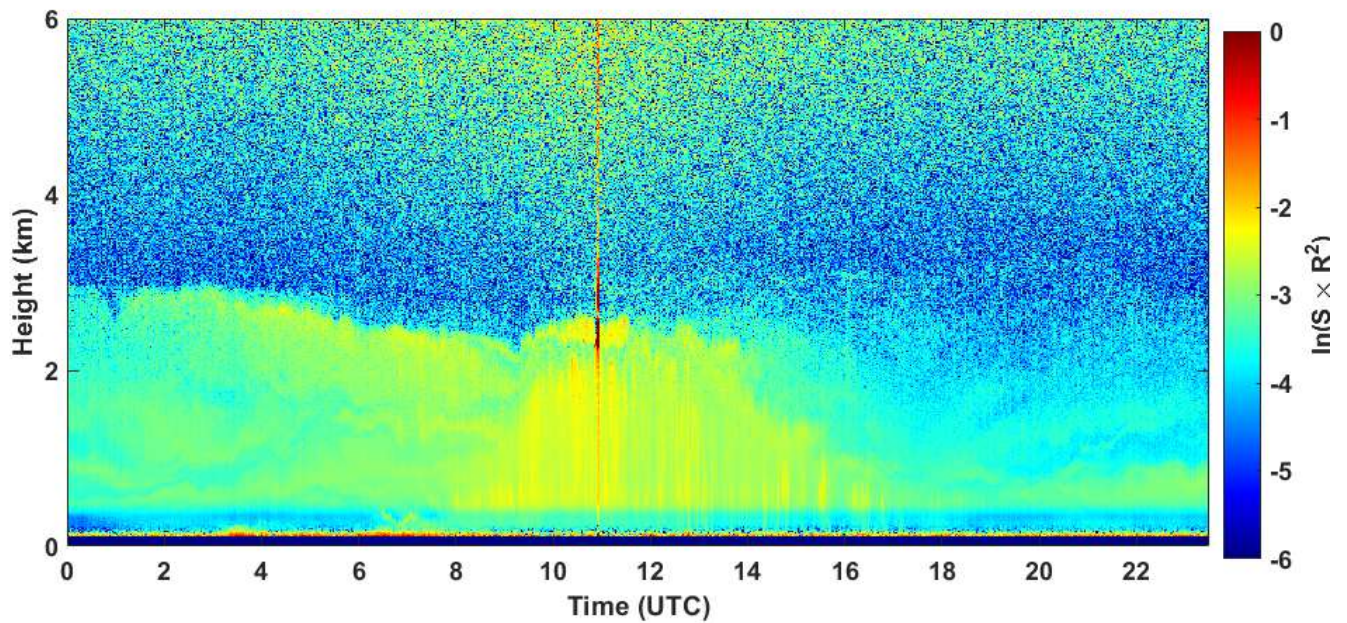
2020-09-10 RCS quick look CHM15k - ILVA LIDAR1 DIREZIONE
