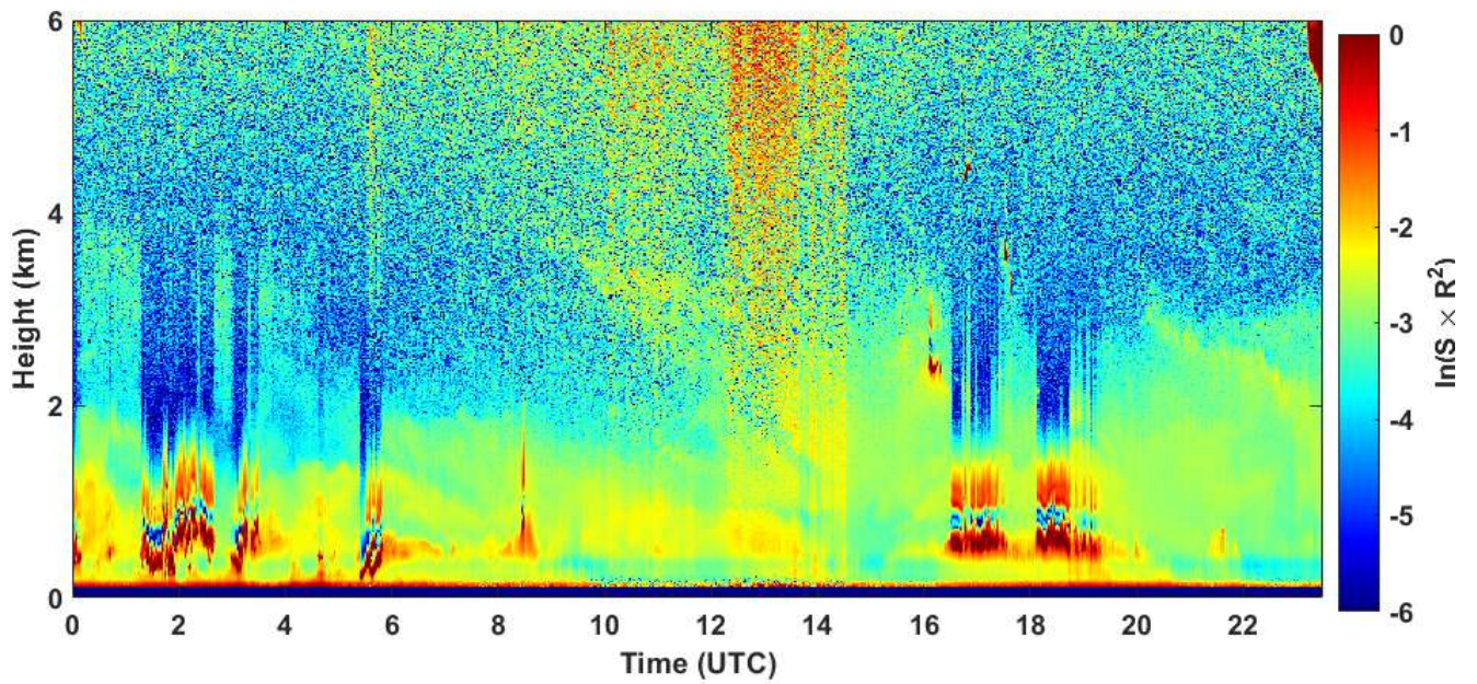
2020-09-22 RCS quick look CHM15k - ILVA LIDAR1 DIREZIONE
