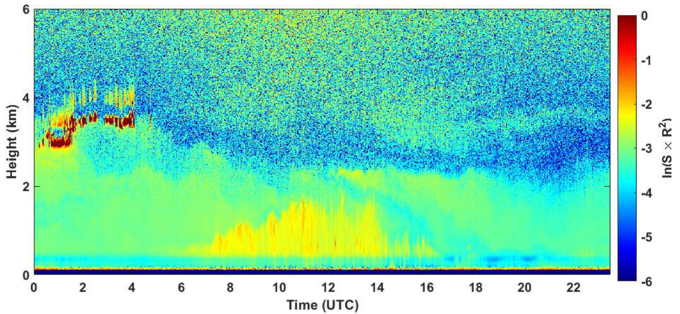
2020-09-14 RCS quick look CHM15k - ILVA LIDAR1 DIREZIONE
