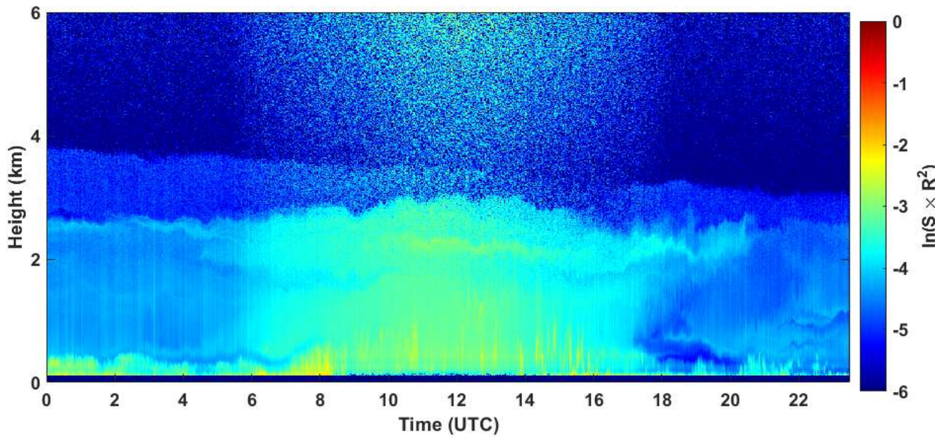
2020-09-10 RCS quick look CHM15k - ILVA LIDAR3 AGGLOMERATO
