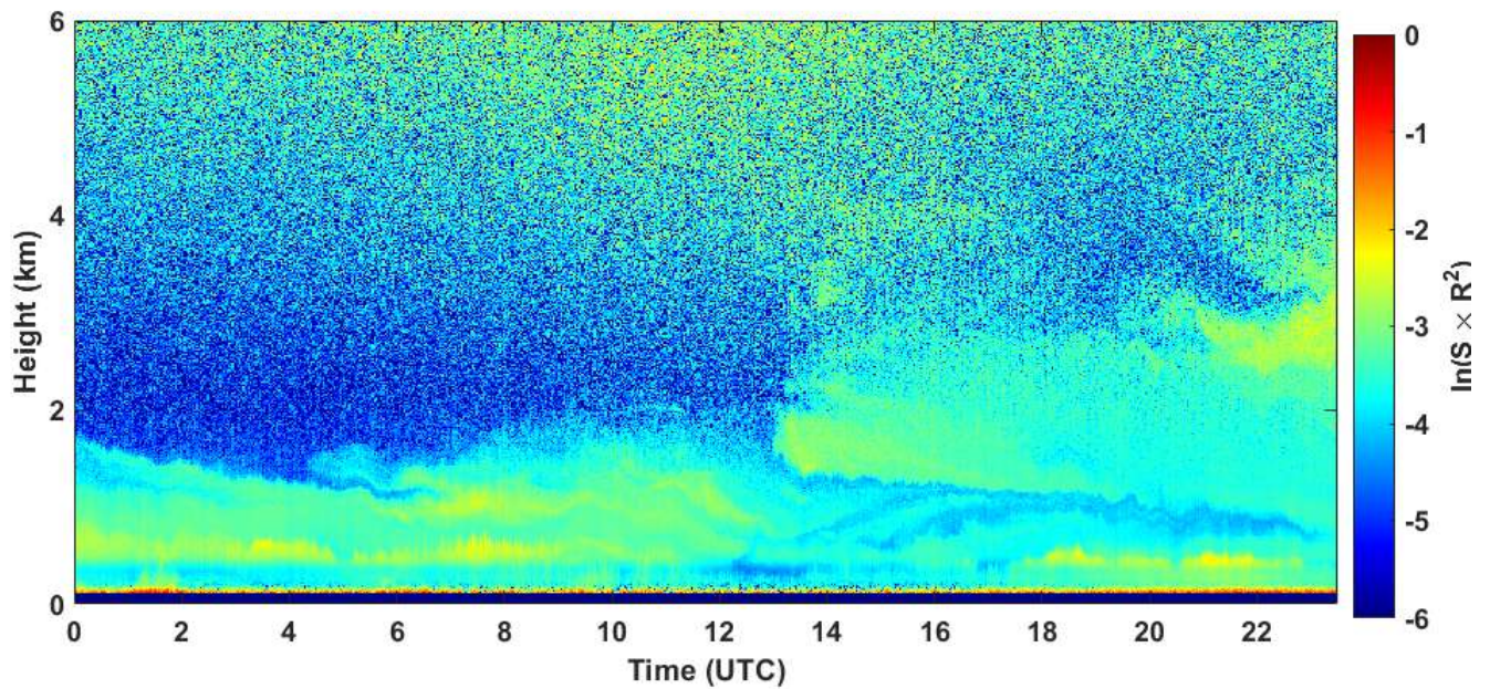
2020-09-06 RCS quick look CHM15k - ILVA LIDAR1 DIREZIONE
