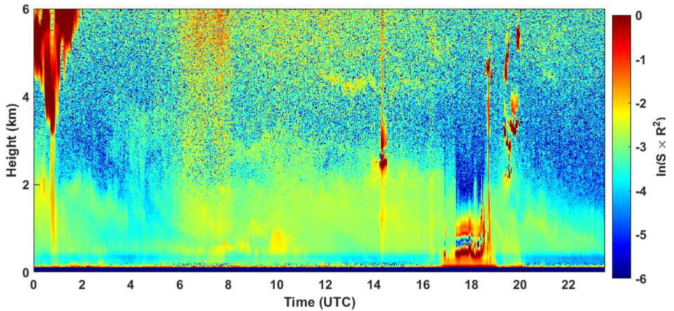
2020-09-24 RCS quick look CHM15k - ILVA LIDAR1 DIREZIONE
