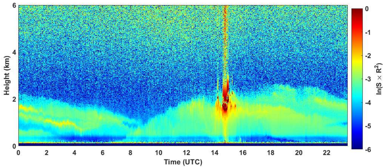
2020-09-30 RCS quick look CHM15k - ILVA LIDAR1 DIREZIONE
