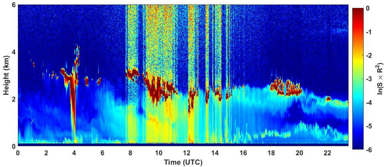
2020-09-30 RCS quick look CHM15k - ILVA LIDAR3 AGGLOMERATO
