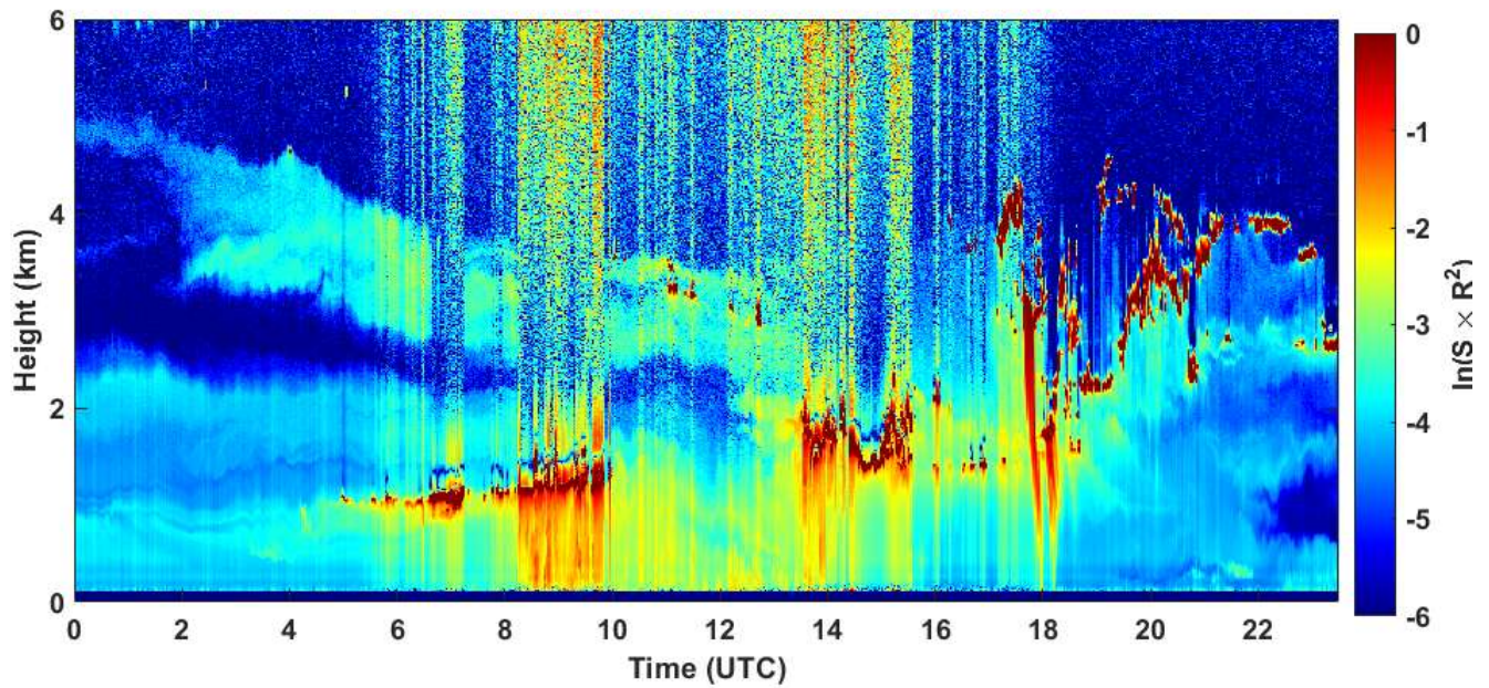
2020-09-04 RCS quick look CHM15k - ILVA LIDAR3 AGGLOMERATO
