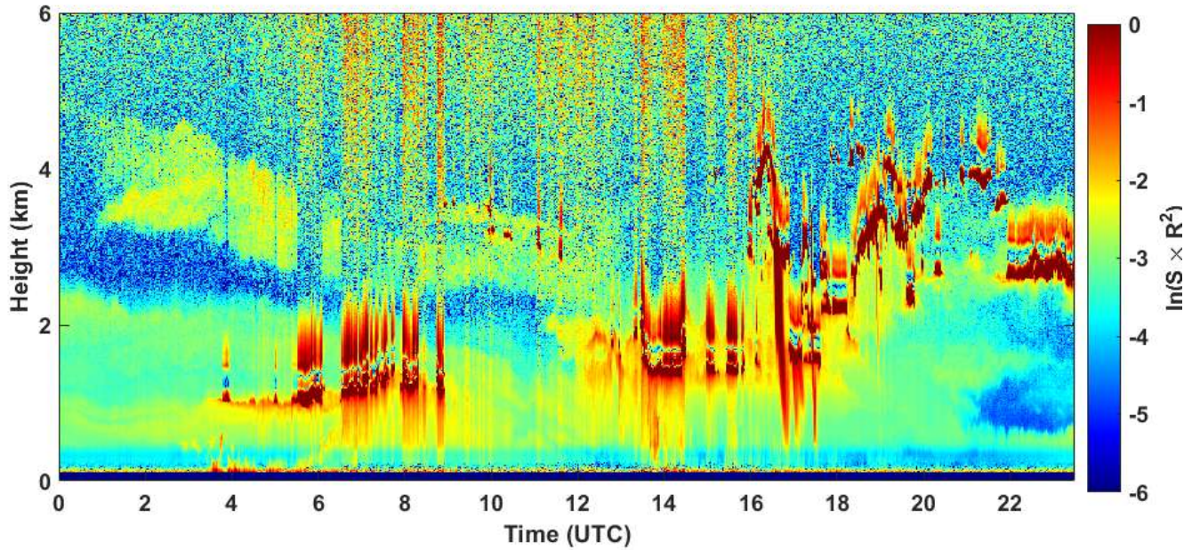
2020-09-04 RCS quick look CHM15k - ILVA LIDAR1 DIREZIONE
