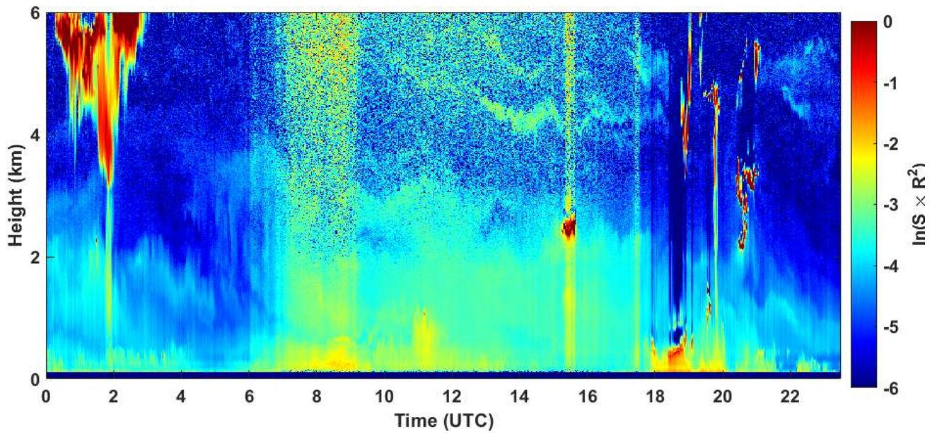
2020-09-24 RCS quick look CHM15k - ILVA LIDAR3 AGGLOMERATO
