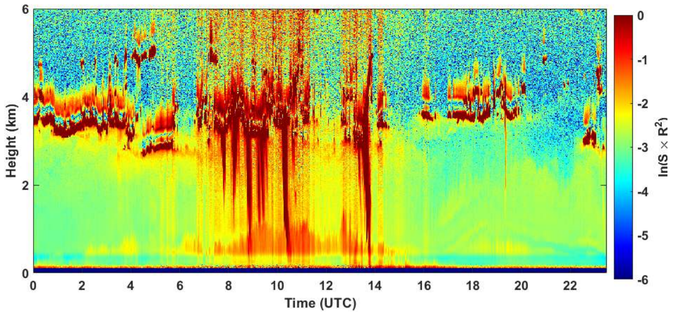
2020-09-18 RCS quick look CHM15k - ILVA LIDAR1 DIREZIONE
