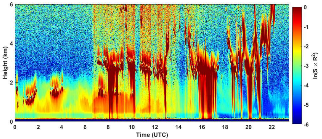
2020-09-28 RCS quick look CHM15k - ILVA LIDAR1 DIREZIONE
