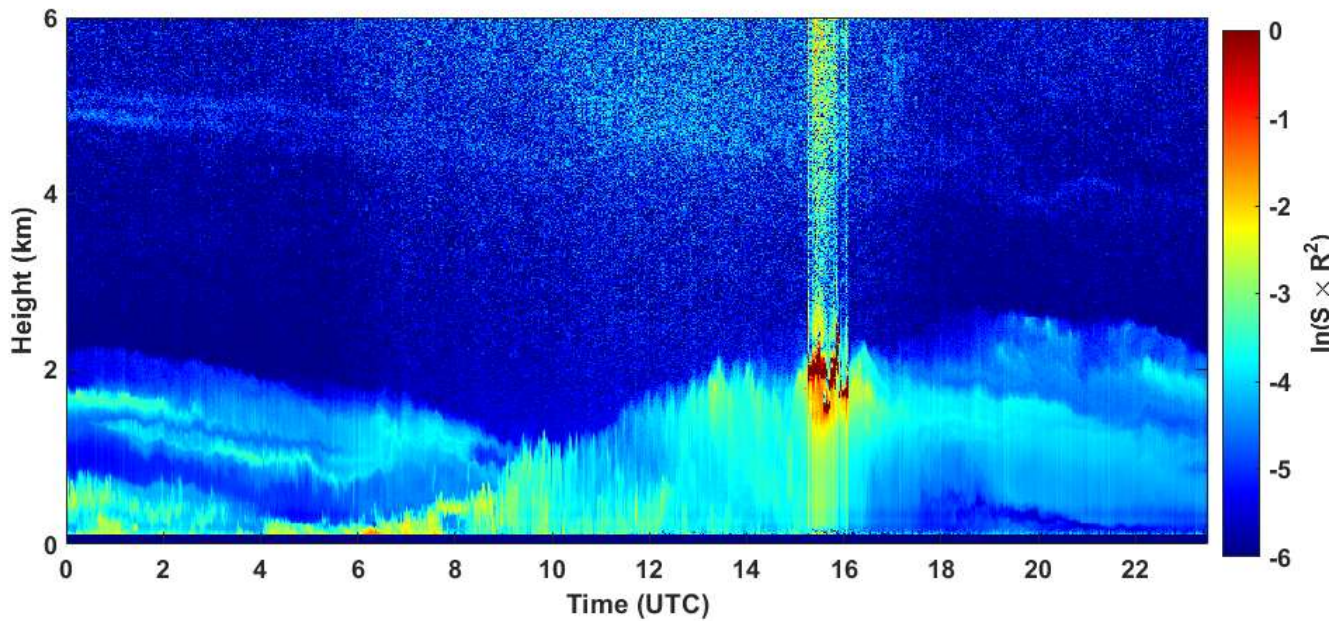
2020-09-30 RCS quick look CHM15k - ILVA LIDAR3 AGGLOMERATO
