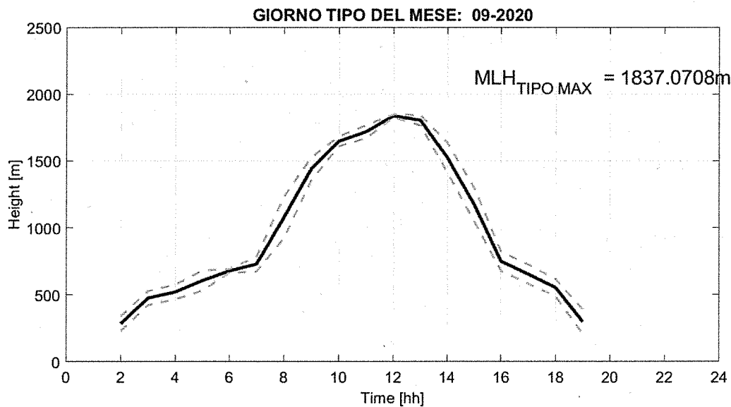
Fig. 2: Giorno tipo del parametro Mixing Layer Height nel mese di SETTEMBRE 2020, rappresentato mediante media oraria (linea blu continua) e deviazione standard (linee celesti tratteggiate).
