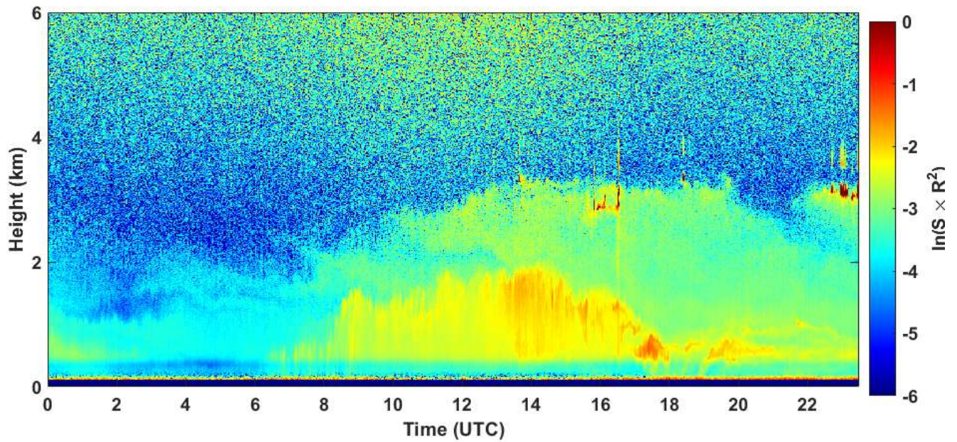
2020-09-12 RCS quick look CHM15k - ILVA LIDAR1 DIREZIONE
