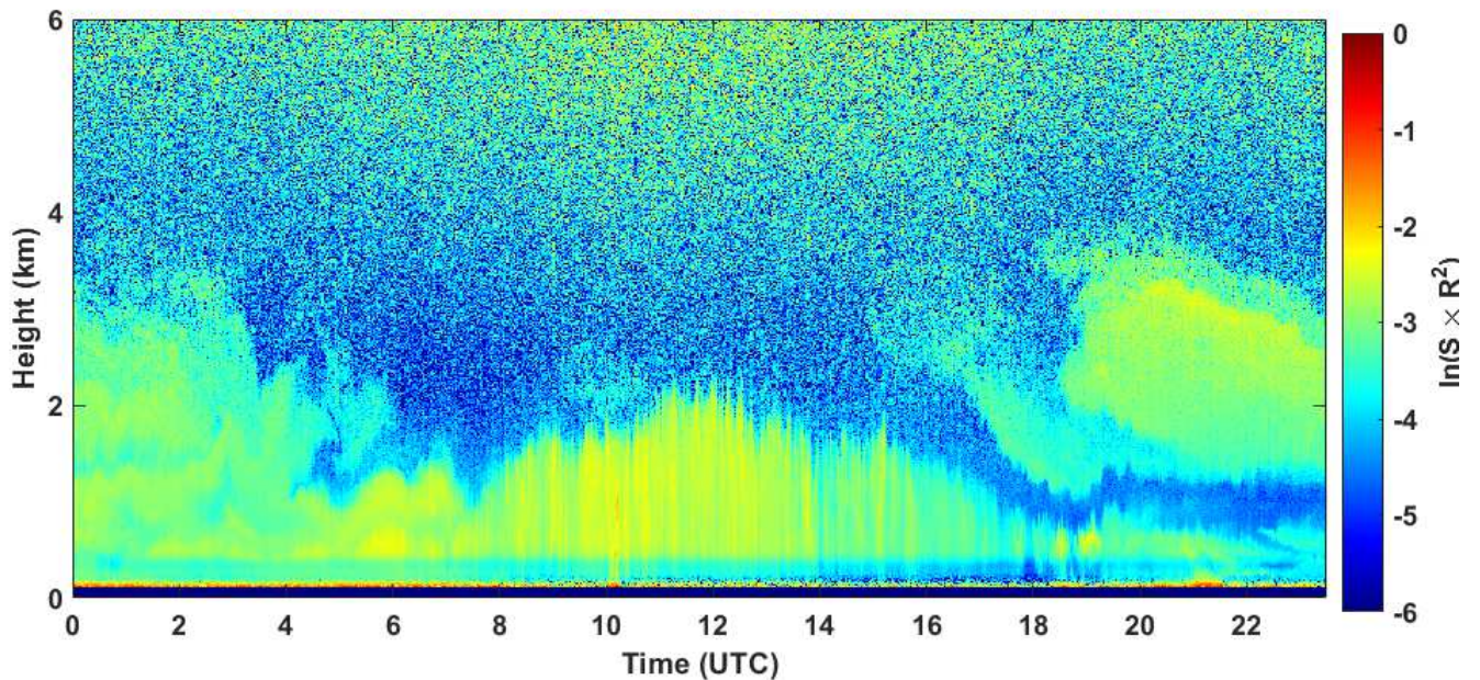
2020-08-02 RCS quick look CHM15k - ILVA LIDAR1 DIREZIONE
