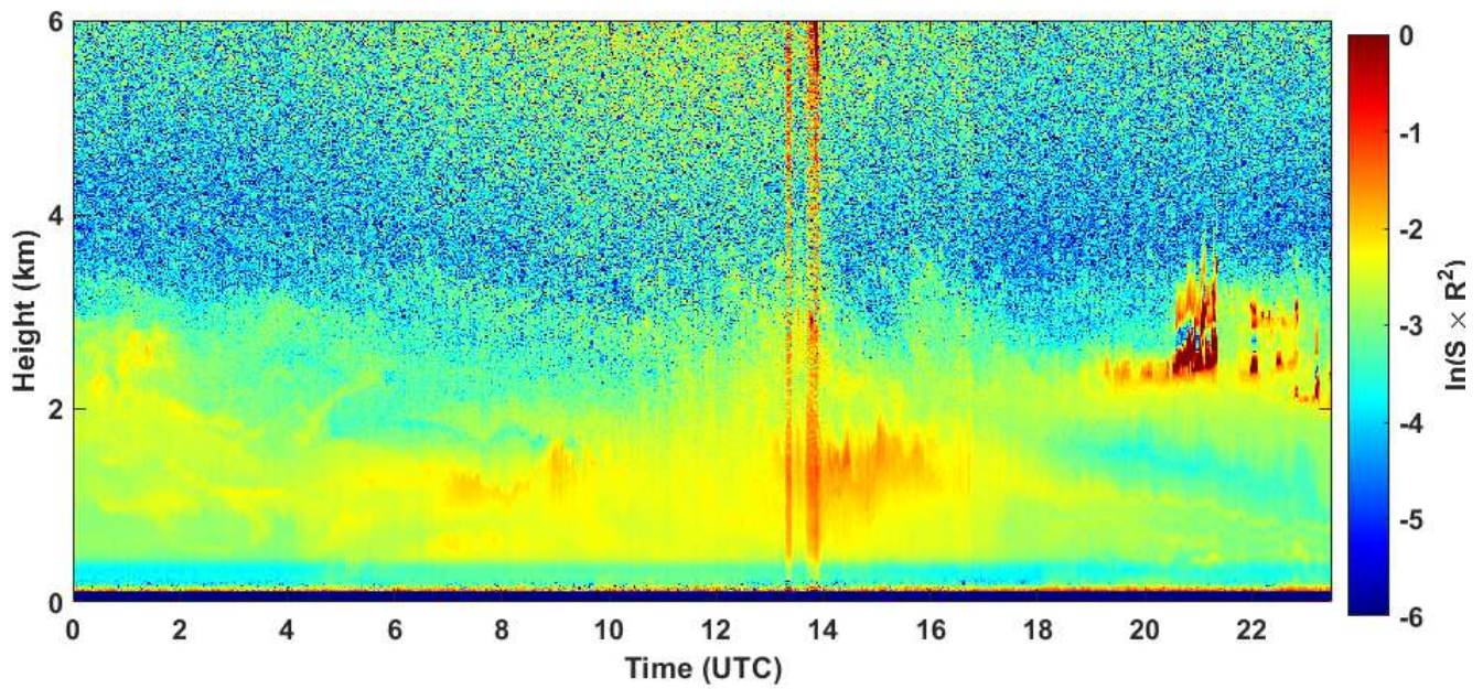
2020-08-16 RCS quick look CHM15k - ILVA LIDAR1 DIREZIONE
