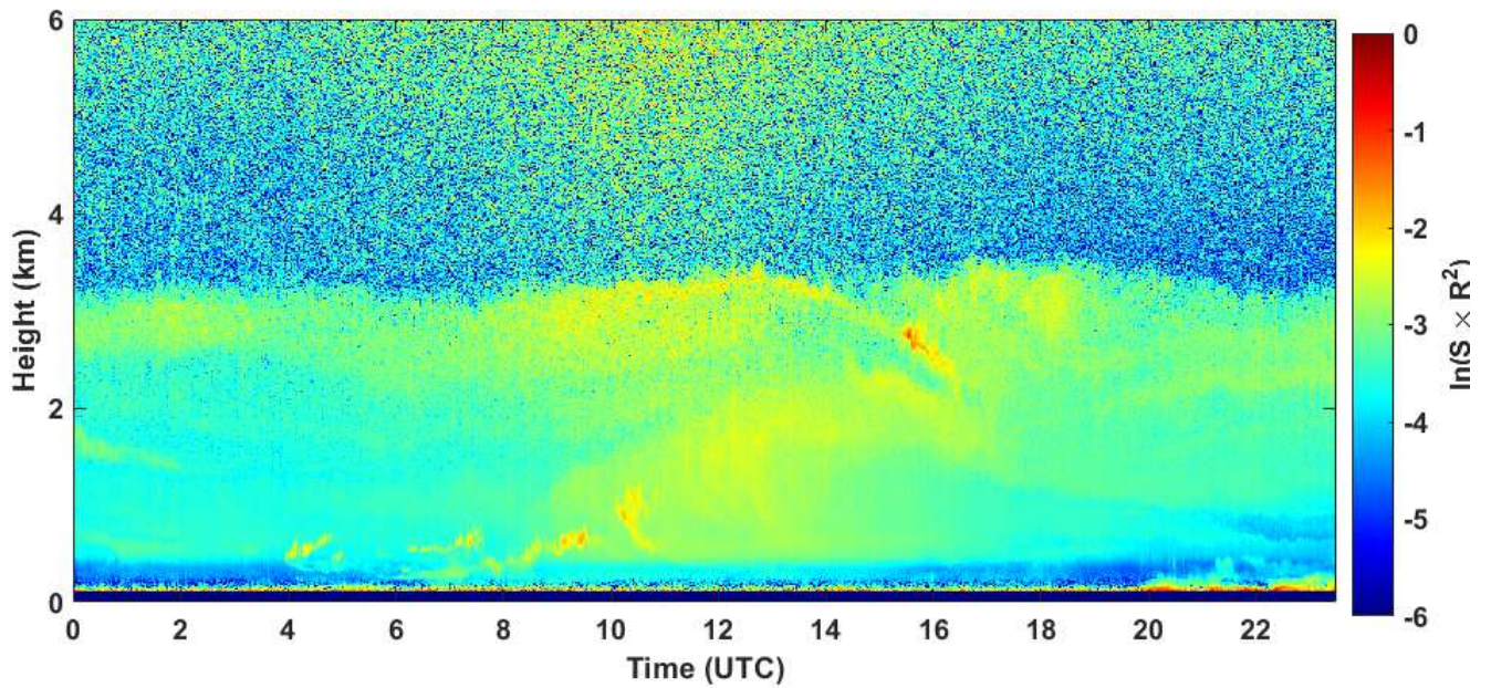
2020-08-24 RCS quick look CHM15k - ILVA LIDAR1 DIREZIONE
