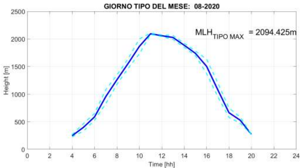
Fig. 2: Giorno tipo del parametro Mixing Layer Height nel mese di AGOSTO 2020, rappresentato mediante media oraria (linea blu continua) e deviazione standard (linee celesti tratteggiate).
