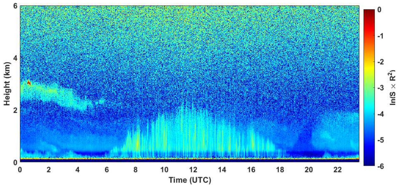
2020-08-20 RCS quick look CHM15k - ILVA LIDAR1 DIREZIONE
