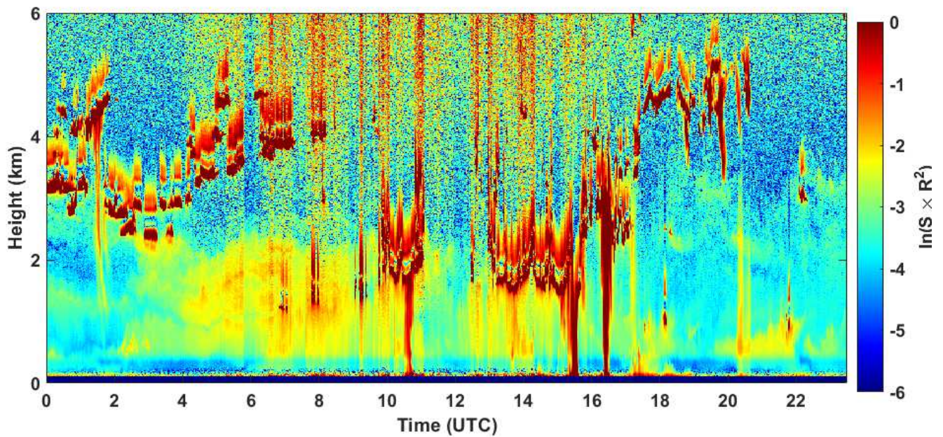
2020-08-06 RCS quick look CHM15k - ILVA LIDAR1 DIREZIONE
