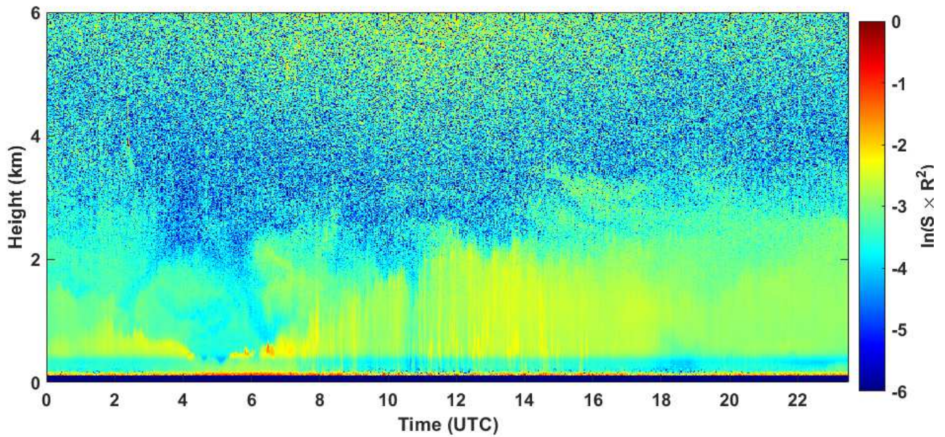
2020-08-10 RCS quick look CHM15k - ILVA LIDAR1 DIREZIONE
