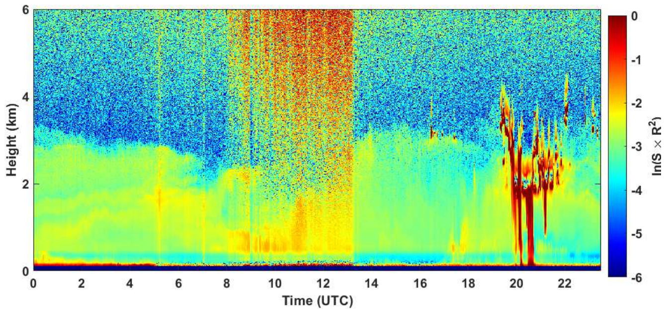
2020-08-18 RCS quick look CHM15k - ILVA LIDAR1 DIREZIONE
