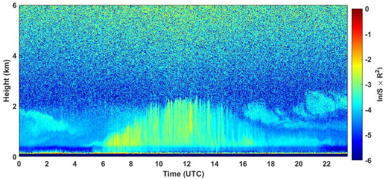
2020-08-22 RCS quick look CHM15k - ILVA LIDAR1 DIREZIONE
