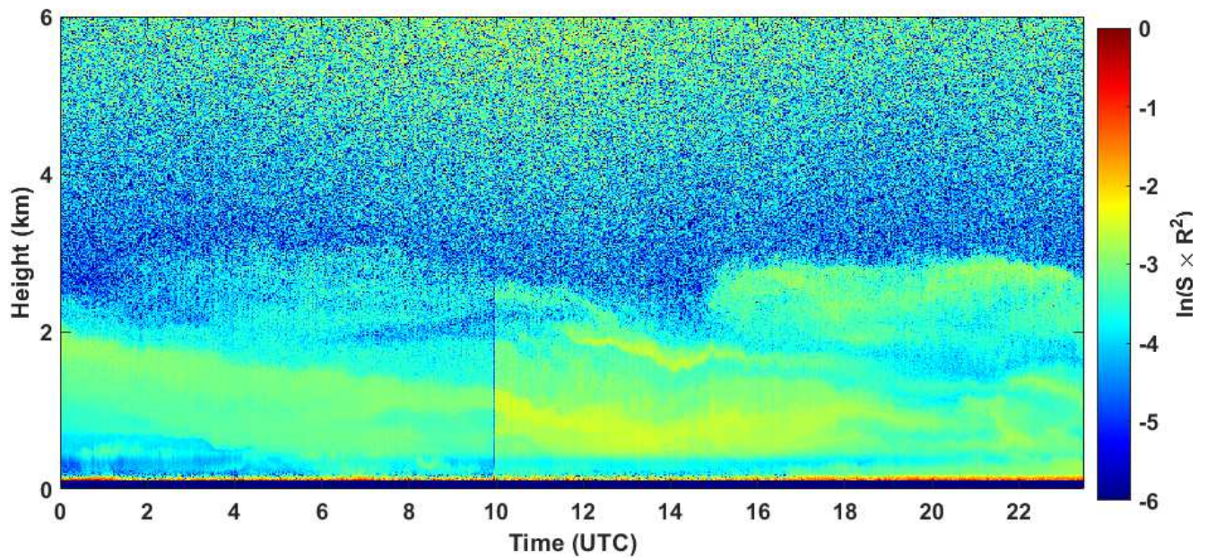
2020-08-28 RCS quick look CHM15k - ILVA LIDAR1 DIREZIONE
