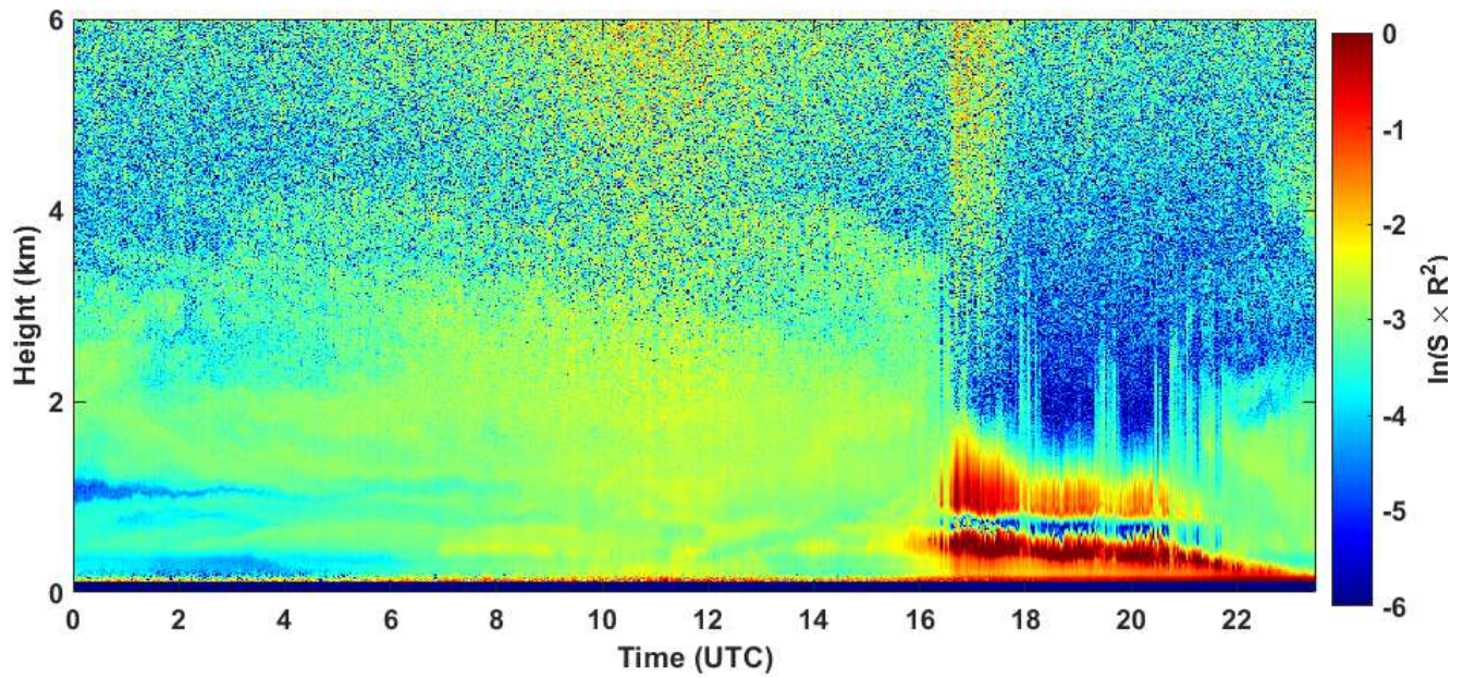
2020-08-04 RCS quick look CHM15k - ILVA LIDAR1 DIREZIONE
