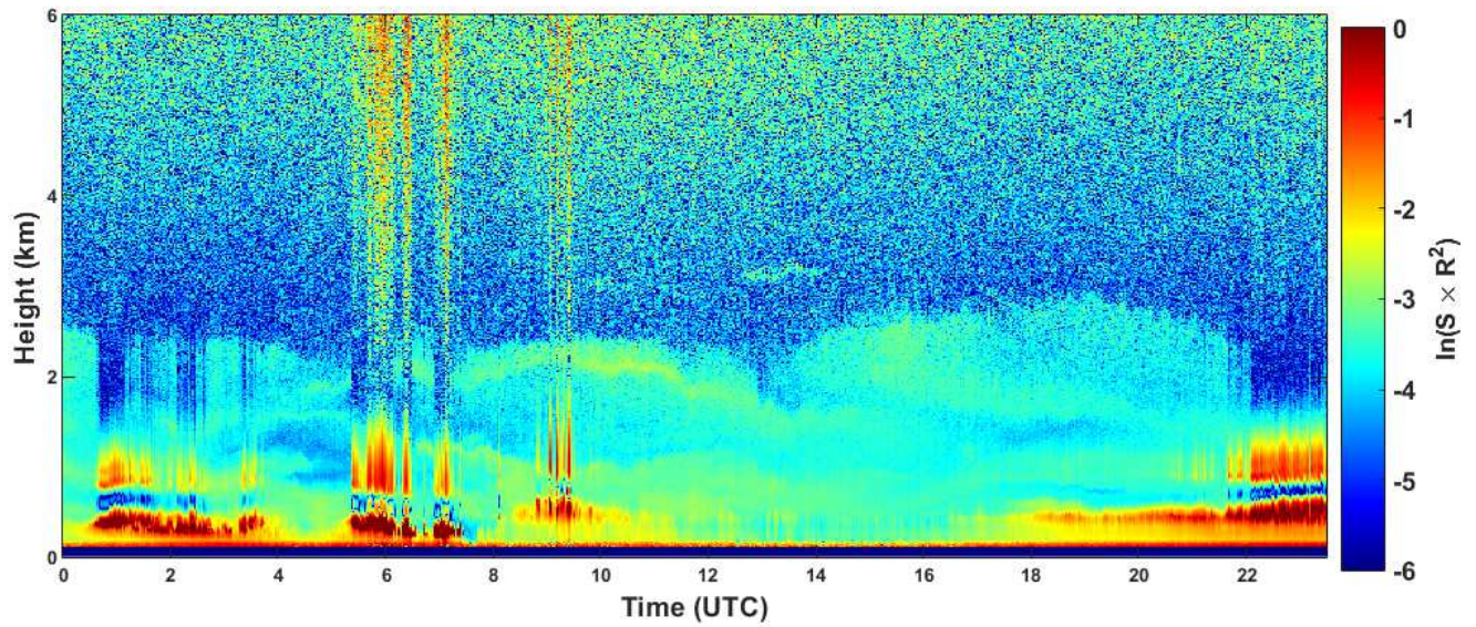
2020-08-30 RCS quick look CHM15k - ILVA LIDAR1 DIREZIONE
