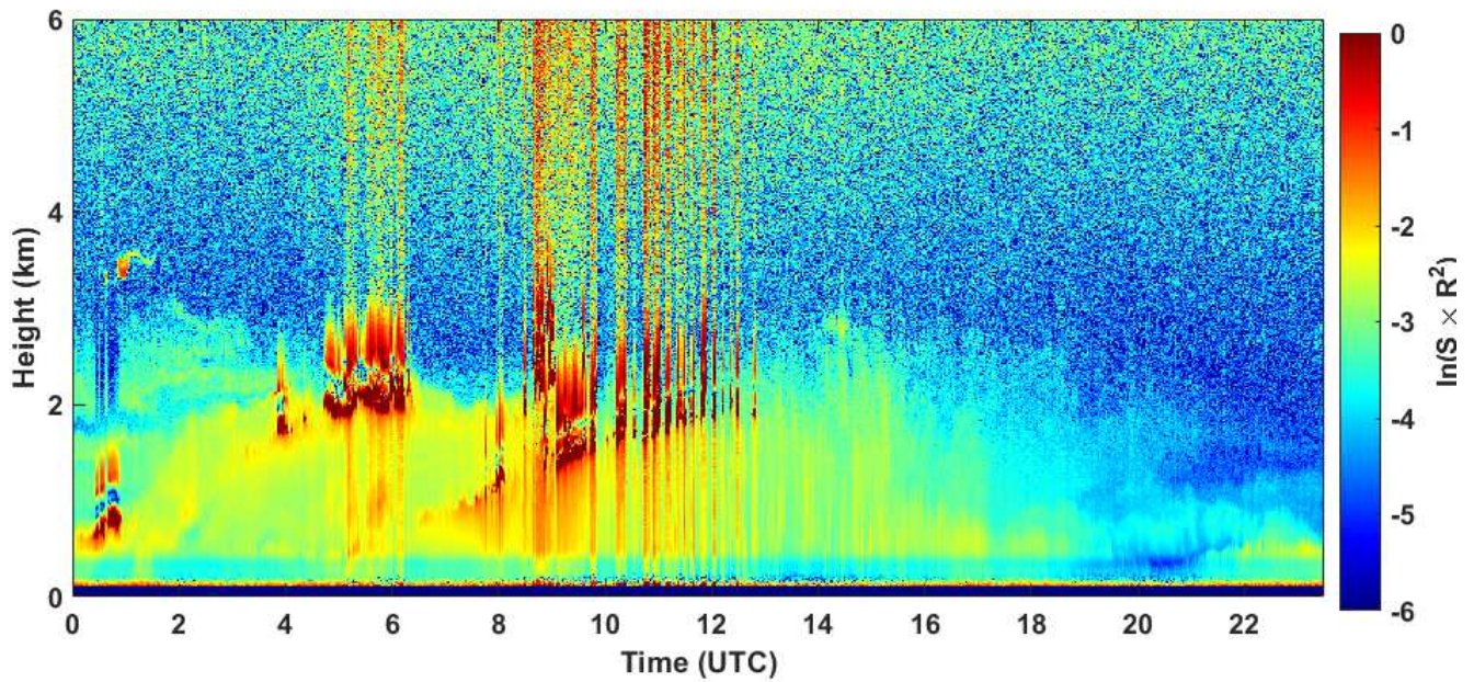
2020-08-26 RCS quick look CHM15k - ILVA LIDAR1 DIREZIONE
