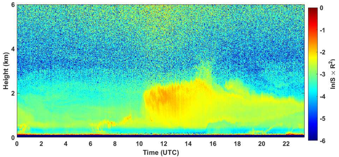
2020-08-12 RCS quick look CHM15k - ILVA LIDAR1 DIREZIONE
