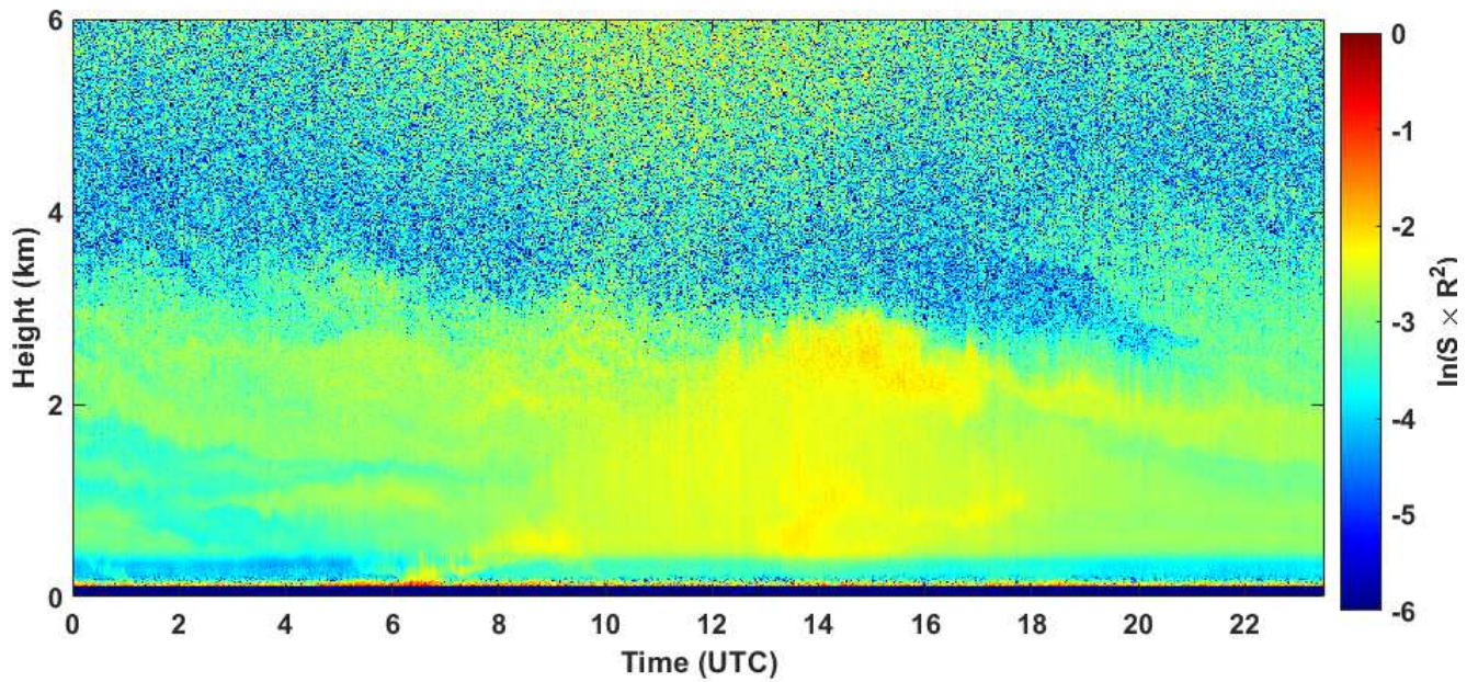
2020-08-14 RCS quick look CHM15k - ILVA LIDAR1 DIREZIONE
