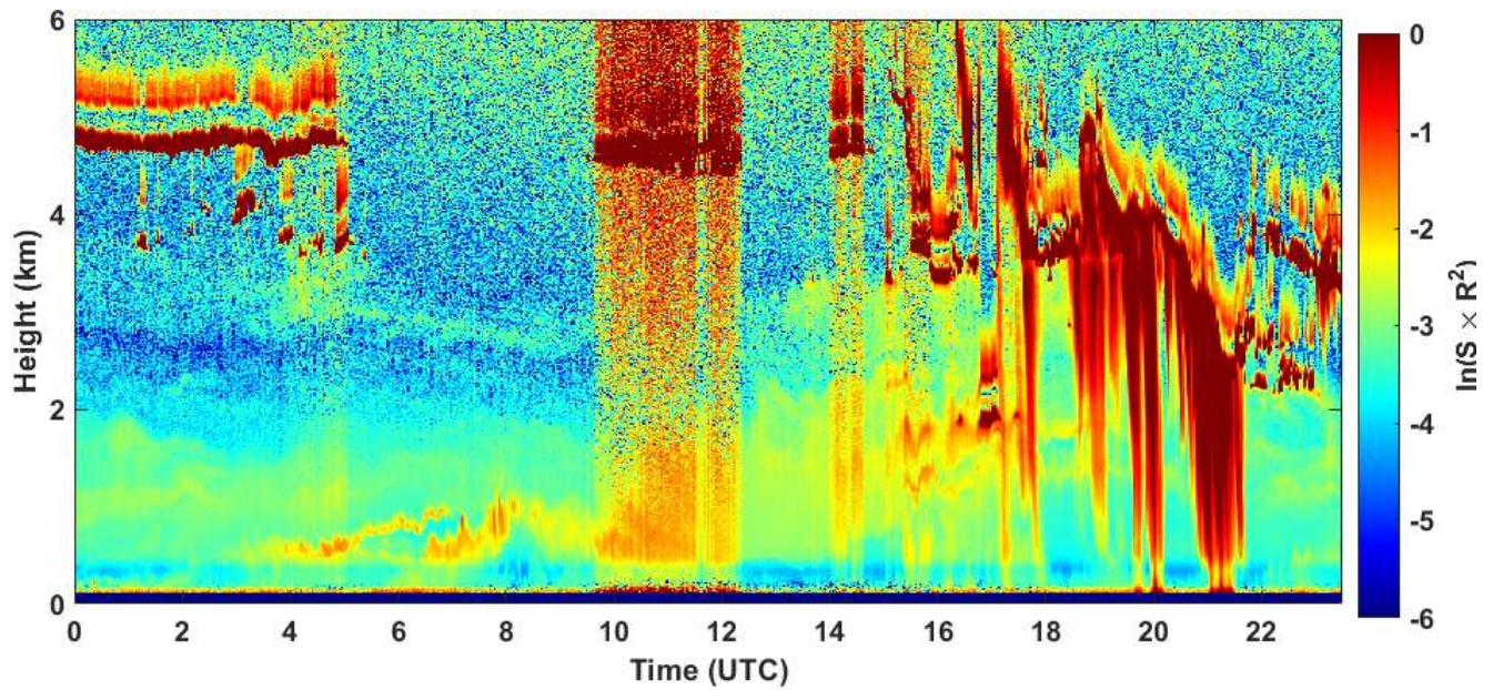
2020-07-18 RCS quick look CHM15k - ILVA LIDAR1 DIREZIONE
