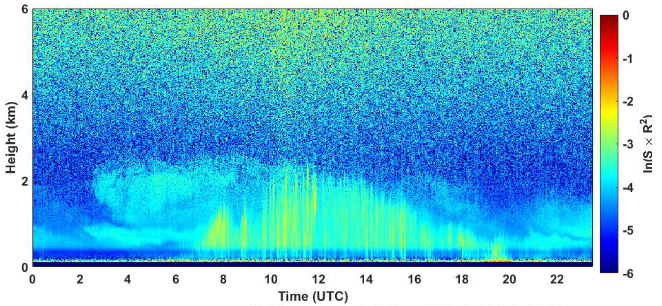
2020-07-22 RCS quick look CHM15k - ILVA LIDAR1 DIREZIONE
