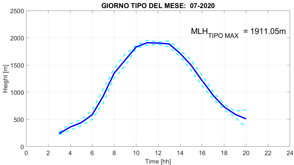
Fig. 2: Giorno tipo del parametro Mixing Layer Height nel mese di LUGLIO 2020, rappresentato mediante media oraria (linea blu continua) e deviazione standard (linee celesti tratteggiate).
