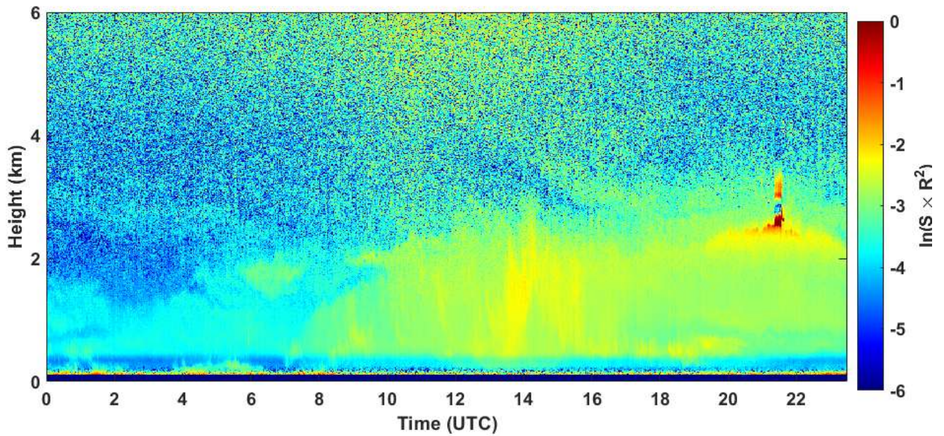
2020-07-24 RCS quick look CHM15k - ILVA LIDAR1 DIREZIONE
