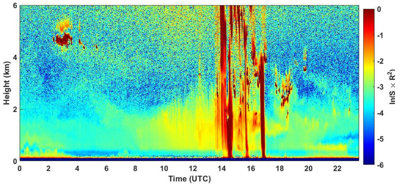
2020-07-26 RCS quick look CHM15k - ILVA LIDAR1 DIREZIONE
