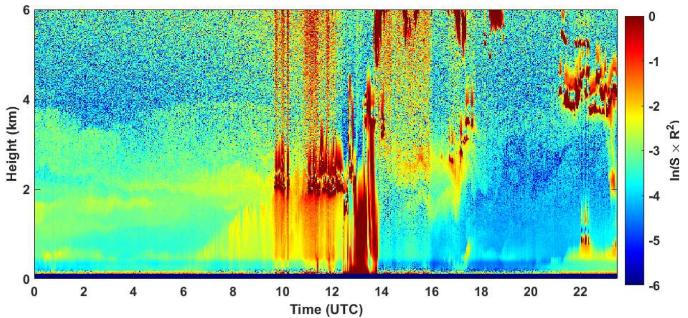
2020-07-04 RCS quick look CHM15k - ILVA LIDAR1 DIREZIONE
