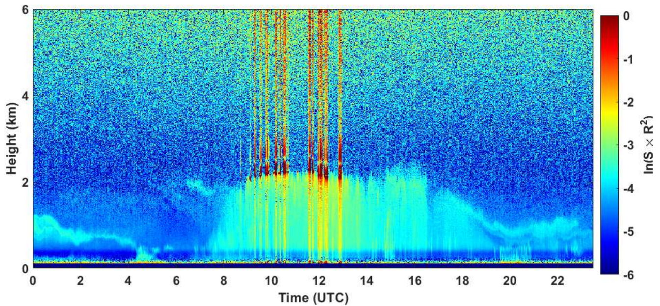
2020-07-20 RCS quick look CHM15k - ILVA LIDAR1 DIREZIONE
