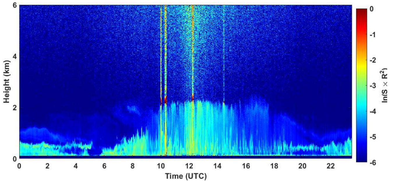
2020-07-20 RCS quick look CHM15k - ILVA LIDAR3 AGGLOMERATO
