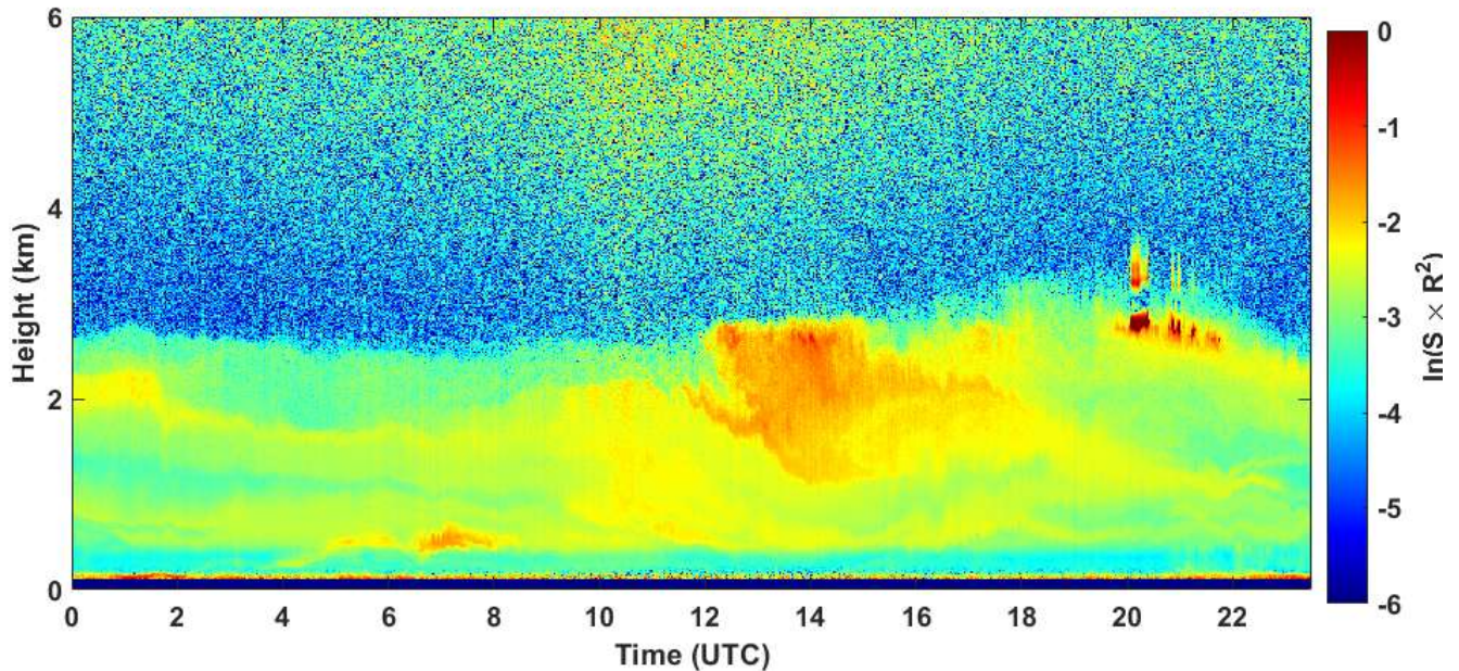
2020-07-02 RCS quick look CHM15k - ILVA LIDAR1 DIREZIONE
