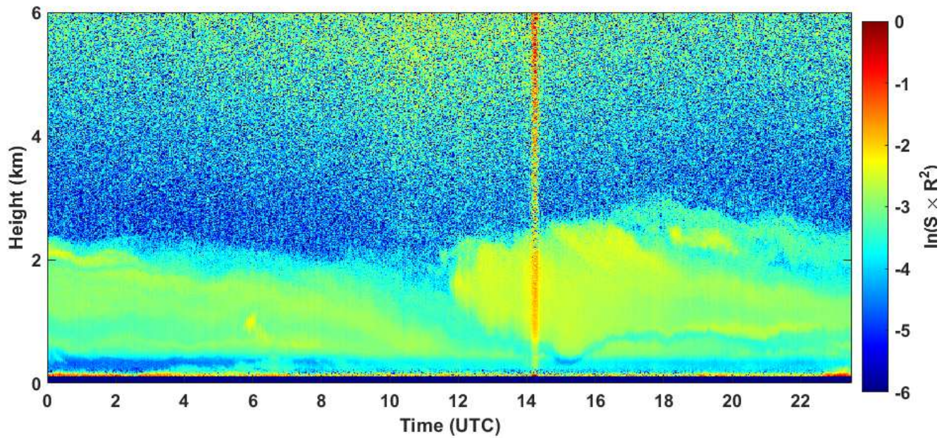
2020-07-12 RCS quick look CHM15k - ILVA LIDAR1 DIREZIONE
