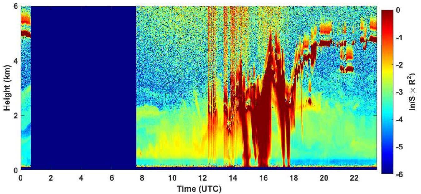
2020-07-16 RCS quick look CHM15k - ILVA LIDAR1 DIREZIONE
