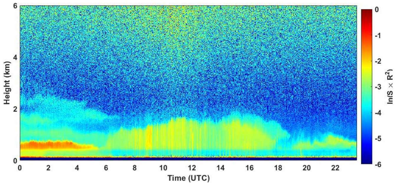
2020-07-08 RCS quick look CHM15k - ILVA LIDAR1 DIREZIONE
