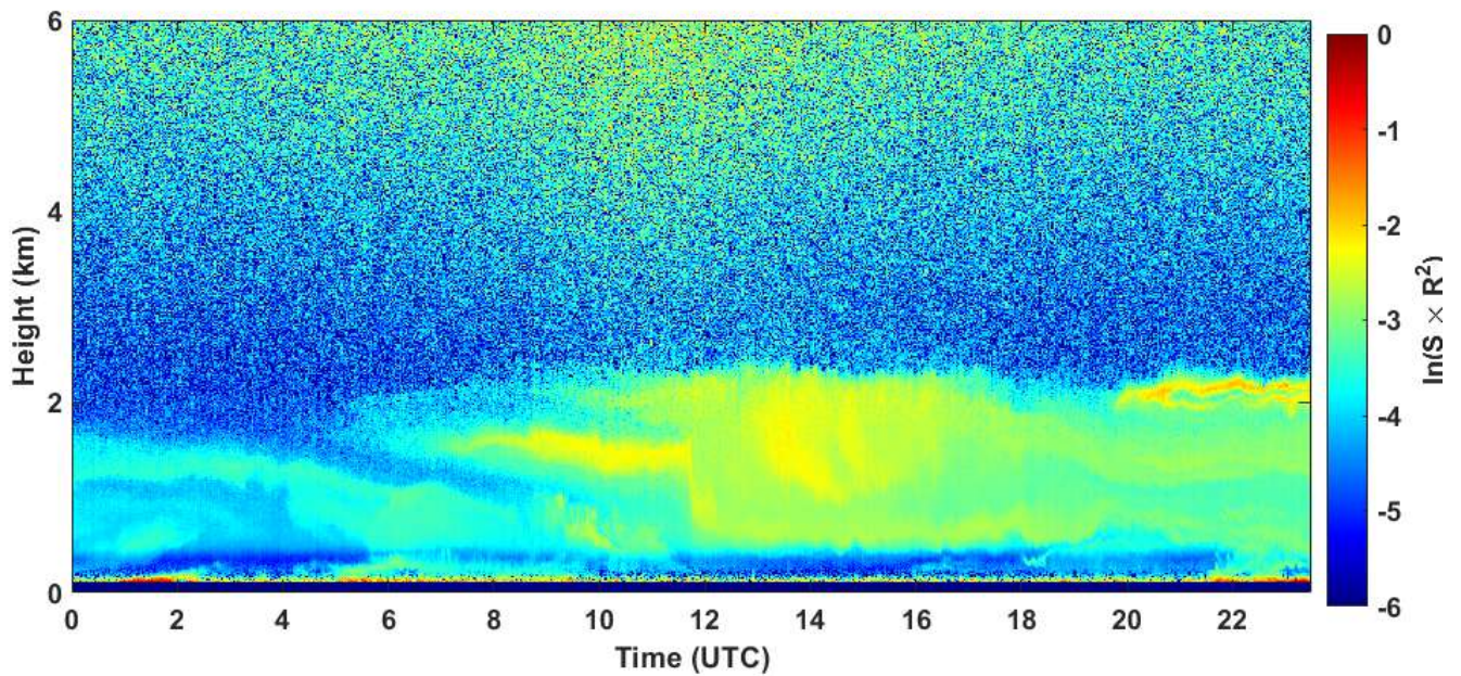
2020-07-10 RCS quick look CHM15k - ILVA LIDAR1 DIREZIONE
