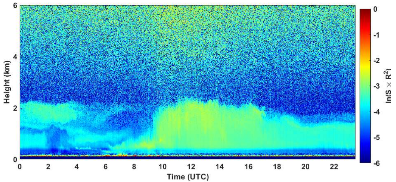
2020-07-30 RCS quick look CHM15k - ILVA LIDAR1 DIREZIONE
