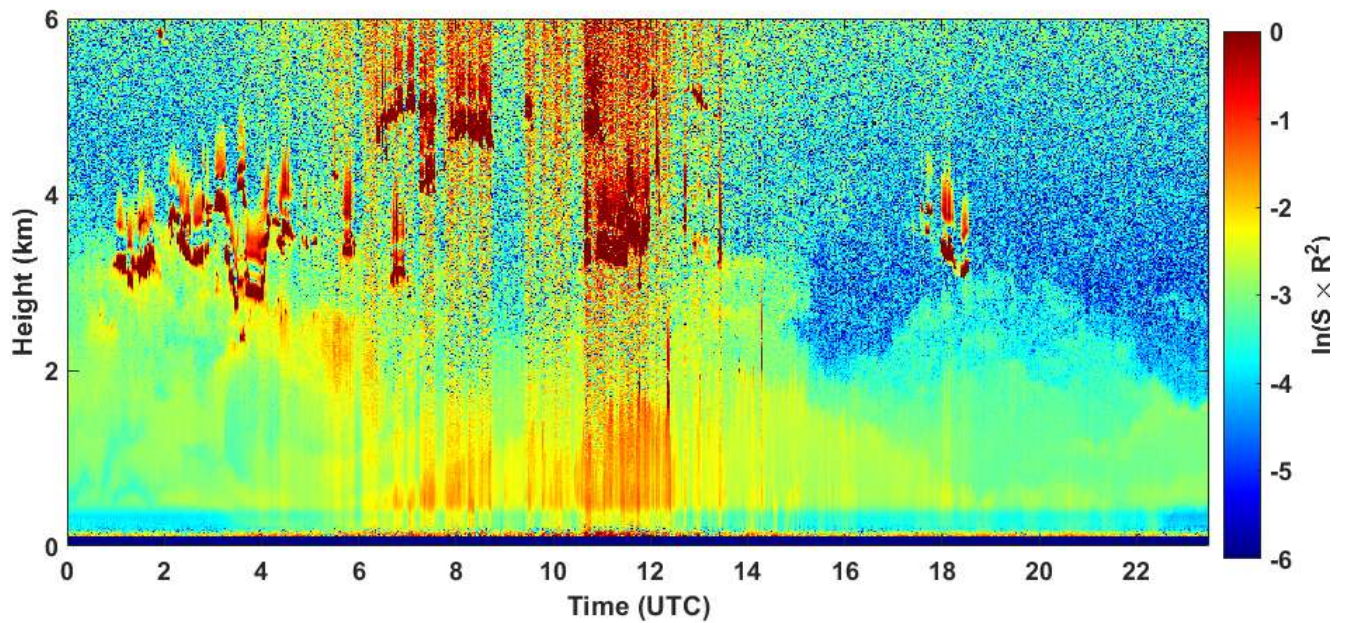
2020-07-06 RCS quick look CHM15k - ILVA LIDAR1 DIREZIONE
