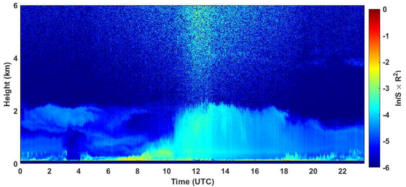
2020-07-30 RCS quick look CHM15k - ILVA LIDAR3 AGGLOMERATO
