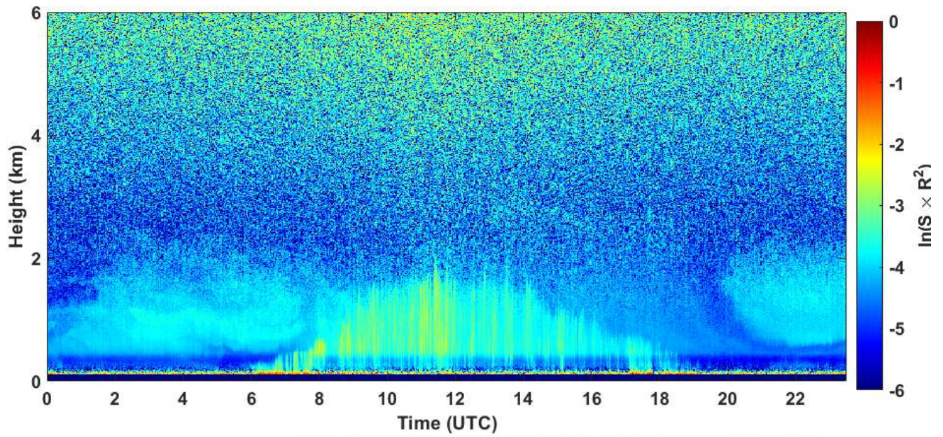
2020-07-28 RCS quick look CHM15k - ILVA LIDAR1 DIREZIONE
