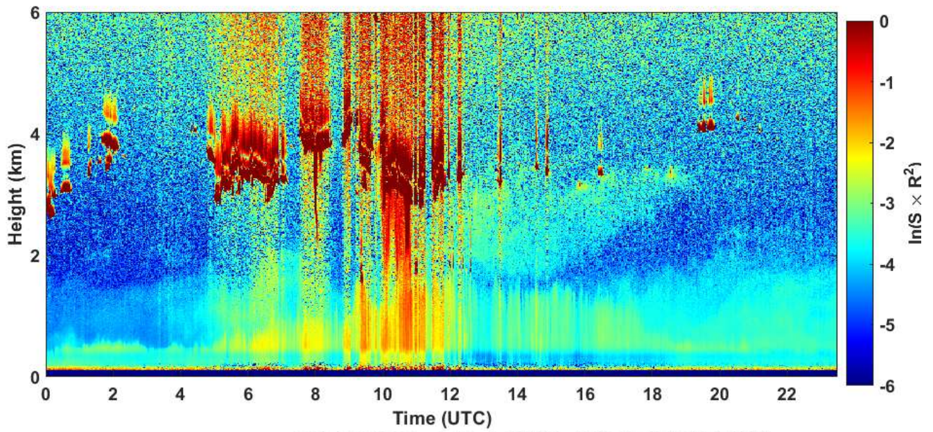
2020-06-24 RCS quick look CHM15k - ILVA LIDAR1 DIREZIONE
