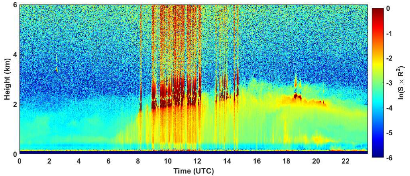
2020-06-24 RCS quick look CHM15k - ILVA LIDAR1 DIREZIONE
