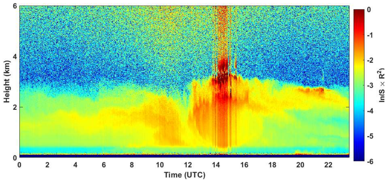
2020-06-30 RCS quick look CHM15k - ILVA LIDAR1 DIREZIONE
