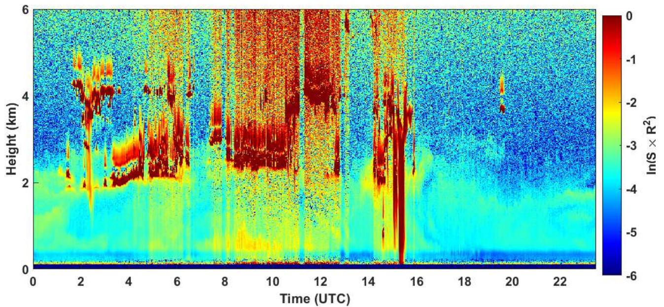
2020-06-10 RCS quick look CHM15k - ILVA LIDAR1 DIREZIONE
