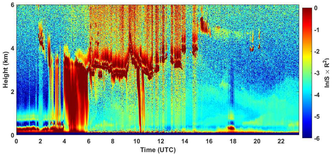
2020-06-08 RCS quick look CHM15k - ILVA LIDAR1 DIREZIONE
