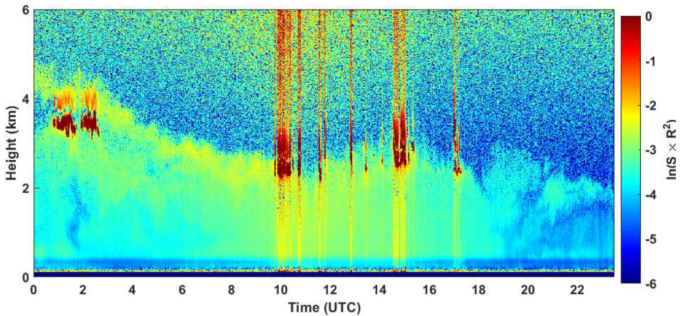
2020-06-14 RCS quick look CHM15k - ILVA LIDAR1 DIREZIONE
