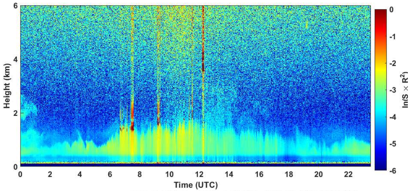
2020-06-22 RCS quick look CHM15k - ILVA LIDAR1 DIREZIONE
