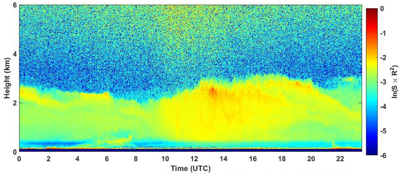
2020-06-30 RCS quick look CHM15k - ILVA LIDAR1 DIREZIONE
