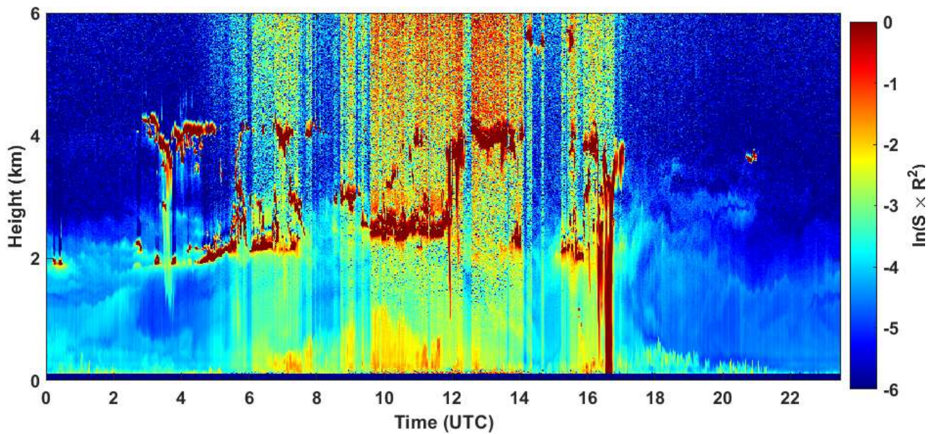
2020-06-10 RCS quick look CHM15k - ILVA LIDAR3 AGGLOMERATO
