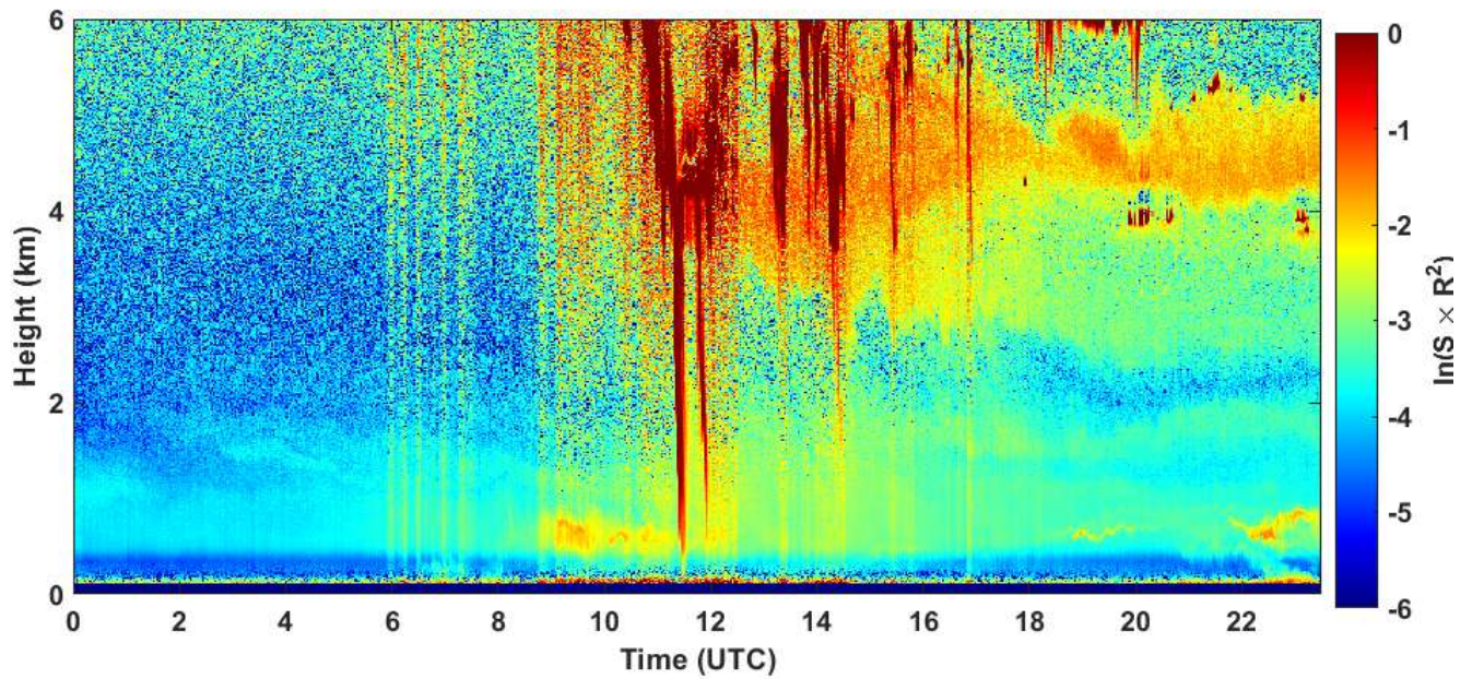
2020-06-20 RCS quick look CHM15k - ILVA LIDAR1 DIREZIONE
