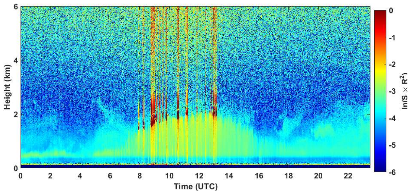
2020-06-02 RCS quick look CHM15k - ILVA LIDAR1 DIREZIONE
