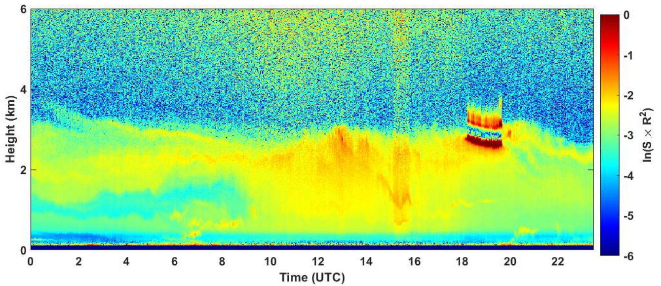
2020-06-28 RCS quick look CHM15k - ILVA LIDAR1 DIREZIONE
