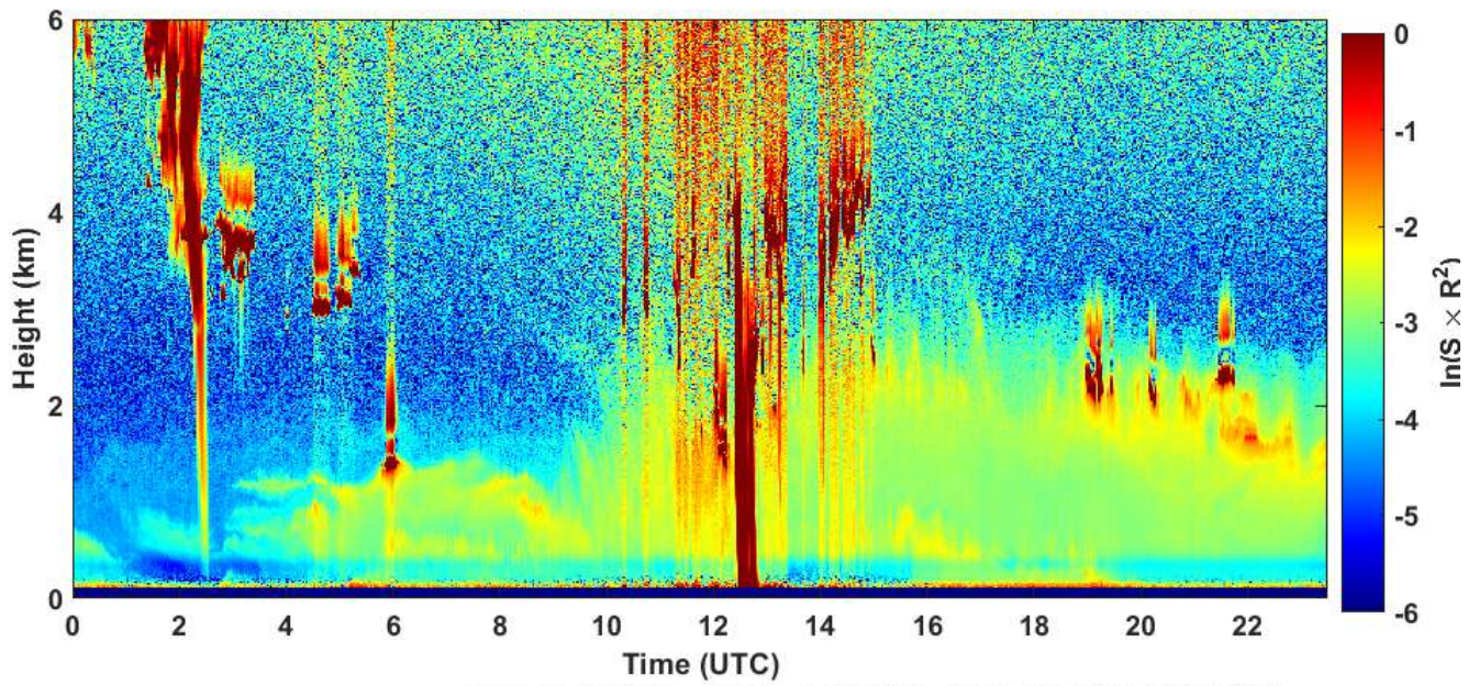
2020-06-18 RCS quick look CHM15k - ILVA LIDAR1 DIREZIONE
