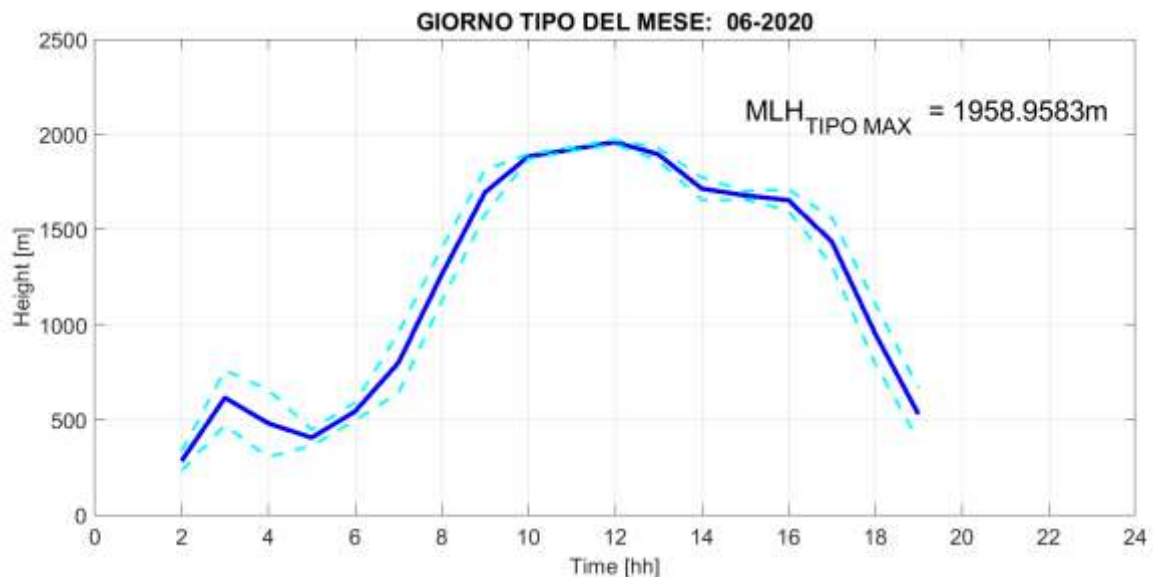
Fig. 2: Giorno tipo del parametro Mixing Layer Height nel mese di GIUGNO 2020, rappresentato mediante media oraria (linea blu continua) e deviazione standard (linee celesti tratteggiate).
