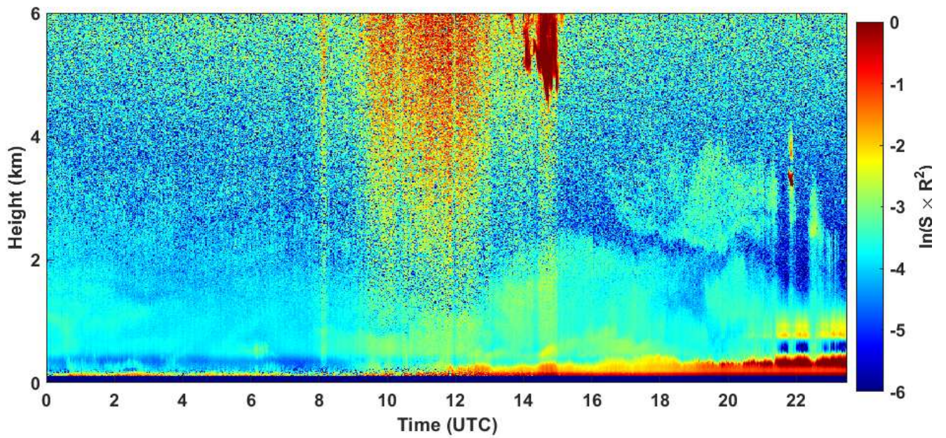
2020-06-04 RCS quick look CHM15k - ILVA LIDAR1 DIREZIONE
