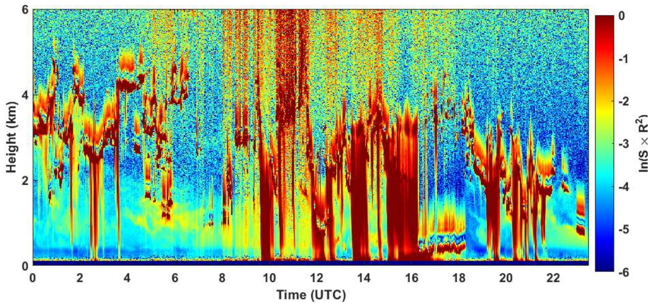
2020-06-16 RCS quick look CHM15k - ILVA LIDAR1 DIREZIONE
