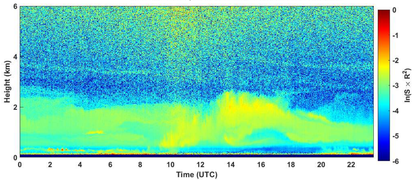
2020-06-26 RCS quick look CHM15k - ILVA LIDAR1 DIREZIONE
