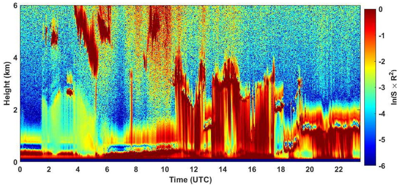
2020-06-06 RCS quick look CHM15k - ILVA LIDAR1 DIREZIONE
