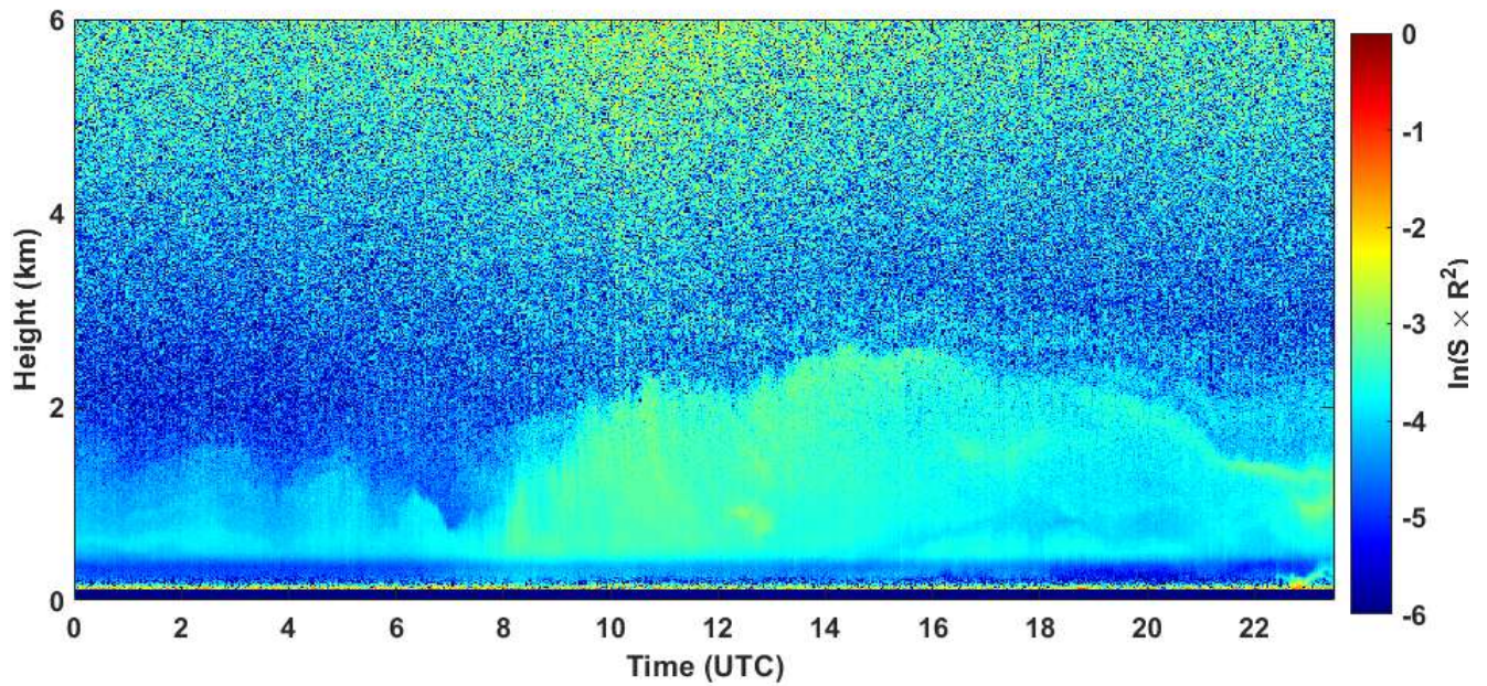
2020-05-24 RCS quick look CHM15k - ILVA LIDAR1 DIREZIONE
