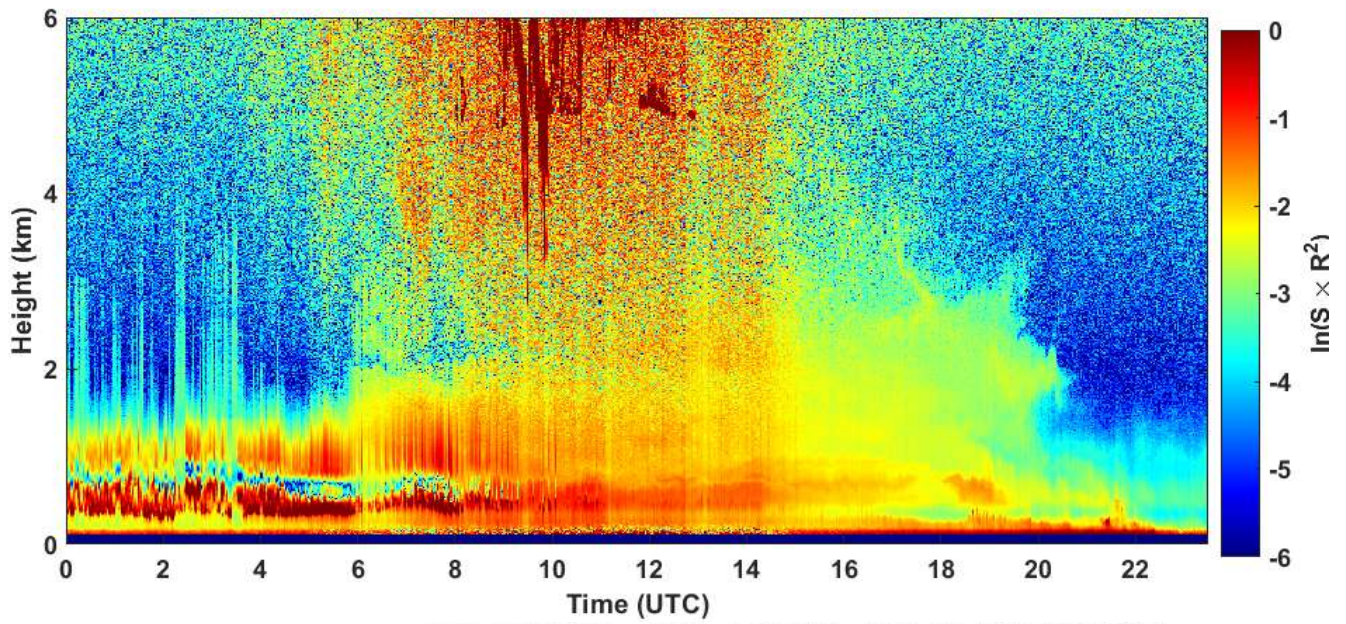
2020-05-12 RCS quick look CHM15k - ILVA LIDAR1 DIREZIONE
