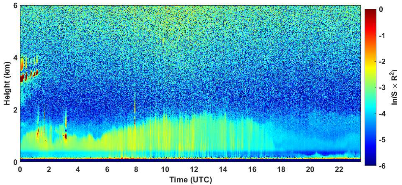
2020-05-08 RCS quick look CHM15k - ILVA LIDAR1 DIREZIONE
