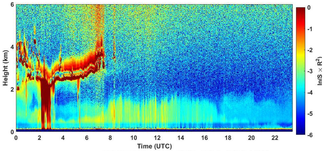
2020-05-26 RCS quick look CHM15k - ILVA LIDAR1 DIREZIONE
