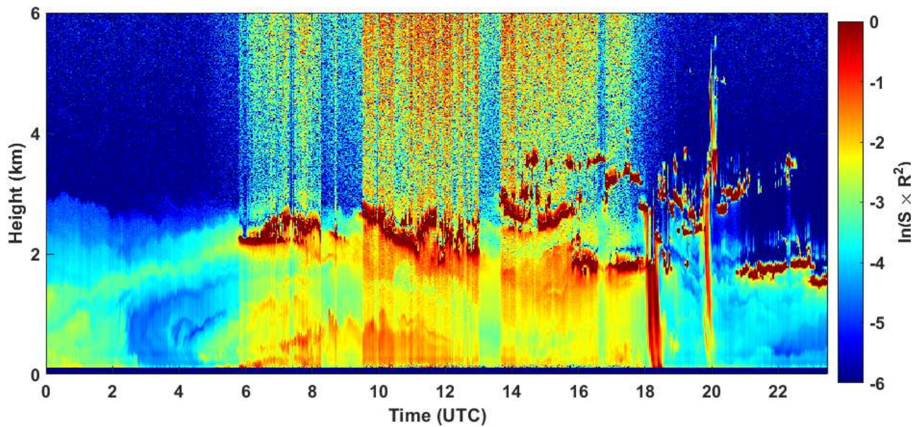
2020-05-20 RCS quick look CHM15k - ILVA LIDAR3 AGGLOMERATO
