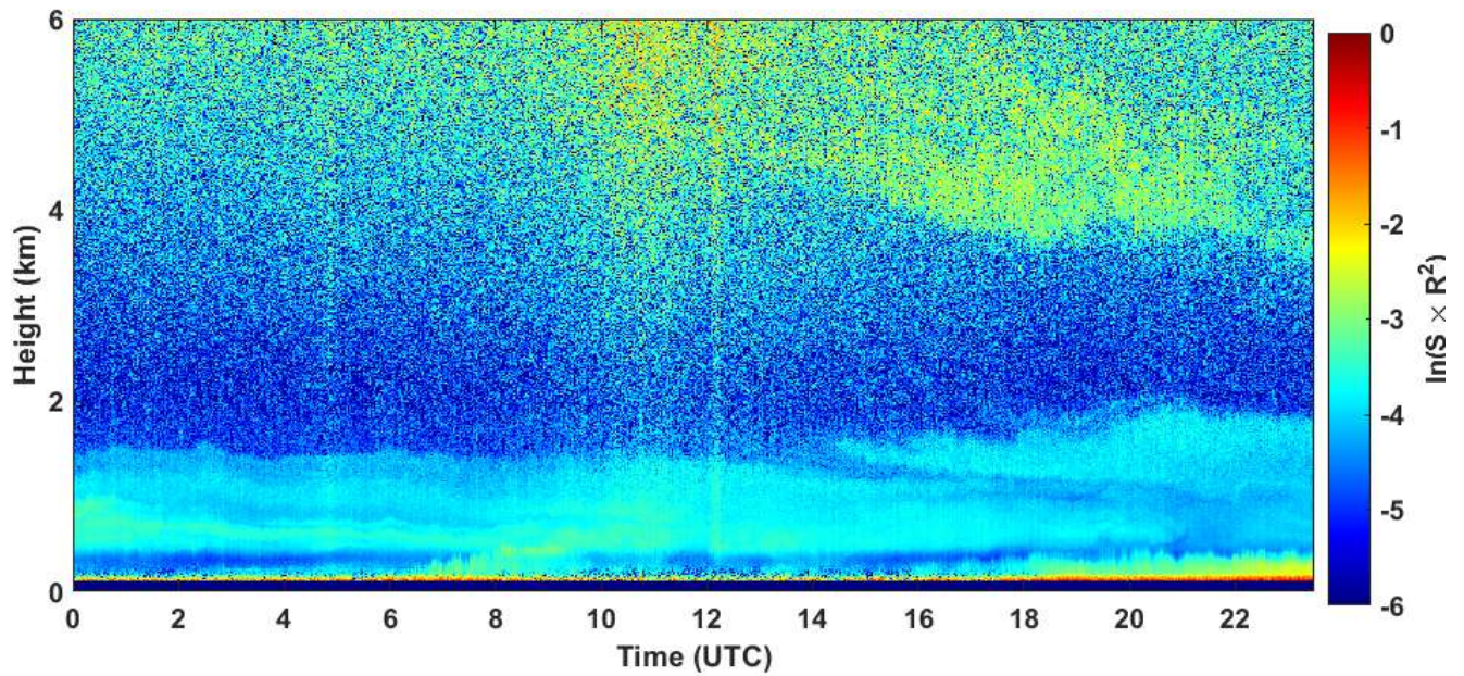
2020-05-10 RCS quick look CHM15k - ILVA LIDAR1 DIREZIONE
