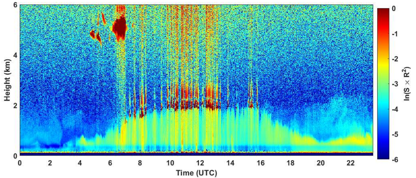
2020-05-26 RCS quick look CHM15k - ILVA LIDAR1 DIREZIONE
