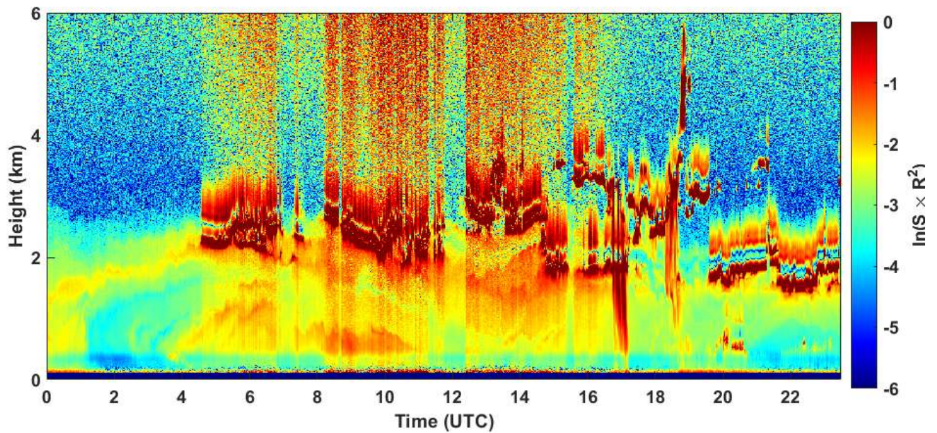
2020-05-20 RCS quick look CHM15k - ILVA LIDAR1 DIREZIONE
