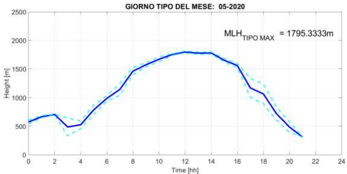
Fig. 2: Giorno tipo del parametro Mixing Layer Height nel mese di MAGGIO 2020, rappresentato mediante media oraria (linea blu continua) e deviazione standard (linee celesti tratteggiate).
