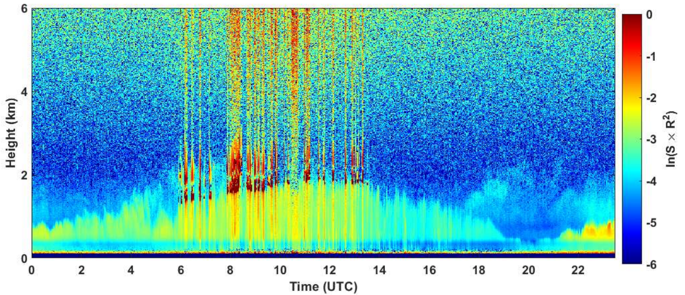
2020-05-28 RCS quick look CHM15k - ILVA LIDAR1 DIREZIONE
