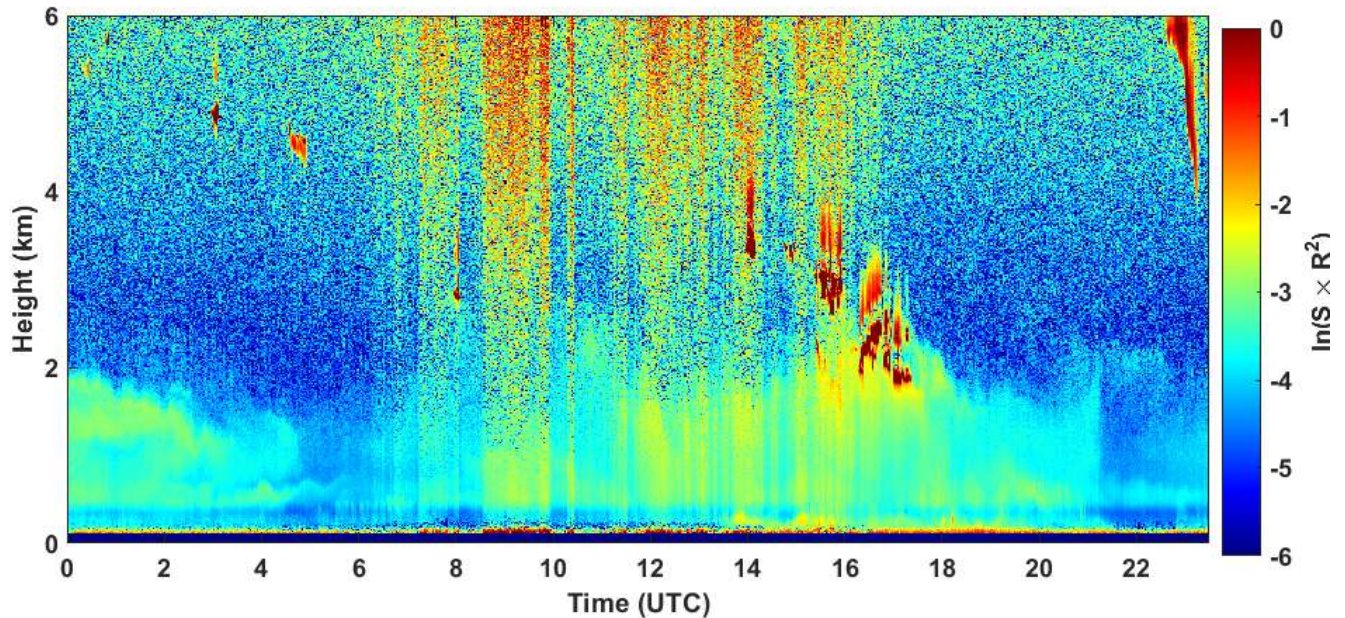
2020-05-02 RCS quick look CHM15k - ILVA LIDAR1 DIREZIONE
