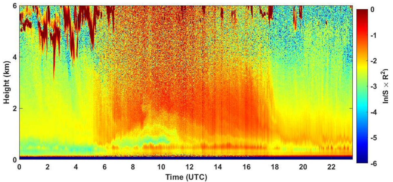
2020-05-14 RCS quick look CHM15k - ILVA LIDAR1 DIREZIONE
