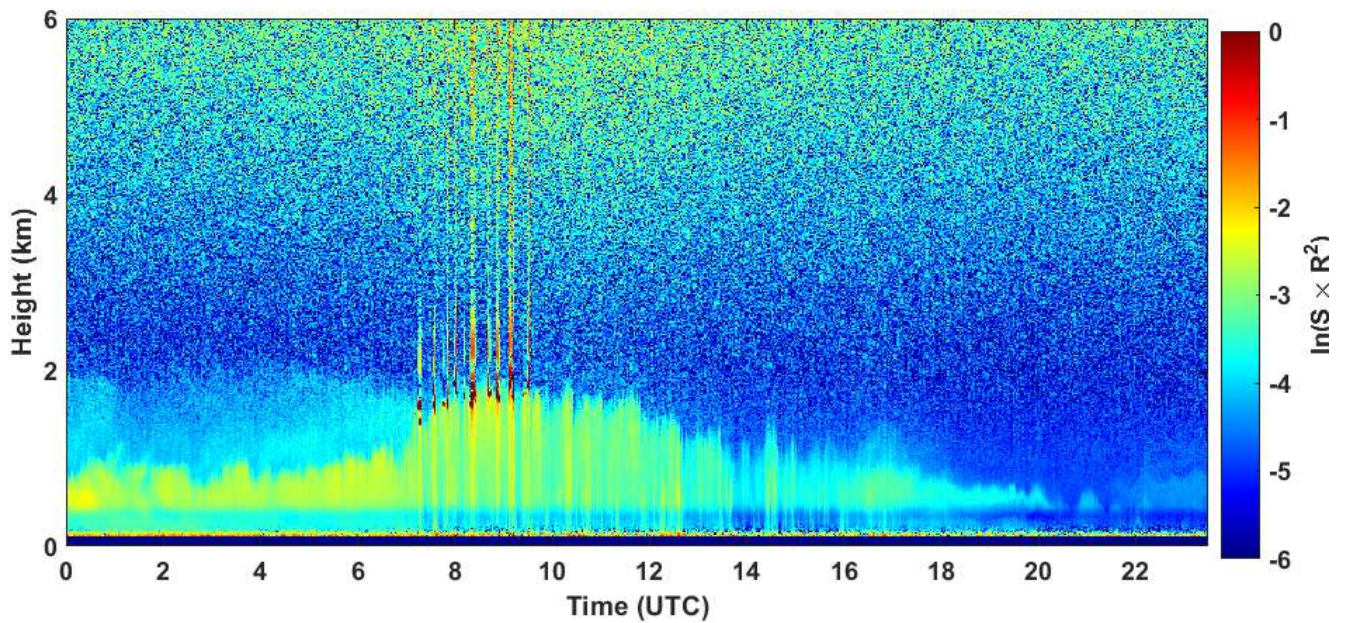
2020-05-04 RCS quick look CHM15k - ILVA LIDAR1 DIREZIONE
