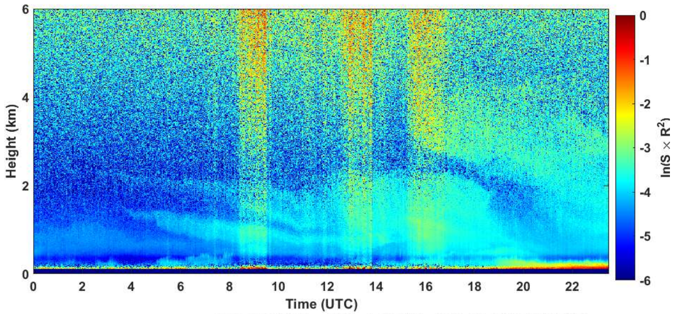
2020-05-06 RCS quick look CHM15k - ILVA LIDAR1 DIREZIONE
