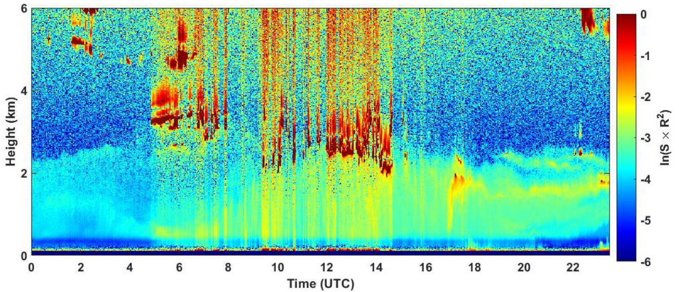
2020-05-30 RCS quick look CHM15k - ILVA LIDAR1 DIREZIONE
