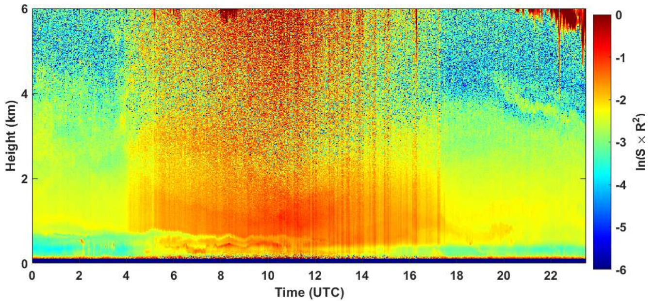
2020-05-18 RCS quick look CHM15k - ILVA LIDAR1 DIREZIONE
