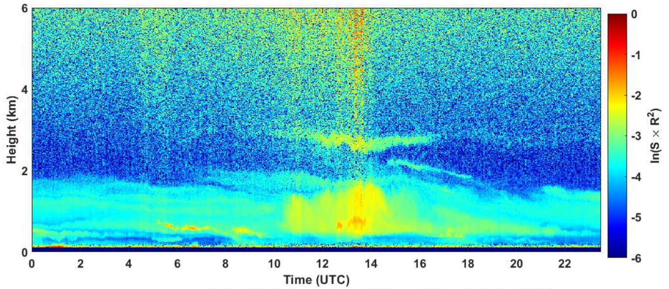
2020-04-18 RCS quick look CHM15k - ILVA LIDAR1 DIREZIONE
