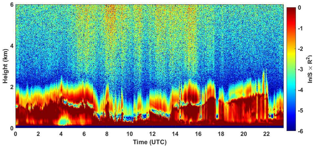
2020-04-22 RCS quick look CHM15k - ILVA LIDAR1 DIREZIONE
