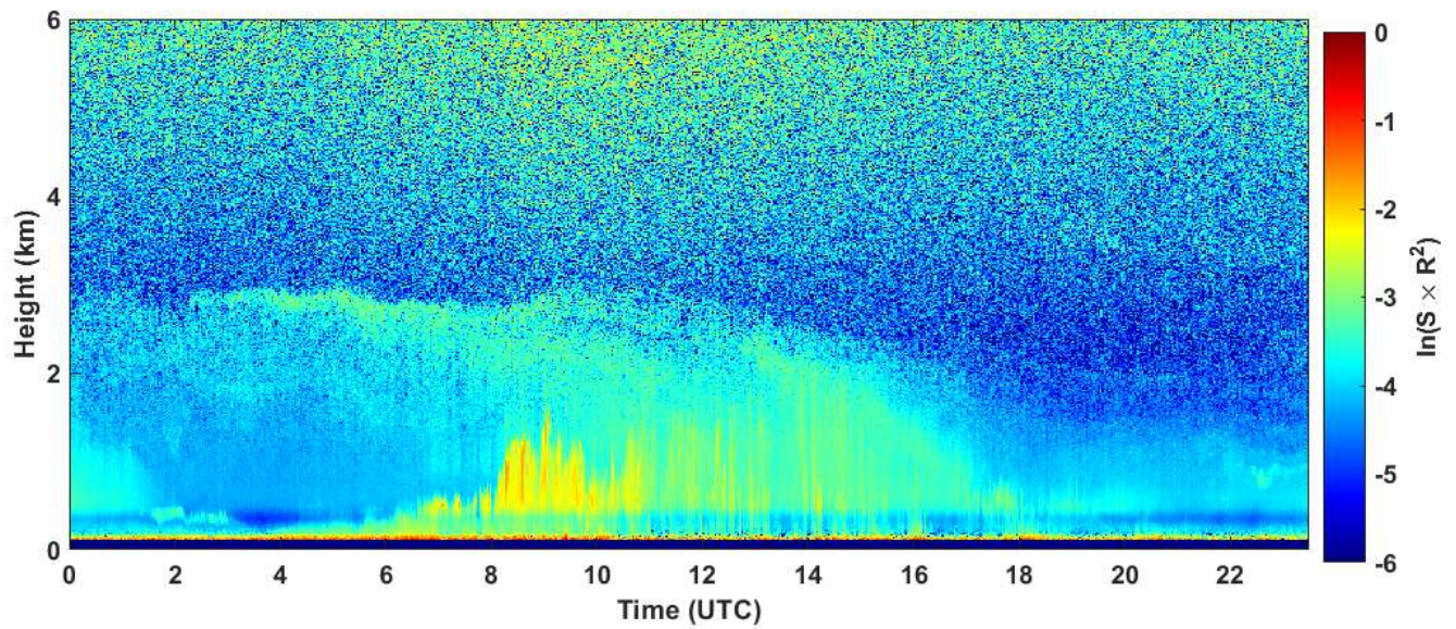
2020-04-08 RCS quick look CHM15k - ILVA LIDAR1 DIREZIONE
