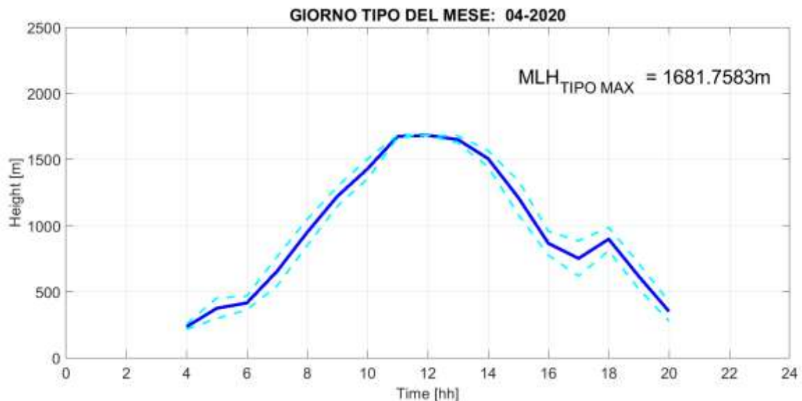
Fig. 2: Giorno tipo del parametro Mixing Layer Height nel mese di APRILE 2020, rappresentato mediante media oraria (linea blu continua) e deviazione standard (linee celesti tratteggiate).
