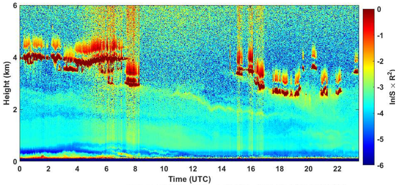
2020-04-28 RCS quick look CHM15k - ILVA LIDAR1 DIREZIONE
