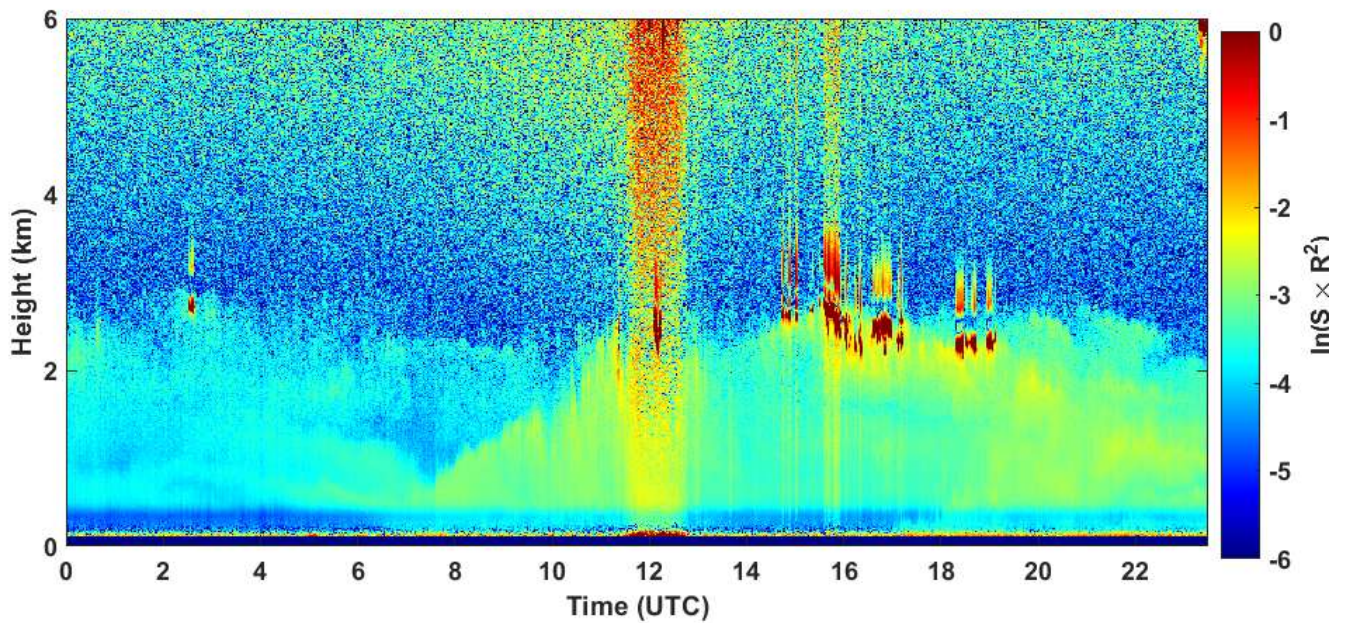
2020-04-30 RCS quick look CHM15k - ILVA LIDAR1 DIREZIONE
