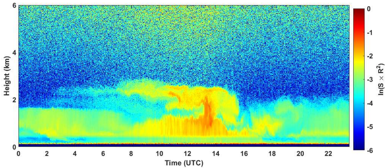
2020-04-10 RCS quick look CHM15k - ILVA LIDAR1 DIREZIONE
