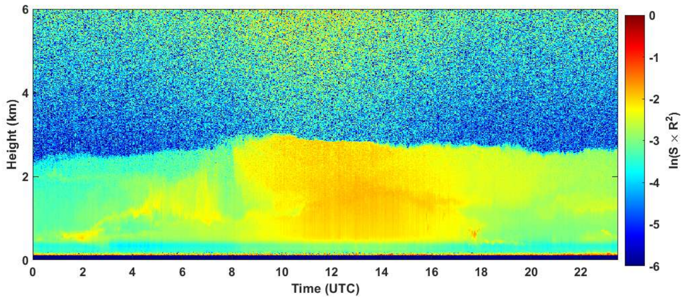
2020-04-12 RCS quick look CHM15k - ILVA LIDAR1 DIREZIONE
