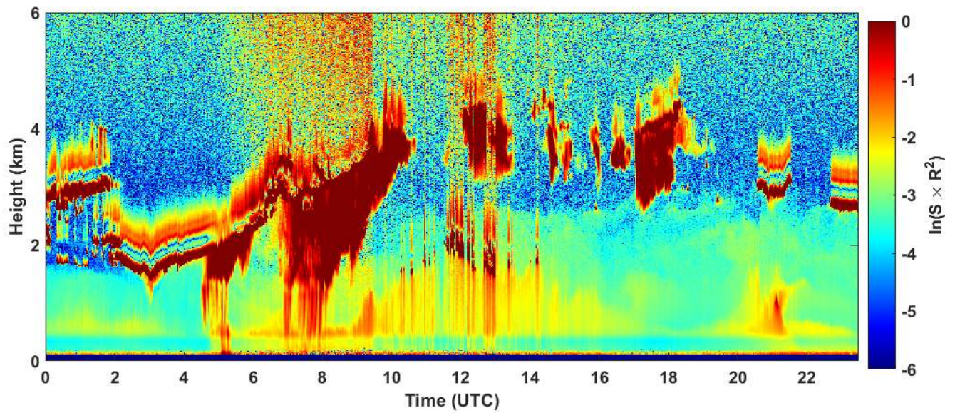
2020-04-04 RCS quick look CHM15k - ILVA LIDAR1 DIREZIONE
