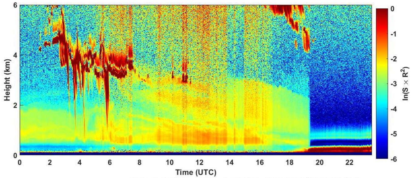
2020-04-20 RCS quick look CHM15k - ILVA LIDAR1 DIREZIONE
