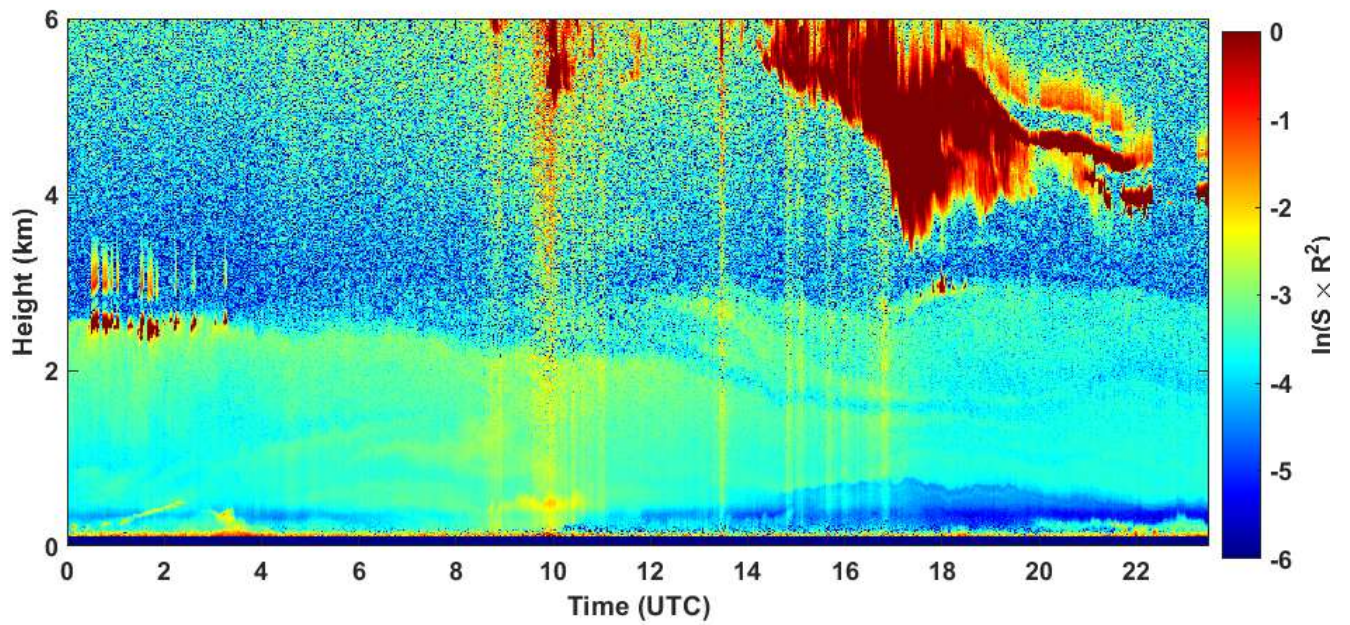
2020-04-26 RCS quick look CHM15k - ILVA LIDAR1 DIREZIONE
