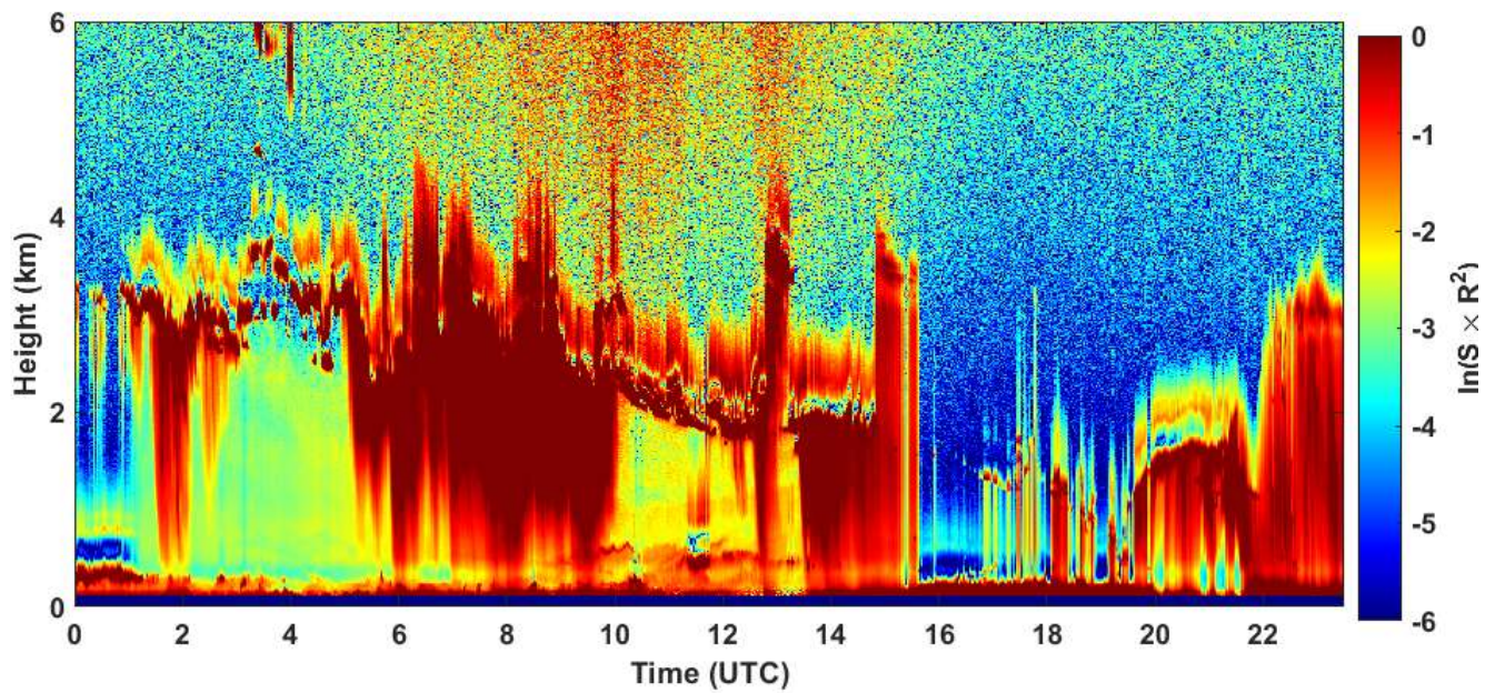
2020-04-20 RCS quick look CHM15k - ILVA LIDAR1 DIREZIONE
