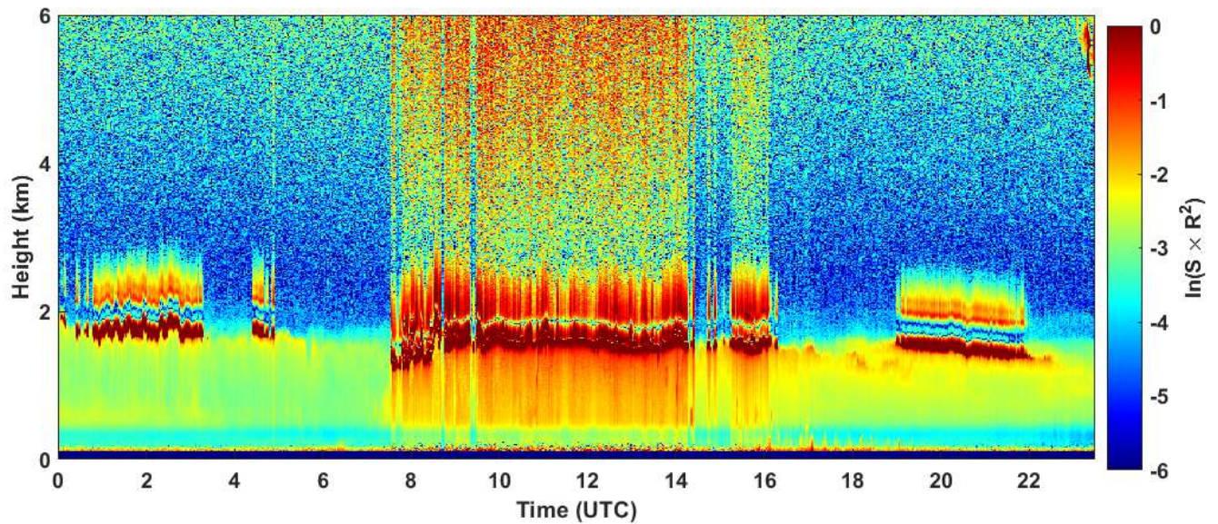
2020-04-02 RCS quick look CHM15k - ILVA LIDAR1 DIREZIONE
