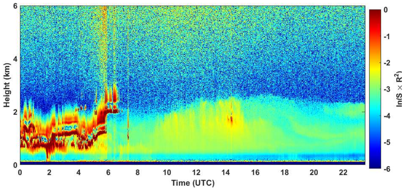
2020-04-24 RCS quick look CHM15k - ILVA LIDAR1 DIREZIONE
