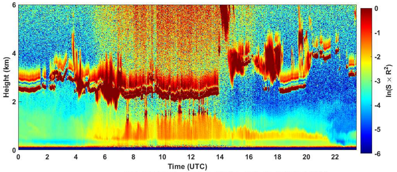
2020-04-06 RCS quick look CHM15k - ILVA LIDAR1 DIREZIONE
