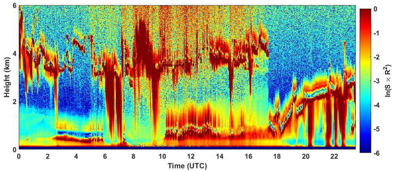
2020-04-14 RCS quick look CHM15k - ILVA LIDAR1 DIREZIONE
